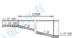
图 11.14 断开画法
