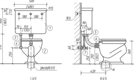
图 10-13 低水箱坐式大便器安装详图
