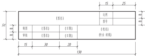
图 1.8 标题栏的格式
