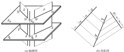
图 6.14 求两平面交线标高投影
