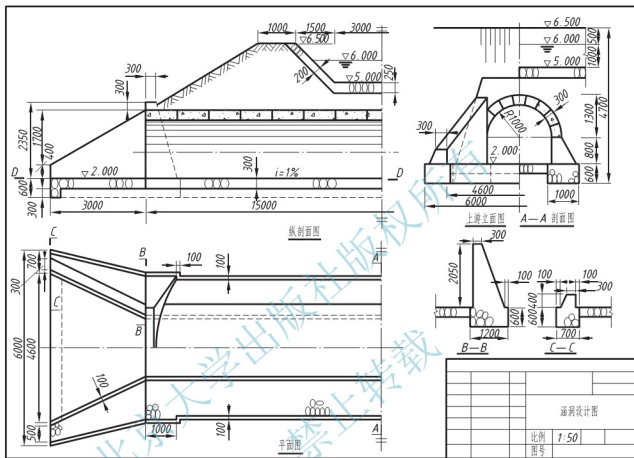
图 11.22 涵洞设计图
