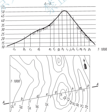
图 6.25 地形断面图
