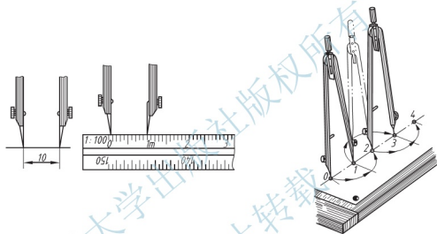
图 1.16 分规的使用
