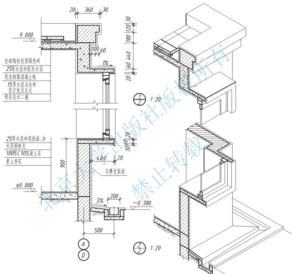
图 8.23 外墙身剖面详图
