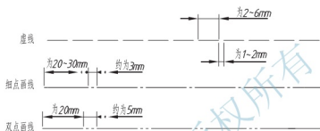
图 1.1 虚线、细点画线及双点画线的画法
