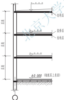
图 8.6 垂直方向上的定位轴线
