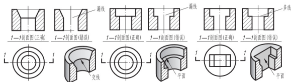
图 7.9 剖面图中漏线、多线的示例
