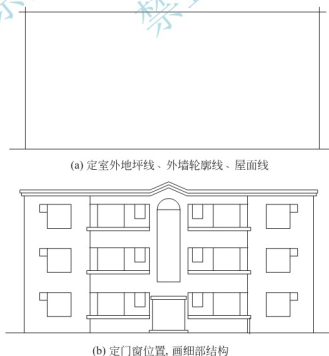
图 8.20 立面图的画图步骤
