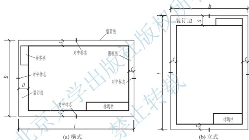
图 1.7 图纸幅面和图框格式
