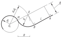
图 1.23 圆弧与直线和圆弧相连
