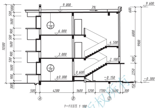
图 8.21 建筑剖面图
