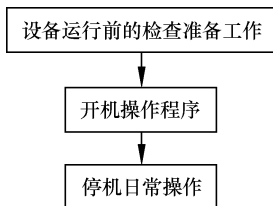
图 2-37 中央空调系统日常操作管理流程图
