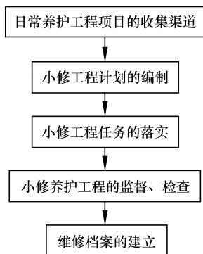
图 2-43 房屋日常维修养护流程图
