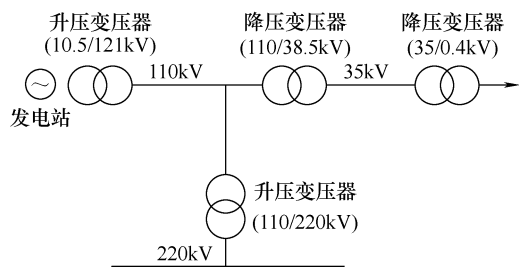
图 3-18 电力变压器用途举例
