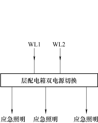
图 4-84 双电源到层配电箱 应急照明配电
