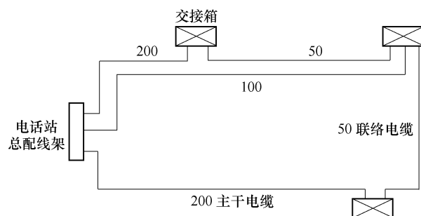
图 4-57 交接箱配线系统示意图
