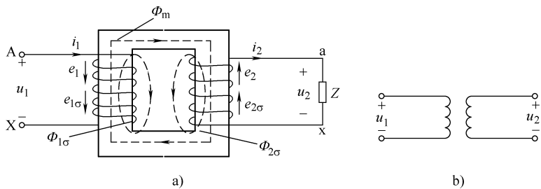
图 3-19 单相变压器
