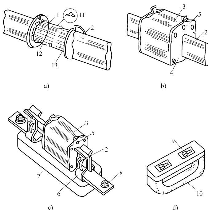
图 3-15 RT0 型有填料封闭管式熔断器
