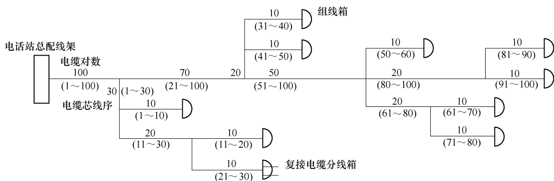
图 4-56 直接配线系统示意图
