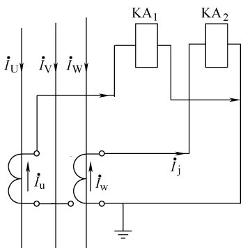
图 4-33 两相两继电器不完全星形联结
