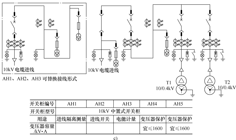
图 4-6 10kV 单电源进线，变压器一次侧采用单母线接线（续）
