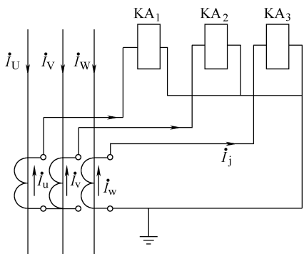
图 4-32 三相三继电器的完全星形联结
