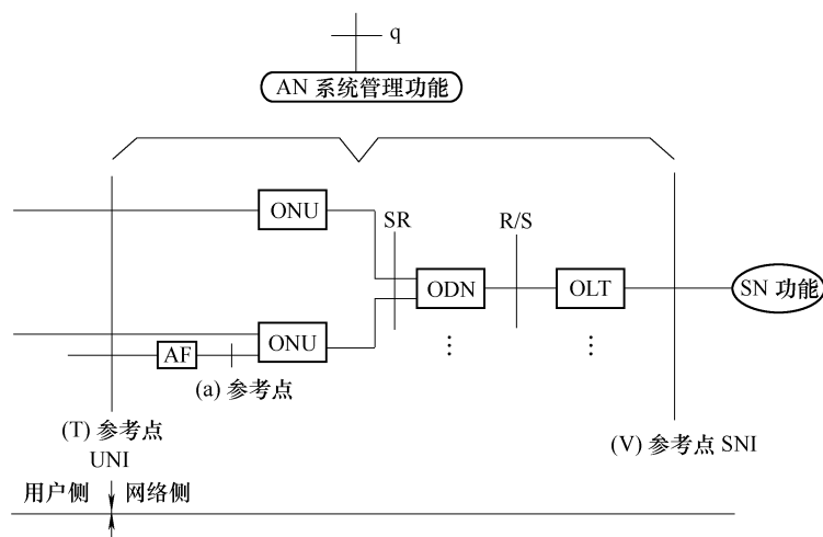
图 4-50 光纤接入网 (OAN) 的系统组成
