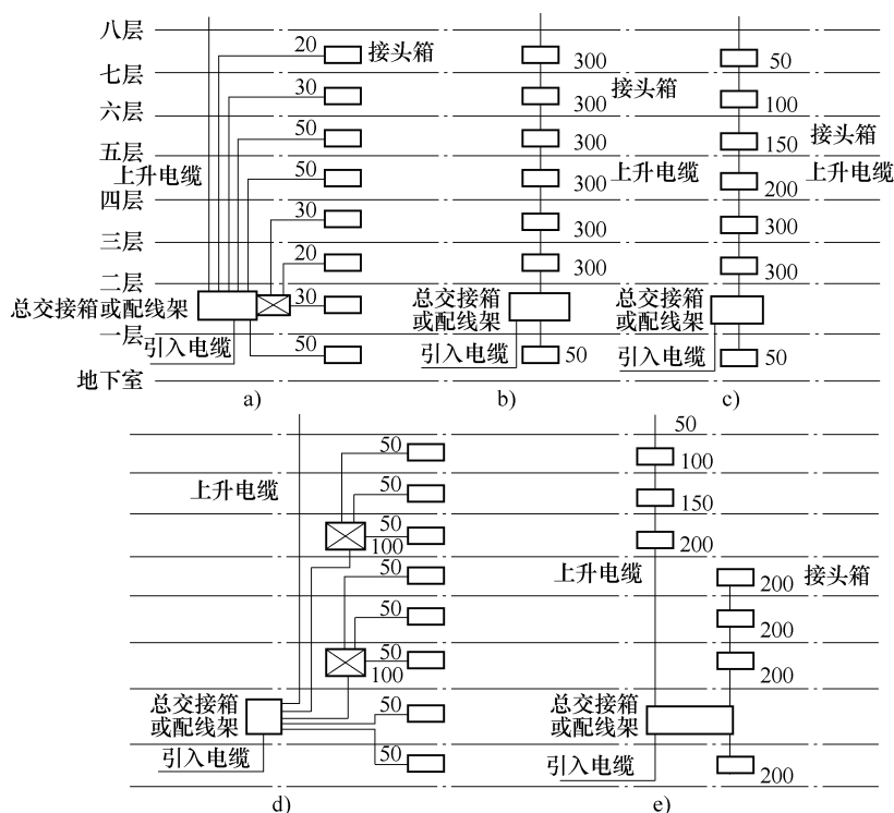
图 4-58 高层建筑电话电缆的配线方式
