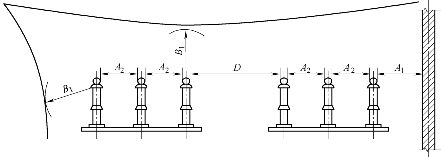
图 4-24 屋外 A_1 、 A_2 、 B_1 、 D 值校验
