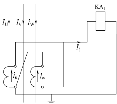
图 4-34 两相一继电器差动式联结
