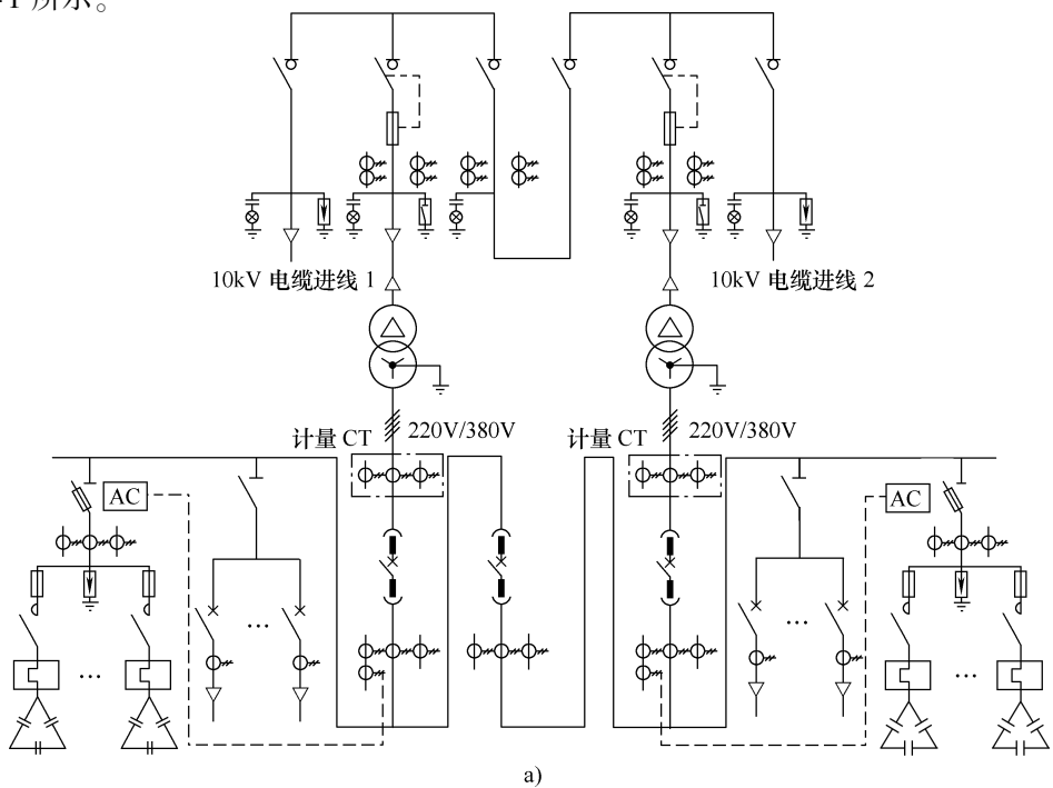
图 4-1 两路电源互为备用的预装式变电站的典型应用方案 a) 电气主接线
