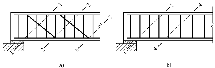
图 3-25 斜截面受剪承载力剪力设计值的计算截面
