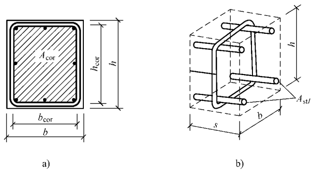
图 6-3 抗扭截面
