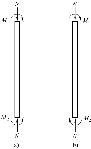
图 4-10 偏心受压构件的弯曲
