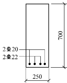
图 3-41 【例题 3-30】 配筋截面
