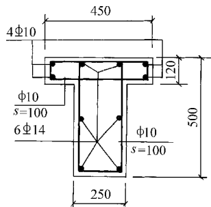
图 6-14 【例题 6-6】
