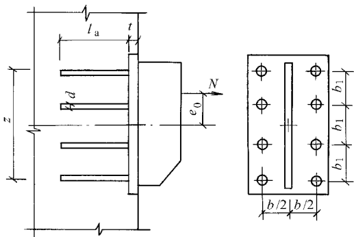
图 9-4 【例题 9-5】示图
