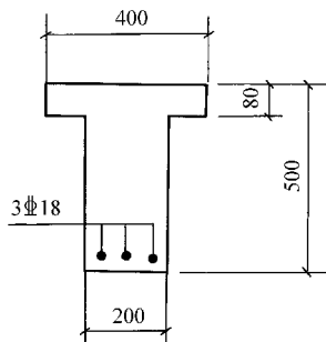
图 3-24 【例题 3-12】截面配筋图
