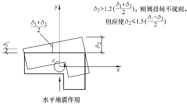
图 12-1 建筑结构平面的扭转不规则示例
