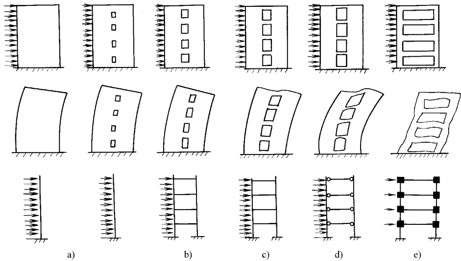
图 11-1 剪力墙的分类简图
