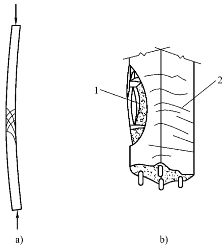
图 4-3 轴心受压长柱的破坏 a) 长柱加载图 b) 长柱破坏形态 1—混凝土被压碎 2—横向裂缝
