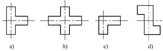
图 12-8 异形柱
