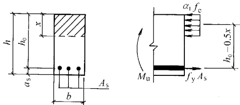
图 3-5 单筋矩形截面受弯构件 正截面受弯承载力计算
