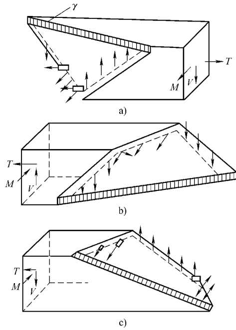
图 6-5 弯剪扭构件的破坏形态
