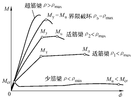
图 3-4 不同配筋率钢筋混凝土梁的 M-\phi 曲线
