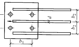
图 9-8 【例题 9-10】示图
