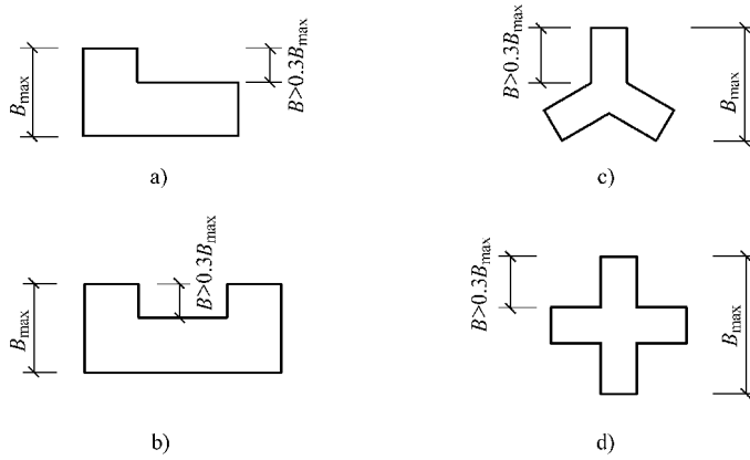
图 12-2 建筑结构平面的凸角或凹角不规则示例
