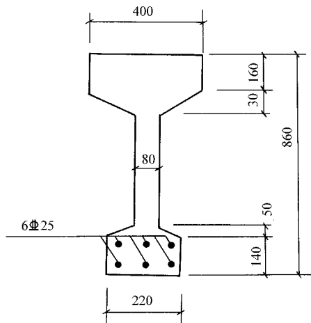
图 3-39 【例题 3-28】截面配筋
