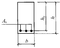
图 3-2 梁正截面示意
