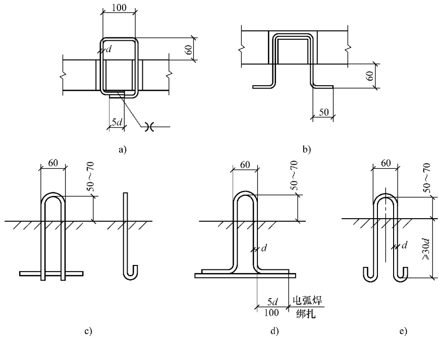
图 9-9 吊环形式
