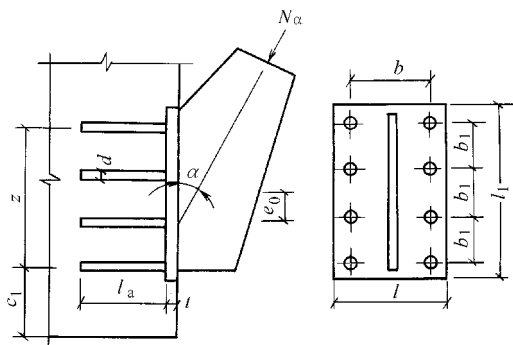
图 9-7 【例题 9-9】示图
