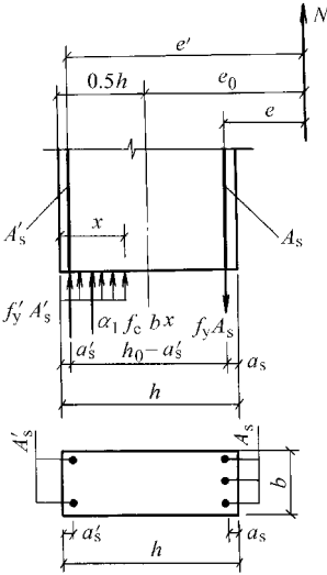
图 5-5 矩形截面大偏心受拉构件示意
