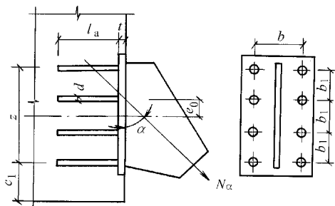
图 9-6 【例题 9-8】示意图
