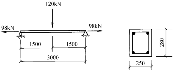
图 5-6 【例题 5-12】计算图
