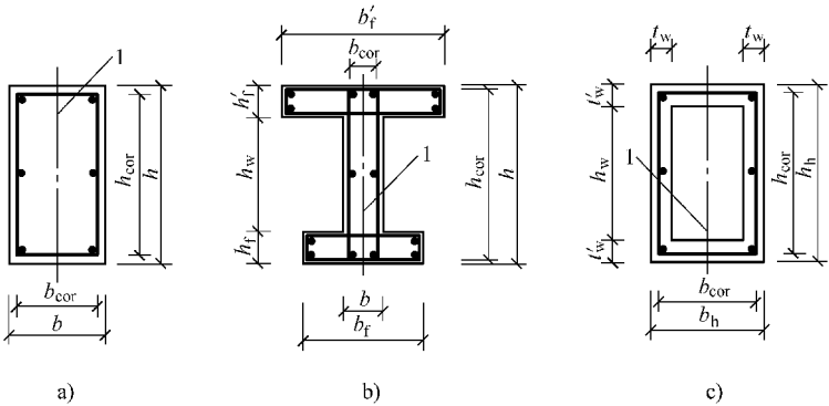
图 6-7 受扭构件截面 a) 矩形截面 b) T 形、I 形截面 c) 箱形截面 ( t_w \leq t_w' ) 1—弯矩、剪力作用平面
