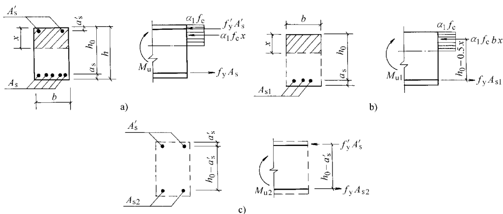
图 3-12 双筋矩形截面计算(一)
