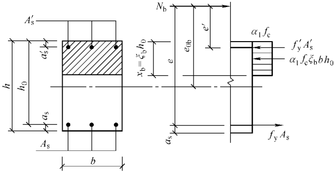
图 4-13 界限破坏的应力图
