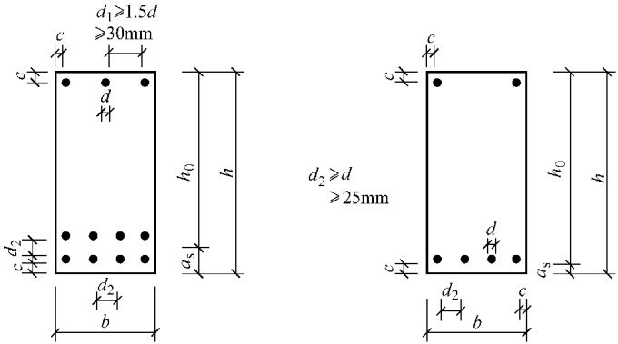
图 3-6 梁截面配筋构造
