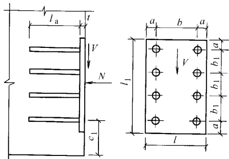
图 9-3 【例题 9-4】 示意图
