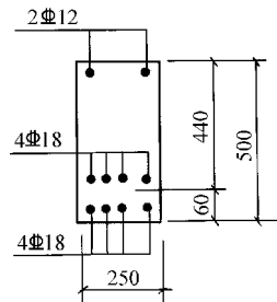
图 3-14 【例题 3-5】 截面配筋图
