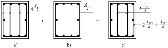
图 6-10 剪扭箍筋的叠加 a) 受剪箍筋 b) 受扭箍筋 c) 箍筋叠加
