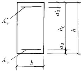
图 4-18 矩形截面配筋简图
