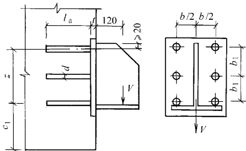
图 9-5 【例题 9-7】示图
