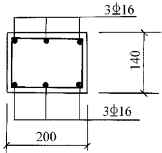
图 5-2 【例题 5-2】 截面配筋
