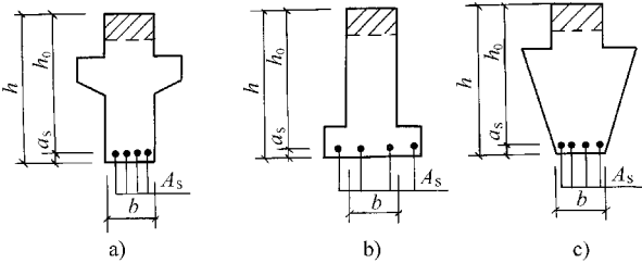
图 3-7 受压区为矩形的三种图形 a) 十字形 b) 倒 T 形 c) 花篮形
