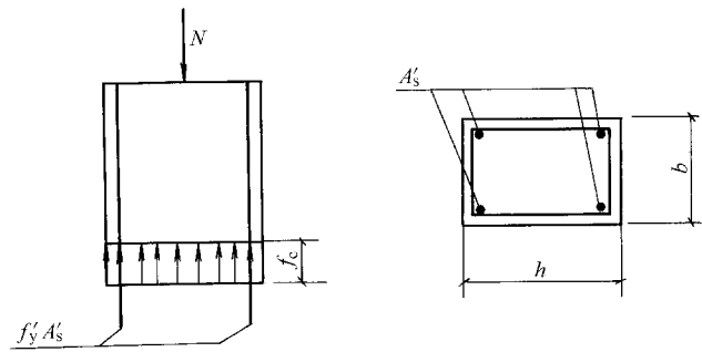
图 4-4 配置箍筋的钢筋混凝土轴心受压构件截面
