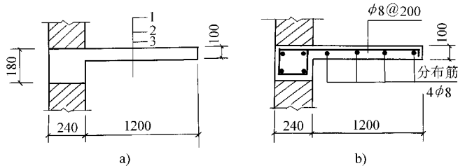
图 3-11 【例题 3-4】剖面图
