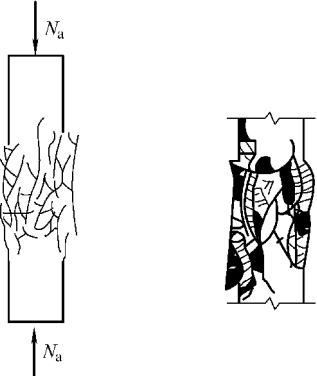
图 4-2 轴心受压短柱的破坏
