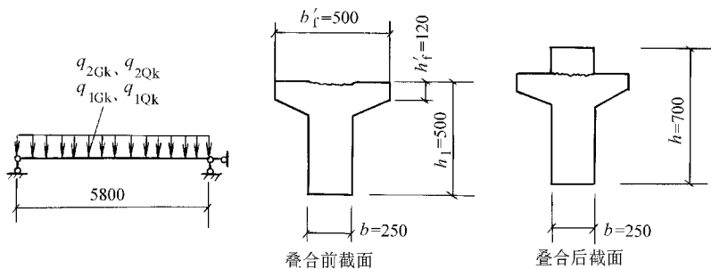
图 10-3 【例题 10-2】叠合构件计算简图
