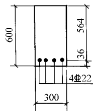
图 3-8 【例题 3-1】
