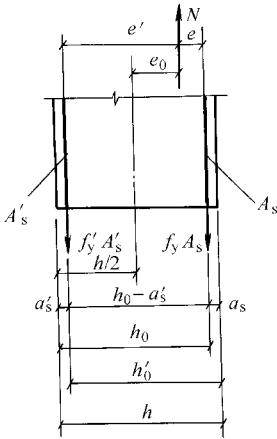
图 5-4 矩形截面小偏心受拉构件示意
