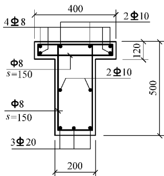
图 6-15 【例题 6-7】截面配筋
