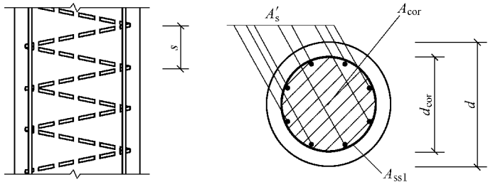
图 4-6 配置螺旋式间接钢筋的钢筋混凝土轴心受压构件
