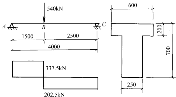
图 3-26 【例题 3-20】计算简图
