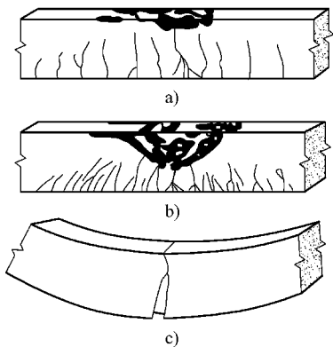
图 3-3 不同配筋率钢筋混凝土梁正截面破坏形态
