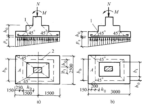
图 7-9 【例题 7-4】阶形基础
