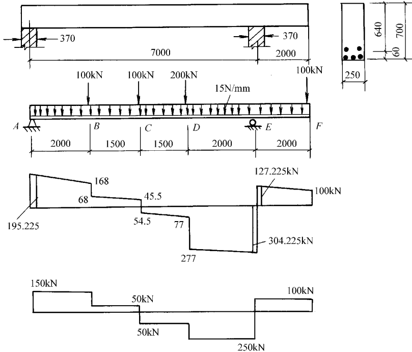
图 3-27 【例题 3-21】计算简图
