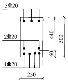
图 3-15 【例题 3-6】 截面配筋图
