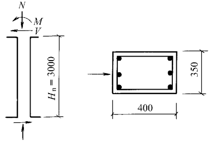
图 4-16 【例题 4-29】示意图
