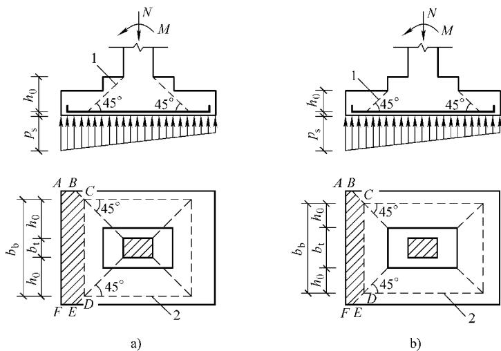
图 7-5 计算阶形基础的受冲切承载力截面位置
