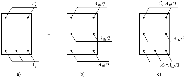
图 6-9 弯扭纵筋的叠加 a) 受弯纵筋 b) 受扭纵筋 c) 纵筋叠加
