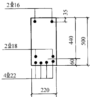
图 3-23 【例题 3-11】截面配筋图
