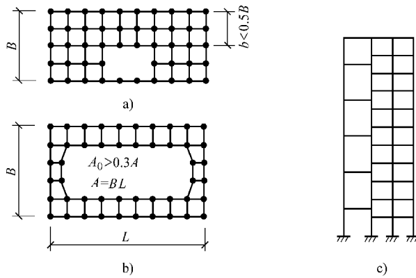
图 12-3 建筑结构平面的局部不连续示例(大开洞及错层)
