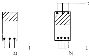
图 3-1 单筋截面与双筋截面 a) 单筋截面 b) 双筋截面 1—受拉钢筋 2—受压钢筋
