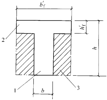
图 3-17 T 形截面
