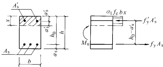
图 3-13 双筋矩形截面计算(二)
