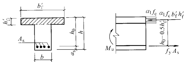
图 3-20 中和轴通过翼缘下边缘的 T 形截面计算
