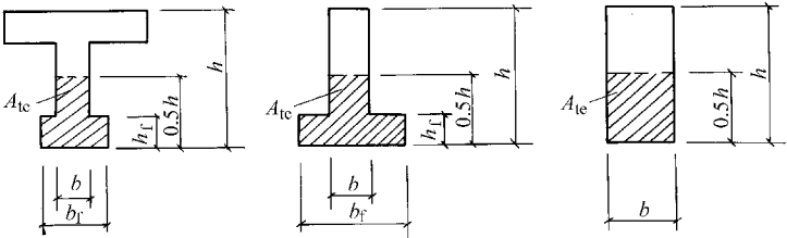
图 3-36 A_{te} 计算图
