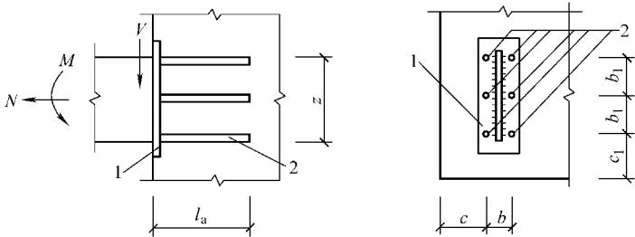
图 9-1 由锚板和直锚筋组成的预埋件 1—锚板 2—直锚筋
