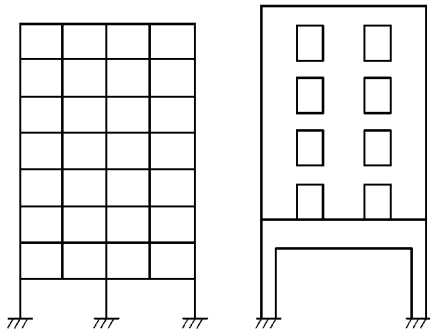
图 12-5 竖向抗侧力构件不连续示例
