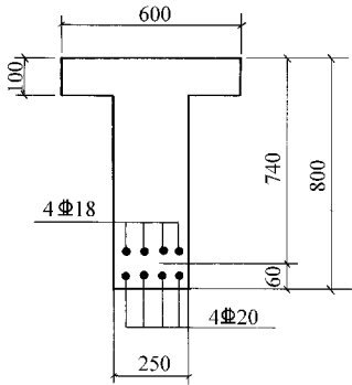
图 3-21 【例题 3-9】截面配筋图
