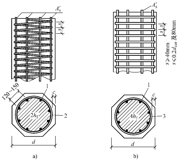
图 4-5 螺旋式和焊接环式箍筋柱
