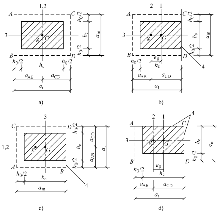
图 7-4 矩形柱及受冲切承载力计算的几何参数
