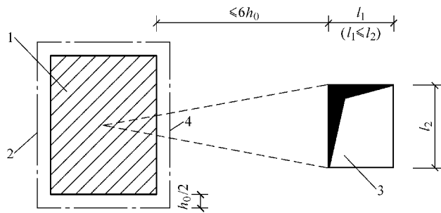
图 7-2 邻近孔洞时的计算截面周长 1—局部荷载或集中反力作用面 2—计算截面周长 3—孔洞 4—应扣除的长度
