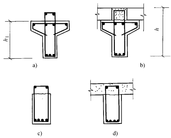
图 10-1 叠合构件
