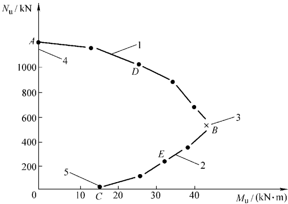
图 4-9 N_u-M_u 相关曲线
