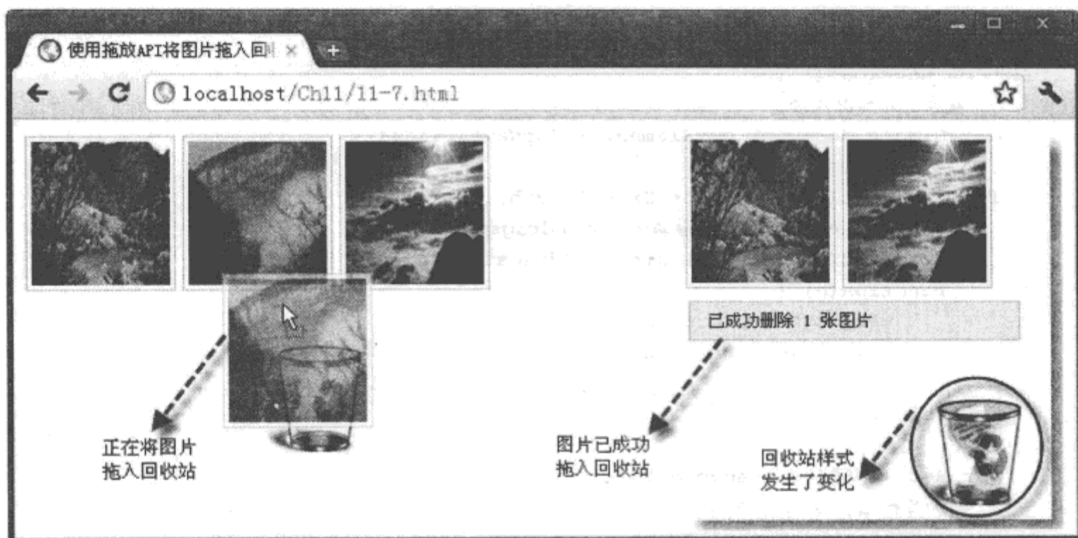
图 11-7 使用拖放 API 将图片拖入回收站
