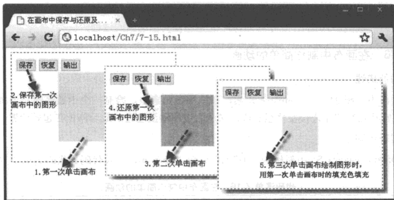
图 7-18 使用 save 与 restore 方法保存、恢复已绘制的图形
