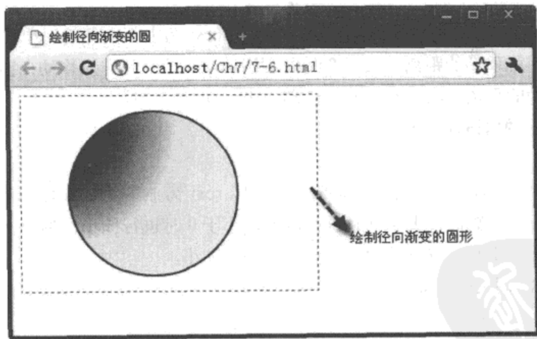
图 7-8 使用 <canvas> 元素绘制径向渐变的圆形
