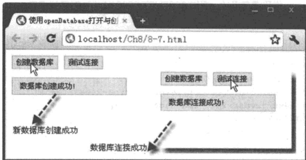
图 8-7 使用 openDatabase 打开与创建数据库
