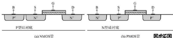
图 1.4 MOS 管的剖面结构
