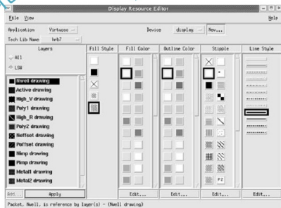
图 6.7 设置层的颜色和图案
