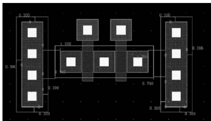
图 8.13 衬底接触 1
