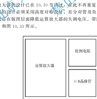
图 10.32 带隙基准源电路布局图
