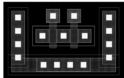
图 8.15 连接衬底接触
