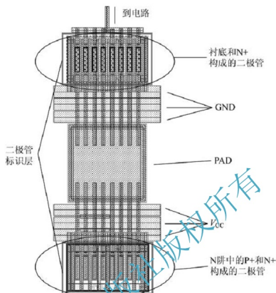
图 10.23 二极管型 ESD 保护电路版图
