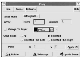
图 6.28 复制对话框
