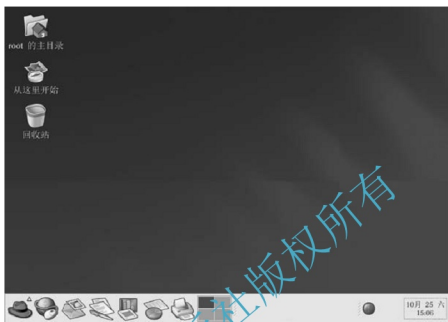
图 2.24 GNOME 界面
