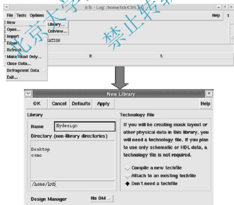
图 3.4 建立设计库
