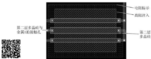
【图 6.48 彩图】
