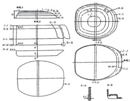
图4-63 三视图
