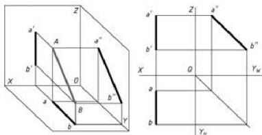
图 3.26 侧平线的投影
