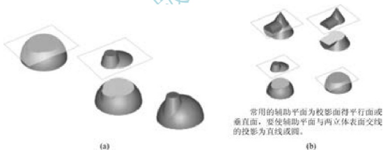
图 4.61 用水平面作为辅助平面求共有点
