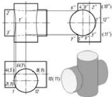
图 4.57 表面取点法求相贯线
