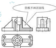
图 7.22 将主视图画成半剖视图
