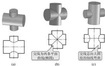
图 4.55 两圆柱的引贯线
