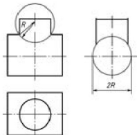
图 4.64 正交圆柱相贯线的近似画法
