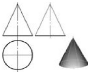
图 4.22 圆锥的投影
