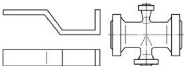
图 2.36 过渡线由粗实线改为细实线
