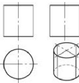
图 4.17 圆柱的投影特点
