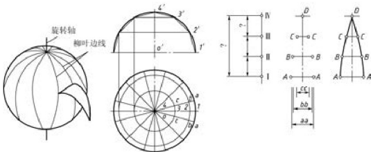
图 6.6 球面的展开图 (柳叶法)
