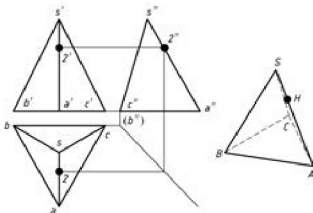
图 4.14 三棱锥棱线上取点
