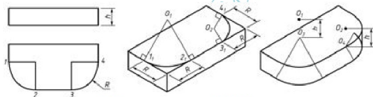
图 5.8 圆角的正等轴测图
