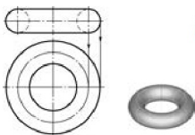
图 4.29 圆环的投影
