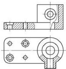
图 7.27 局部剖视图
