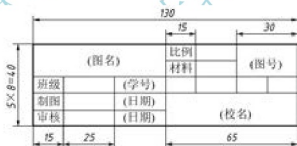
图 2.4 学校用简易标题栏
