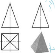
图 4.11 四棱锥三视图
