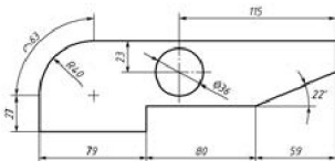
图 8.100 角度标注图形
