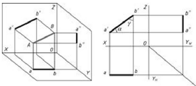
图 3.25 正平线的投影
