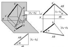
图 3.31 求直线的实长及对水平投影面的夹角
