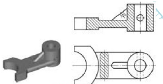
图 7.56 对称的重合断面图画法
