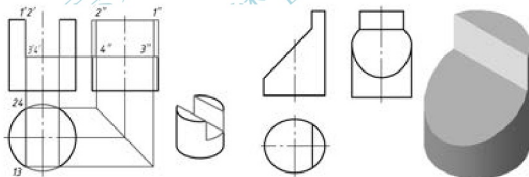
图 4.46 圆柱截交线
