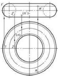
图 4.32 圆环表面取点的投影
