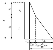
图 7.3 成层地基土中自重应力分布
