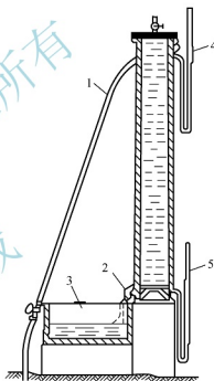
图 1.55 达西试验装置
