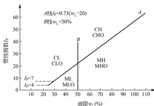
图 6.13 塑性图
