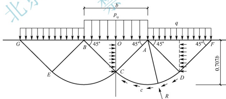
图 8.55 斯肯普顿滑动面
