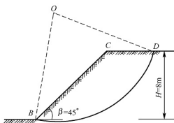
图 8.48 均质黏性土简单土坡
