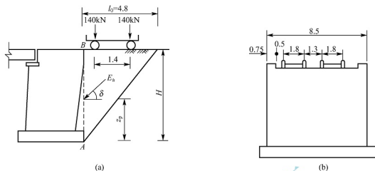
图 8.38 某高速公路桥梁桥台布置(尺寸单位: m)
