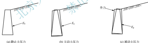
图 8.17 土压力分类
