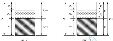
图 6.18 三相草图
