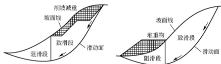
图 2.16 减载与反压
