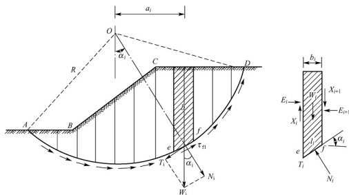
图 8.49 用条分法计算土坡稳定性
