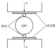
图 1.11 劈裂法试验装置
