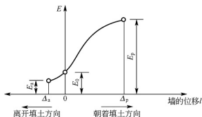
图 8.18 土压力与挡土结构位移的关系
