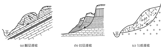
图 4.11 滑坡的分类
