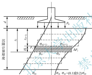
图 7.15 分层总和法计算地基最终沉降量
