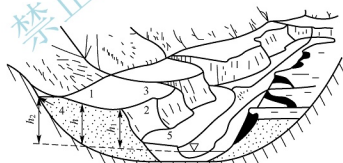
图 1.43 河流阶地的形态要素
