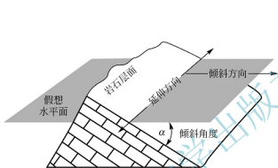
图 1.13 岩层产状要素
