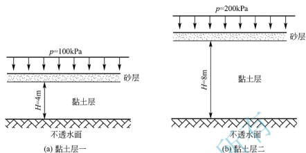
图 7.26 第 6 题图
