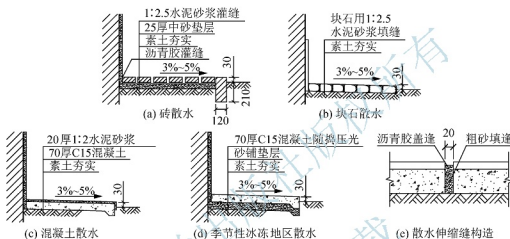
图 3.25 散水构造
