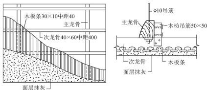
图 4.41 板条抹灰顶棚构造
