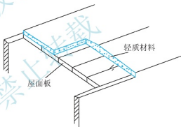
图 6.11 材料找坡
