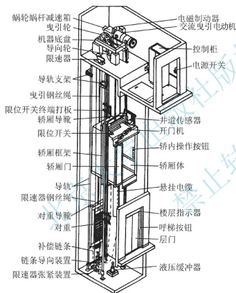
图 5.44 交流调速乘客电梯的部件组装示意
