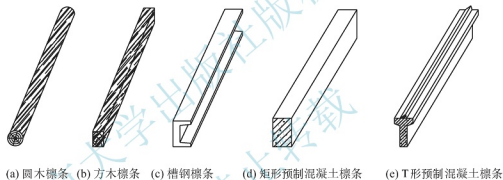
图 6.33 檩条断面形式
