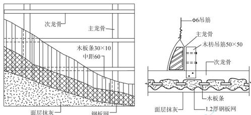
图 4.42 板条钢板网抹灰顶棚构造
