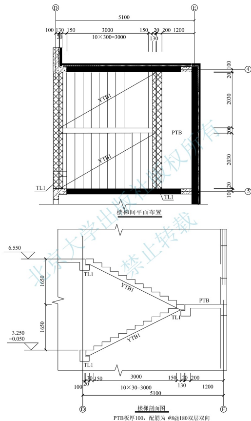
图 10.13 装配式楼梯平面图、剖面图及节点详图
