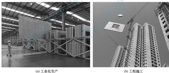
图 10.4 远大住工装配式建筑工业化生产与工程施工
