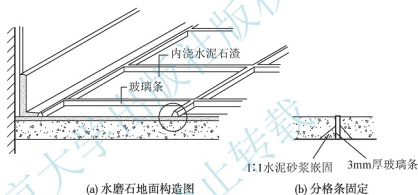
图 4.26 水磨石地面
