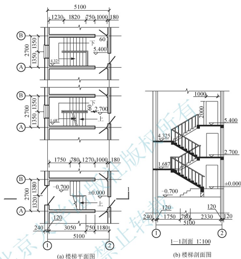
图 9.2 楼梯平面及剖面图
