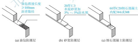
图 3.31 墙身水平防潮层
