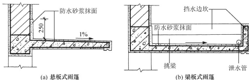
图 4.48 雨篷构造 1
