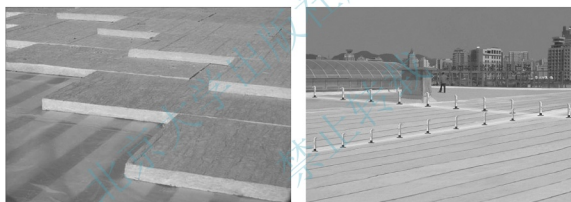
图 6.26 板状材料保温层
