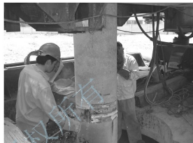
图 2.28 静力压桩施工
