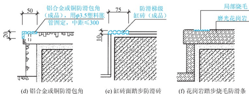
图 5.27 踏步面层防滑构造 (续)
