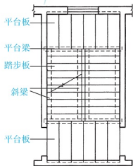
图 5.17 梁承式楼梯平面
