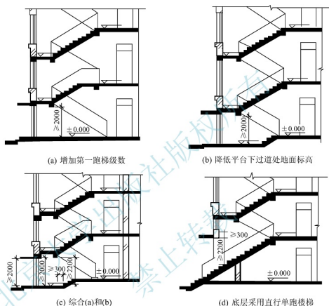
图 5.10 楼梯间入口处净空尺寸调整的示意图
