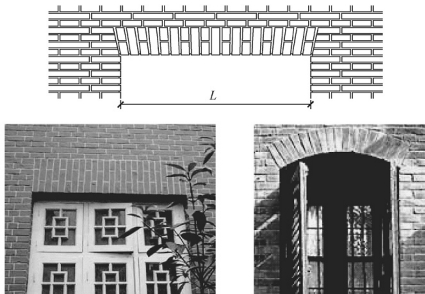
图 3.33 砖拱过梁构造
