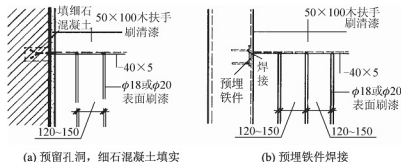
图 5.35 顶层栏杆扶手入墙做法
