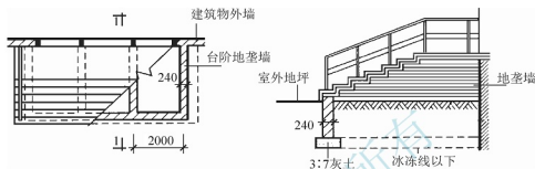
(a) 架空台阶平面图
