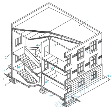
1—基础；2—外墙；3—内横墙；4—内纵墙；5—楼板；6—屋顶；7—地坪； 8—门；9—窗；10—楼梯；11—台阶；12—雨篷；13—散水
