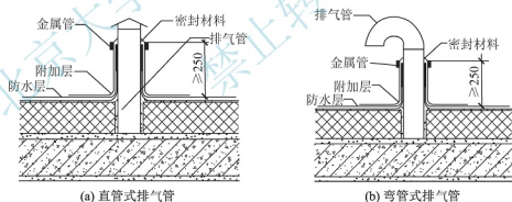
图 6.27 屋面排气出口构造
