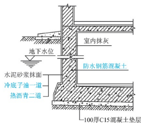
图 2.40 防水混凝土自防水构造
