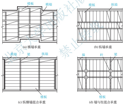
图 3.10 墙体的承重方案
