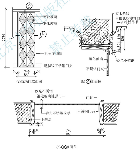
图 7.13 玻璃门构造
