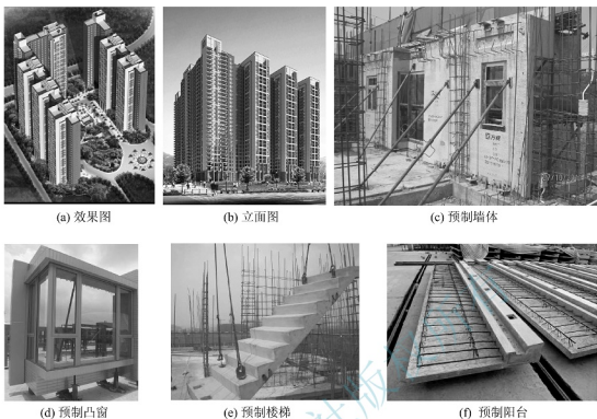
图 10.3 南沙府前一号装配式建筑
