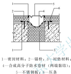
图 8.7 墙体变形缝防水构造
