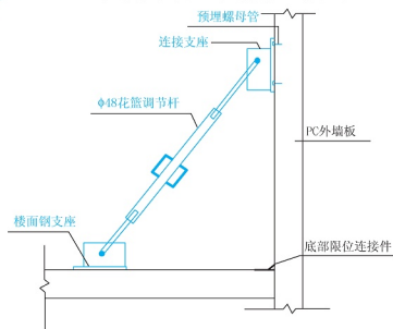
(a) PC 外墙斜撑示意图
