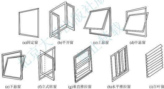
图 7.14 窗按开启方式分类
