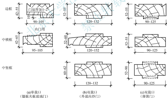
图 7.7 木门框的断面形式与尺寸
