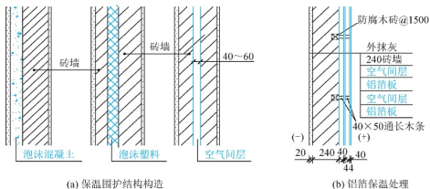
图 3.11 保温复合墙构造图
