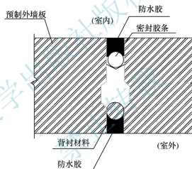
(b) 竖向构造防水缝
