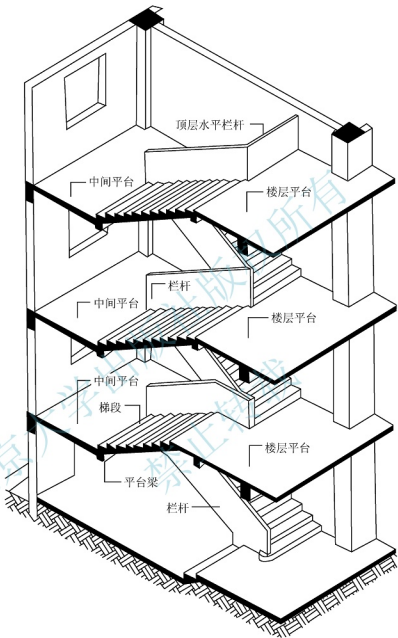
图 5.2 楼梯的构造组成
