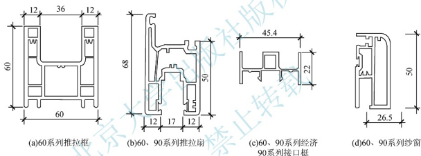
图 7.21 塑钢窗专用型材示意
