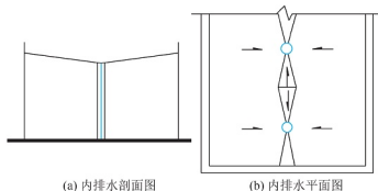
图 6.16 内排水方案
