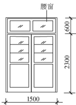
图 7.4 门窗高度和宽度示意
