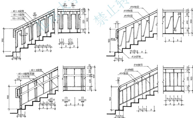
图 9.4 楼梯栏杆参考构造
