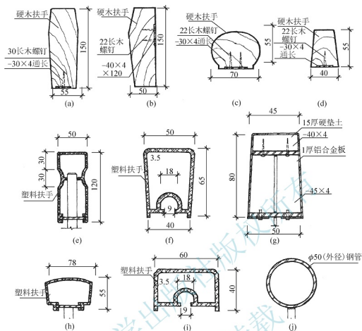
图 9.7 楼梯扶手参考构造
