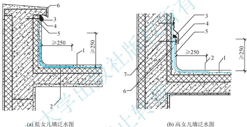
(a) 低女儿墙泛水图
