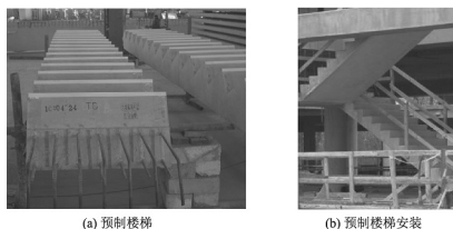
图 5.24 预制板式实心楼梯
