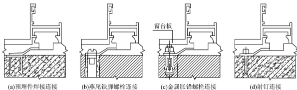
图 7.19 铝合金窗的安装构造
