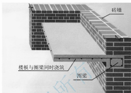
(b) 圈梁与楼板同时浇筑
