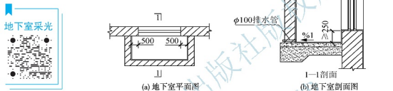
图 2.32 地下室采光井的构造
