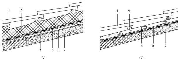
1—块瓦；2—挂瓦条；3—顺水条；4—防水垫层；5—持钉层；6—保温隔热层； 7—屋面板；8—防水垫层或隔热防水垫层；9—带挂瓦条的保温板；10—找平层
