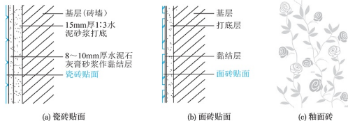
图 3.53 瓷砖、面砖贴面
