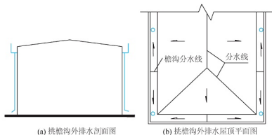
图 6.13 挑檐沟外排水方案
