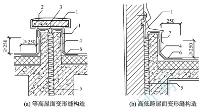
1—卷材封盖; 2—混凝土盖板; 3—衬垫材料; 4—附加层; 5—不燃保温材料; 6—防水层; 7—金属盖板
