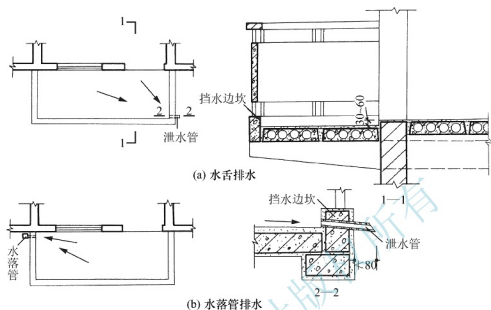
图 4.47 阳台的外排水构造
