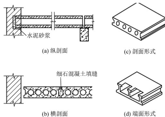
图 4.18 空心板
