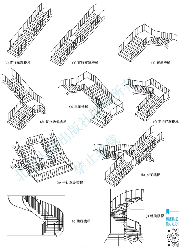
图 5.4 楼梯按平面形式分类
