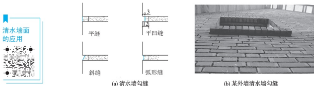
图 3.60 清水墙的勾缝形式
