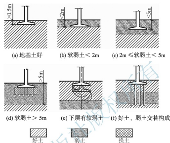
图 2.12 地质构造与基础埋深的关系
