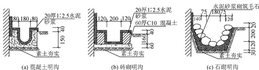
图 3.28 明沟的构造
