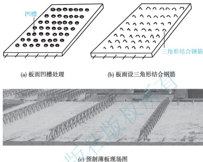
图 4.25 预制薄板表面的处理
