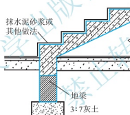
图 5.36 首层第一踏步下的基础
