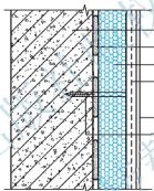
图 3.14 粘贴保温板薄抹灰外保温系统
