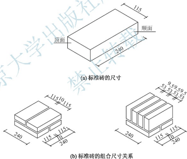
图 3.21 标准砖的尺寸关系
