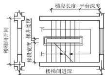
图 5.5 楼梯各部位尺寸定义
