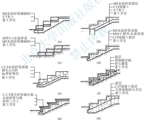
图 5.38 台阶的构造
