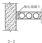
(c) 梁板式剖面图(2)
