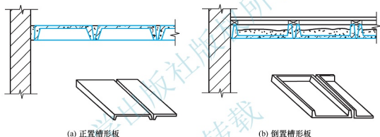
图 4.17 槽形板
