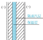
图 3.12 隔蒸汽构造
