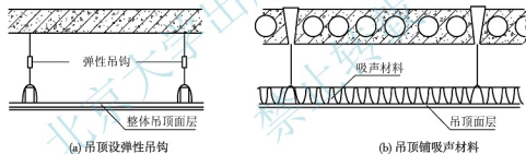
图 4.7 楼板下设吊顶
