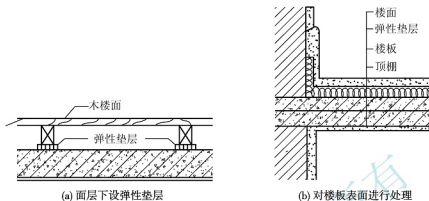
图 4.6 浮筑式楼板
