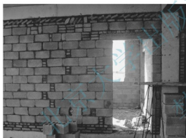
(b) 砌块隔墙施工图
