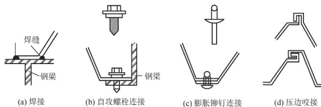
图 4.15 钢衬板之间及钢衬板与钢梁之间的连接方式
