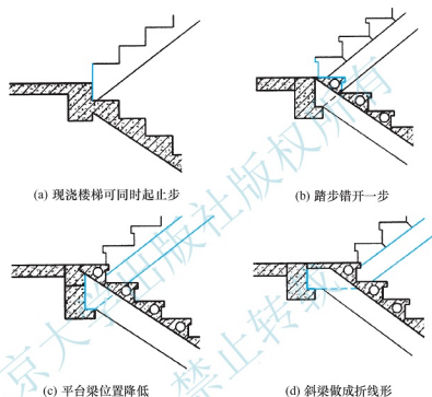
图 5.20 楼梯起止步的处理
