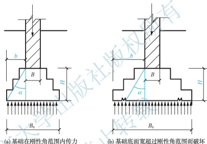
图 2.15 刚性基础
