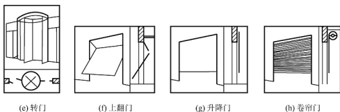
图 7.3 门按开启方式分类 (续)
