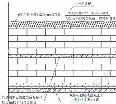
(a) 砌块隔墙立面图
