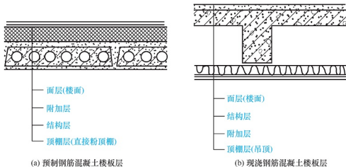
图 4.1 楼板层构造组成
