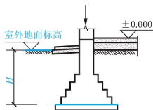
图 2.11 基础埋深
