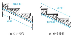
图 5.16 明步楼梯和暗步楼梯
