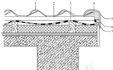
1—瓦；2—挂瓦条；3—防水垫层；4—水泥砂浆封边； 5—檐口封边瓦；6—镀锌钢钉；7—木条
