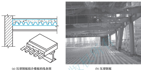
图 4.5 压型钢板组合楼板
