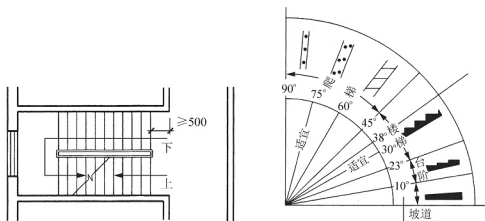
图 5.7 敞开楼梯间楼层平台的宽度
