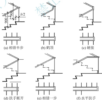
图 5.34 楼梯转弯处扶手高差的处理
