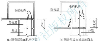
图 5.48 机房隔音层
