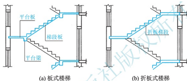
图 5.14 板式楼梯
