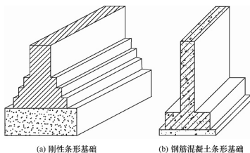
图 2.19 墙下条形基础
