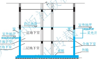
图 2.31 地下室组成构造
