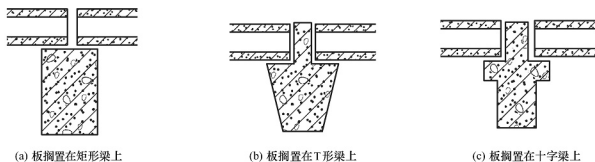
图 4.20 板在梁上的搁置方式
