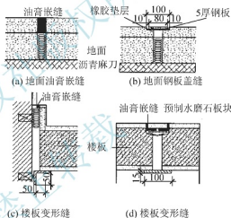
图 8.8 楼地板伸缩缝构造
