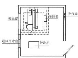
图 5.47 电梯机房平面示例
