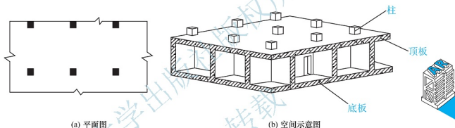
图 2.23 箱形基础
