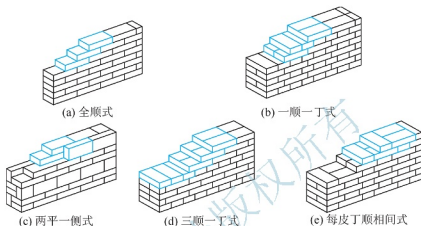
图 3.22 砖墙砌筑方式
