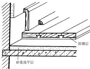
(a) 粘贴式木地板构造图
