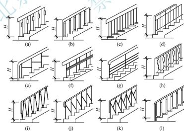
图 5.28 常见栏杆形式
