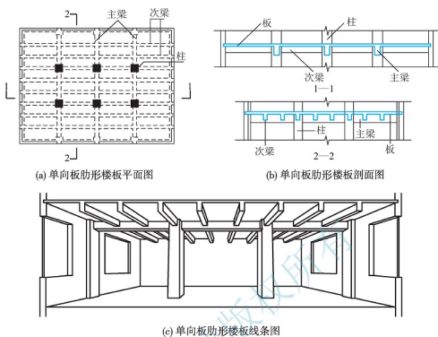
图 4-10 单向板肋形楼板
