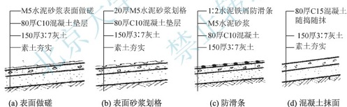
图 5.41 坡道构造示例
