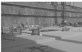
(a) 防水卷材铺贴完成后
