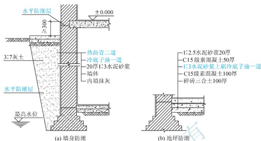
图 2.33 地下室防潮构造
