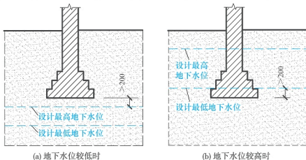
图 2.13 地下水位对基础埋深的影响
