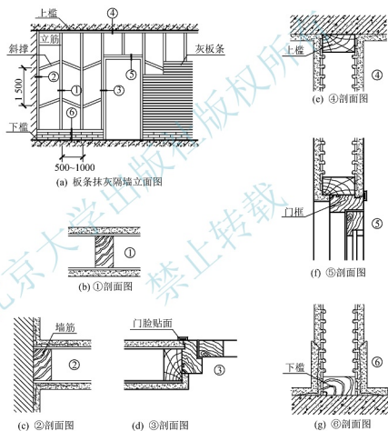
图 3.43 板条抹灰隔墙构造
