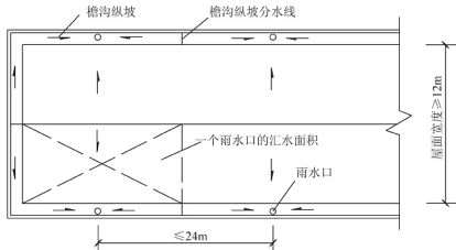
图 6.17 屋面雨水口间距示意
