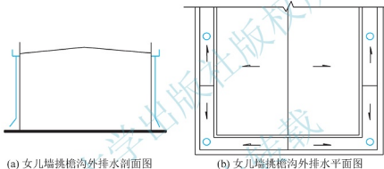
图 6.15 女儿墙挑檐沟外排水
