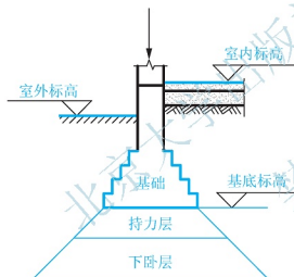
图 2.2 基础与地基
