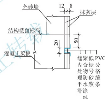
图 3.47 抹灰面的分块与设缝
