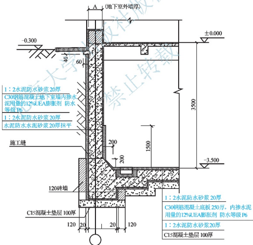
图 2.41 某建筑地下室防水混凝土构造大样图
