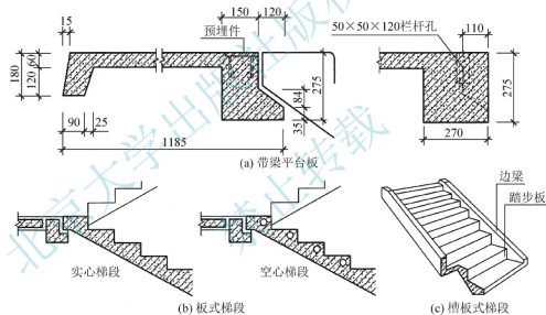
图 5.23 中型、大型预制装配式楼梯
