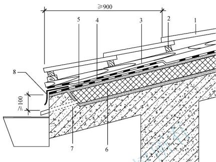
1—块瓦；2—挂瓦条；3—顺水条；4—防水垫层；5—防水垫层附加层； 6—保温隔热层；7—排水管；8—金属泛水板
