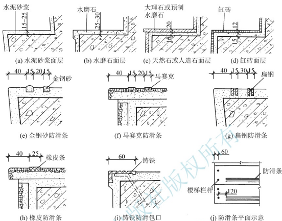
图 9.3 楼梯踏步参考构造
