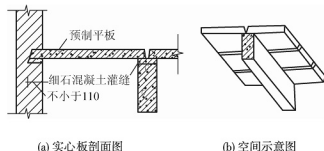
图 4.16 实心板
