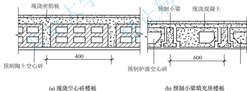
图 4.24 密肋填充块楼板
