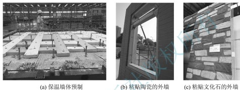
图 10.8 预制墙体
