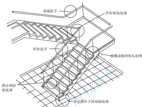
图 5.26 楼梯细部构造
