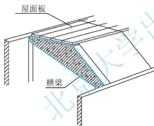
图 6.10 结构找坡
