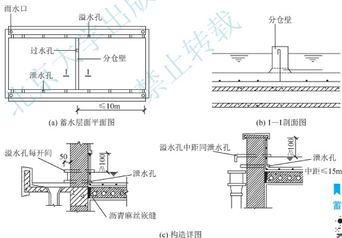
图 6.29 蓄水屋面构造
