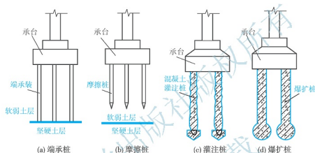
图 2.25 桩基础
