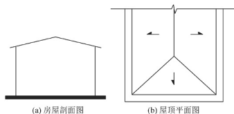
图 6.12 无组织排水
