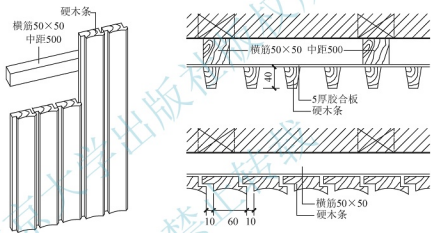
图 3.58 木质面板墙面装饰构造
