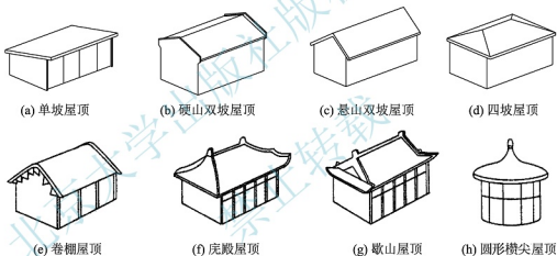
图6.2 常见坡屋顶的形式
