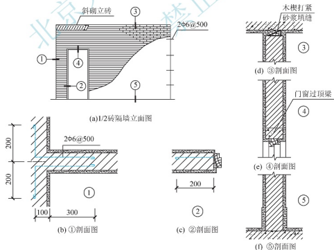
图 3.40 1/2 砖隔墙构造
