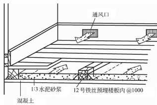
(a) 铺钉式木地板
