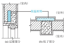
图 3.13 热桥部位保温处理
