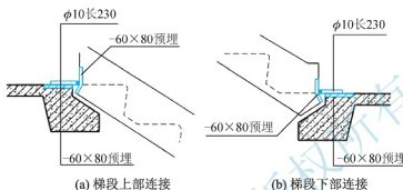
图 5.25 梯段与平台板连接的构造示例
