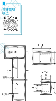
图 5.45 乘客电梯井道剖面图
