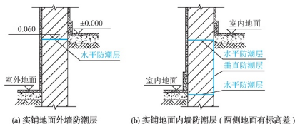
图 3.30 防潮层的位置
