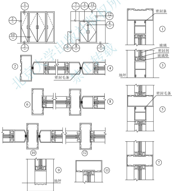
图 7.17 铝合金弹簧门的构造示意
