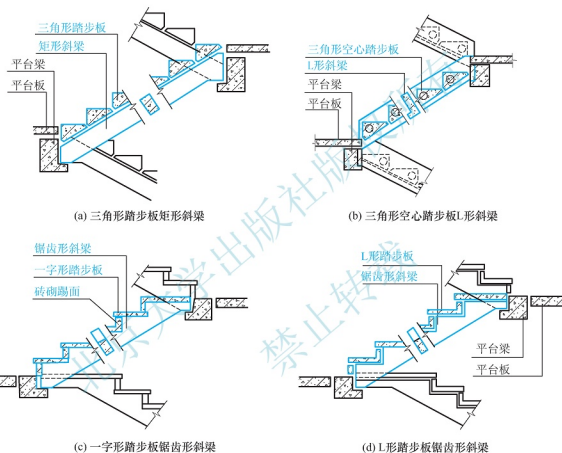
图 5.18 梁承式楼梯构造
