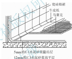
(b) 陶瓷锦砖地面构造示意图
