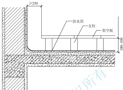
图 6.28 架空屋面构造
