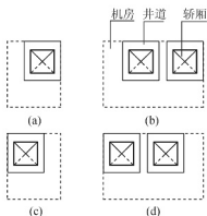
图 5.46 电梯机房与井道平面位置
