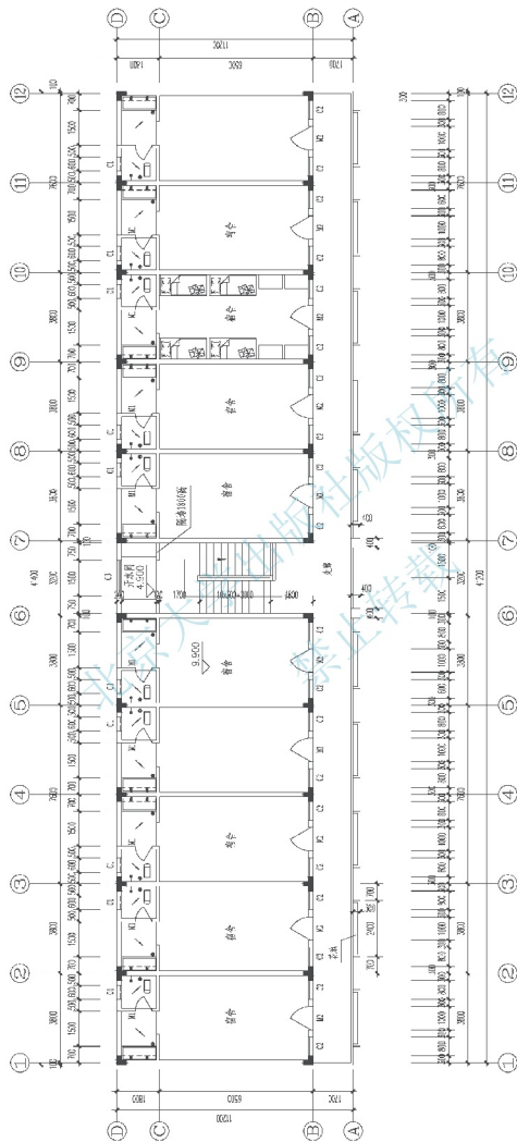
六层平面 1:100
