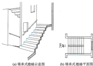
图 5.21 墙承式楼梯
