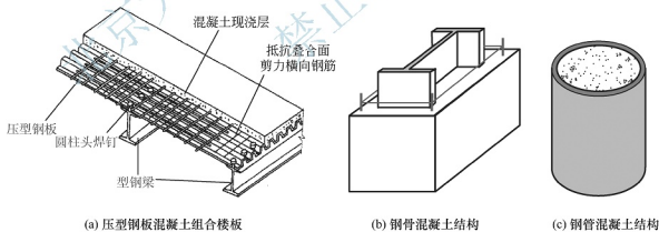
图 0.21 钢-混凝土组合结构
