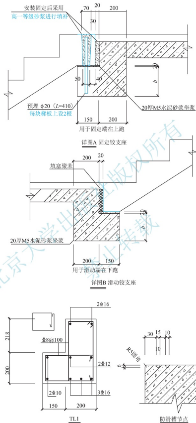
图 10.13 装配式楼梯平面图、剖面图及节点详图 (续)
