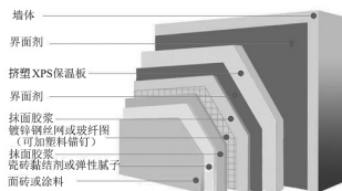
图 3.16 挤塑板外墙保温构造
