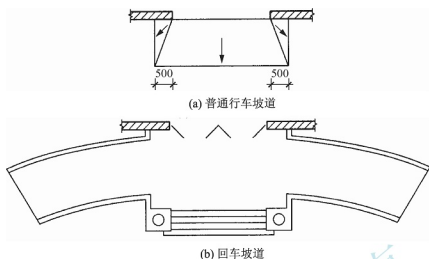
图 5.40 行车坡道
