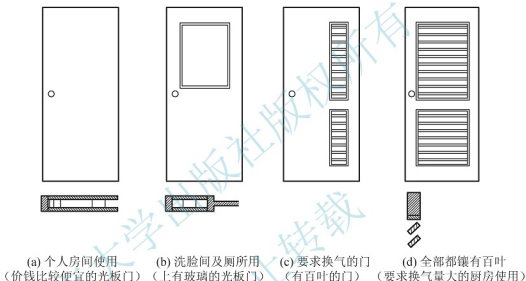
图 7.8 夹板门示意图
