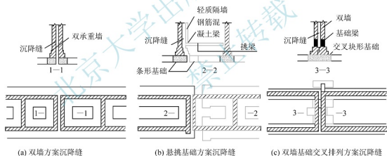
图 8.6 基础沉降缝处理示意
