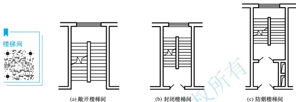
图 5.3 按楼梯间的平面形式分类
