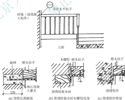
图 9.6 扶手端部与墙的连接
