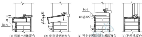
图 3.32 窗台形式
