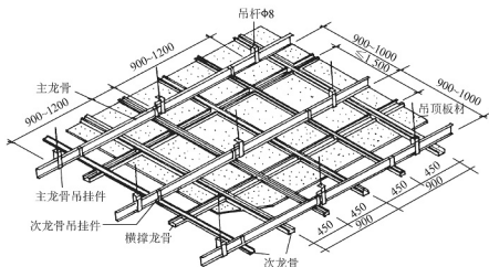
(a) 不露龙骨吊顶示意图
