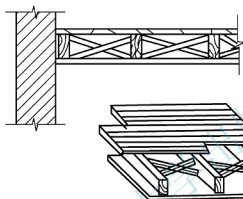
(a) 砖木结构中的木楼板
