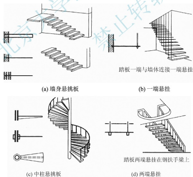
图 5.22 悬臂楼梯
