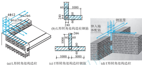
图 3.38 转角处的钢筋混凝土构造柱
