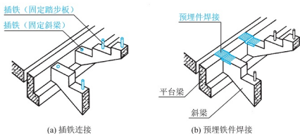
图 5.19 斜梁与平台梁的连接
