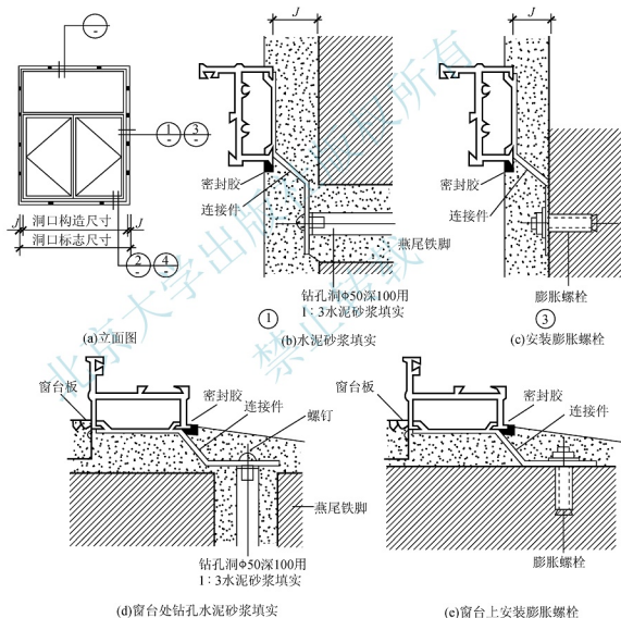
图 7.20 铝合金窗安装构造示意
