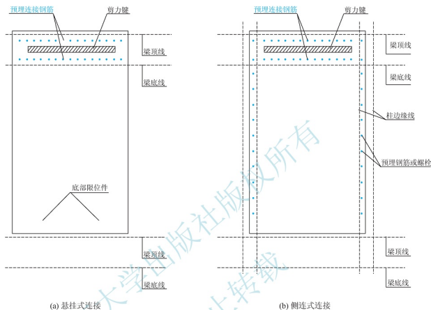
图 10.5 PC 外墙的连接方式示意
