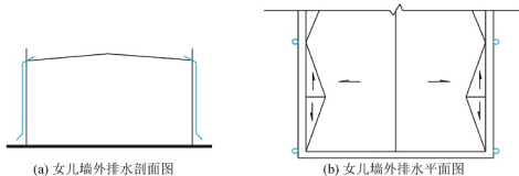
图 6.14 女儿墙外排水
