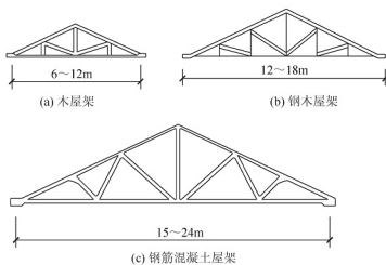
图 6.34 屋架形式
