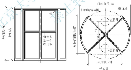
图 7.12 转门构造图
