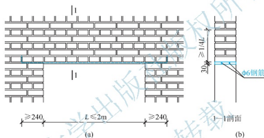
图 3.34 钢筋砖过梁构造
