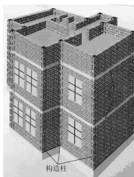
(a) 图中每层都设置圈梁
