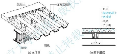
图 4.14 压型钢板组合楼板构造图
