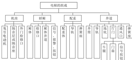
图 5.43 电梯的组成
