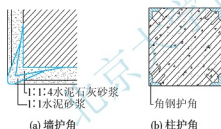
图 3.46 墙和柱的护角
