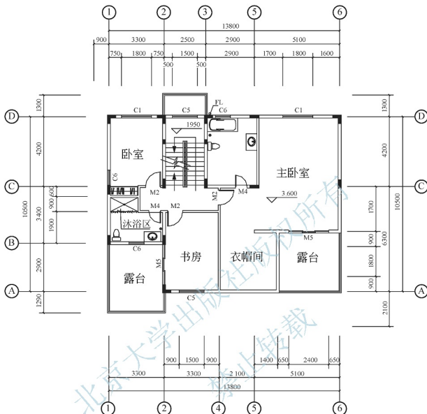
图 0.25 某住宅建筑平面图
