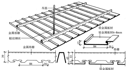
图 4.45 金属板材顶棚
