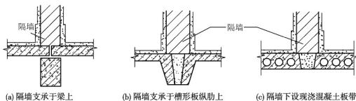
图 4.23 楼板与隔墙
