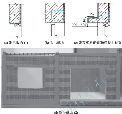
图 3.35 钢筋混凝土过梁构造
