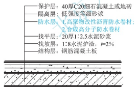
图 6.18 高聚物改性沥青防水卷材、合成高分子防水卷材防水上人屋面做法
