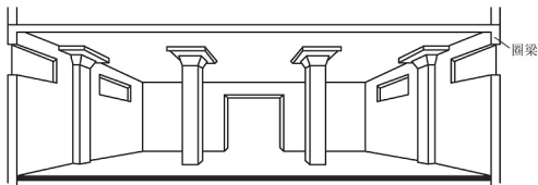
图 4.13 无梁楼板
