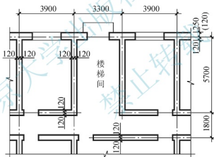
图 9.1 某3层砖混结构内廊式办公楼底层局部平面
