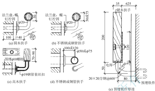
图 5.33 靠墙扶手的连接方式
