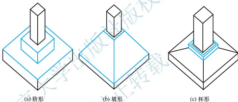
图 2.18 独立基础
