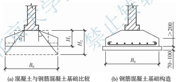
(a) 混凝土与钢筋混凝土基础比较 (b) 钢筋混凝土基础构造
