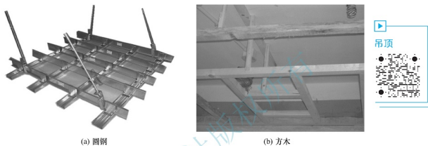
图 4.40 吊筋形式
