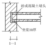
(b) 梁板式剖面图(1)
