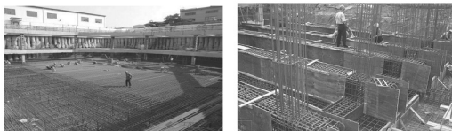
图 2.22 筏形基础 (续)
