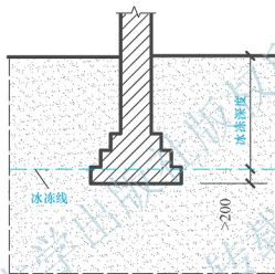
图 2.14 基础埋深与冰冻线的关系
