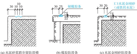
图 5.27 踏步面层防滑构造
