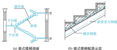
图 5.15 梁式楼梯
