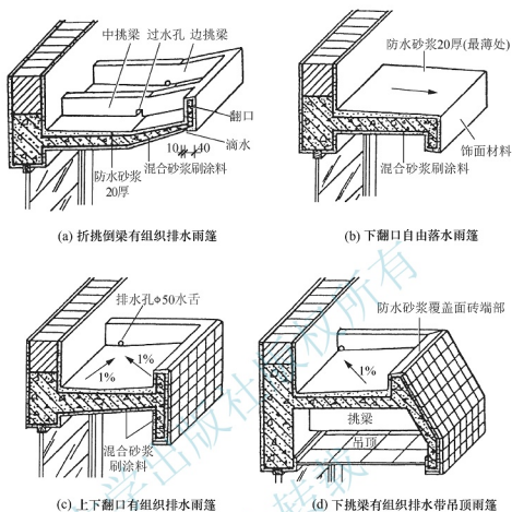
图 4.49 雨篷构造 2
