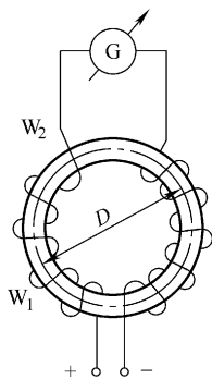
图 8-2 闭磁路试样
