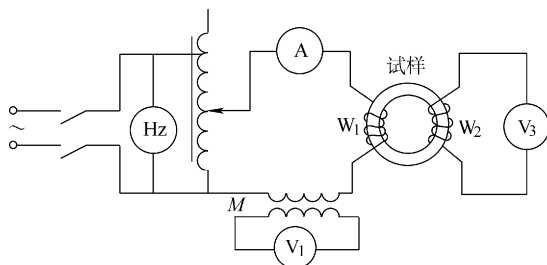
图 8-8 指示仪表测量动态磁化曲线的原理图
