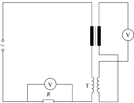
图 8-55 用峰值电压表测量
