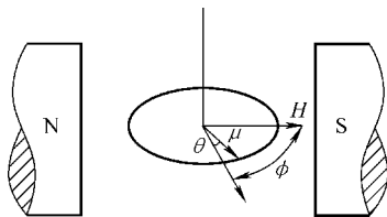
图 8-10 转矩磁强计结构示意图
