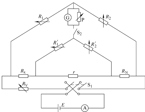
图 6-9 开尔文电桥
