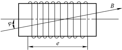
图 8-1 探测线圈
