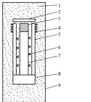
图 5-6 高温圆棒法测量装置
