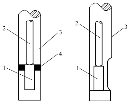
图 4-7 试样载体与推杆及试样接触面的典型形状
