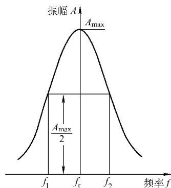
图 9-21 共振峰曲线
