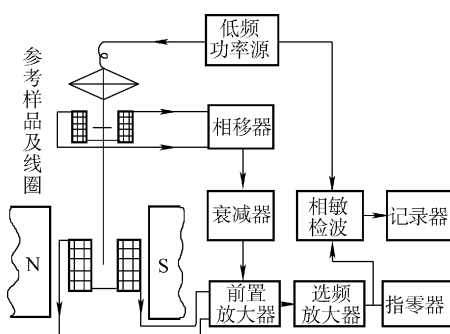
图 8-6 振动样品磁强计的原理
