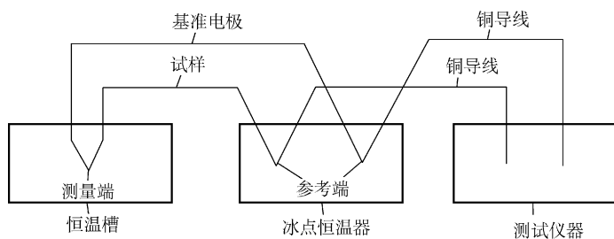
图 7-14 测试装置与试样的连接示意图
