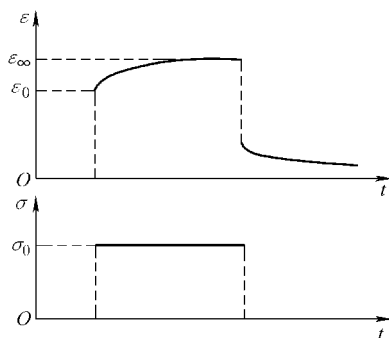
图 9-19 应变弛豫
