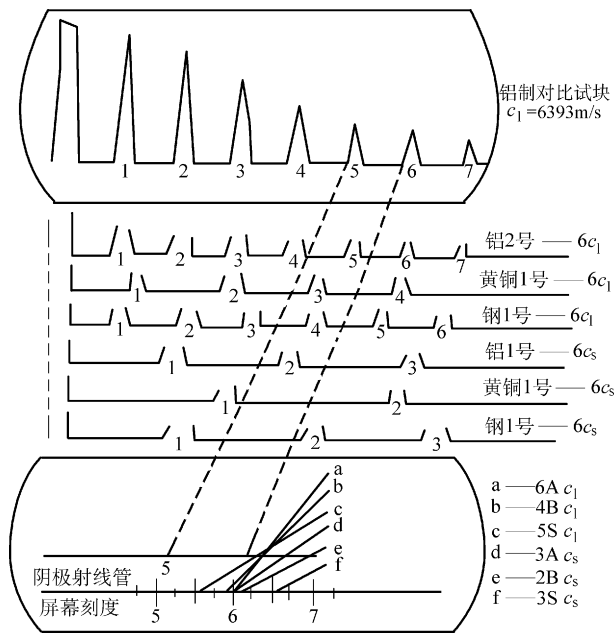
图 10-7 避免因视差引起误差所进行的仪器设置
