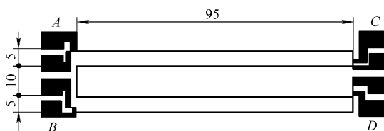
图 6-12 试验板推荐的试验图形
