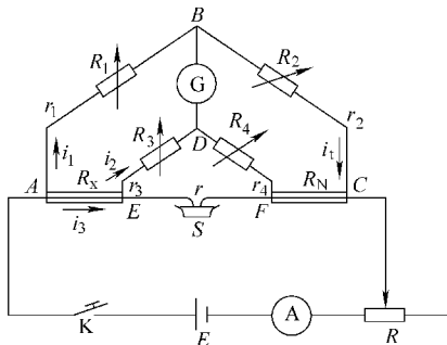
图 6-4 开尔文电桥测量原理图
