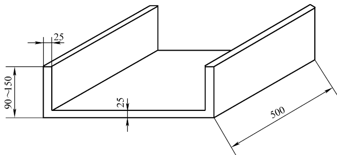
图 8-48 磁轭尺寸图
