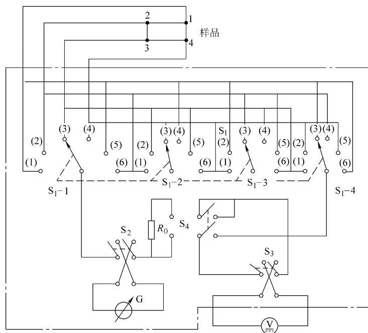
图 6-19 薄片样品的测试电路
