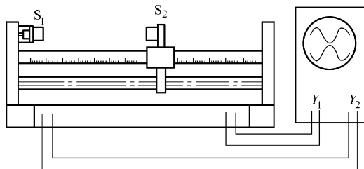
图 10-3 试验装置图
