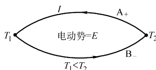
图 7-2 塞贝克效应示意图
