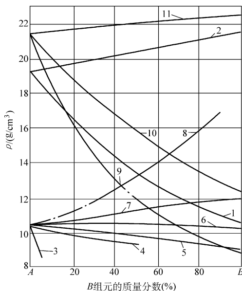
图 2-1 合金密度随成分的变化曲线
