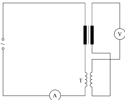
M—空气磁通补偿的互感线圈
