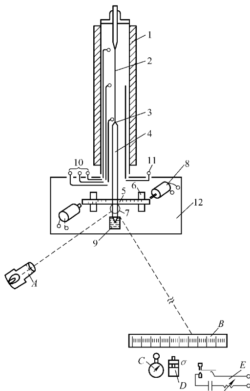
图 9-22 葛摆仪装置
