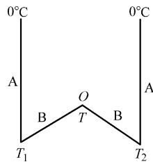
图 7-8 示差法测量热电势的原理
