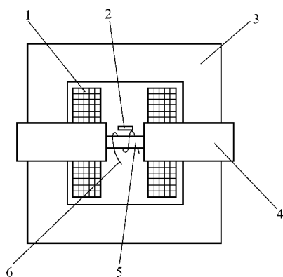
图 8-35 磁化装置
