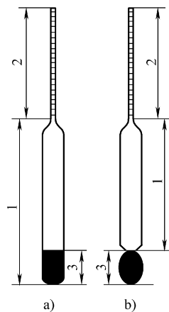
图 2-6 浮计的结构
