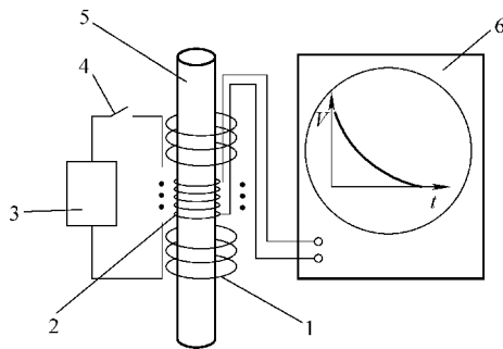
图 6-6 涡流衰减法测量试样电阻率原理图
