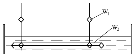
图 2-11 在液体中称量示意图
