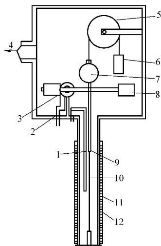
图 9-24 倒置扭摆仪
