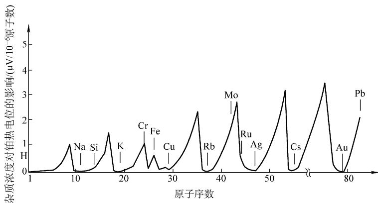
图 7-4 杂质对铂热电势的影响
