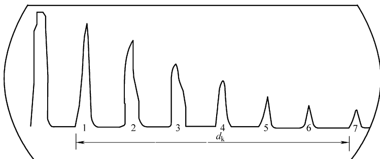
图 10-2 始波脉冲和 7 个反射回波
