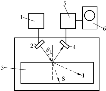
图 10-5 浸入式波速检测装置 1—脉冲发生器 2—发射换能器 3—试样 4—接收换能器 5—放大器 6—示波器 I—非全反射时折射的纵波 S—切变波 \theta_1 —入射角
