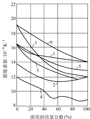
图 4-1 固溶体的膨胀系数
