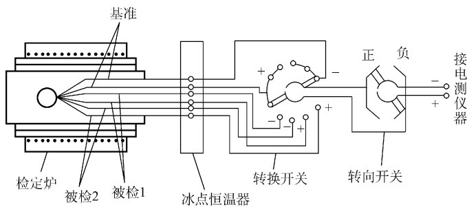
图 7-10 同名极比较法试验连接电路
