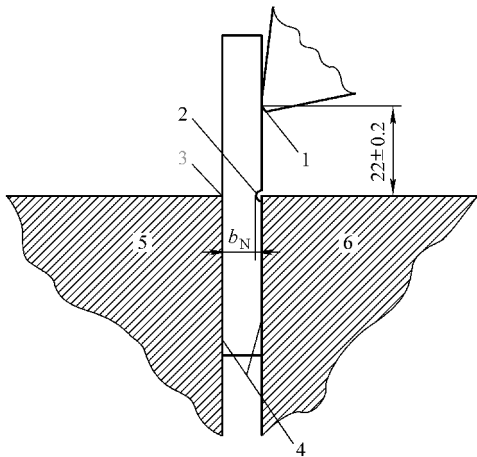
图 4-20 夹具、试样（缺口）和冲击刃冲击示意图
