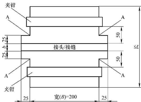
图 2-142 试样尺寸
