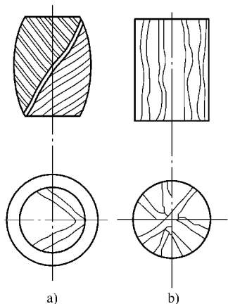
图 7-15 脆性材料端面摩擦力对压缩破坏的影响
