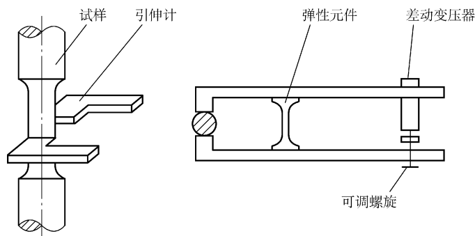
图 10-40 径向应变引伸计
