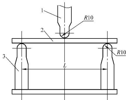
图 8-61 试验装置
