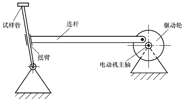
图 4-40 振动装置示意图
