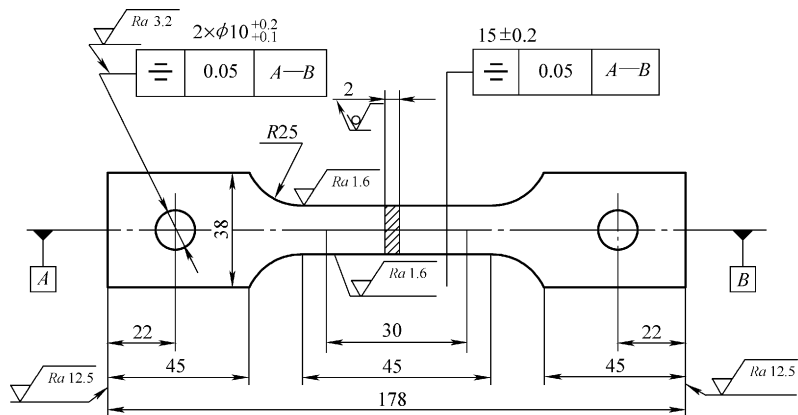
图 2-31 第 1 类低温拉伸试样
