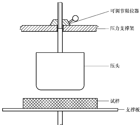
图 10-42 手动调节装置示意图
