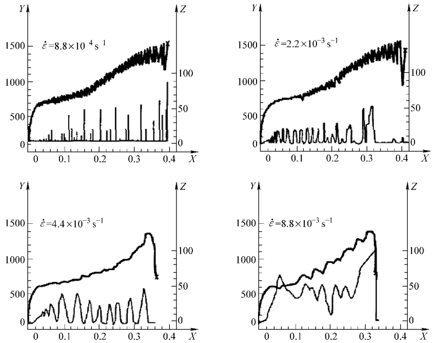
图 2-35 应力-应变曲线图及温度记录 X—应变 Y—应力 Z—温度 (K)
