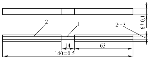
图 7-22 压缩试样
