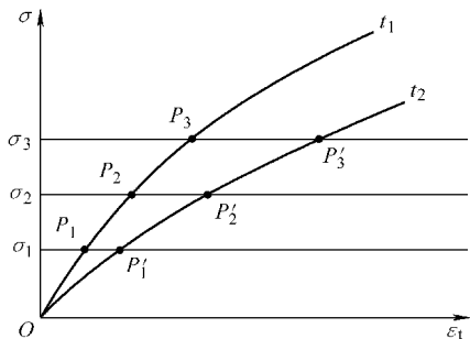
图 2-96 等时应力-应变曲线
