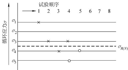
图 10-13 第三种情况的试验顺序
