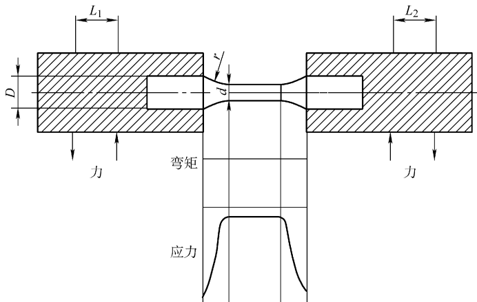
图 10-16 圆柱形试样（四点加力）
