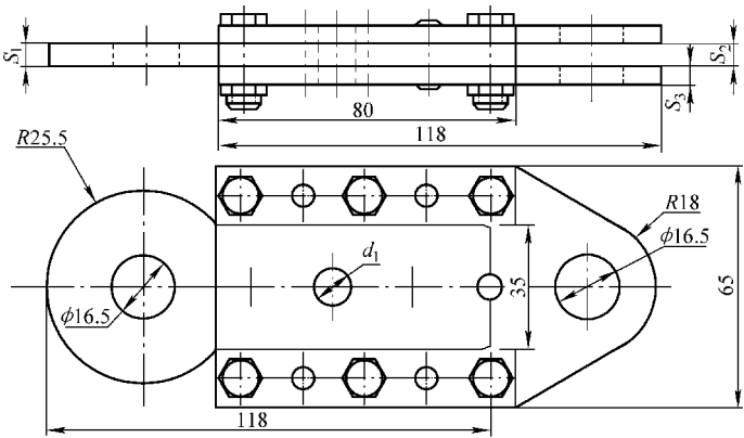
图 6-12 室温拉式双剪夹具尺寸
