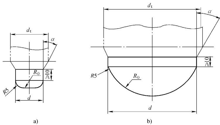
图 4-32 落锤的锤头
