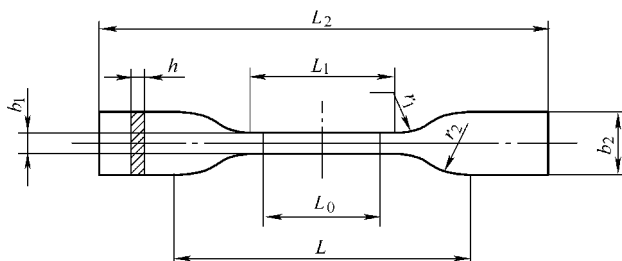
图 2-82 5A 型和 5B 型试样的形状
