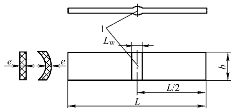
图 8-49 平行面（板材、管材）试样形状
