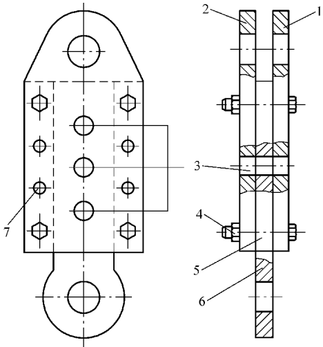
图 6-11 室温拉式双剪夹具
