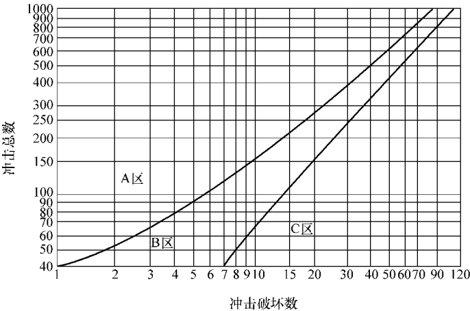
图 4-33 TIR 值为 10% 时判定图
