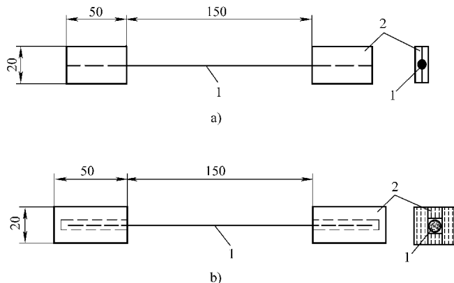
图 2-148 试样的形状及尺寸
