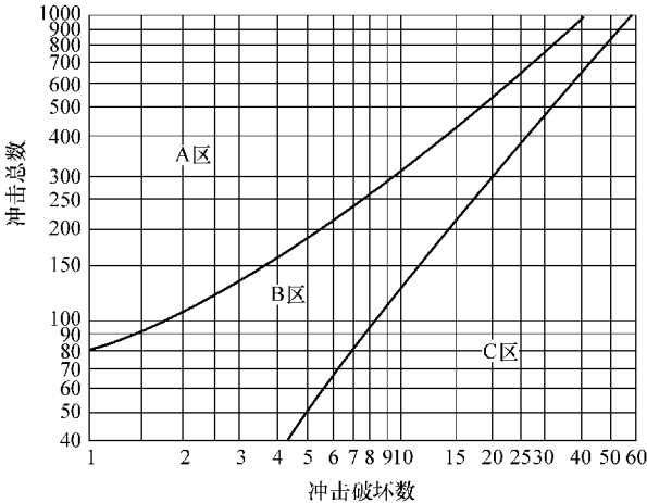
图 4-34 TIR 值为 5% 时判定图
