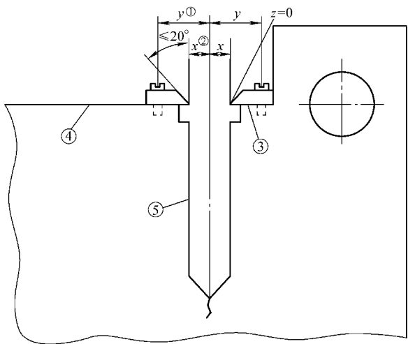
图 9-29 内置刀口和相应的缺口几何尺寸
