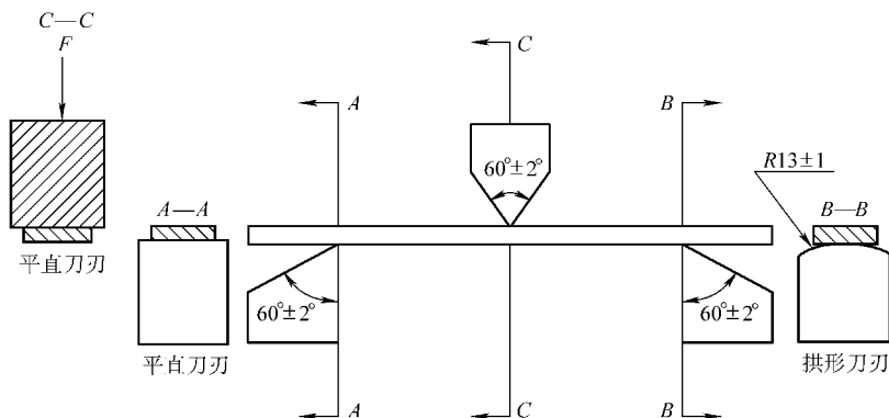
图 8-3 薄板试样用三点弯曲试验装置
