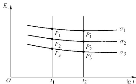
图 2-95 蠕变模量-时间曲线
