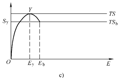
图 2-131 拉伸示意图
