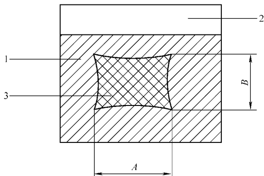
图 4-6 剪切断面率百分比的尺寸
