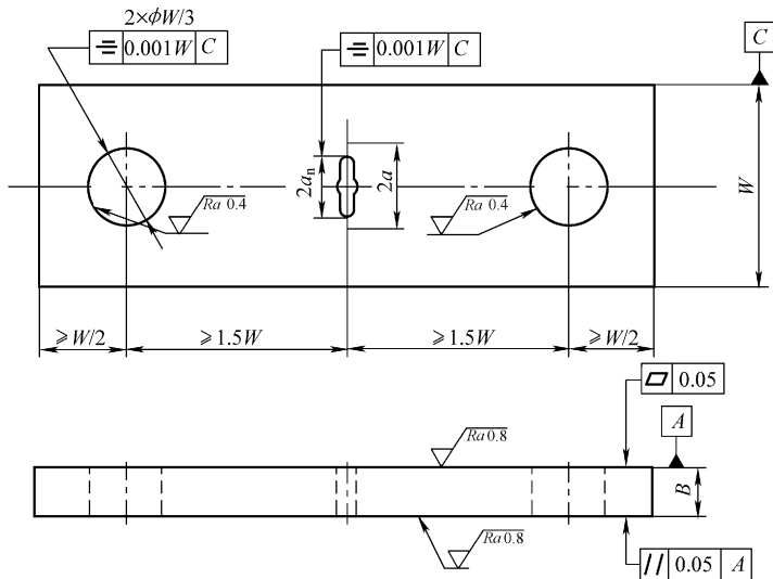
图 10-26 W 不大于 75\text{mm} 的 M (T) 试样
