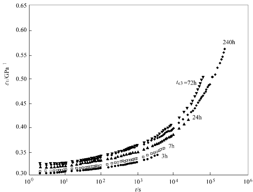
图 2-100 由 23℃ 加热至 44℃ 并保温不同时间 t_{e2} 的 PVC 试样蠕变曲线
