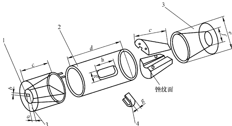
图 7-23 试验夹具示意图
