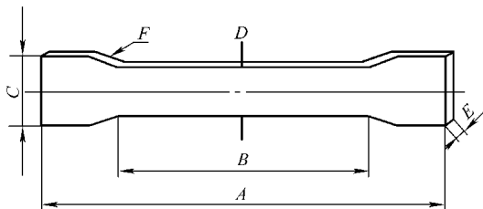
图 2-133 硬质橡胶拉伸试样
