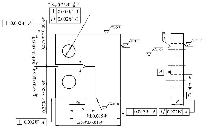
图 10-25 标准 C (T) 试样
