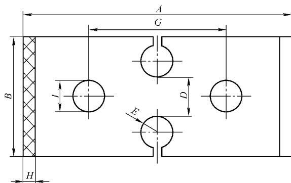
图 2-124 A 型试样
