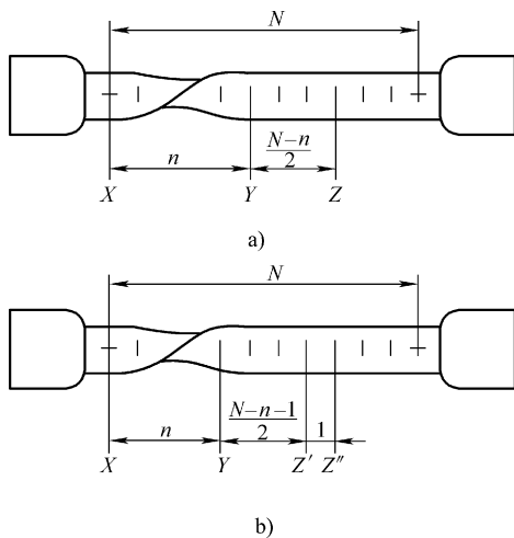
图 2-22 移位法图示说明 (试样头部仅为示意性)
