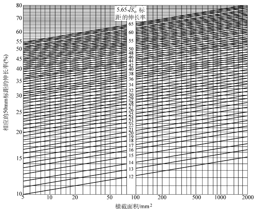
图 2-27 奥氏体钢 5.65√S 0 与 50mm 定标距的断后伸长率的换算关系
