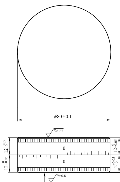
图 7-7 调平垫块
