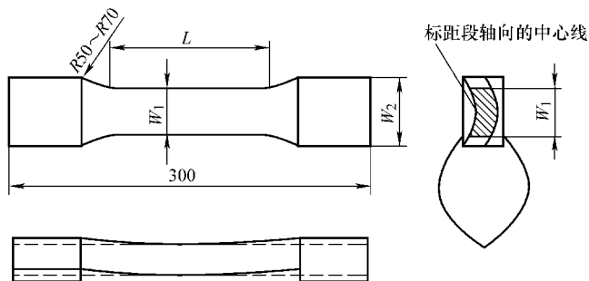
图 2-108 取样拉伸试样
