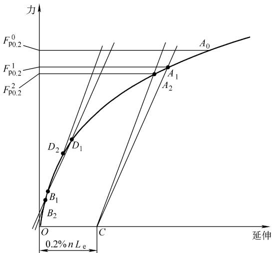
图 2-19 逐步逼近法测定规定塑性延伸强度 R_{p0.2}
