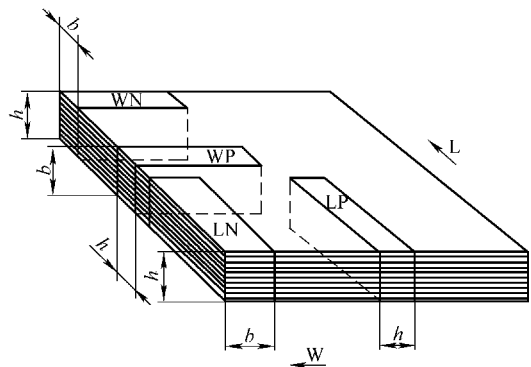
图 8-44 相对于产品方向和施力方向的试样位置
