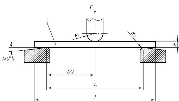
图 8-45 支座和压头
