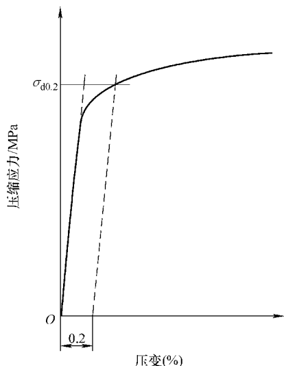
图 7-17 用 0.2% 压缩应变处胡克直线的行线确定 0.2% 压缩极限 \sigma_{d0.2} 的示意图
