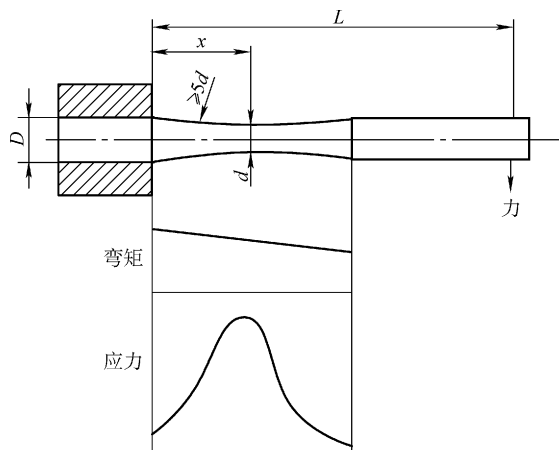
图 10-18 漏斗形试样 (单点加力)
