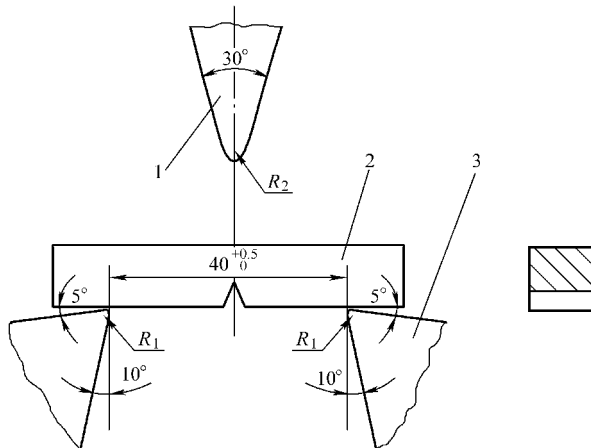
图 4-39 试样支座及摆锤刀刃尺寸
