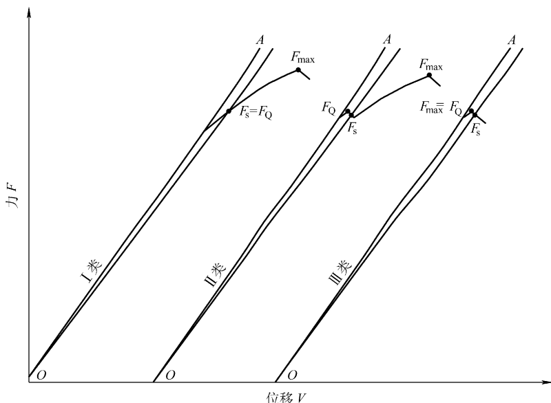
图 9-14 典型的力-位移记录曲线
