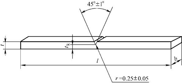
图 4-22 A 型缺口试样
