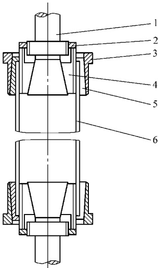
图 2-107 试样的夹持装置
