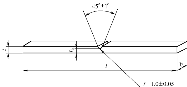
图 4-23 B 型缺口试样
