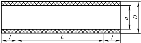
图 2-106 整体拉伸试样
