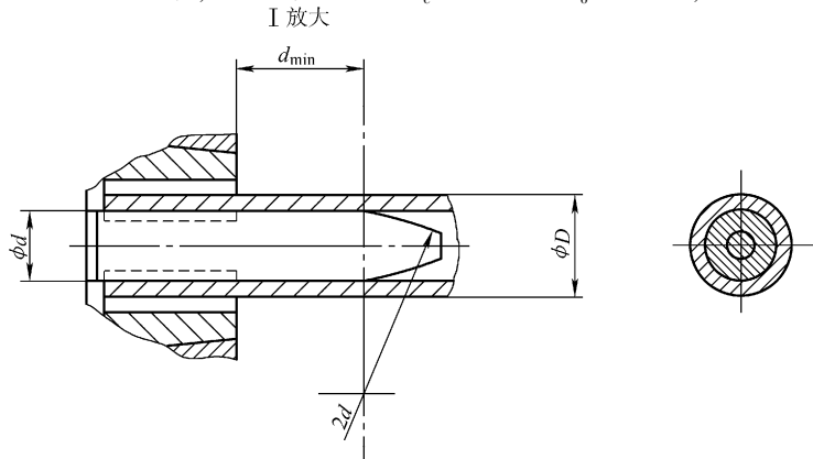
图 2-55 整管拉伸试样
