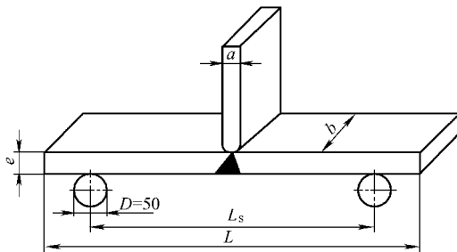
图 8-54 弯曲试验示意图
