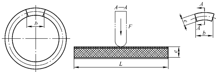
图 8-53 辐射面取样和受力方向
