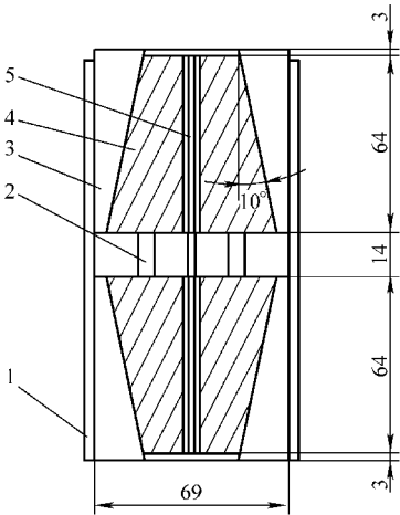
图 7-24 试验夹具装配图
