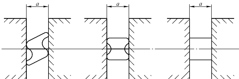
图 8-17 非圆形试样的夹持
