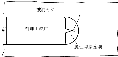
图 9-17 使用缺口脆性焊接引发裂纹
