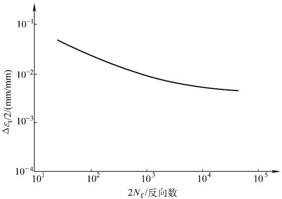
图 10-32 \Delta\varepsilon_t/2-2N_f 曲线
