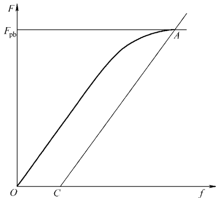
图 8-6 图解法测定规定非比例弯曲应力
