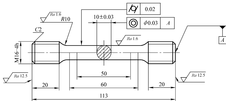
图 2-34 第 4 类低温拉伸试样
