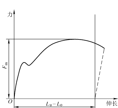
图 2-15 最大力 F_m
