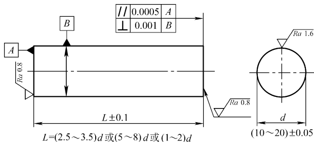
图 7-2 圆柱体试样
