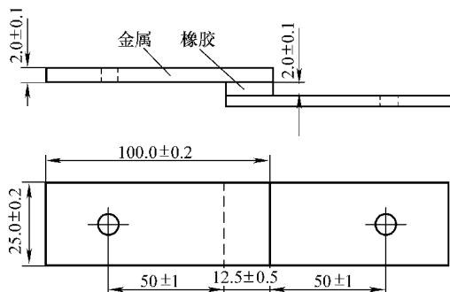
图 6-24 试样形状和尺寸
