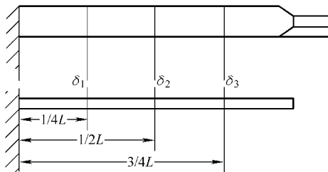
图 8-30 试样尺寸测量图
