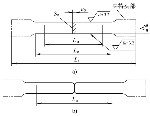
图 2-7 机加工的矩形横截面试样（试样头部仅为示意性）
