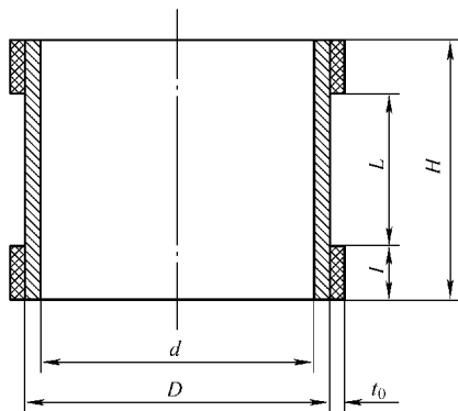
图 7-31 轴向压缩试样
