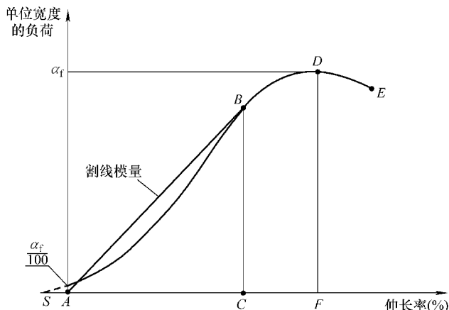
图 2-141 典型负荷-伸长率曲线图
