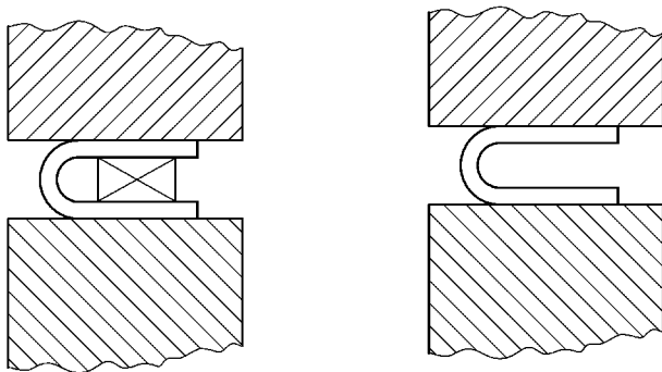
图 8-14 平行压板之间的后续弯曲
