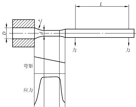
图 10-15 圆柱形试样（两点加力）
