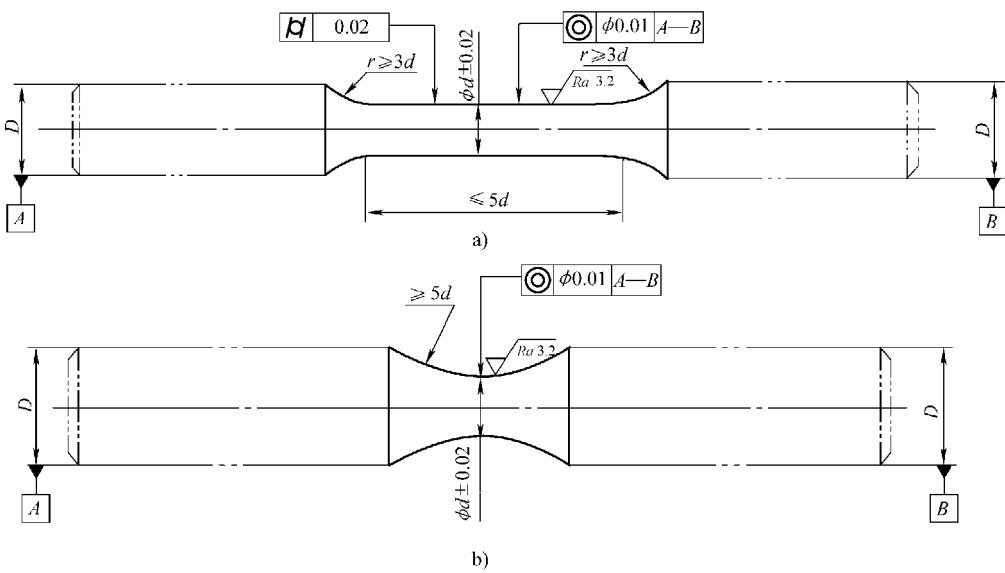
图 10-1 试样形状
