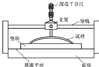
图 8-31 固定装置
