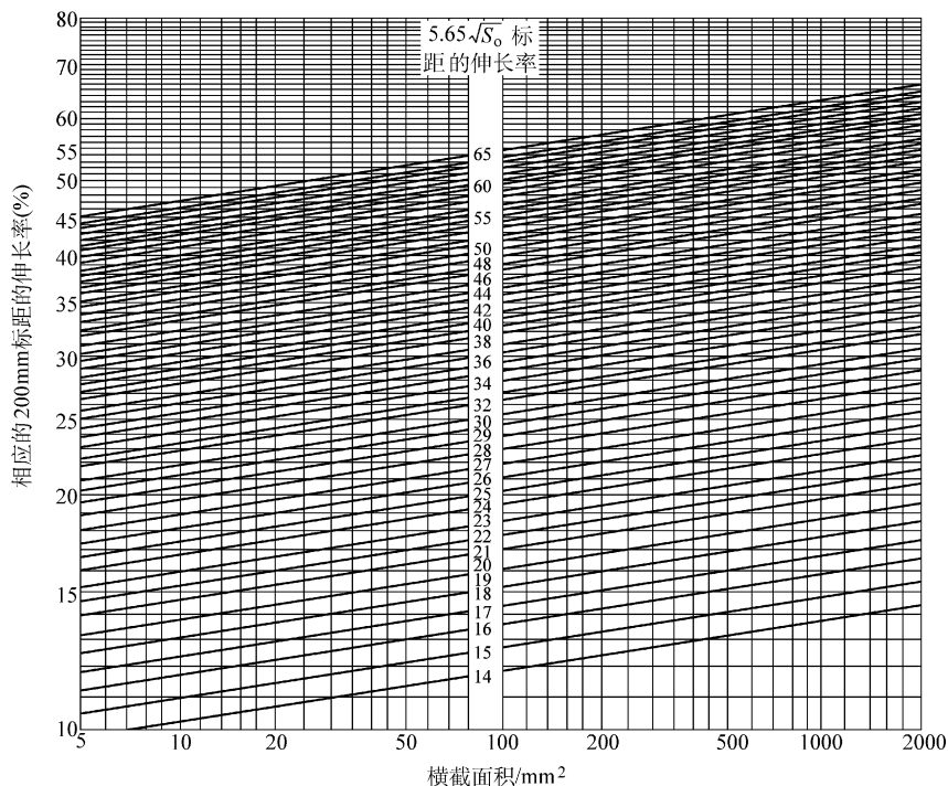
图 2-28 奥氏体钢 5.65√S 0 与 200mm 定标距的断后伸长率的换算关系
