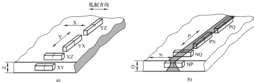
图 9-39 母材和焊缝断裂韧性试样裂纹面取样方位
