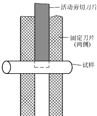
图 6-1 双剪切试验
