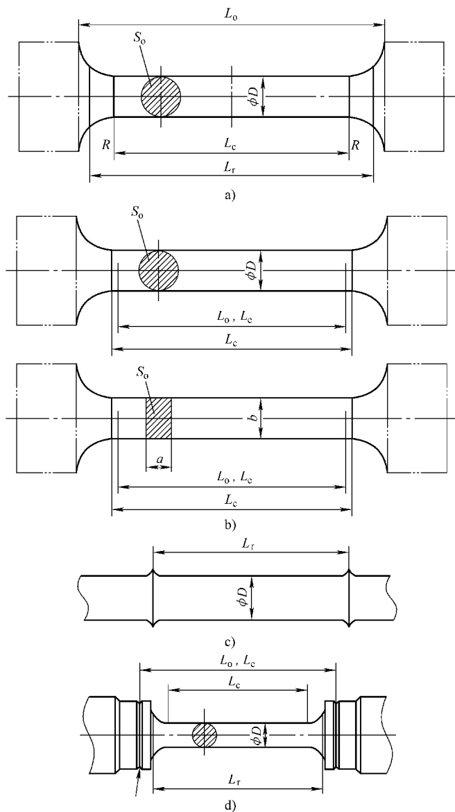
图 2-45 试样示例图
