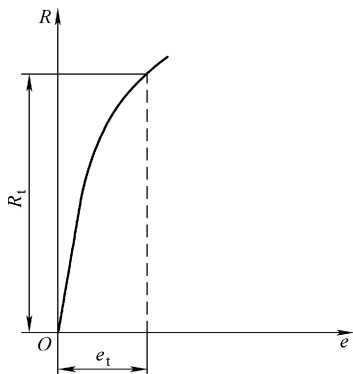
图2-5 规定总延伸强度( R_t )
