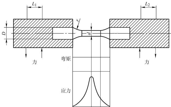
图 10-20 漏斗形试样（四点加力）
