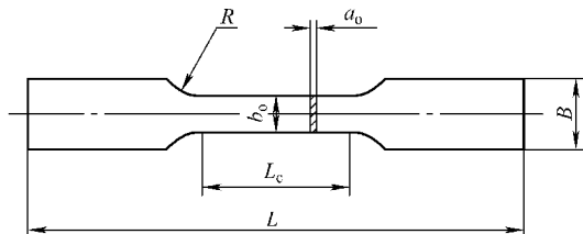
图 2-37 矩形横截面试样的形状
