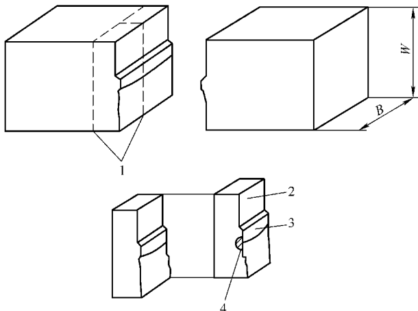
图 9-51 表面缺口试样试验后金相检查切片的切取方法
