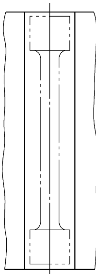
图 2-62 试样的位置示例 (纵向截面)
