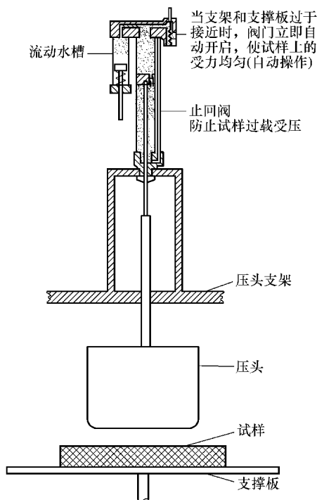
图 10-43 自动调节装置示意图
