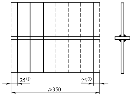
图 2-57 十字接头的取样部位
