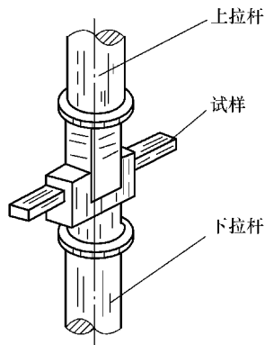
图 6-23 剪切试验装置
