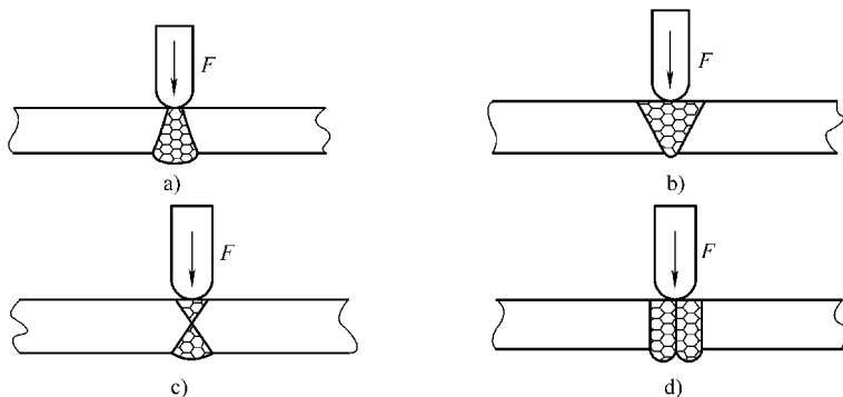
图 8-55 焊接试样的各种弯曲类型
