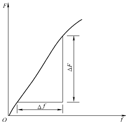
图 8-5 图解法测定弯曲弹性模量
