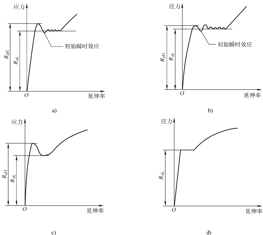
图 2-3 不同类型曲线的上屈服强度和下屈服强度 ( R_{eH} 和 R_{eL} )
