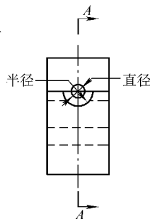
图 6-2 双剪切试验夹具刀口形状
