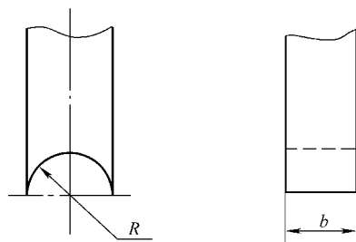
图 8-62 石墨管试验用上压头
