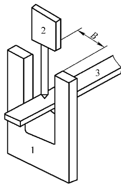
图 8-24 压持器
