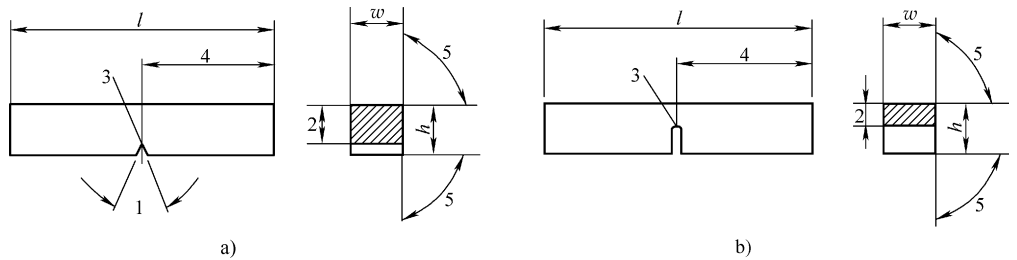
图 4-2 夏比冲击试样
