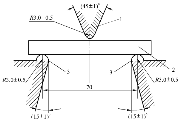
图 4-36 B 型试验机
