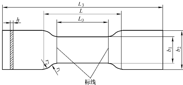
图 2-85 4 型试样
