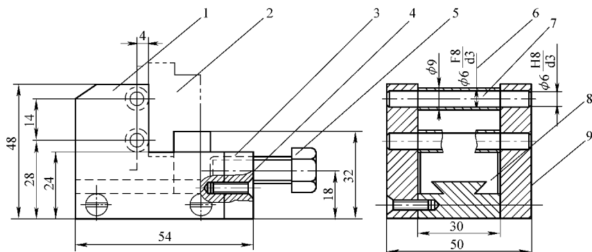
图 6-18 剪切夹具
