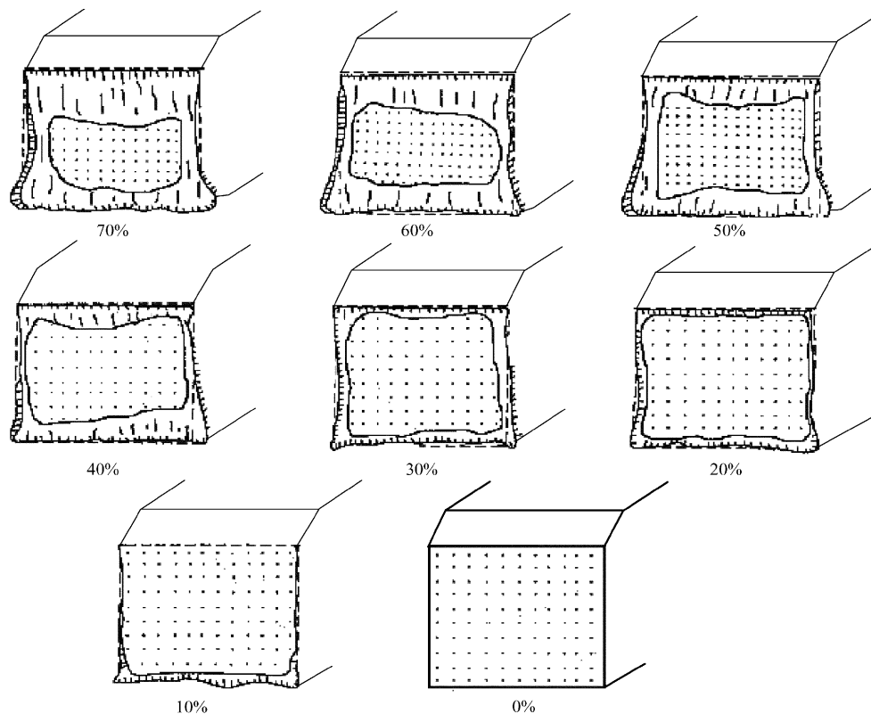
图 4-8 冲击试样断口纤维断面率示意图 (续)
