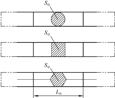
图 2-9 产品一部分不经机加工试样 (试样头部形状仅为示意性)
