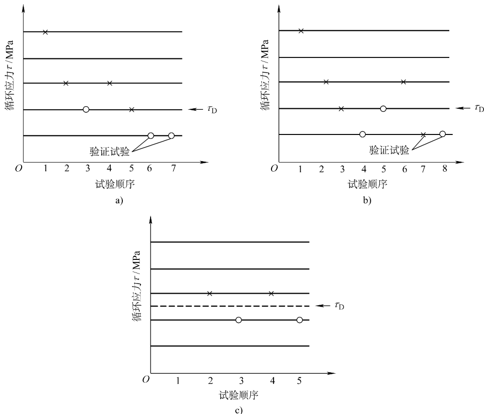
图 10-4 测定 \tau_D 的试验顺序
