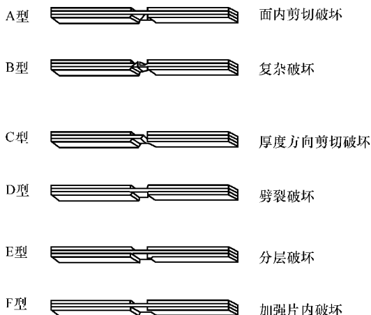
图 7-30 典型破坏模式
