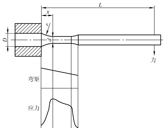
图 10-14 圆柱形试样（单点加力）
