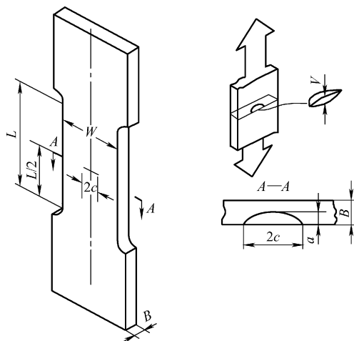
图 9-1 典型表面裂纹试样
