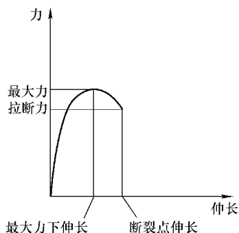
图 2-136 断裂点拉伸力
