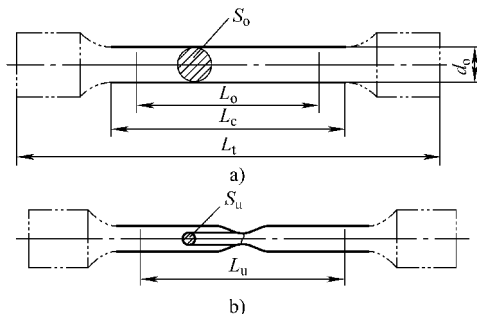
图 2-8 圆形横截面机加工试样
