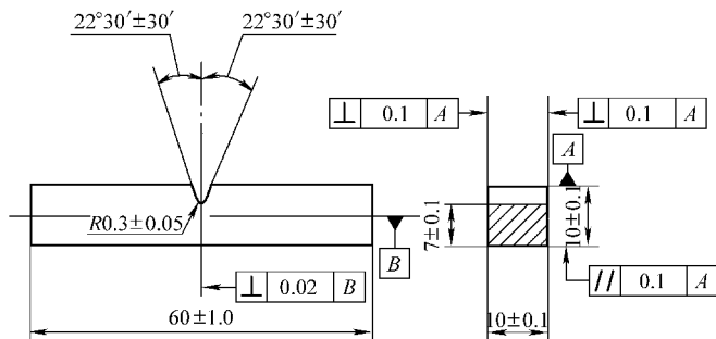
图 4-37 标准试样
