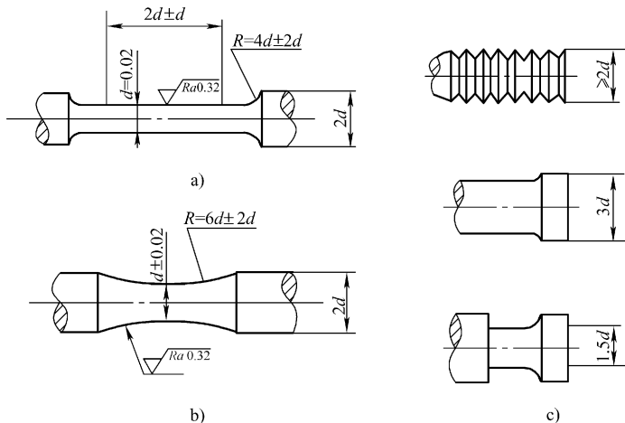
图 10-37 低循环疲劳试样
