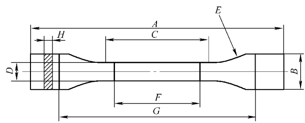
图 2-118 机械加工试样（类型 1）
