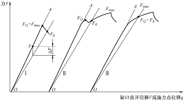
图 9-36 F_Q 的定义
