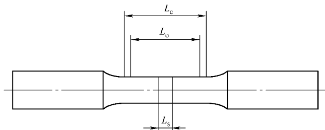
图 2-56 实心圆柱形试样
