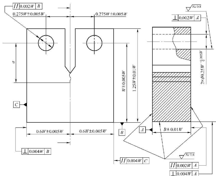
图 9-9 台阶形缺口紧拉试样
