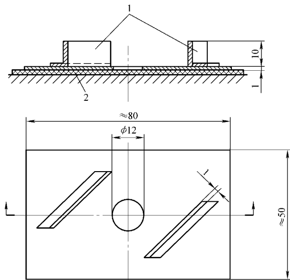
图 2-130 固定胶片的工具
