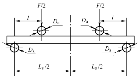
图 8-2 四点弯曲试验装置
