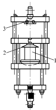
图 7-32 压缩器示意图
