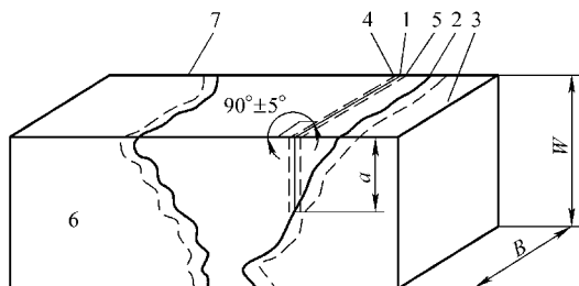
图 9-46 表面缺口试样缺口位置的确定
