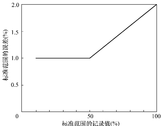
图 4-12 标准力范围内的记录值的允许误差
