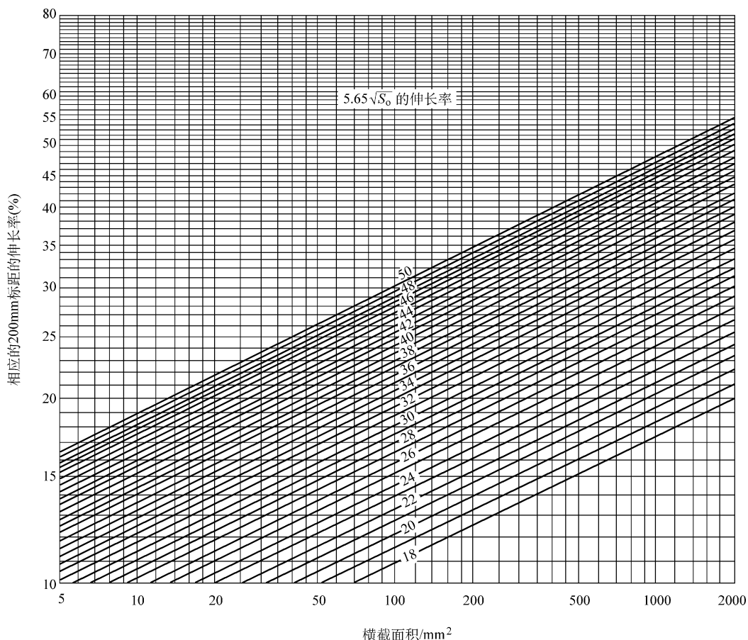
图 2-24 碳素钢和低合金钢 5.65\sqrt{S_0} 与 200mm 定标距的断后伸长率的换算关系
