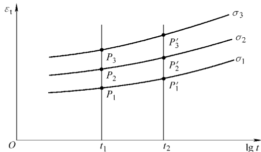
图 2-94 蠕变曲线
