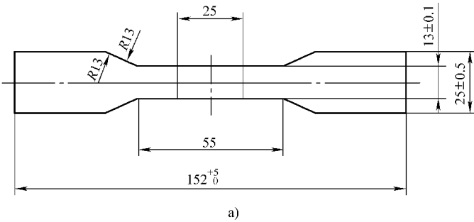
图 2-126 刀模尺寸示意图 a) 第一类刀模
