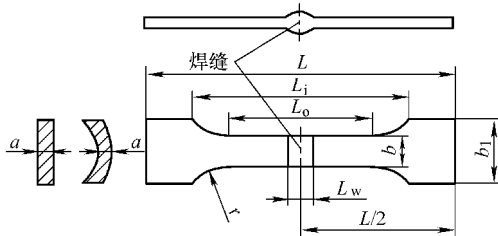
图 2-111 板材、管材拉伸试验哑铃形试样 L —试样总长度 (mm) L_0 —原始标距 (mm) L_i —带过渡弧试样长度 (mm) L_w —焊缝宽度 (mm) a —试样厚度 (mm) b —平行长度部分宽度 (mm) b_1 —夹持端宽度 (mm)
