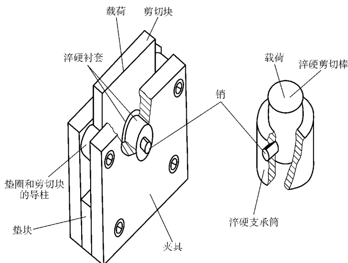
图 6-14 销剪切试验夹具
