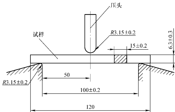
图 8-60 试验装置
