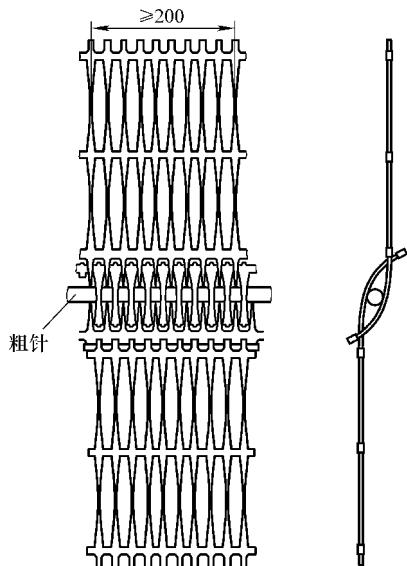
图 2-143 土工格栅试样图
