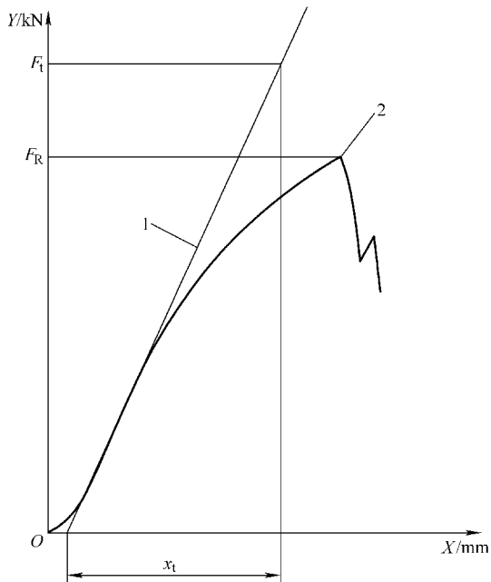
图 8-59 典型负荷-应变图
