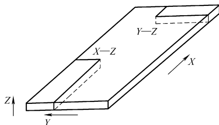
图 9-2 表面裂纹试样的取向标记
