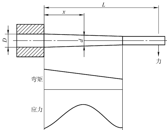
图 10-17 圆锥形试样（单点加力）
