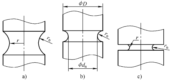
图 2-47 缺口试样
