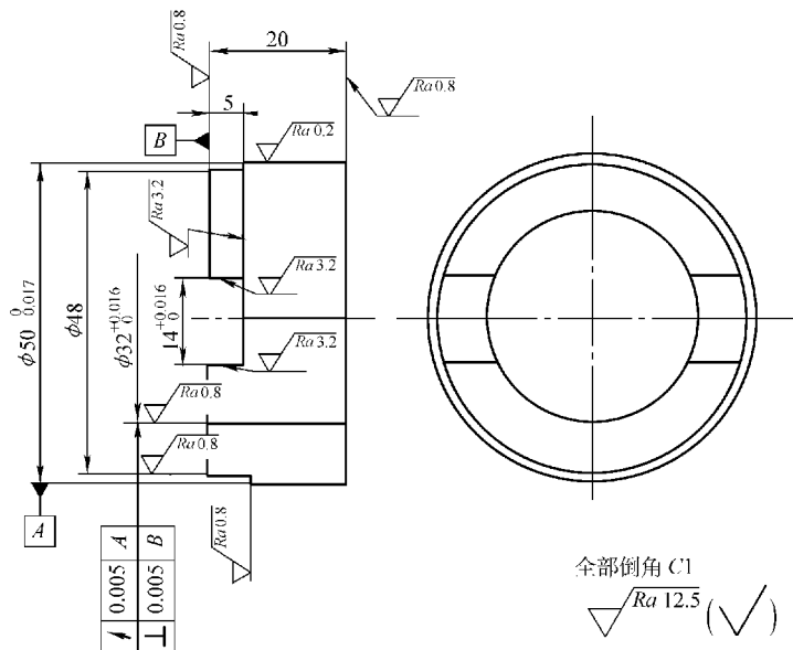
图 10-10 PS-2 试样
