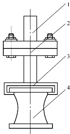
图 2-117 层间拉伸强度 试验专用夹具示意图
