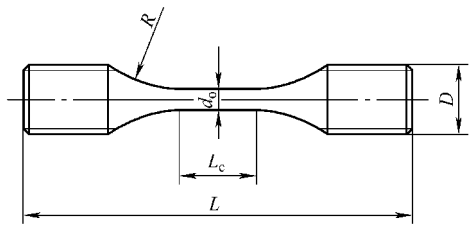
图 2-36 标准圆柱试样的形状 L—试样总长度 (mm) L c —试样平行长度 (mm) D—端头直径 (mm) d 0 —试样平行长度的直径 (mm) R—过渡圆弧 (mm)
