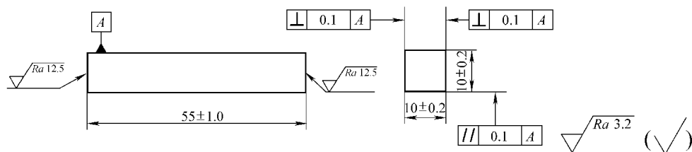
图 4-17 无缺口试样
