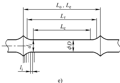
图 2-45 试样示例图 (续)
