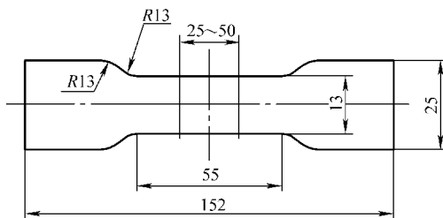
图 2-138 裁刀尺寸示意图
