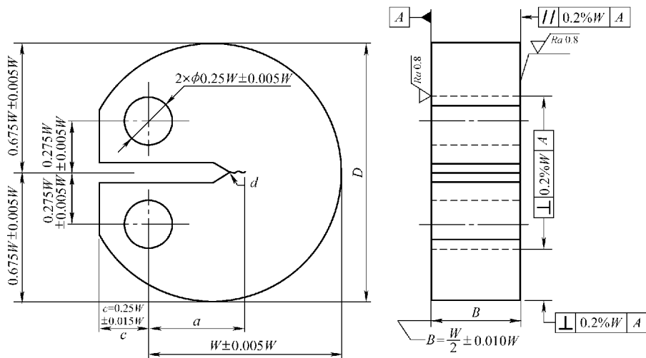
图 9-11 圆形紧凑拉伸试样
