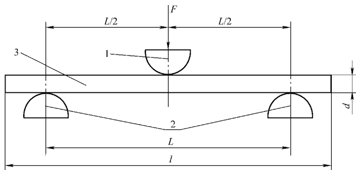
图 8-58 试验原理示意图
