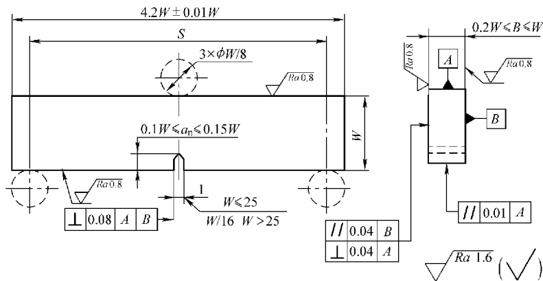
图 10-27 标准 SE (B) 试样
