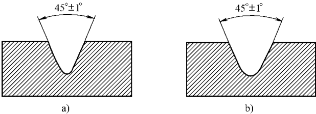
图 4-19 缺口类型 a) A 型 b) B 型
