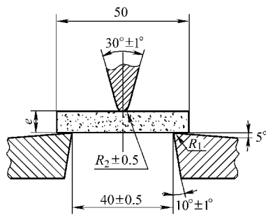
图 4-30 小试样的冲击刀刃和支座
