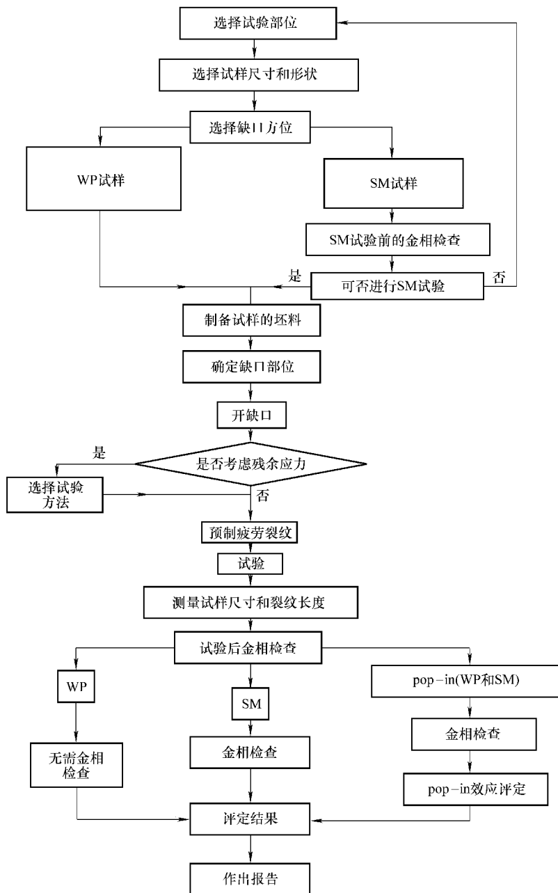
图 9-47 断裂韧性试验流程
