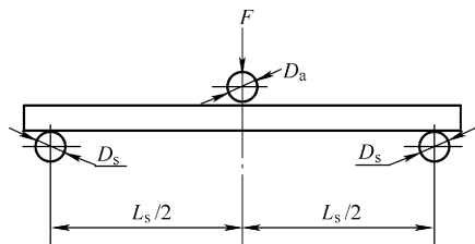
图 8-1 三点弯曲试验装置
