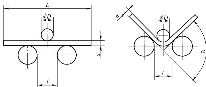
图 8-9 支辊式弯曲装置
