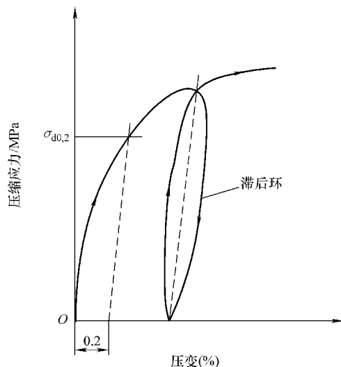
图 7-18 用 0.2% 压缩应变处滞后环中心线的平行线确定 0.2% 压缩极限 \sigma_{d0.2} 的示意图
