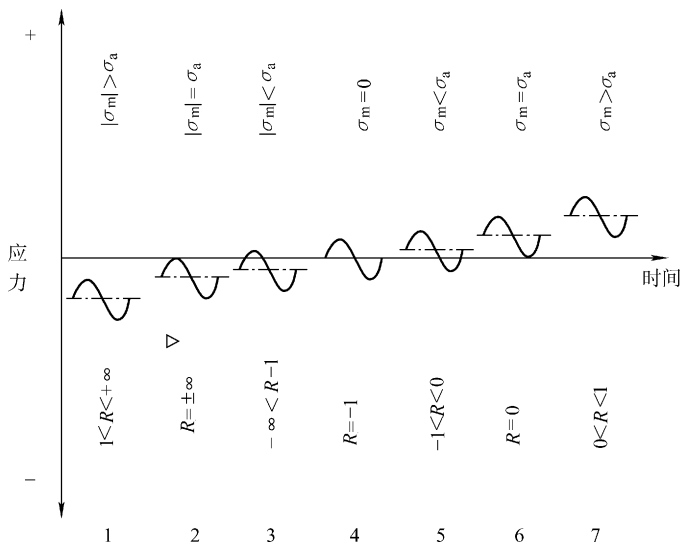
图 10-3 循环应力的类型
