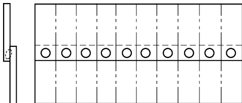
图 1-21 点焊接头抗剪样坯截取位置
