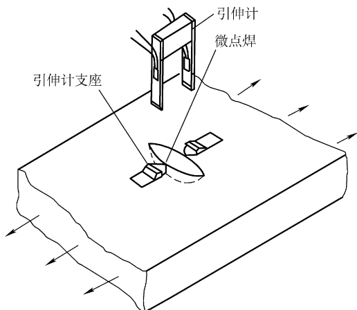
图 9-4 裂纹尖端张开位移典型的测量装置
