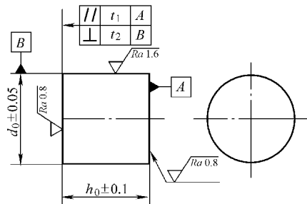
图 7-16 试样的几何精度
