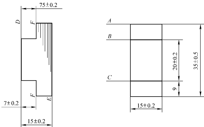
图 6-17 试样的形状和尺寸
