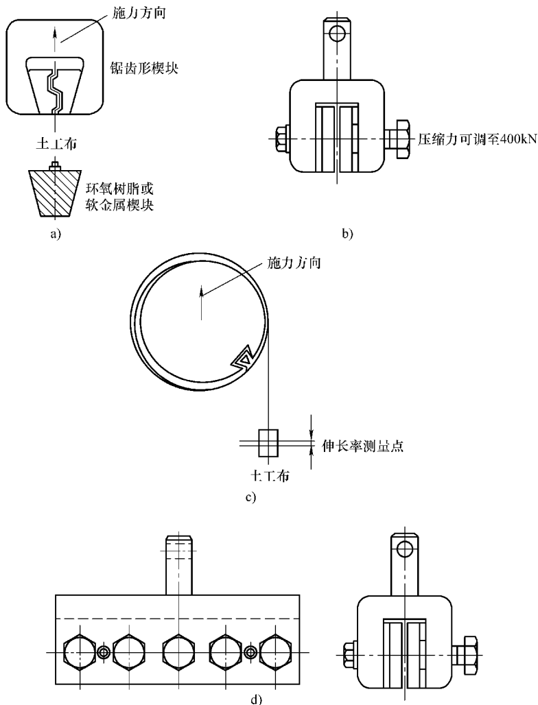
图 2-140 用于土工布拉伸试验的夹具示例
