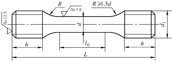
图 1-25 灰铸铁的拉伸试样
