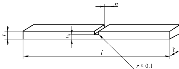
图 4-24 C 型缺口试样
