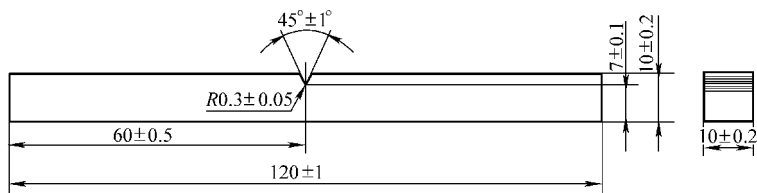
图 4-26 缺口方向与布层平行的纤维织物试样
