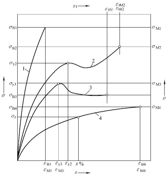
图 2-92 典型的应力-应变曲线
