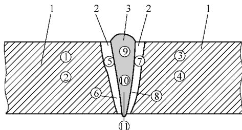
图 3-25 单点测定 (E) 硬度检验区域示例
