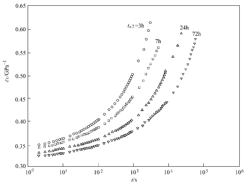
图 2-99 由 23℃ 加热至 44℃ 并保温不同时间 t_{e2} 的 PVC 试样蠕变曲线
