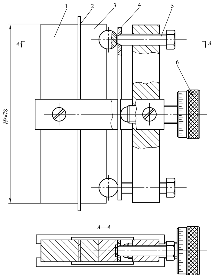
图 7-8 约束装置
