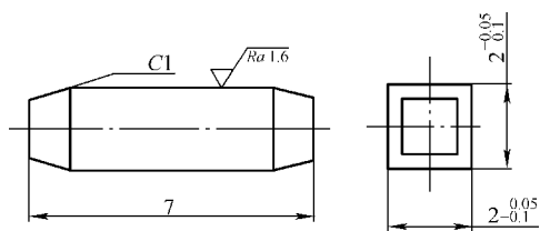
图 6-7 键
