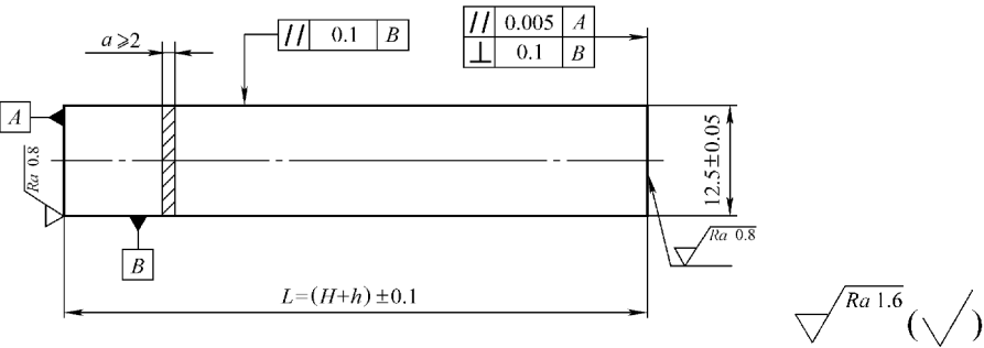
图 7-4 矩形板试样
