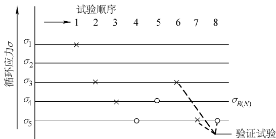
图 10-12 第二种情况的试验顺序
