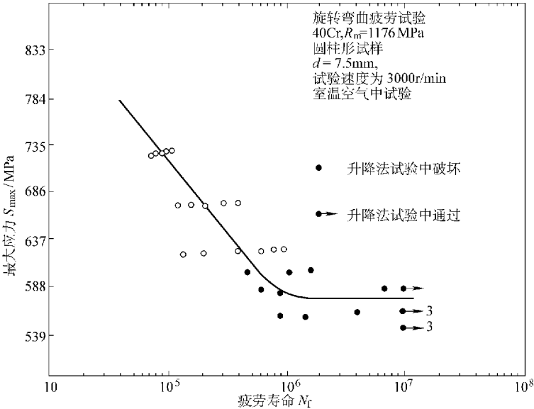
图 10-24 S-N 曲线图
