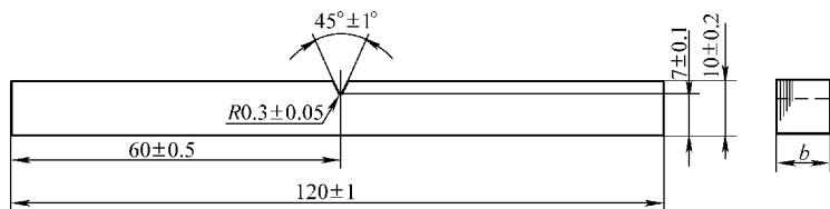
图 4-25 缺口方向与布层垂直的纤维织物试样
