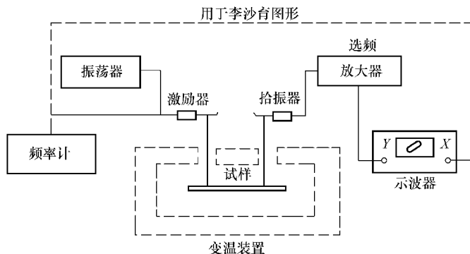
图 2-74 共振检测装置方框图
