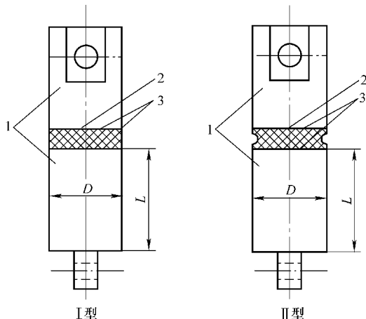
图 2-115 试样组合件
