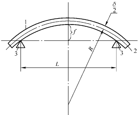
图 8-28 挠度的测量
