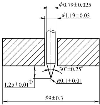
图 3-36 邵氏 AM 型硬度计压针 ① 压针伸出量对应硬度计读数为 0。
