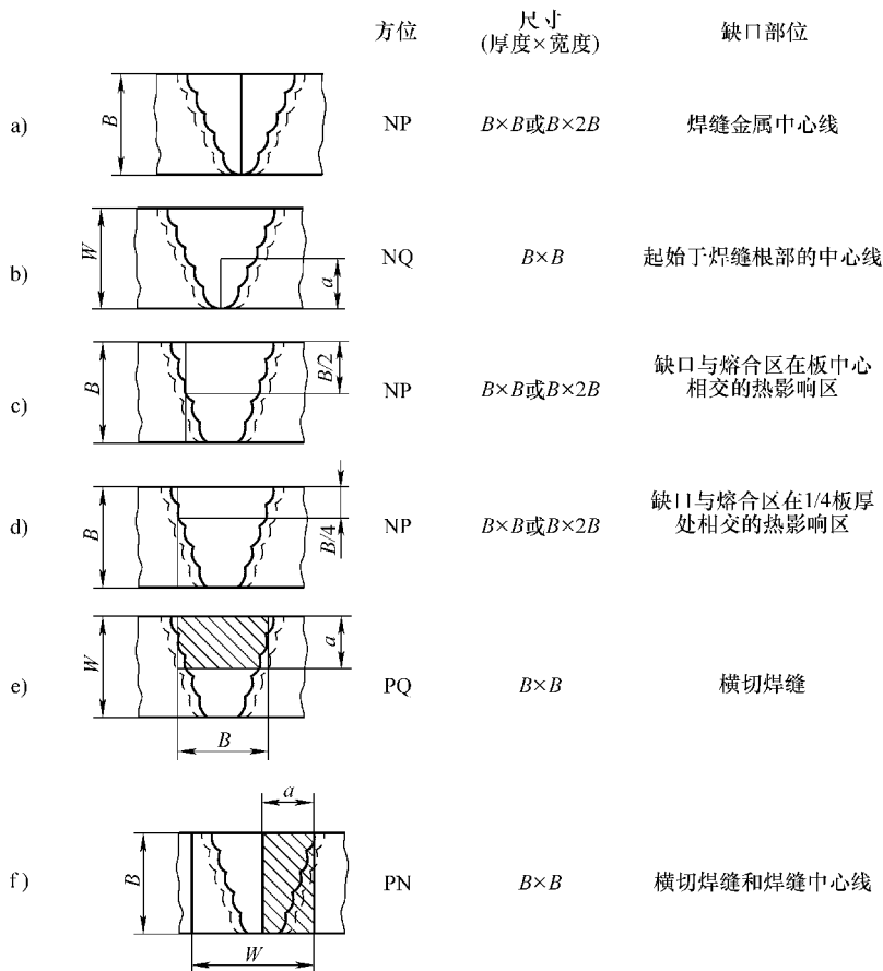
图 9-37 WP 试样缺口位置示例
