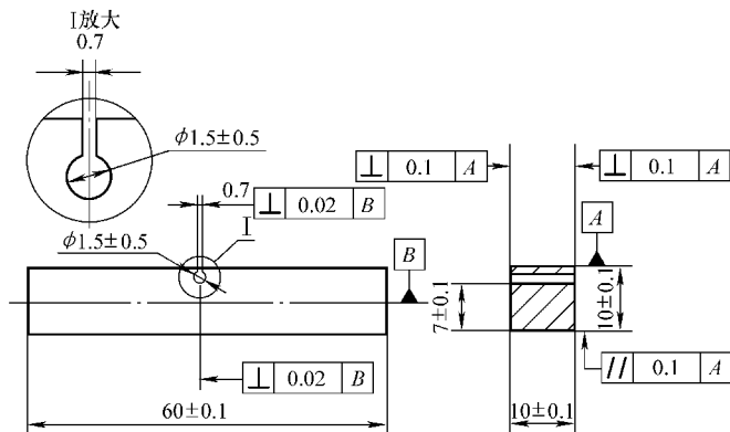
图 4-38 辅助试样
