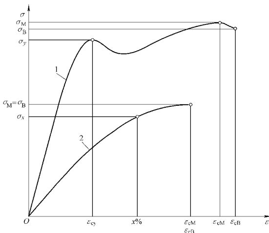
图 7-20 典型的应力-应变曲线
