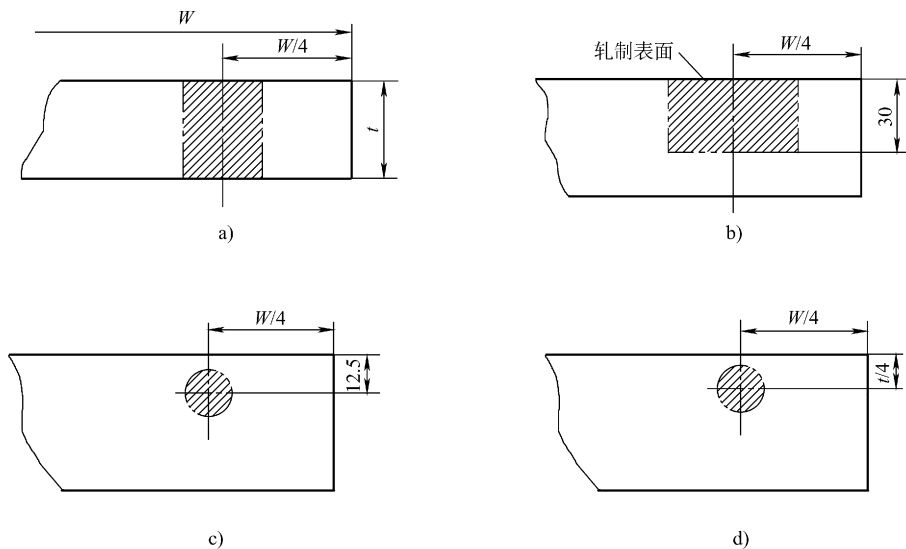
图 1-13 在钢板上截取拉伸样坯的位置
