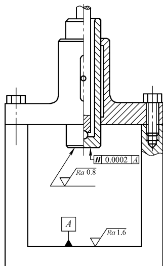
图 7-6 力导向装置
