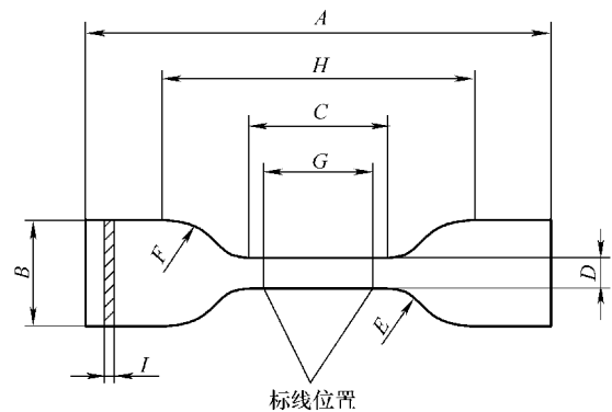
图 2-119 冲裁试样（类型 2）
