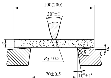
图 4-29 标准试样的冲击刀刃和支座
