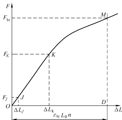
图 7-12 图解法求 F_{tc}
