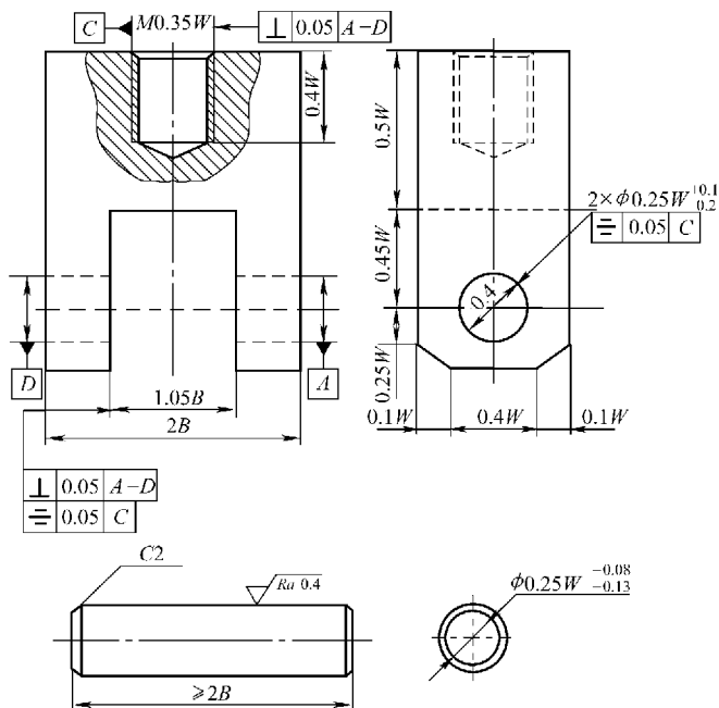
图 10-30 C (T) 试样 U 形夹具和销钉图
