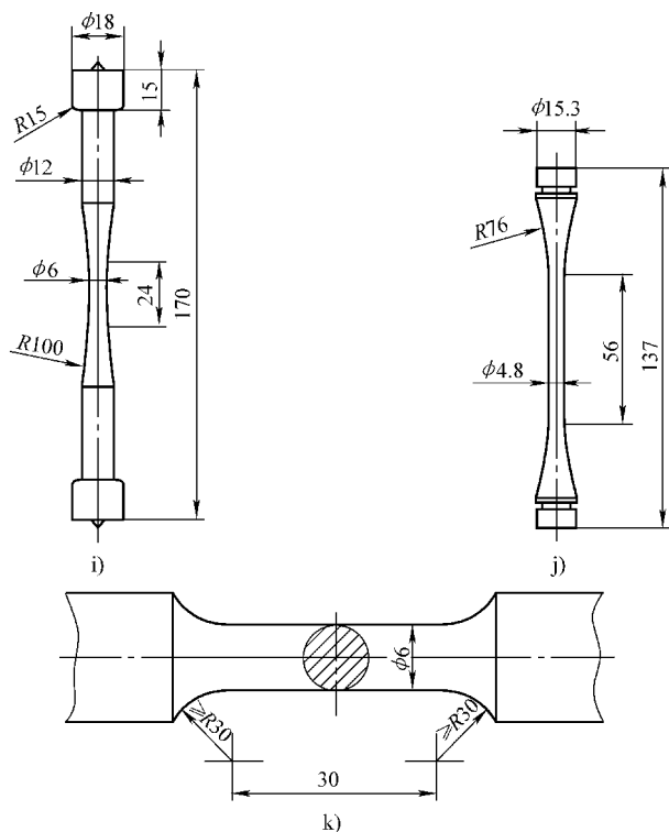
图 2-149 常用的试样形状和尺寸 (续)
