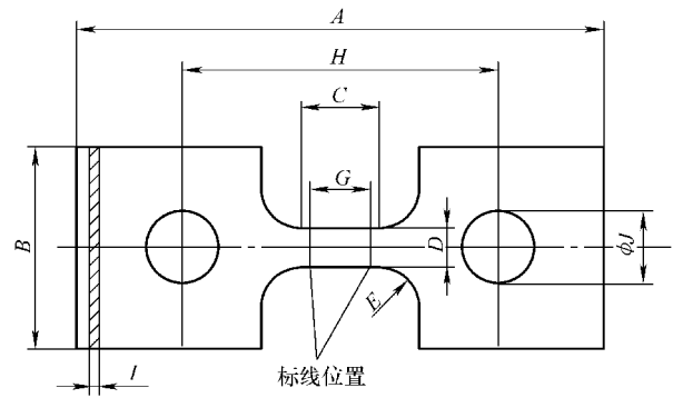
图 2-122 类型 3 试样
