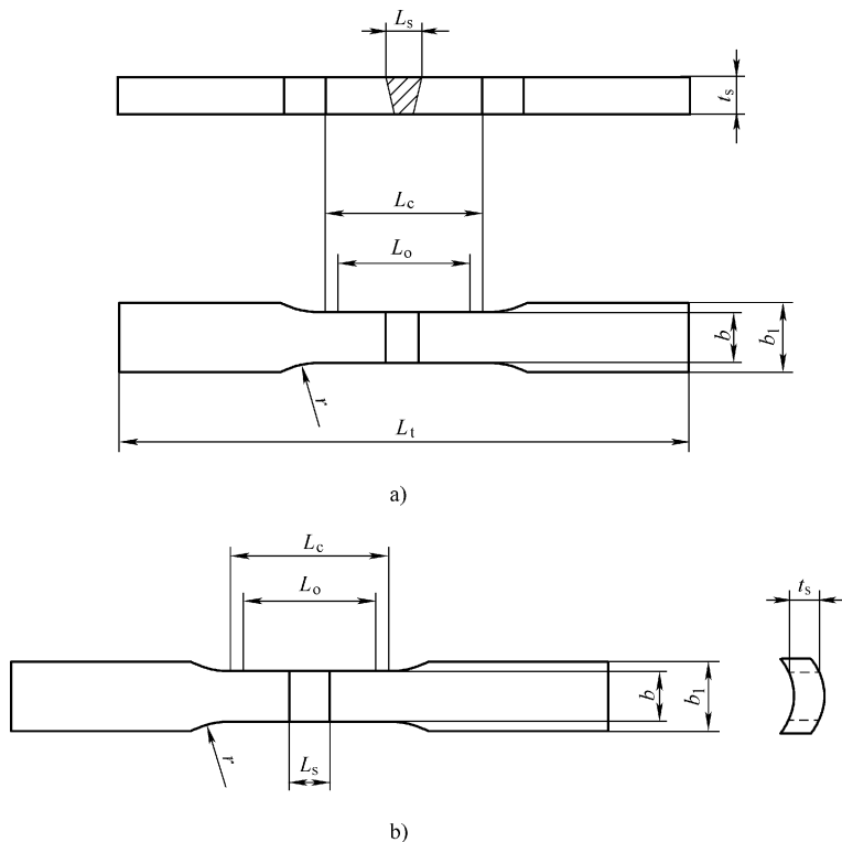
图 2-54 板和管接头板状试样
