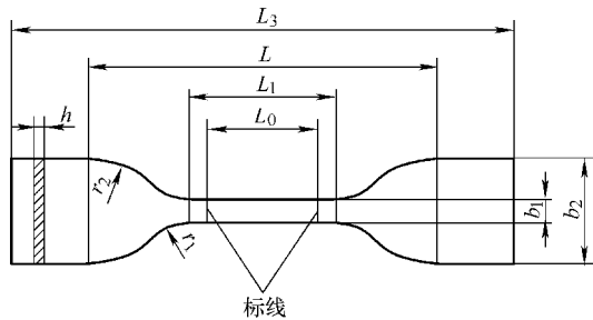
图 2-84 5 型试样
