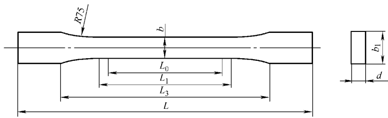
图 2-101 I 型试样
