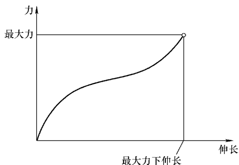
图 2-135 拉伸最大力
