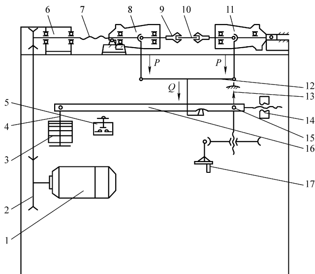
图 10-23 旋转弯曲疲劳试验机的原理图
