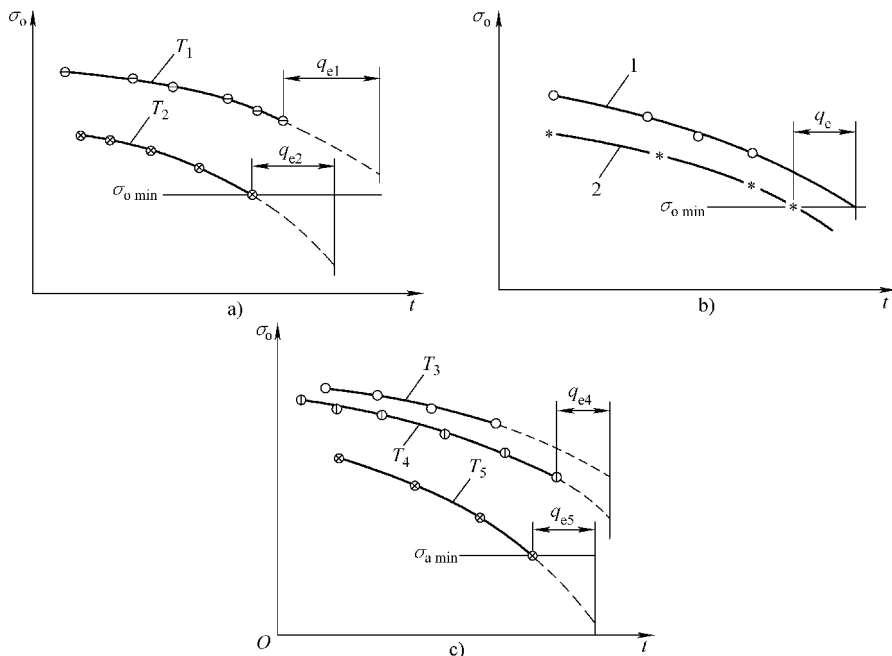
图 2-52 蠕变应变（断裂）图解法外推示例
