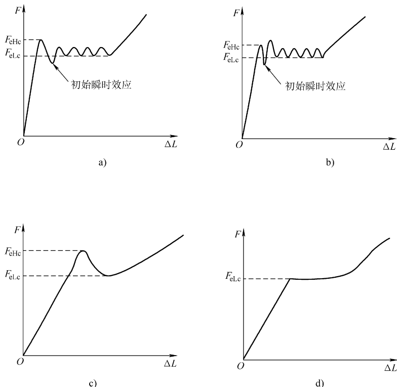
图 7-13 图解法求 F_{eHc} 和 F_{eLc}
