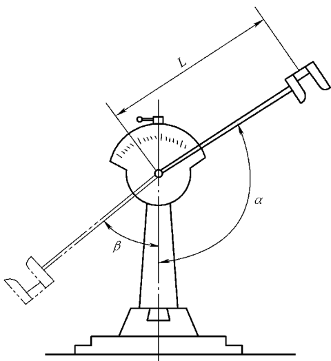
图 4-16 试验原理图
