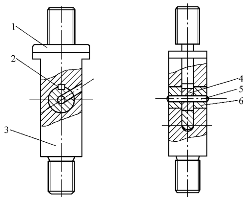
图 6-5 高温剪切夹具
