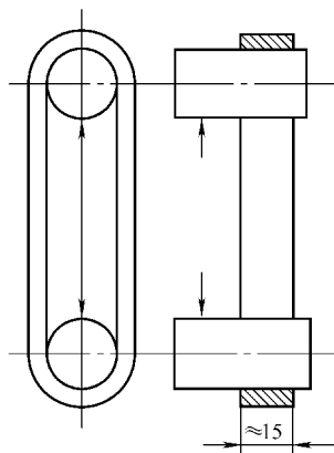
图 2-64 试验装置示意图
