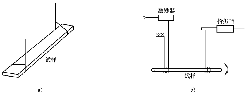
图 2-75 用于弯曲共振与扭转共振的悬丝耦合方法
