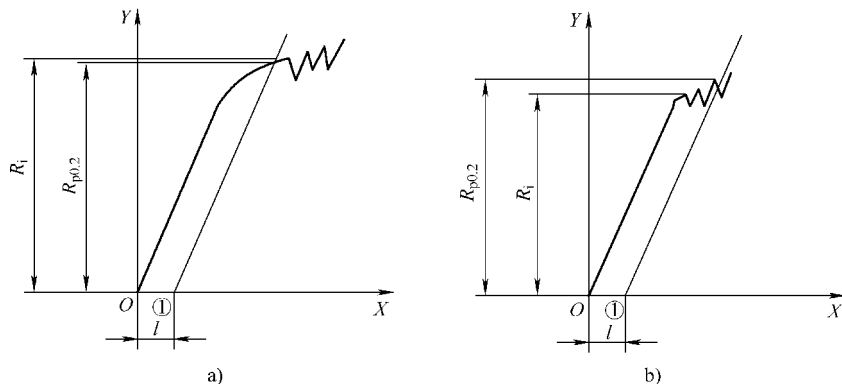
图 2-39 应力-应变曲线图
