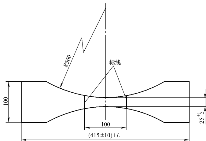
图 2-145 B 型试样
