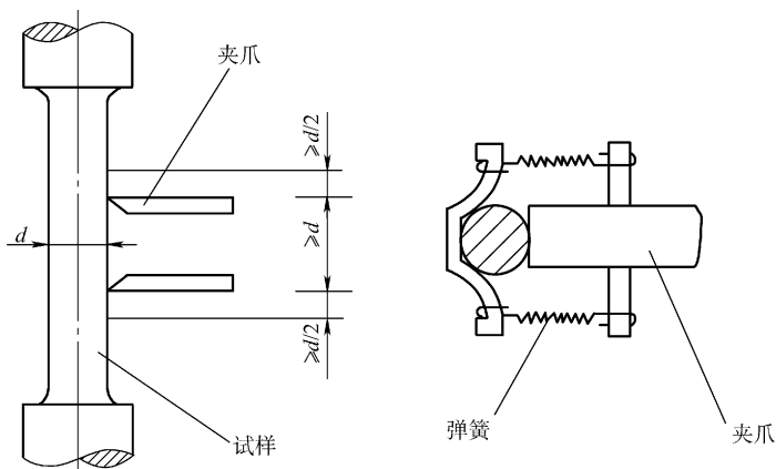
图 10-39 轴向应变引伸计
