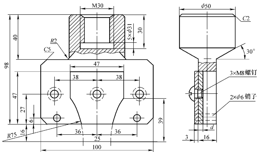
图2-105 III型试样使用的夹具
