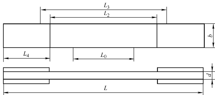
图 2-102 II 型试样
