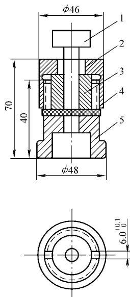
图 6-21 剪切夹具
