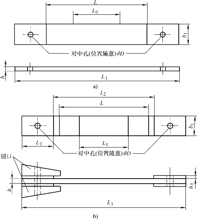
图 2-87 2 型试样和 3 型试样的形状
