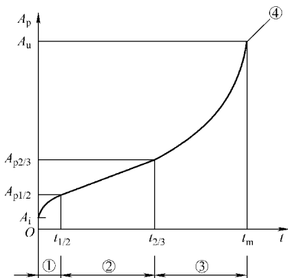
图 2-51 线性坐标的蠕变示意图
