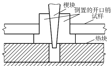
图 9-20 在较高温度下测定试样止裂韧度加载装置的截面图
