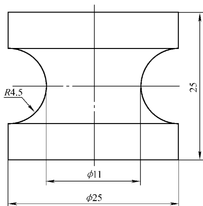
图 2-114 III 型试样
