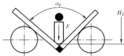
图 8-57 试样最终弯曲角及最终挤压位移示意图
