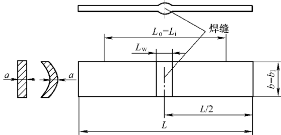
图 2-110 板材、管材拉伸试验矩形试样 L —试样总长度 (mm) L_0 —原始标距 (mm) L_i —带过渡弧试样长度 (mm) L_w —焊缝宽度 (mm) a —试样厚度 (mm) b —平行长度部分宽度 (mm) b_1 —夹持端宽度 (mm)
