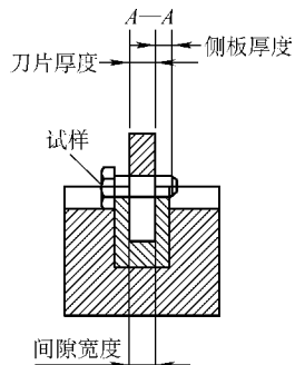
图 6-2 双剪切试验夹具刀口形状
