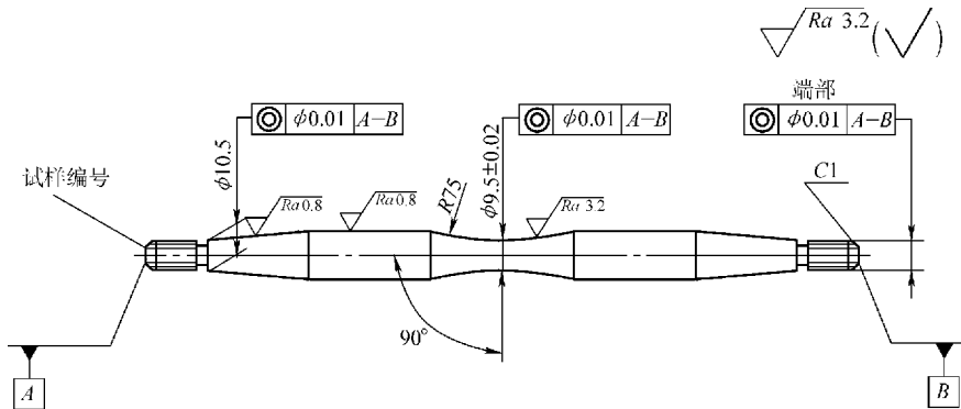
图 10-22 圆弧形光滑试样
