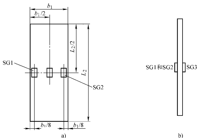
图 2-91 用于对中校核系统应变片 (SG1、SG2 和 SG3) 的位置
