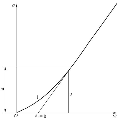
图 8-46 带有曲线起始部分和测定零应变点的应力-应变曲线示例
