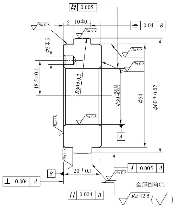
图 10-5 JP-1 试样
