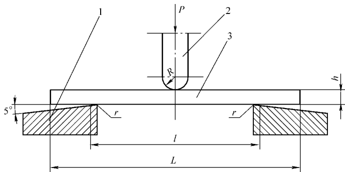
图 8-48 弯曲试验装置
