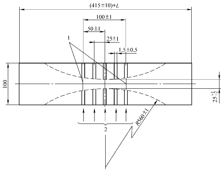
图 2-147 D 型试样
