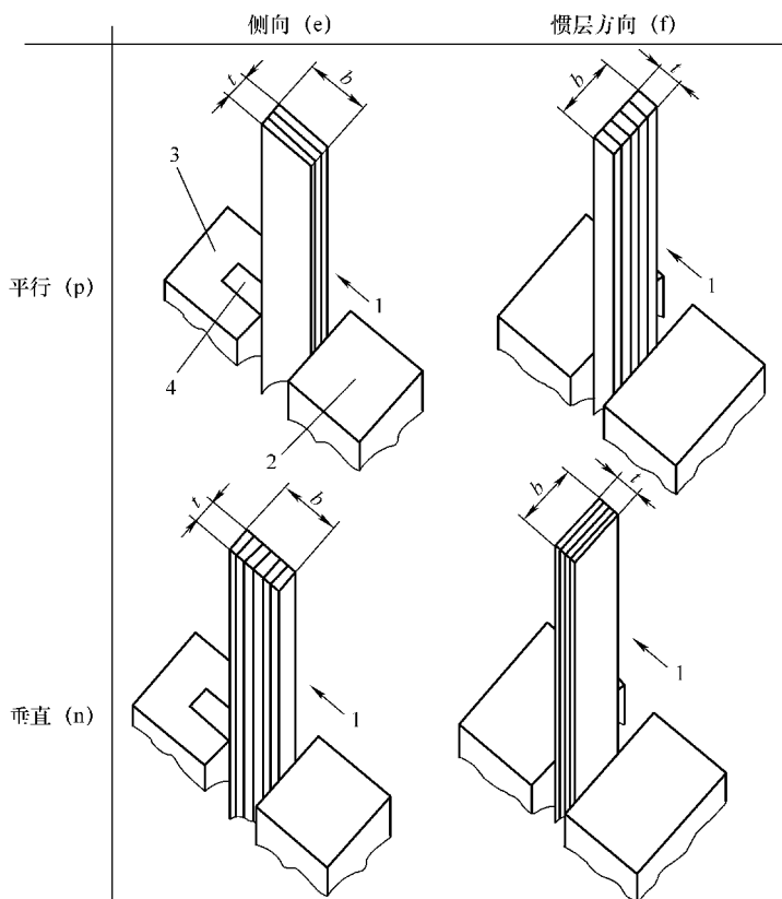
图 4-21 冲击方向的命名图
