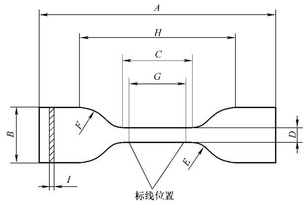
图 2-121 类型 2 试样
