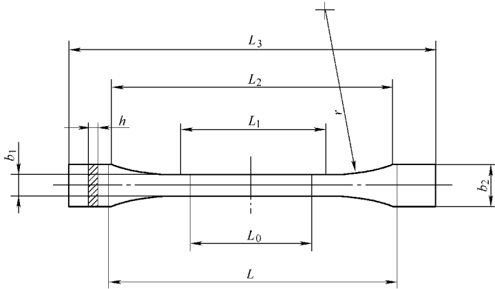
图 2-80 1A 型和 1B 型试样的形状
