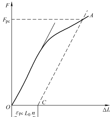
图 7-10 图解法求 F_{pc}
