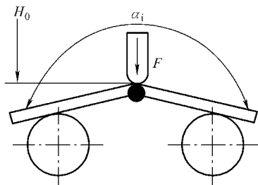
图 8-56 试样原始弯曲角及挤压位移示意图
