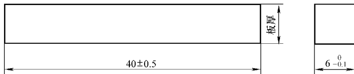
图 6-19 纤维增强塑料板材试样
