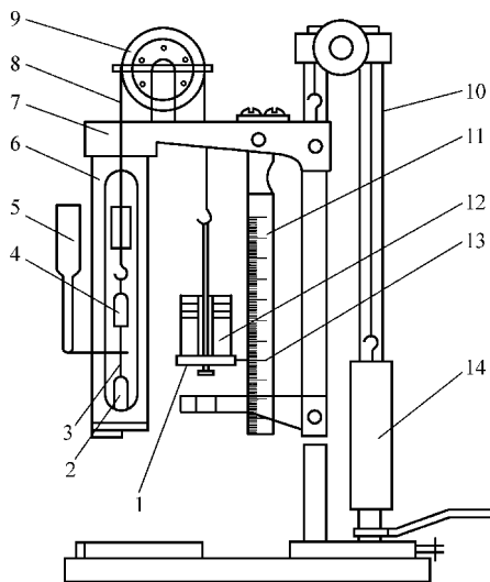
图 2-132 拉伸与测量装置
