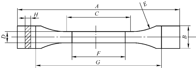
图 2-120 类型 1 试样
