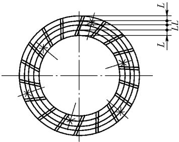
图 3-39 离合器面片
