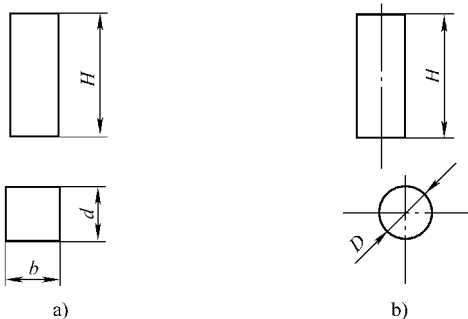
图 7-21 试样的形状
