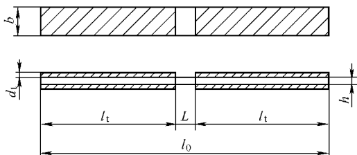
图 7-25 试样的形状
