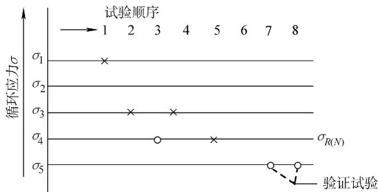
图 10-11 第一种情况的试验顺序
