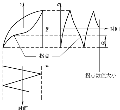
图 10-41 确定失效拐点的定义
