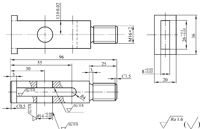
图 6-8 夹板
