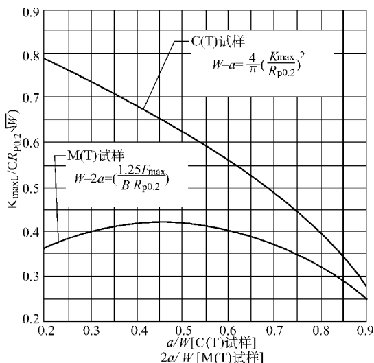
图 10-28 C (T) 和 M (T) 标准试样尺寸标准化曲线图
