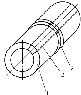
图 8-51 管材焊接弯曲试样取样立体示意图 1—焊件 2—所取的试样 3—焊缝
