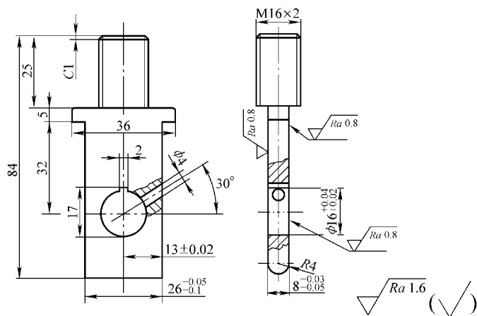
图 6-6 切刀
