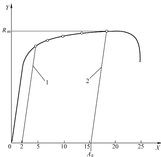
图 2-66 n_{2-20/A_g} 或 n_{2-A_g} 应变取值范围
