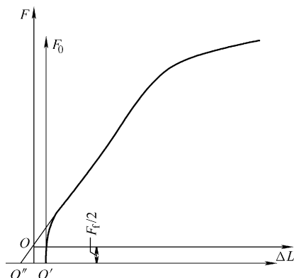
图 7-9 图解法确定实际压缩力
