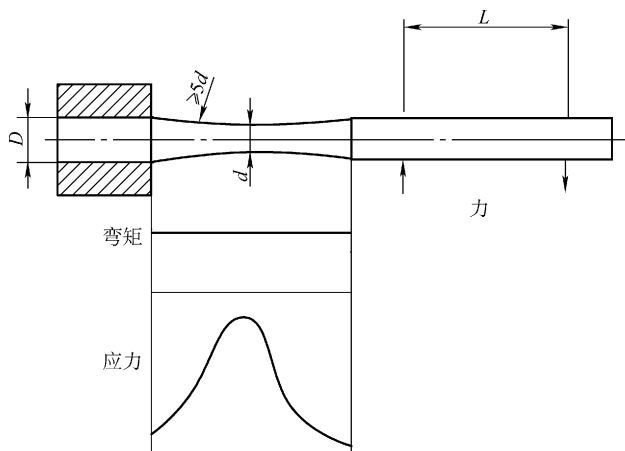
图 10-19 漏斗形试样 (两点加力)
