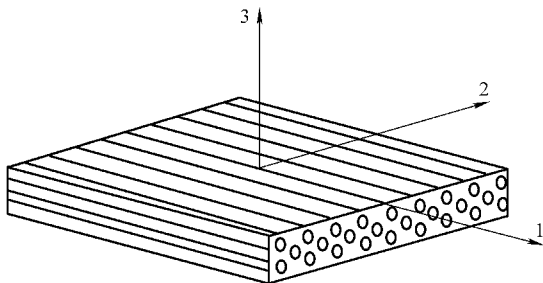
图 2-88 各向同性和正交各向异性纤维增强复合材料试样的坐标轴
