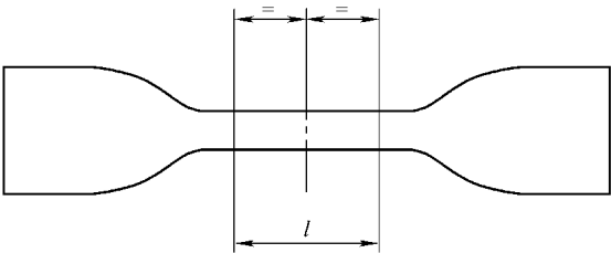
图 2-127 哑铃状试样 l —试验长度
