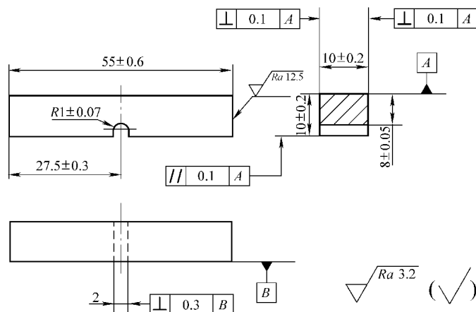
图 4-18 U 型缺口试样
