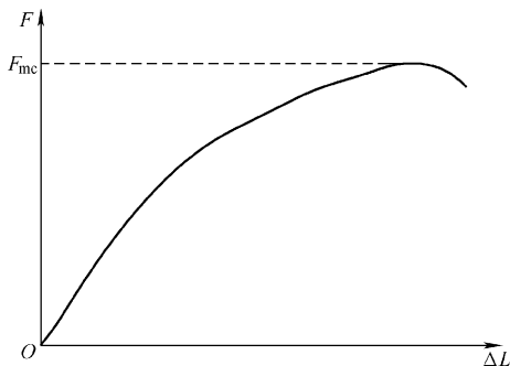
图 7-14 图解法求 R_{mc}
