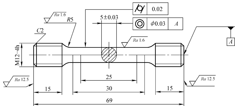
图 2-33 第 3 类低温拉伸试样
