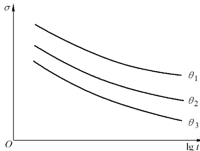
图 2-97 蠕变破裂曲线
