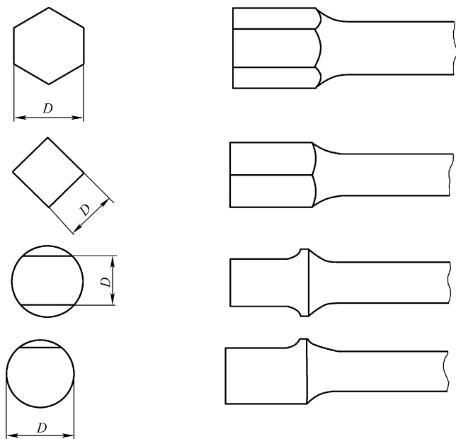
图 10-2 试样典型夹持端
