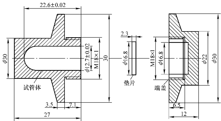
图 4-41 试样管
