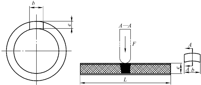
图 8-52 平行面取样和受力方向
