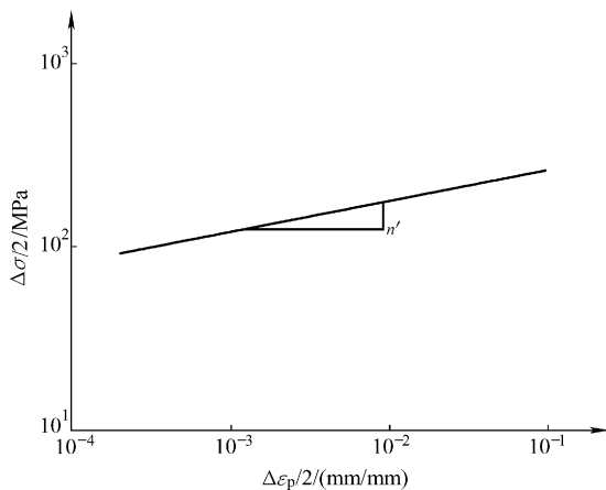
图 10-36 \Delta\sigma/2 - \Delta\varepsilon_p/2 曲线
