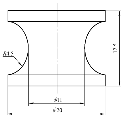
图 2-113 II 型试样
