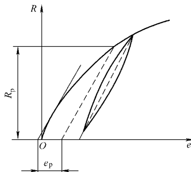
图 2-18 规定塑性延伸强度 R_p
