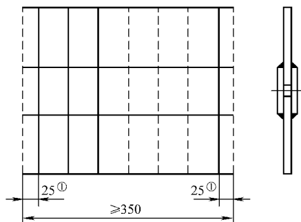
图 2-59 搭接接头的取样部位
