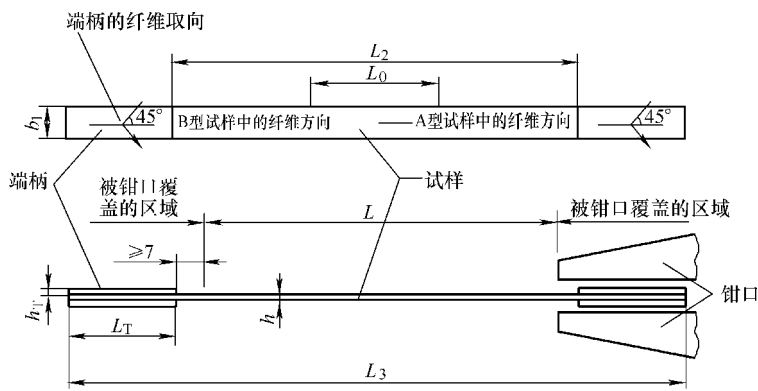
图 2-90 单向纤维增强复合材料试样
