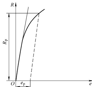
图2-4 规定塑性延伸强度( R_p )
