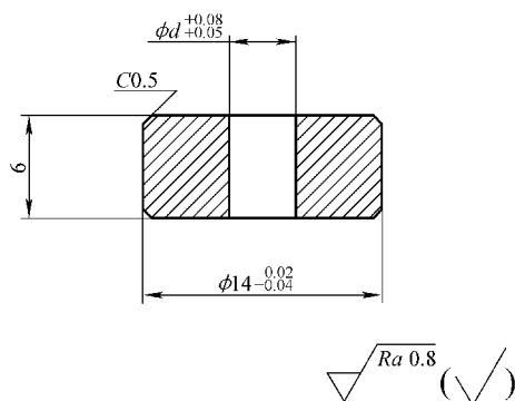
图 6-10 支承圈
