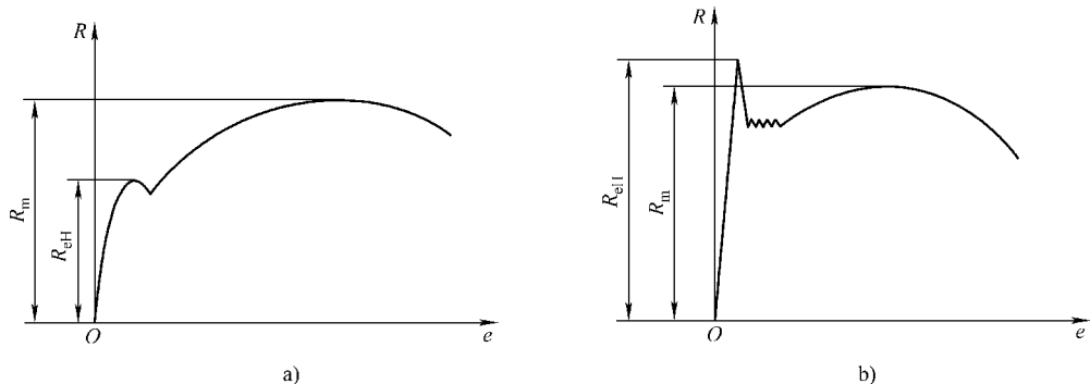
图 2-17 从应力-延伸率曲线测定抗拉强度
