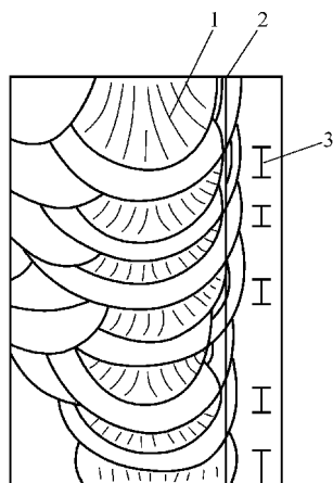
图 9-49 在宏观金相切面上紧邻柱状焊缝金属的 HAZ 理想缺口线
