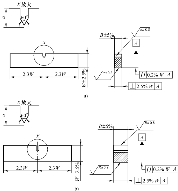
图 9-42 弯曲试样的尺寸及所允许的尺寸公差
