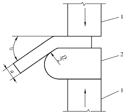
图 8-11 台虎钳式弯曲装置
