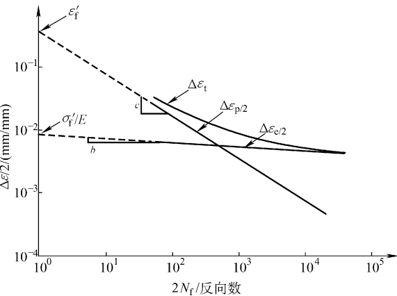
图 10-33 \Delta\varepsilon_t = \Delta\varepsilon_e + \Delta\varepsilon_p 状态 \Delta\varepsilon_t/2-2N_f 曲线
