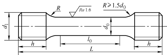
图 1-27 球墨铸铁拉伸试样
