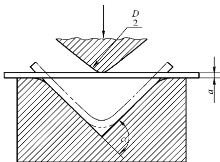
图 8-10 V 形模具式弯曲装置
