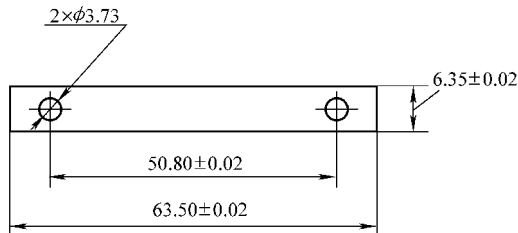
图 5-8 试样的尺寸
