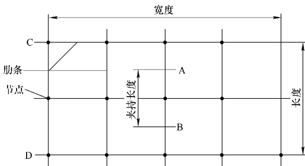
图 2-139 典型土工格栅
