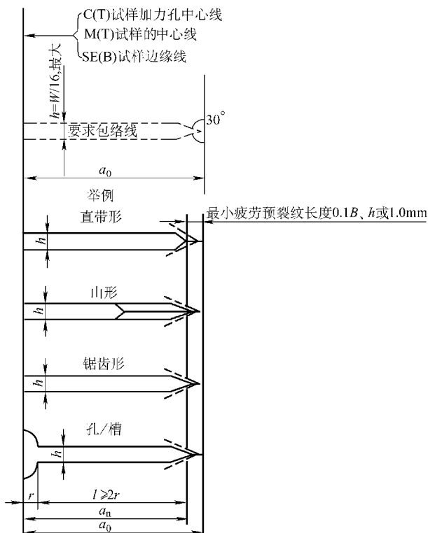
图 10-29 切口详图及最小疲劳预裂纹长度的要求
