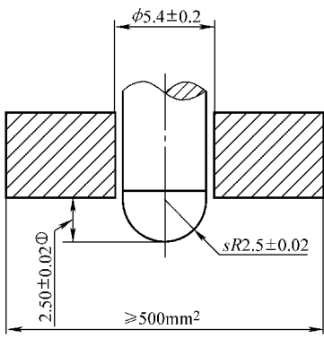
图 3-35 邵氏 AO 型硬度计压针 ① 压针伸出量对应硬度计读数为 0。
