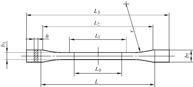
图 2-81 1BA 型和 1BB 型试样的形状
