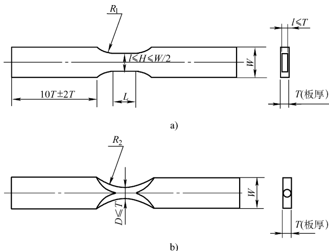
图 10-38 低循环疲劳板材试样
