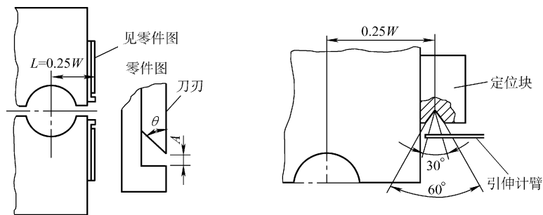
图 9-21 借助刀口和定位块的两端引伸计的安装方式
