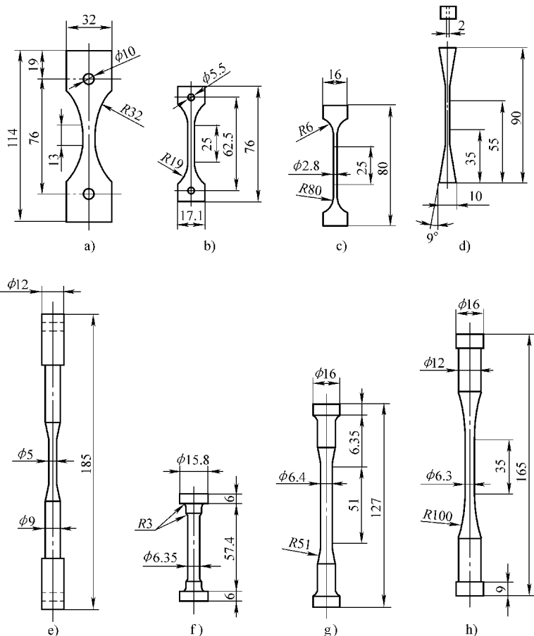
图 2-149 常用的试样形状和尺寸
