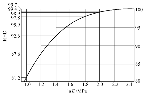
图 3-32 \lg E 和国际硬度 (80 ~ 1000IRHD) 之间的关系
