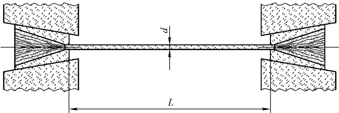
图 2-79 浇铸法试样
