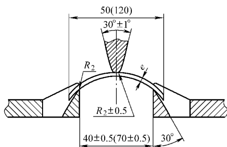
图 4-31 弧形试样的冲击刀刃和支座
