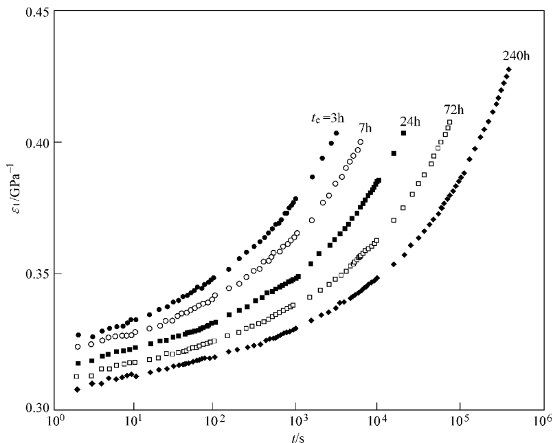
图 2-98 由 85℃ 迅速降温至 23℃ 并恒温 t_e 的 PVC 物理老化试样的蠕变曲线
