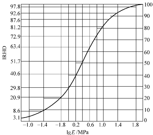
图 3-30 \lg E 和国际硬度 (3 ~ 100IRHD) 之间的关系
