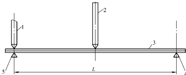
图 8-23 热双金属温曲率试验装置
