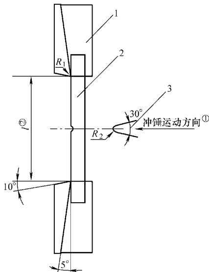
图 4-28 试验机主要尺寸
