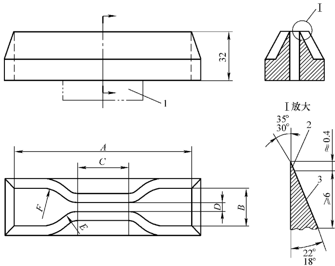
图 2-128 哑铃状试样用的裁刀 1—固定在配套机器上的刀架头 2—需研磨 3—需抛光
