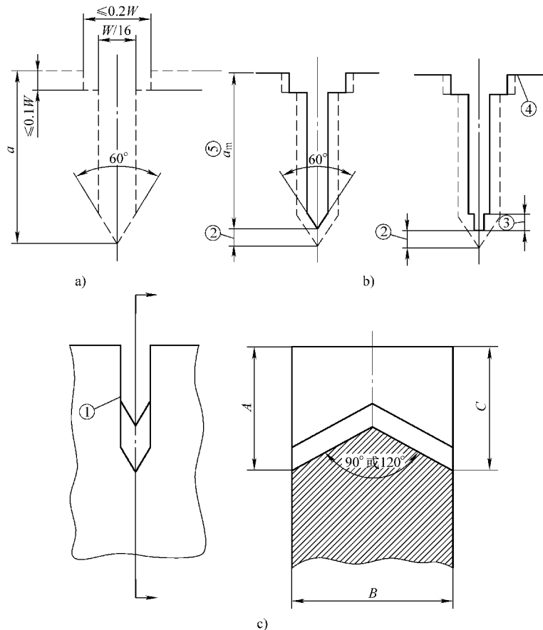
图 9-27 疲劳裂纹包迹和裂纹引发缺口
