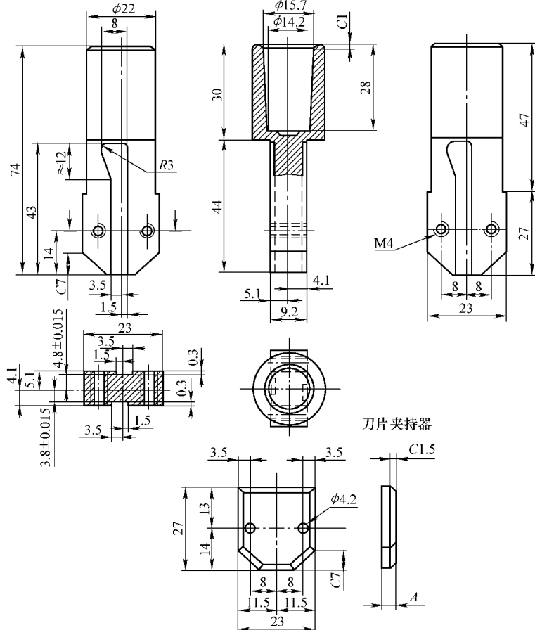
图 2-129 可拆装刀具的专用夹持工具
