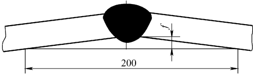
图 1-19 焊接试板挠度 f 示意图
