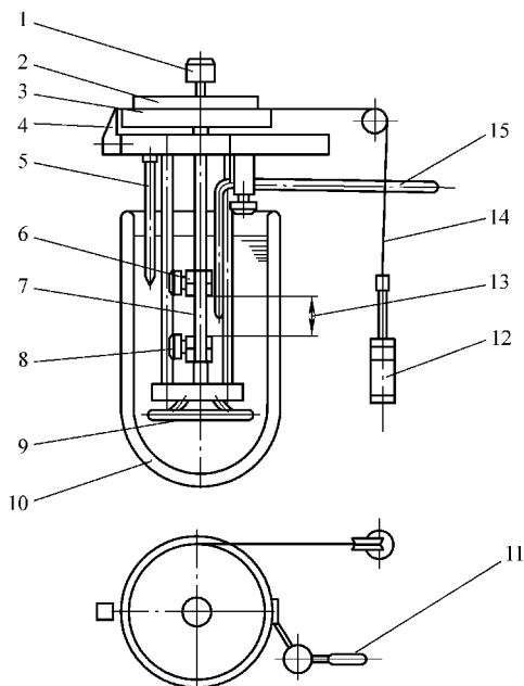
图 5-9 扭转试验机
