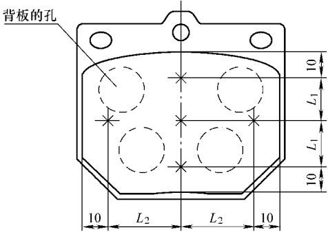
图 3-38 盘式制动器衬片
