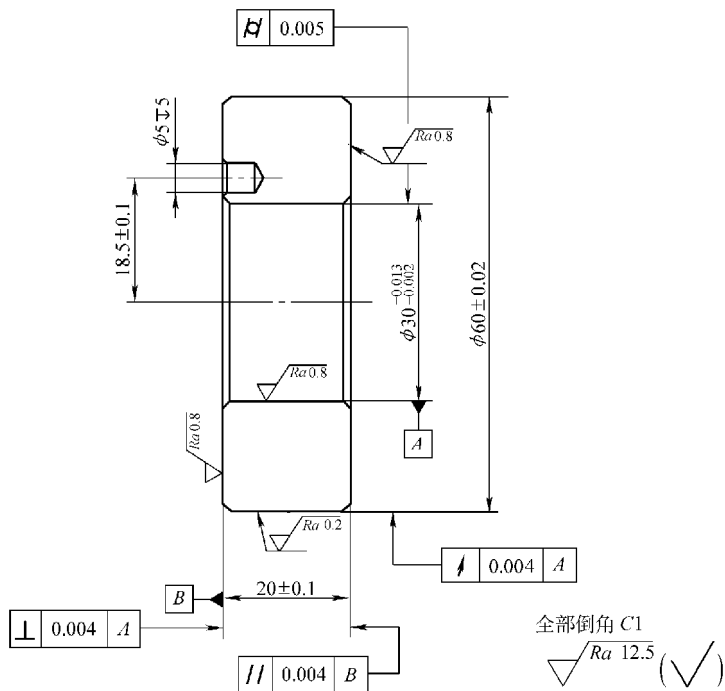
图 10-9 PS-1 试样
