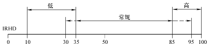
图 3-29 硬度测试的应用范围
