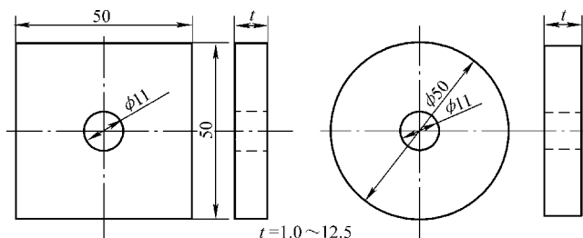
图 6-15 剪切试样
