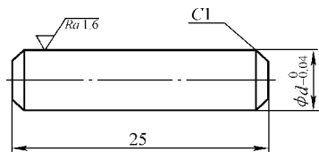
图 6-4 剪切试样
