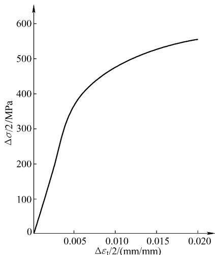
图 10-35 循环应力-应变曲线
