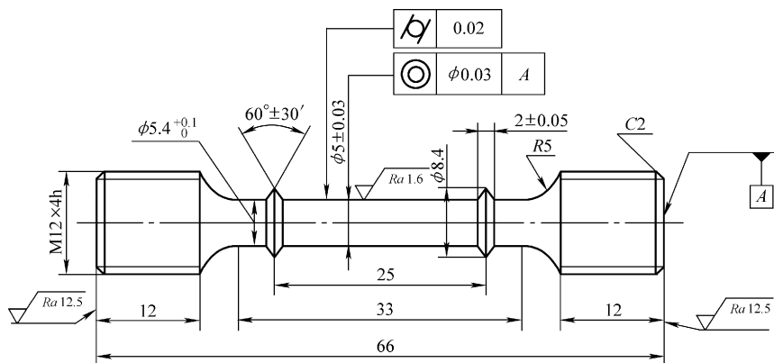
图 2-32 第 2 类低温拉伸试样
