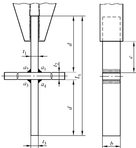
图 2-58 十字接头试样的尺寸
