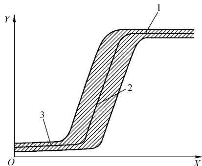
图 4-7 冲击吸收能量-温度曲线示意图
