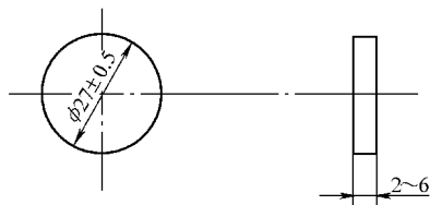
图 6-20 短切纤维增强塑料剪切试样
