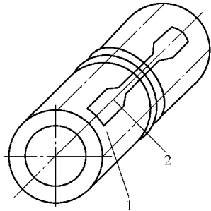
图 2-109 管材取样方法 1—试件 2—所取的试样
