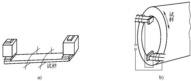
图 2-77 电磁耦合方法 a) 弯曲共振用耦合 b) 扭转共振用耦合
