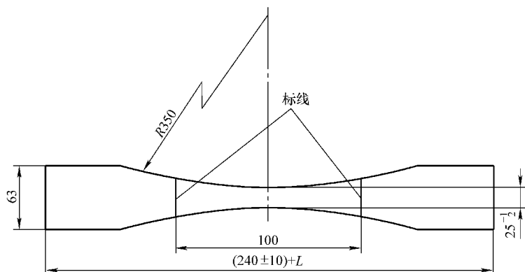
图 2-146 C 型试样
