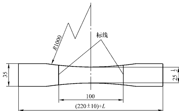
图 2-144 A 型试样
