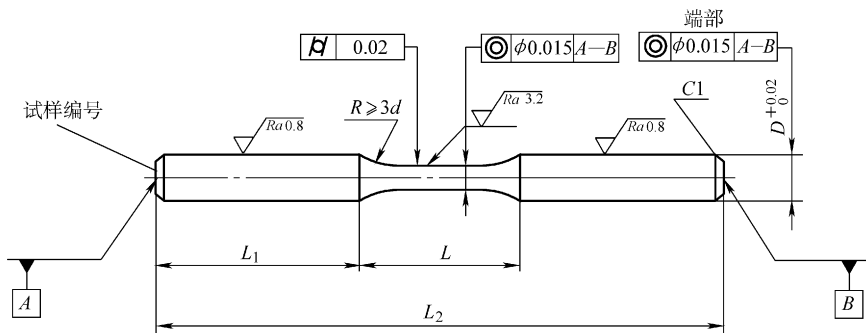
图 10-21 圆柱形光滑试样
