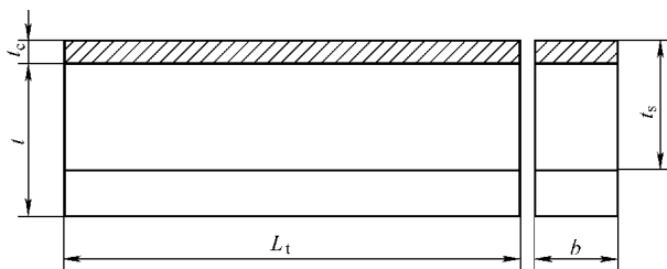
图 8-36 带堆焊层正弯试样
