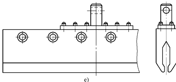
图 2-140 用于土工布拉伸试验的夹具示例 (续)
