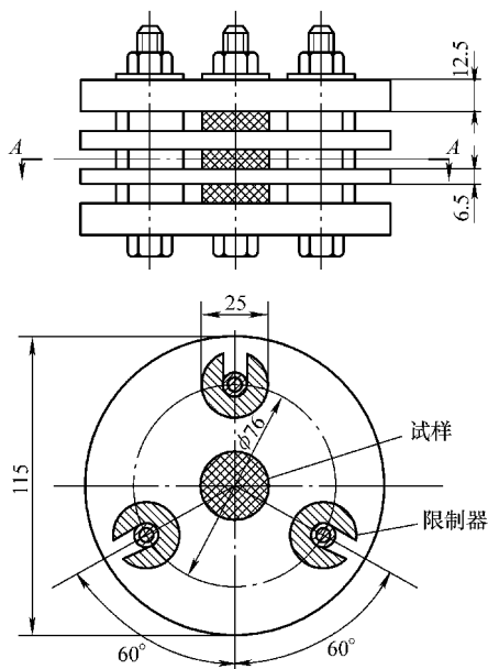
图 7-33 压缩装置
