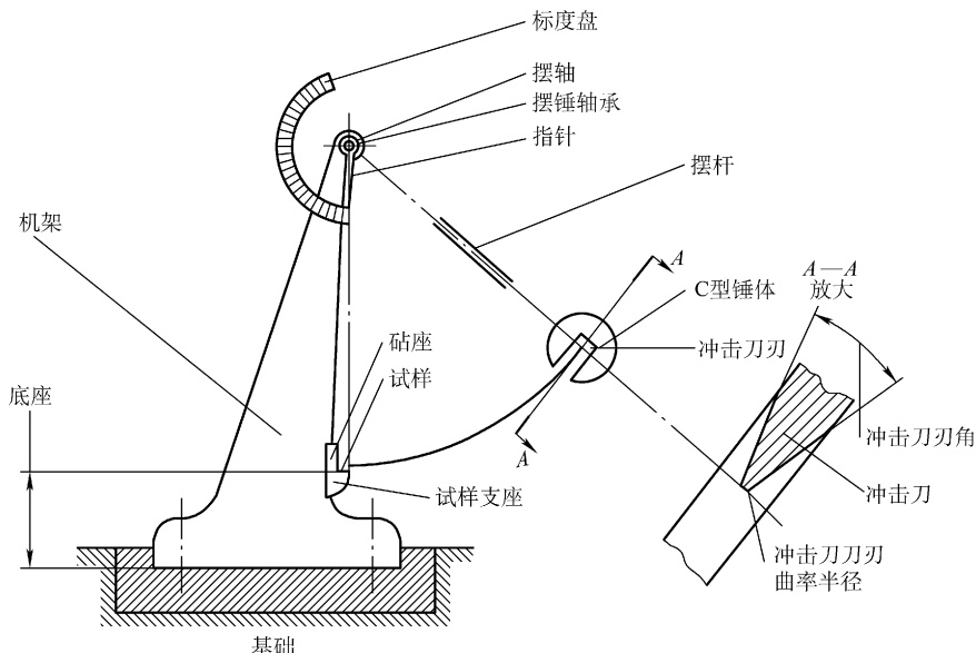
图 4-3 摆锤冲击试验机的组成部分
