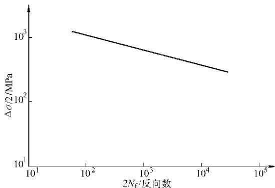
图 10-31 \Delta\sigma/2-2N_f 曲线
