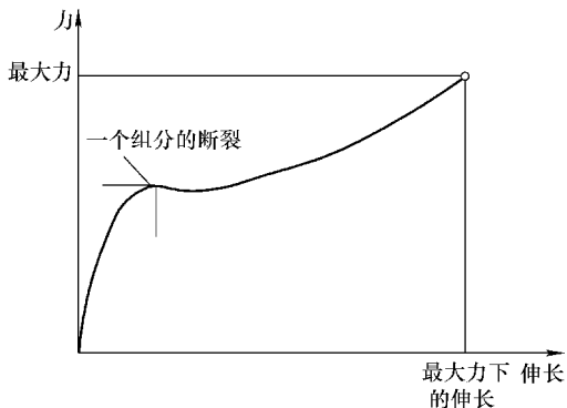
图 2-137 涂覆织物的一个组分的断裂
