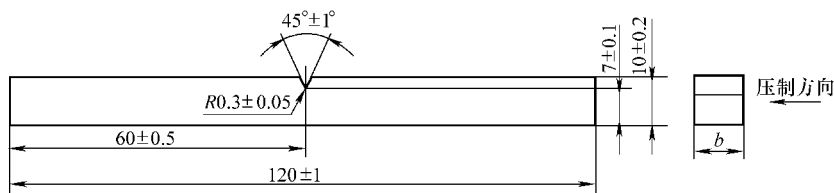
图 4-27 短切纤维增强塑料的试样
