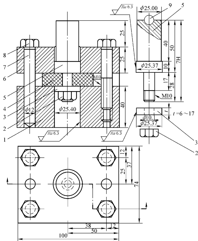
图 6-16 剪切夹具
