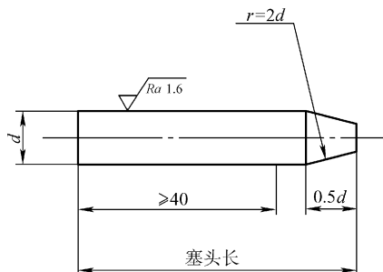
图 5-2 管形试样塞头
