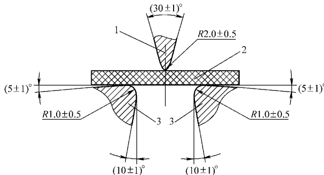
图 4-35 A 型试验机
