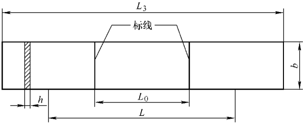
图 2-83 2 型试样
