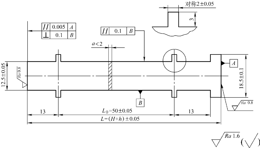
图 7-5 带凸耳板状试样
