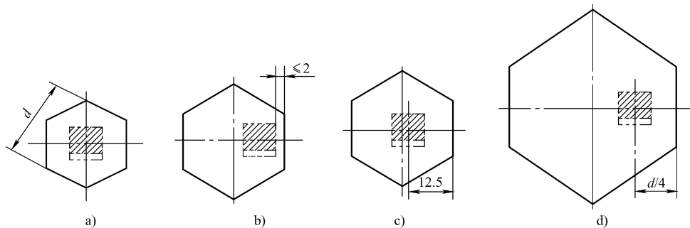
图 1-10 在六角钢上选取冲击样坯的位置
