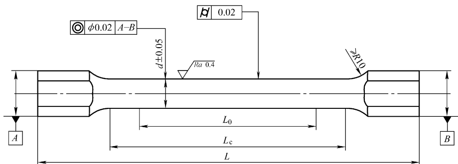
图 5-1 圆柱形试样
