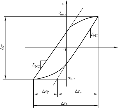
图 10-34 应力-应变迟滞回线
