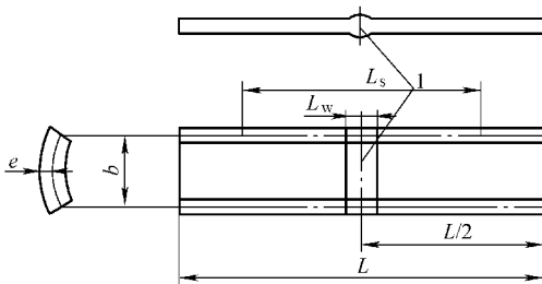
图 8-50 辐射面（管材）试样形状
