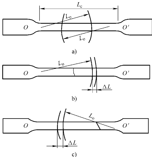
图 2-21 断后伸长率小于 5% 的测定方法
