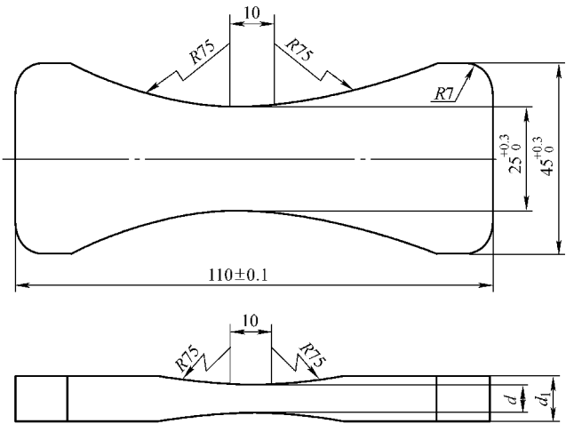
图 2-103 III 型试样
