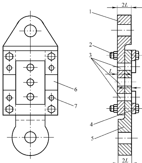
图 6-13 室温拉式单剪夹具
