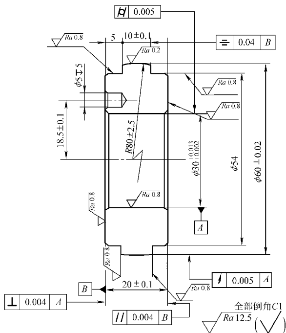
图 10-6 JP-2 试样
