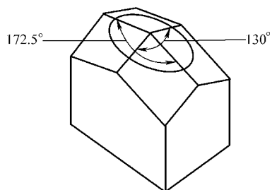
图 3-40 金刚石压头
