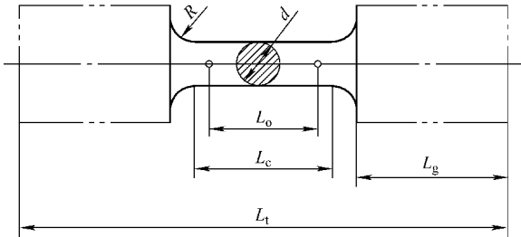
图 2-42 圆柱状试样的形状
