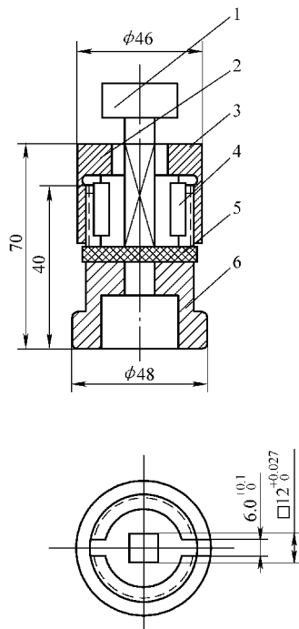
图 6-22 方柱冲头剪切夹具
