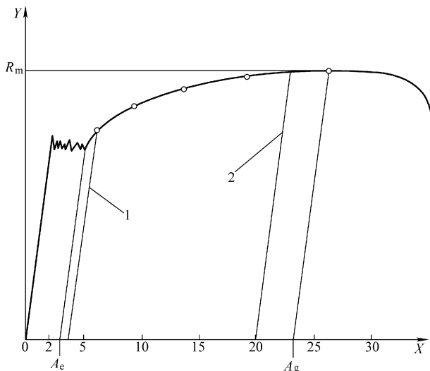
图 2-67 n_{4-20}/A_g 或 n_{4-20} 应变取值范围
