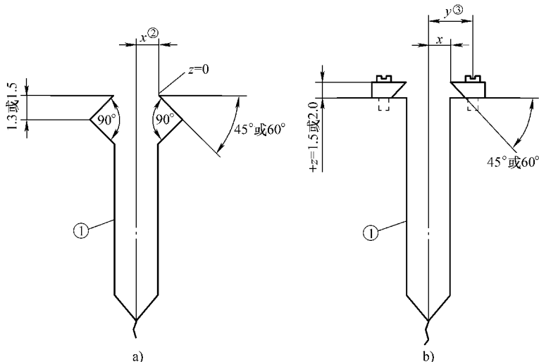
图 9-28 外置刀口和相应的缺口几何尺寸
