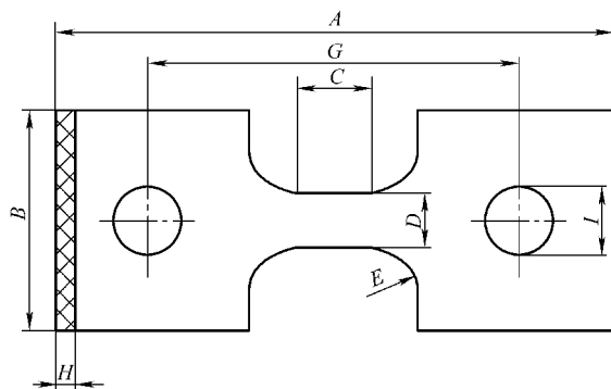
图 2-125 B 型试样
