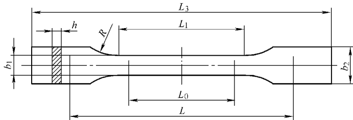
图 2-86 1B 型试样
