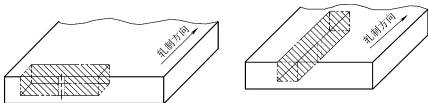
图 1-6 冲击试样缺口取向
