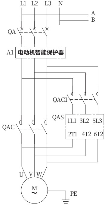
主电路
