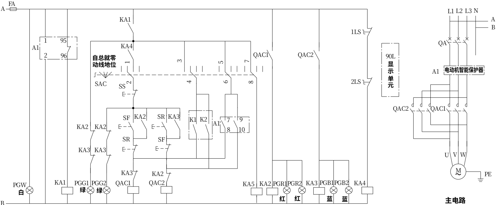
主电路
