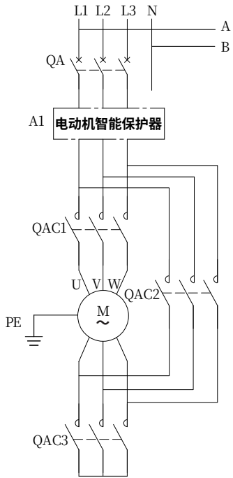
主电路
