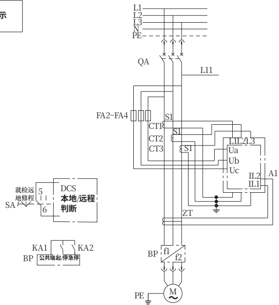
主电路
