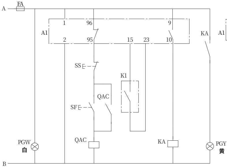
控制原理图
