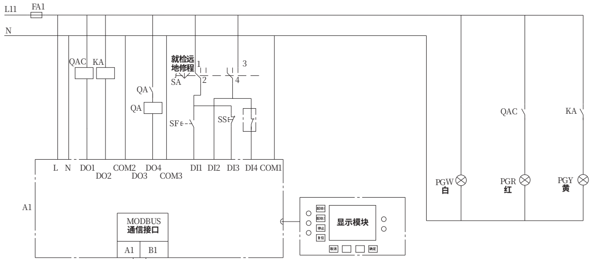
控制原理图
