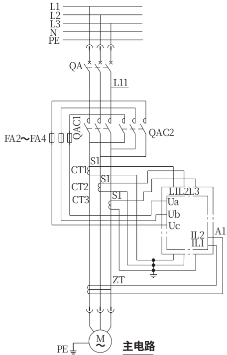
主电路
