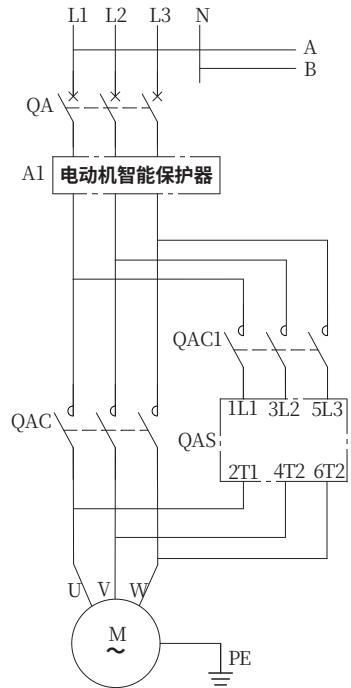
主电路
