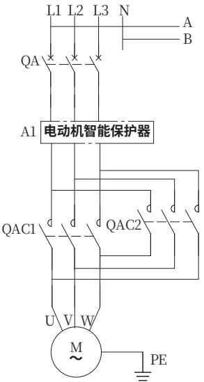
主电路
