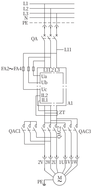
主电路
