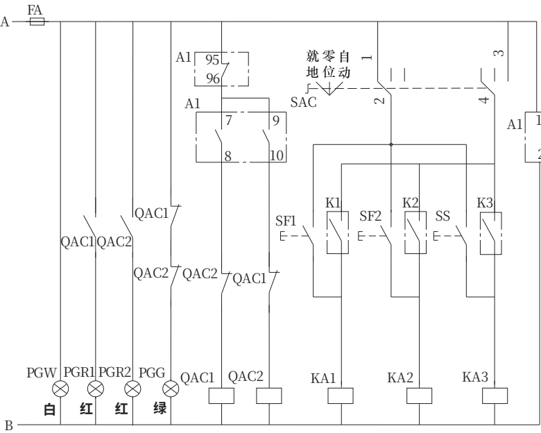
控制原理图
