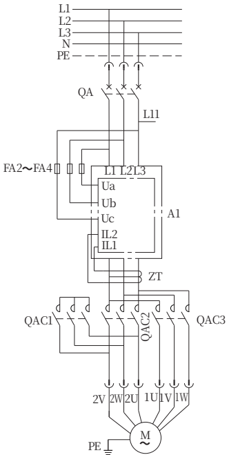
主电路
