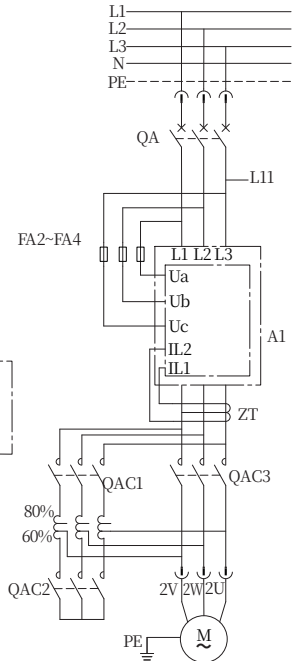
主电路
