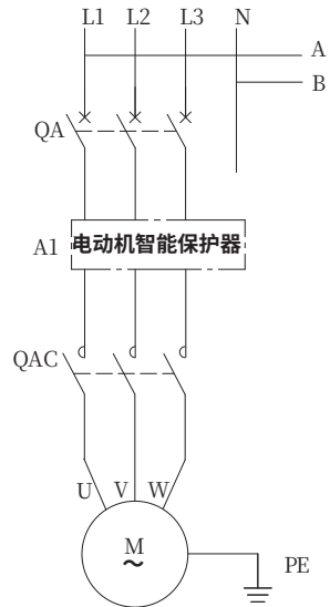
主电路
