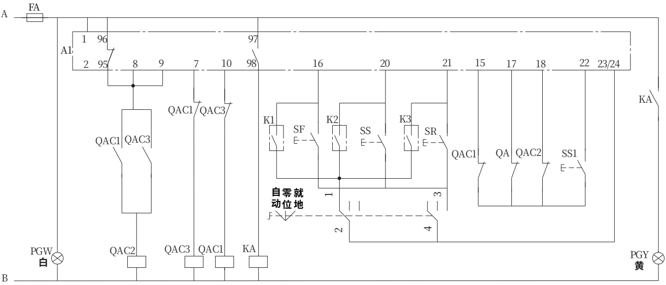
控制原理图
