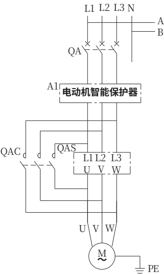
主电路
