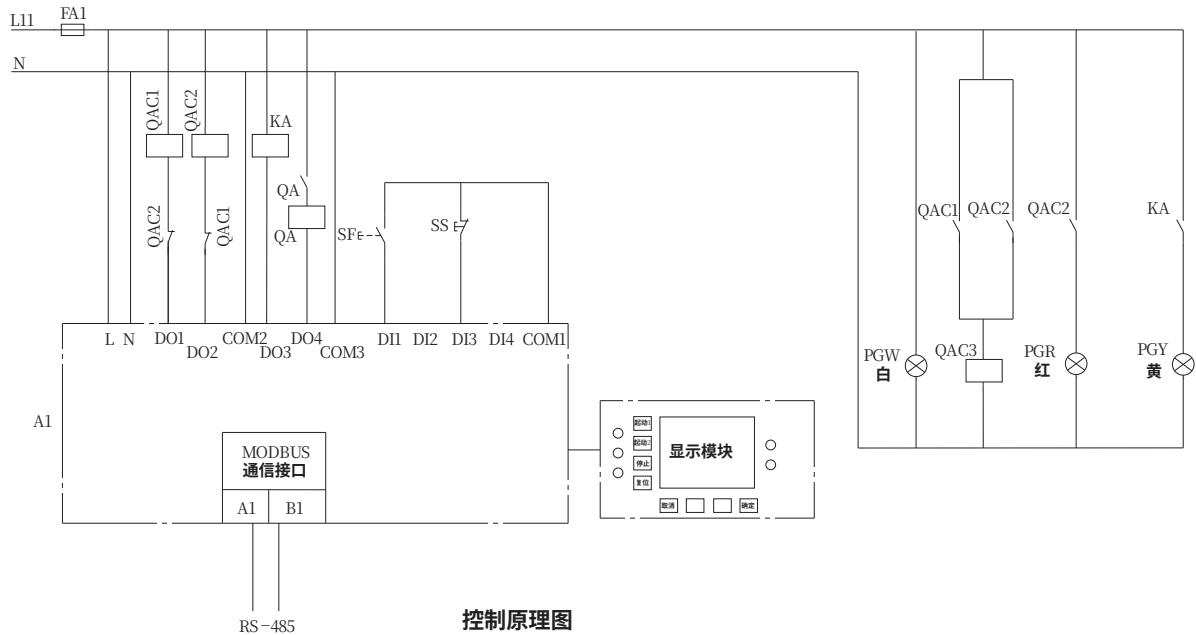
控制原理图
