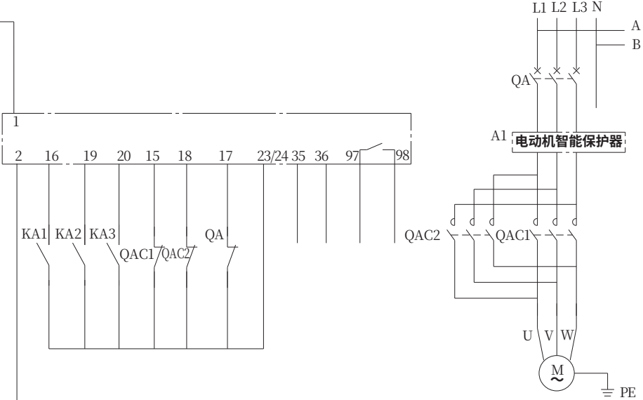
主电路
