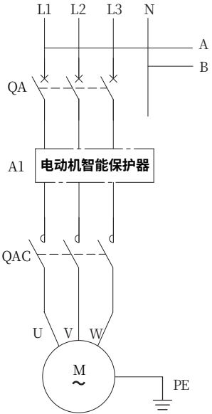
主电路
