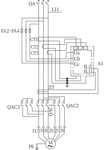
主电路
