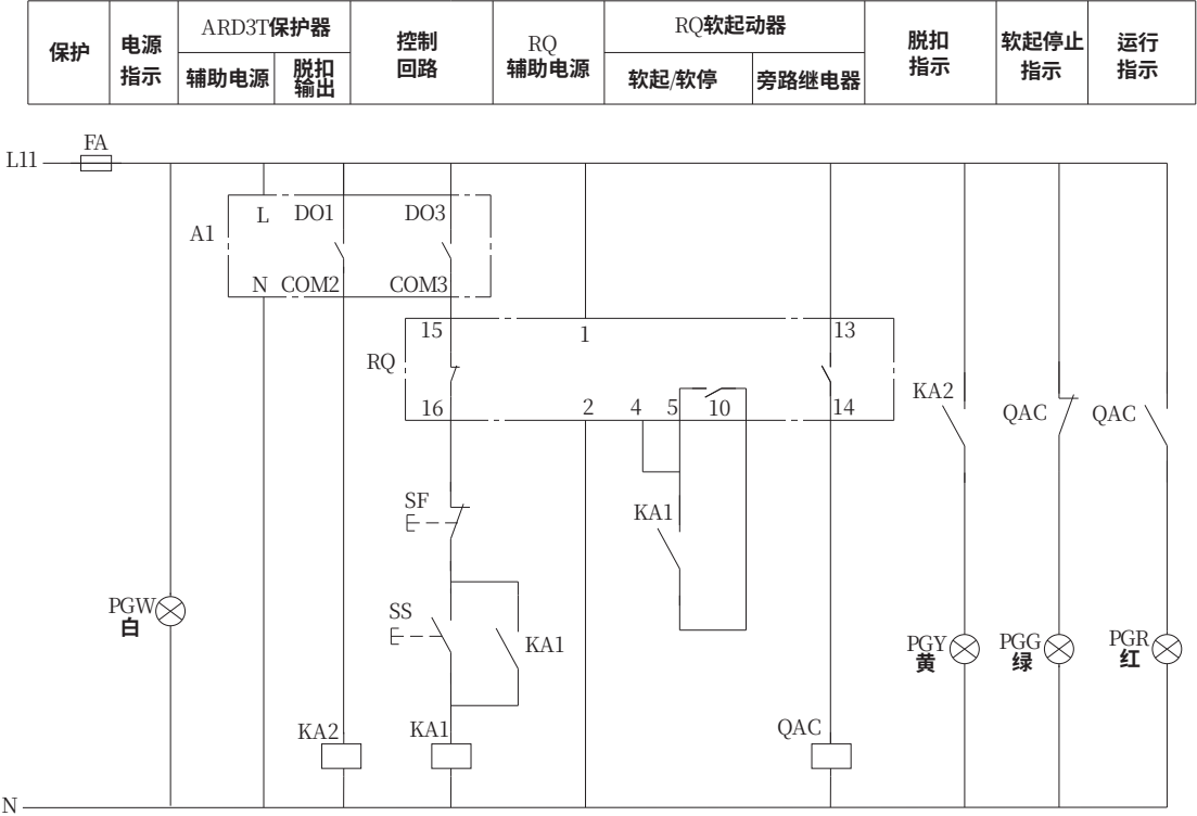
控制原理图
