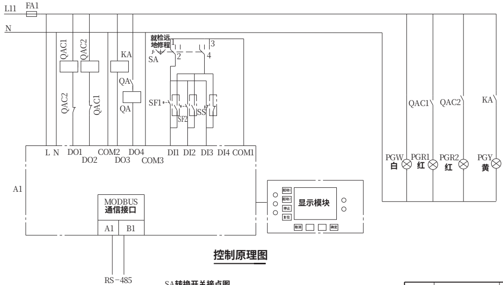
SA转换开关接点图
