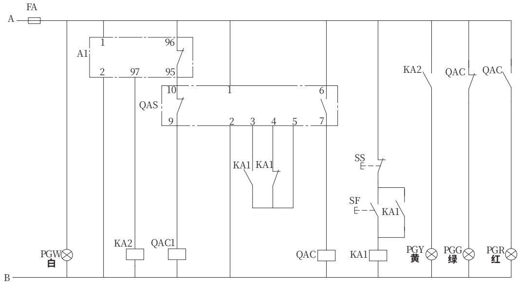
控制原理图
