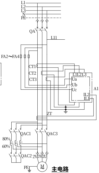
主电路
