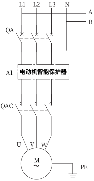
主电路
