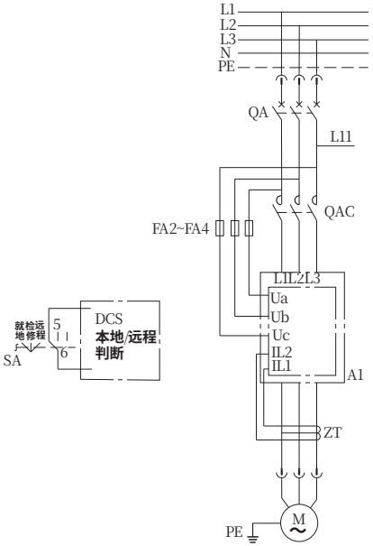
主电路
