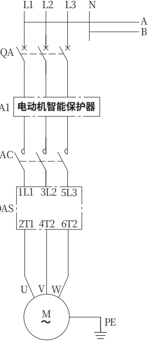
主电路
