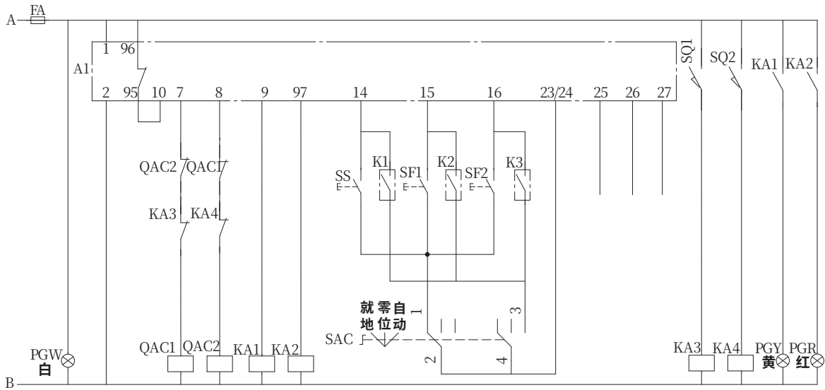
控制原理图
