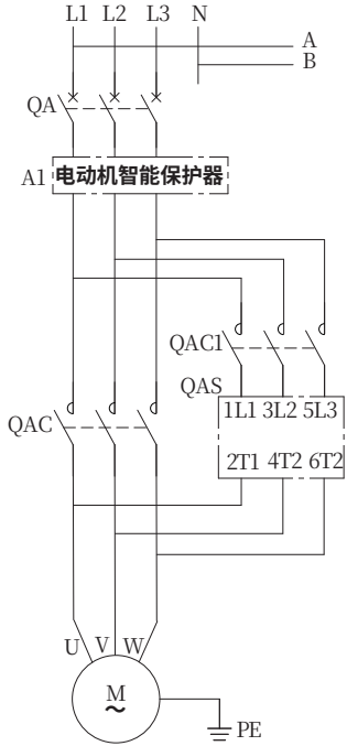
主电路
