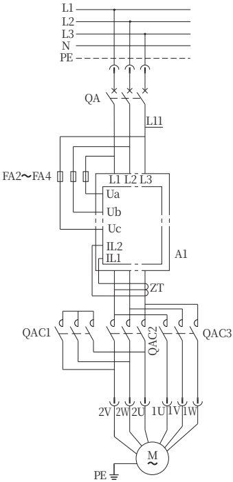
主电路
