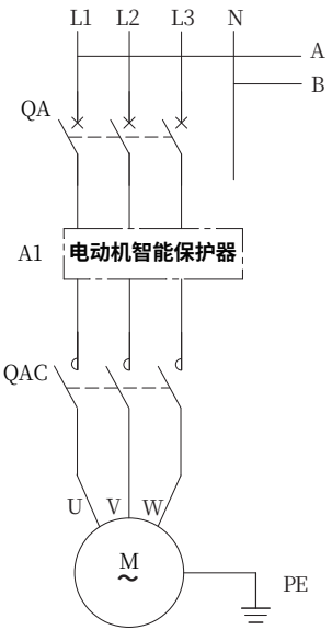
主电路
