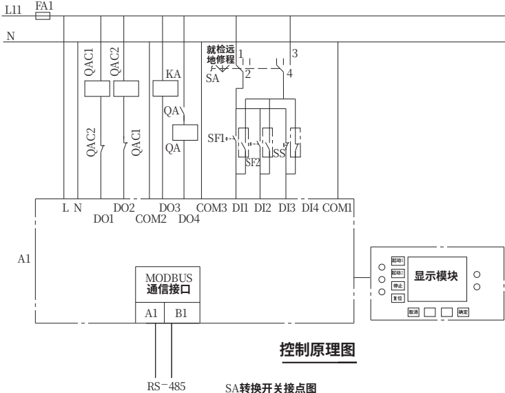
SA转换开关接点图
