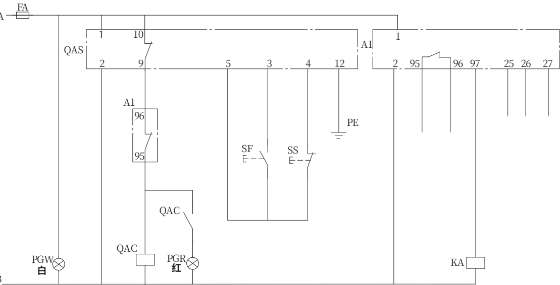
控制原理图
