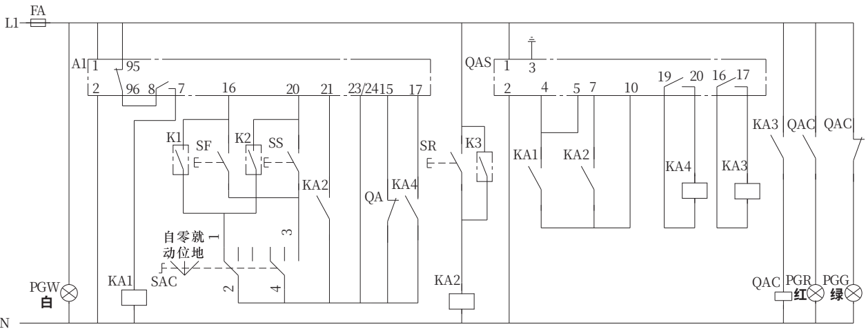
控制原理图
