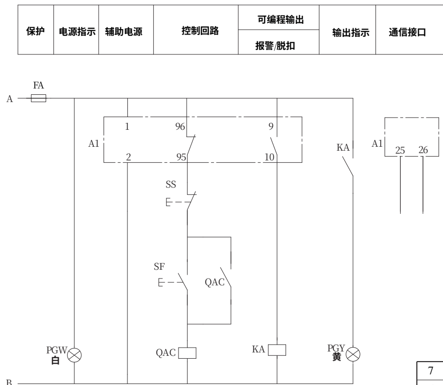
控制原理图
