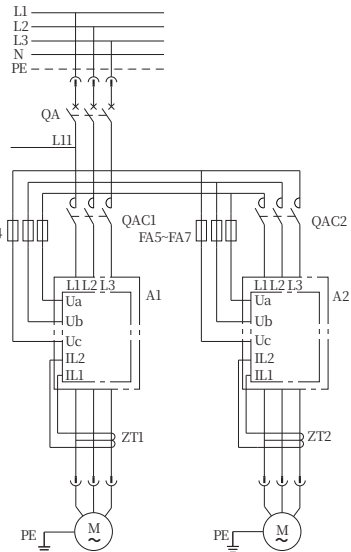
主电路
