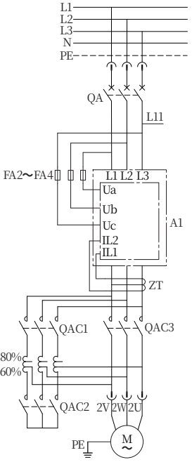
主电路
