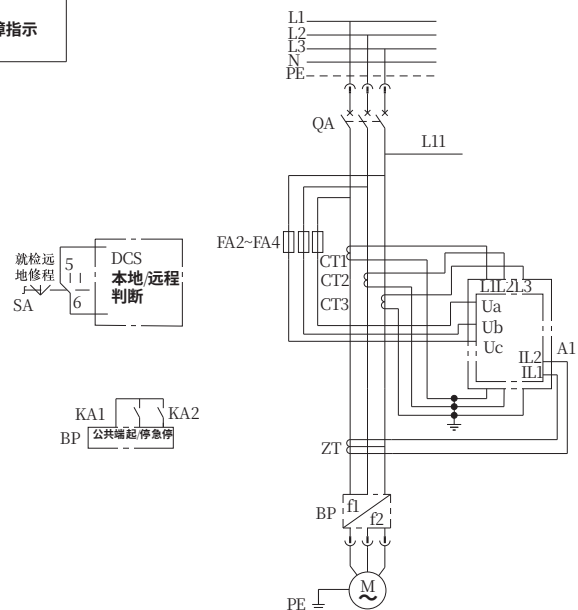
主电路
