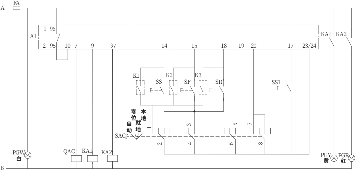
控制原理图
