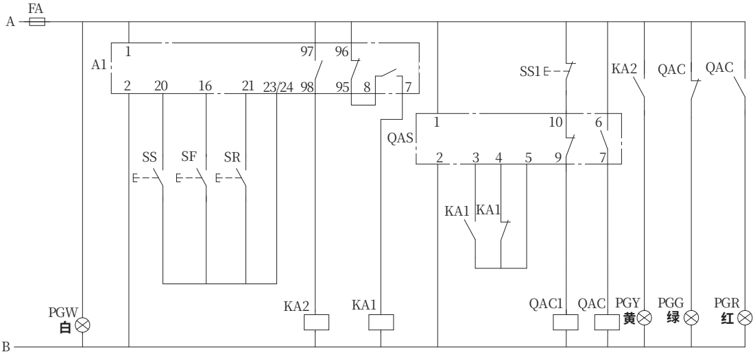
控制原理图
