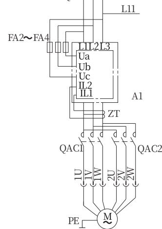
主电路
