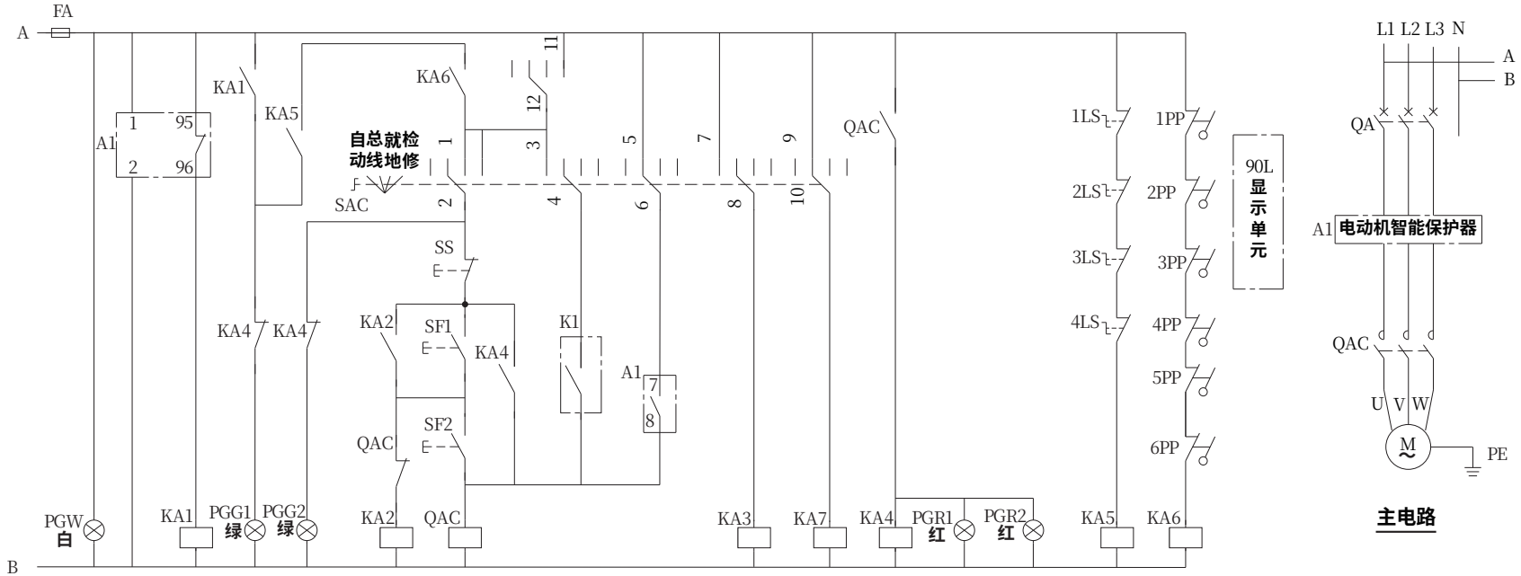
控制原理图
