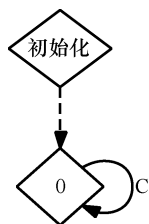
图 5-21 识别语言 C^* 的 DFA
