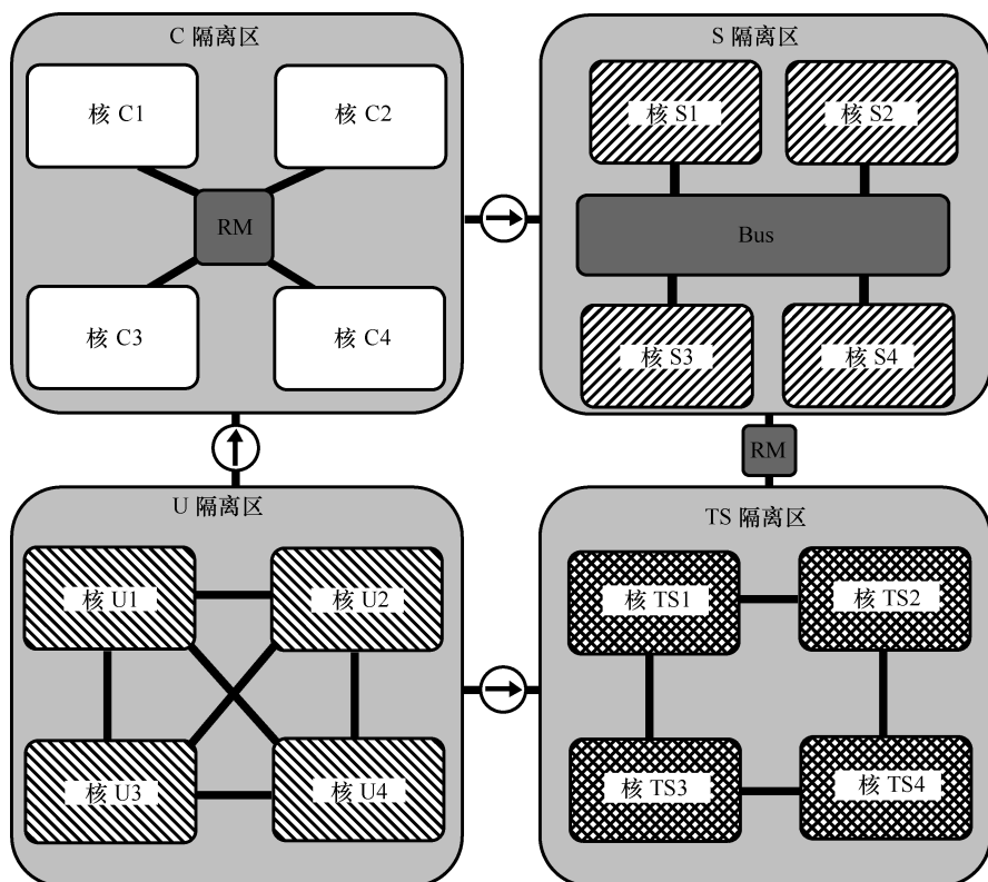
图 7-8 该图显示的是按层次方式排列的各种通信拓扑结构。TS 隔离区所拥有的四个核是呈网格状排列的。S 隔离区拥有的四个核是通过一条总线相连的。C 隔离区所拥有的四个核是呈“星形”结构排列的，并带有一个拥有最低权限的引用监视器。U 隔离区所拥有的四个核是呈网状排列的。二极管可以确保数据只从 U 流向 TS，从 U 流向 C，以及从 C 流向 S，TS 与 S 之间的连接线路上放置了一只引用监视器，以便执行更为精细的策略（比如仅在某些情况下从 S 流向 TS）
