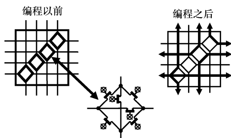
图 1-7 内部链接点上带有六个传输晶体管的开关盒（晶体管用作可编程开关，晶体管门由配置存储单元驱动。为了实现完整的交叉开关，需要 16 个晶体管）
