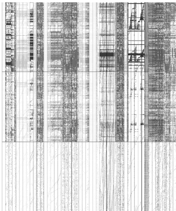
图 A-3 Firefox 在加载网页时处理 5000 万条指令的一块缓存区域。 x 轴为时间， y 轴为存储访问地址的一个函数。每一条“垂直线”或间隔区代表 100 万条指令。顶部区段显示的是一级缓存的命中次数，中部区段显示的是一级缓存的未命中次数，而底部区段显示的是二级缓存的未命中次数。根据基于微波的相位分类算法为间隔区进行了着色 [13]
