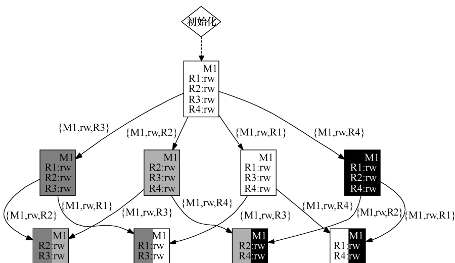
图 5-10 DFA 强制执行中国墙策略。访问过 \text{Range}_1 （白色）的某个核随即就被禁止访问 \text{Range}_2 （浅灰色），但是该核仍旧可以访问 \text{Range}_3 （深灰色）或者 \text{Range}_4 （黑色），因为 \text{Range}_1 和 \text{Range}_4 与 \text{Range}_1 和 \text{Range}_2 属于不同利益冲突类
