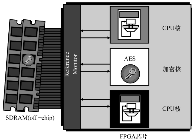
图 5-1 拥有两颗 CPU 和一颗 AES 加密核的 FPGA， 以及置于 FPGA 之上的引用验证机制（RVM）
