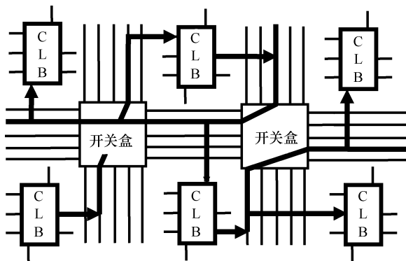
图 1-3 FPGA 内部连线体系结构（每个 CLB 模拟一个基本的逻辑门功能。通过将 CLB 连接在一起可以实现更加复杂的电路。内部连线负责将 CLB 连接起来。开关矩阵需要进行仔细设计，因为实现完整一个交叉开关时需要 N^2 个连接点。采用可重构硬件实现存储逻辑的效率较低，这主要由于能够取任何值的存储需要开关阵列为完整的交叉开关。由于这个原因，在 FPGA 中，在可重配置逻辑之间嵌入了硬线连接的存储单元（BRAM），甚至处理器）
