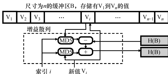
图 4-1 安全增益散列是一种它在缓冲区修改后不需要重新检查完整缓冲区域。保持任意长缓冲区 H(B) 加密安全散列值的方法。修改同时作用在散列和缓冲区域上，代替它的是将原始的散列值从 H(B) 中减去，再加上由于修改后的散列值，即可以得到新的散列值 H(B')
