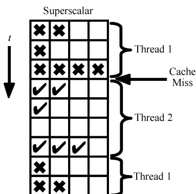
图 A-9 超标量计算机展示的垂直浪费
