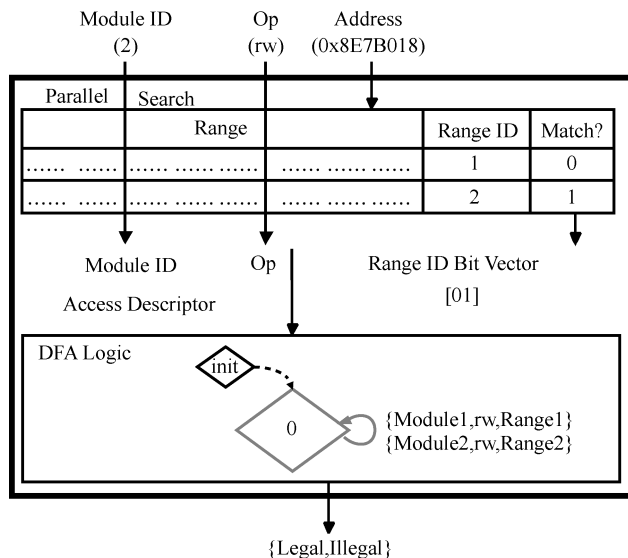
图 5-6 执行模块可接受三种输入值：模块 ID、操作码和地址。通过并行检索可以确定范围 ID。模块 ID、操作码和范围 ID 位矢共同组成了访问描述符，状态机使用该描述符来确定输出值：“1”（同意）或“0”（拒绝）
