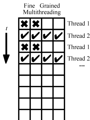
图 A-10 细粒度多线程计算机展示的水平浪费
