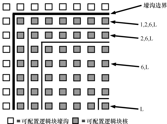
图 6-3 检查法在壕沟构建过程中所产生的间隔更小或根本没有间隔，这种壕沟被称为“无缝”壕沟。设计工具必须对越过边界的片段进行静态校验。
