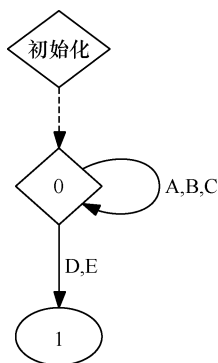
图 5-19 识别该语言 (A|B|C)^* 的 DFA。 输入值为 D 或 E 时会导致该 DFA 转变为 拒绝状态(状态“1”)
