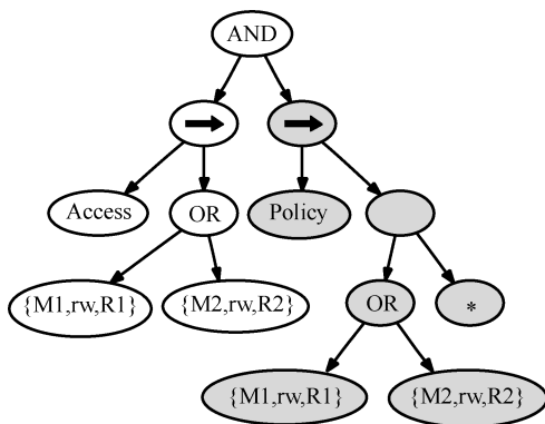
图 5-3 扩展分析树（阴影部分是与该策略中的第二条规则相对应的“右子树”，而“Access”（访问）已被替换为 \{\text{Module}_1, \text{rw}, \text{Range}_1\} \mid \{\text{Module}_2, \text{rw}, \text{Range}_2\} ）
