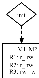
图 5-11 与 B&L 策略对应的 DFA
