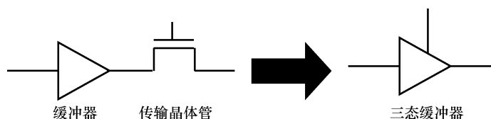
图 1-8 在 FPGA 内部结构设计过程中，较长的距离通常使用缓冲器，这主要是由于电阻和电容以距离长度的二次方增加
