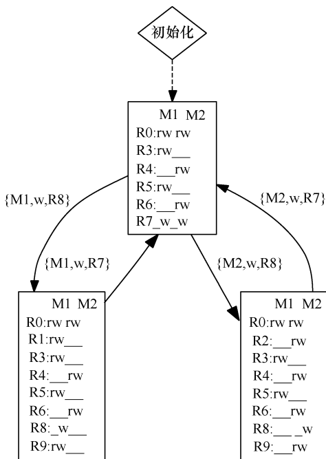
图 7-3 执行嵌入式系统状态性策略的 DFA (确定性有限自动机)
