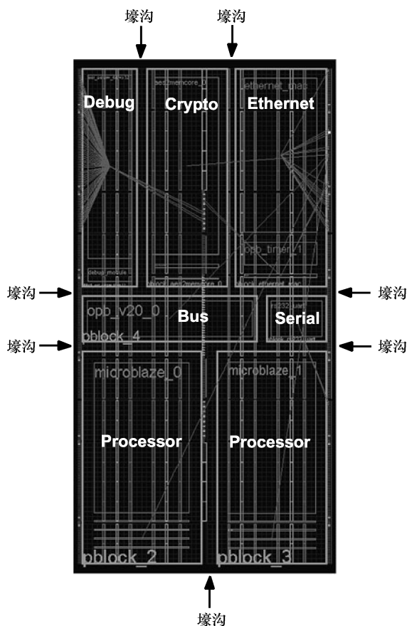
图 7-5 被划分为七个由壕沟加以防护的核后在 PlanAhead 工具中观察到的系统布局图
