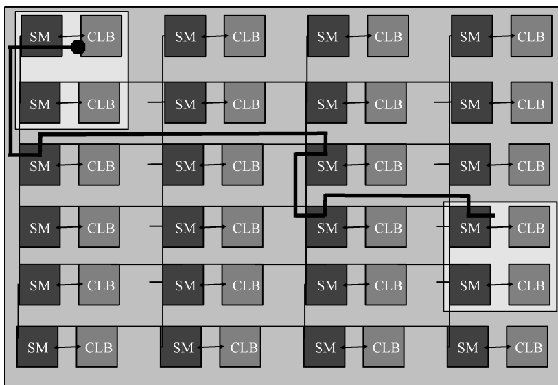
图 6-4 路线跟踪。图中黑线显示的是从位于左上角的浅灰色区域开始一直延伸到右下角的浅灰色区域的一条路线，区域中包含两个可配置逻辑块和两个开关矩阵。
