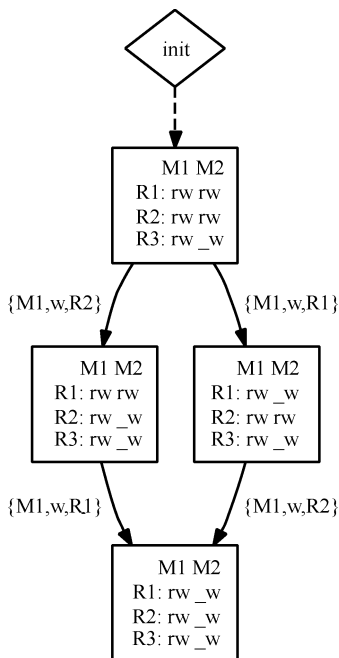
图 5-12 与高水位线策略对应的 DFA
