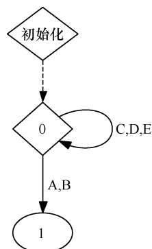
图 5-20 识别语言 (C|D|E)^* 的 DFA。 输入值为 D 或 E 时会导致该 DFA 转变为 拒绝状态(状态“1”)
