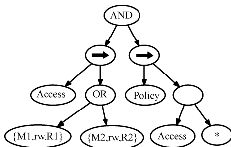
图 5-2 简单策略的分析树（“AND”为根节点，其两个子节点中的每一个都是与该策略的两条规则相对应的一棵子树。
