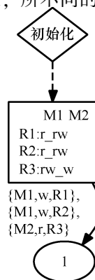
图 5-22 这是 5.5.4 小节中的 B&L 策略的 DFA。输入值为 \{\text{Module}_1, w, \text{Range}_1\} 或 者 \{\text{Module}_1, w, \text{Range}_2\} 时，可导致该 DFA 转变为拒绝状态(状态“1”)
