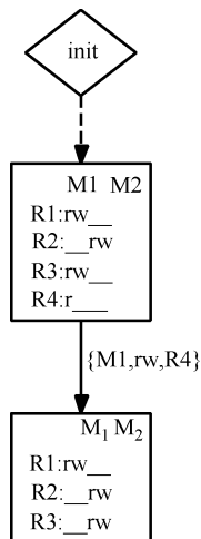
图 5-7 与受控共享策略对应的 DFA
