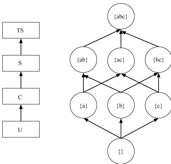
图 2-4 左侧方格内显示的是秘密级的顺序(U: 非密, C: 机密, S: 秘密, TS: 绝密),右侧显示的是秘密级层对应的集合
