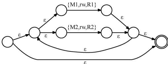
图 5-4 正则表达式衍生出的 NFA（“OR” 需要有四个 Epsilon 转换过程顶部中央位置，最靠近 \{\text{M1}, \text{rw}, \text{R1}\} 和 \{\text{M2}, \text{rw}, \text{R2}\} ）。其他 4 个 Epsilon 转换过程是为 Kleene star 的运行而做的）
