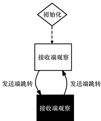
图 3-1 状态策略可以通过定向图的方式表述，其中包含不同状态（节点）之间的跳转（定向边）。此图形中包含有一个循环，说明存在潜在的隐蔽信道。发送端可以在两个状态之间自由切换，接收端可以观察到两个状态之间的差别
