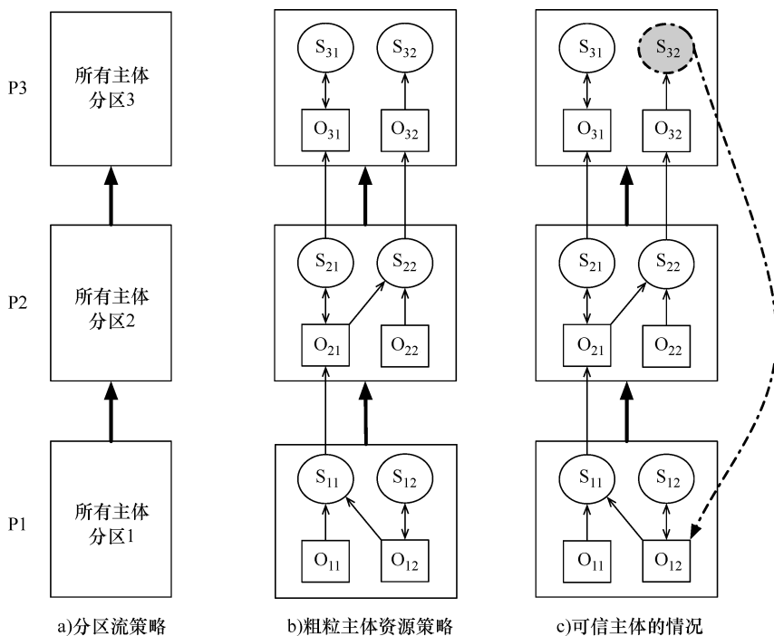
图 2-6 SKPP 策略
