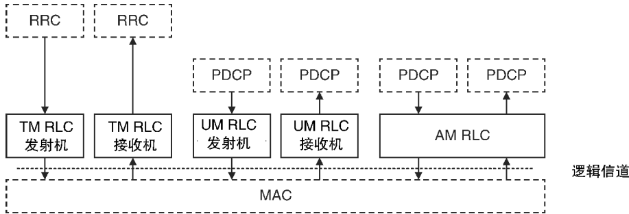
图 10.4 RLC 协议的高级结构（来源：TS 36.322。经 ETSI 许可转载）
