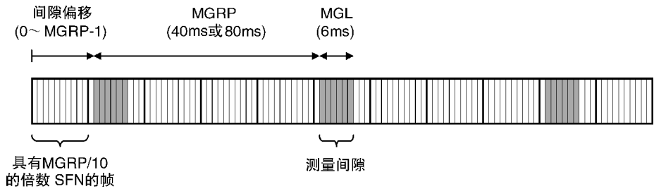
图 14.8 测量间隙
