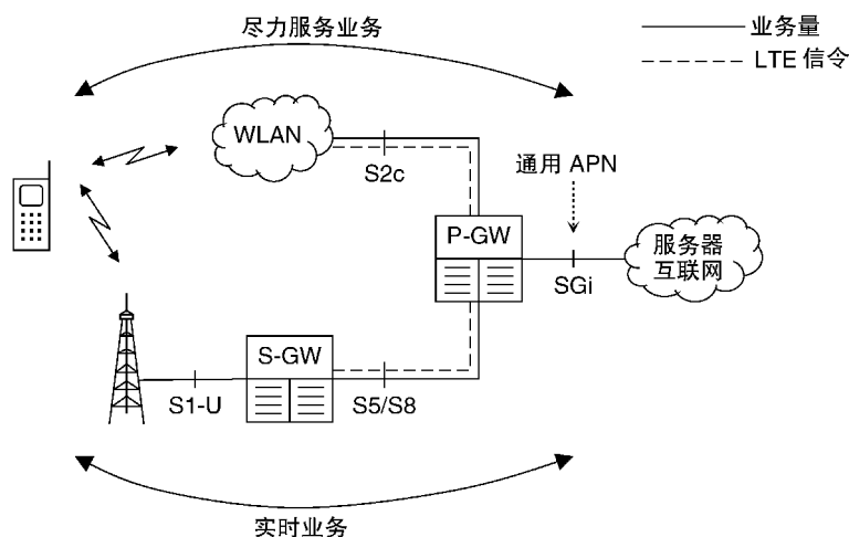
图 19.13 IFOM 的示例网络架构
