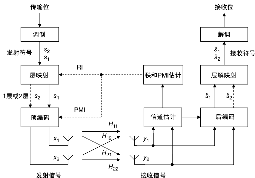
图 5.6 2 \times 2 闭环空间复用系统的操作
