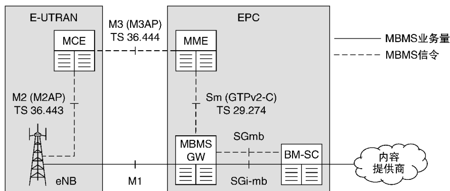
图 18.4 LTE 中的 MBMS 架构
