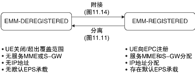
图 2.23 EPS 移动性管理（EMM）状态图
