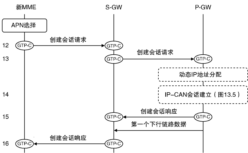
图 11.8 附接过程。(4) 默认承载建立（来源：TS 23.401。经 ETSI 许可转载）
