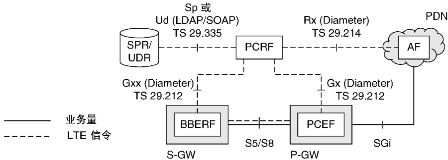
图 13.4 策略和计费控制架构，基于 PMIP 的 S5/S8 接口 (来源：TS 23.203。经 ETSI 许可转载)
