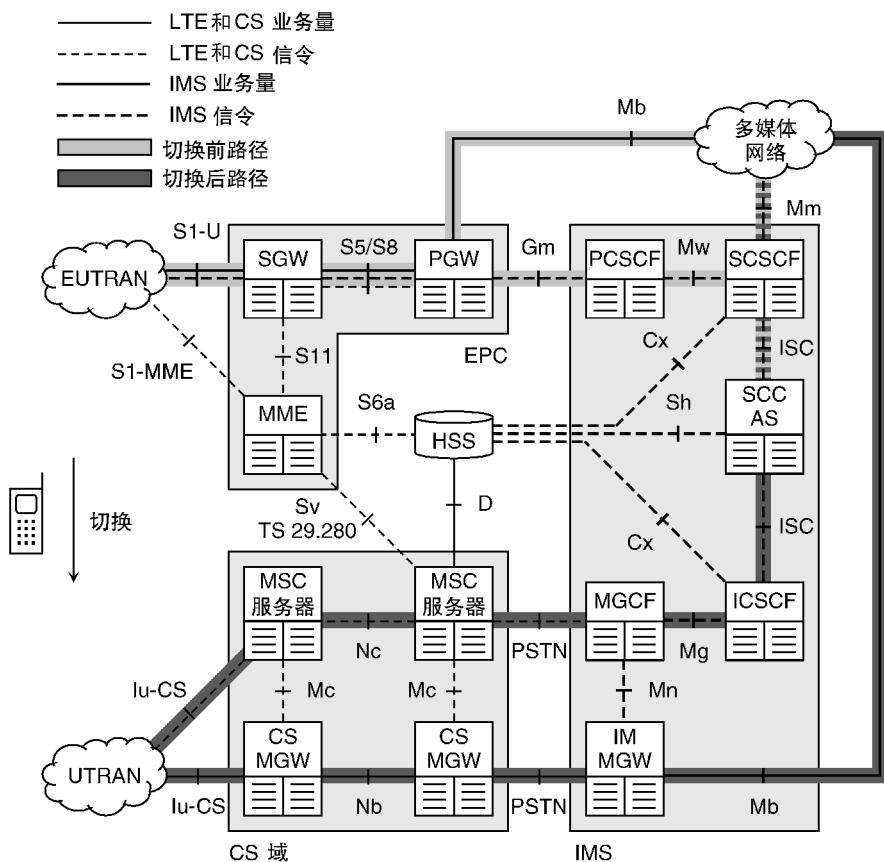
图 22.15 单一无线语音呼叫连续性的架构
