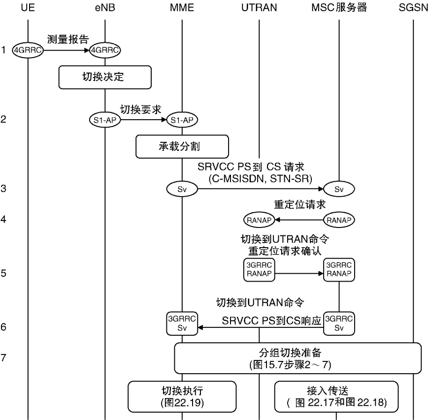
图 22.16 使用 SRVCC 从 LTE 切换到 UMTS。(1) 切换准备 (来源：TS 23.216。经 ETSI 许可转载)
