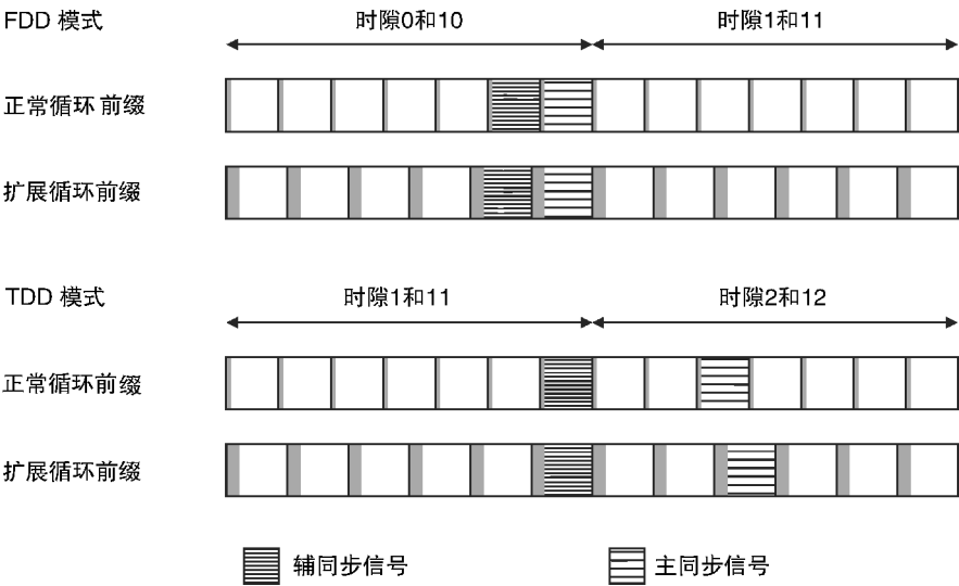
图 7.1 主、辅同步信号的时域映射
