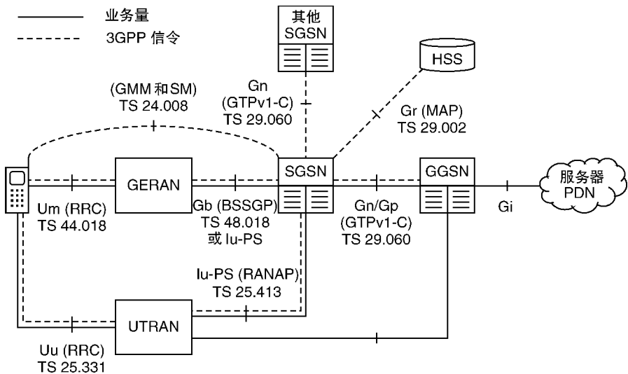
图 15.1 UMTS 和 GSM 分组交换域的架构
