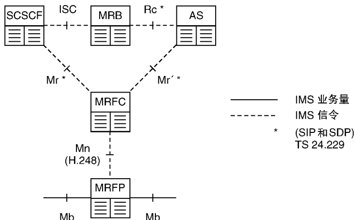
图 22.5 IMS 多媒体资源功能架构
