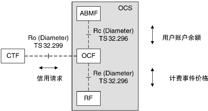
图 13.14 在线计费系统的架构（来源：TS 32.240。经 ETSI 许可转载）
