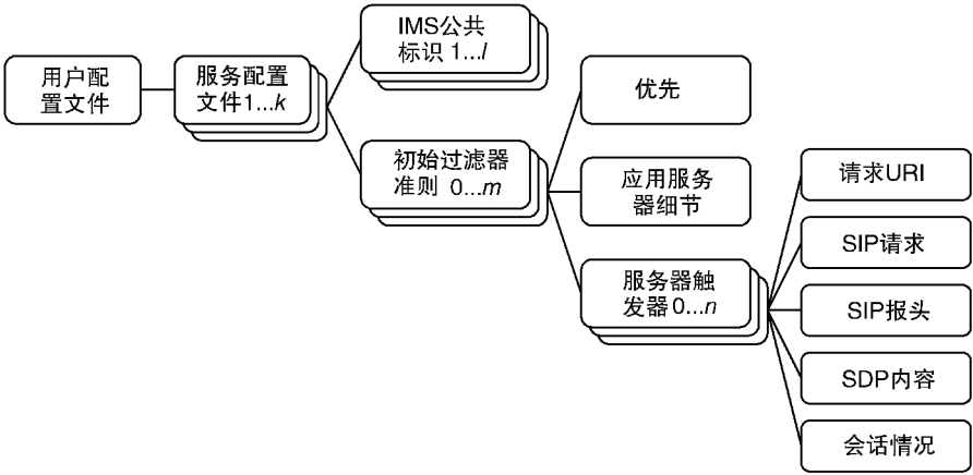
图 22.7 IMS 用户配置文件的主要内容
