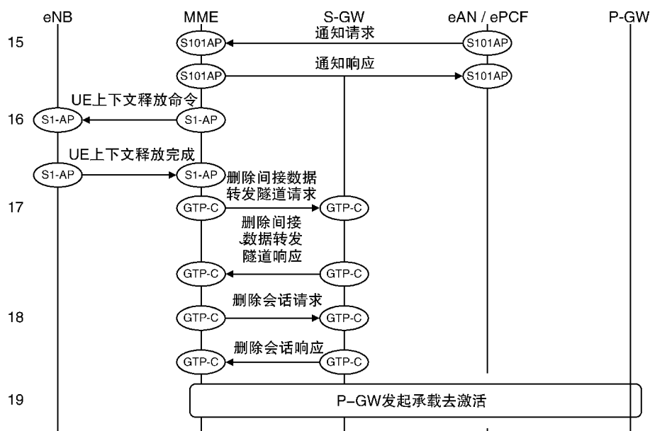
图 16.11 从 LTE 到 cdma2000 HRPD 的系统间切换。(3) 切换完成
