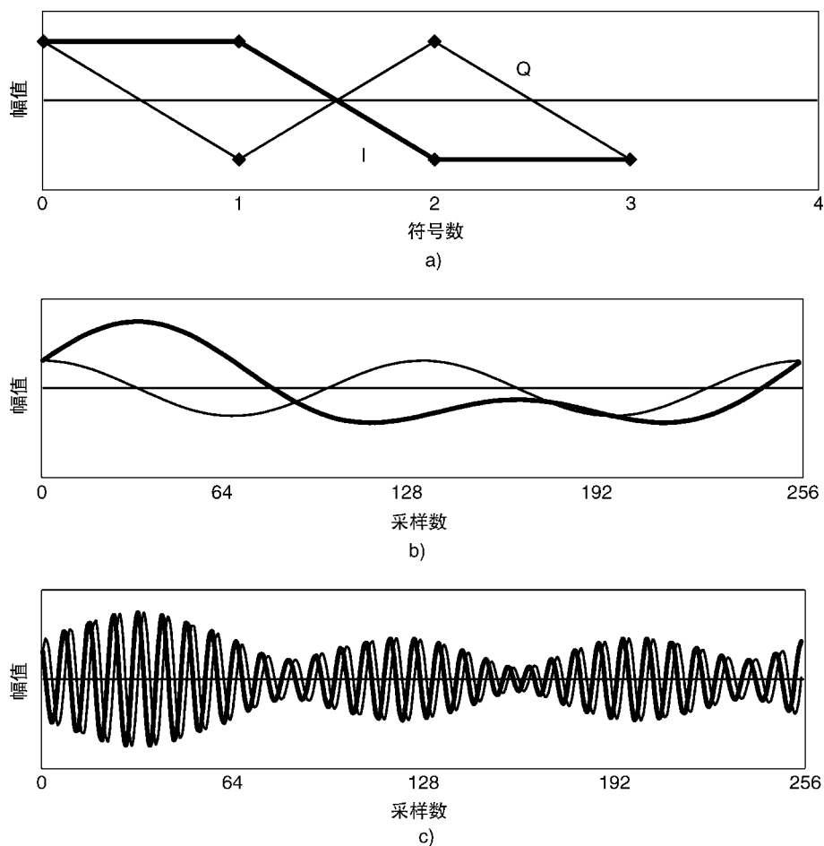
图 4.13 SC-FDMA 波形示例
