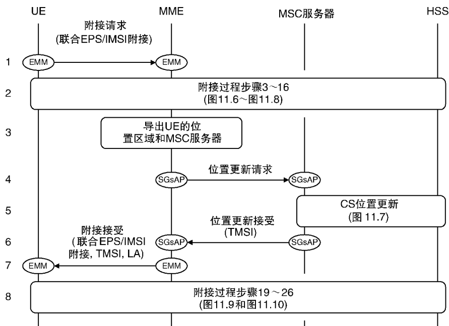
图 21.5 联合 EPS/IMSI 附接过程（来源：TS 23.272。经 ETSI 许可转载）
