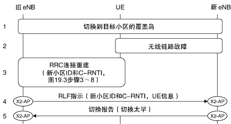
图 17.4 移动性鲁棒优化，由过早的切换触发
