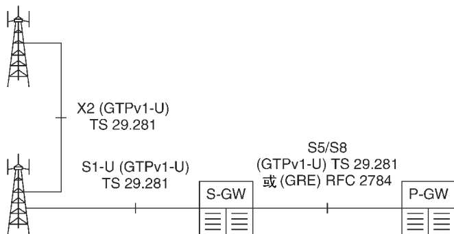
图 2.14 LTE 使用的用户平面协议
