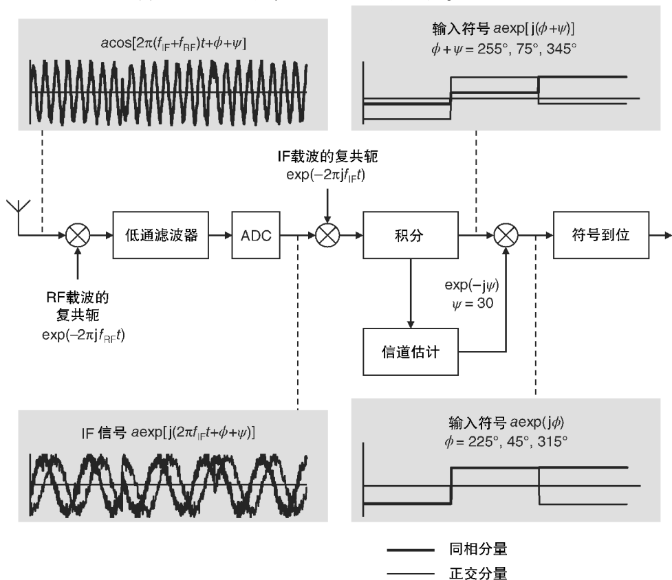
图 3.5 无线通信系统中的解调器的框图
