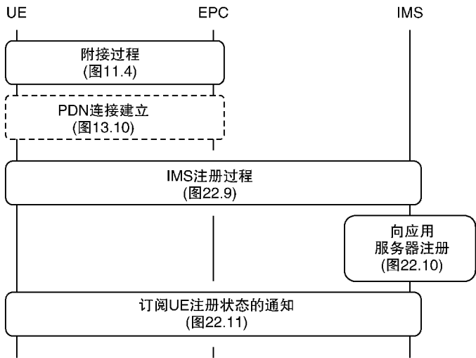
图 22.8 VoLTE 注册过程概述
