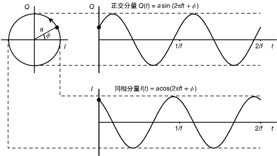
图 3.1 载波信号的同相和正交分量的产生
