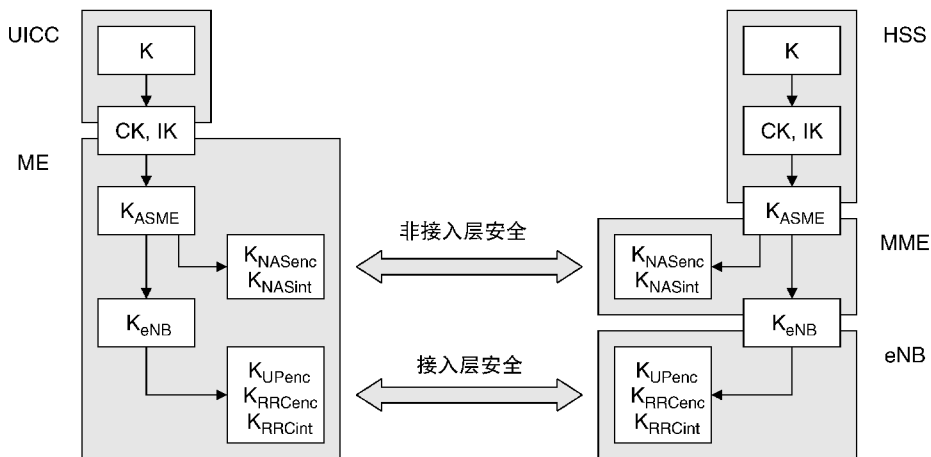
图 12.2 LTE 使用的安全密钥的体系
