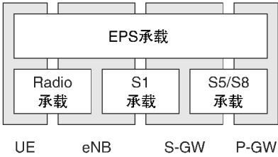
图 2.21 当使用基于 GTP 的 S5/S8 接口时的 LTE 承载架构（来源：TS 36.300。由 ETSI 许可转载）
