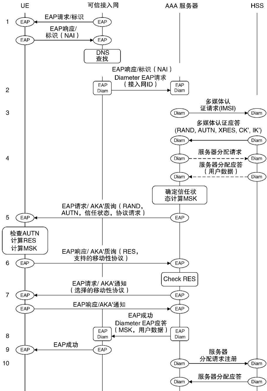
图 16.5 非 3GPP 附着过程。(1) 可信接入网的认证和密钥协商
