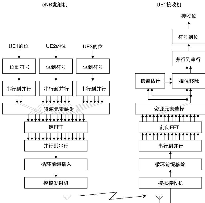
图 4.4 OFDMA 发射机和接收机的结构图
