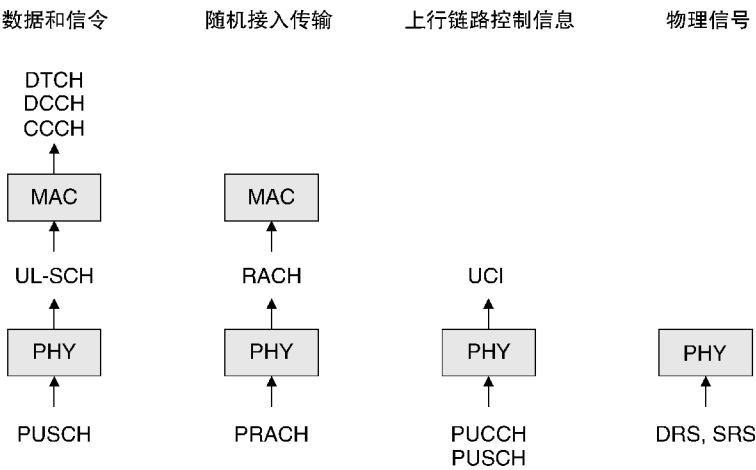
图 6.2 LTE 使用的上行链路信息流
