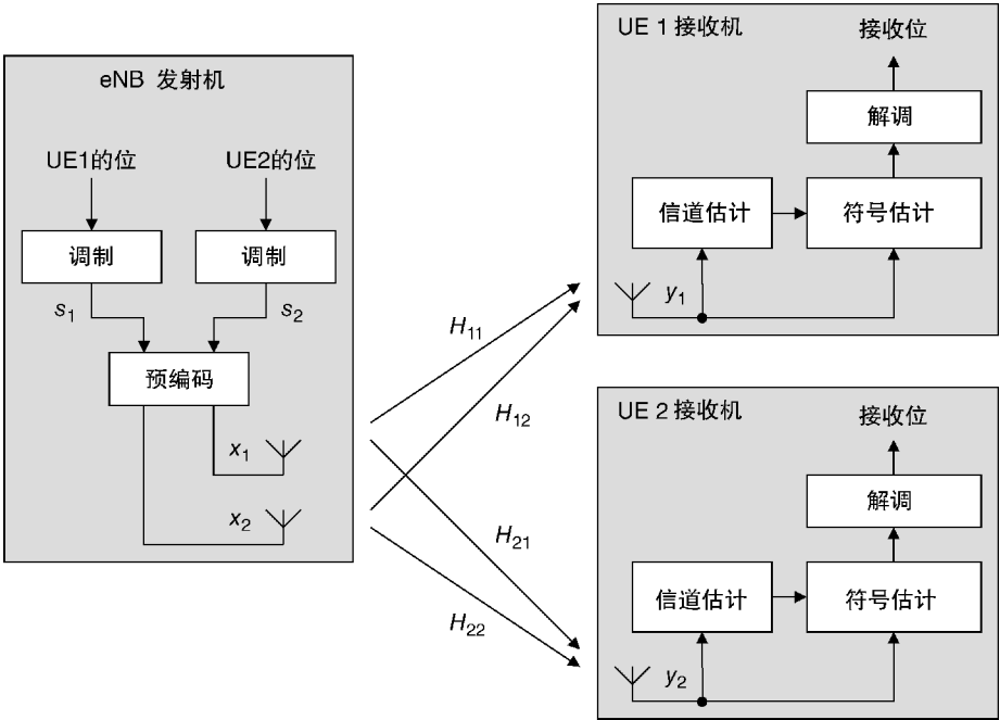
图 5.9 下行链路多用户 MIMO
