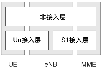
图 2.11 空中接口接入层和非接入层的关系
