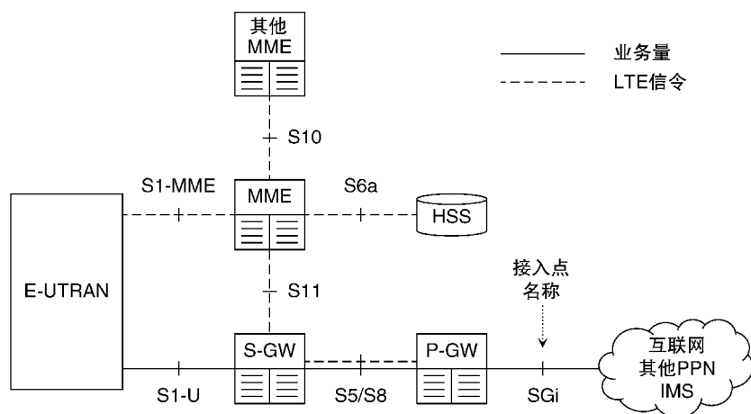
图 2.5 演进分组核心网的主要组件
