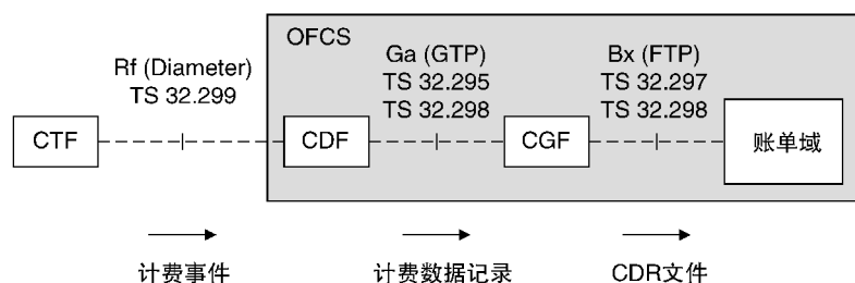
图 13.13 离线计费系统的架构（来源：TS 32.240。经 ETSI 许可转载）
