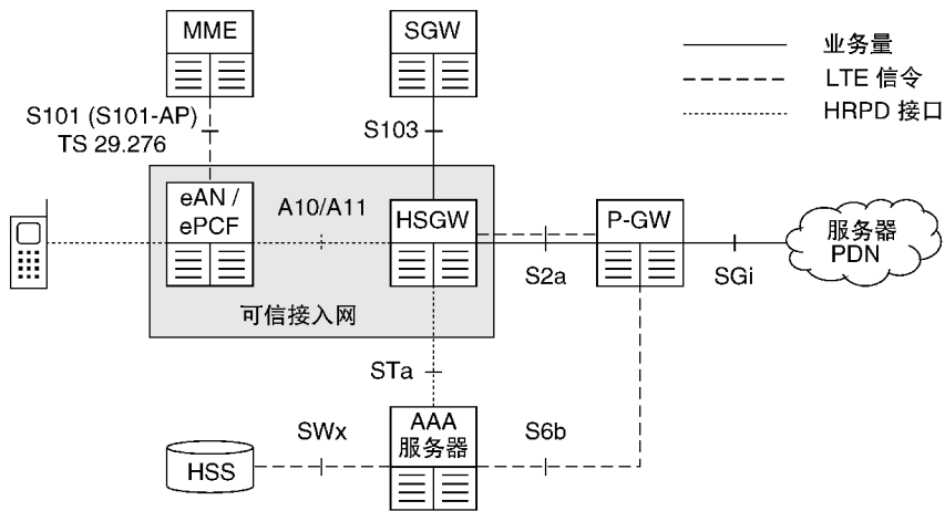
图 16.7 用于与 cdma2000 HRPD 互操作的架构
