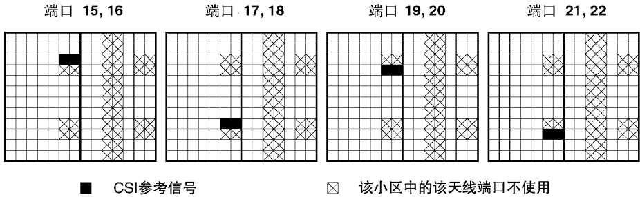
图 19.4 用于 CSI 参考信号的示例资源元素映射, 使用 FDD 模式和正常循环前缀 (来源: TS 36. 211。经 ETSI 许可转载)
