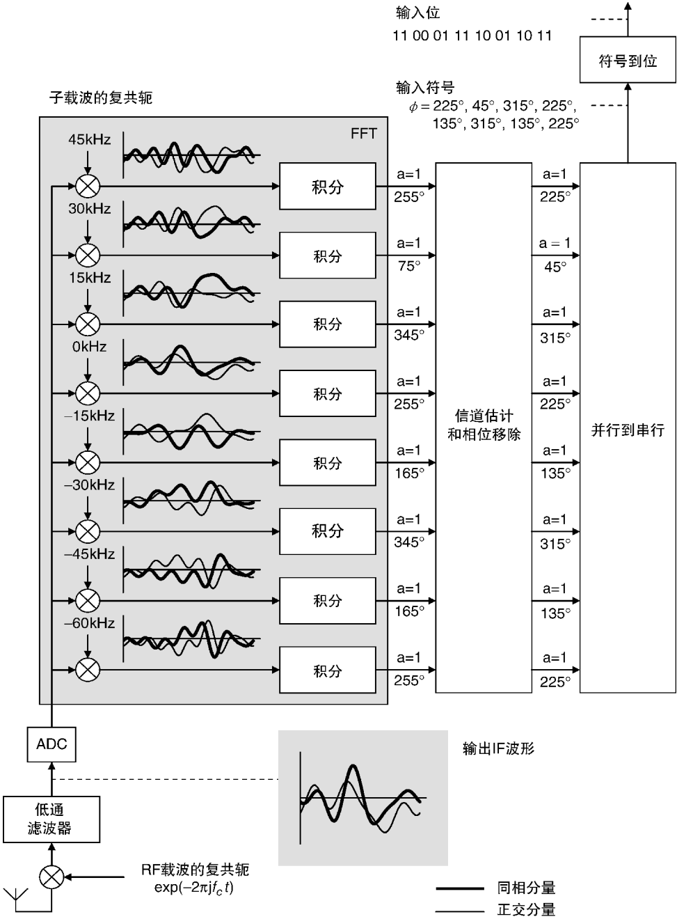
图 4.3 OFDM 接收机的处理步骤
