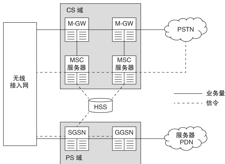
图 1.3 UMTS 与 GSM 核心网的架构
