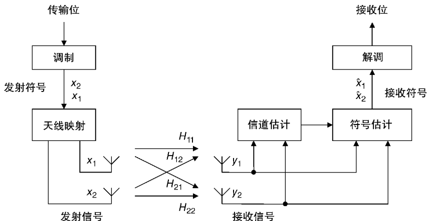
图 5.4 2 \times 2 空间复用系统的基本原理
