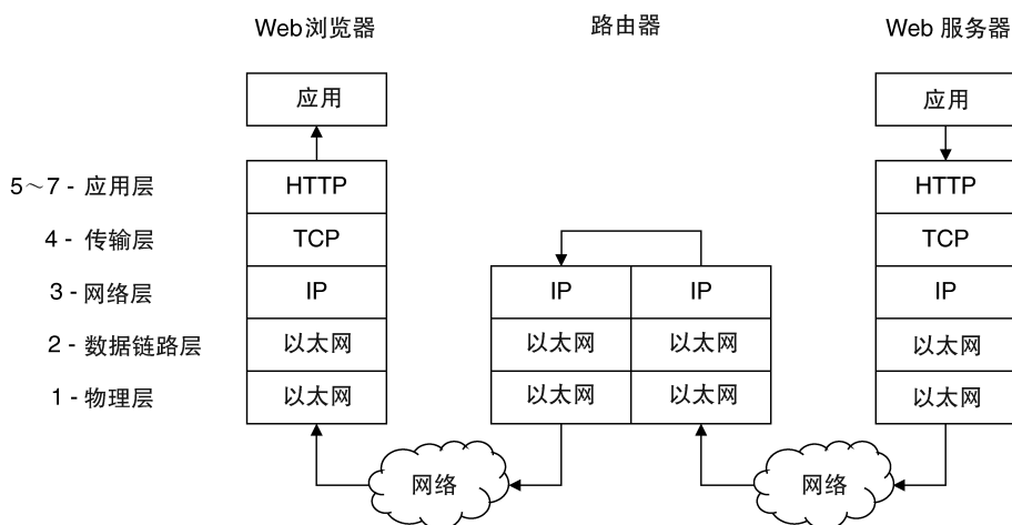
图 1.4 互联网通信协议，OSI 模型层图
