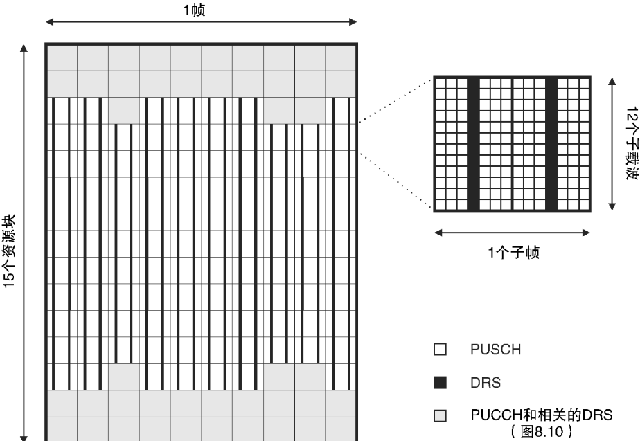
图 8.8 使用 FDD 模式、正常循环前缀、3MHz 带宽和用于 PUCCH 的示例分配的 PUSCH 及其解调参考信号的资源元素映射
