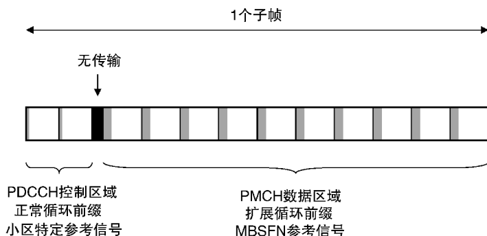
图 18.3 使用正常循环前缀的两符号控制区域的 MBSFN 子帧的示例结构
