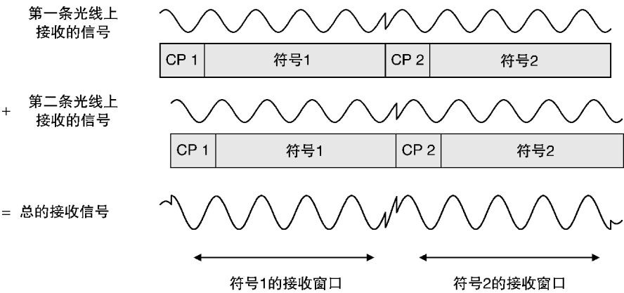
图 4.9 单个子载波上的循环前缀的操作
