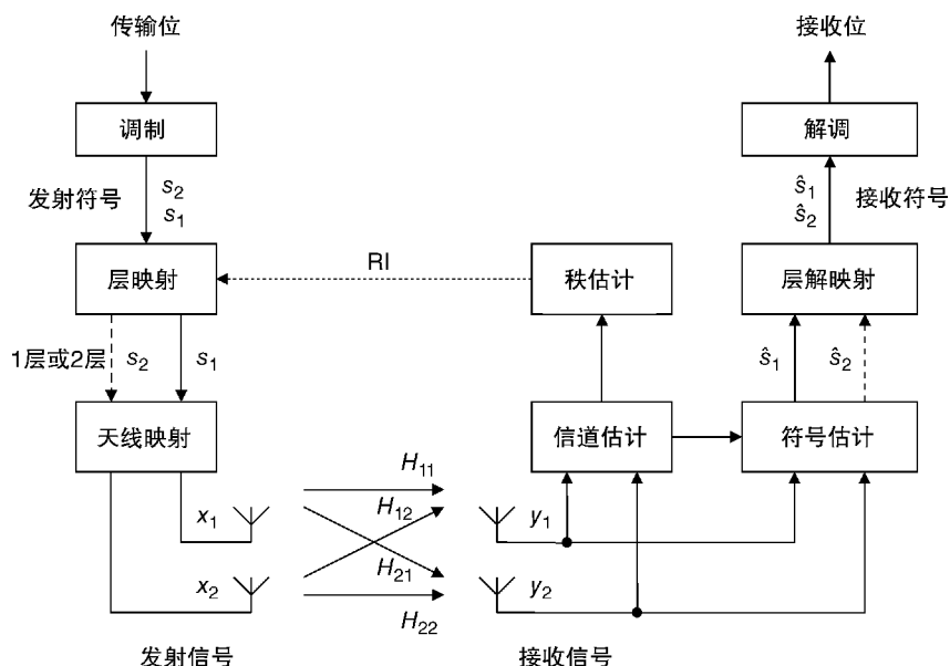
图 5.5 2 \times 2 开环空间复用系统的操作
