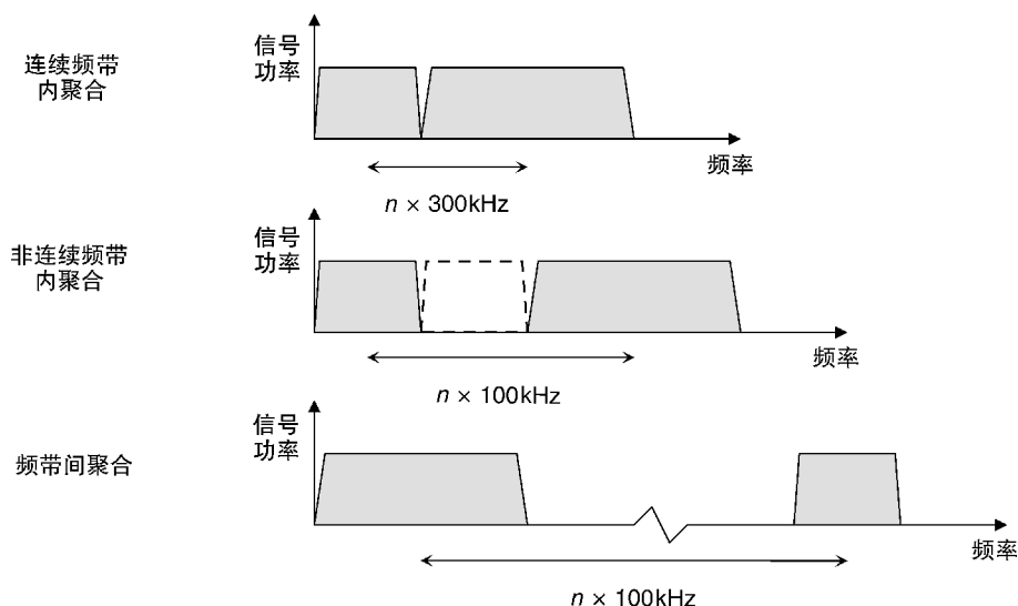
图 19.1 载波聚合场景
