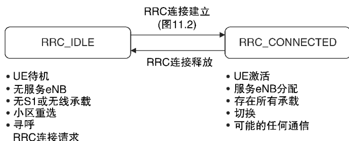
图 2.25 无线资源控制（RRC）状态图
