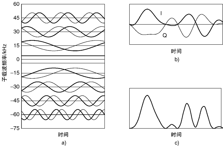
图 4.11 OFDMA 波形示例
