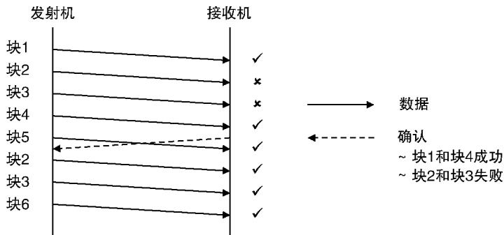
图 3.14 选择性重传 ARQ 方案的操作
