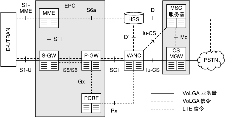
图 21.3 VoLGA 架构
