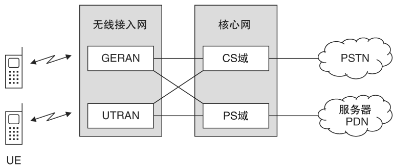
图 1.1 UMTS 与 GSM 的高层体系架构
