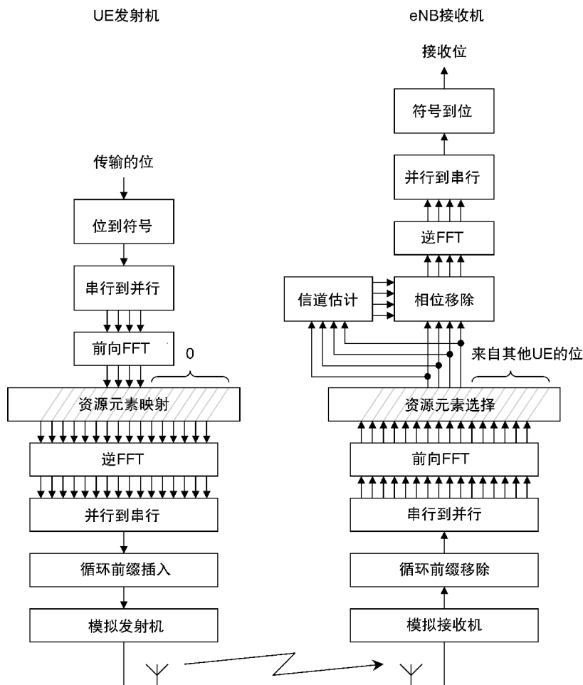
图 4.12 SC-FDMA 发射机和接收机的结构图
