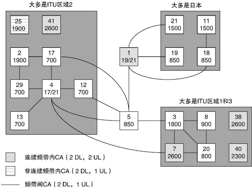
图 19.2 支持版本 11 中的载波聚合的频带
