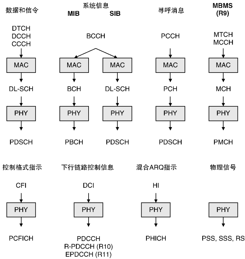
图 6.3 LTE 使用的下行链路信息流
