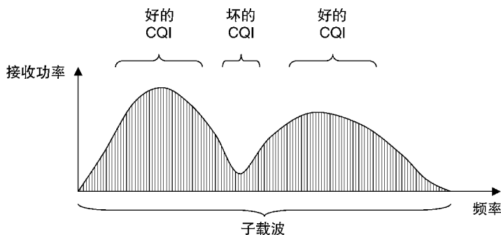
图 4.6 采用 OFDMA 频率特定调度
