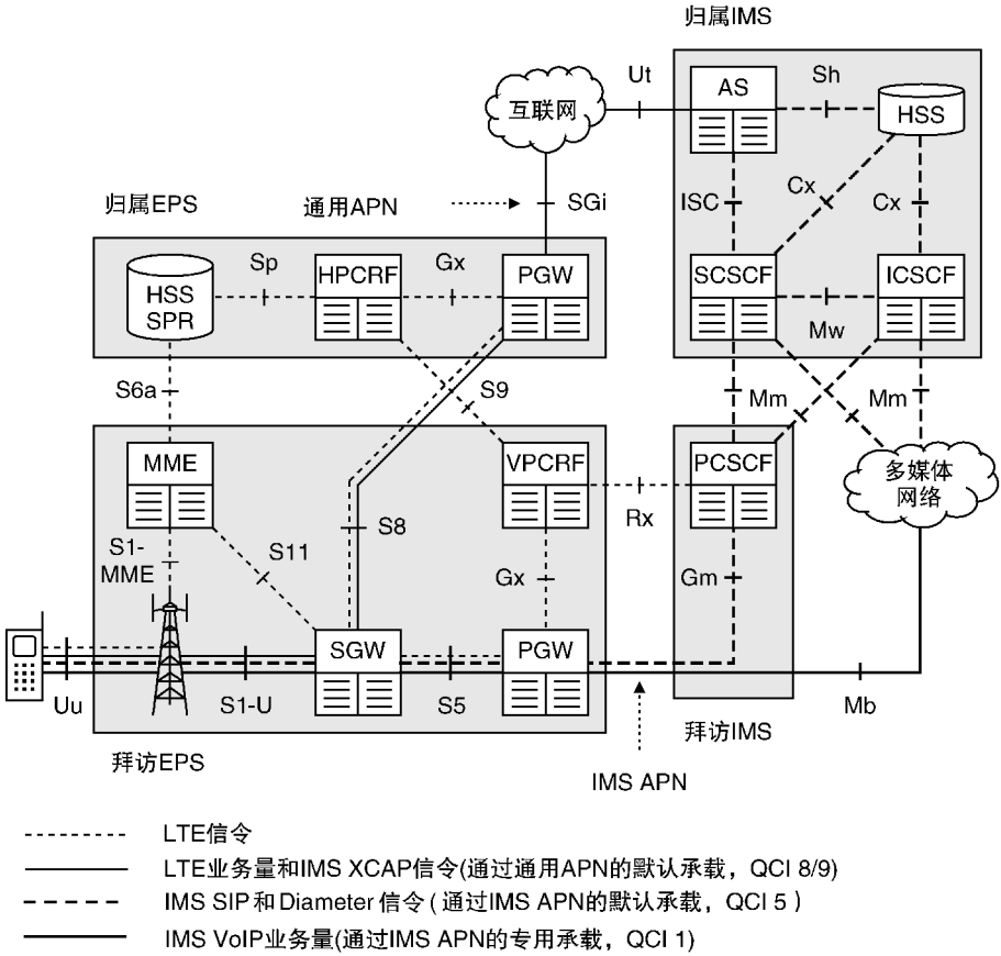
图 22.2 漫游 VoLTE 移动台的系统架构
