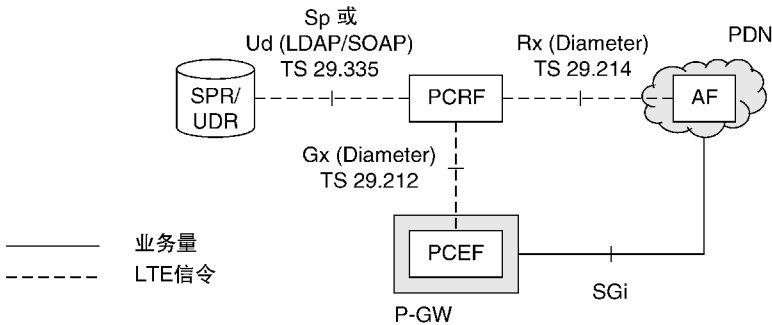
图 13.2 基于 GTP 的 S5/S8 接口的策略控制架构（来源：TS 23. 203。经 ETSI 许可转载）
