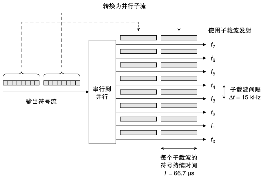
图 4.1 使用 OFDM 将频带划分为子载波
