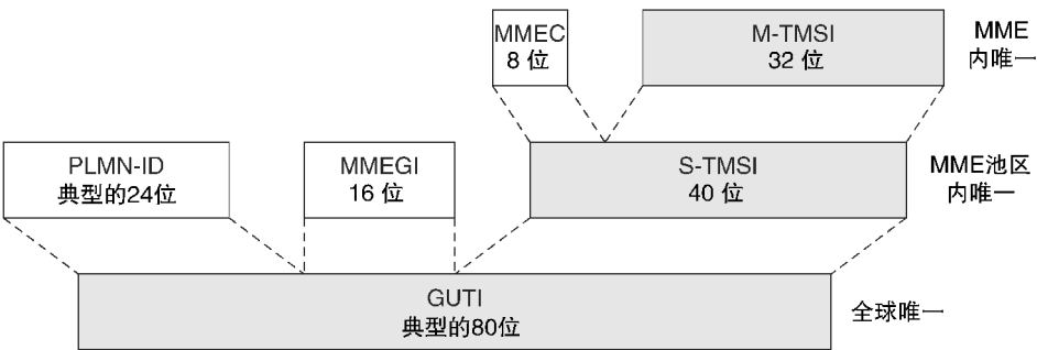
图 2.9 移动台使用的临时标识
