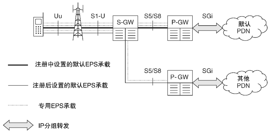
图 2.20 当使用基于 GTP 的 S5/S8 接口时的默认和专用 EPS 承载
