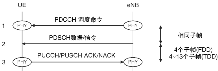
图 8.1 下行链路发送和接收过程
