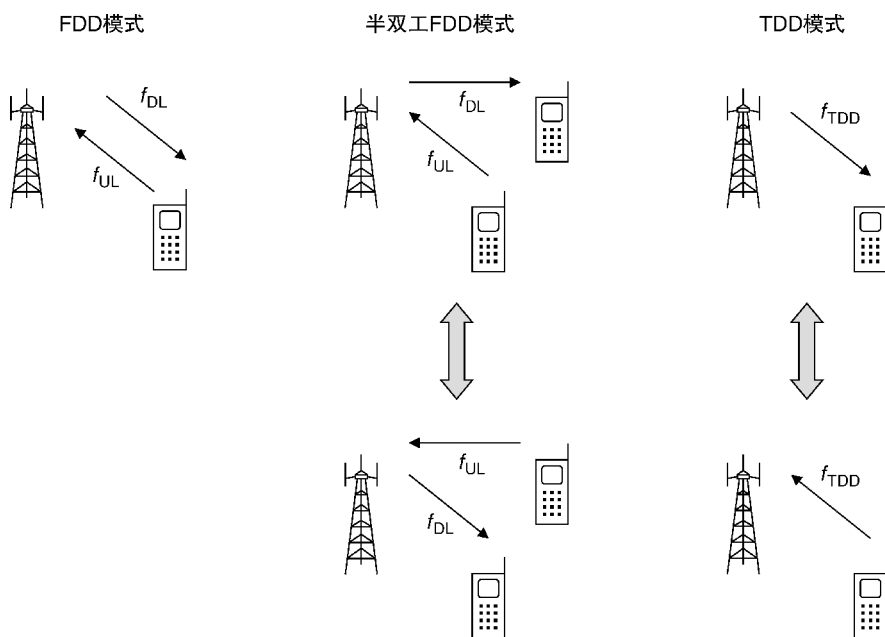
图 3.8 FDD 和 TDD 模式运作
