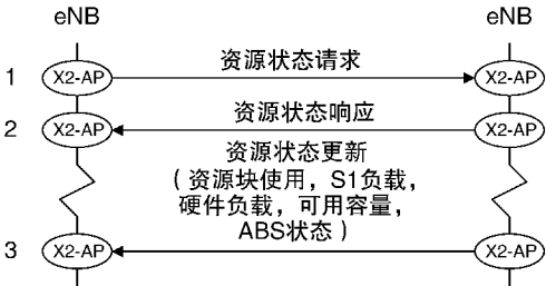
图 17.2 资源状态报告过程
