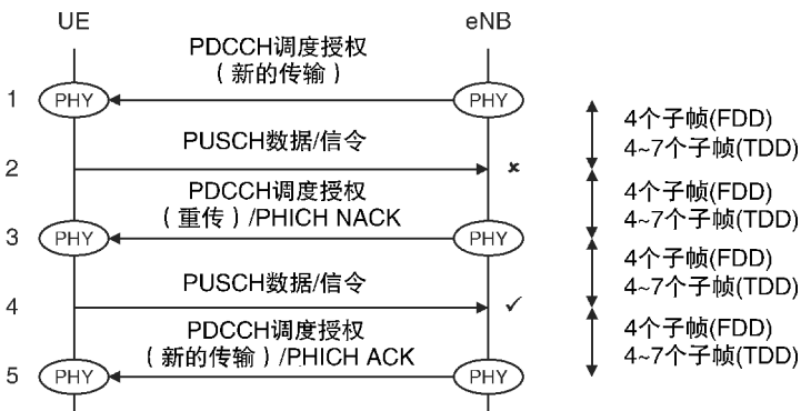
图 8.3 上行链路发送和接收程序
