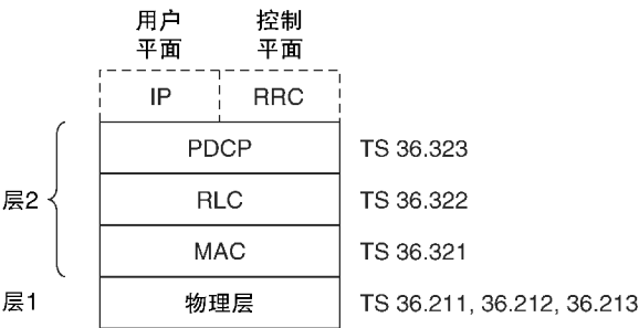
图 2. 12 空中接口的传输协议（来源：TS 36. 300。由 ETSI 许可转载）
