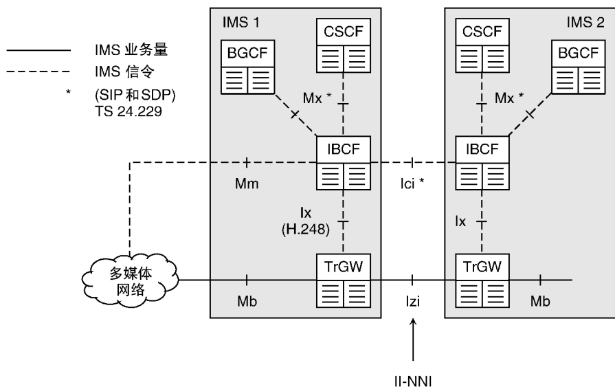
图 22.3 IMS 边界控制架构
