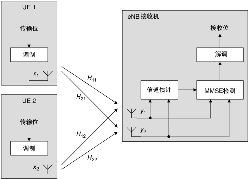
图 5.8 上行链路多用户 MIMO
