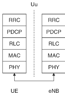
图 2.17 用来交换移动台和基站之间的 RRC 信令信息的协议栈
