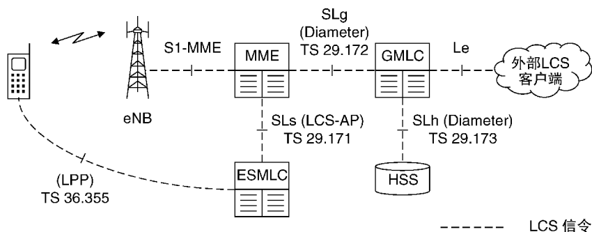
图 18.5 LTE 中定位服务的架构
