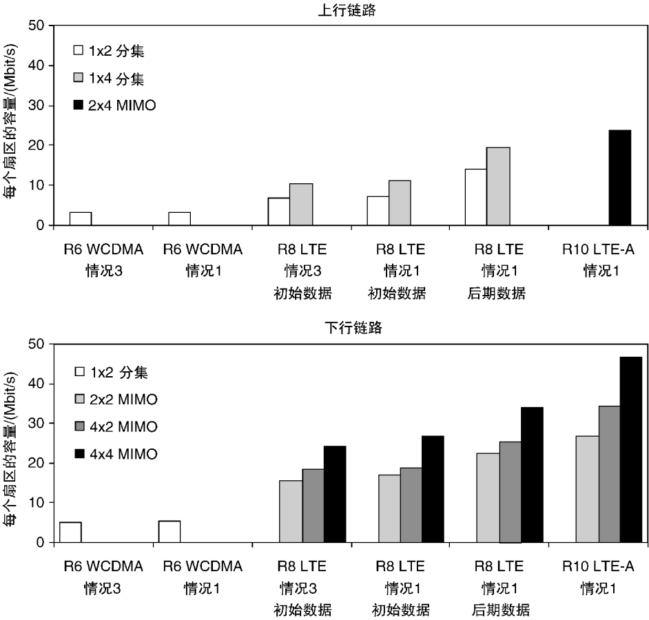
图 23.4 在 10MHz 带宽中的典型 LTE 宏小区每个扇区的容量
