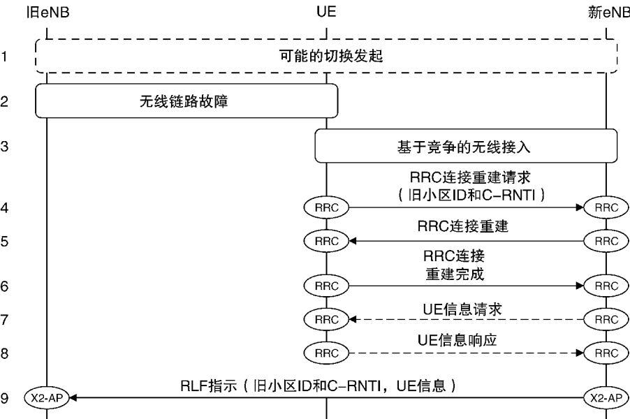
图 17.3 移动性鲁棒优化，由太晚的切换触发
