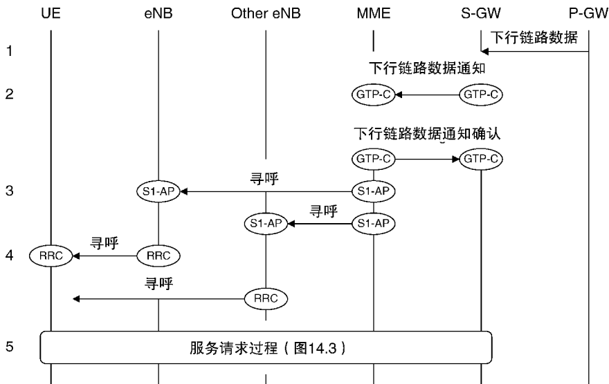
图 14.2 寻呼过程 (来源: TS 23. 401. 经 ETSI 许可转载)
