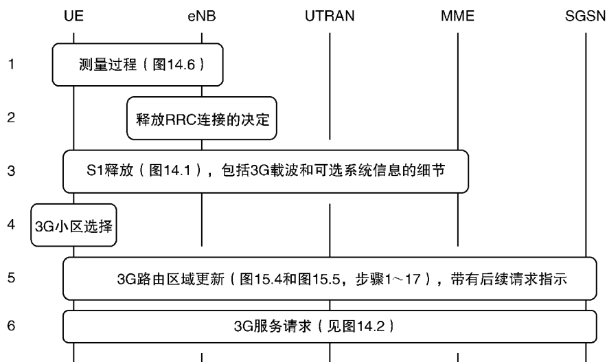
图 15.6 重新定向到 UMTS 载波频率的 RRC 连接释放
