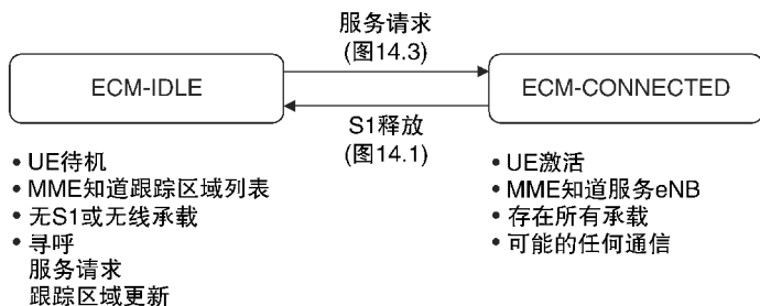
图 2.24 EPS 连接性管理 (ECM) 状态图
