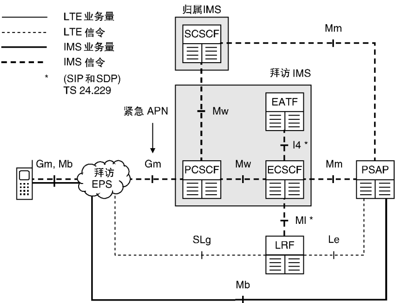
图 22.21 IMS 紧急呼叫的架构（来源：TS 23.167。经 ETSI 许可转载）
