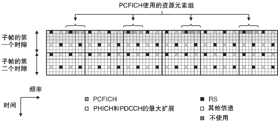
图 7.4 物理控制格式指示信道的资源元素映射，使用正常循环前缀、1.4MHz 带宽、第一个天线端口为 2、物理小区 ID 为 1
