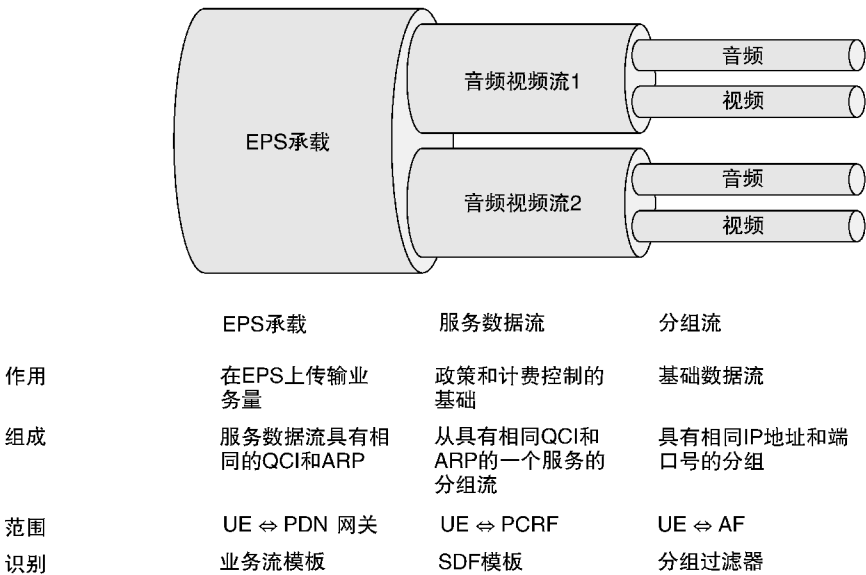
图 13.1 EPS 承载、服务数据流和分组流之间的关系
