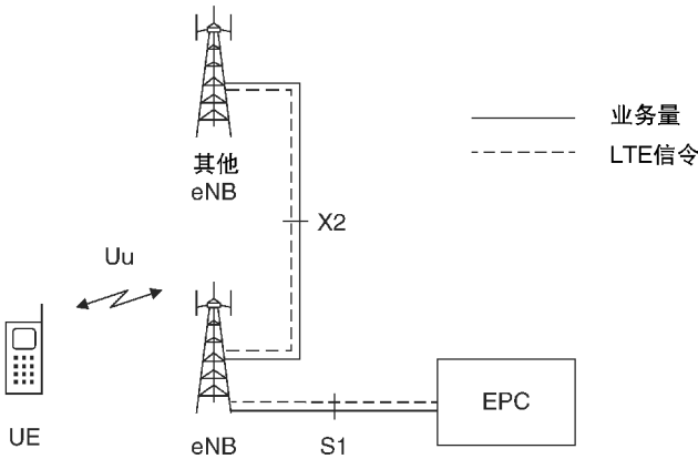
图 2.3 演进 UMTS 陆地无线接入网的架构
