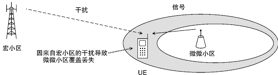
图 19.7 由于来自附近宏小区的干扰导致微微小区的覆盖区域减小
