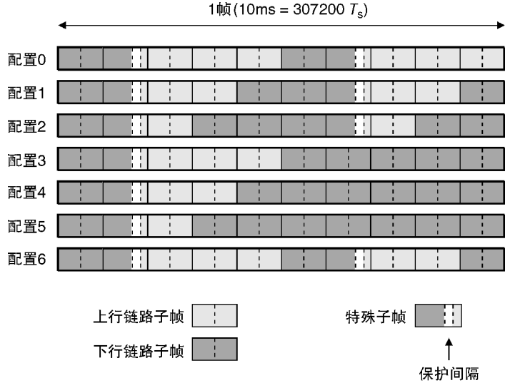
图 6.6 使用帧结构类型 2 的 TDD 配置
