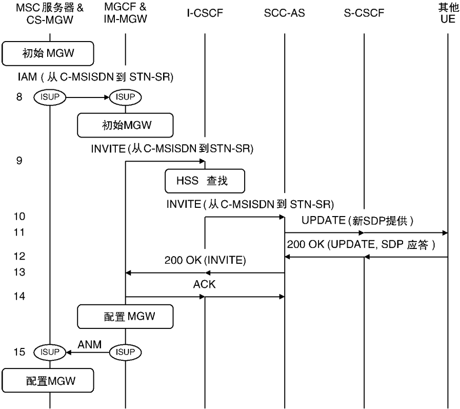
图 22.17 使用 SRVCC 从 LTE 切换到 UMTS。(2) 接入转移和远程分支更新 (来源：TS 23.237。经 ETSI 许可转载)
