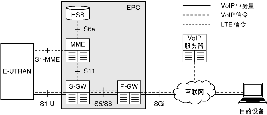
图 21.2 通用第三方 VoIP 系统的架构
