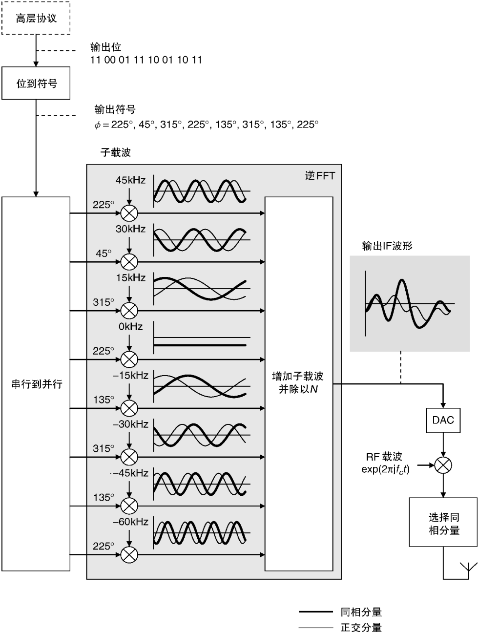
图 4.2 OFDM 发射机的处理步骤
