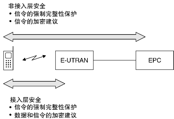
图 12.1 网络接入安全架构
