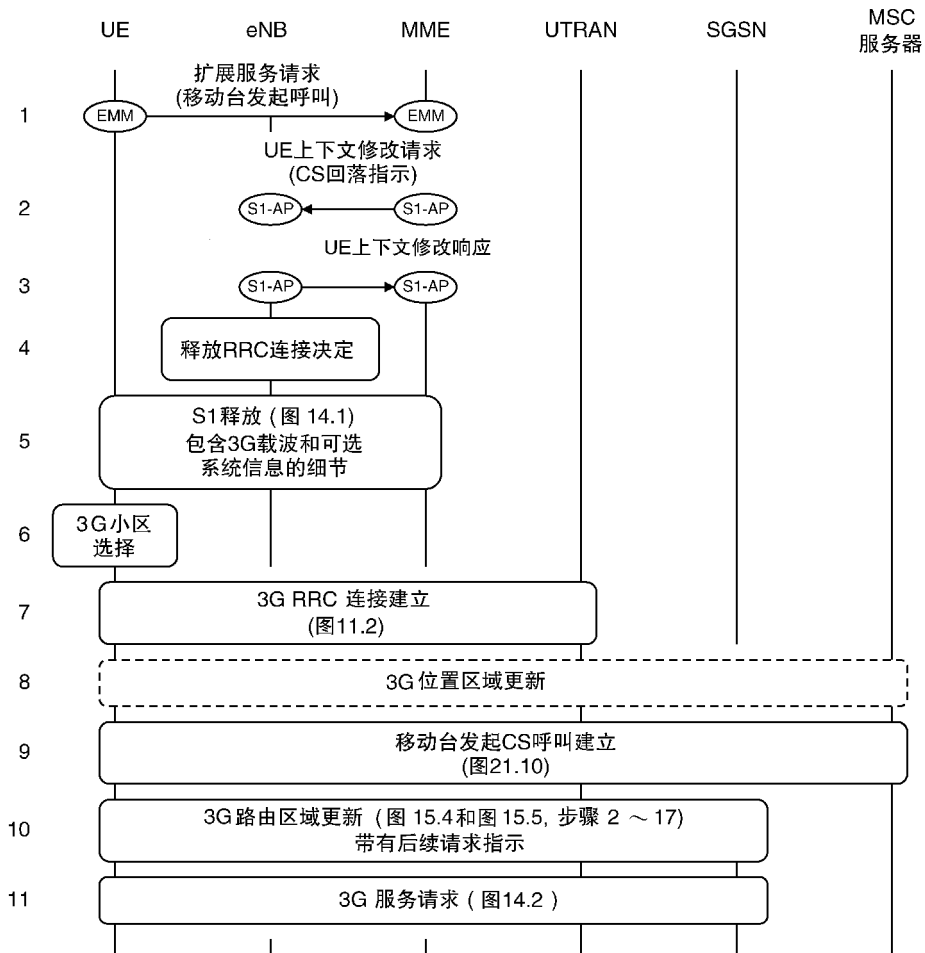
图 21.8 来自 RRC_CONNECTED 状态的移动台的移动发起呼叫建立，使用 CS 回落和 RRC 连接释放，并重新定向到 3G 载波（来源：TS 23.272。经 ETSI 许可转载） 虽然通信中断并且数据速率比之前更低。
