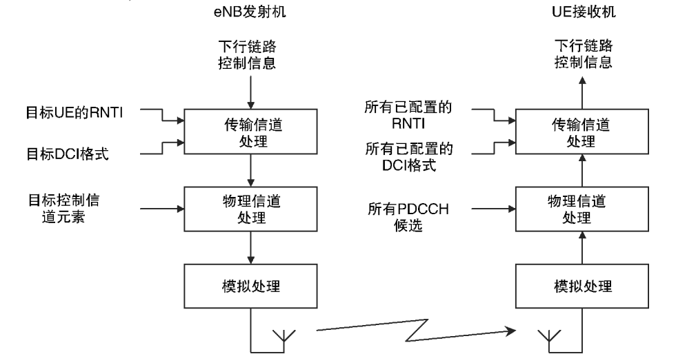
图 8.5 PDCCH 的发送和接收
