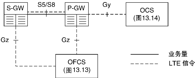
图 13.12 高层计费架构
