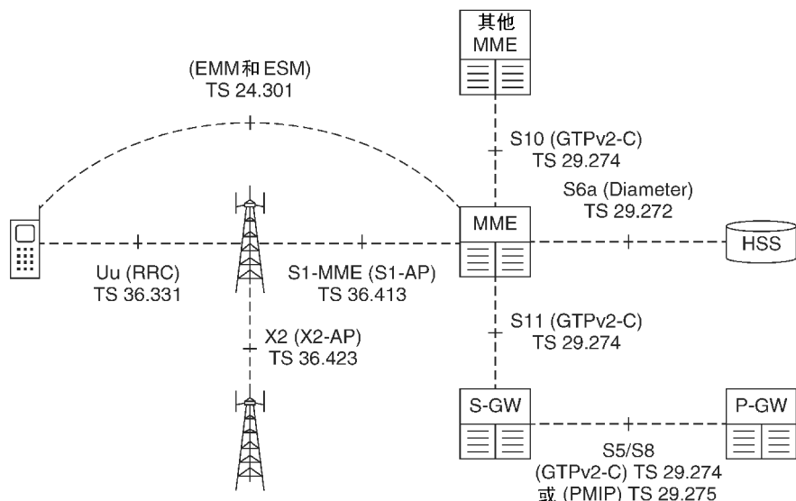
图 2.15 LTE 所使用的协议
