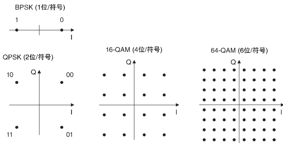
图 3.3 LTE 所使用的调制方案
