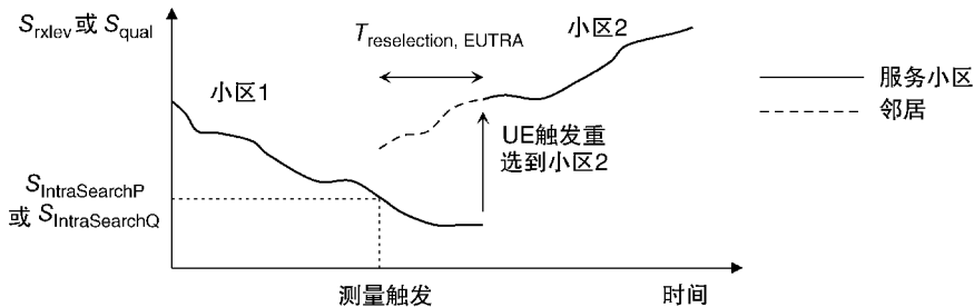
图 14.4 频率内小区重选
