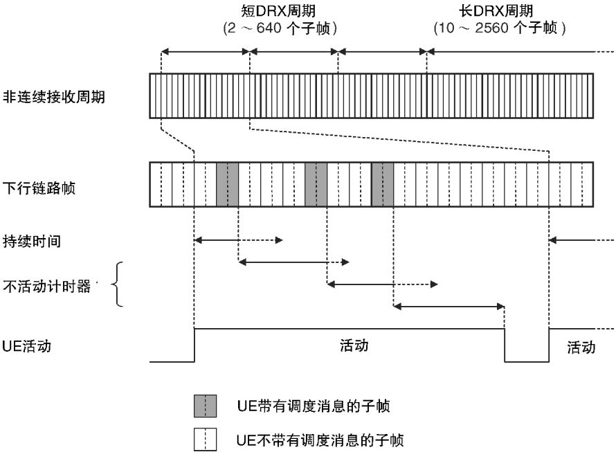
图 8.13 RRC_CONNECTED 状态下的非连续接收的操作
