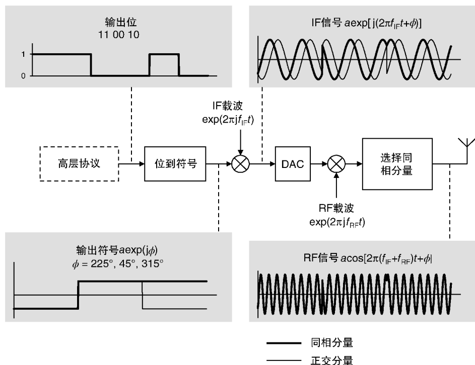
图 3.4 无线通信系统中的调制器的框图
