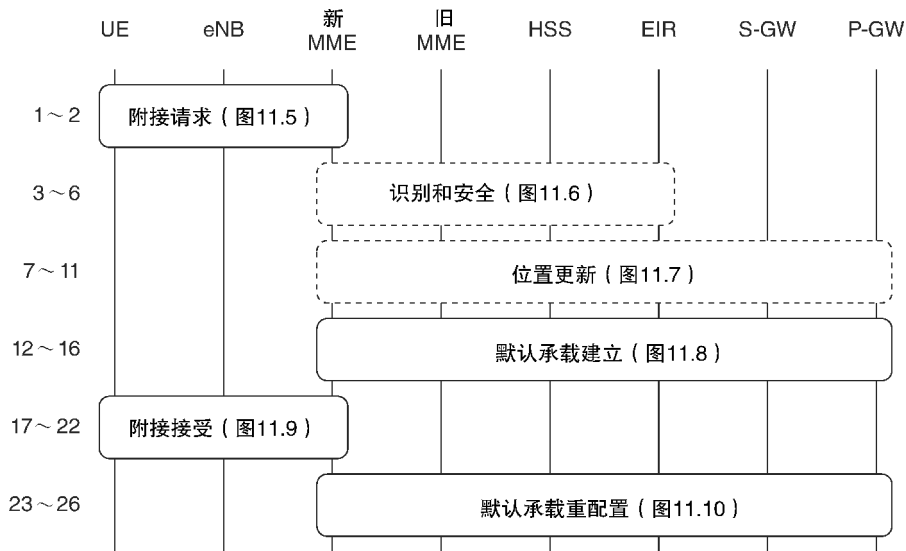
图 11.4 附着过程概述
