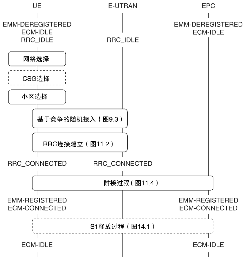
图 11.1 移动台上电过程概述
