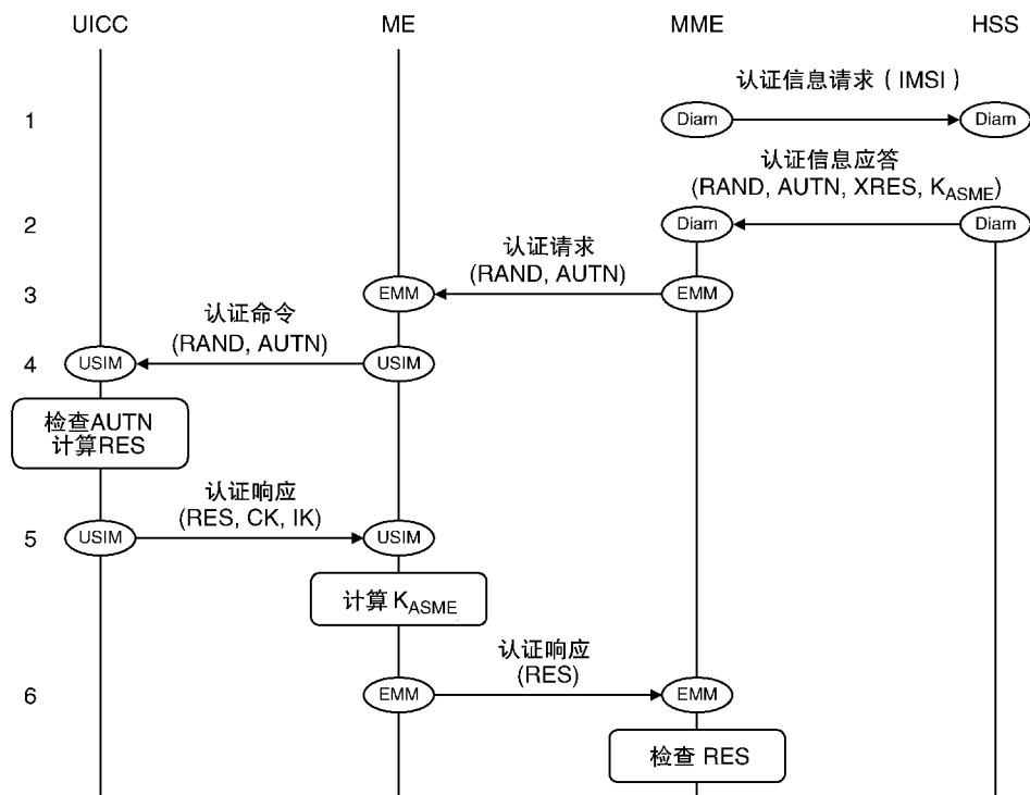
图 12.3 认证和密钥协商过程
