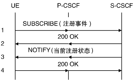
图 22.11 订阅未来移动台注册状态的通知 (来源: TS 24.228。经 ETSI 许可转载)
