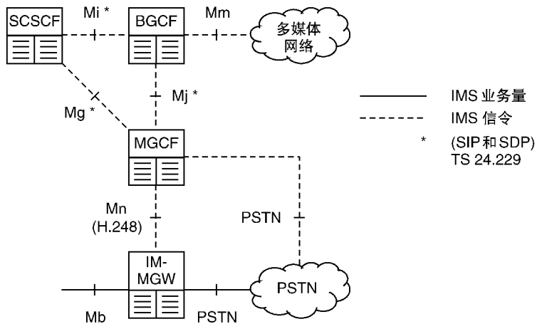
图 22.4 IMS 媒体网关架构
