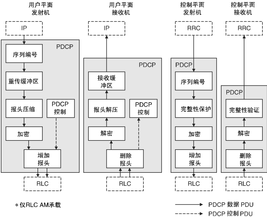
图 10.9 PDCP 的架构
