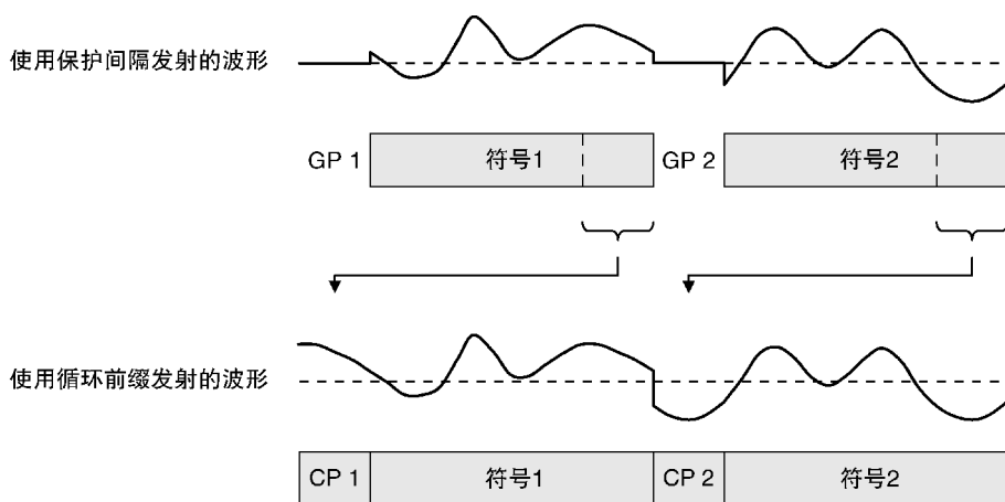
图 4.8 循环前缀插入的操作
