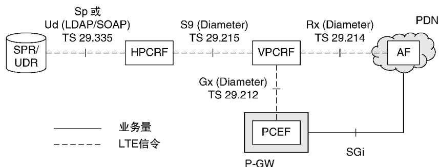
图 13.3 策略和计费控制架构, 基于 GTP 的 S5/S8 接口和使用本地疏导的漫游 (来源: TS 23.203。经 ETSI 许可转载)
