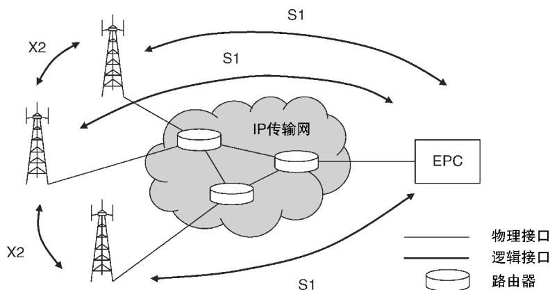
图 2.4 E-UTRAN 传输网的内部架构
