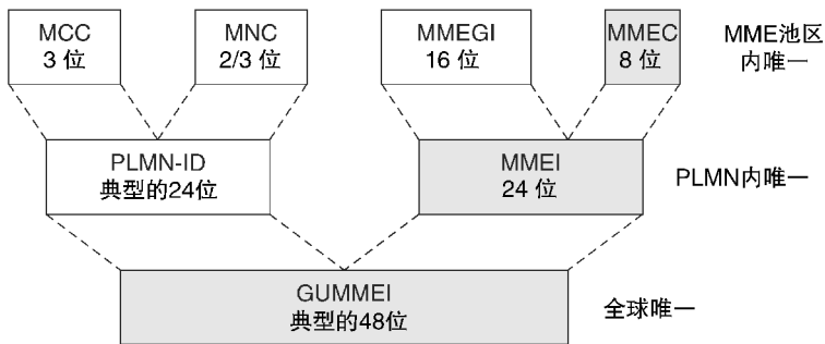
图 2.8 MME 使用的标识
