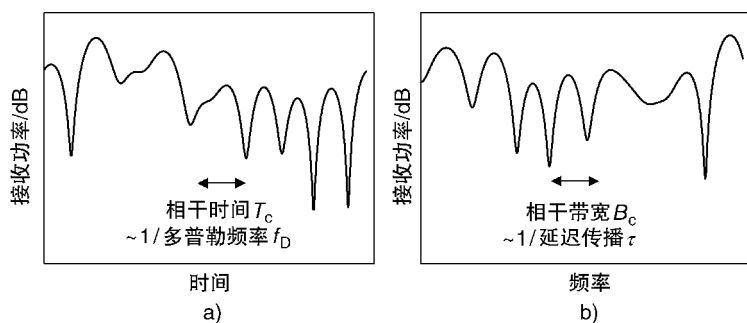
图 3.10 衰落作为时间和频率的函数
