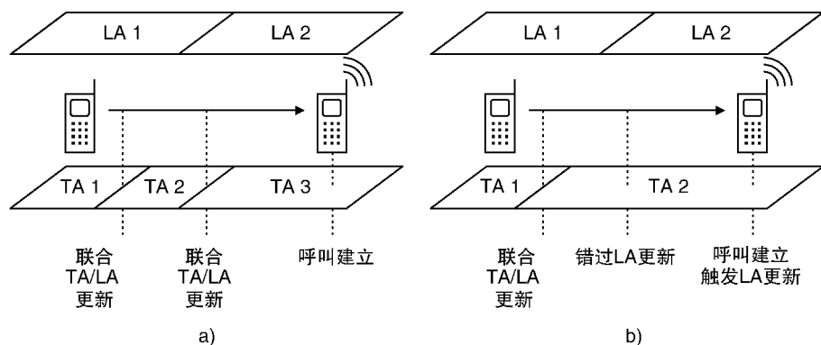
图 21.7 跟踪区域和位置区域的对齐
