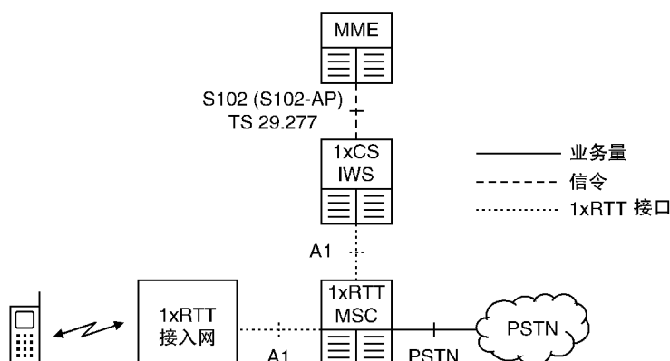
图 21.14 电路域回落到 cdma2000 1xRTT 的架构（来源：TS 23.272。经 ETSI 许可转载）
