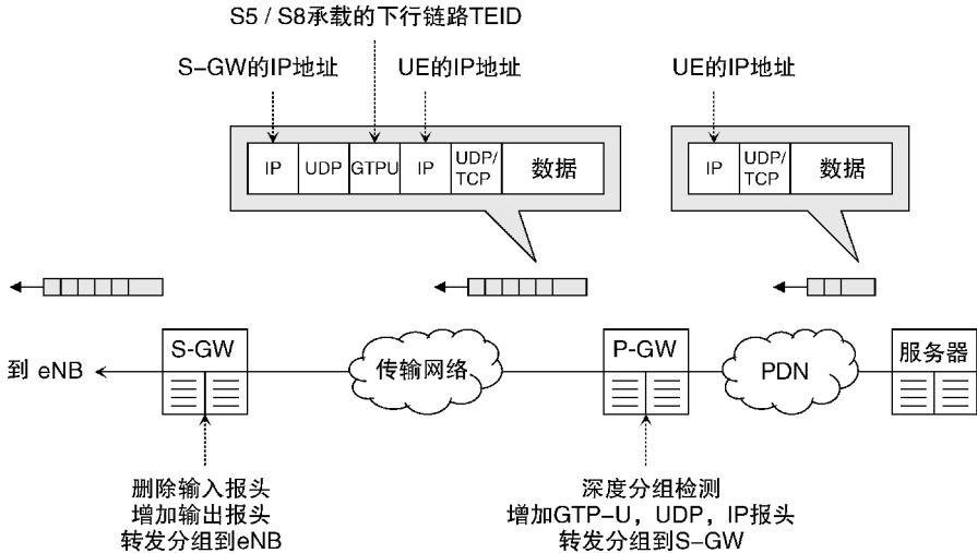
图 13.11 使用 GTP 在 S5/S8 接口上进行分组转发
