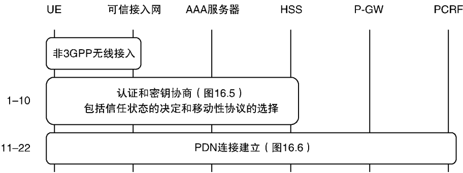
图 16.4 非 3GPP 接入网的附着过程的概述
