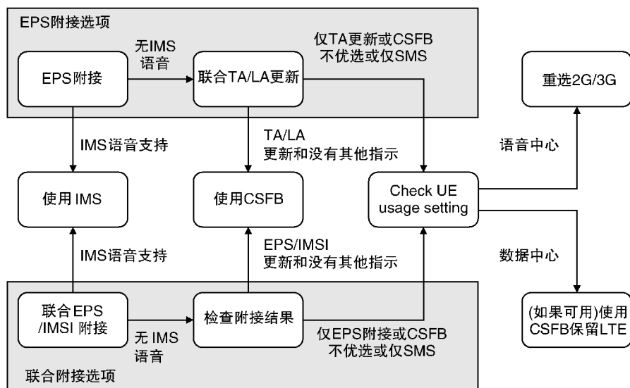
图 22.14 其语音域优选是 IMS 语音优选/CS 语音辅助的移动台的行为
