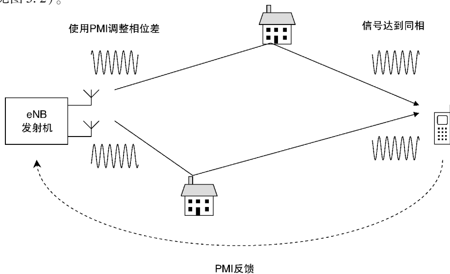
图 5.2 闭环发射分集的操作
