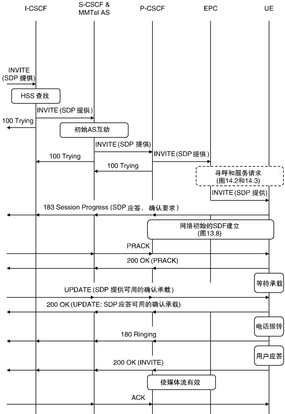
图 22.13 IMS 会话发起过程。(2) 终接网络中的消息 (来源: TS 23.228。经 ETSI 许可转载)
