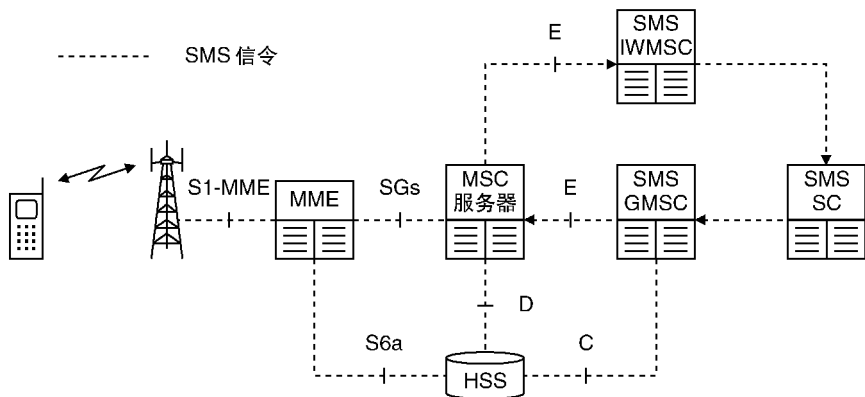
图 21.12 基于 SGs 的 SMS 架构
