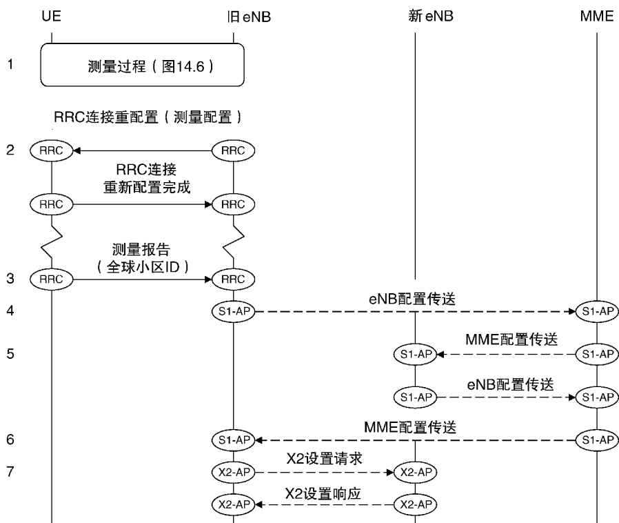
图 17.1 自动邻居关系过程
