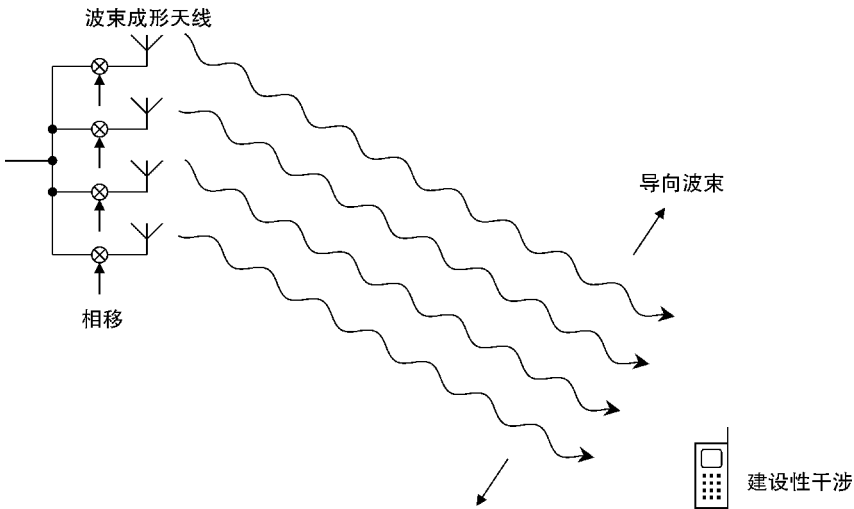
图 5.11 使用一组相移的波束控制
