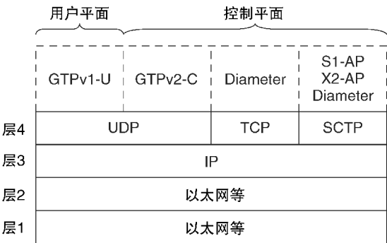
图 2. 13 固网的传输协议
