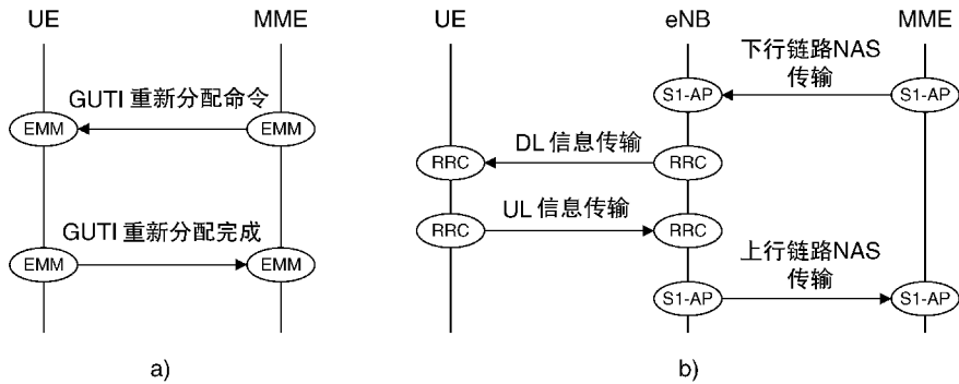
图 2. 18 GUTI 重新分配的过程 a) 非接入层 b) 接入层
