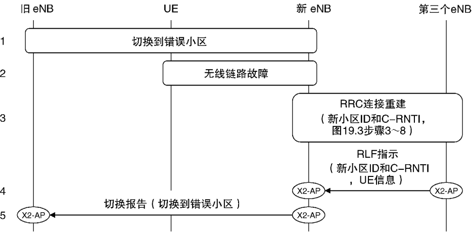
图 17.5 移动性鲁棒优化，由切换到错误的小区触发
