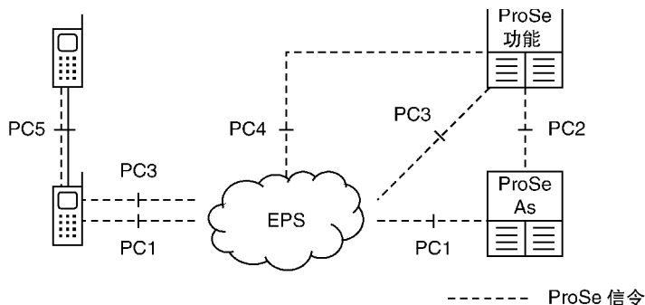
图 20.6 LTE 接近服务的架构
