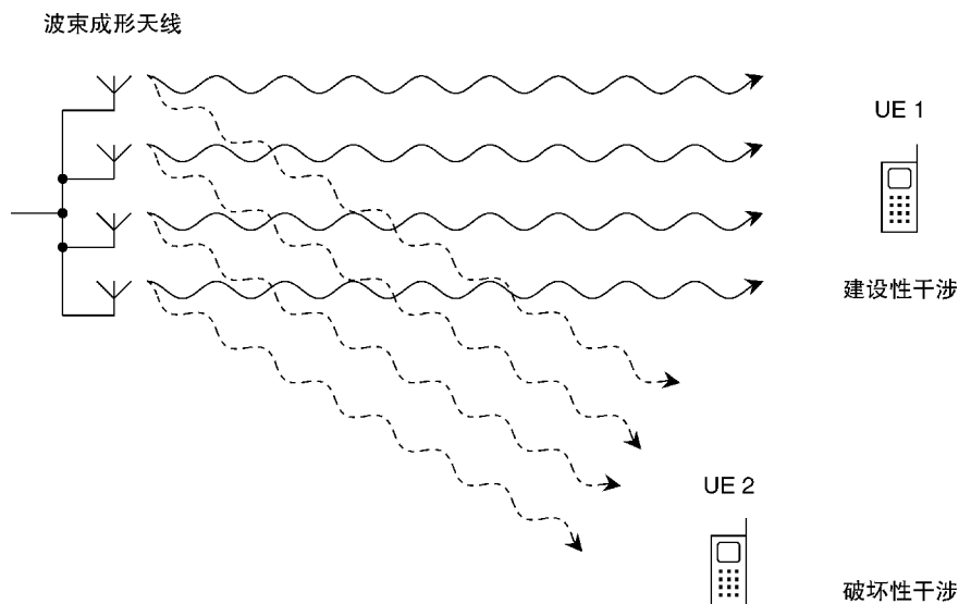
图 5.10 波束成形的基本原理
