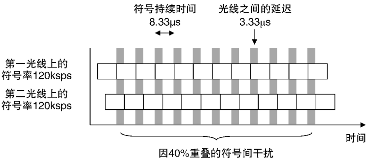
图 3.11 在多径环境中符号间干扰的产生
