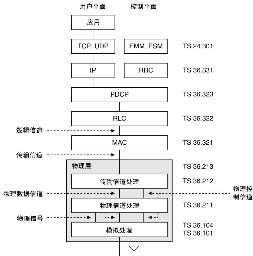
图 6.1 空中接口协议栈的架构
