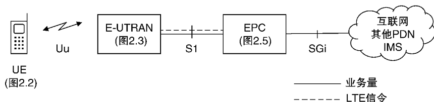
图 2.1 LTE 的高层体系架构
