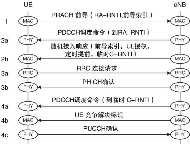
图 9.3 在 RRC 连接建立期间使用的基于竞争的随机接入过程
