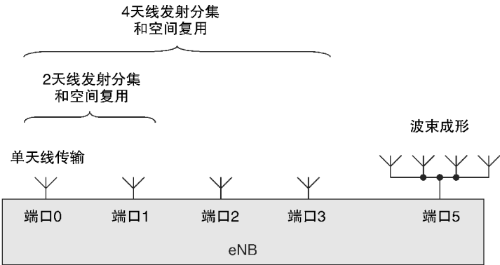
图 6.9 版本 8 基站使用的天线端口
