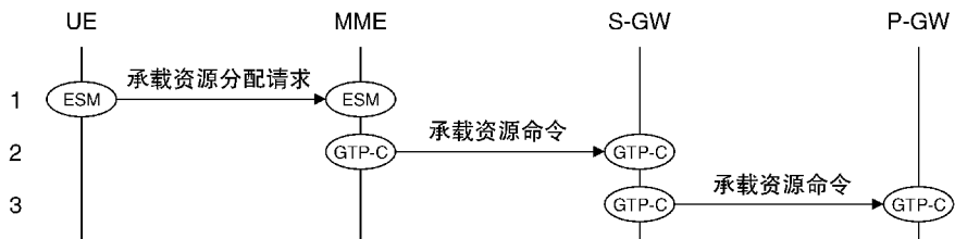
图 13.6 移动台发起的 SDF 建立过程。(1) 承载资源分配请求 (来源：TS 23.401。经 ETSI 许可转载)
