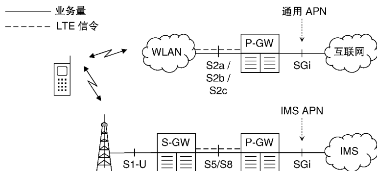
图 19.12 MAPCON 的示例网络架构
