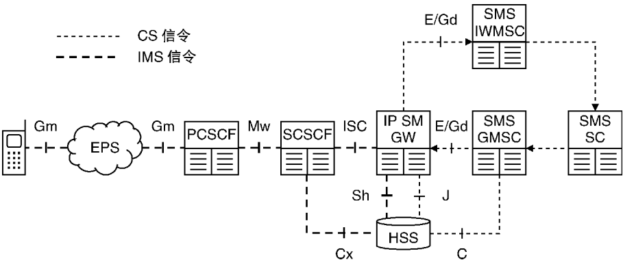
图 22.23 用于通过 IP 多媒体子系统传送 SMS 消息的架构 (来源：TS 23.204。经 ETSI 许可转载)
