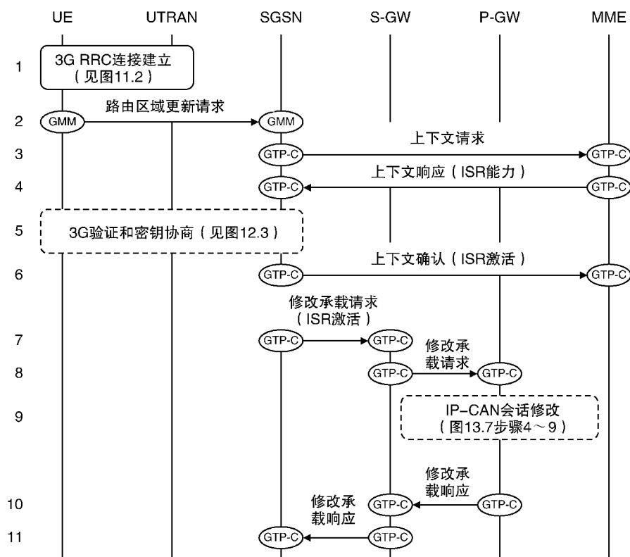
图 15.4 从 MME 到基于 S3/S4 的 SGSN 的路由区域更新，保留服务网关。
