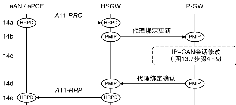
图 16.10 从 LTE 到 cdma2000 HRPD 的系统间切换。
