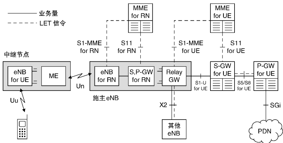
图 19.6 LTE 中继架构
