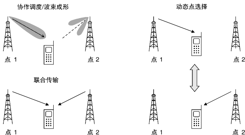
图 20.3 多点协作传输技术
