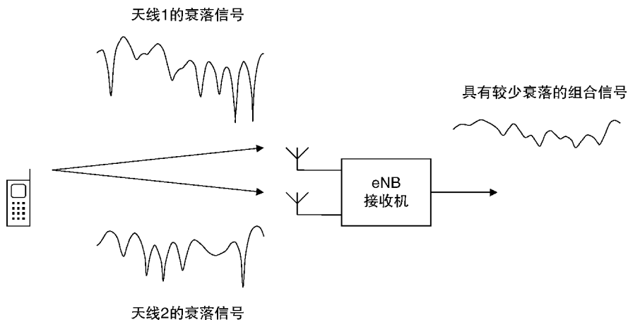
图 5.1 通过分集接收机的使用减少衰落
