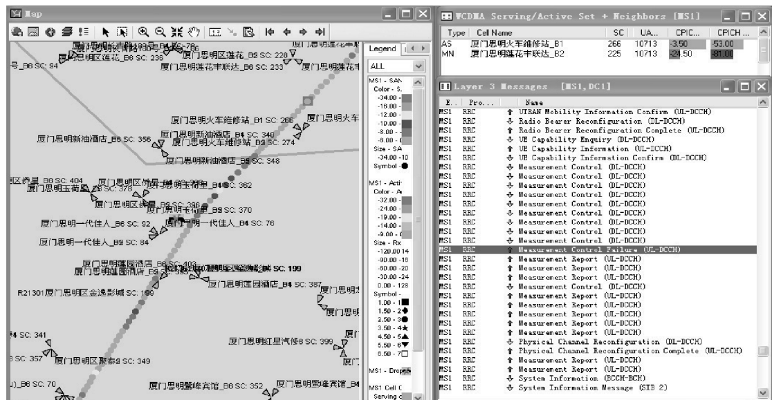
图 6-1 迁移过程中掉话
