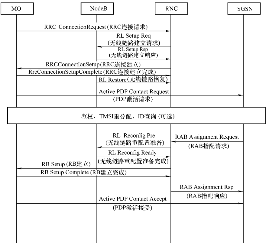
图 3-11 HSDPA 业务的信令流程
