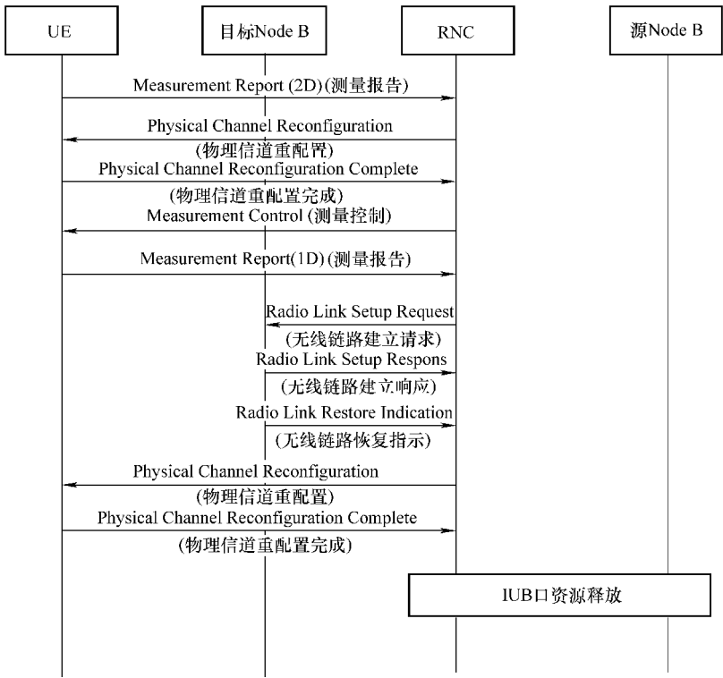
图 3-17 异频硬切换信令流程
