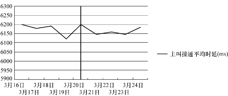
图 8-8 主叫业务建立时延变化
