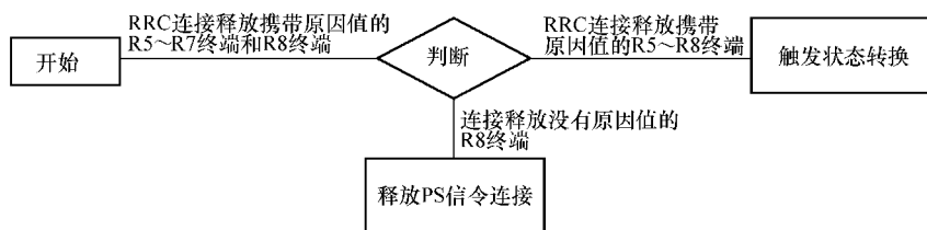
图 7-14 快速休眠原理
