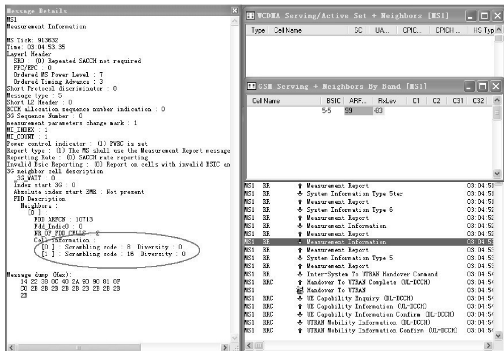
图 5-5 2G 中下发 3G 邻区
