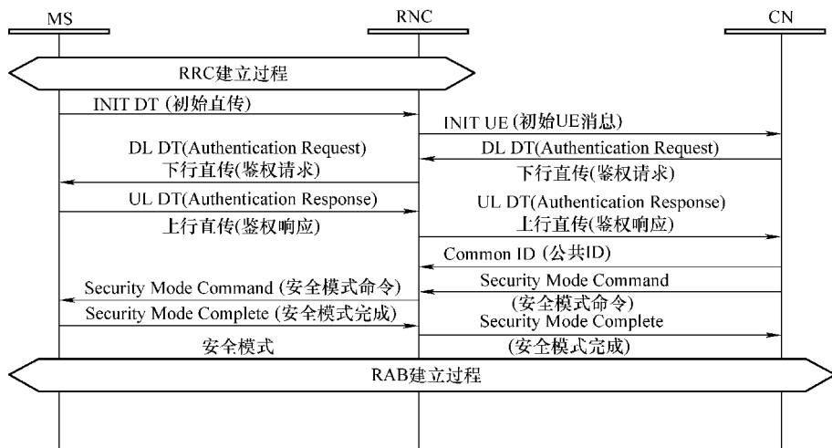
图 3-4 直传消息信令流程
