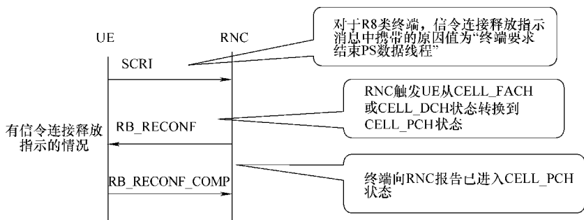
图 7-15 快速休眠信令流程
