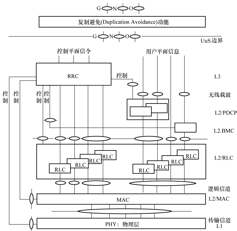
图 2-2 UU 口的协议层
