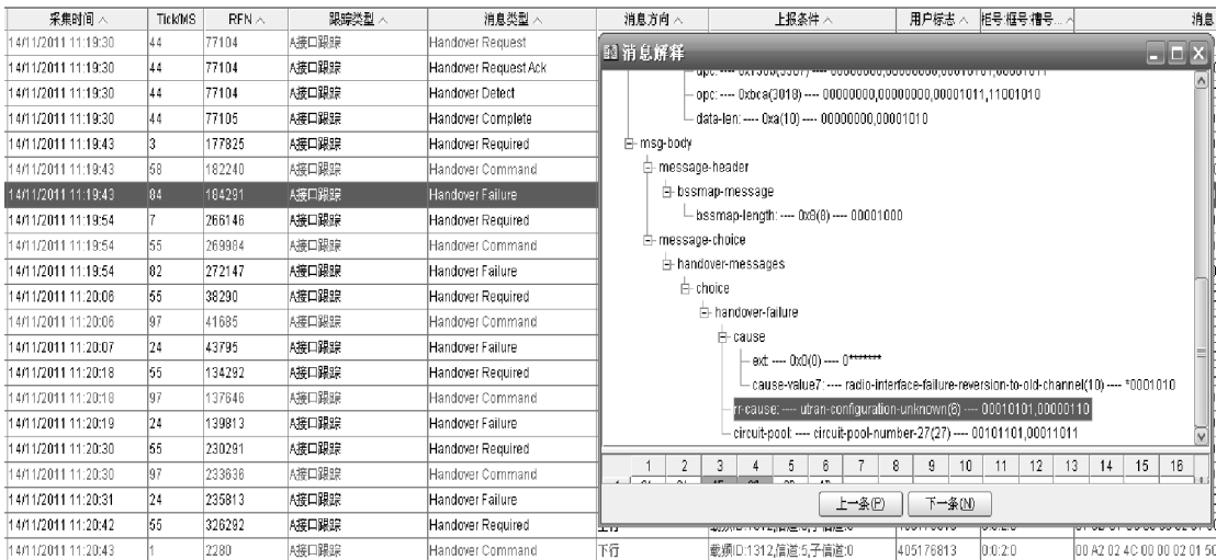
图 5-12 iPhone4 切换失败
