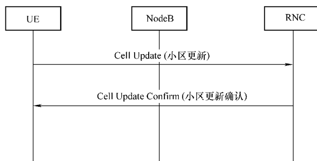
图 3-28 小区更新信令流程
