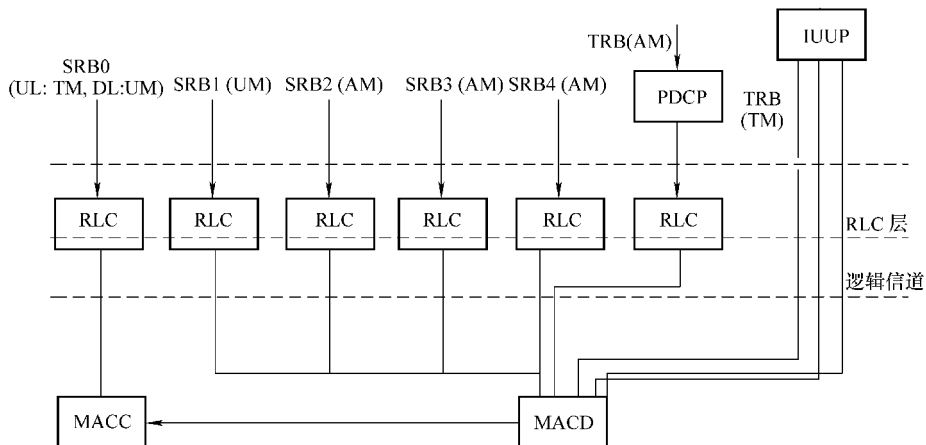
图 3-12 信令无线承载映射
