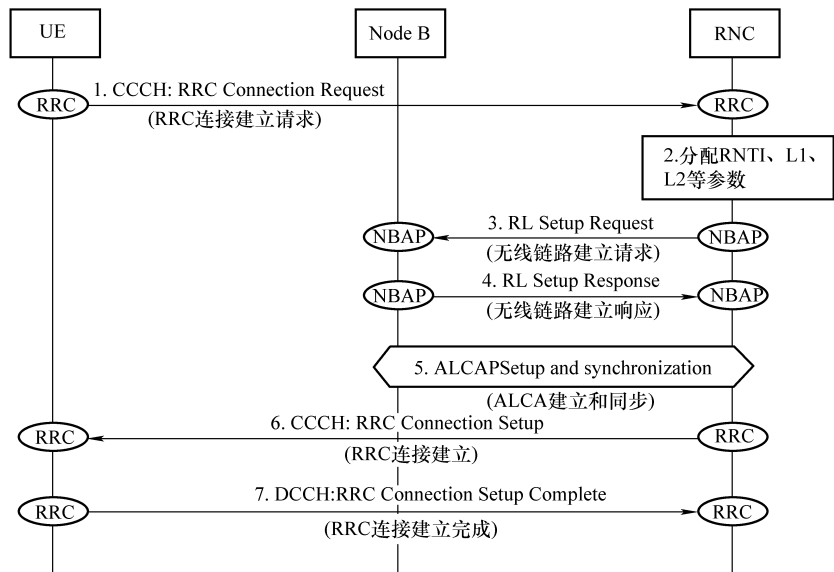
图 3-3 RRC 连接建立流程
