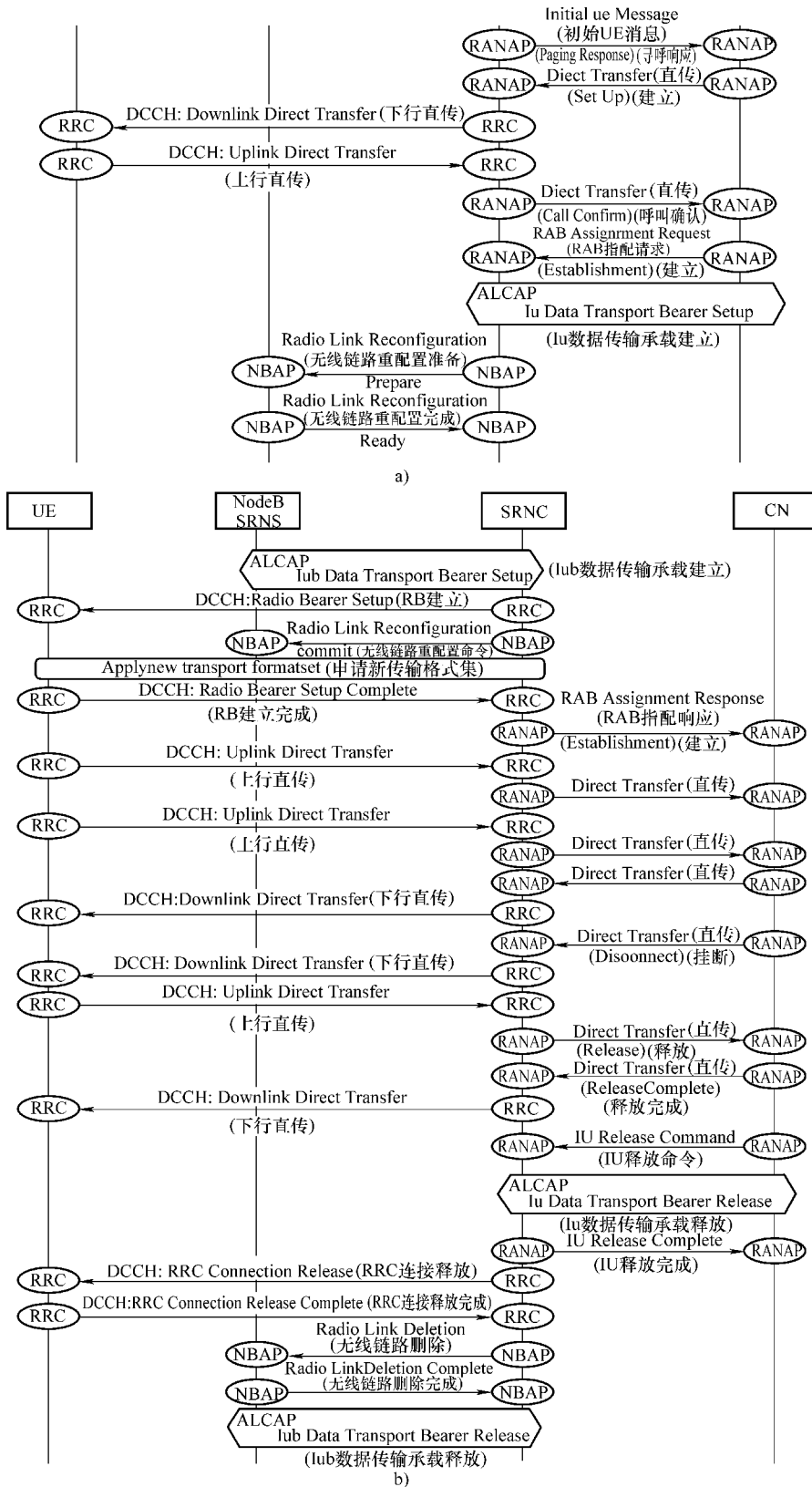
图 3-10 被叫信令流程 (续)
