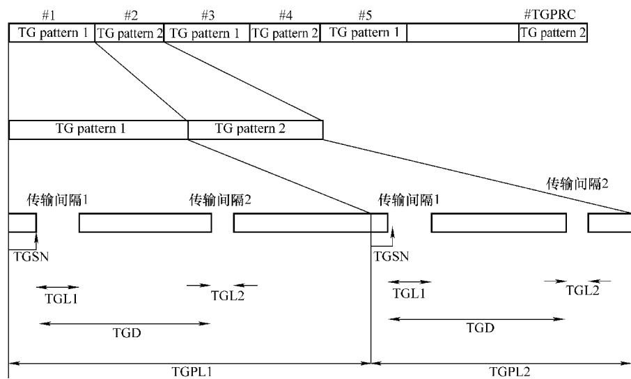
图 3-19 压缩模式传输格式
