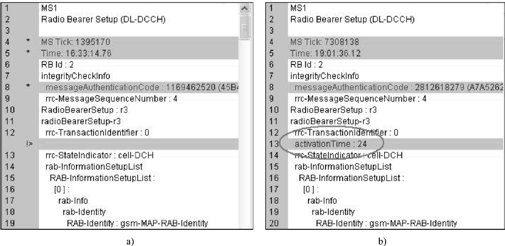
图 7-7 RB 建立消息 a) 之后 b) 之前
