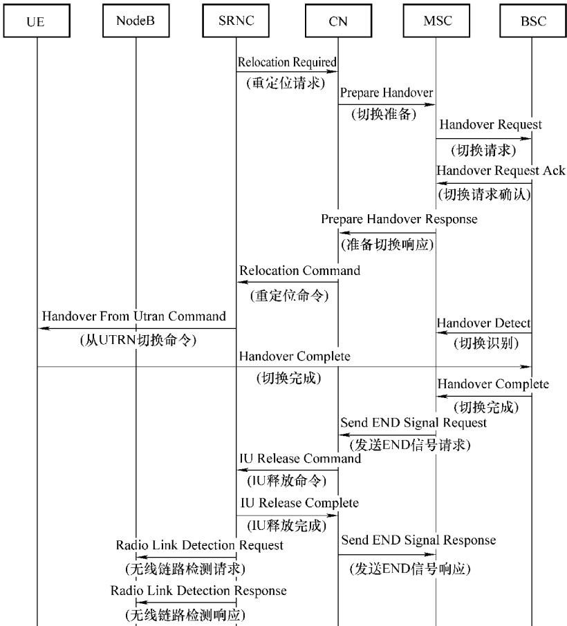
图 3-20 3G 到 2G 的电路域切换信令流程
