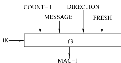
图 3-5 完整性保护算法原理
