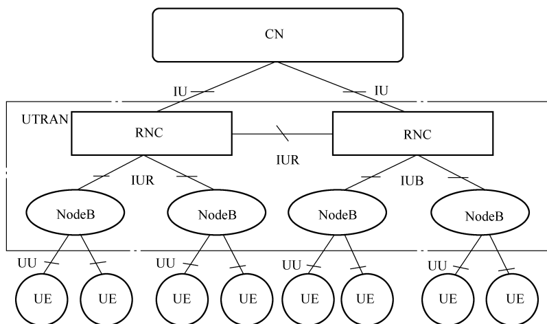
图 2-1 WCDMA 网络结构和接口
