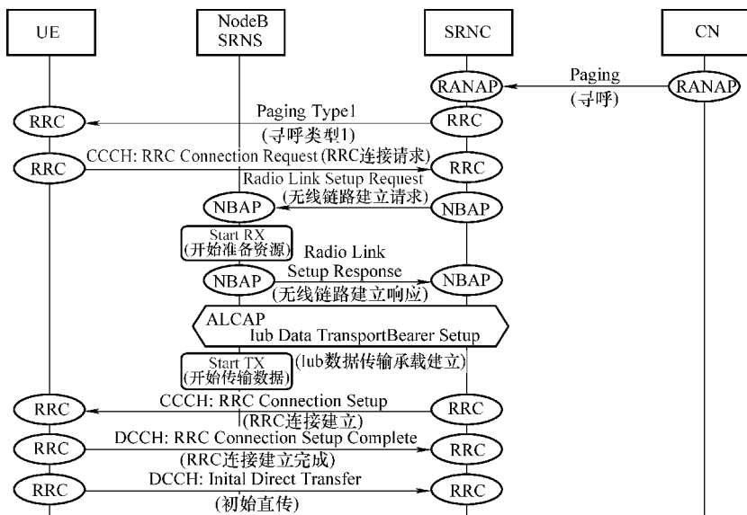
图 3-10 被叫信令流程
