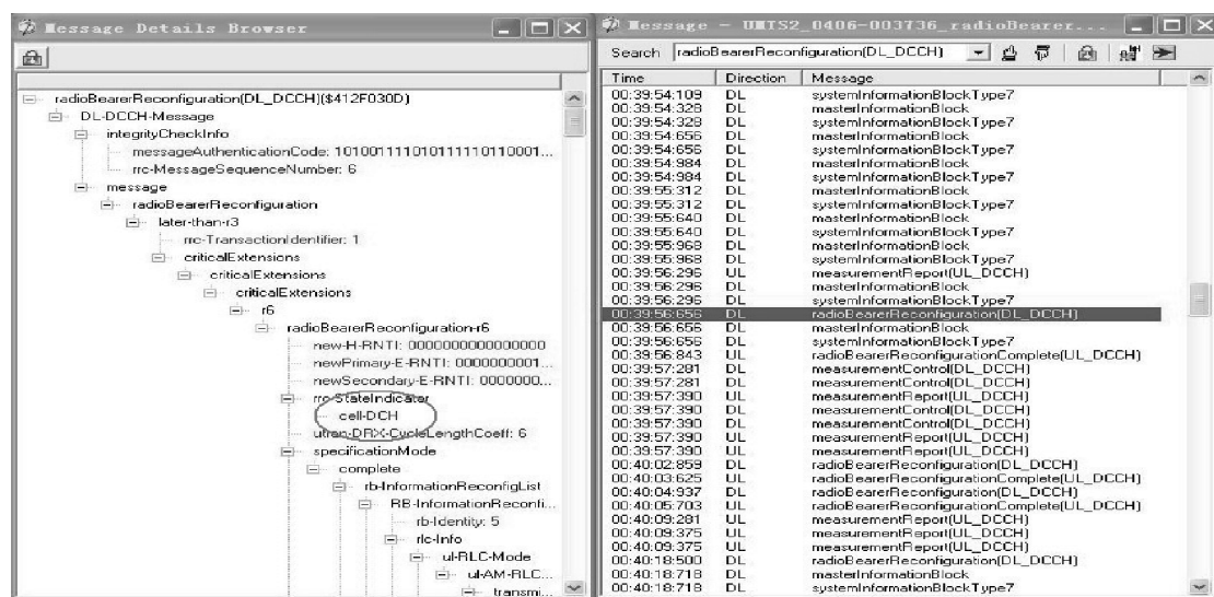
图 7-11 FACH 到 DCH 的信道转换
