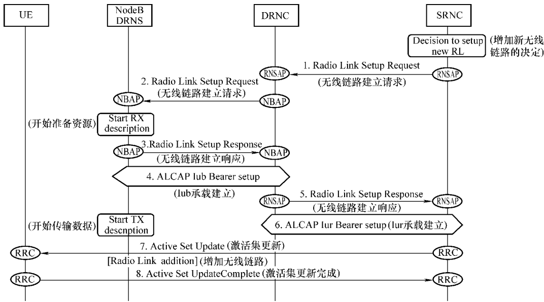
图 3-15 软切换信令流程
