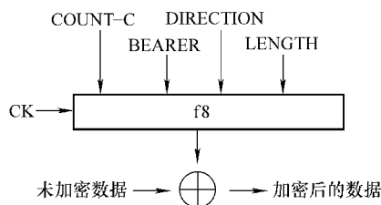
图 3-6 加密算法原理
