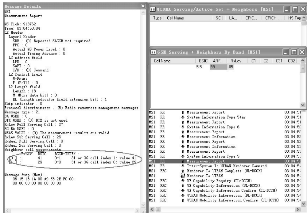
图 5-6 上报 3G 测量结果
