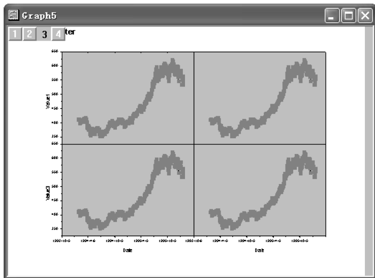
图 14-42 合并的图形
