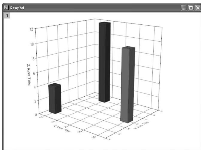
图 14-27 用转换后的矩阵绘制的 3D 棒图
