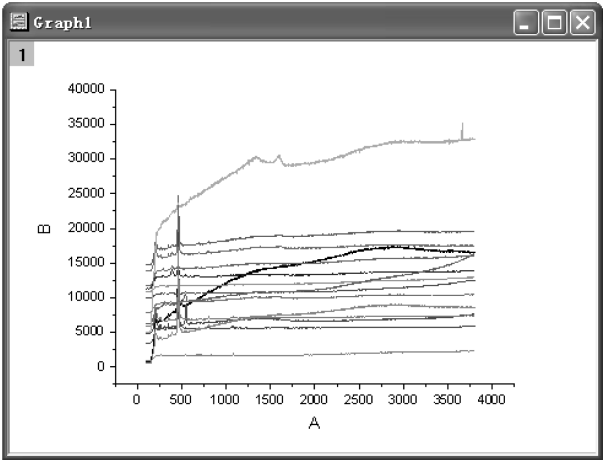
图 14-104 绘制线图
