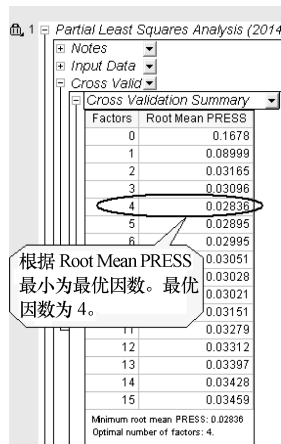
图 12-102 交叉验证 (Cross Validation) 表
