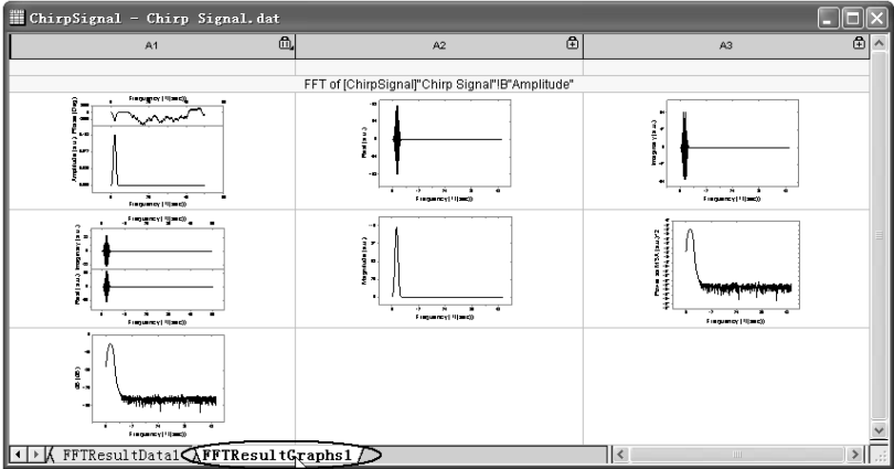
图 10-24 分析结果数据和图形
