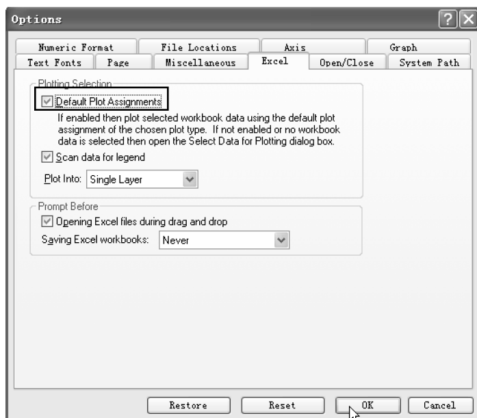
图 3-35 【Options】对话框
