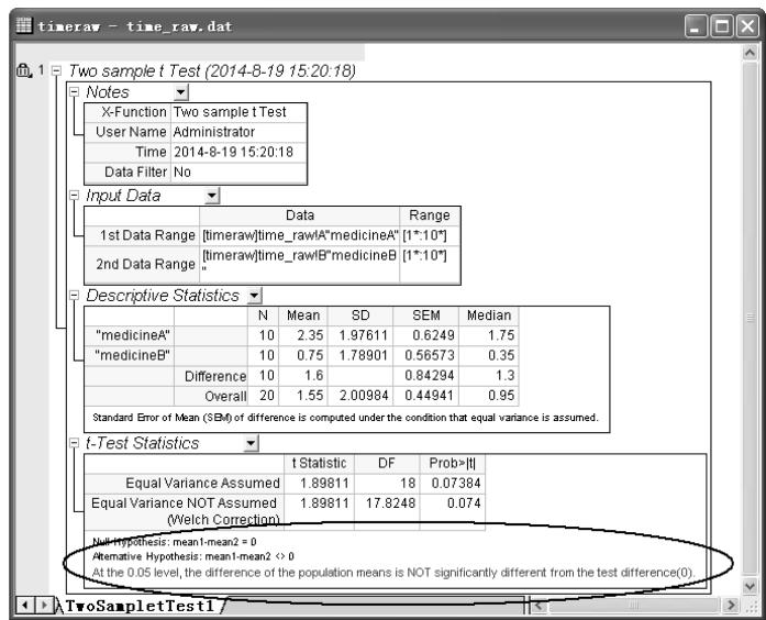
图 12-45 双独立样本 t 检验分析报告工作表
