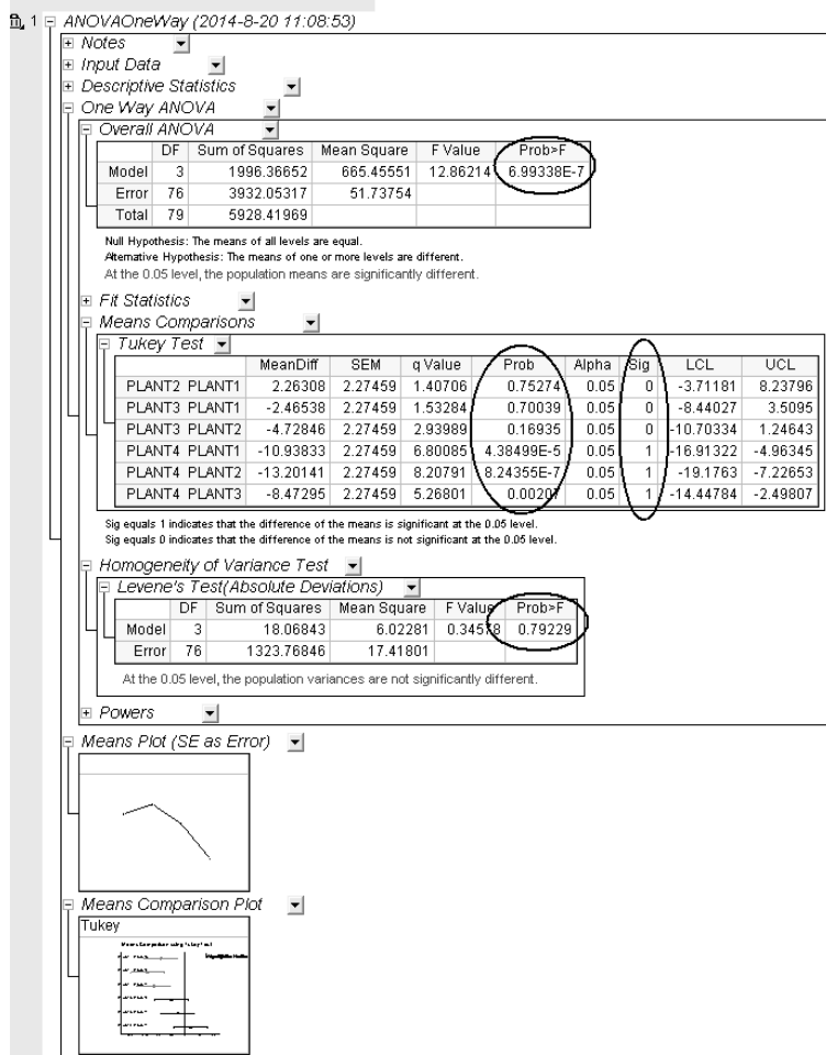
图 12-55 创建单因素方差分析报告
