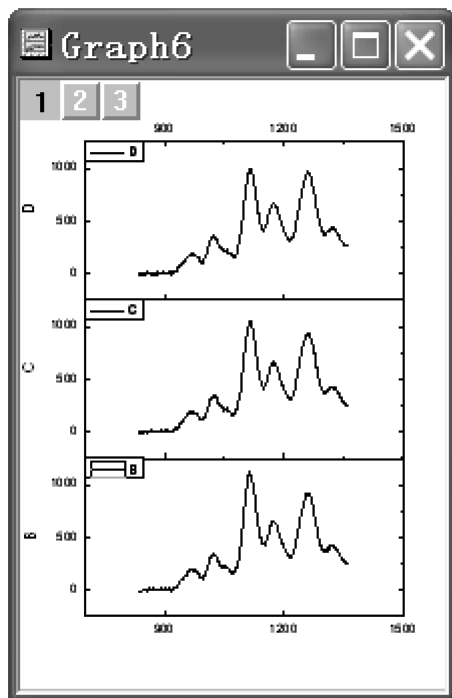
图 4-52 叠层图形
