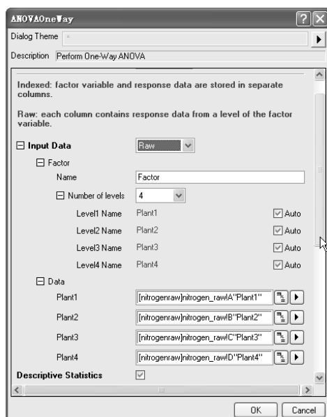
图 12-57 【ANOVAOneWay】对话框
