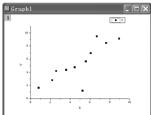
a) 散点图
