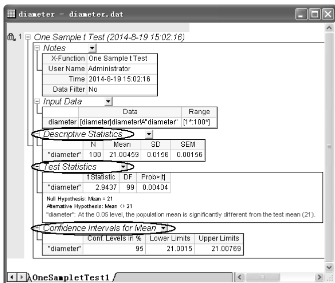
图 12-43 单样本 t 检验分析报告工作表
