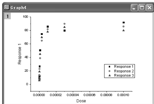
图 8-62 绘制散点图
