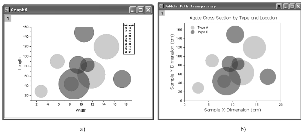
图 4-24 气泡图
