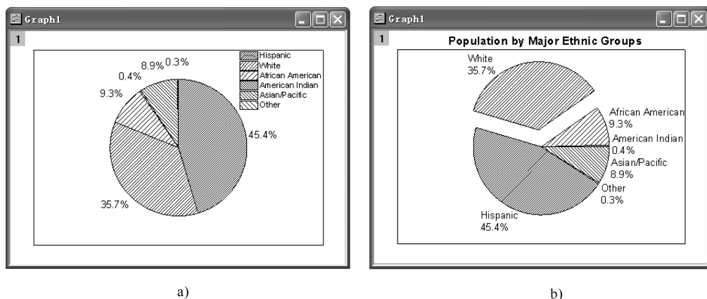
图 4-37 黑白饼图
