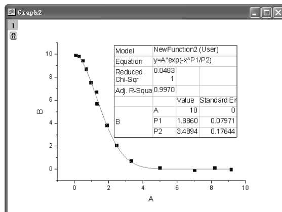
图 8-49 拟合结果
