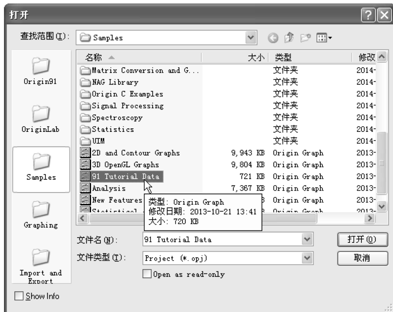
图 2-45 【打开】对话框
