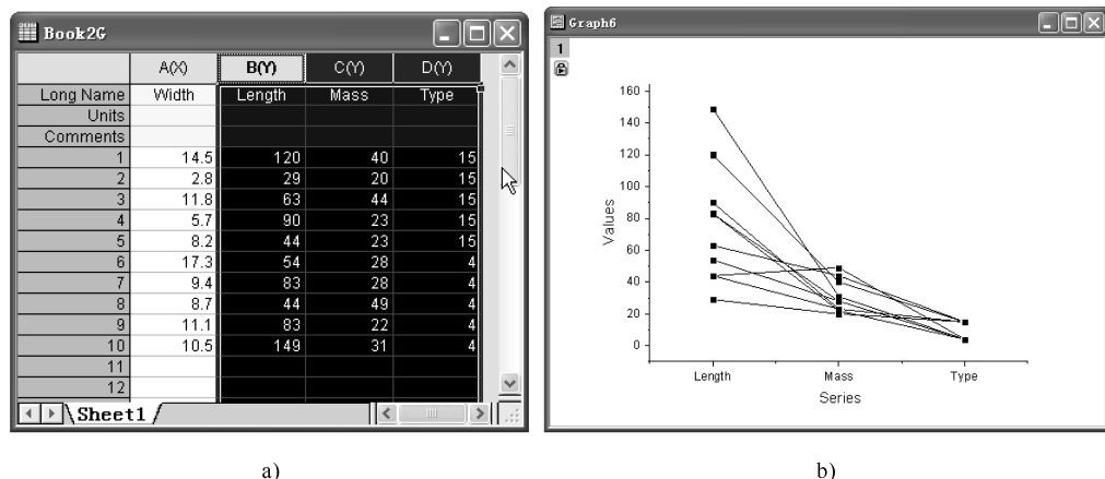
图 4-28 线列图
