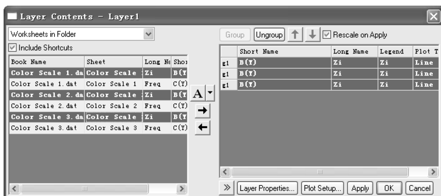
图 14-64 图层对话框
