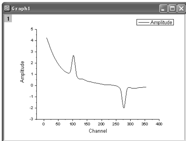
图 11-14 绘制的线图
