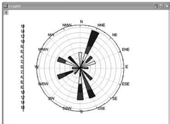
图 4-75 基本 Wind Rose-Bin 风场玫瑰图
