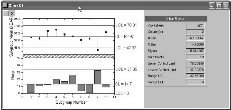
图 12-18 质量控制（QC）图
