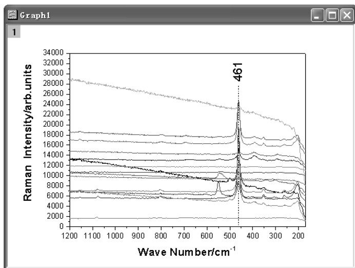
图 14-107 修改完成的 Micro-Raman 谱线图
