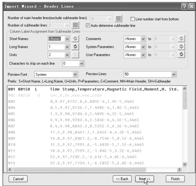
图 3-42 【Import Wizard-Header Lines】 页面
