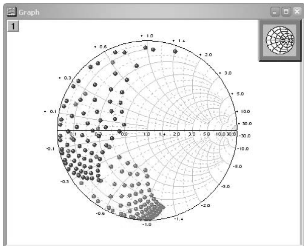
图 4-72 绘制出的史密斯圆图
