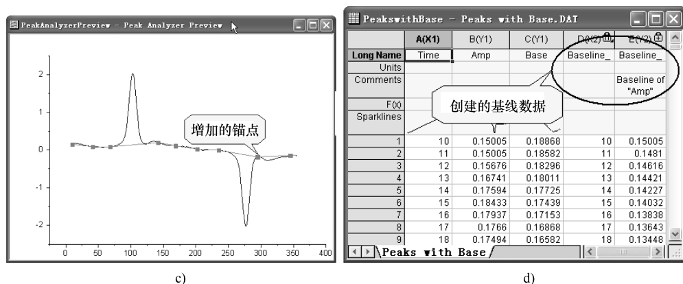
图 11-8 创建基线 (续)
