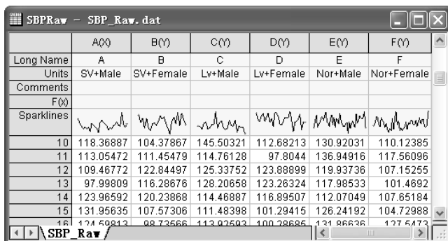
图 12-69 “SBP_Raw.dat”工作表
