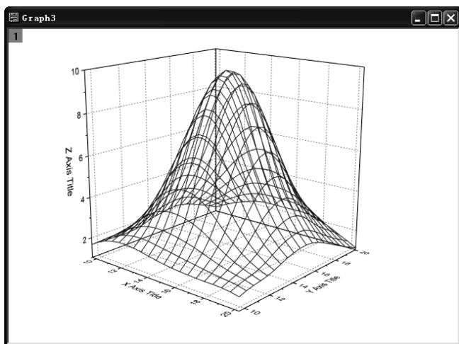
图 5-11 三维框线图
