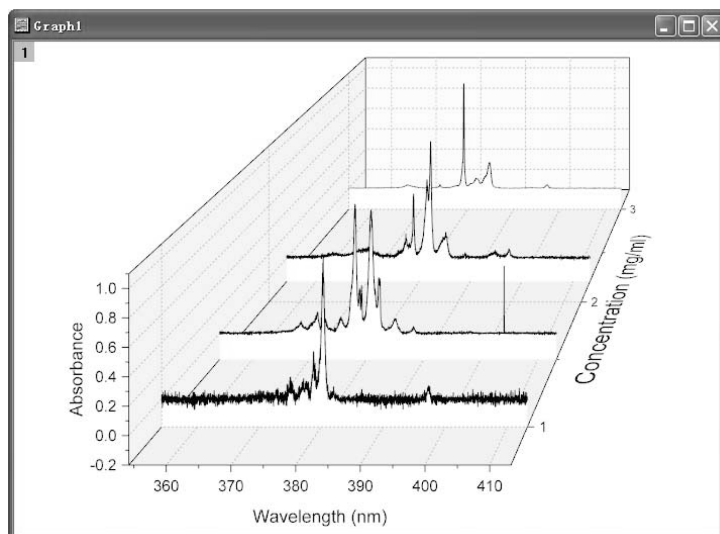
图 14-87 三维瀑布图
