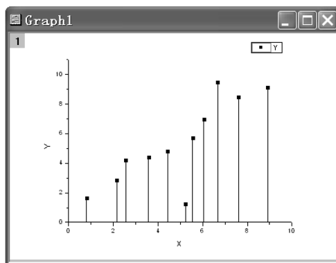
c) 垂线图
