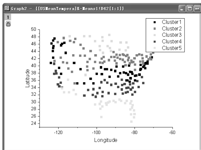
图 12-99 “Group Plots” 图
