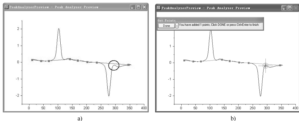
图 11-8 创建基线
