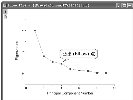
图12-84 “Scree plot”图
