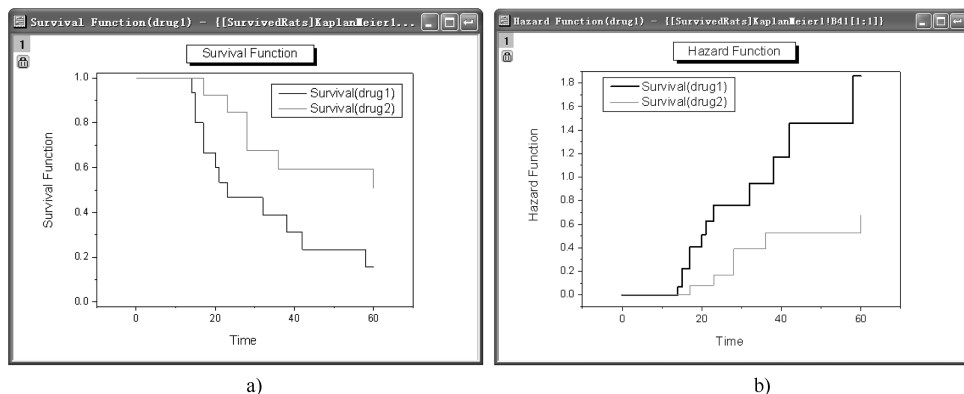
图 12-76 存活率函数图和风险函数图
