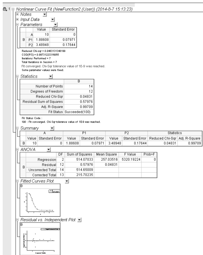
图 8-50 拟合报告
