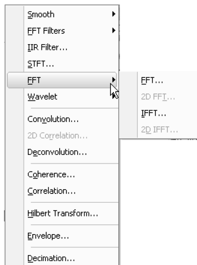
图 10-7 FFT 菜单
