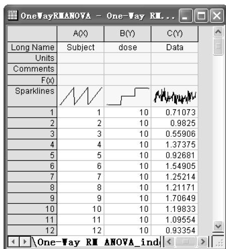
图 12-58 “One-Way_RM_ANOVA_indexed.dat” 工作表
