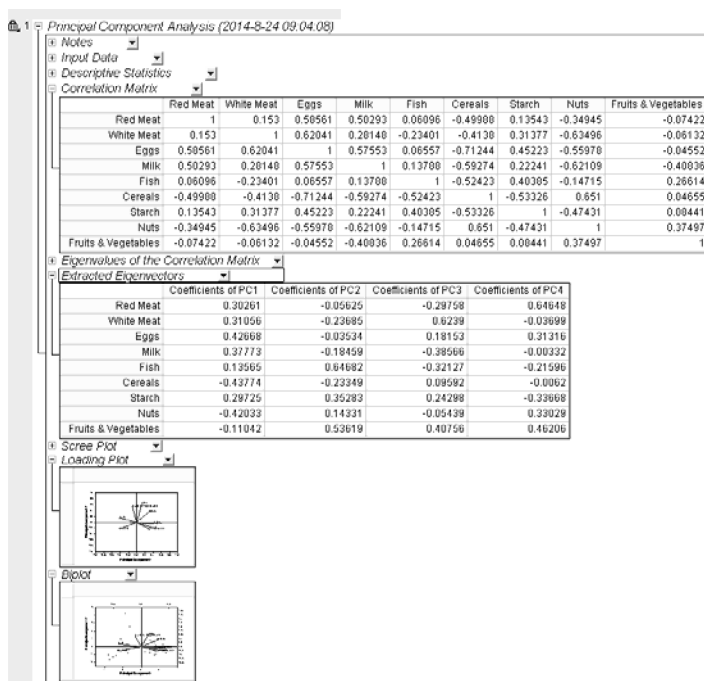
图 12-86 主成分分析报告
