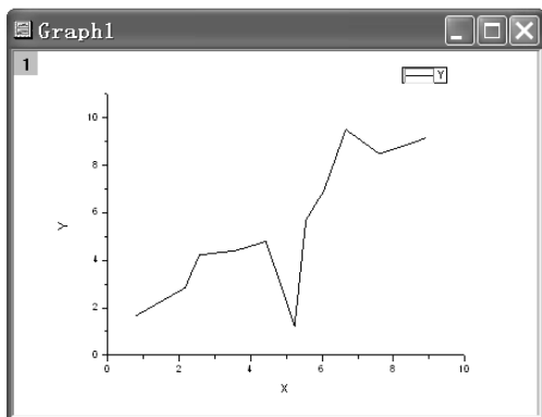
a) 线图
