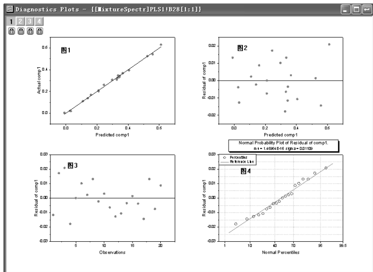
图 12-103 诊断图
