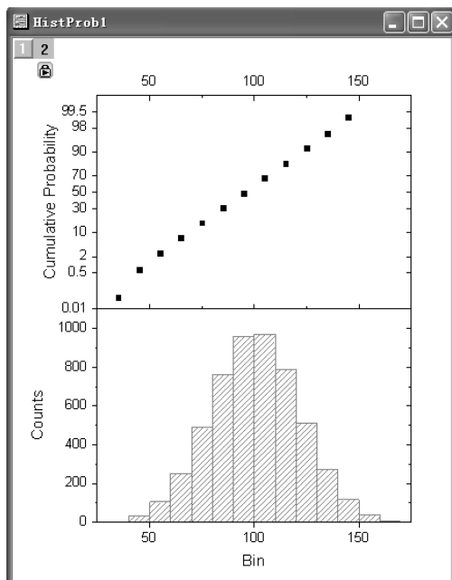
图 12-5 概率直方统计图
