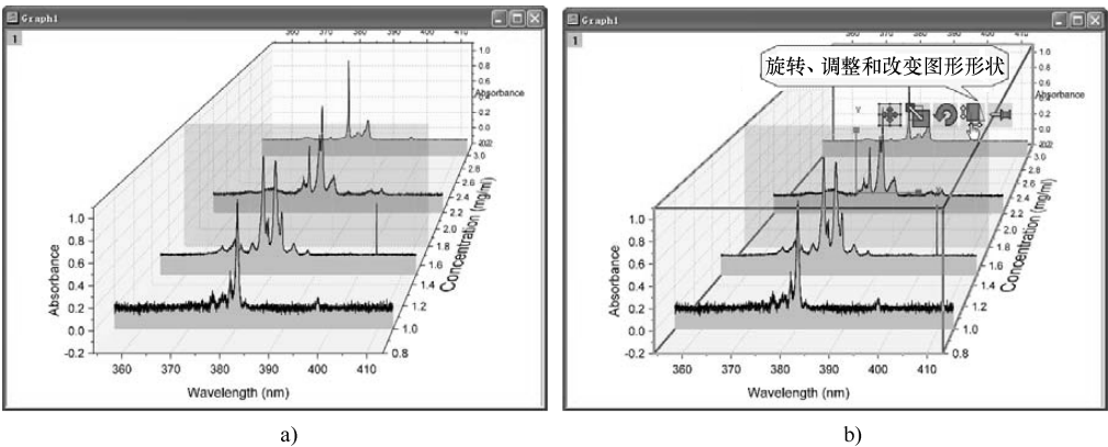
图 14-90 谱线三维瀑布图
