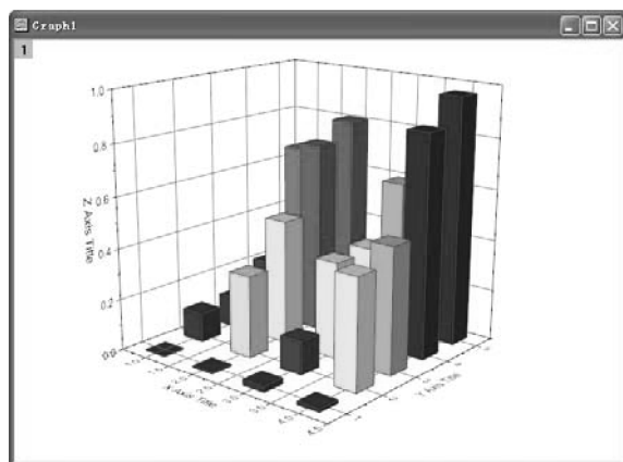
图 14-19 绘图结果
