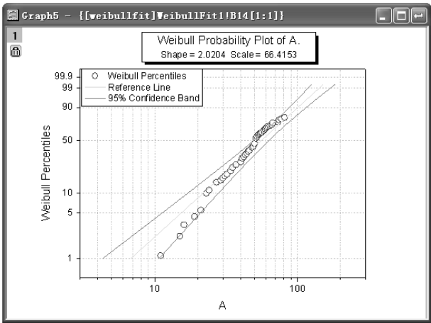
图 12-80 Weibull 概率图
