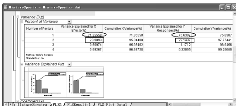
图 12-105 方差解释表
