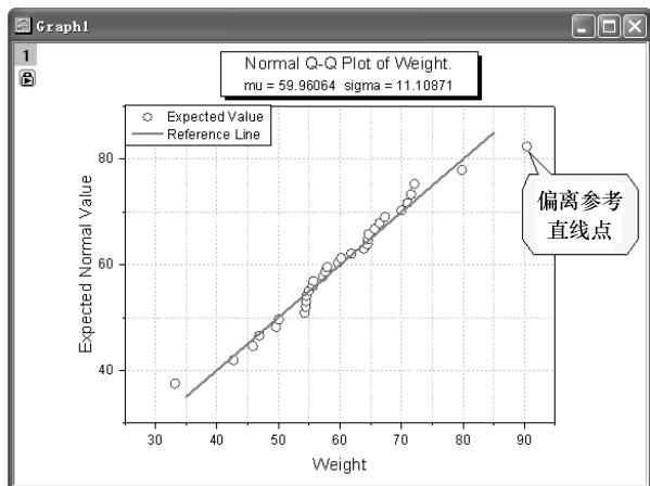
图 12-24 绘制 Q-Q 统计图
