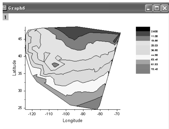
图 4-58 等值线图
