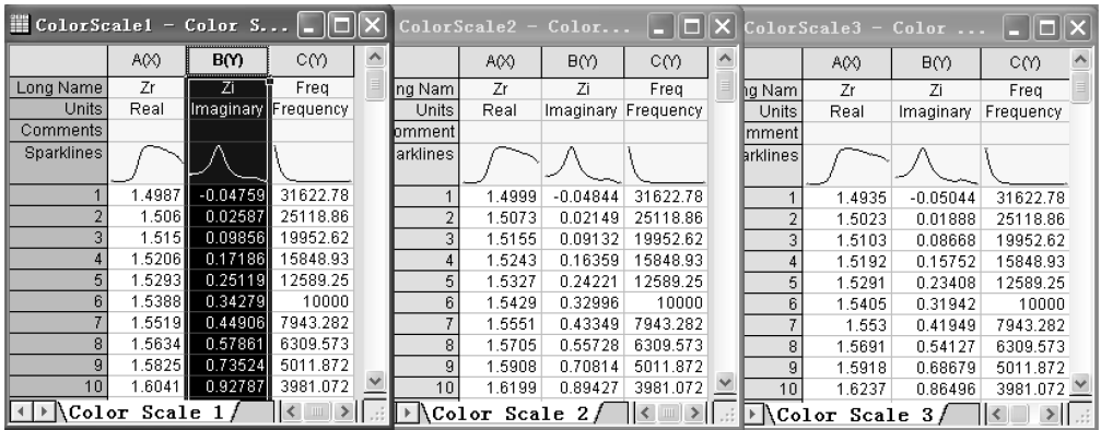
图 14-63 导入的 3 个工作表
