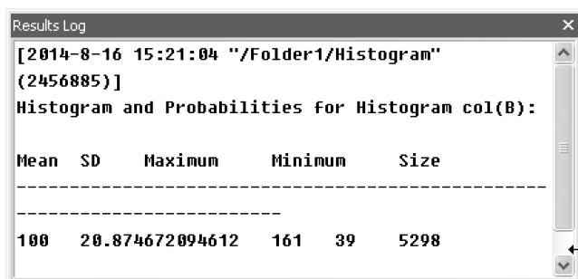
图 12-6 概率直方统计图的统计结果
