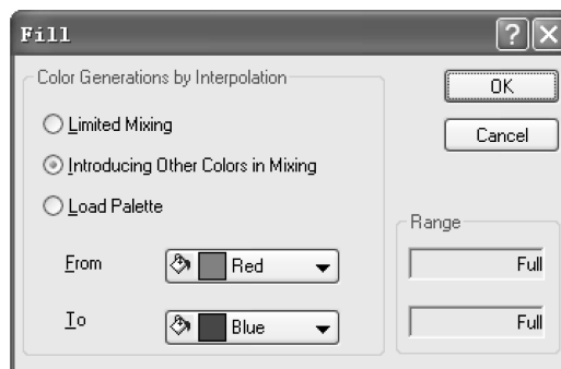
图 14-69 【Fill】对话框
