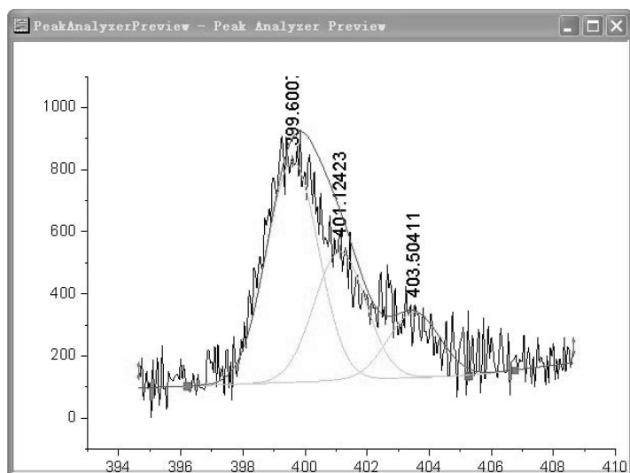
图 14-101 拟合曲线图
