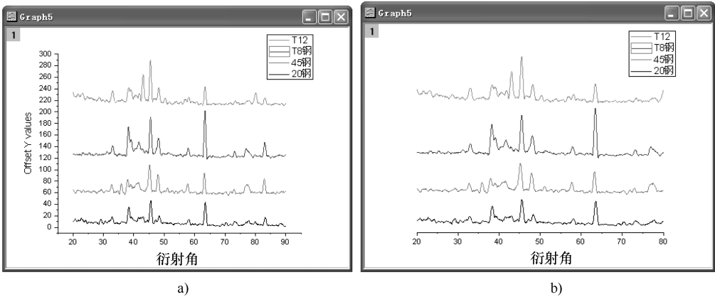
图 14-85 4 个样品的 XRD 谱线
