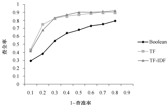
图 6-9 采用不同特征权重的分类效果
