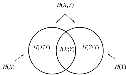
图 6-5 互信息和熵之间的关系示意图
