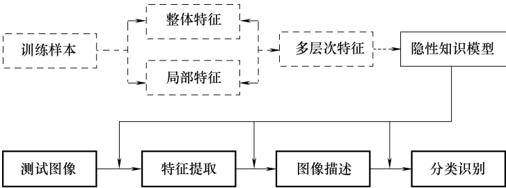
图 6-1 知识驱动的图像识别模型
