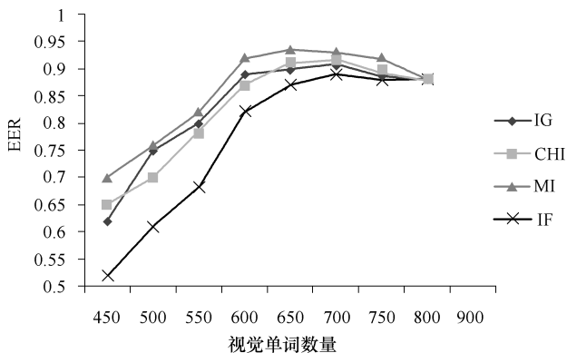
图 6-10 特征选择后的分类性能
