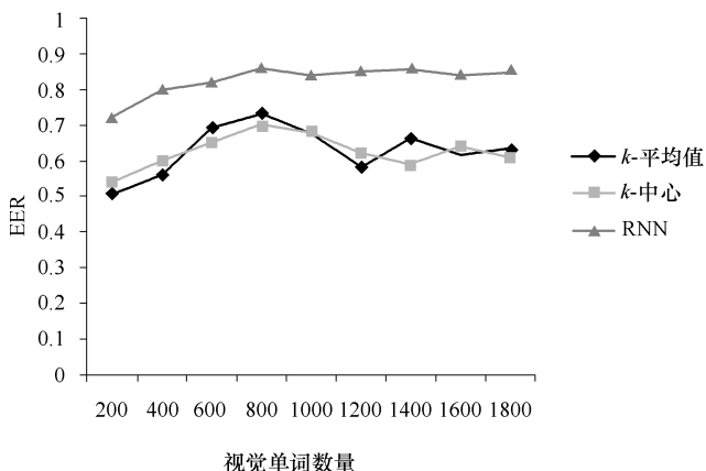
图 6-7 不同视觉单词库构造方法的性能
