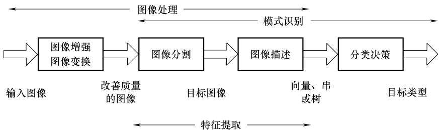
图 1-1 图像目标识别系统的基本框架图
