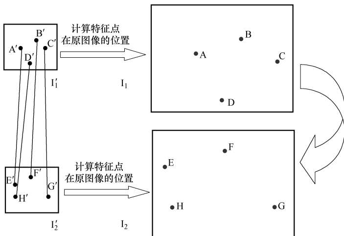
图 5-6 基于多分辨率技术的图像配准
