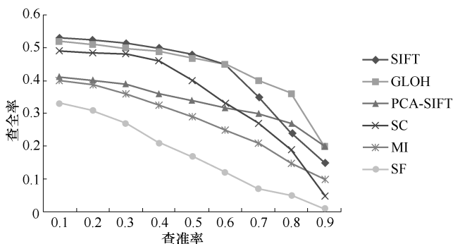
图 5-12 局部特征描述子的性能比较
