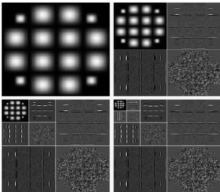
图 2-16 三个尺度下的二维小波变换
