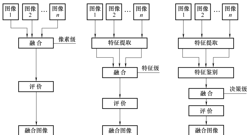
图 5-8 图像融合的层次
