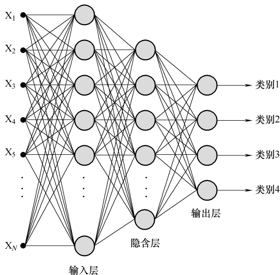
图 3-3 用于目标分类的三层 BP 网络
