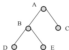
图 B-1 树
