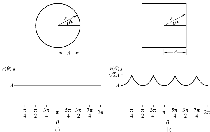
图 7-8 距离-角度的函数标记图
