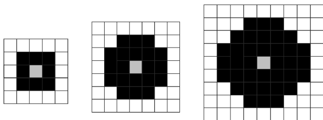
图 4-8 SUSAN 算法的模板
