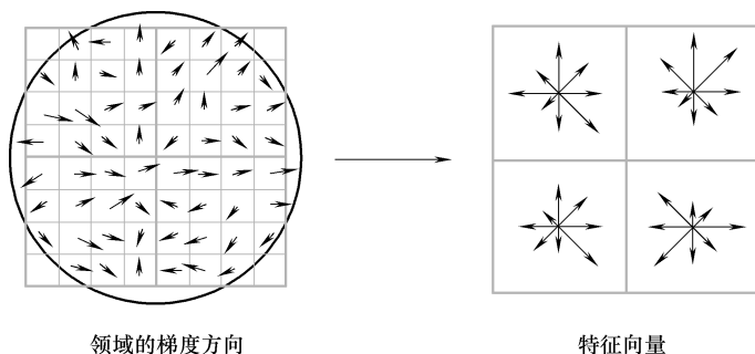
图 4-6 由邻域梯度信息生成特征向量
