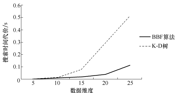
图 5-2 BBF 算法与 K-D 树的搜索时间代价
