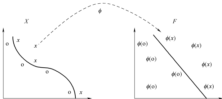
图 3-6 简化分类任务的特征映射
