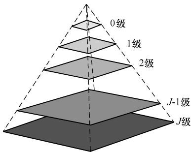
图 5-5 图像金字塔的结构
