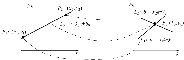
图 5-3 直线检测中的霍夫变换
