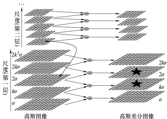
图 4-2 高斯金字塔和高斯差分金字塔的构造示意图
