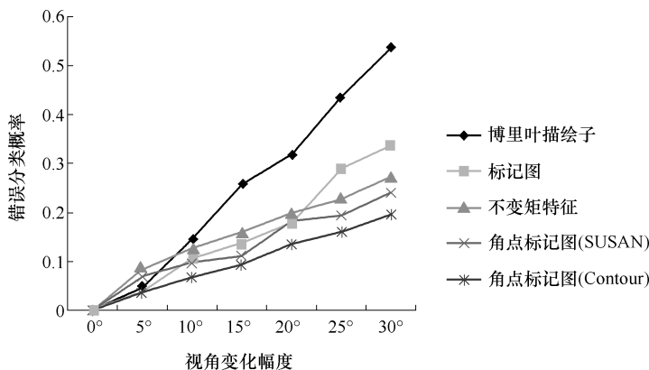
图 7-11 五种特征在视点变化下的识别效果
