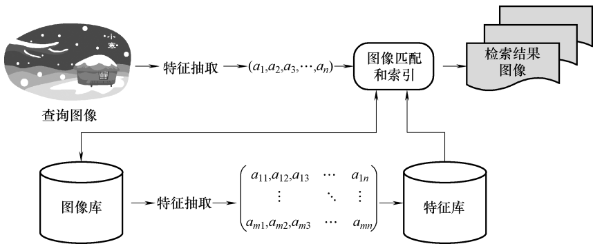
图 5-9 图像检索系统的结构流程（来源：杨红菊，2009 年）
