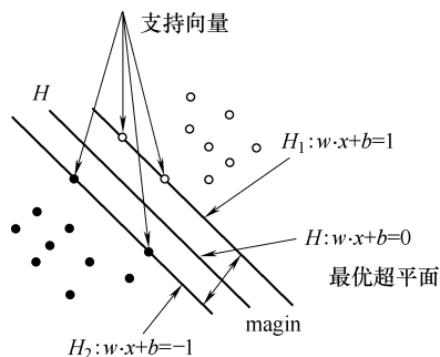
图 3-5 最优超平面
