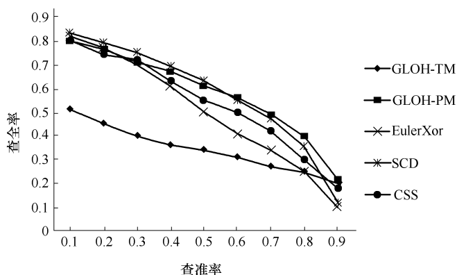
图 5-17 五种图像检索方法的性能比较
