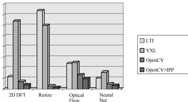
图 1-3 OpenCV 与其他视觉函数库的性能比较
