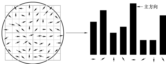
图 4-5 由梯度方向直方图确定主梯度方向
