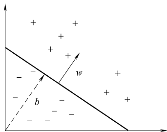
图 3-4 二维训练集的分开超平面 ( w, b )
