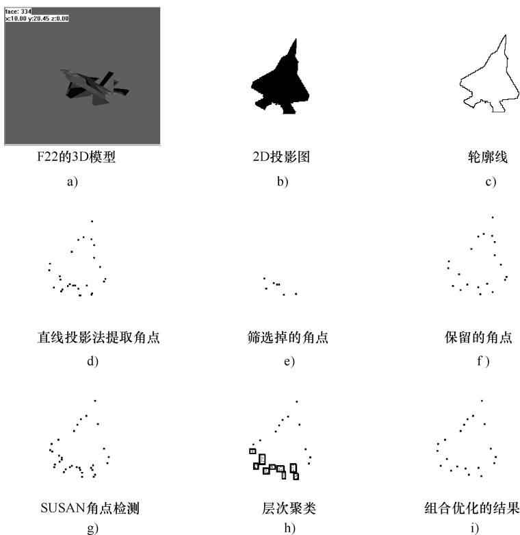
图 7-7 对角点特征空间进行优化设计
