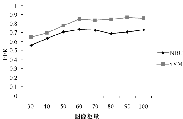
图 6-8 不同样本数量和分类方法的效果
