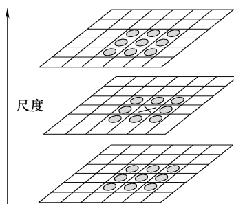
图 4-4 尺度空间的极值检测
