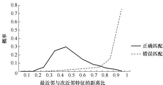
图 5-1 特征点匹配的概率分布
