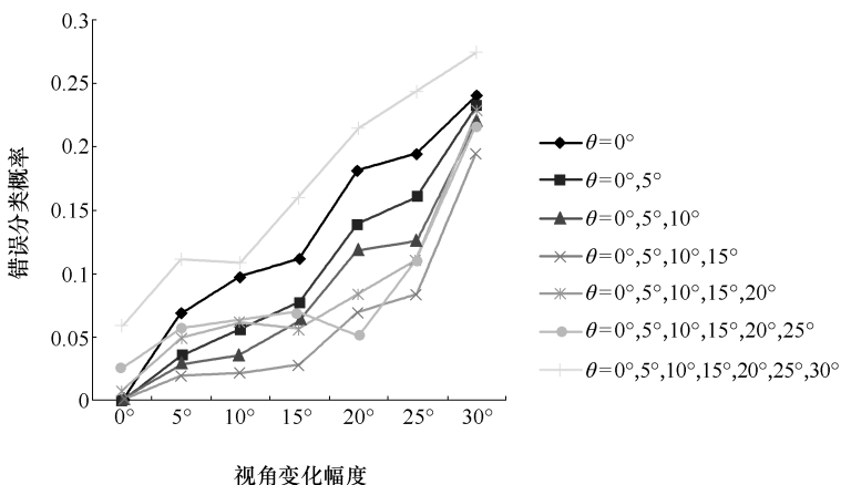
图 7-12 通过增加训练模式改进识别效果
