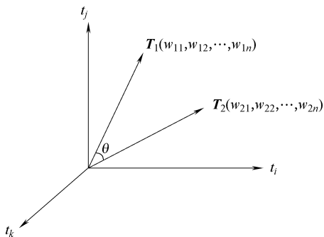
图 6-2 目标的向量空间模型示意图
