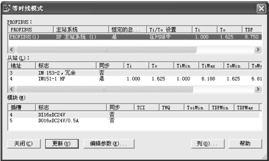
图 5-48 等时线模式对话框
