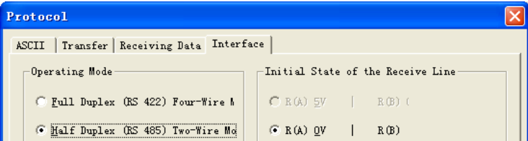
图 15-5 设置 CP 340 的接口参数
