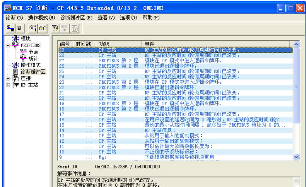
图 6-36 CP 443-5 Ext 的诊断缓冲区
