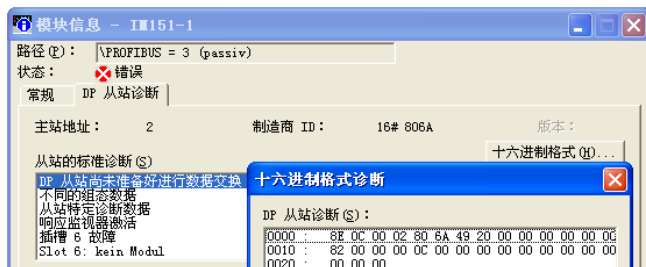
图 6-52 IM 151-1 的模块信息
