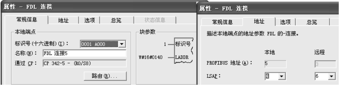
图 4-34 5 号站的 FDL 连接属性对话框
