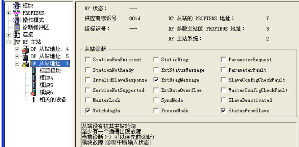
图 6-40 CP 443-5 Ext 诊断视图中 7 号从站的信息
