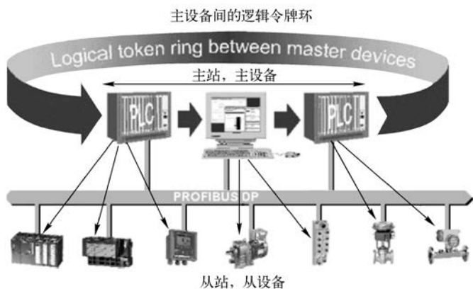
图 2-6 PROFIBUS-DP 的总线访问方式
