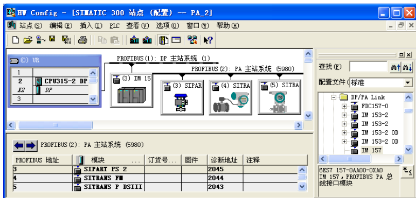
图 9-6 组态 DP、PA 网络
