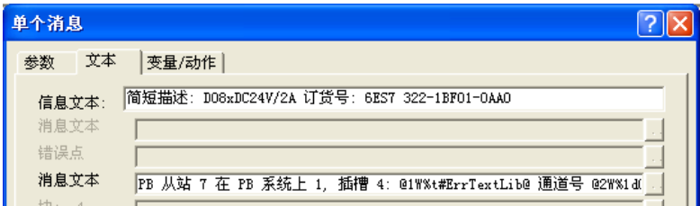
图 8-38 消息属性对话框
