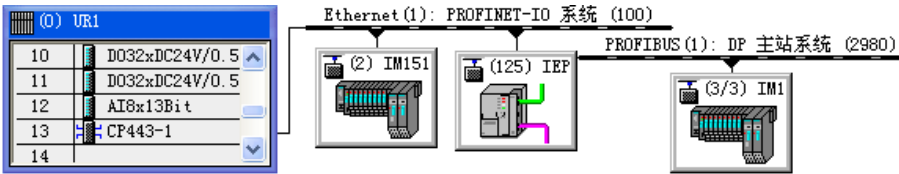
图 11-25 硬件与网络组态
