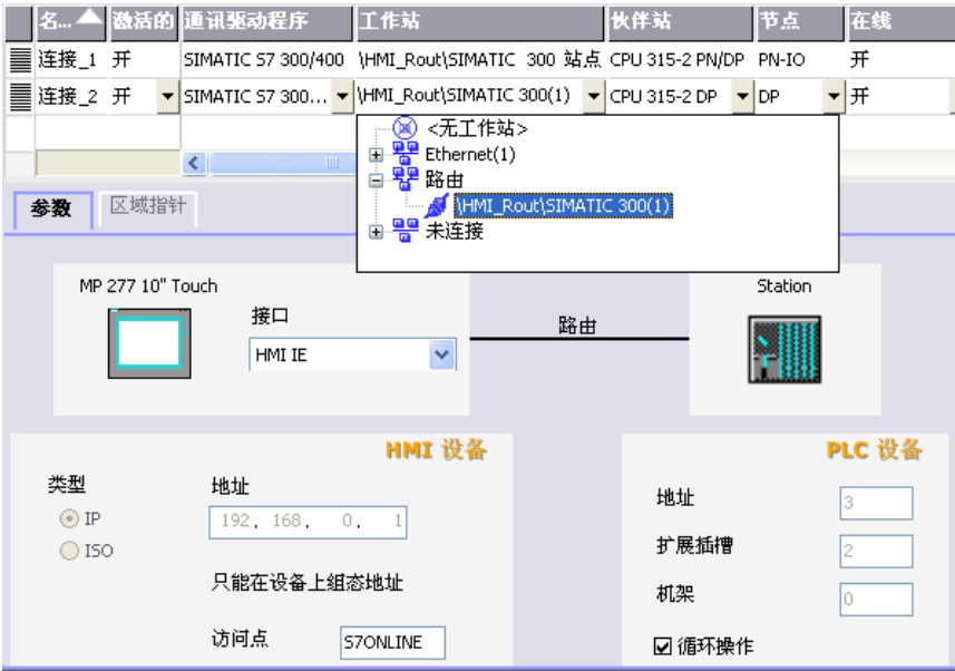
图 15-20 连接属性对话框
