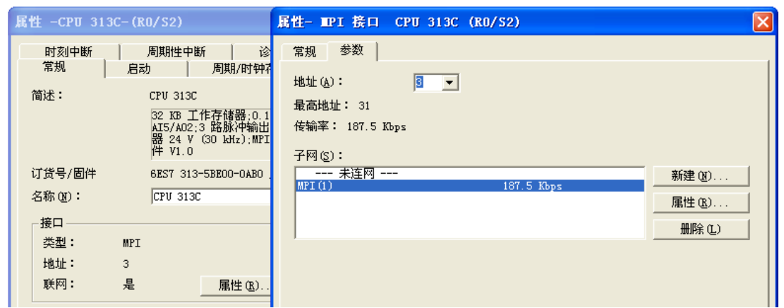
图 14-5 MPI 接口属性对话框
