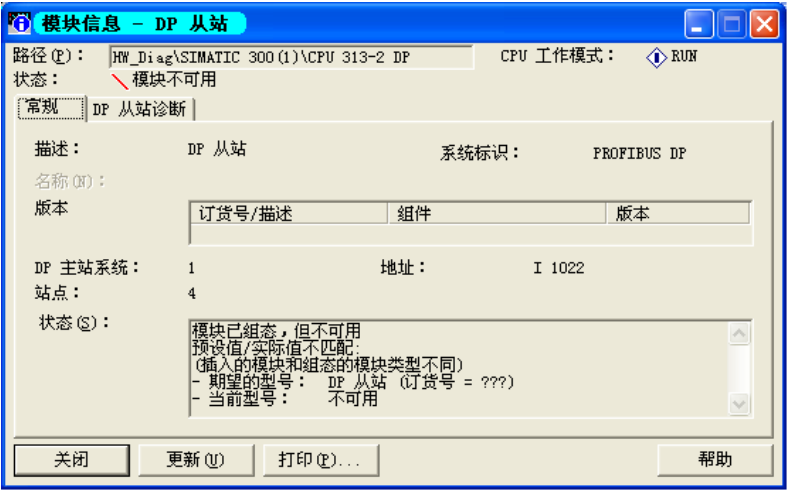
图 6-11 4 号从站的模块信息对话框
