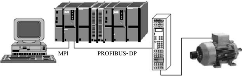
图 3-33 PLC 与变频器通信示意图
