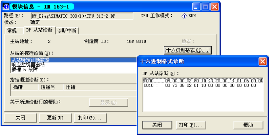
图 6-12 IM 153-1 的模块信息对话框
