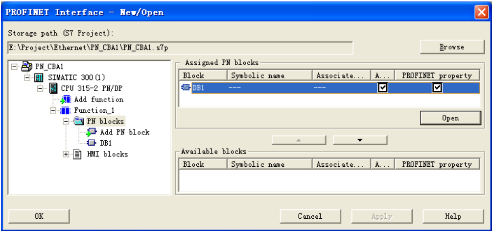
图 11-38 PROFINET 接口属性对话框
