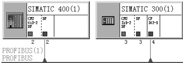
图 3-59 NetPro 中的 DP 网络
