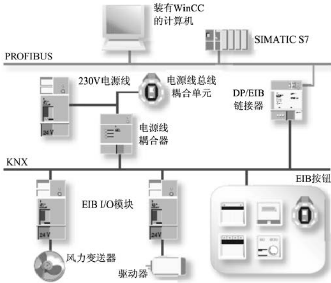
图 15-23 KNX 网络
