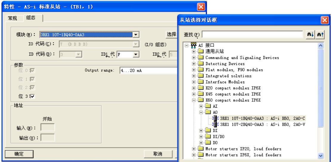
图 12-26 选择 AS-i 从站
