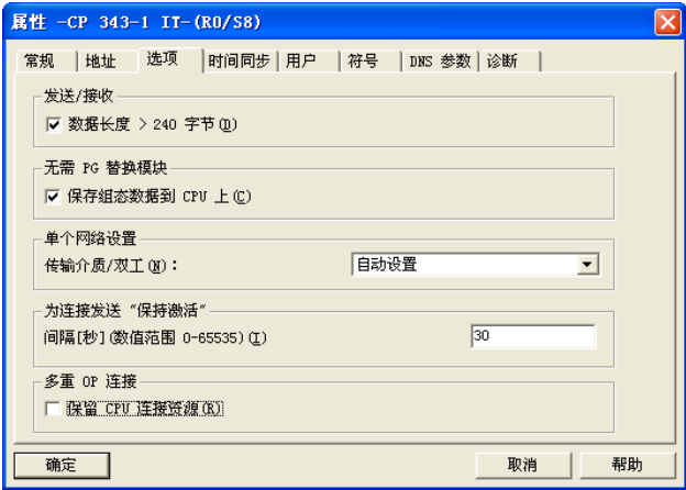
图 10-19 CP 属性对话框
