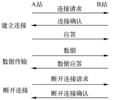
图 10-17 ISO 传输协议的传输过程
