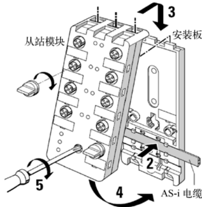
图 12-2 AS-i 从站模块的安装
