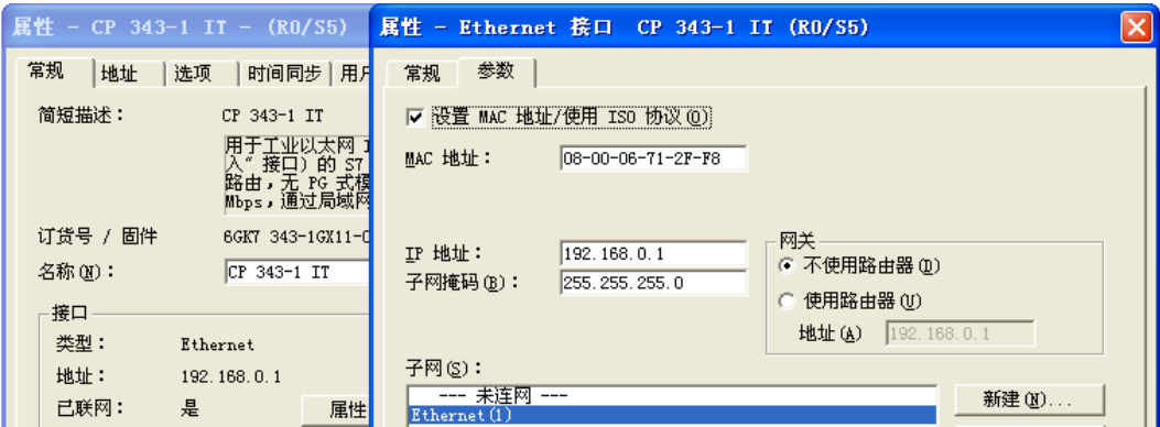
图 13-40 CP 343-1 IT 的以太网接口属性对话框
