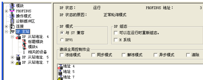
图 6-38 CP 443-5 Ext 诊断视图中 DP 主站的信息
