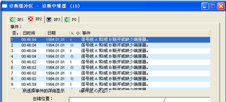
图 6-56 诊断中继器网段 DP2 的诊断缓冲区
