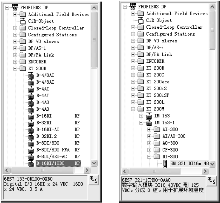
图 3-9 HW Config 右边的硬件目录窗口
