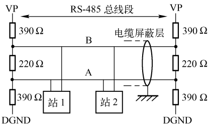
图 2-3 DP/FMS 总线段的结构
