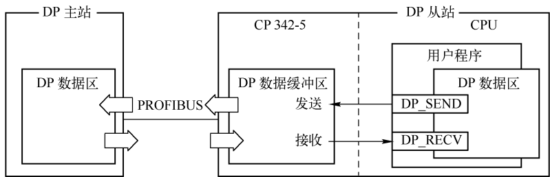
图 3-60 数据交换原理
