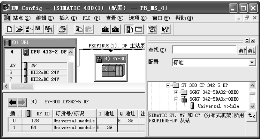
图 3-57 组态 DP 从站
