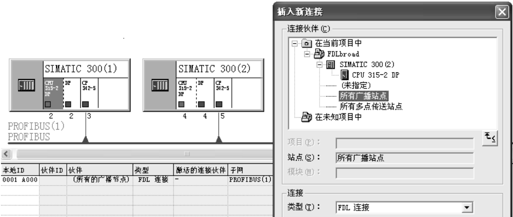
图 4-53 网络与 FDL 连接组态
