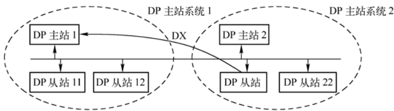
图 5-2 多主站系统中从站发送数据到其他主站
