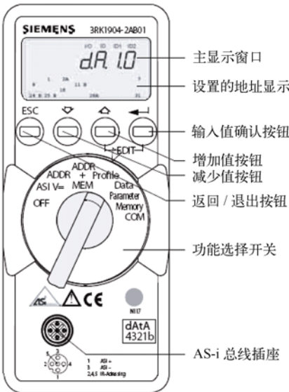
图 12-3 AS-i 编址与诊断单元
