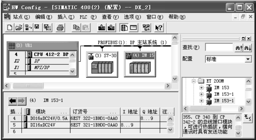
图 5-12 组态 DP 网络
