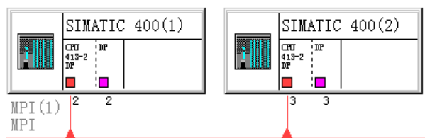
图 14-22 组态好的 MPI 网络
