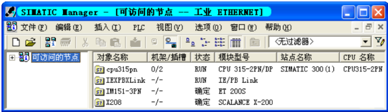
图 6-6 PROFINET 网络上的可访问节点
