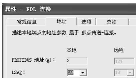
图 4-59 3 号站的 FDL 连接的地址信息
