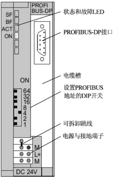
图 3-11 IM 153 的正面视图
