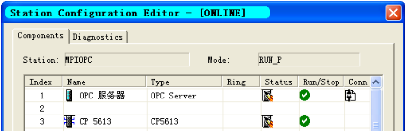
图 13-17 PC 站点的在线状态
