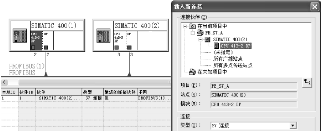
图 4-16 网络与连接的组态
