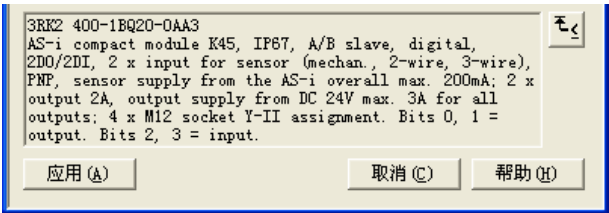
图 12-23 2DI/2DO AS-i 从站模块的信息
