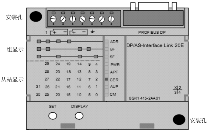
图 12-24 DP/AS-i Link 20E
