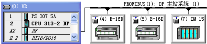
图 6-8 HW Config 中的 DP 网络
