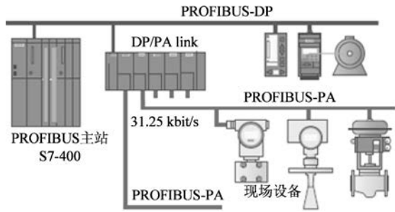
图 2-2 PROFIBUS-PA
