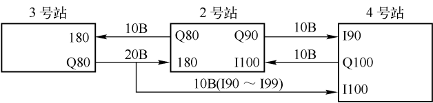
图 5-3 直接数据交换通信示意图
