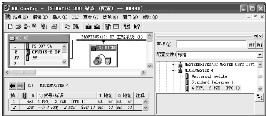
图 3-46 组态 DP 网络中的变频器
