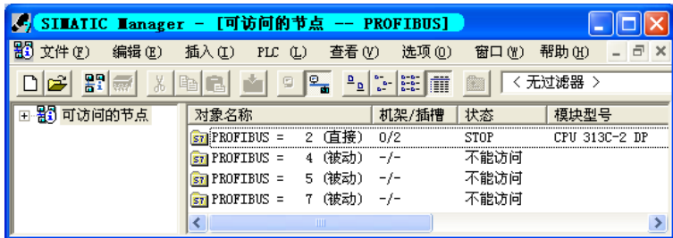
图 6-4 PROFIBUS 网络上的可访问节点
