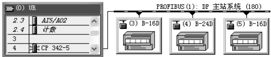
图 5-32 组态 DP 从站
