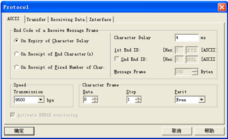
图 15-4 设置 CP 340 的协议参数
