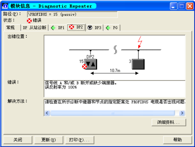
图 6-54 诊断中继器的模块信息
