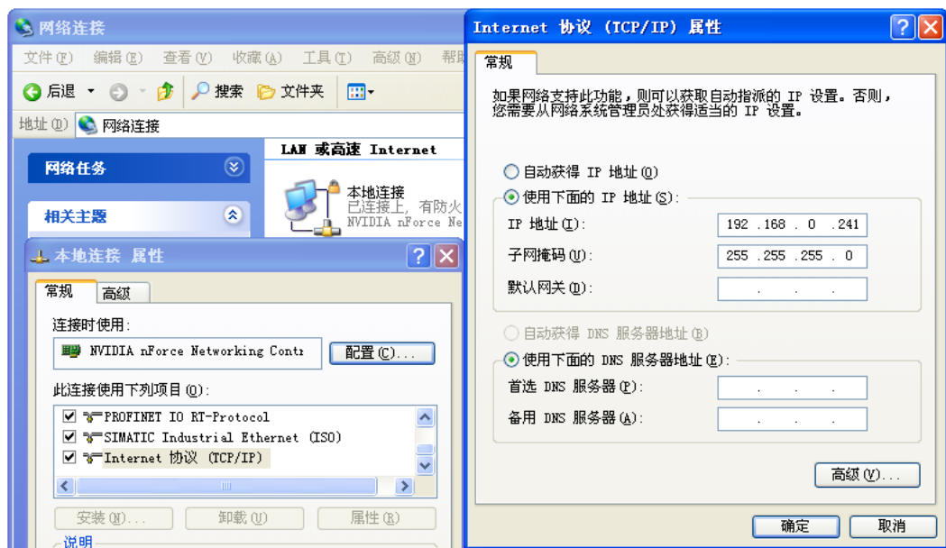
图 10-13 设置计算机网卡的 IP 地址
