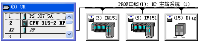
图 6-47 HW Config 中的 DP 网络
