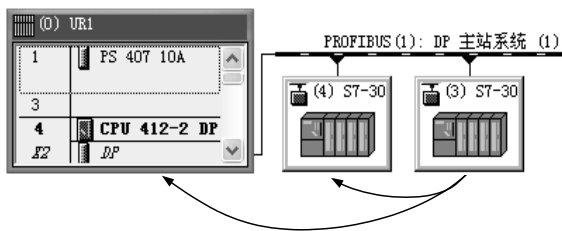
图 5-4 HW Config 中的 DP 网络
