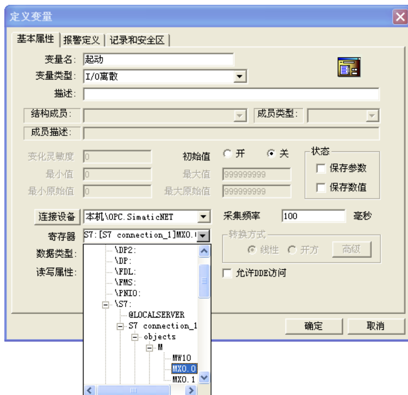
图 13-29 定义变量 M0.0
