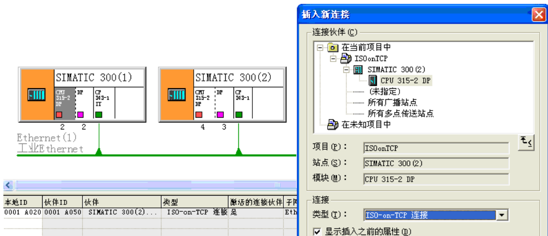
图 10-29 组态 ISO-on-TCP 连接
