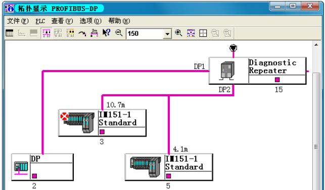
图 6-49 网络拓扑与电缆长度显示
