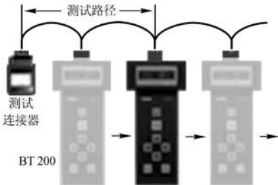
图 6-59 用 BT 200 测试线路
