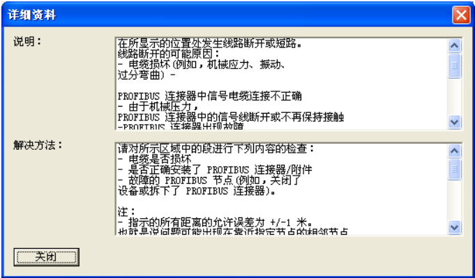
图 6-55 DP2 网段的详细信息
