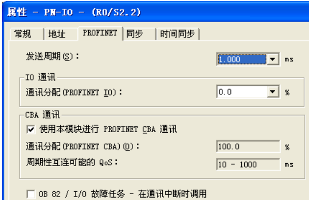
图 11-37 PN IO 属性对话框
