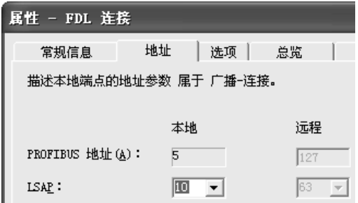
图 4-55 5 号站的 FDL 连接的地址信息
