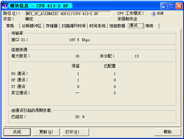
图 14-28 模块信息中的“通讯”选项卡
