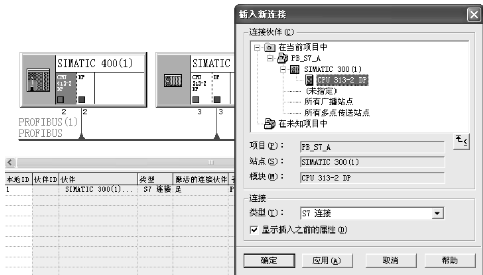
图 4-3 网络与连接的组态
