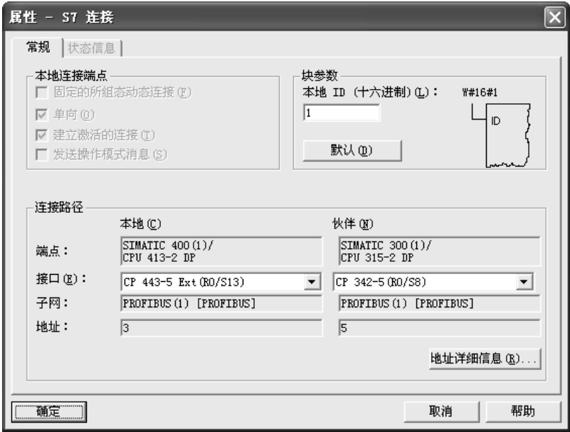
图 4-12 S7 连接属性对话框
