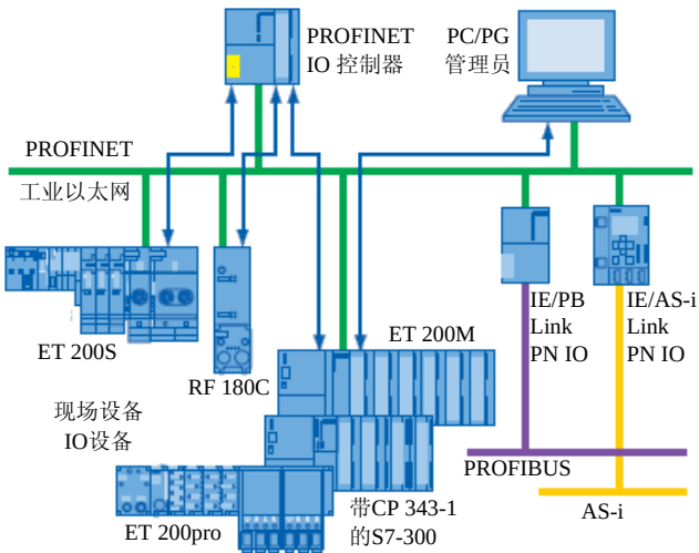
图 11-2 PROFINET
