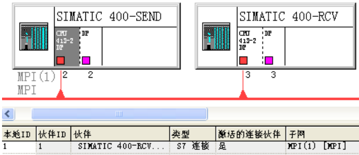
图 14-56 S7 连接组态
