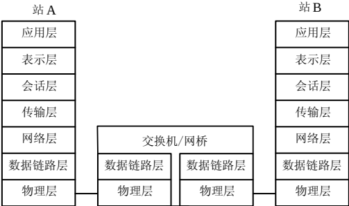
图 10-5 交换机
