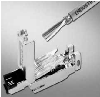
图 10-3 快速连接电缆与 TP RJ45 接头
