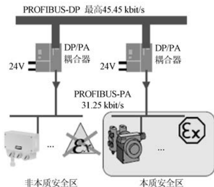
图 9-2 DP/PA 耦合器
