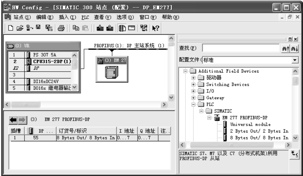
图 3-13 组态 PROFIBUS 从站
