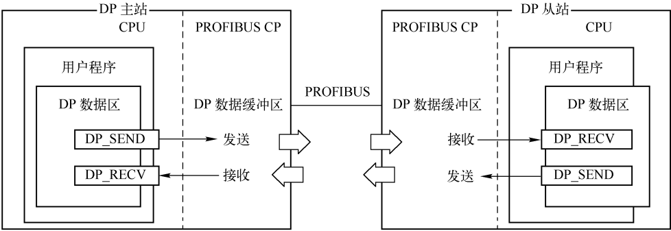
图 3-71 数据交换原理
