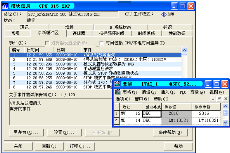
图 8-14 CPU 模块信息的诊断缓冲区
