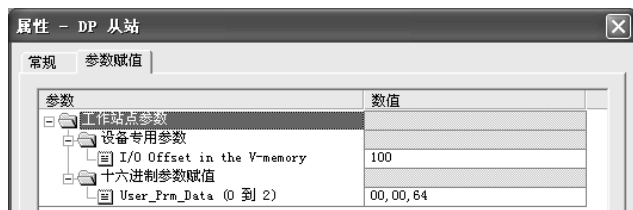
图 3-14 DP 从站属性对话框
