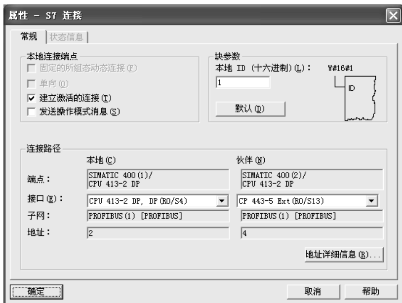
图 4-24 S7 连接属性对话框
