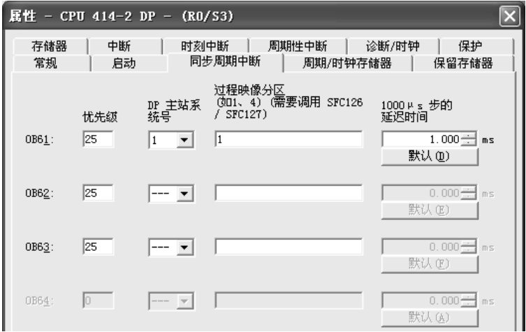
图 5-44 设置同步周期中断
