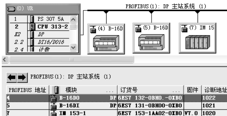
图 5-35 组态 DP 从站
