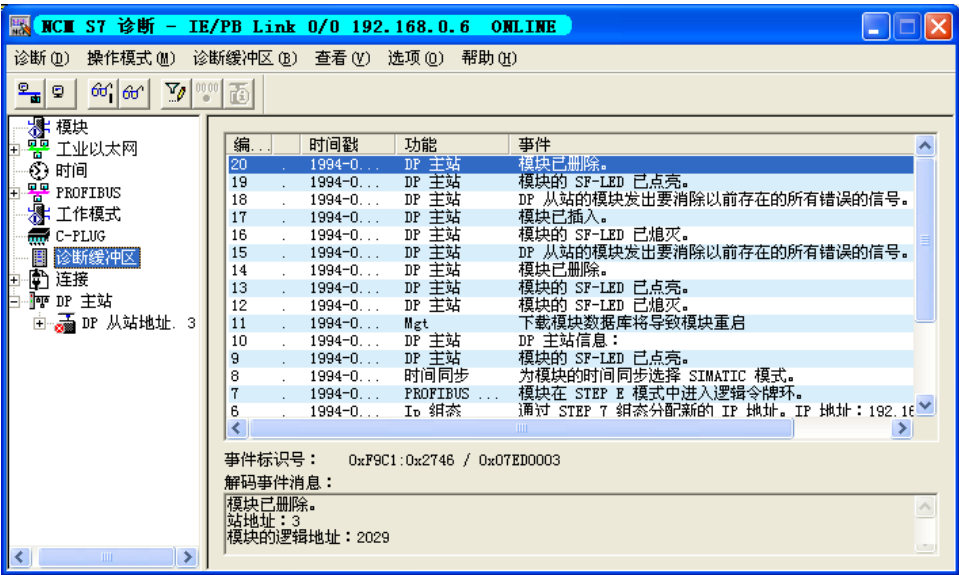
图 11-33 IE/PB Link 的诊断缓冲区
