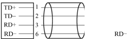
图 10-2 直通连接
