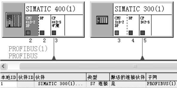
图 4-11 网络与连接的组态
