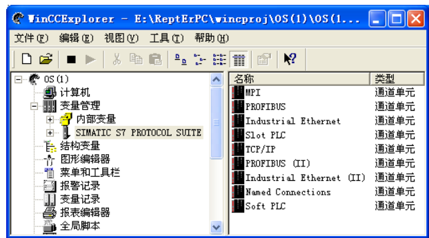
图 8-32 WinCC 管理器
