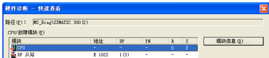
图 7-44 快速视图
