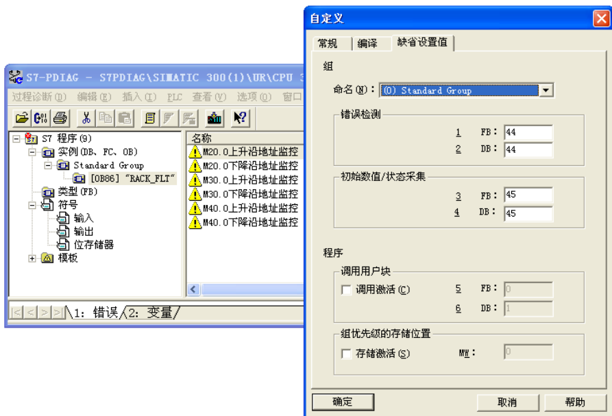
图 8-17 S7-PDIAG
