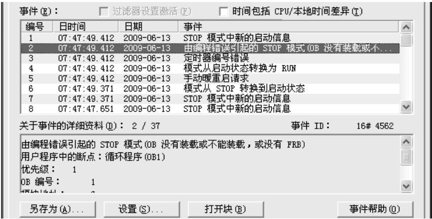
图 6-18 诊断缓冲区
