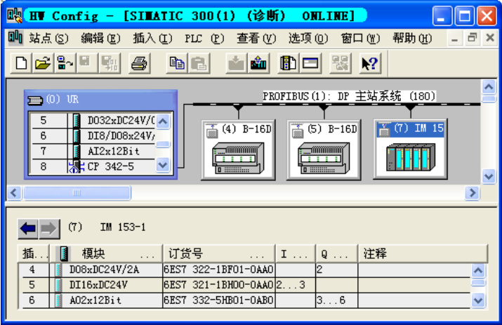
图 7-62 诊断视图
