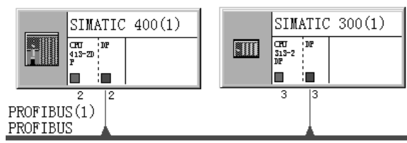
图 3-21 NetPro
