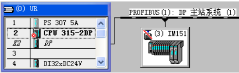
图 7-17 诊断视图
