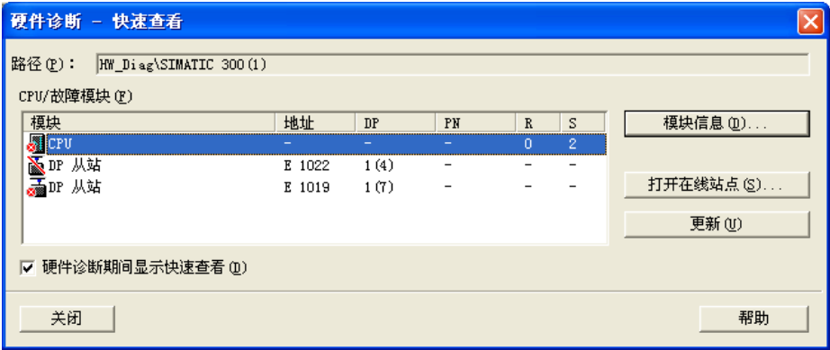
图 6-10 快速视图
