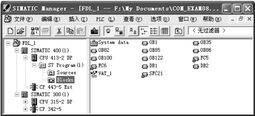
图 4-30 SIMATIC 管理器
