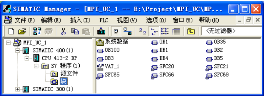
图 14-27 SIMATIC 管理器
