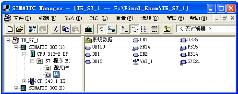
图 10-42 SIMATIC 管理器
