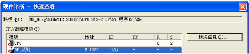
图 7-41 快速视图
