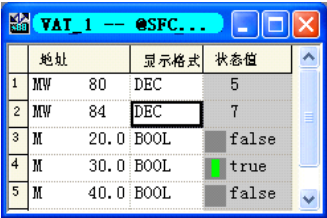
图 7-1 变量表
