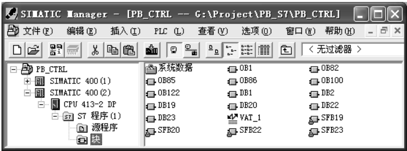
图 4-25 SIMATIC 管理器
