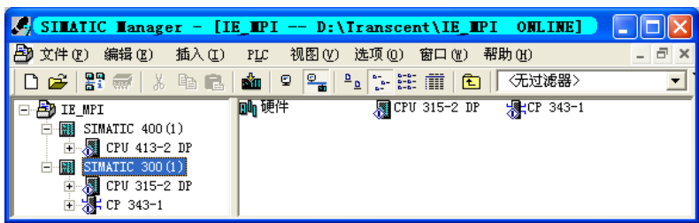
图 15-13 在线视图
