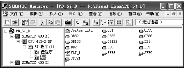
图 4-15 SIMATIC 管理器
