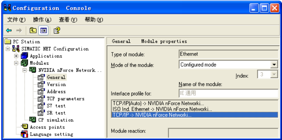
图 13-37 组态控制台
