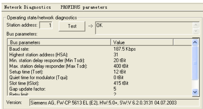
图 13-9 网络诊断
