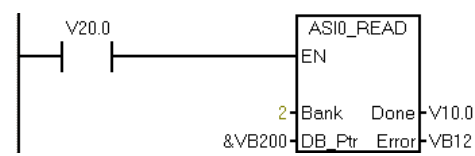
图 12-16 调用 ASI0_READ
