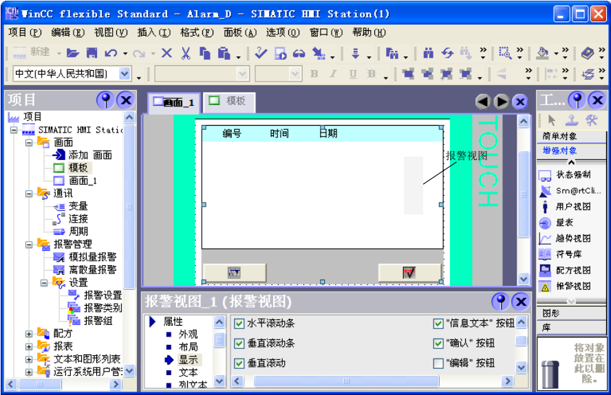
图 8-5 WinCC flexible
