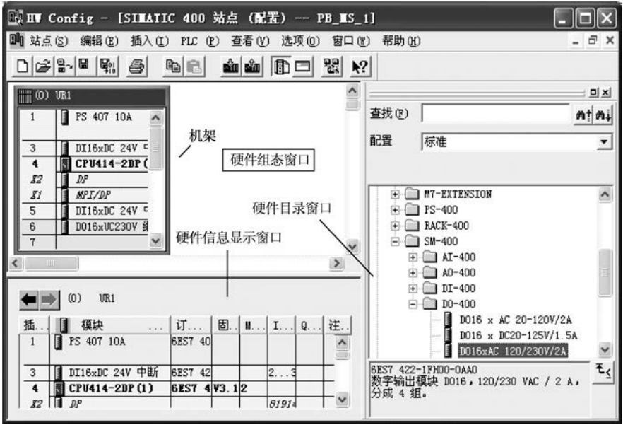
图 3-3 HW Config
