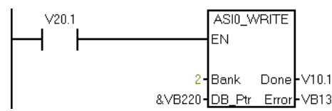
图 12-17 调用 ASI0_WRITE
