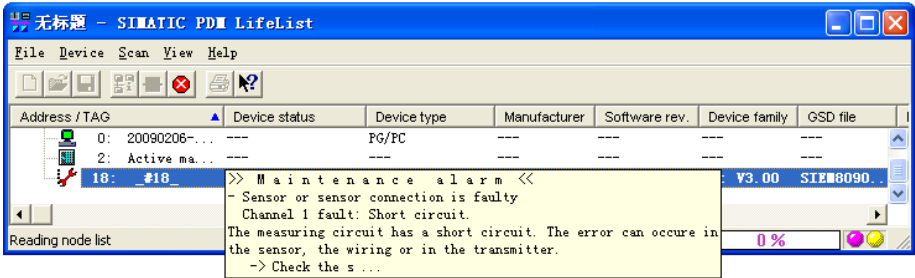
图 9-17 短路故障时的 PDM Lifelist
