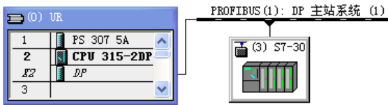
图 7-28 HW Config 中的 DP 主站和智能从站
