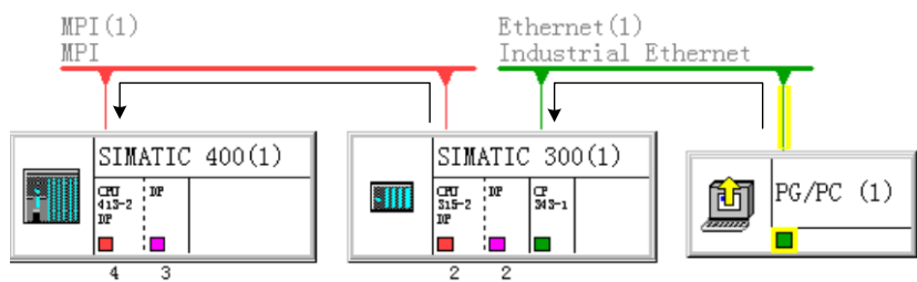
图 15-7 PG/PC 的 S7 路由功能
