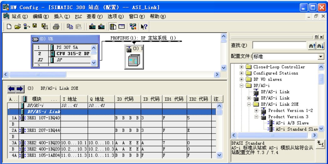
图 12-25 组态 DP/AS-i Link
