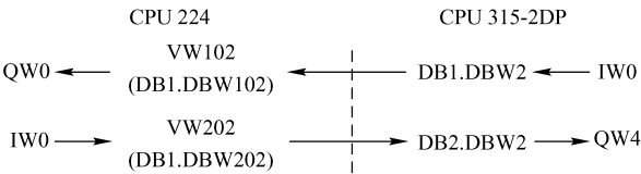
图 14-41 数据传送关系
