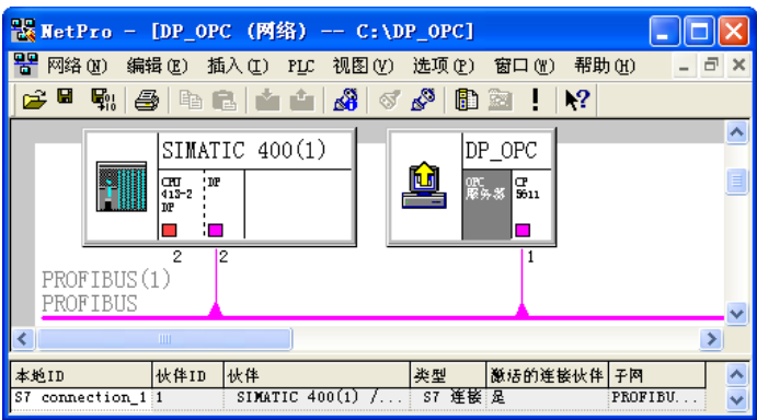
图 13-25 组态 S7 连接
