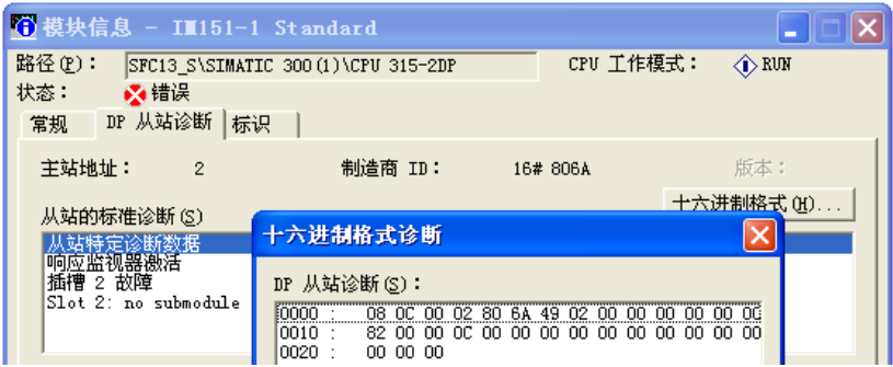
图 7-24 IM 151-1 模块信息中的诊断信息
