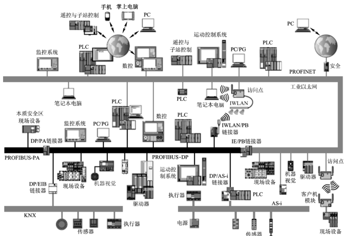
图 1-4 西门子的工业自动化通信网络
