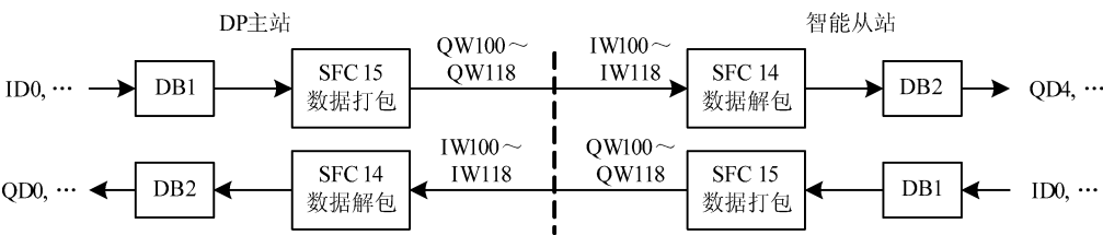
图 3-28 DP 主站与智能从站的数据传输
