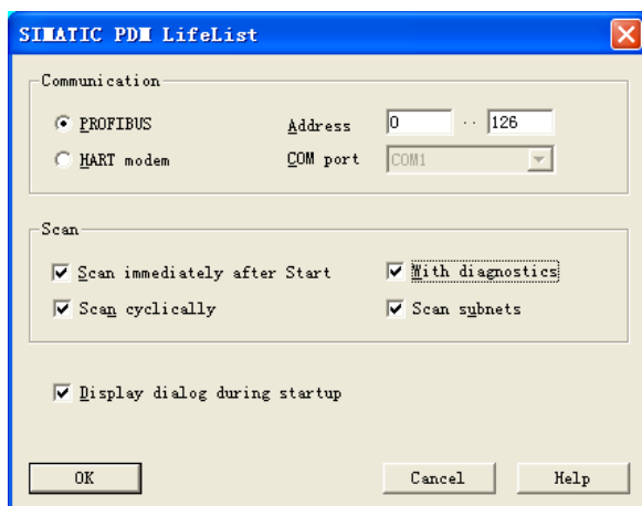
图 9-13 设置 PDM 的参数
