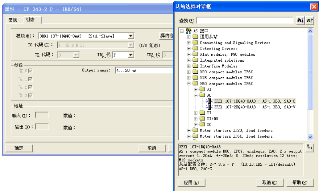
图 12-22 选择 AS-i 从站
