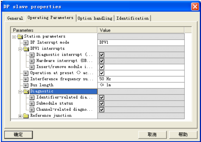
图 11-10 IM 151-1 属性对话框
