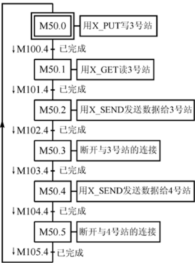
图 14-33 2 号站的顺序功能图
