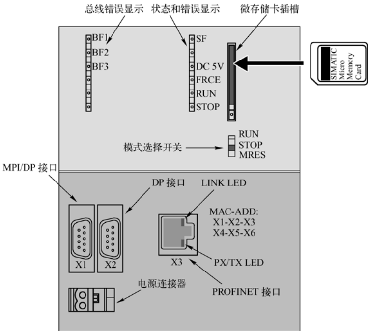
图 6-1 CPU 319-3PN/DP 的面板图
