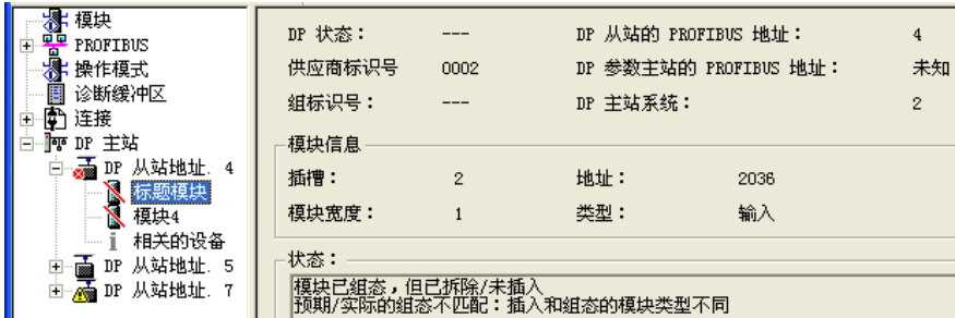
图 6-39 CP 443-5 Ext 诊断视图中 DP 从站的标题模块信息
