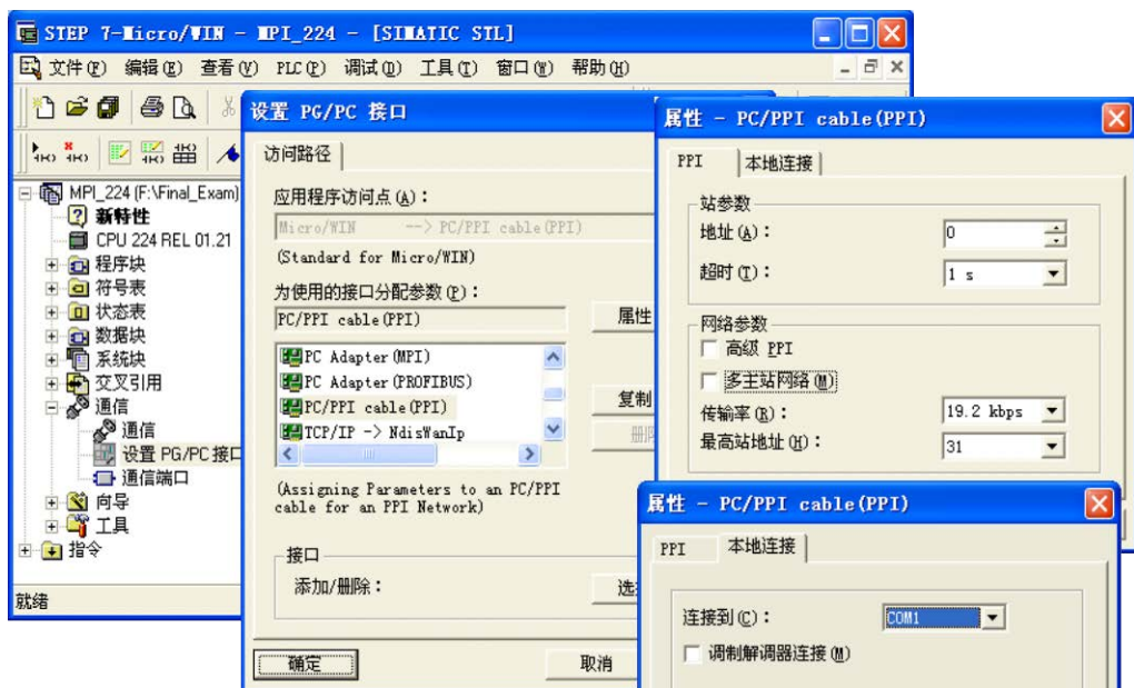
图 14-39 设置 PG/PC 接口
