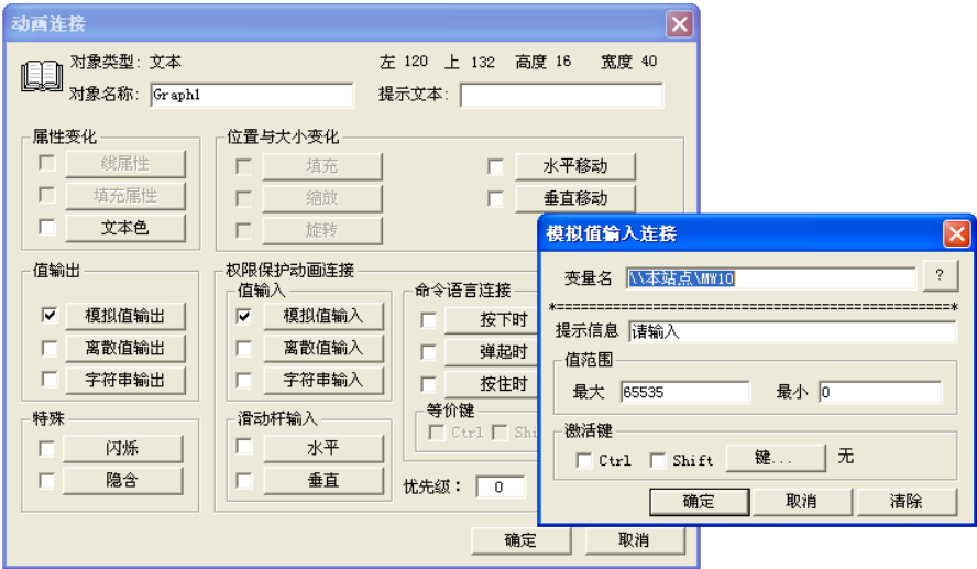
图 13-32 组态显示和修改 MW10 的动画连接
