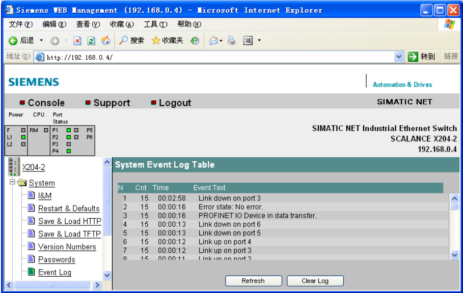
图 11-19 X204-2 的事件记录表
