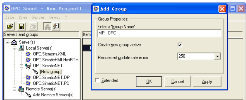
图 13-18 在 OPC Scout 中添加组
