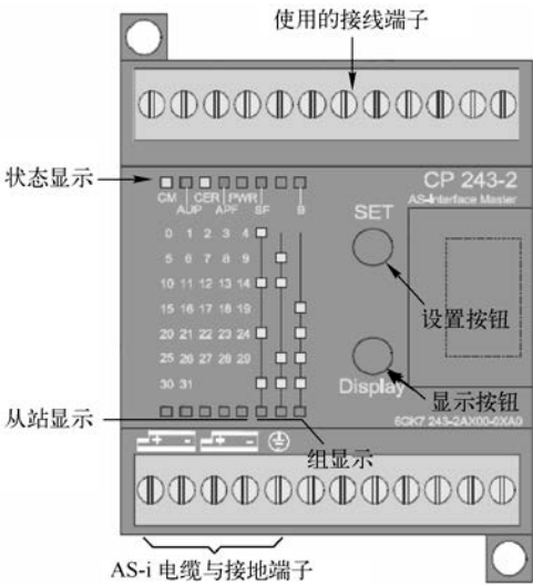
图 12-4 CP243-2
