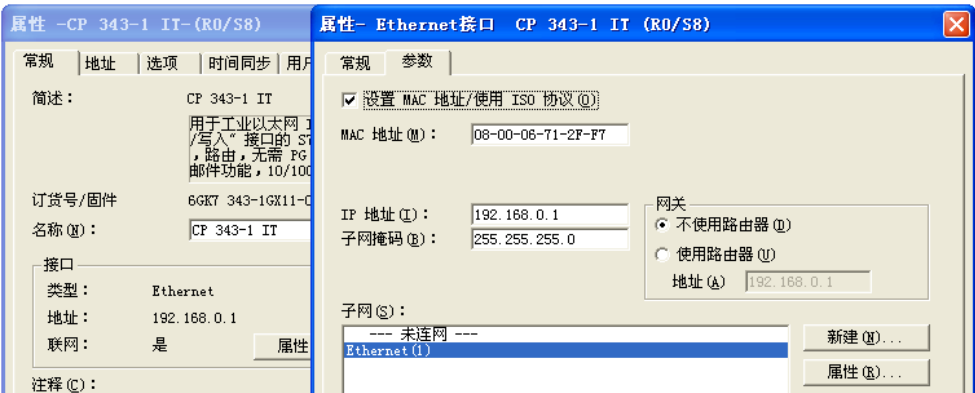
图 10-43 CP 的以太网接口属性对话框
