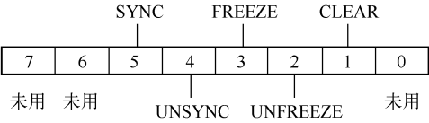
图 3-72 命令模式字节
