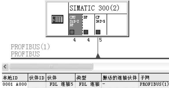
图 4-46 项目 FDL_Pro2 中的网络
