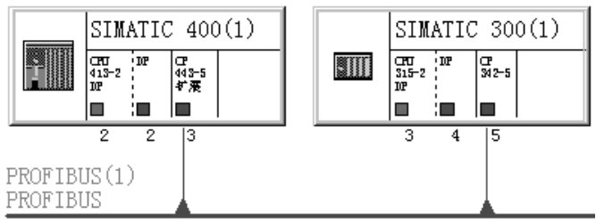
图 3-65 NetPro 中的 DP 网络
