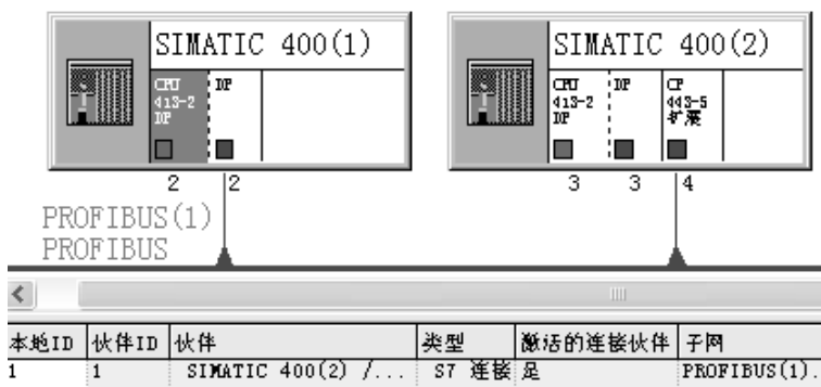
图 4-23 网络与连接组态
