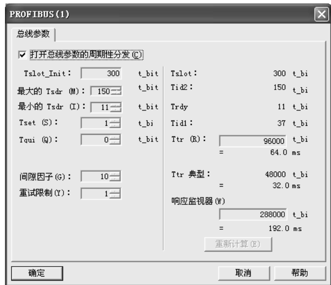
图 3-8 总线参数选项卡
