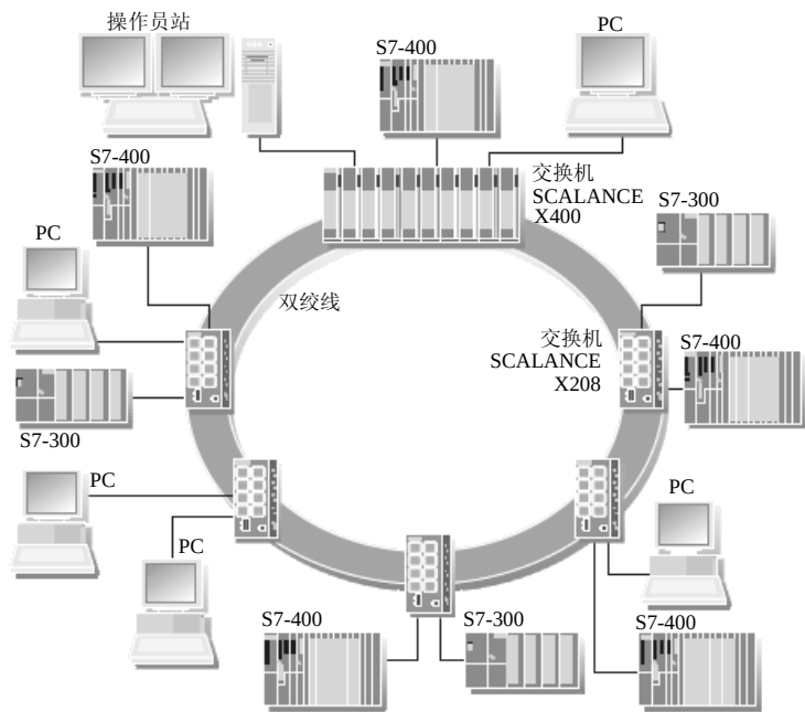
图 10-8 工业以太网中的电气环型冗余
