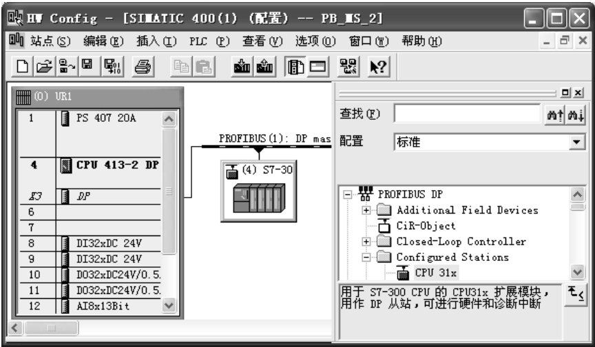
图 3-16 组态 PROFIBUS 智能从站
