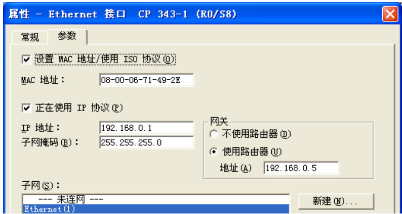
图 15-8 组态 CP 343-1 的以太网接口
