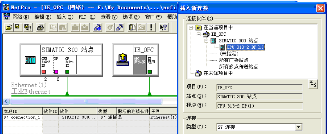
图 13-41 组态 S7 连接
