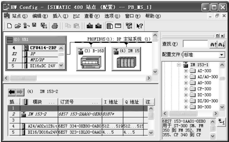
图 3-6 组态好的 PROFIBUS 网络
