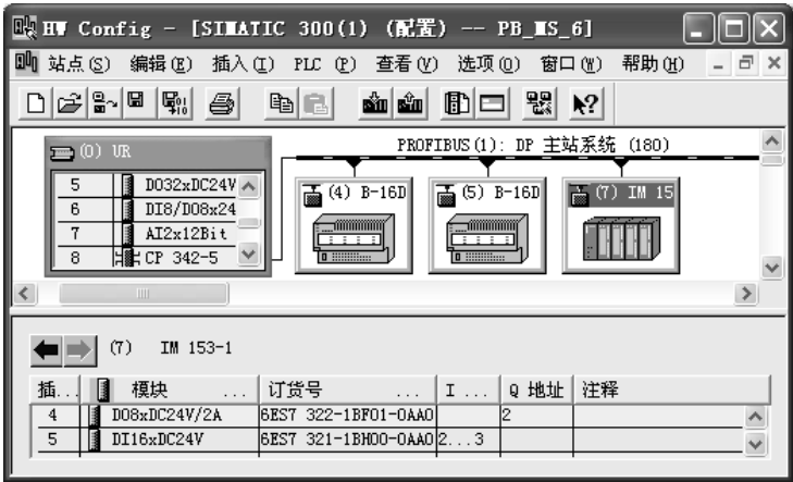
图 3-67 CP 342-5 作主站的 DP 网络
