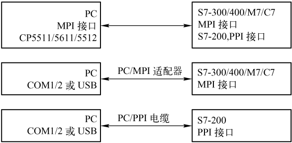
图 14-59 PC 与 PLC 的连接方式
