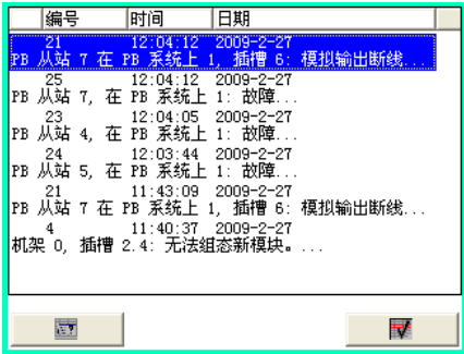
图 8-27 硬件 PLC 的诊断消息
