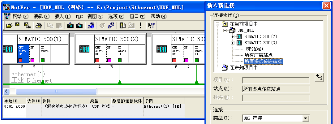
图 10-37 组态 UDP 连接
