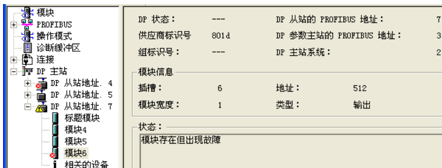
图 6-41 7 号从站的 AO 模块的诊断信息
