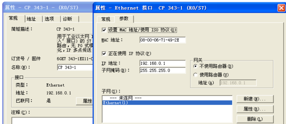
图 10-11 设置 CP 的以太网接口
