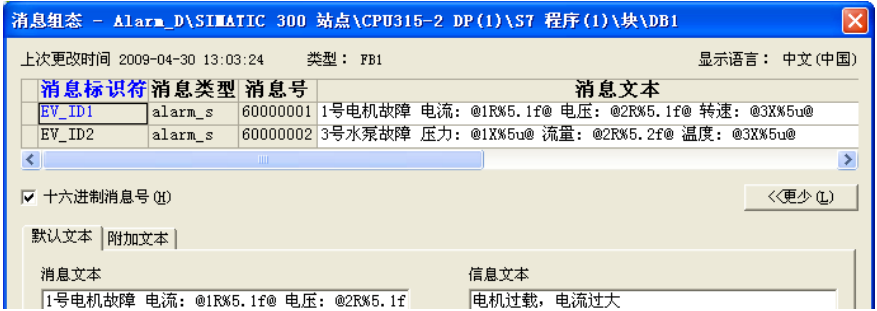
图 8-4 消息组态对话框
