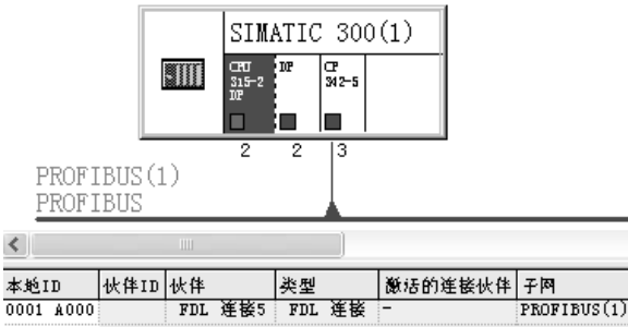
图 4-44 项目 FDL_Pro1 中的网络
