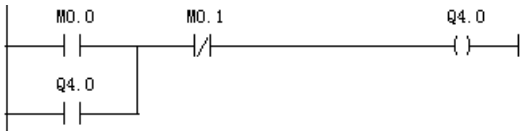
图 13-14 梯形图
