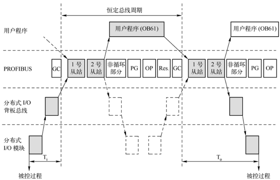
图 5-41 恒定总线周期示意图
