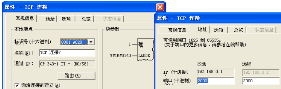
图 10-21 TCP 连接属性对话框
