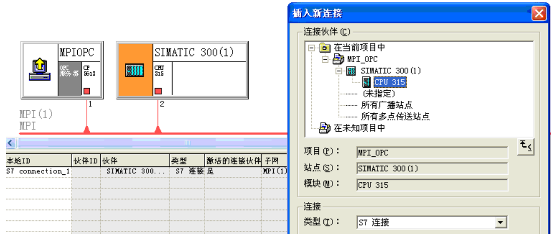
图 13-15 组态 S7 连接
