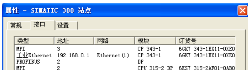
图 10-15 300 站点的通信接口
