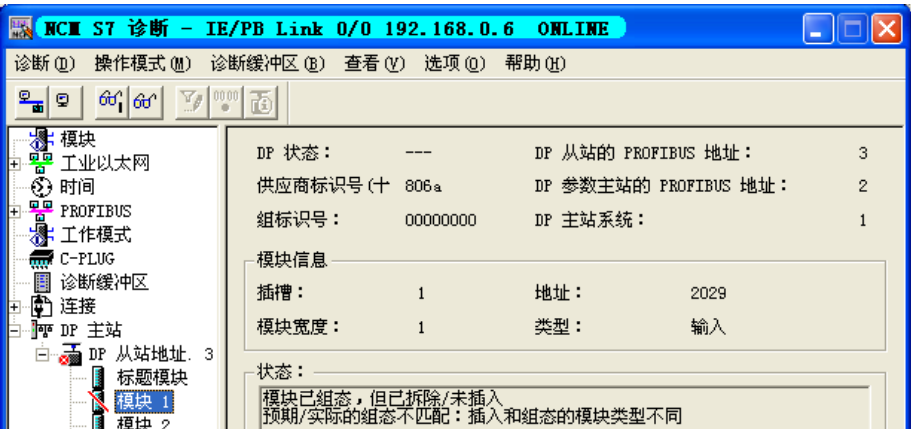
图 11-34 IE/PB Link 的 DP 从站信息
