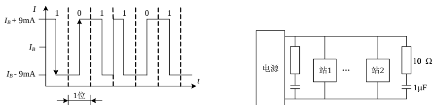
图 9-1 PROFIBUS-PA 的数据传输
