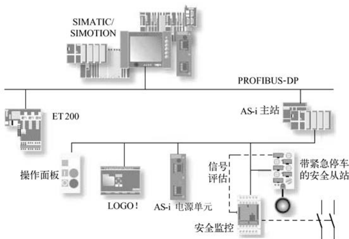
图 12-1 AS-i 网络
