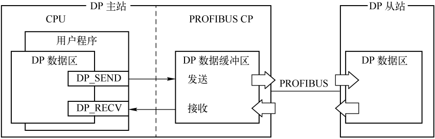
图 3-68 数据交换原理
