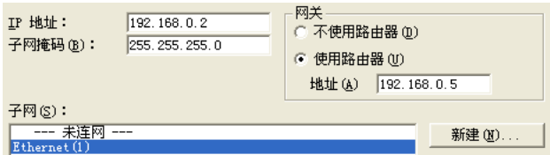
图 15-18 CPU 315-2PN/DP 的以太网接口属性对话框
