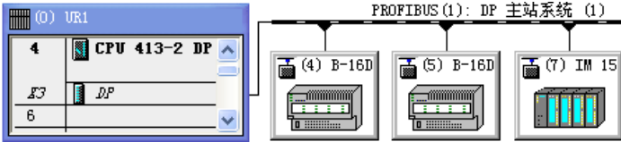
图 6-26 HW Config 中的 DP 网络
