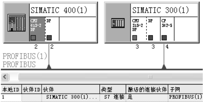
图 4-9 网络与连接的组态
