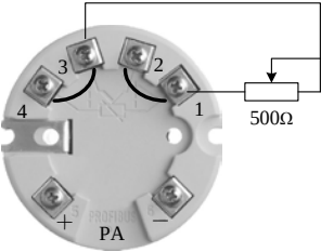
图 9-12 T3K 的接线
