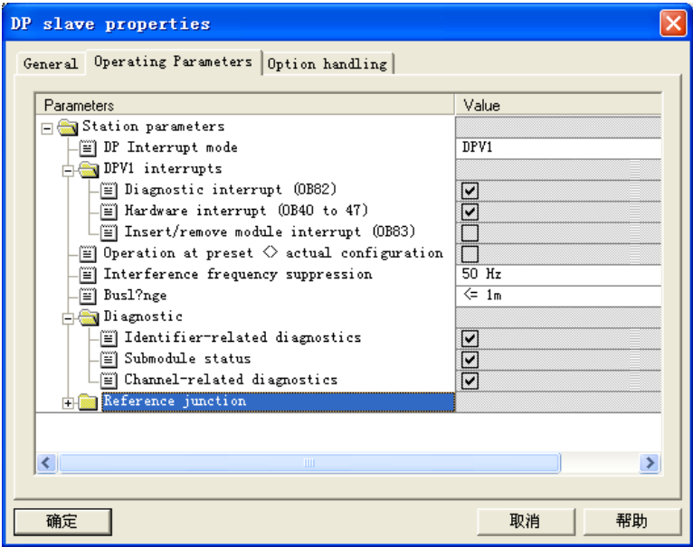
图 7-13 ET 200S 从站属性对话框
