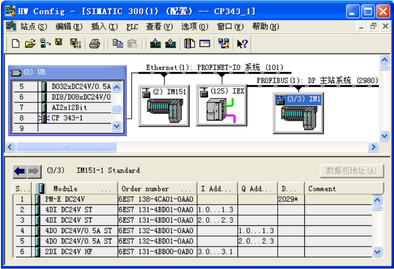
图 11-21 硬件与网络组态
