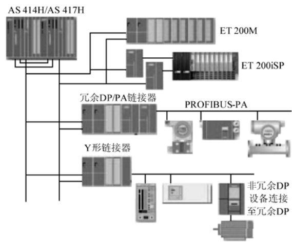
图 2-8 PROFIBUS 在冗余系统中的应用
