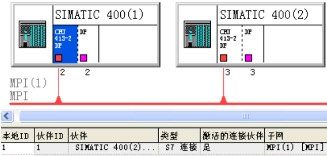
图 14-48 网络与 S7 连接组态
