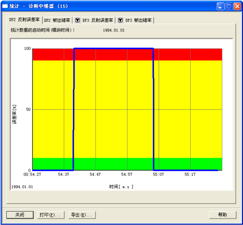
图 6-57 诊断中继器网段 DP2 反射误差率的统计图
