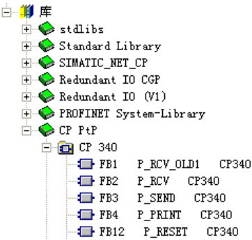
图 15-2 PtP 通信的 FB
