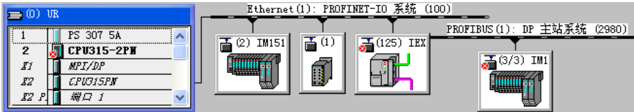
图 11-31 诊断视图
