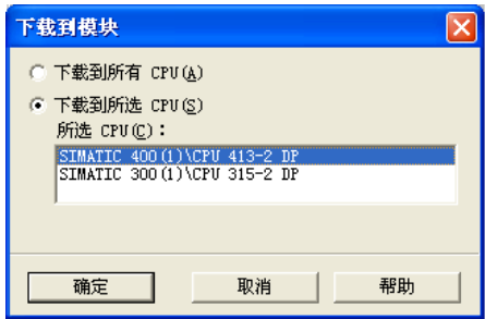
图 14-9 下载对话框
