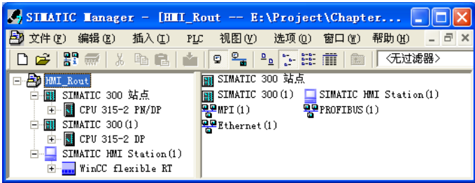
图 15-16 SIMATIC 管理器
