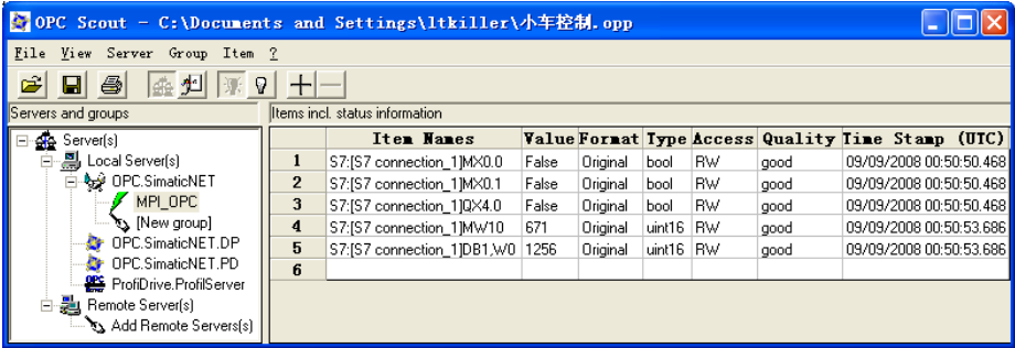
图 13-22 OPC Scout
