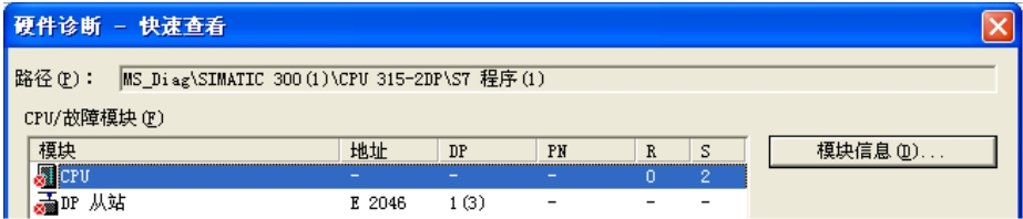
图 7-33 快速视图
