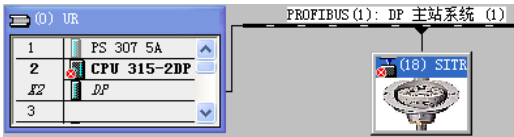
图 9-24 诊断视图
