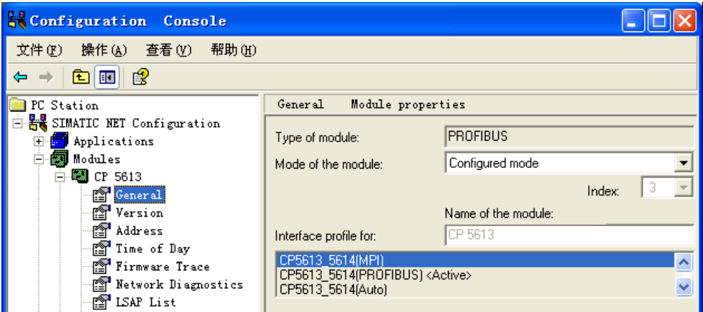
图 13-7 组态控制台
