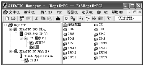
图 8-30 SIMATIC 管理器
