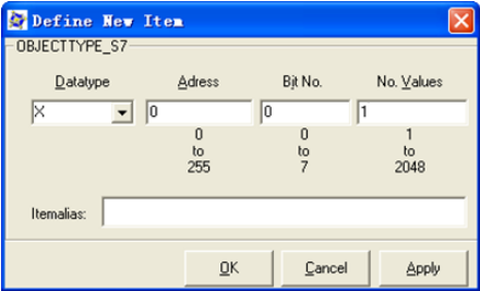
图 13-20 定义新条目
