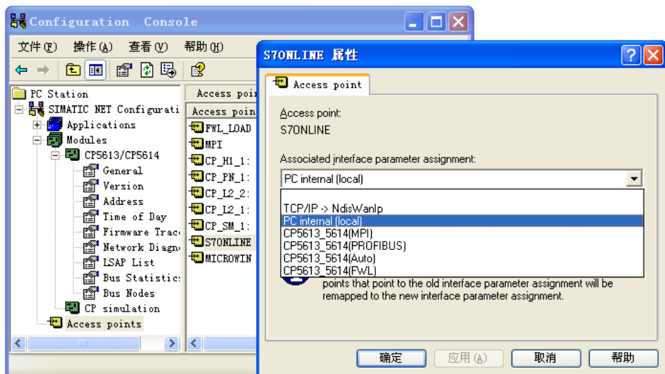
图 13-8 组态访问点
