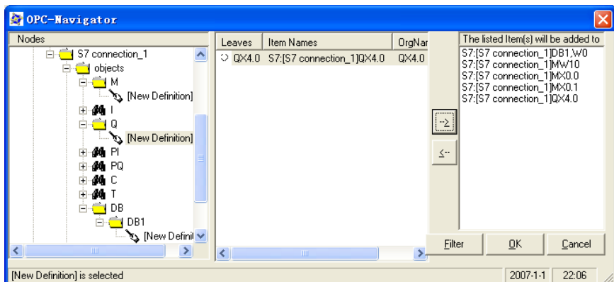
图 13-19 OPC 浏览器
