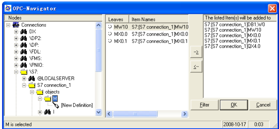
图 13-42 OPC 浏览器
