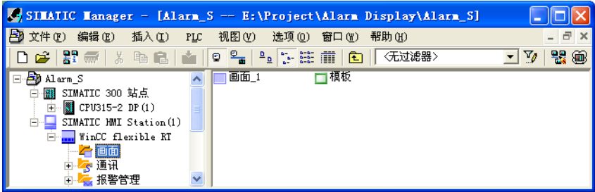
图 8-1 SIMATIC 管理器
