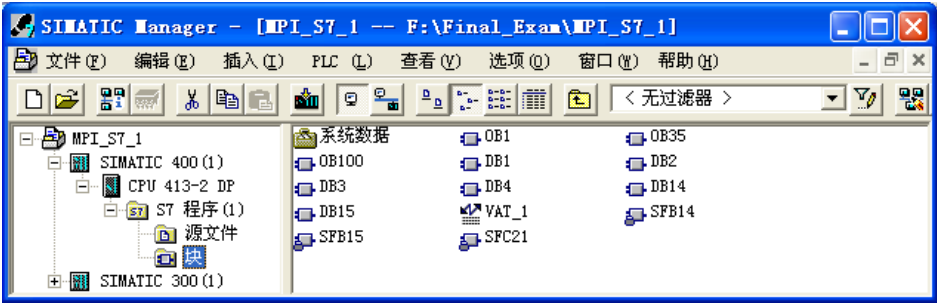
图 14-43 SIMATIC 管理器
