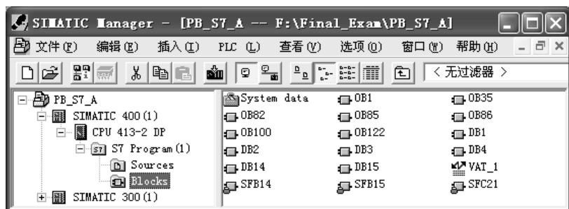
图 4-2 SIMATIC 管理器
