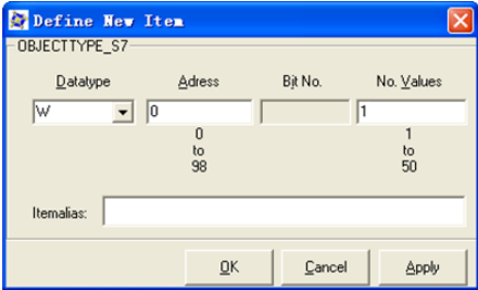
图 13-21 定义新条目
