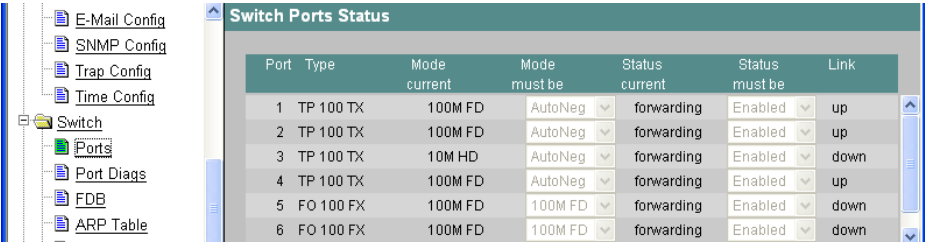
图 11-20 204-2 的接口状态
