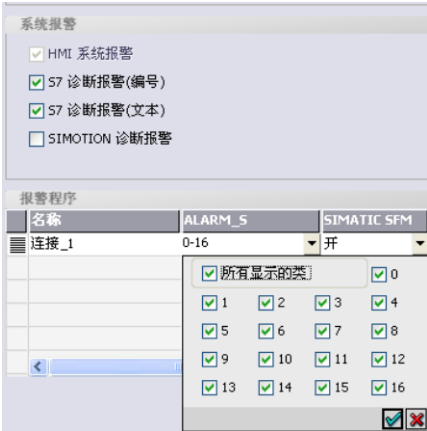
图 8-7 设置报警
