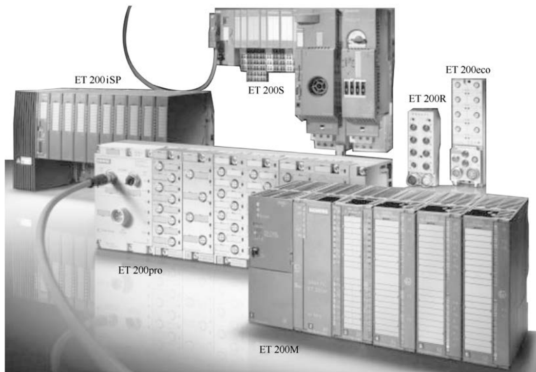
图 2-4 ET 200
