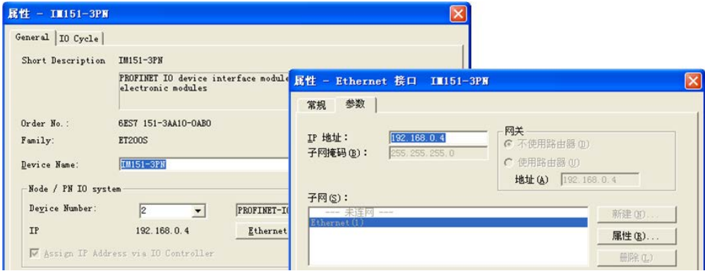
图 11-6 IM151-3PN 属性对话框
