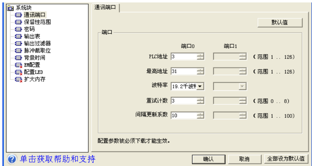
图 14-40 设置 S7-200 的通信接口
