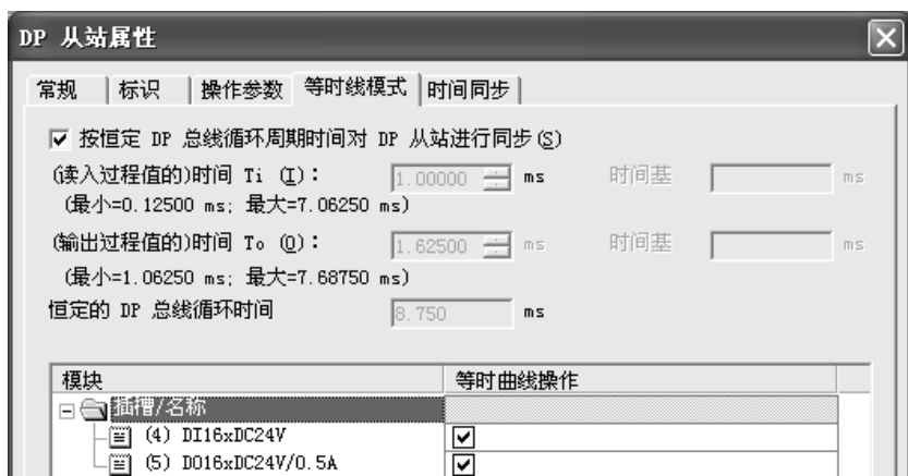
图 5-46 设置从站的等时线模式属性
