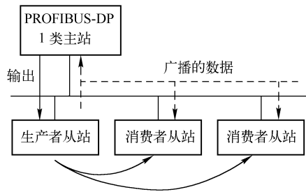
图 5-1 从站与从站的直接数据交换
