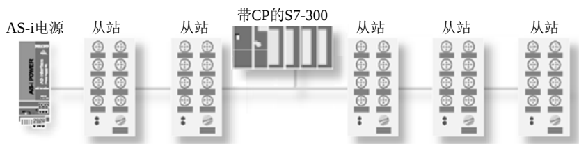
图 12-19 AS-i 网络
