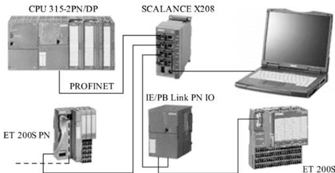
图 11-3 系统硬件与接线
