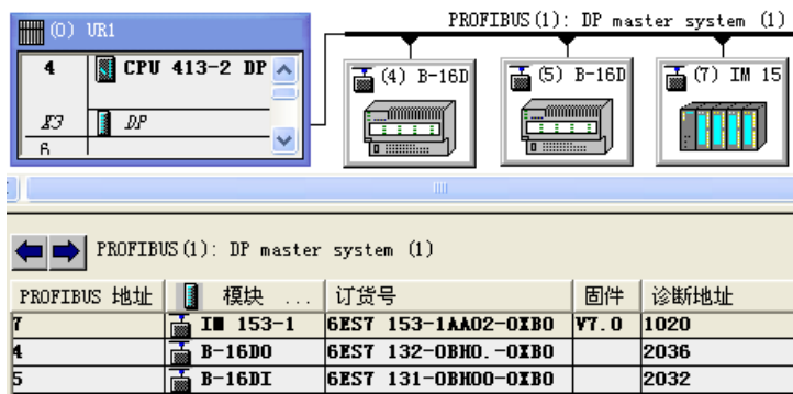
图 6-30 HW Config 中的 DP 网络
