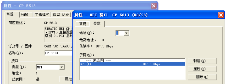
图 13-13 CP 5613 的参数设置
