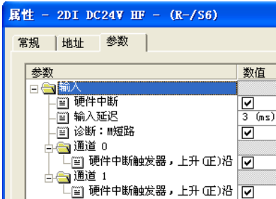
图 7-15 组态 2DI 模块
