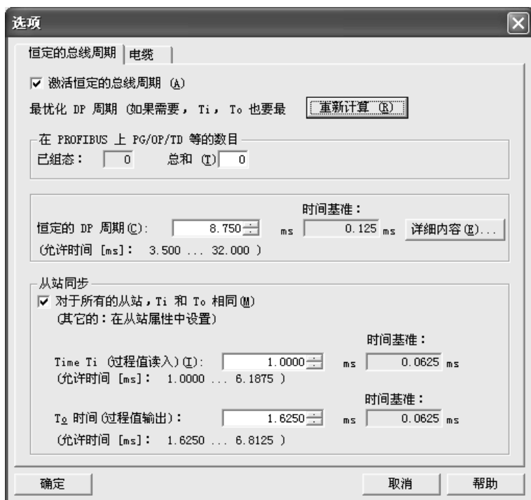
图 5-45 设置恒定的总线周期
