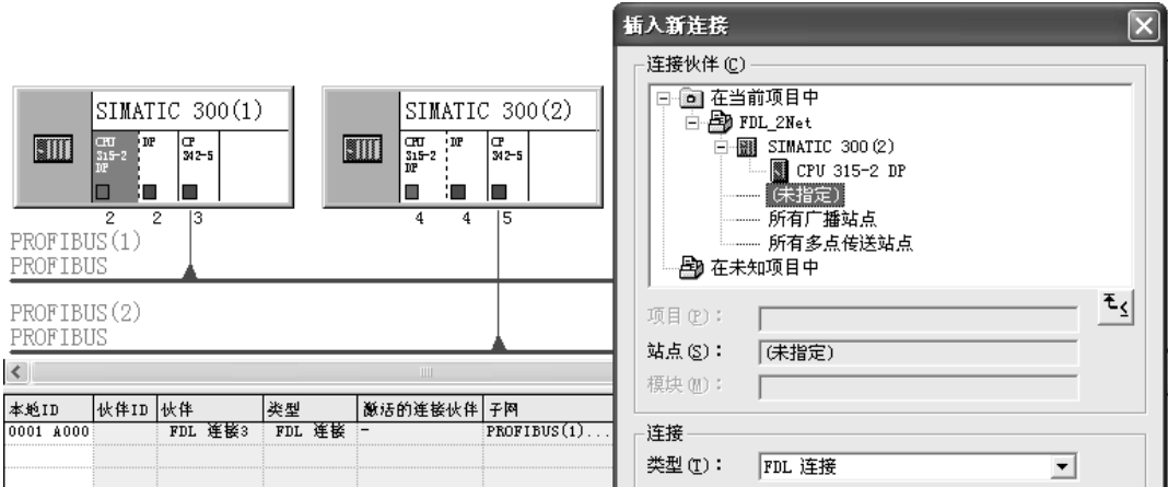
图 4-40 组态 FDL 连接
