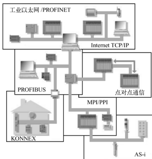
图 1-3 西门子的工业自动化通信网络
