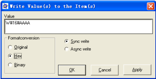
图 13-23 对变量进行写操作
