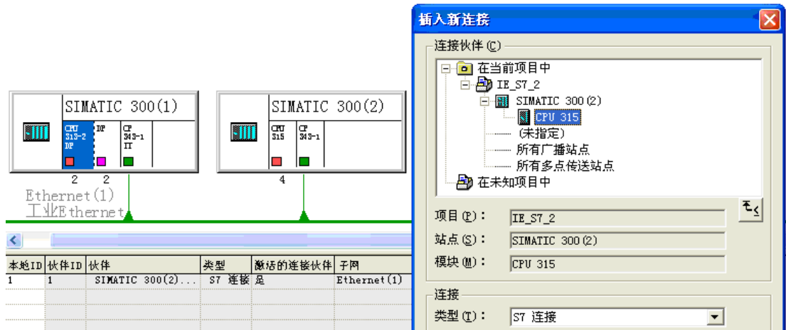
图 10-48 组态 S7 连接
