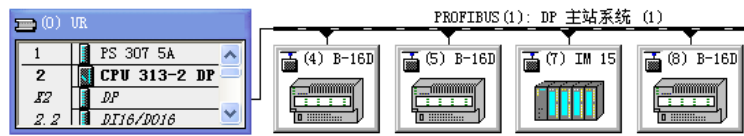
图 7-47 HW Config 中组态的 DP 从站
