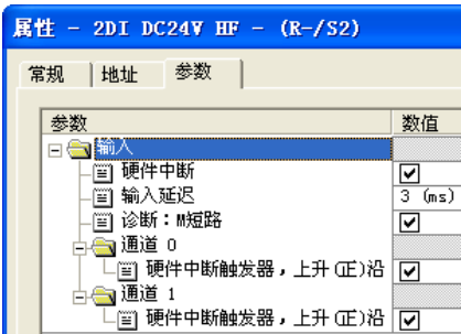
图 11-8 ET 200S DI 模块组态
