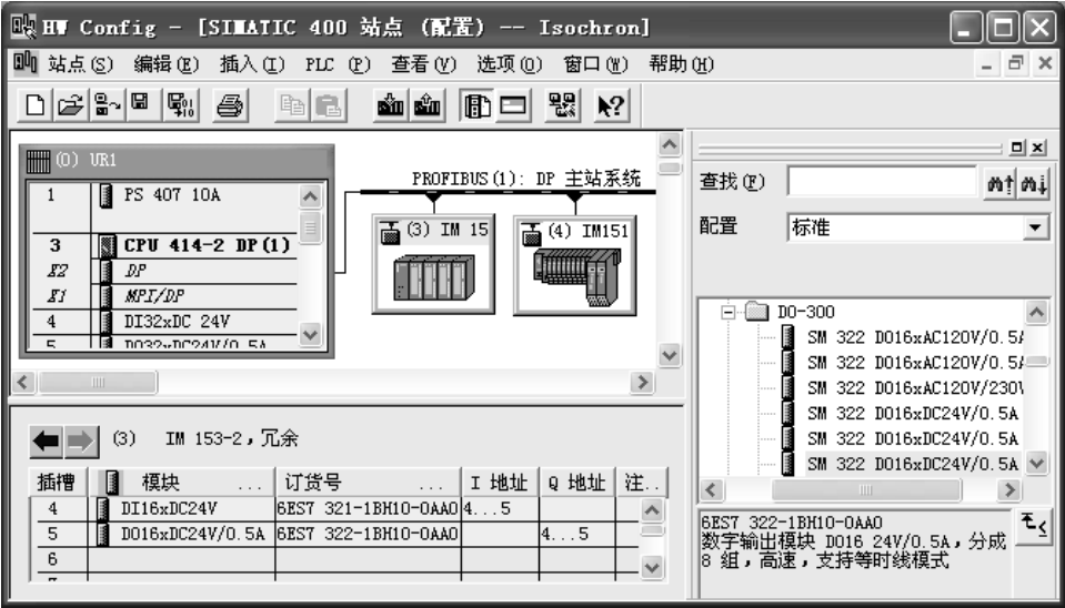
图 5-42 组态 DP 从站
