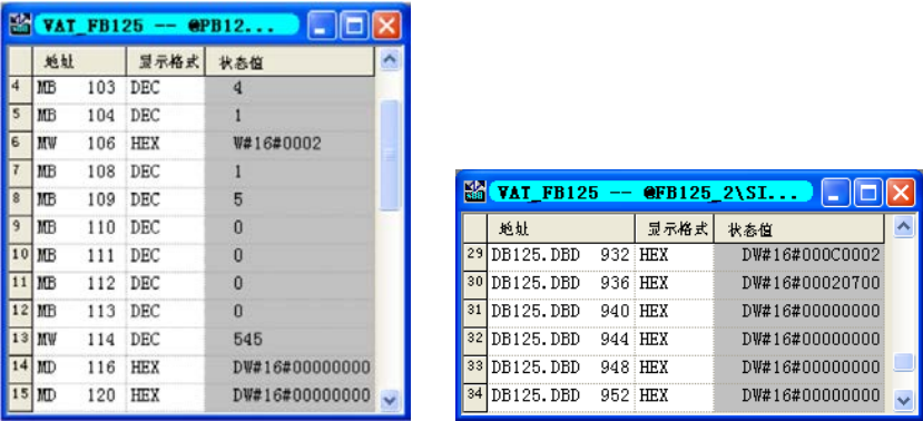
图 7-54 4 号从站断电的诊断数据
