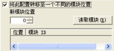
图 12-6 设置 AS-i 模块的位置
