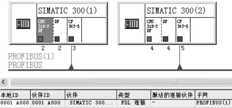
图 4-37 网络与连接组态
