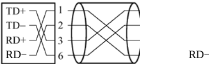
图 10-1 交叉连接
