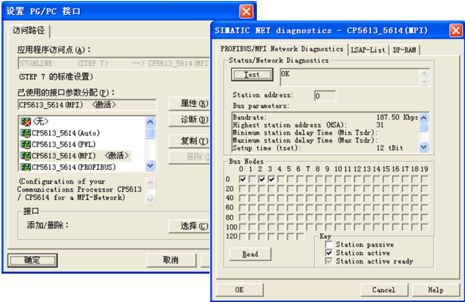
图 6-42 用 CP 5613 诊断 MPI 网络
