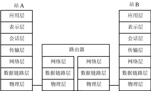
图 10-6 路由器
