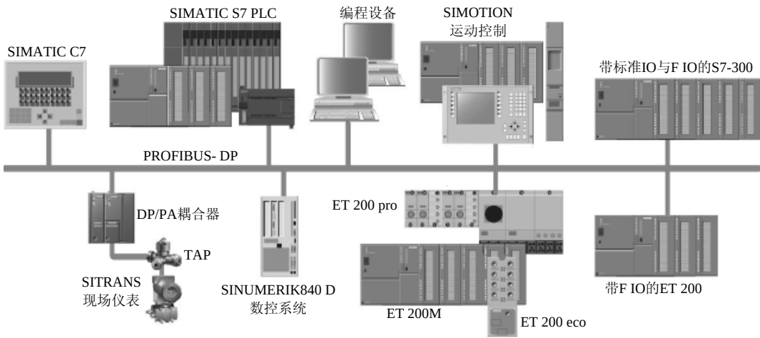
图 2-1 PROFIBUS-DP
