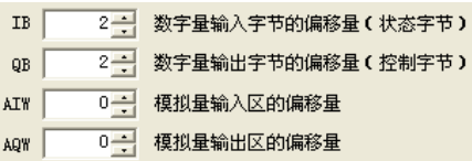
图 12-7 设置 AS-i 主站模块的地址
