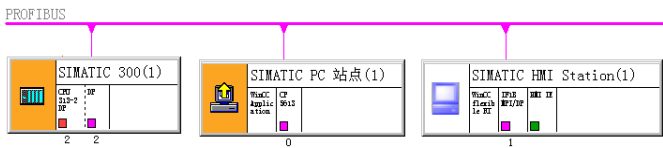
图 8-48 NetPro 中的站点
