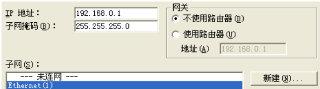
图 15-17 HMI 的以太网接口属性对话框
