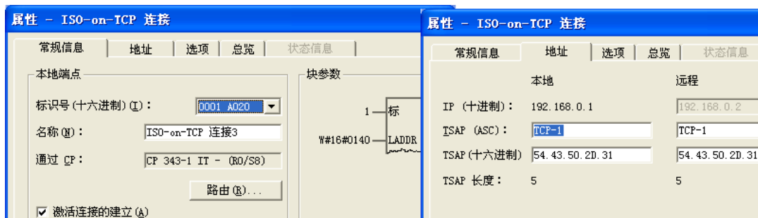
图 10-30 ISO-on-TCP 连接属性对话框
