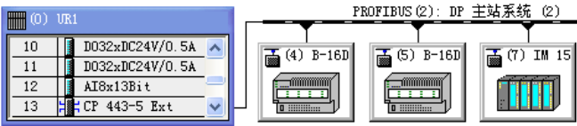
图 6-34 HW Config 中的 DP 网络
