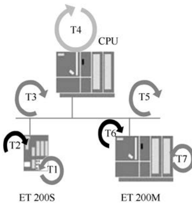
图 5-40 DP 网络的信号传输
