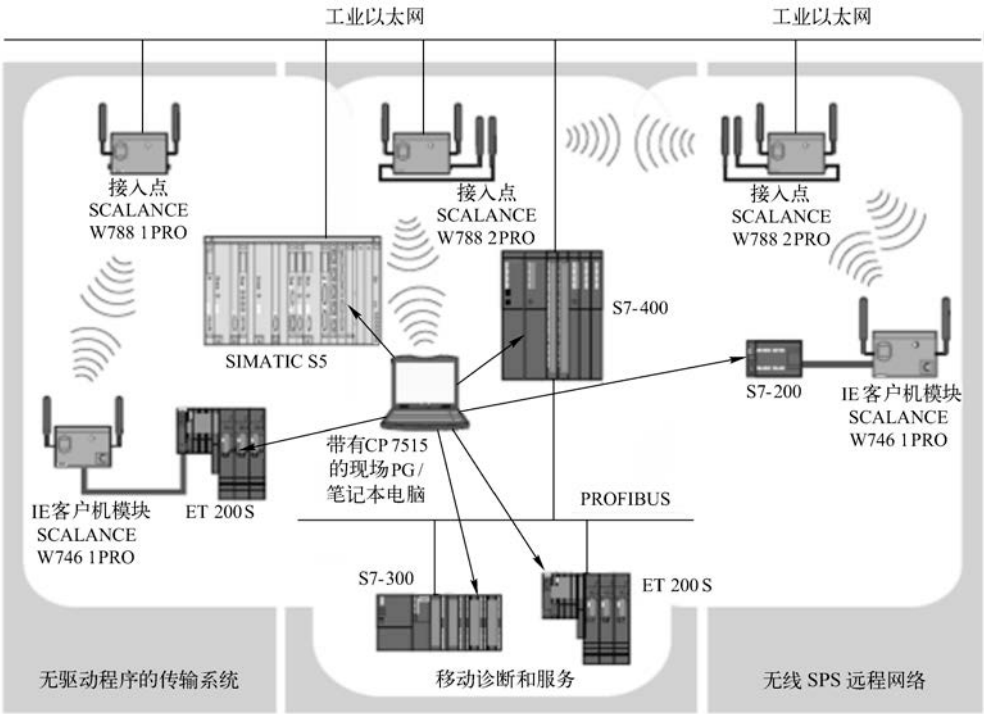
图 15-22 工业无线局域网
