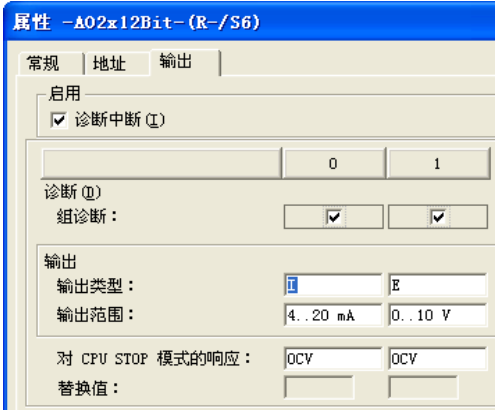
图 6-9 2AO 模块的属性对话框
