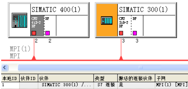
图 14-44 网络与连接的组态
