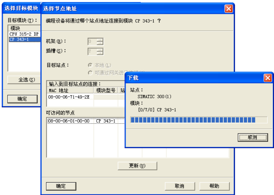
图 10-12 下载硬件组态信息
