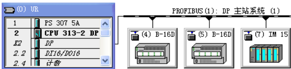
图 8-45 组态 DP 从站
