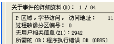
图 11-35 CPU 的模块信息对话框
