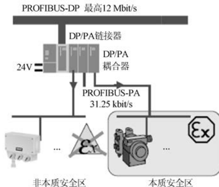
图 9-3 DP/PA 链接器
