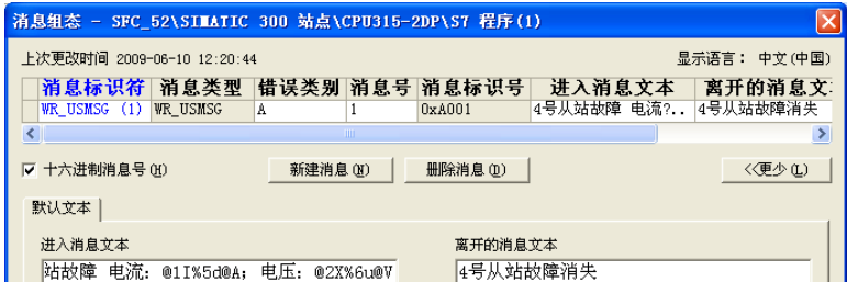
图 8-13 消息组态对话框
