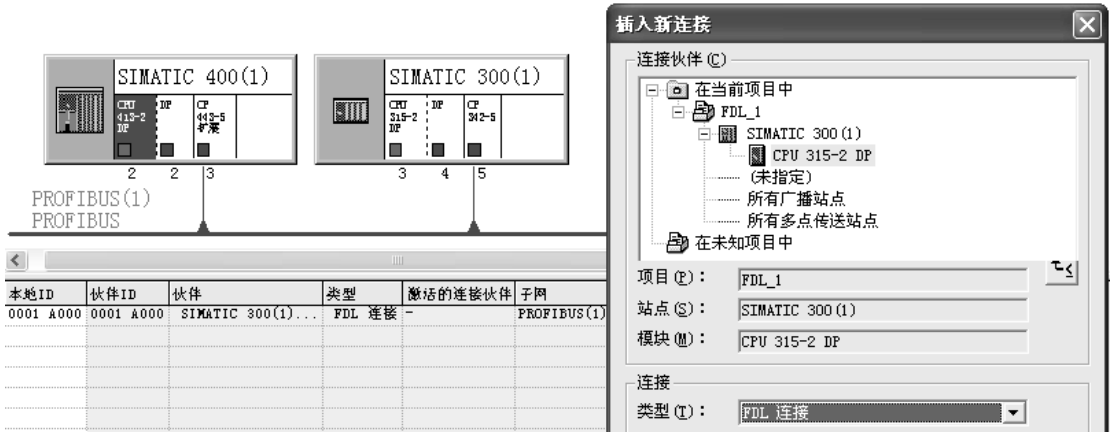
图 4-31 网络与连接组态
