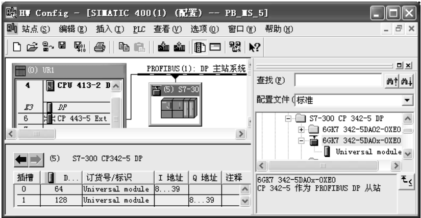
图 3-64 组态 DP 从站
