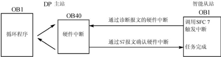
图 5-29 硬件中断执行过程示意图
