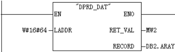
图 3-27 调用 SFC 14 的梯形图
