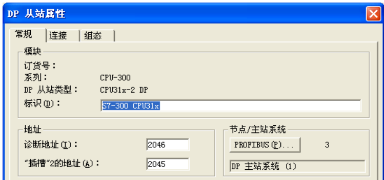
图 7-29 DP 从站属性对话框
