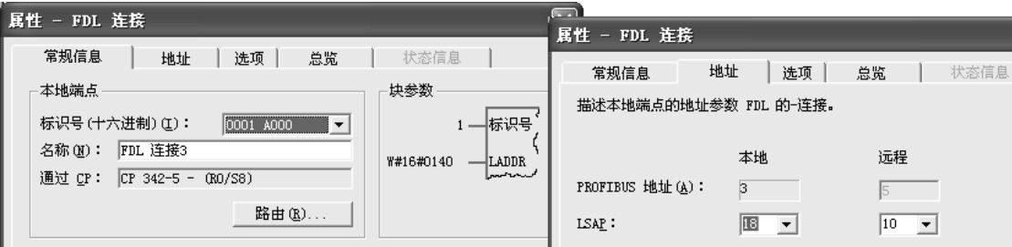
图 4-38 3 号站的 FDL 连接属性对话框
