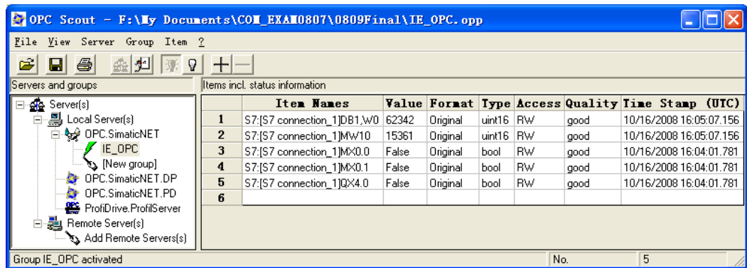
图 13-43 运行中的 OPC Scout
