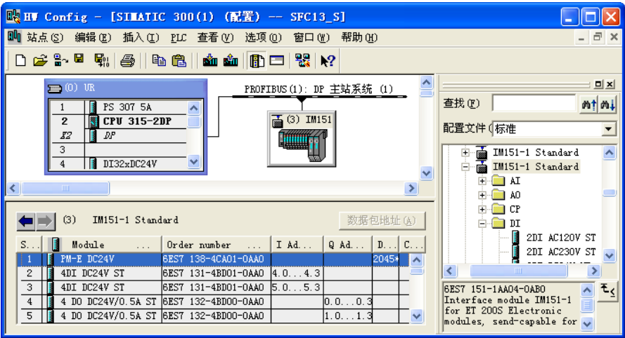
图 7-10 组态 ET 200S 从站
