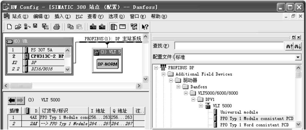
图 3-47 组态 DP 网络中的变频器
