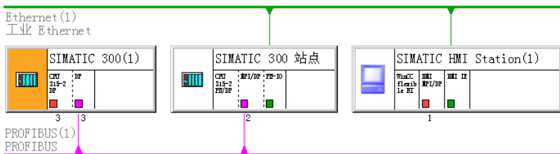
图 15-15 HMI 的 S7 路由功能
