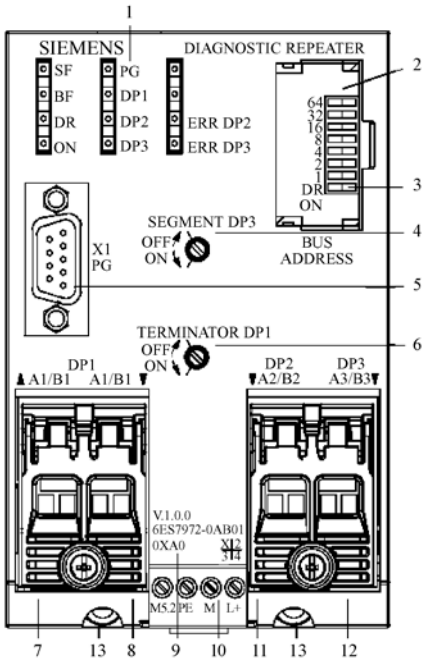
图 6-46 诊断中继器的面板
