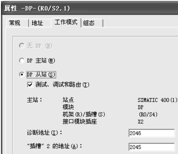
图 5-25 组态 DP 从站的工作模式
