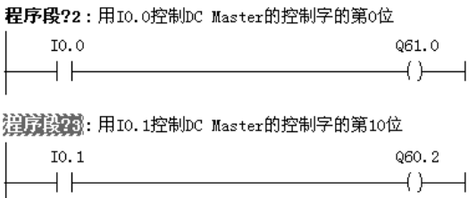
图 3-51 梯形图
