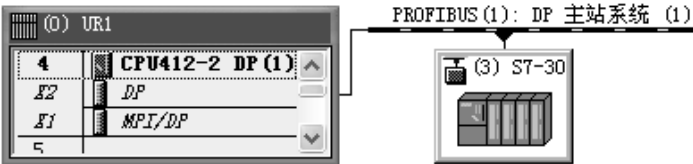
图 5-18 组态 DP 从站
