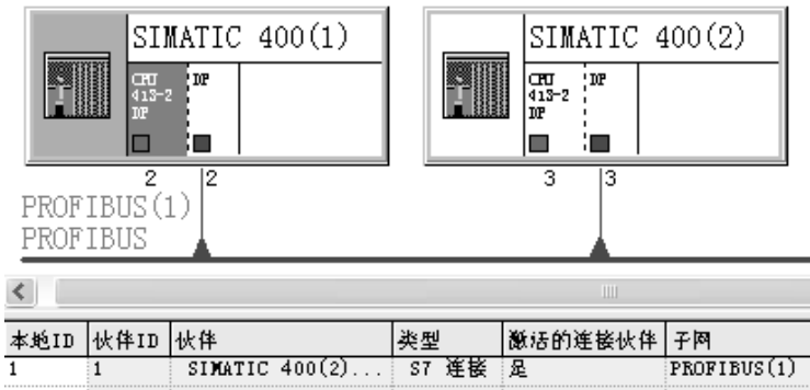
图 4-26 网络与连接的组态
