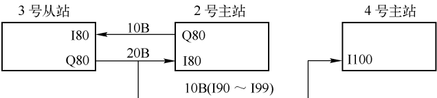
图 5-17 直接数据交换通信示意图
