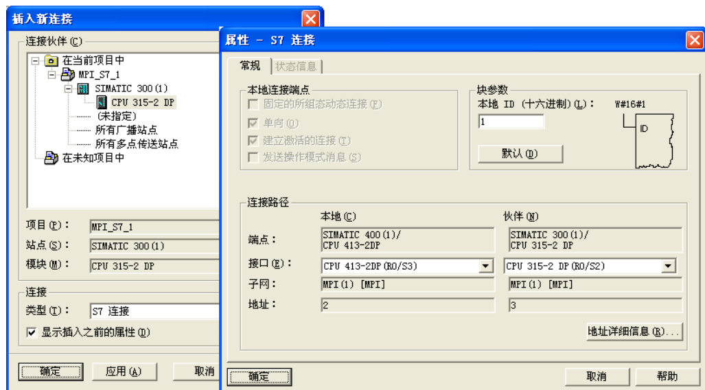
图 14-45 建立新的连接
