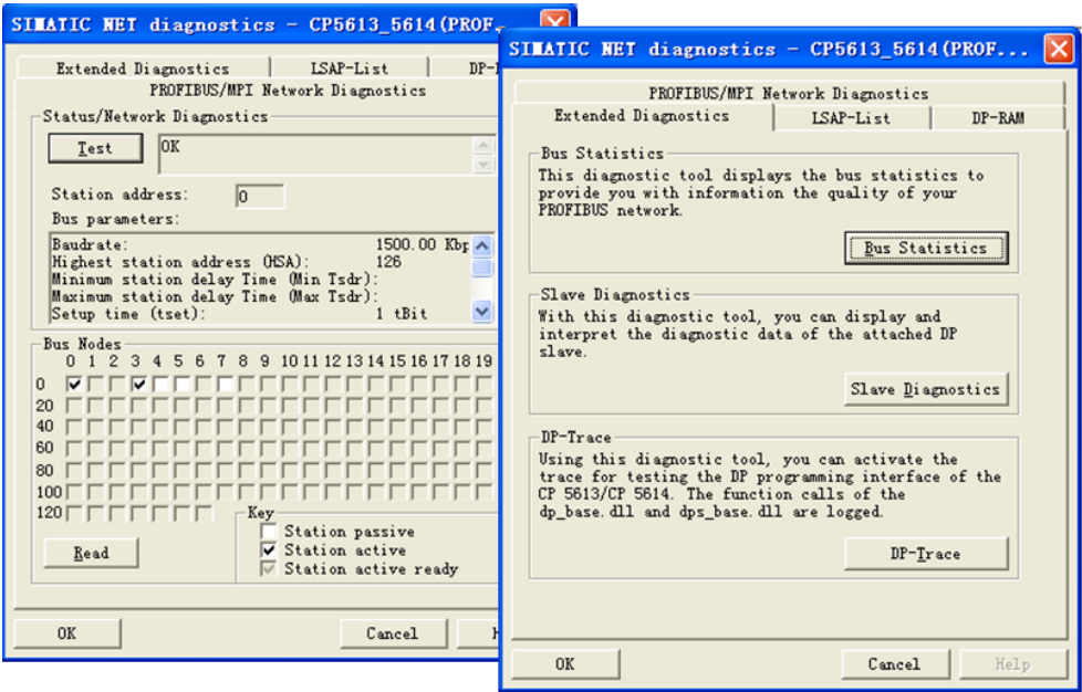
图 6-44 用 CP 5613 诊断 PROFIBUS 网络
