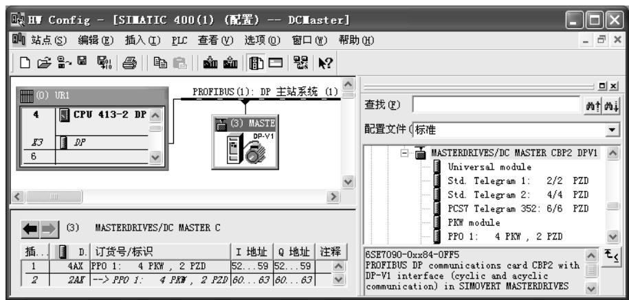
图 3-50 组态 DP 网络中的直流调速装置
