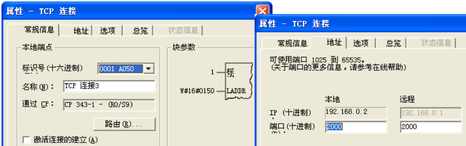
图 10-23 TCP 连接属性对话框
