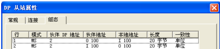
图 7-30 组态用于通信的输入/输出地址区
