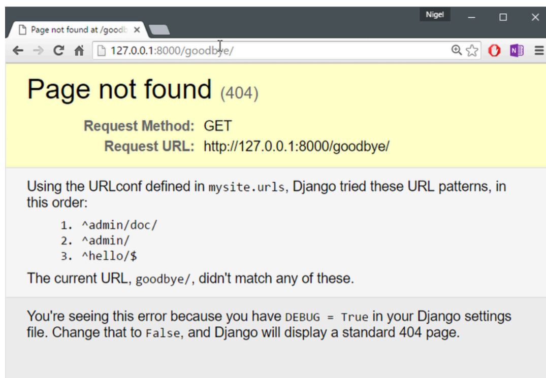
图 2-2: Django 的 404 页面
