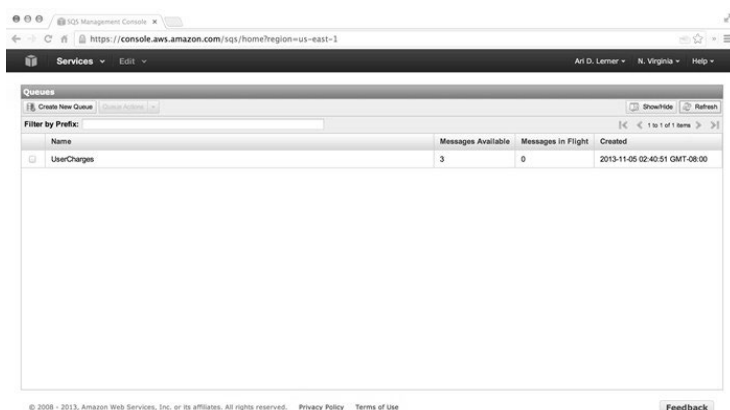
图18-19 SQS队列
