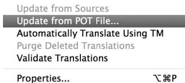
图27-4 翻译应用
