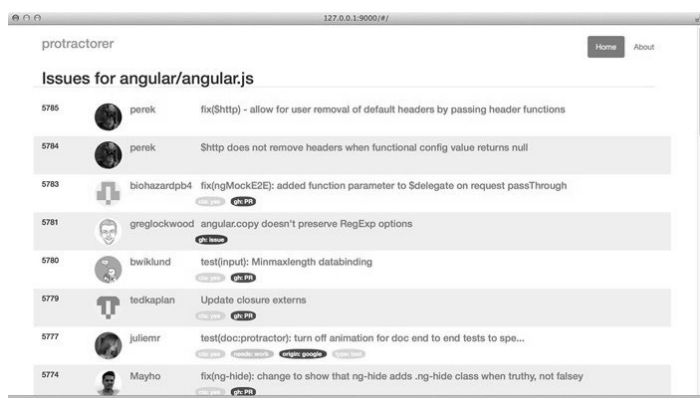
图19-10 最终应用
