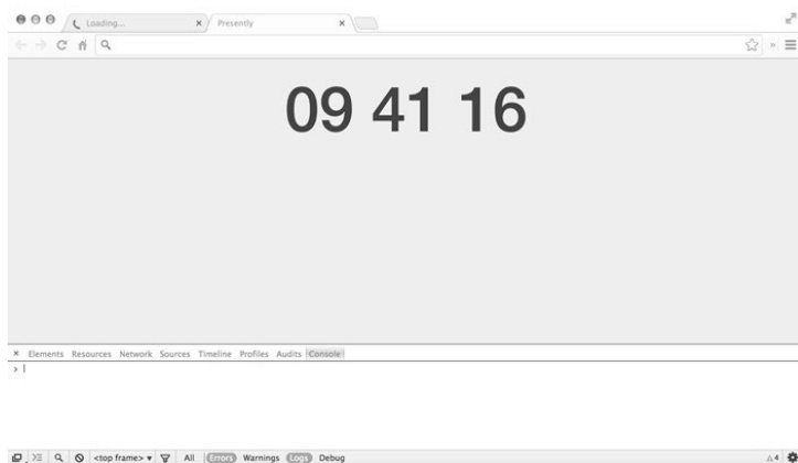
图31-5 第一个界面
