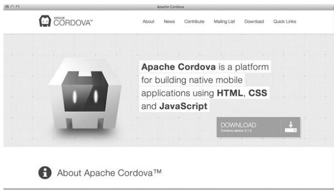
图26-2 Cordova
