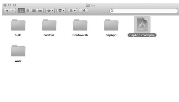
图26-5 生成的项目
