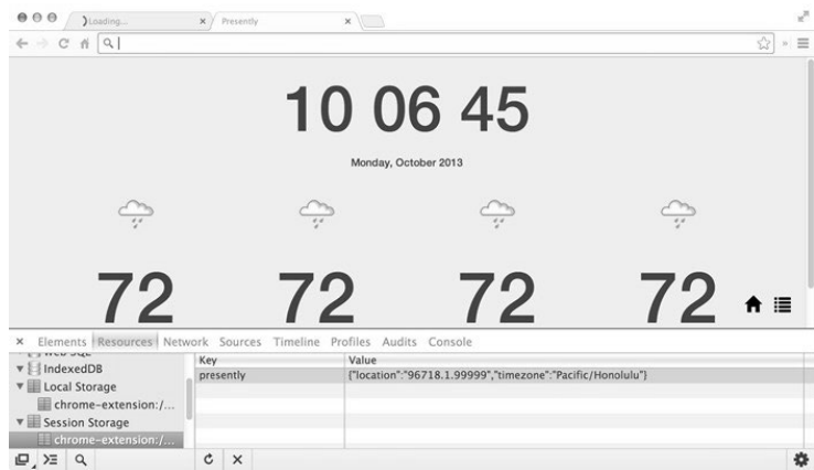
图31-14 夏威夷时区
