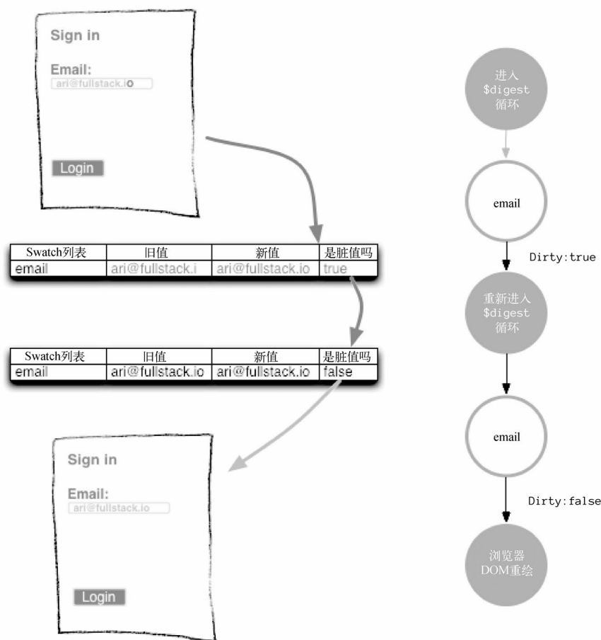
图23-1 digest循环
