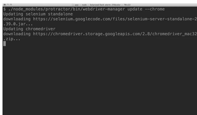
图19-7 安装Selenium
