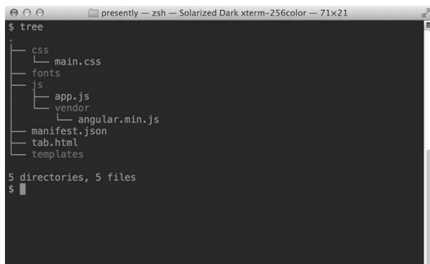
图31-2 文件结构
