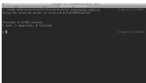
图19-11 运行过程
