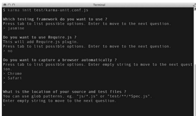
图19-2 Karma初始化
