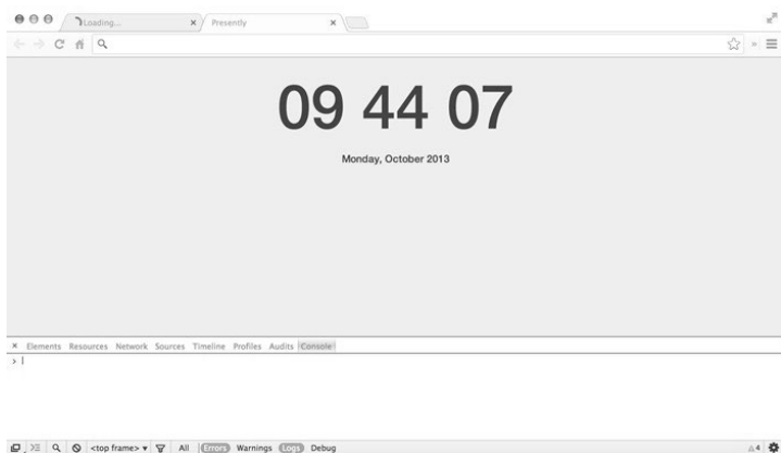
图31-6 完整的日期
