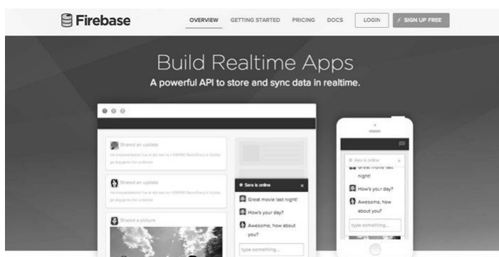
图18-21 注册过程
