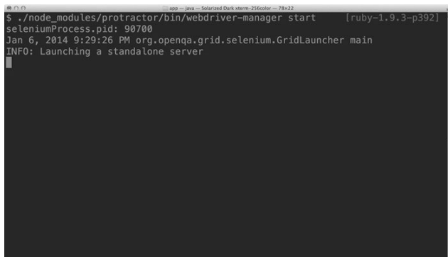
图19-8 安装Selenium
