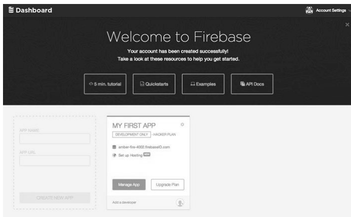
图18-23 注册过程
