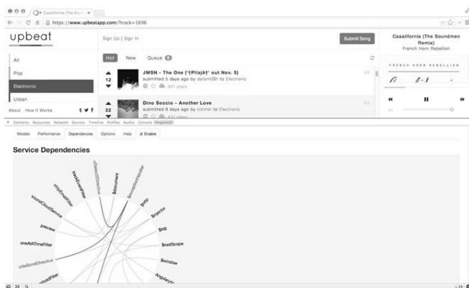
图33-4 依赖图表
