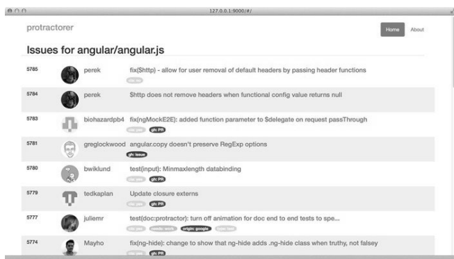
图19-13 测试列表页
