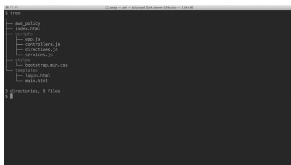
图18-5 Angular结构
