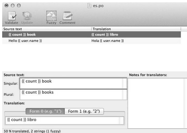
图27-3 翻译应用
