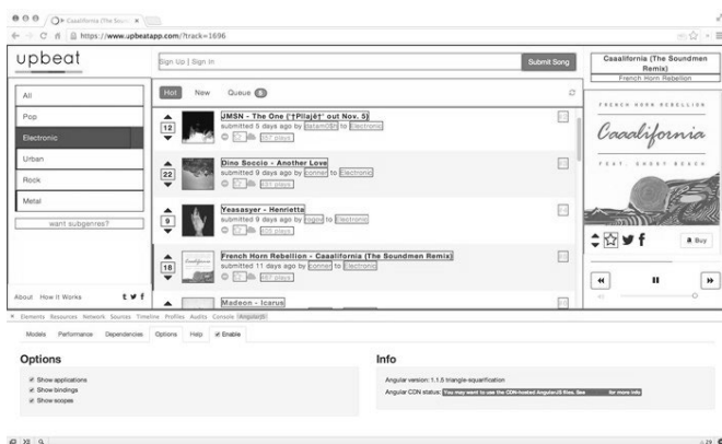
图33-5 选项面板
