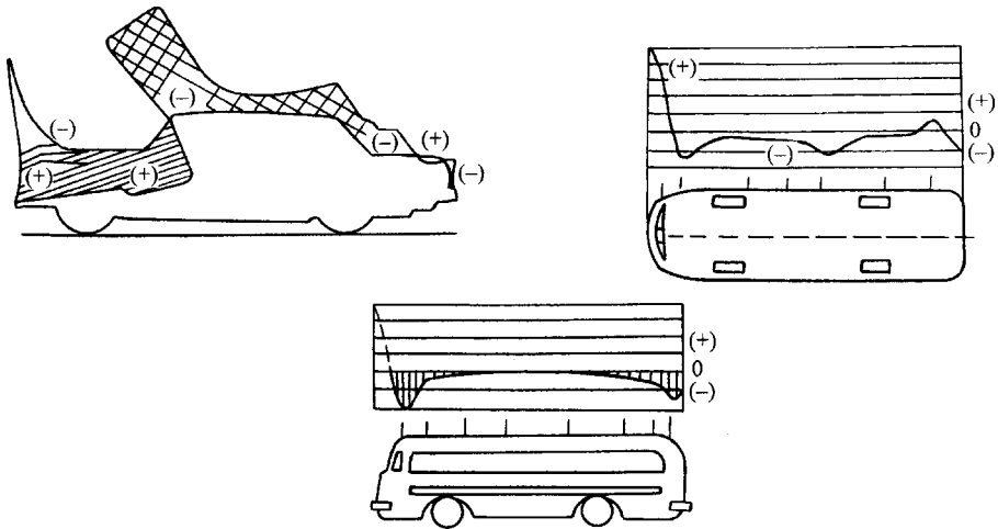
图 6-1 轿车和客车行车时车厢内外空气压力分布
