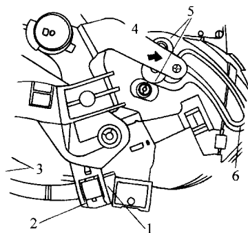
图 11-24 恒温开关的调整方法示意图
