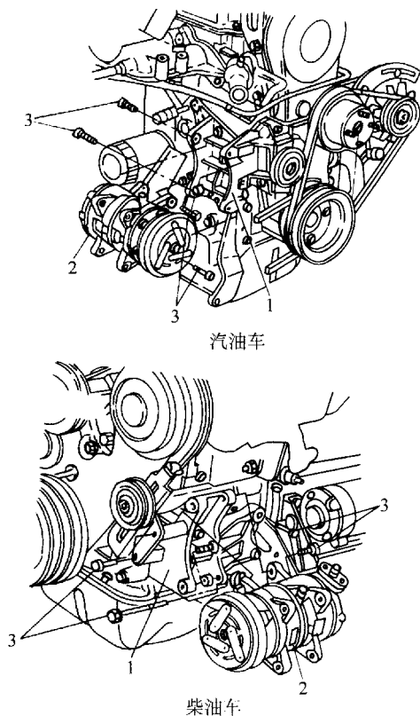
图 10-36 汽车空调压缩机的拆卸
