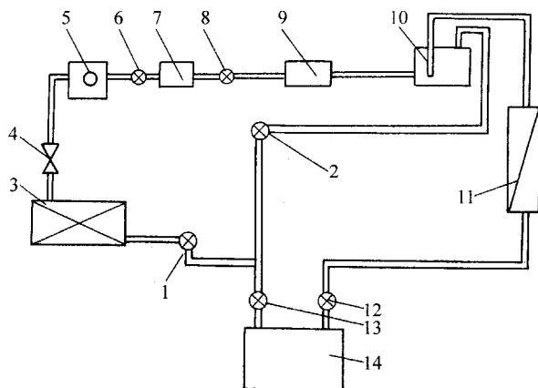
图 12-24 独立空调中几个维修用阀的位置
