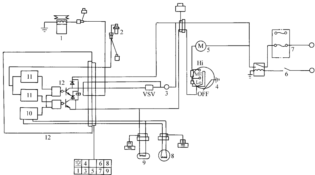
图 8-2 轿车空调电路
