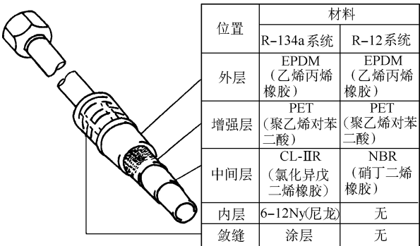
图 2-36 R—12 与 R—134a 橡胶管结构
