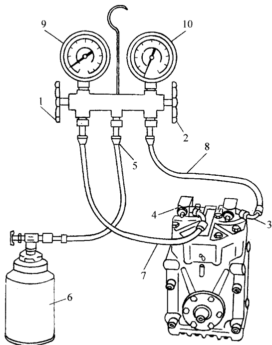
图 12-12 从低压端充注气态制冷剂
