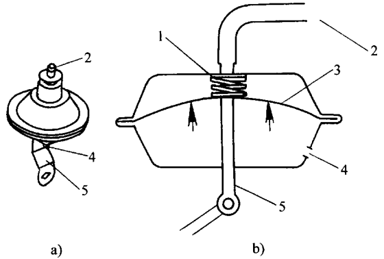
图 6-16 单膜片式真空驱动器
