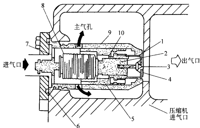
图 4-22 EPR- II 型阀
