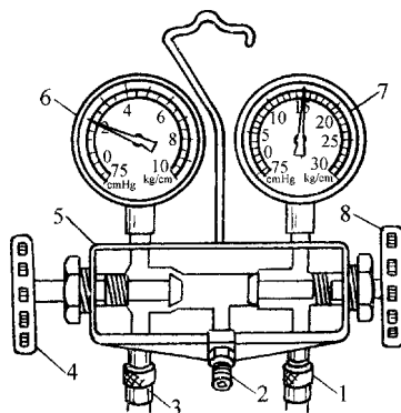
图 12-2 歧管压力表组
