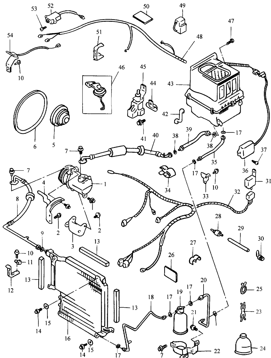
图 10-15 奥拓轿车空调制冷气装置结构组成图
