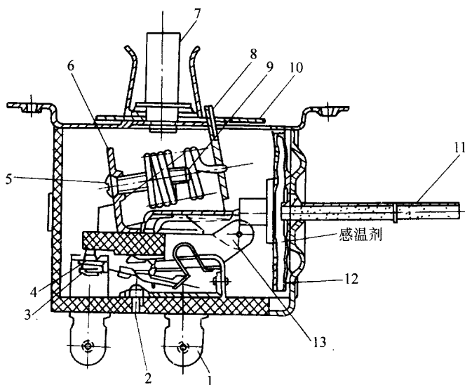
图 4-2 恒温器结构
