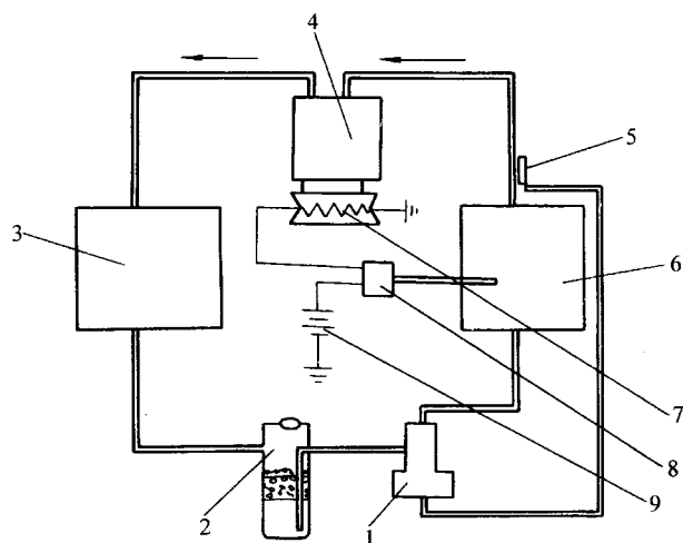
图 4-1 内平衡膨胀阀系统
