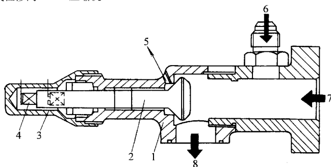
图 12-26 压缩机检修阀结构
