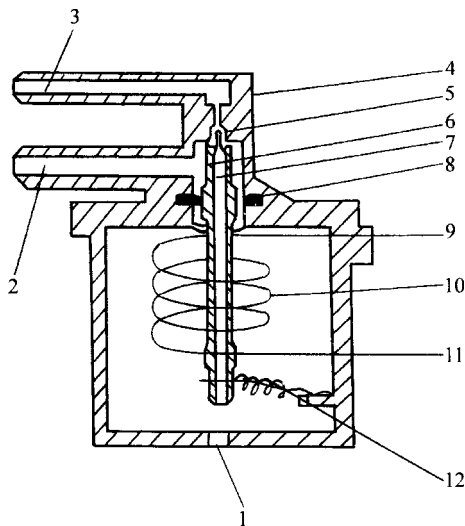
图 6-23 真空换能器（通用公司用）
