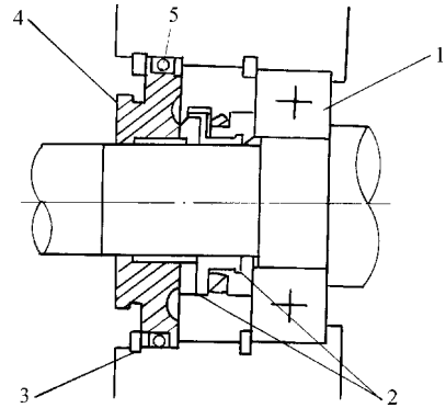
图 2-6 轴封结构
