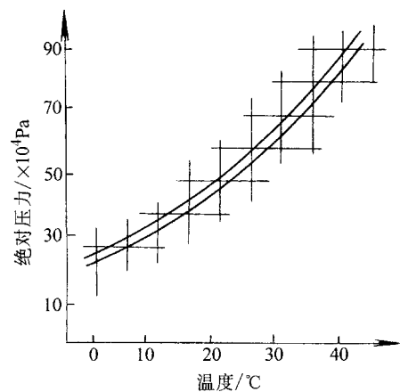
图 11-20 红旗 CA630 轿车空调膨 胀阀调整曲线
