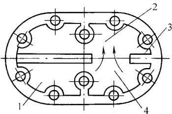
图 17-3 垫片中筋击穿 1—高压腔 2—低压腔 3—中筋 4—气流
