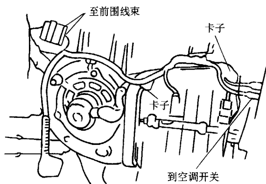
图 10-9 拆开空调前围线束导线插头、卡子
