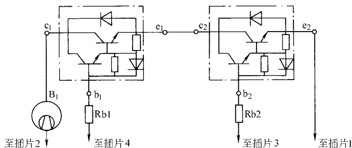
图 17-25 用富士 EVL31—055 模块代换接线图
