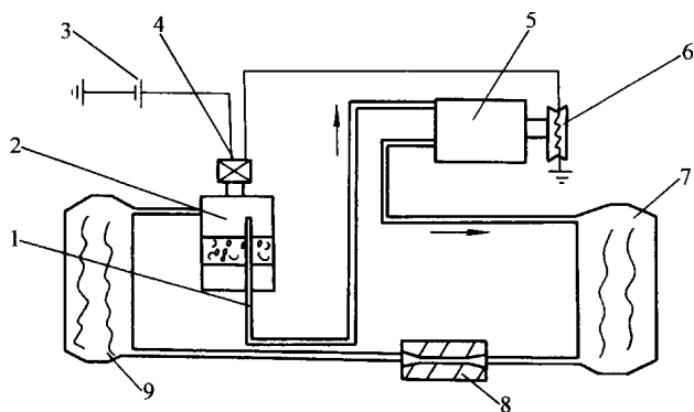
图 4-11 用压力开关控制的 CCOT 制冷系统
