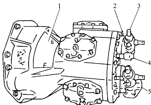
图 12-25 压缩机上吸、排气检修阀
