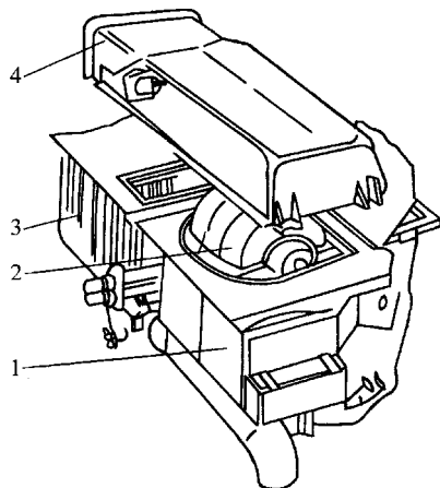
图 5-3 整体空调器
