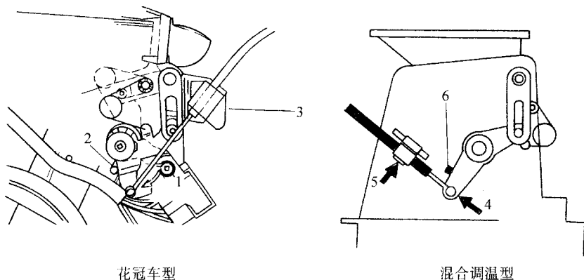
图 11-1 固定住进气风门钢索
