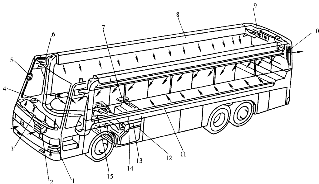
图 6-35 高级豪华旅游车空调系统的布局
