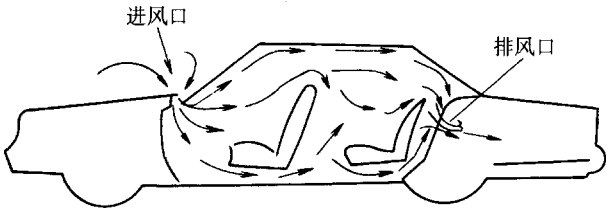
图 6-3 轿车空调风的循环
