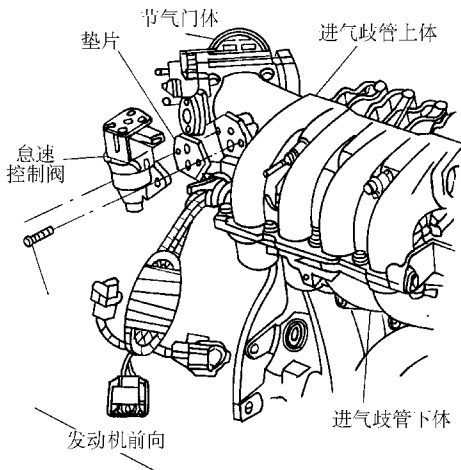
图 17-20 福特天霸轿车怠速控制阀的位置
