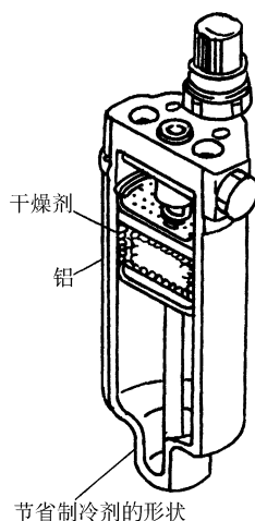
图 2-34 R—134a 储液干燥器结构
