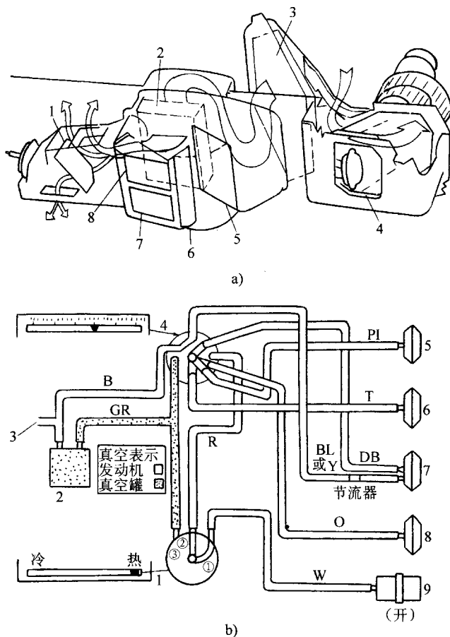
图 6-12 供暖时的空气流路与真空回路状态
