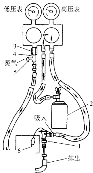
图 11-19 膨胀阀的检查调整方法 1—膨胀阀 2—制冷剂罐 3—螺纹活接头 4—活三通接头 5—接头盖 6—感温包
