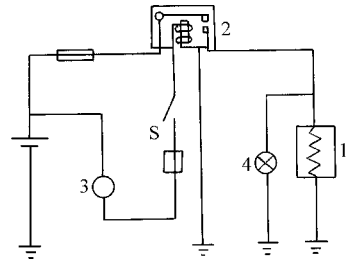
图 8-14 除霜电路
