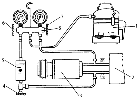
图 12-16 加注冷冻润滑油装置
