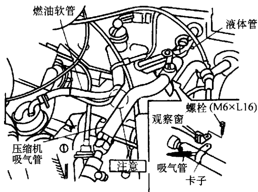
图 10-8 拆卸压缩机吸气管和液体管
