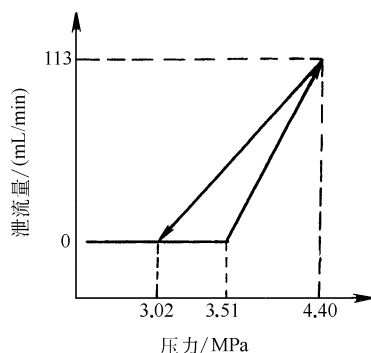
图 2-33 压缩机安全泄压阀工作特性
