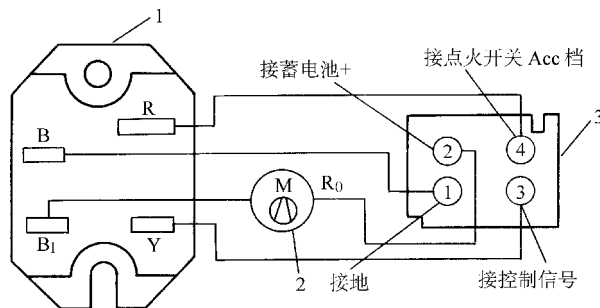
图 17-24 奔驰 600 轿车空调鼓风机控制线路图
