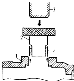
图 12-44 滑动轴承的安装
