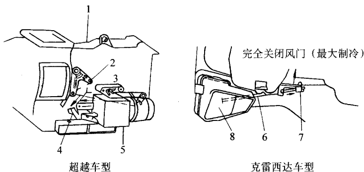
图 11-12 混合空气风门连杆调整方法
