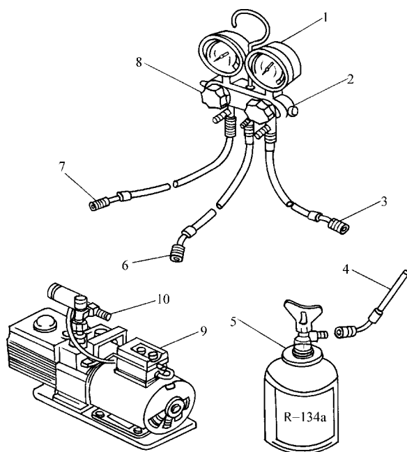
图 17-13 制冷剂的加注
