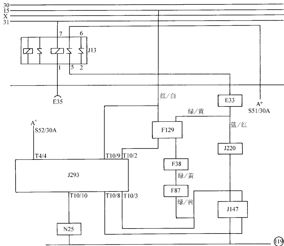
图 17-10 捷达前卫轿车空调系统电路图
