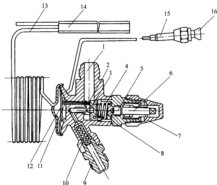
图 4-25 外平衡膨胀阀构造
