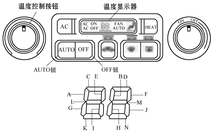
图 17-33 车内温湿度控制面板
