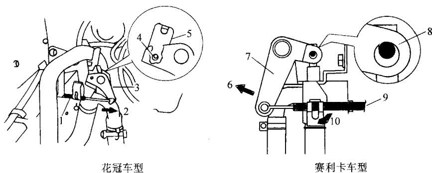
图 11-4 固定住热水开关钢索
