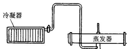
图 9-11 冷凝器与蒸发器之间的接管方式
