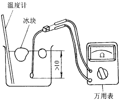
图 11-21 热敏电阻检查方法
