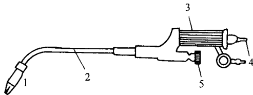
图 9-14 焊枪
