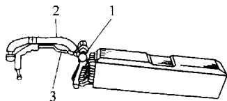
图 10-30 后梁上蒸发器 and 膨胀阀的布置 1—膨胀阀 2—回气管 3—供液管
