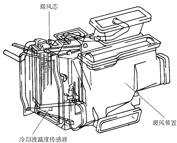
图 1-11 冷却液温度传感器
