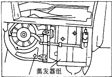
图 10-25 仪表板下部的冷风机
