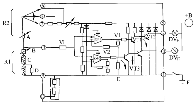
图 8-13 自动温度控制电路
