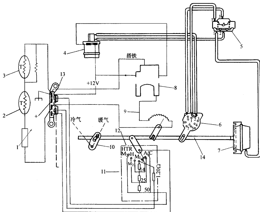
图 6-22 半自动空调的工作原理
