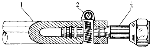
图12-10 软管与接头之连接 1—软管 2—管夹 3—插入接头
