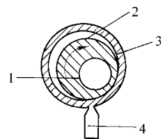
图 2-20 活塞滚动原理
