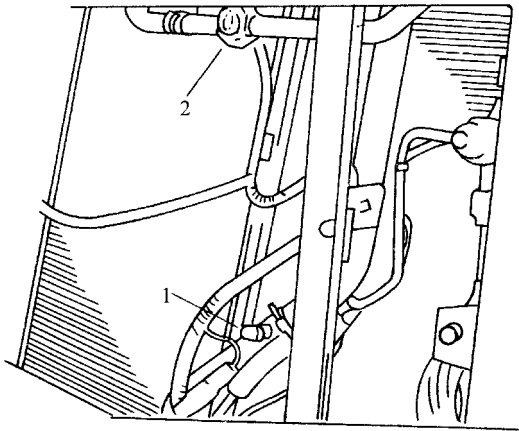
图 12-27 独立空调吸气管上的制冷剂注入阀 1—制冷剂注入阀 2—视液镜
