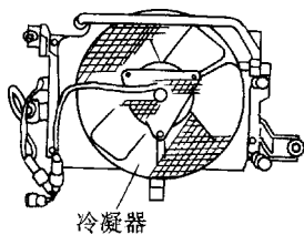
图 10-31 底部冷凝器机组
