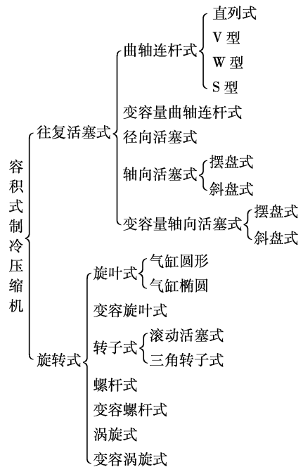
图 2-2 汽车空调压缩机分类
