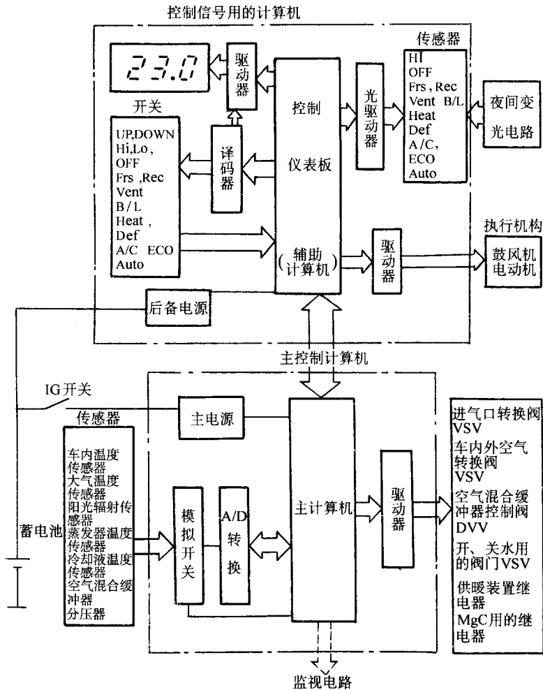
图 6-29 微电脑控制汽车空调的组成和接口
