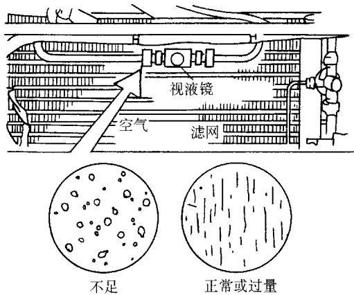
图 12-28 视液镜的制冷剂流动状态
