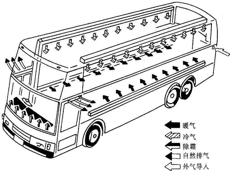
图 6-2 大客车空调风在车内的循环
