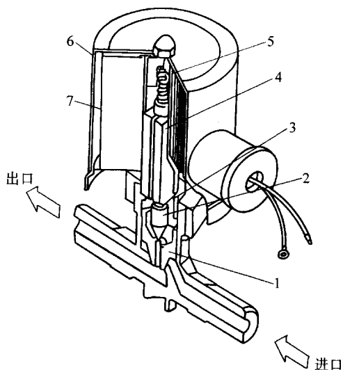
图 4-26 电磁旁通阀
