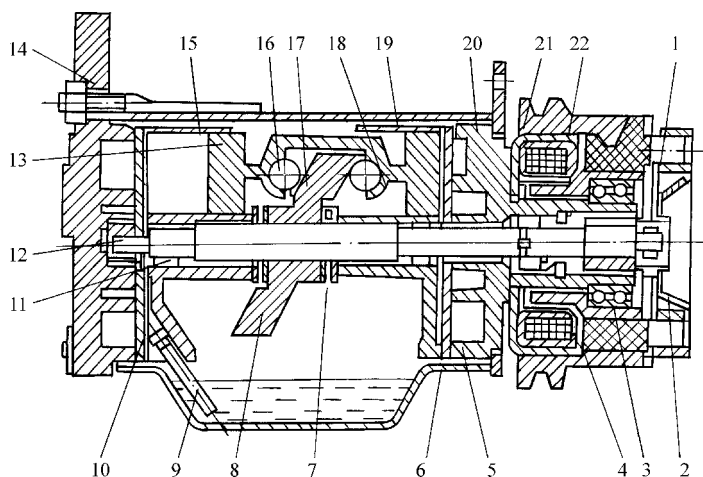
图 2-12 斜盘式压缩机剖视图
