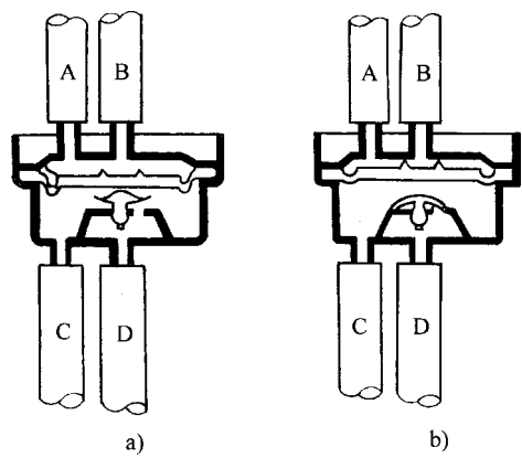
图 6-24 真空保持器
