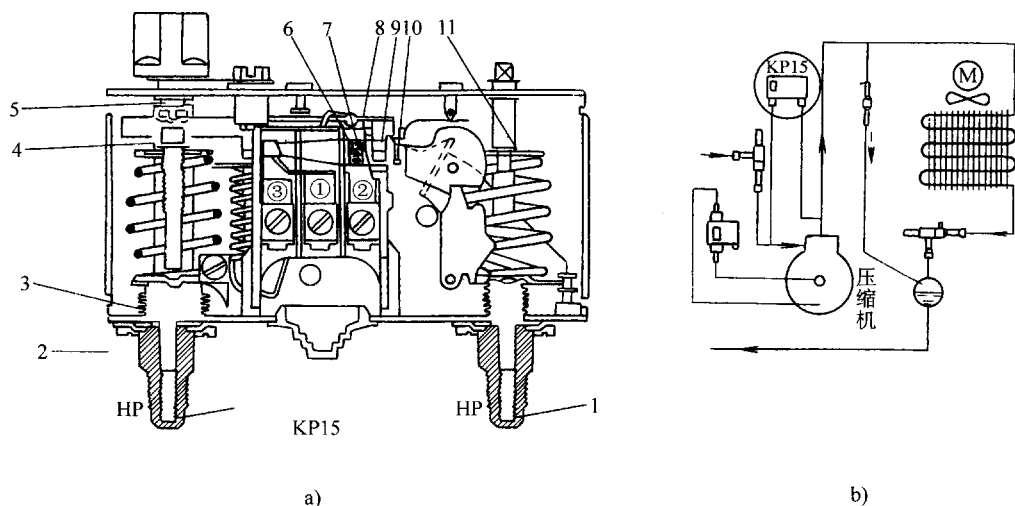
图 7-6 KP 型高低压控制器结构及在系统中的安装
