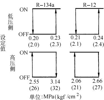
图 2-35 R—134a 与 R—12 压力开关动作特性对比
