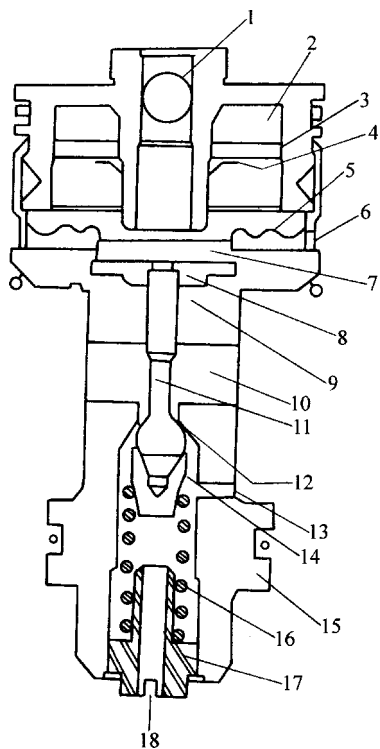
图 4-21 VIR 阀中的膨胀阀
