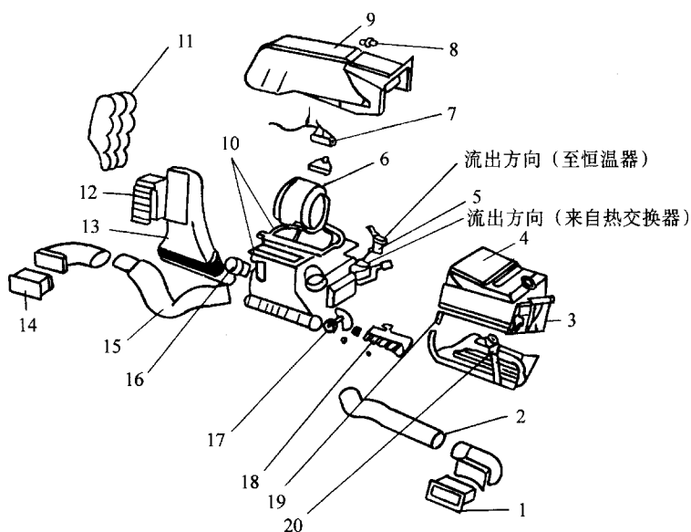
图 10-2 可不用专用设备拆装的零部件
