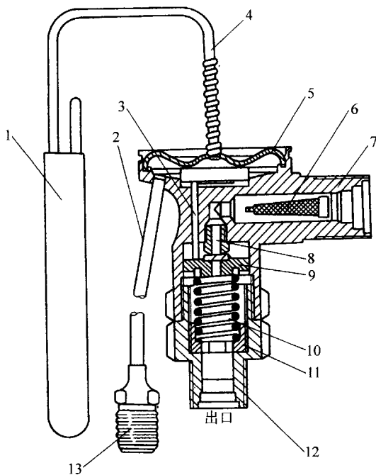
图4-15 外平衡膨胀阀
