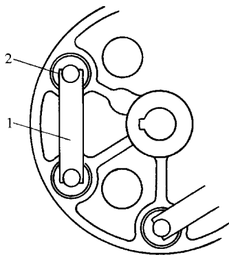
图 12-40 法兰盘的防松装置
