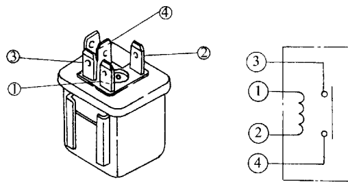
图 11-17 马自达汽车空调后侧继电器
