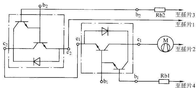
图 17-26 用三菱 QW100DY—H 模块代换的接线图
