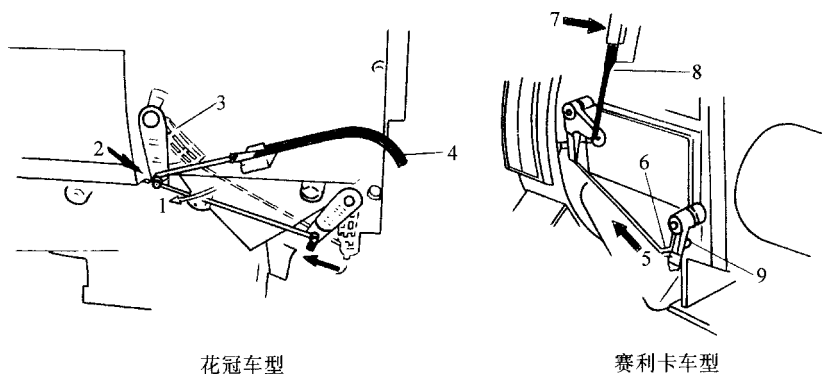
图 11-3 固定住混合调温风门钢索
