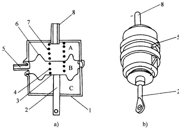
图 6-17 双膜片式真空驱动器
