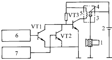
图 8-3 放大电路原理图
