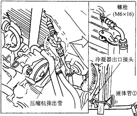
图 10-14 拆下冷凝器、储液罐
