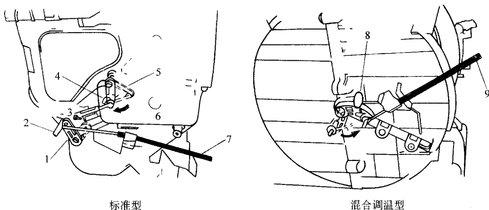
图 11-2 固定住功能选择风门钢索
