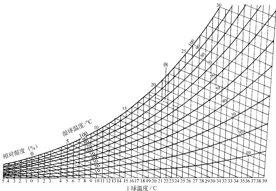
图 16-7 空气温湿图
