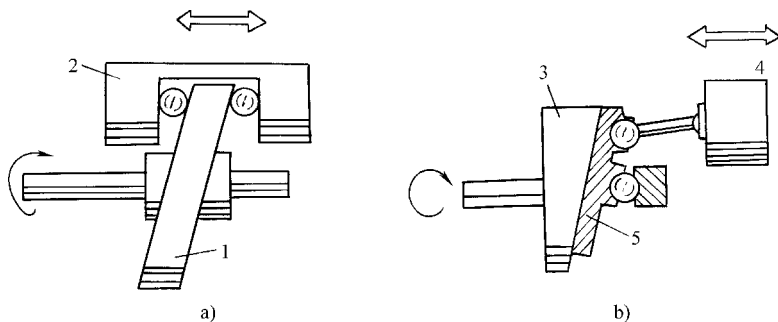
图 2-11 斜盘式与摆盘式压缩机原理和结构比较
