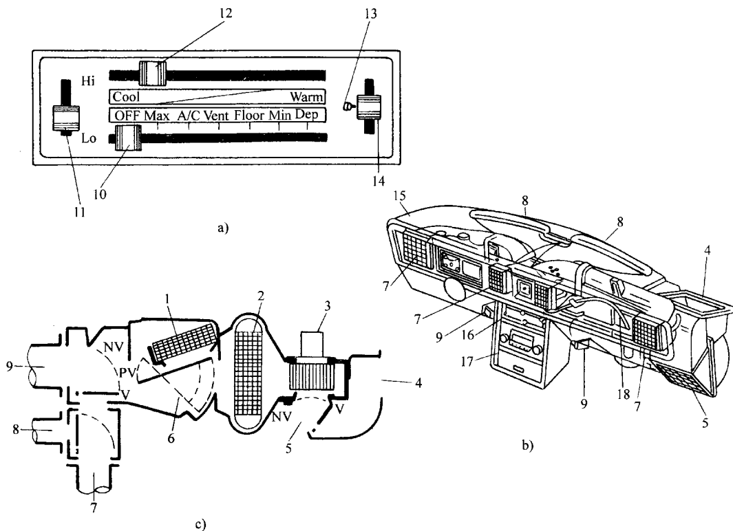
图 6-6 关闭空调时, 空调器工作状态
