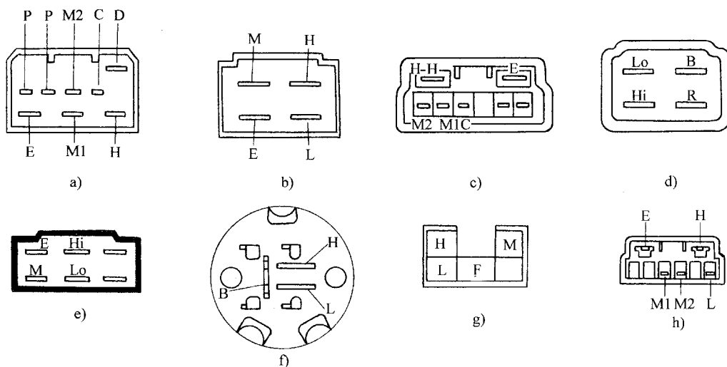
图 11-5 送风开关终端标志图
