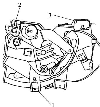
图 11-25 微动开关的调整方法示意图
