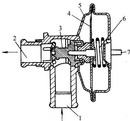
图 5-5 真空冷却液控制阀
