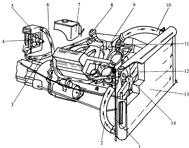
图 5-1 水暖系统工作原理
