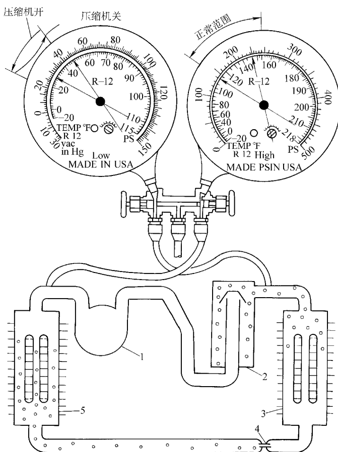
图 16-2 CCOT 系统高、低压力测试
