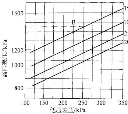
图 16-6 大型客车独立 空调标准高压值
