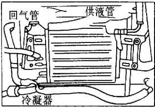
图 10-22 冷凝器的安装方法
