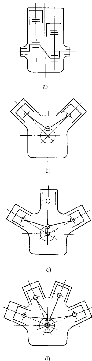
图 2-4 气缸的布置形式
