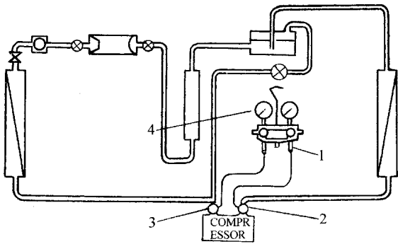
图 12-29 泵储制冷剂 1—高压接口 2—排气检修阀 3—吸气检修阀 4—低压接口
