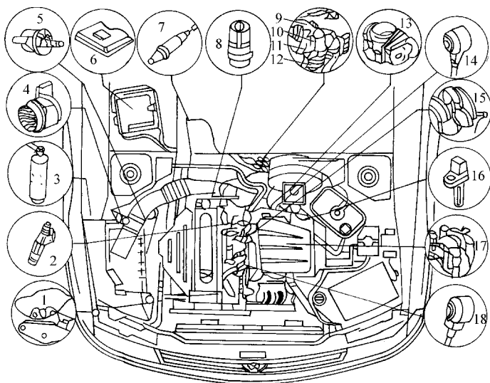
图 8-1 桑塔纳 2000GSi 时代超人轿车发动机部分传感器和执行器安装位置图
