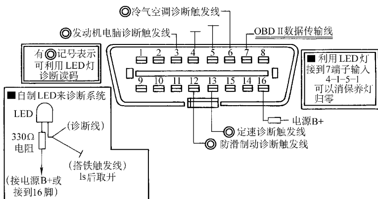
图 17-27 沃尔沃 960 轿车发动机故障码的读取方法
