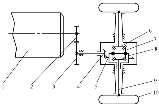
图 1-29 电动叉车传动系统
