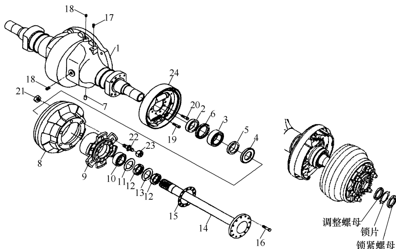
图 3-29 驱动桥轮毂轴承调整及润滑脂加注
