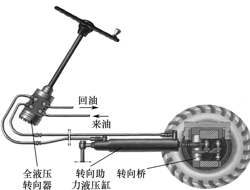
图 1-36 叉车全液压式转向器
