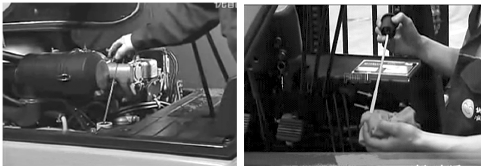
图 3-46 液压油检查
