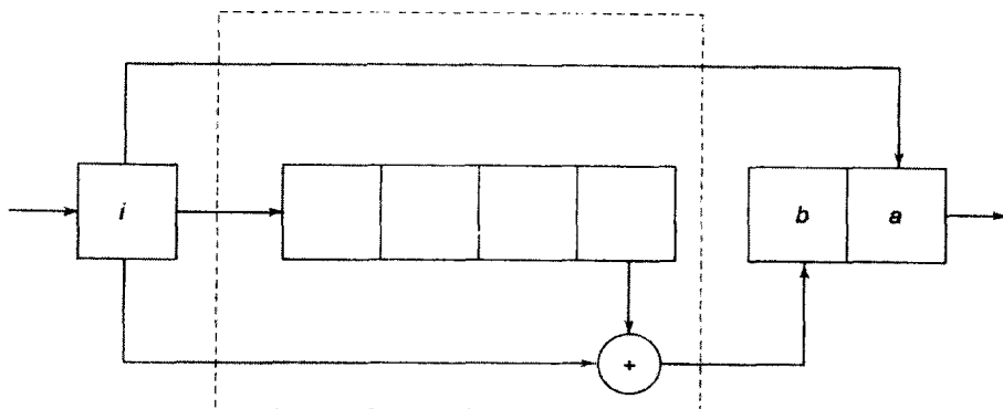
图6-10 码率为1/2的卷积编码器，其中 G(D)=[1 \ D^4+1]
