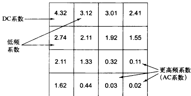
图1-19 一些典型离散余弦变换（DCT）值
