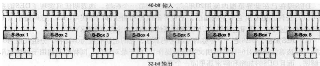
图8-3 S盒替换
