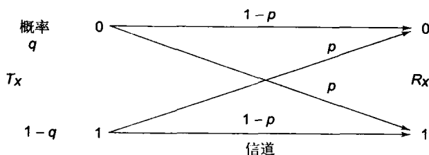
图1-6 一个输入符号概率为 q 和 1-q 的二元对称信道 (BSC)
