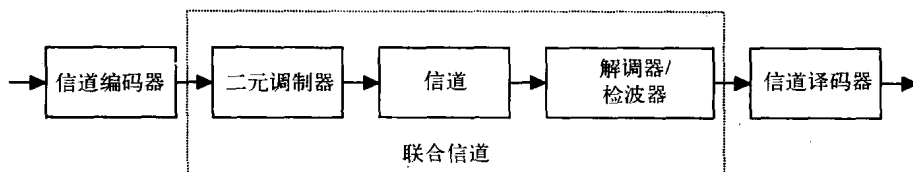
图2-2 一种联合的离散输入离散输出信道（由调制器和解调器/检波器组成）
