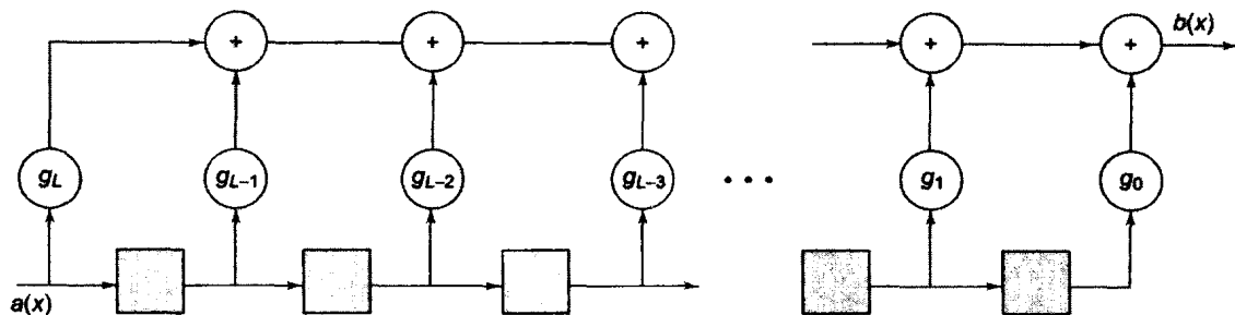
图4-5 两个多项式 b(x) = a(x)g(x) 产生的有限脉冲响应过滤器实现
