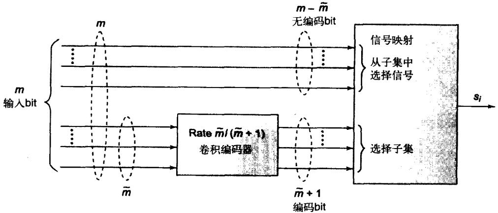
图7-7 TCM编码器的一般结构
