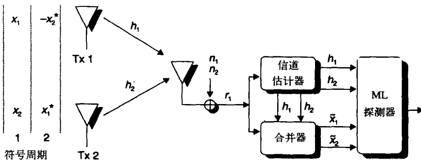
图3-7 Alamouti的两天线发射分集机制
