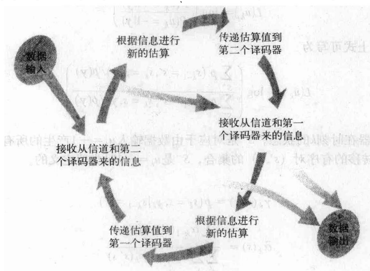
图6-30 Turbo码的迭代译码
