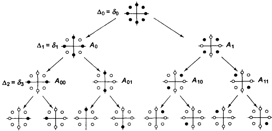
图7-6 8PSK信号集的集合分割
