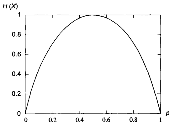
图1-4 二元熵函数 H(X) = -p \log_2(p) - (1-p) \log_2(1-p)
