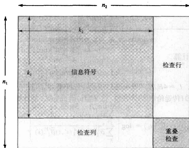
图6-32 一个乘积码 P=C_1 * C_2 的例子
