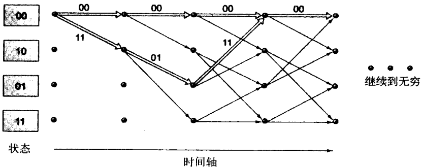
图6-14 在网格图中有多于一对的路径可用于计算 d_{free}
