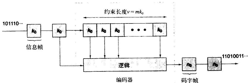
图6-2 生成树码的移位寄存器编码器
