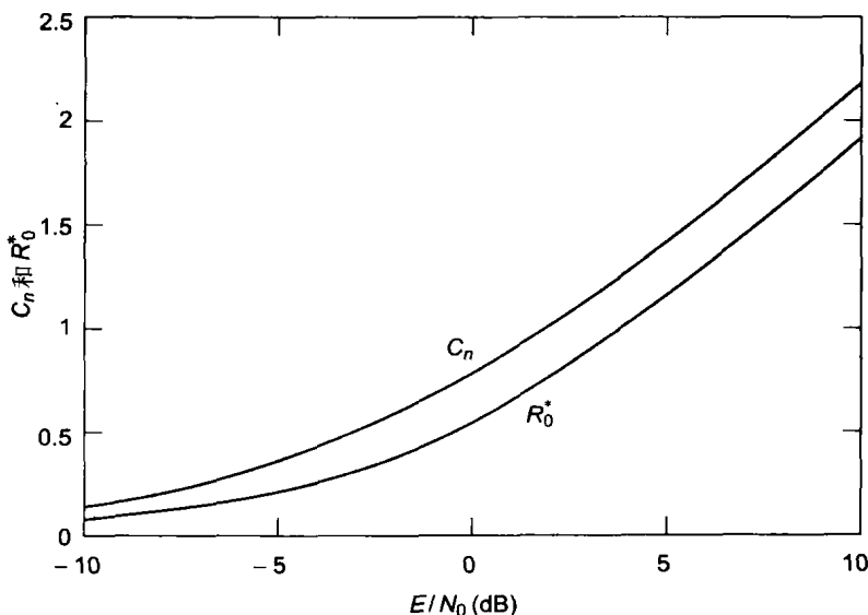
图2-9 AWGN信道的规范容量 C_n 和切断率 R_0^*
