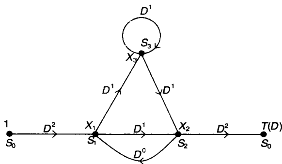
图6-15 图6-3中的卷积码的修改过的状态图
