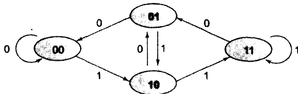
图6-4 例6.1中的编码器的状态图
