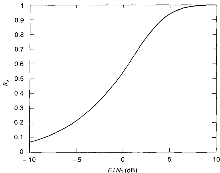
图2-8 切断率 R_0 相对每维的 SNR (dB数)
