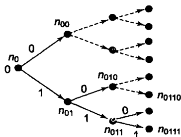
图1-10 利用二叉树构造二元前缀码
