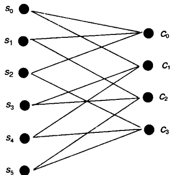
图3-6 例3-28中1/3线性码对应的Tanner 图
