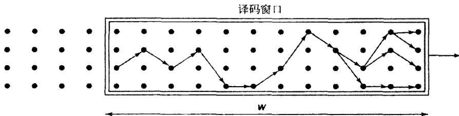
图6-23 维特比译码器就像一个滑动窗从中可以看到网格
