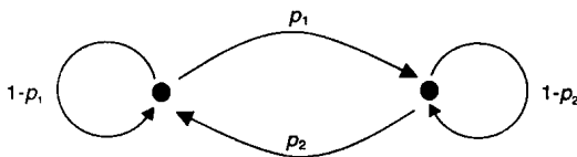
图1-18 两状态马尔可夫链的状态转换图
