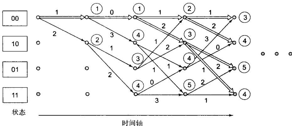
图6-22 维特比译码第四步后的路径尺度
