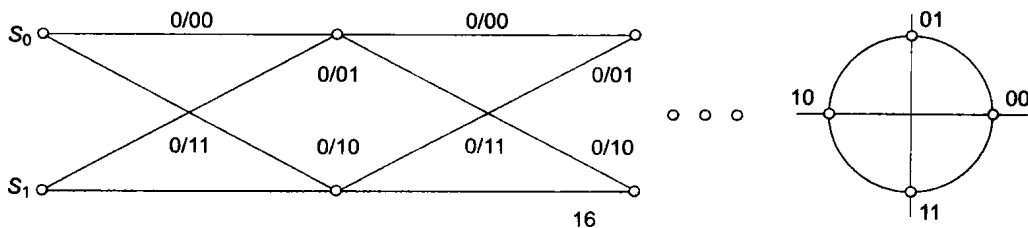
图7-15 两个状态的网格图
