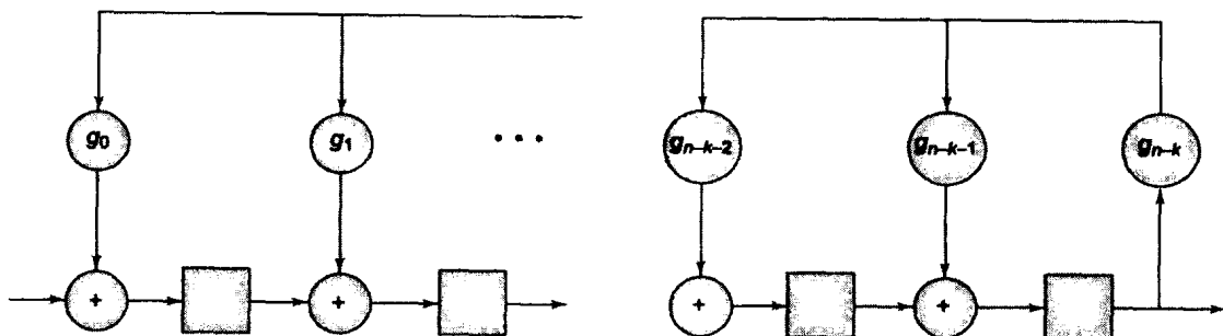
图4-7 用移位寄存器做对 g(x) 的除法
