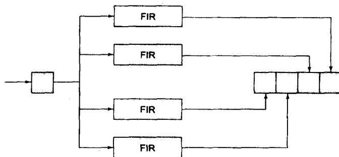
图6-7 k_0 = 1 和 n_0 = 4 的FIR过滤器中的卷积编码器
