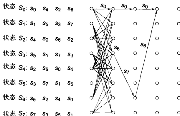
图7-10 例7.7中的编码器的网格图
