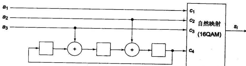
图7-14 与图7-13中网格图等价的系统编码器
