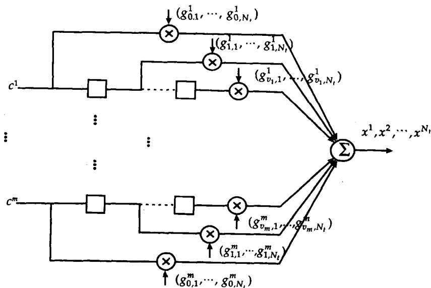
图7-20 STTC的编码器
