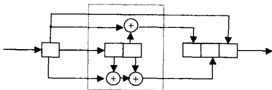
图6-25 例6.11的卷积编码器
