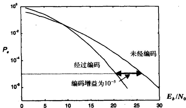
图3-4 编码增益图示
