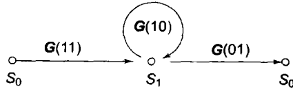
图7-18 错误状态图
