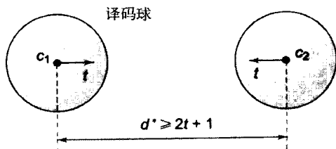
图3-2 译码球
