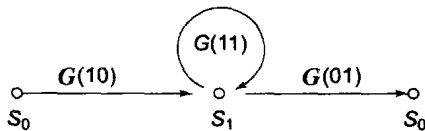
图7-16 错误状态图
