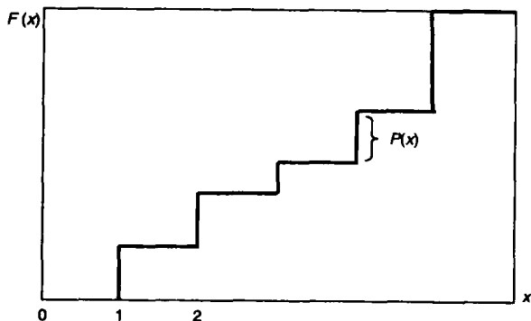
图1-15 累积分布函数
