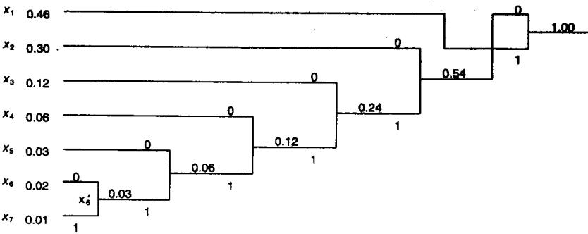
图1-13 例1.13中的霍夫曼编码
