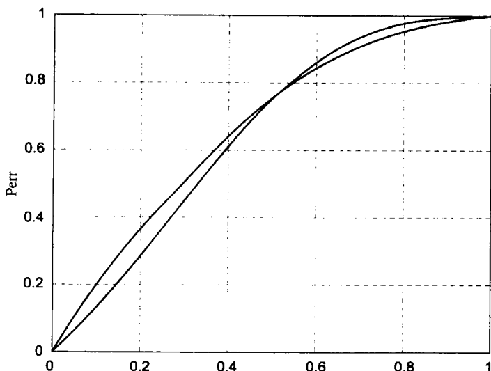
图3-3 对2比特消息有编码和无编码下的 P_{err} 的比较
