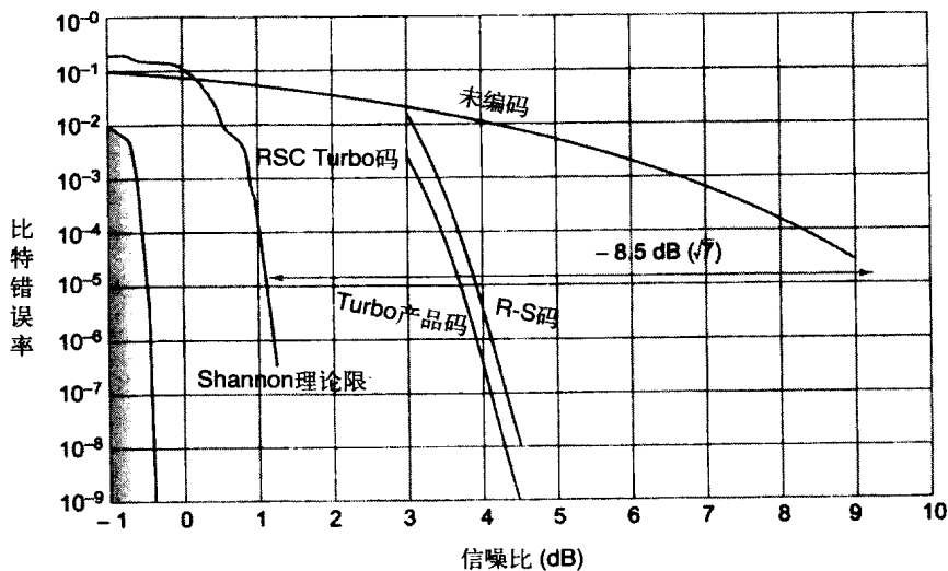
图6-34 不同编码系统的比较
