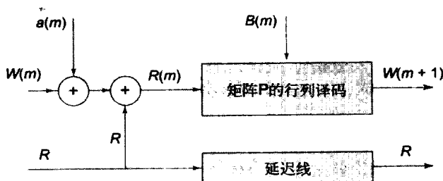
图6-33 基本分组Turbo译码器框图
