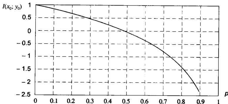
图1-3 互信息 I(x_0; y_0) 关于错误概率 p 的对应平面图
