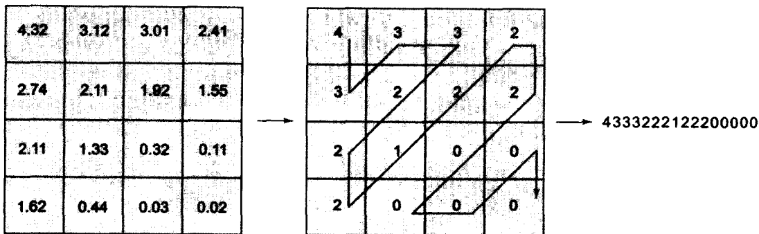
图1-20 一个量化后用锯齿形编码的例子
