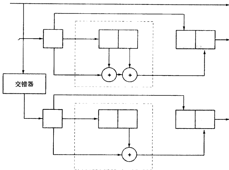
图6-37 习题6.18的Turbo编码器
