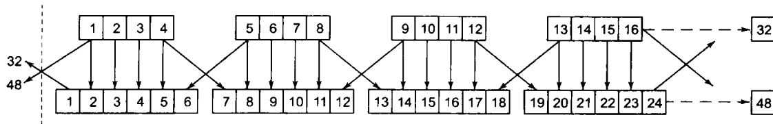
图8-2 扩展置换
