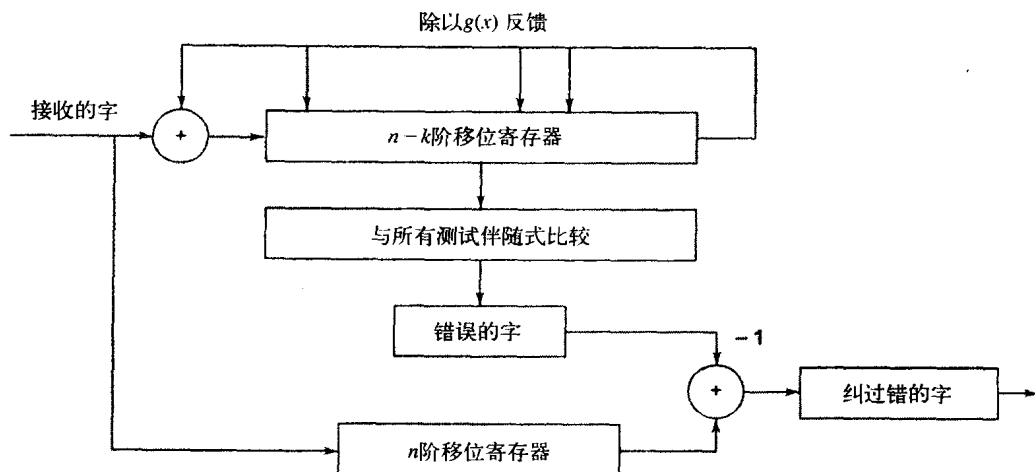
图4-9 Meggit译码器的流程图
