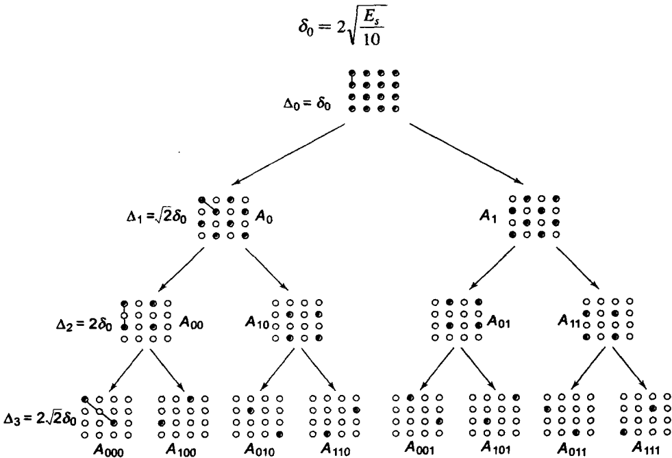
图7-12 16QAM的集合分割
