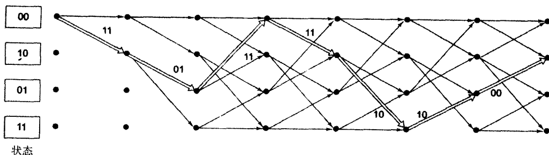
图6-6 用网格图对一个输入序列编码
