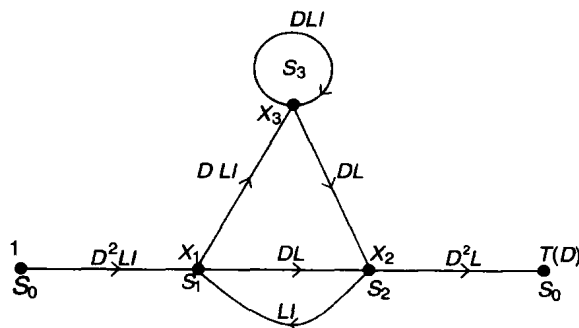
图6-16 用于确定扩张生成函数的修改状态图
