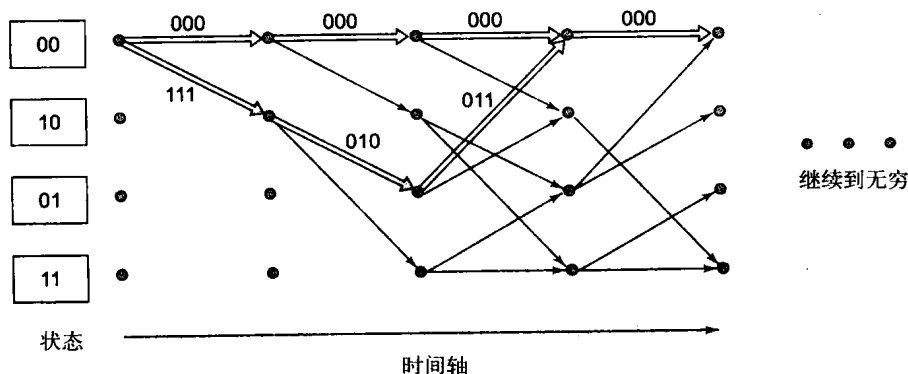
图 6-27 图 6-25 中的卷积编码器的网格图
