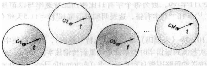
图3-5 GF(q^n) 中球的概念
