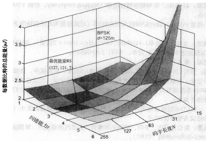
图5-6 总能量与码长及纠错能力的对比
