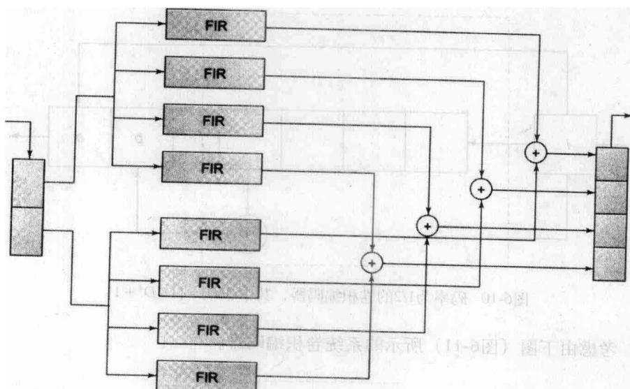
图6-8 k_0=2 和 n_0=4 的FIR过滤器中的卷积编码器。该编码器的码率为 R=1/2
