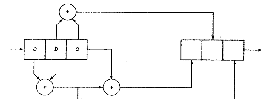
图4-4 GF(8) 上任意域元素 (ax^2 + bx + c) 与元素 (x^2 + x) 的乘法
