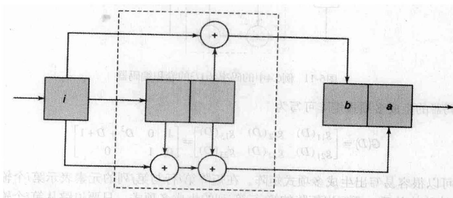
图6-9 码率为1/2的卷积编码器，其中 G(D)=[D^2+D+1 \ D^2+1]
