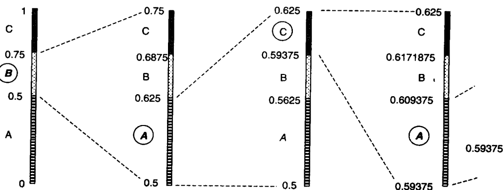
图1-16 对BACA进行算术编码的例子
