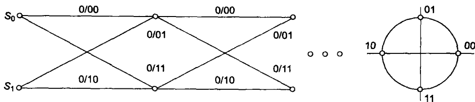
图7-17 两个状态的网格图
