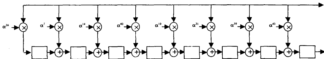
图5-3 RS(63, 55)编码器中移位寄存器部分
