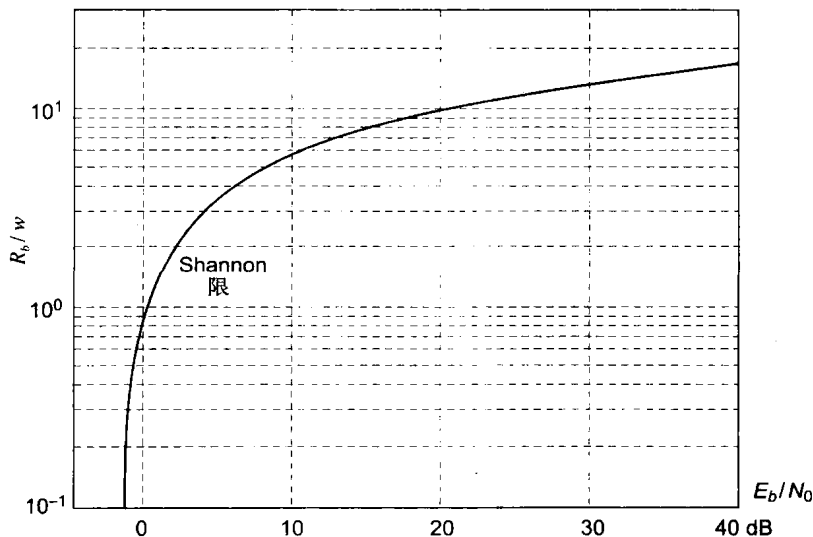
图2-7 带宽效率图
