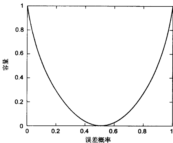
图2-5 BSC的信道容量
