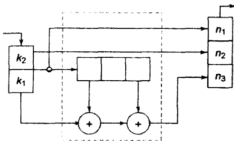
图6-11 例6.4中的码率为1/3的卷积编码器
