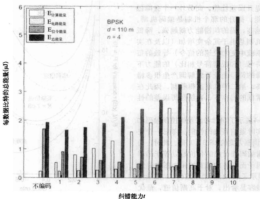
图5-5 RS(31, k )的总能量和纠错能力的对比
