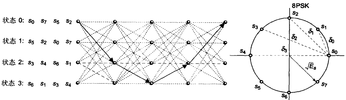
图7-3 对应于输入序列10 11 10 00...的网格中的路径
