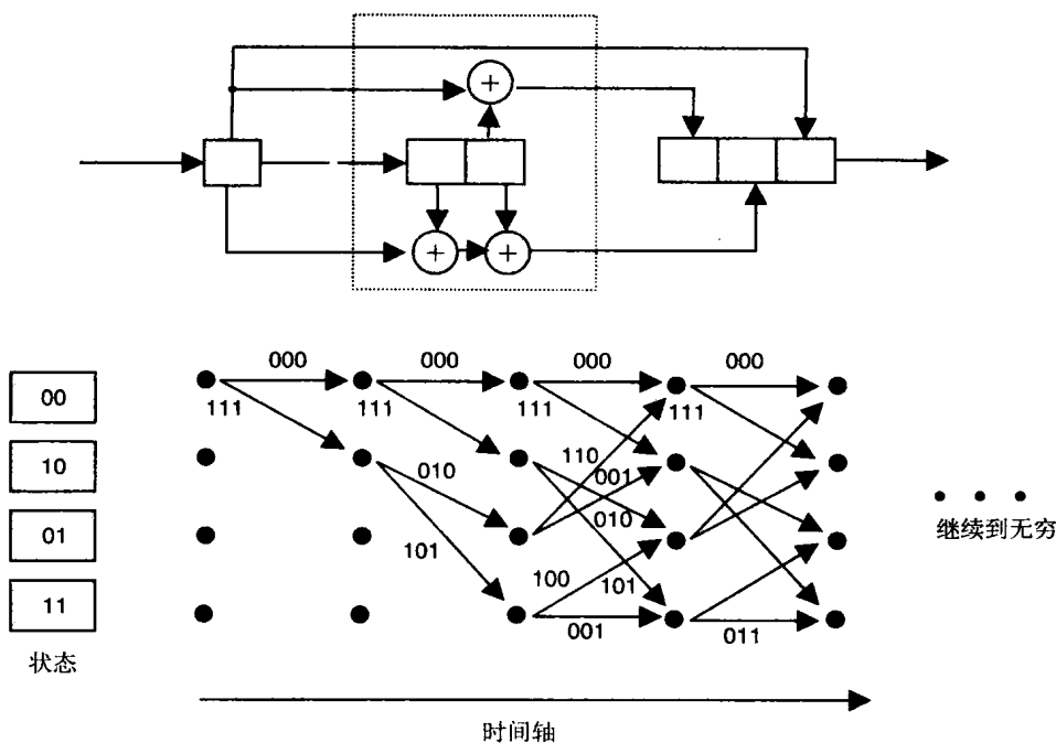
图6-18 码率为1/3的卷积编码器及其网格图
