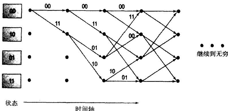
图6-12 例6.1中卷积编码器的网格图
