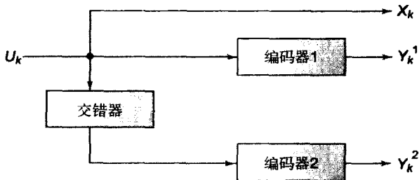
图6-28 码率为1/3的PCCC Turbo码编码器框图
