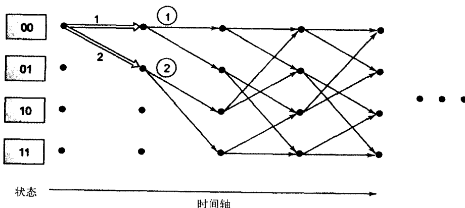
图6-19 维特比译码第一步后的路径尺度
