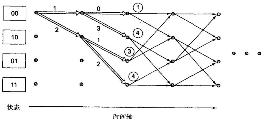
图6-20 维特比译码第二步后的路径尺度
