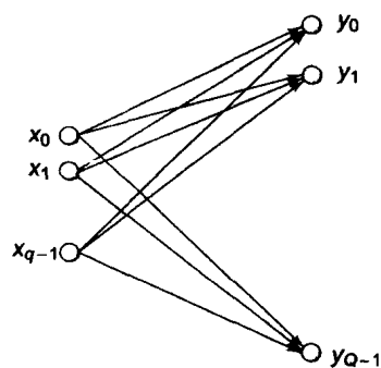
图2-4 一个具有 q -元输入和 Q -元输出的离散无记忆信道 (DMC)
