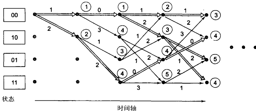
图6-24 在维特比译码过程中不完备译码器的例子
