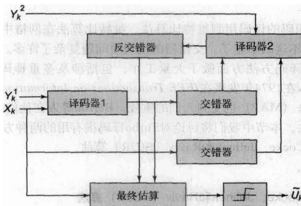
图6-29 Turbo译码器框图
