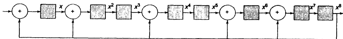
图4-8 对 g(x) = x^8 + x^6 + x^5 + x^3 + x + 1 做除法的移位寄存器电路图
