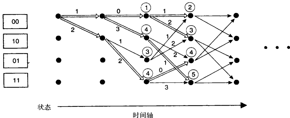
图6-21 维特比译码第三步后的路径尺度
