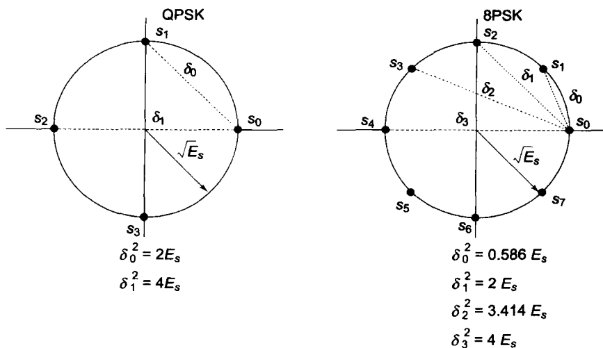
图7-1 QPSK和8PSK的信号点之间的欧几里得距离
