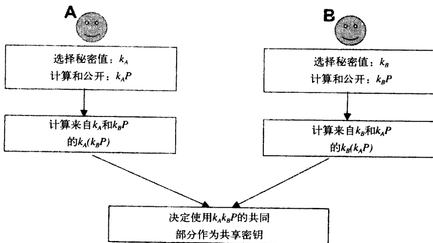
图8-5 使用椭圆曲线的Diffie-Hellman密钥协商协议
