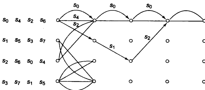
图7-9 例7.6中的编码器的网格图
