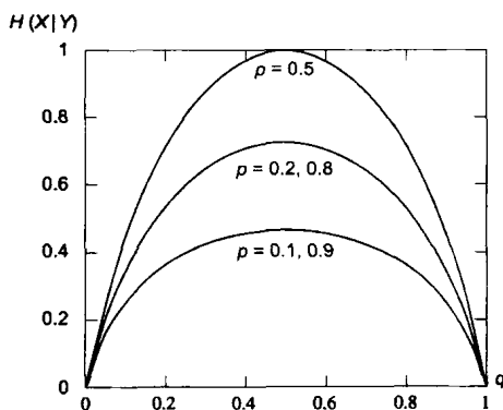
图1-7 条件熵 H(X|Y) 相对 q 的平面图
