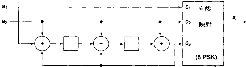
图7-2 例7.2中的TCM方案
