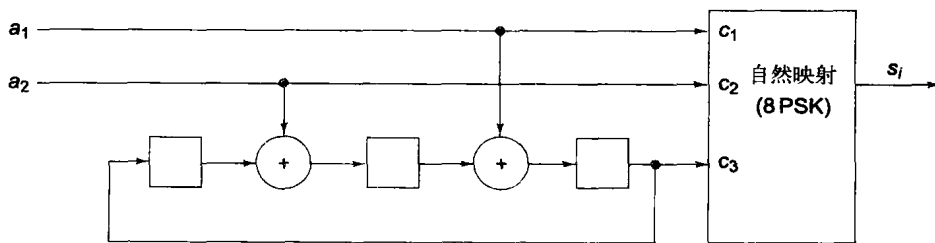
图7-11 例7.7中TCM的编码器
