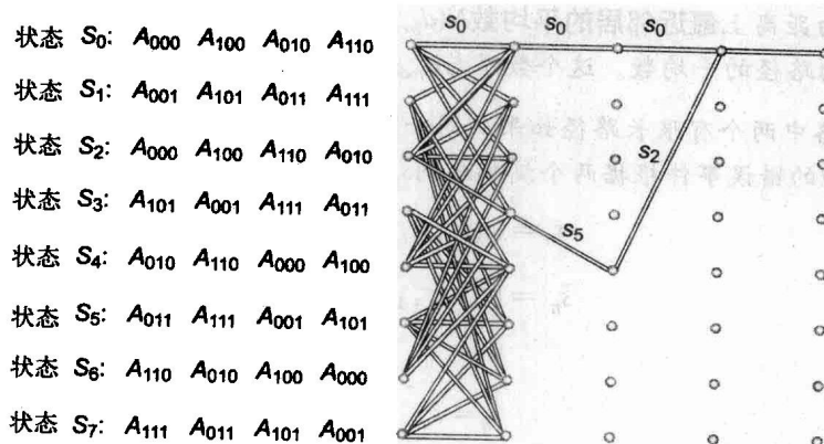
图7-13 16QAM TCM方案的网格图
