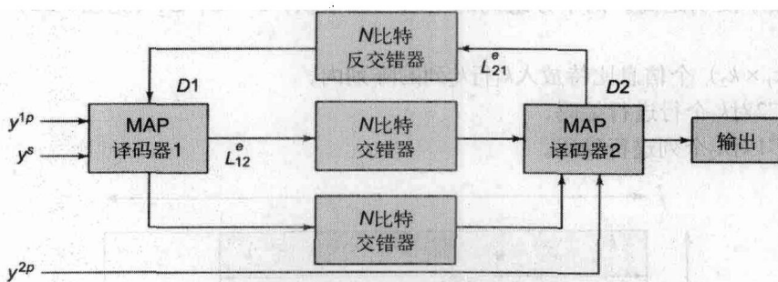
图6-31 Turbo译码器的迭代实现
