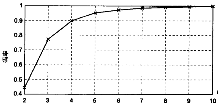
图4-1 不同Fire码的码率
