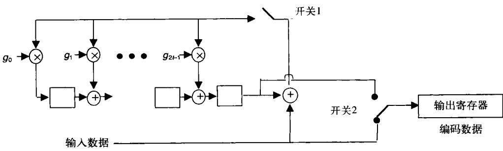
图5-2 生成多项式为 g(x) = g_0 + g_1x + g_2x^2 + \cdots + g_{2t-1}x^{2t-1} + x^{2t} 的RS编码器的硬件实现
