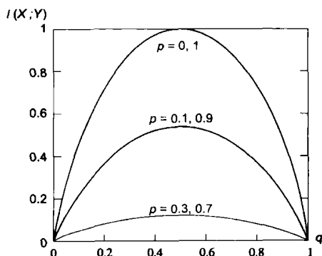
图1-8 平均互信息 I(X; Y) 相对 q 的平面图
