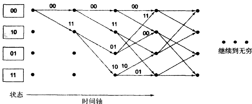
图6-5 图6-3所表示的编码器的网格图
