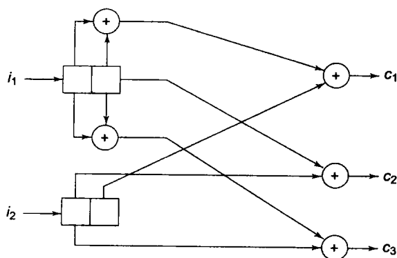
图6-17 码率为2/3的卷积编码器
