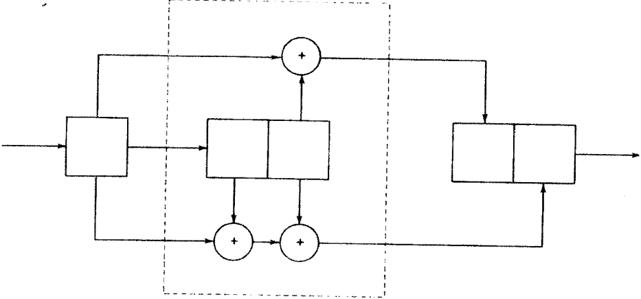
图6-3 例6.1的卷积编码器，此处 k_0 = 1 , n_0 = 2 和 m = 2
