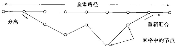
图6-13 自由距离 d_{free} 是指从全零路径偏离和后来又回到全零路径的一条路径的最小距离
