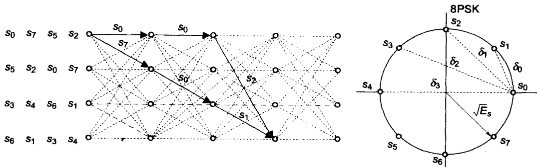
图7-4 网格中两个具有自由欧几里得距离 d_{free}^2 的路径
