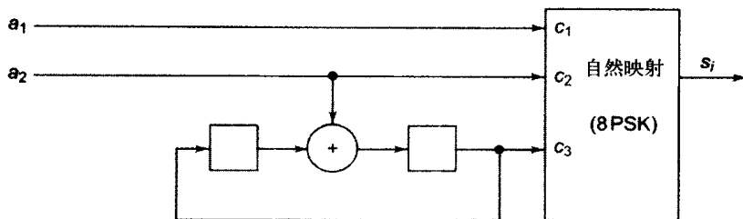
图7-8 例7.6中的TCM编码器
