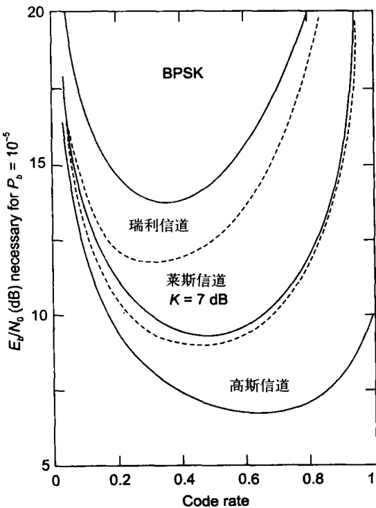
图5-4 使用BPSK的RS(31, k )解码器 相对于码率的性能函数
