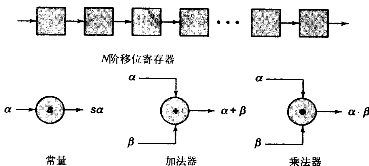
图4-2 用于构造循环码编码器和译码器的电路元素
