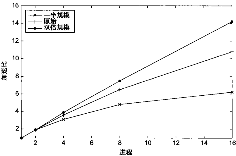
图 2-18 不同问题规模下并程序的加速比
