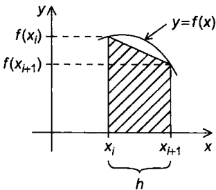
图 3-4 一个梯形
