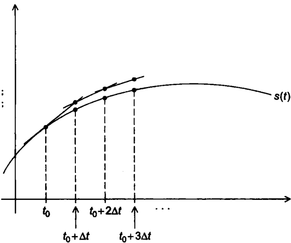
图 6-2 欧拉方法
