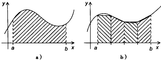
图 5-3 梯形积分法：a) 需要估计的区域；b) 使用梯形计算的近似面积
