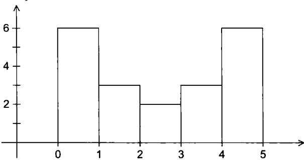
图 2-20 一个直方图
