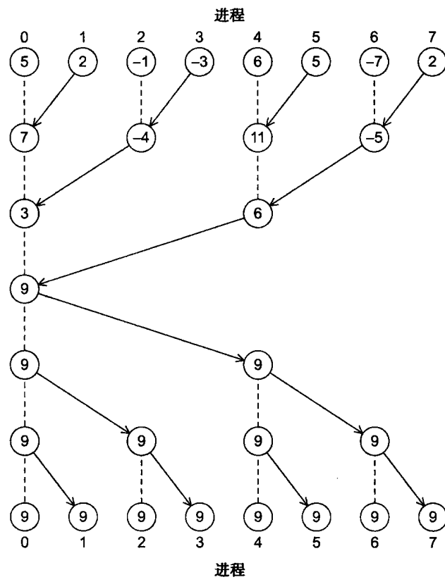
图 3-8 全局求和计算结果的发布
