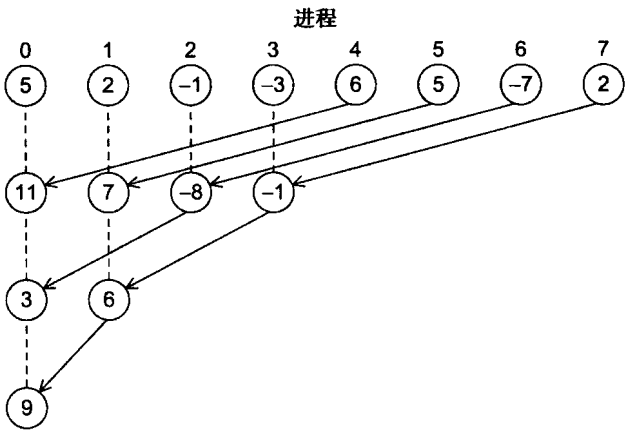
图 3-7 树形结构全局求和的另一种方法
