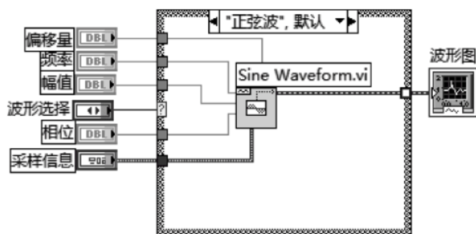
图 7.58 正弦波分支接线
