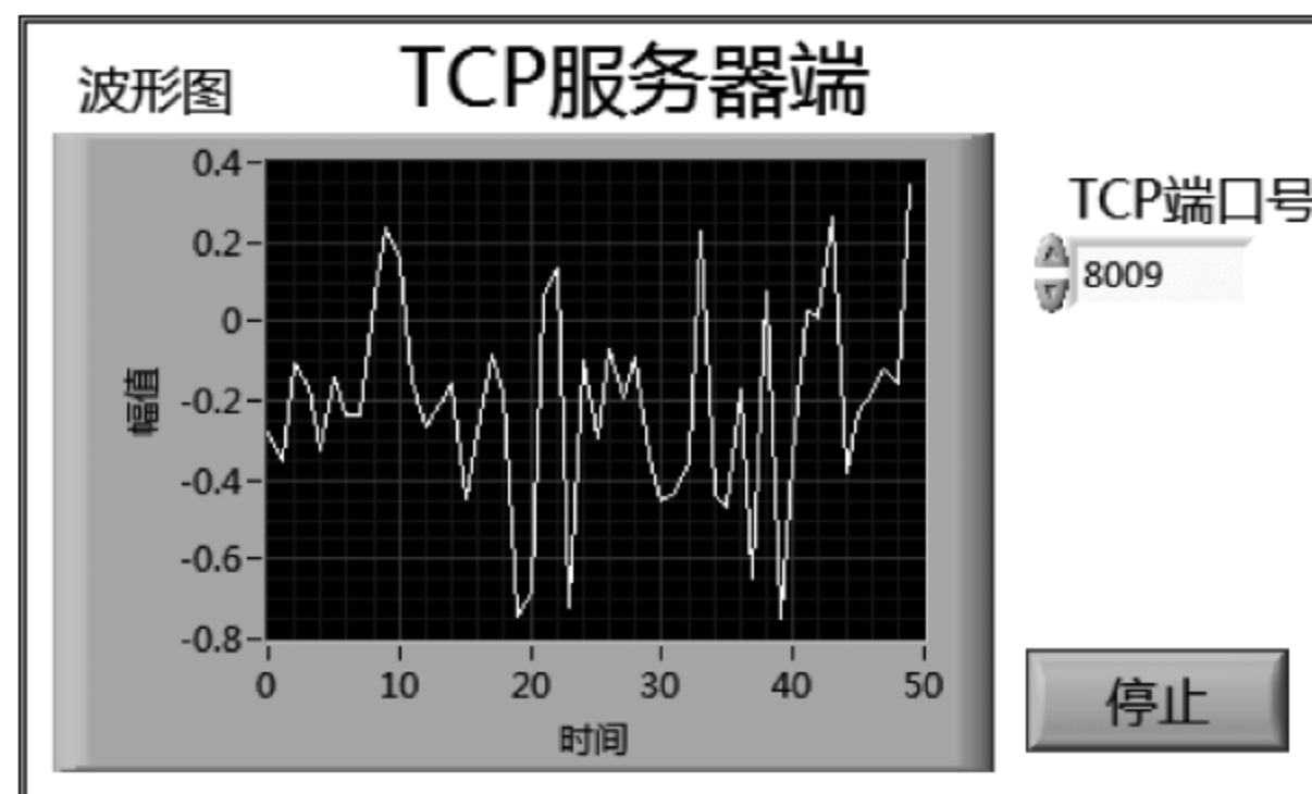
图 6.35 TCP 通信服务器程序前面板
