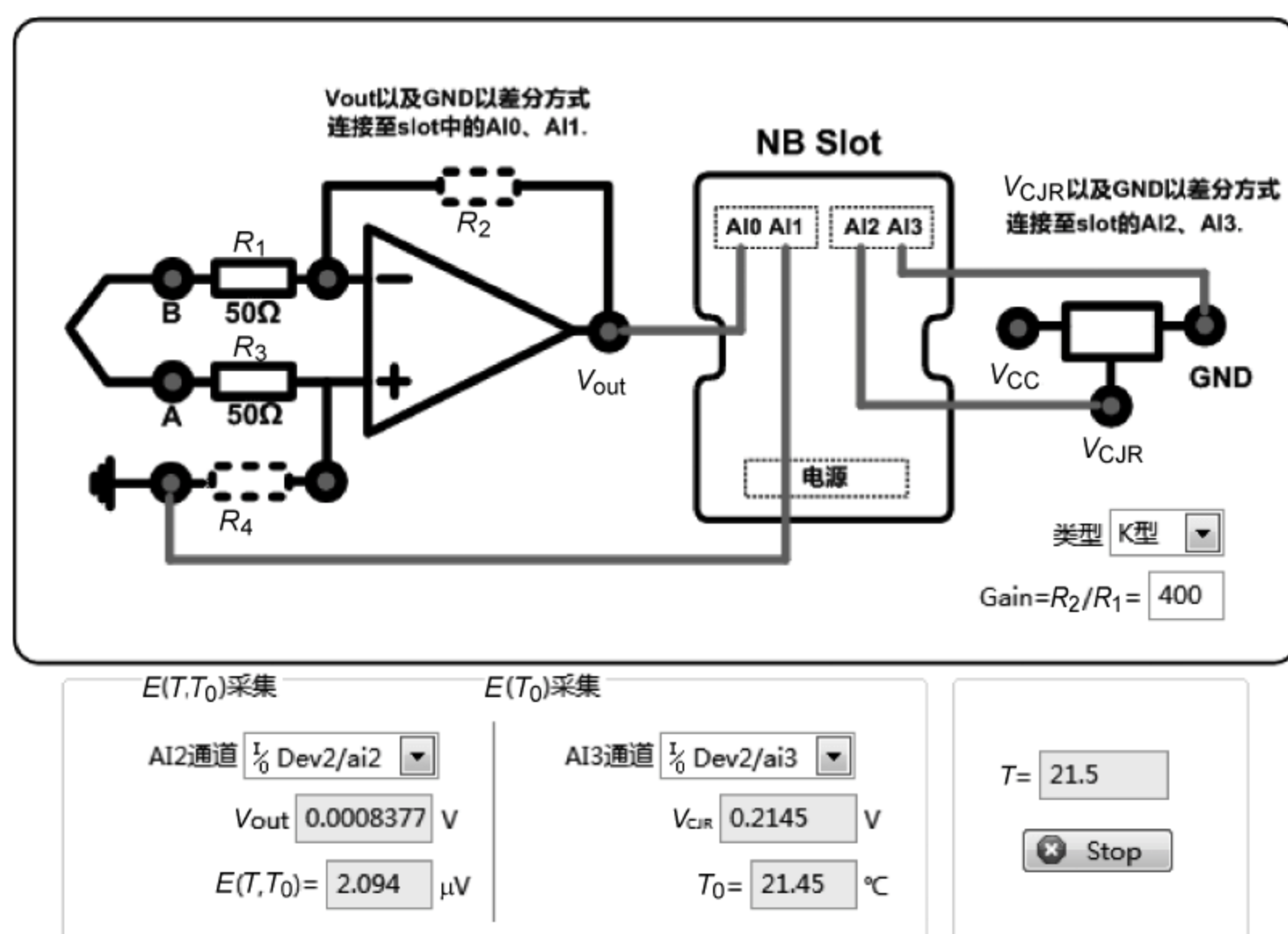
图 11.21 LabVIEW 温度调零数据显示
