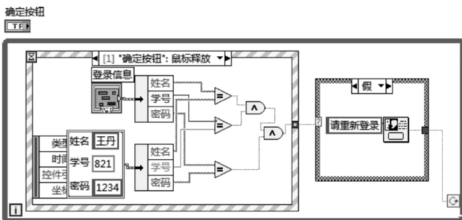
图 7.63 登录界面程序框图
