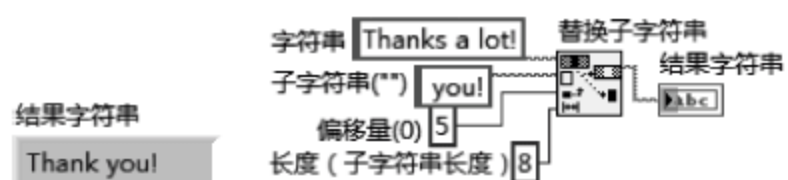
图 3.28 例 3.5 前面板和程序框图
