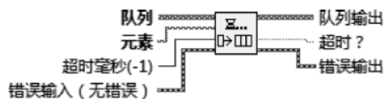
图 6.4 元素入队列函数
