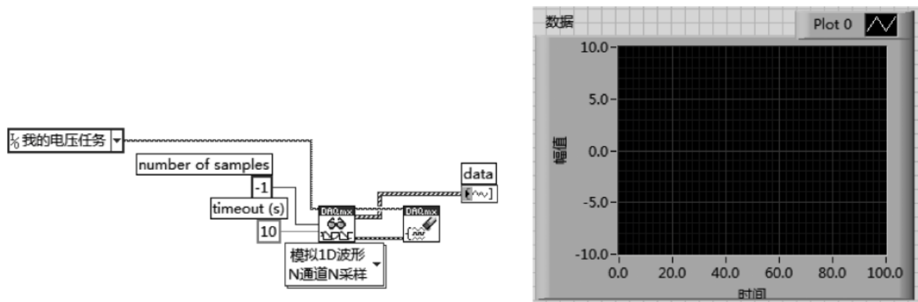
图 10.18 任务生成代码的前后面板
