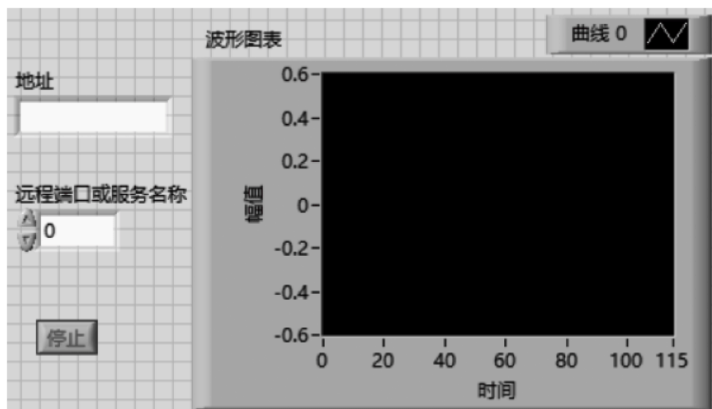
图 12.22 TCP/IP 采集系统接收端前面板设计
