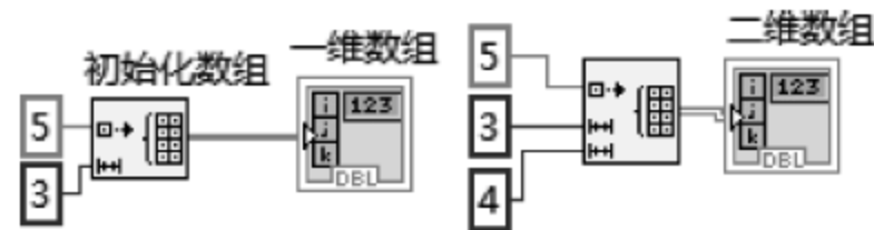
图 3.42 “初始化数组”举例的程序框图
