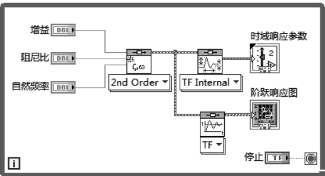
图 9.20 例 9.4 的程序框图
