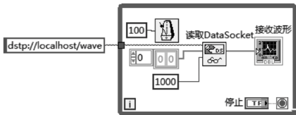
图 6.24 例 6.3 客户机的程序框图
