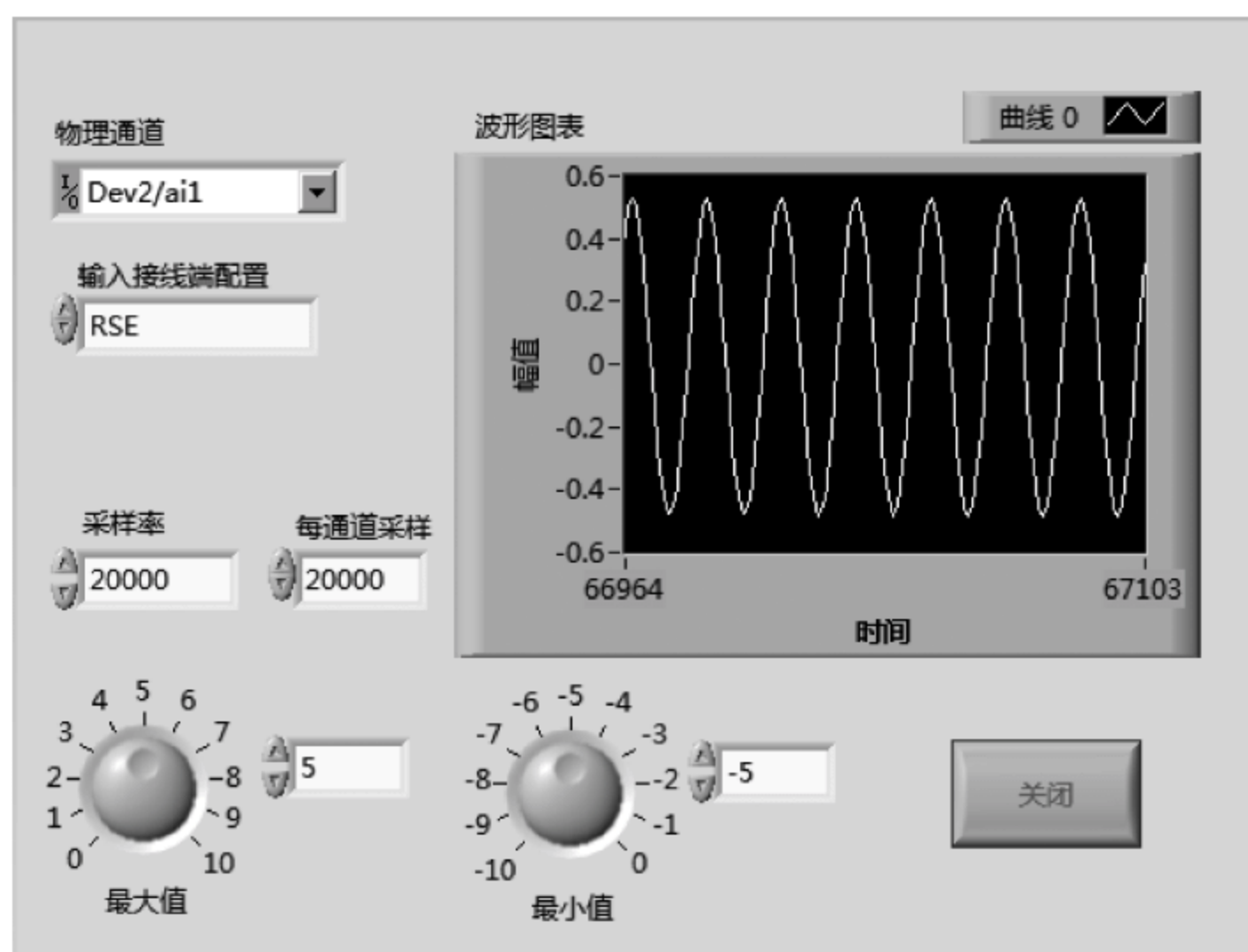
图 12.16 单机数据采集系统 LabVIEW 前面板程序调试界面
