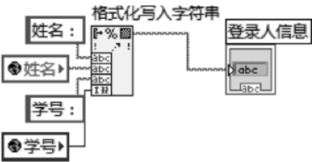
图 7.66 信号发生器中“姓名”及“学号”编程
