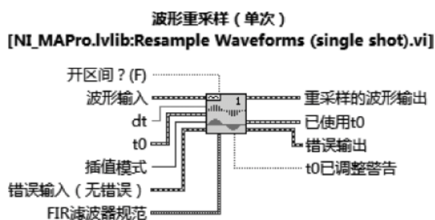
图 8.8 波形重采样(单次)端口定义和接口
