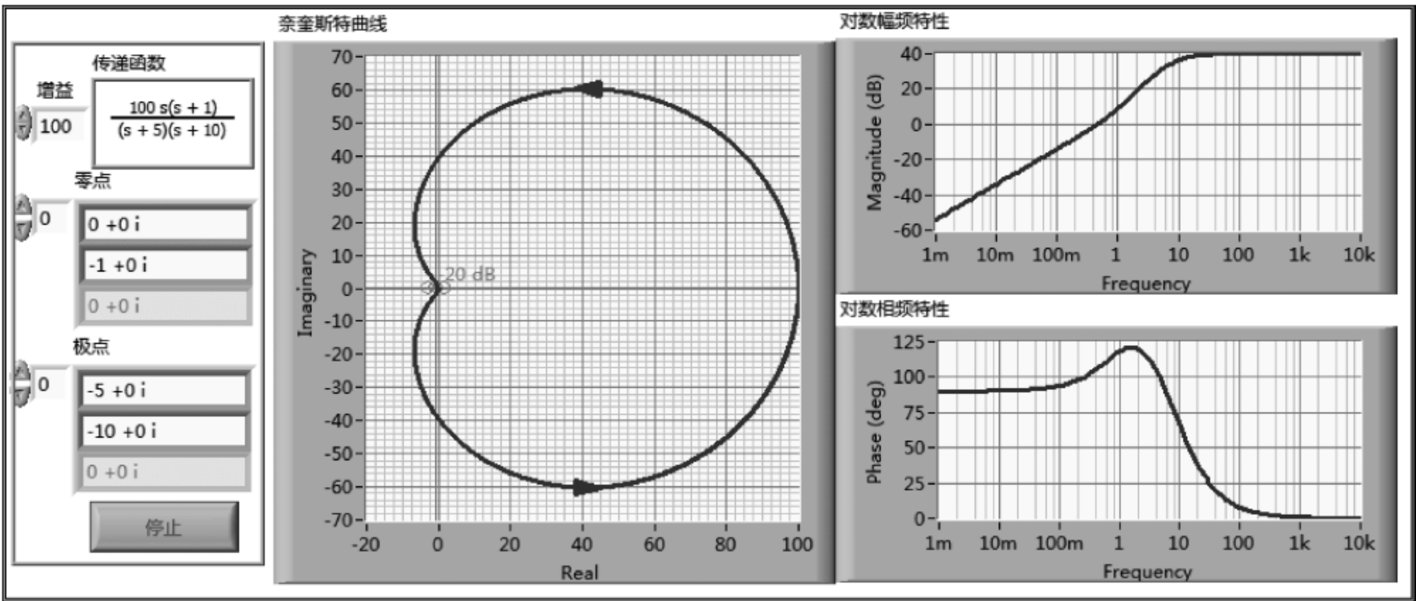
图 9.26 例 9.5 前面板
