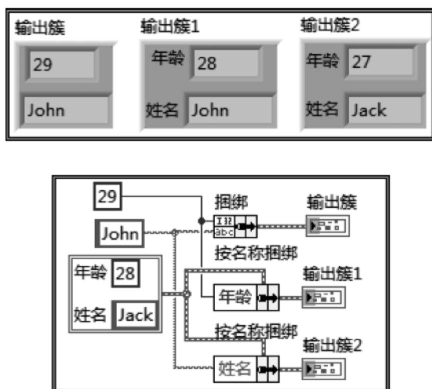
图 3.61 例 3.6 的前面板和程序框图
