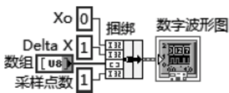
图 5.20 例 5.7 的程序框图
