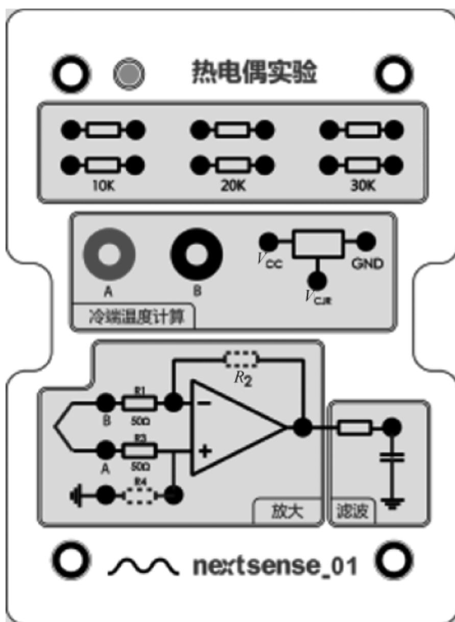
图 11.14 热电偶实验模块
