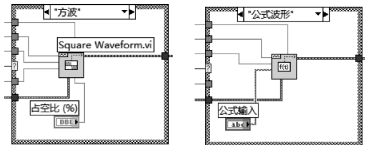
图 7.59 方波和公式波形的特殊接线端
