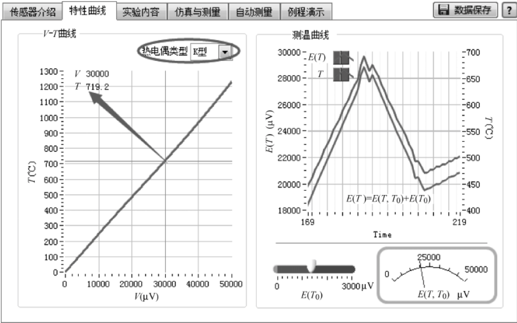
图 11.8 特性曲线
