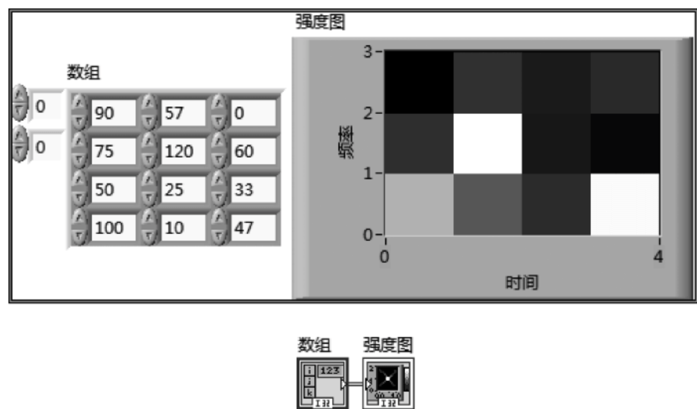
图 5.19 例 5.6 的前面板和程序框图
