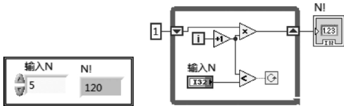
图 4.14 例 4.3 前面板和程序框图
