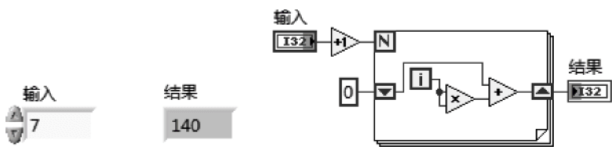
图 4.6 例 4.2 的前面板和程序框图
