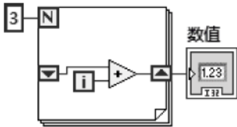
图 4.7 for 循环寄存器无输入情况
