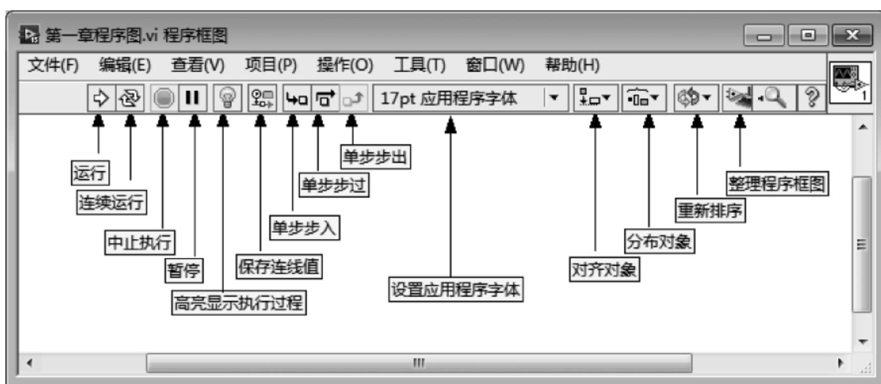
图 1.18 程序框图的工具栏
