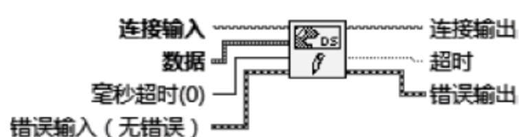
图 6.15 写入 DataSocket 函数
