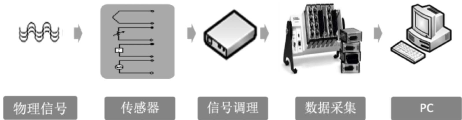
图 10.1 基于 PC 的数据采集系统
