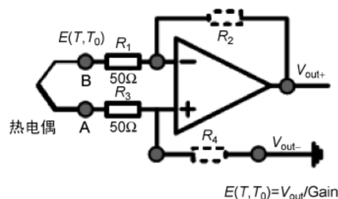
图 11.15 热电偶实验模块调理电路
