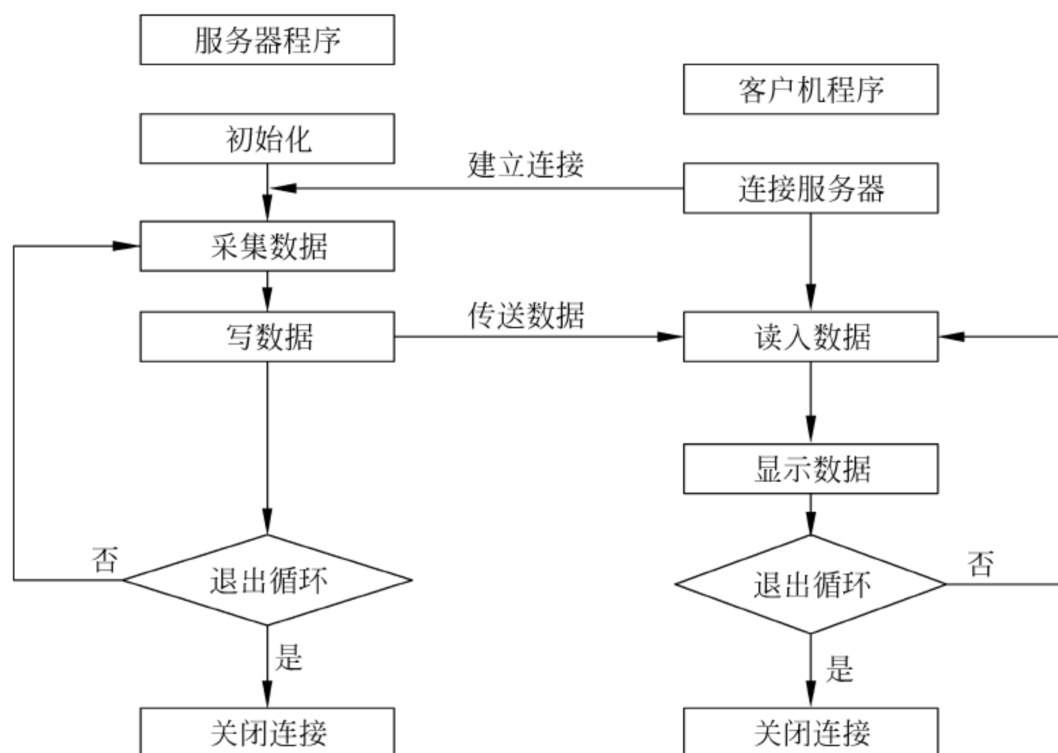
图 6.34 双机 TCP 通信流程
