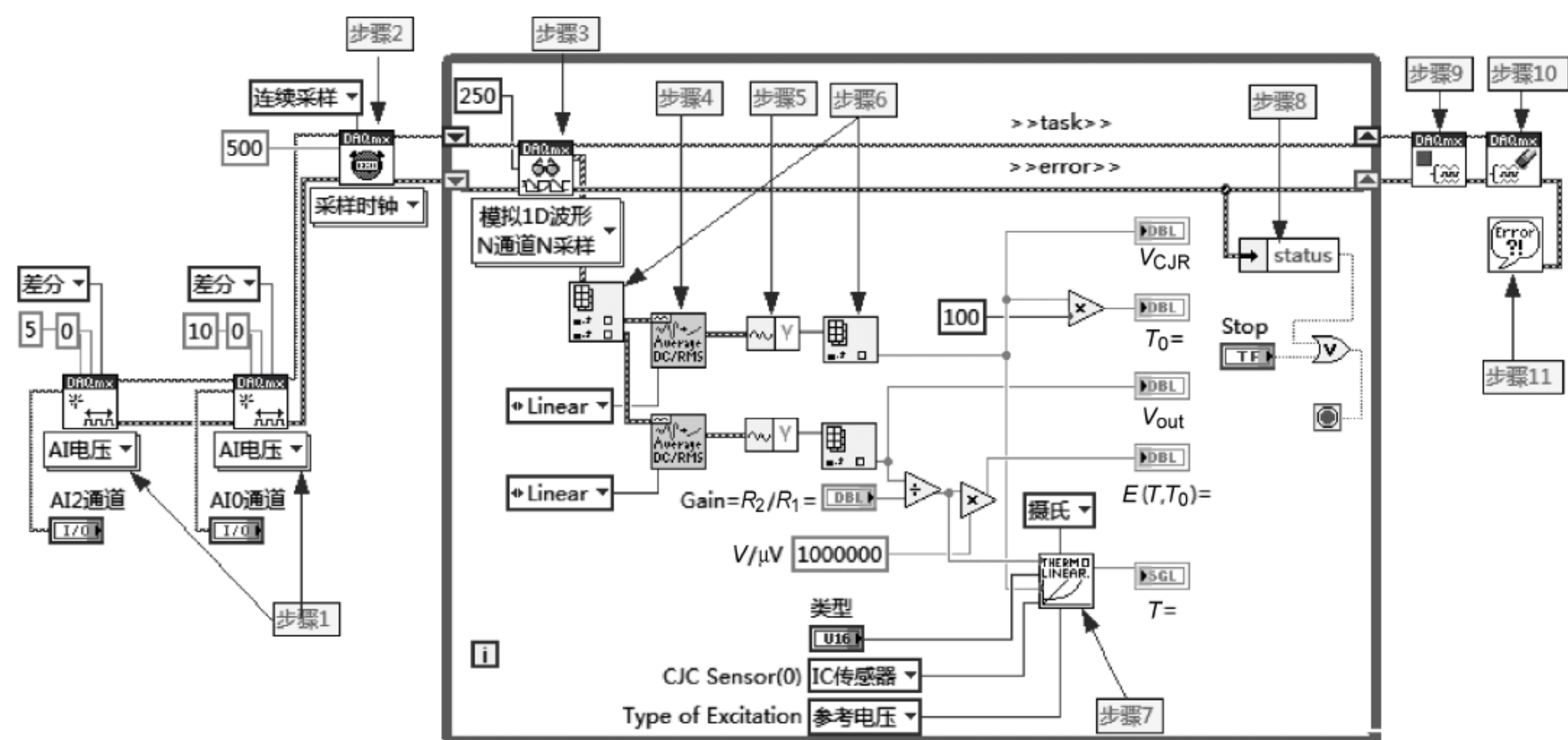
图 11.19 程序框图
