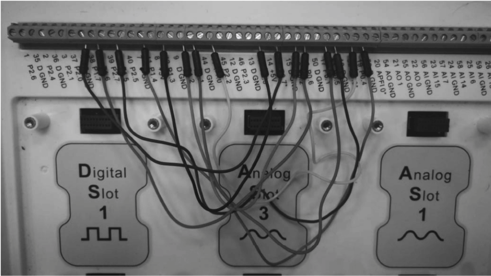
图 11.26 Nextboard 数据采集实物图
