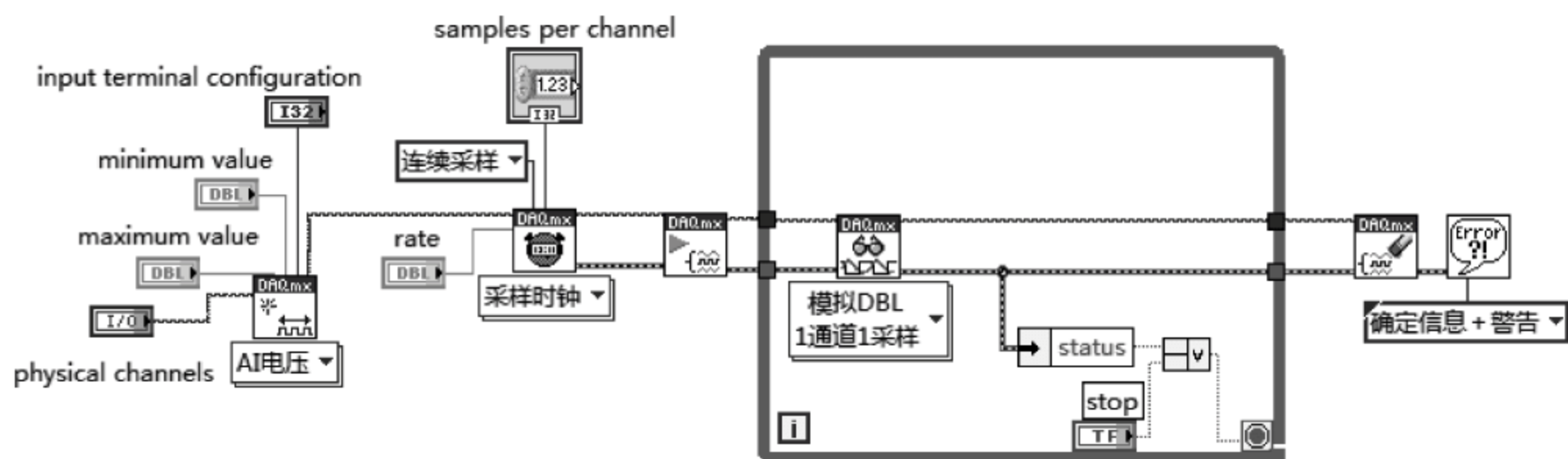
图 12.14 单机数据采集程序设计
