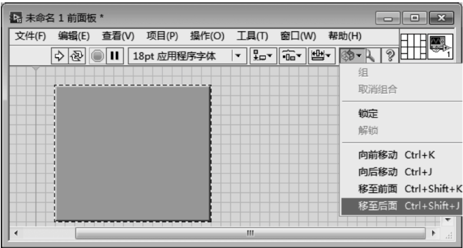
图 2.3 调整控件显示层次
