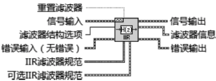
图 7.17 数字 IIR 滤波器函数
