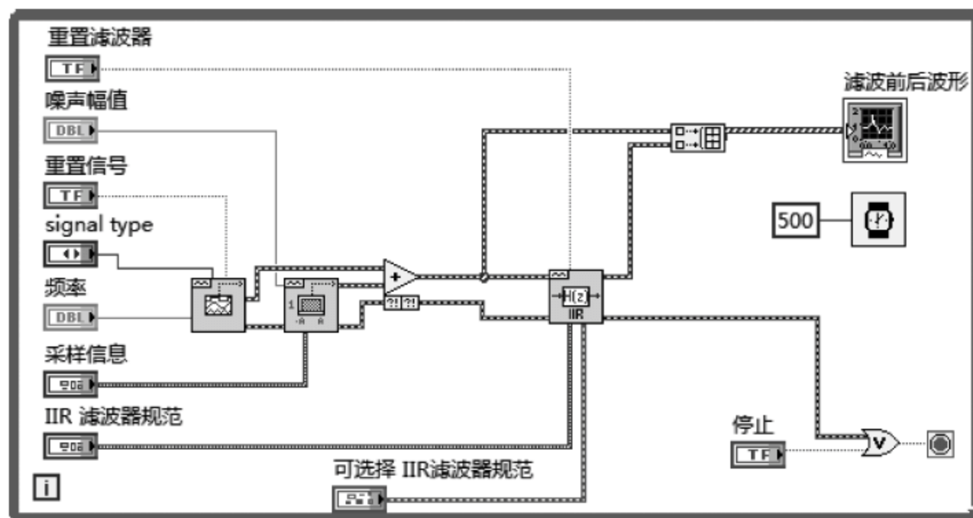
图 7.19 例 7.5 的程序框图
