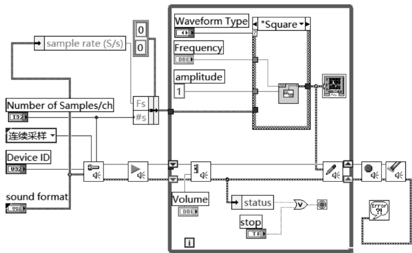
图 13.12 声音播放模块程序框图
