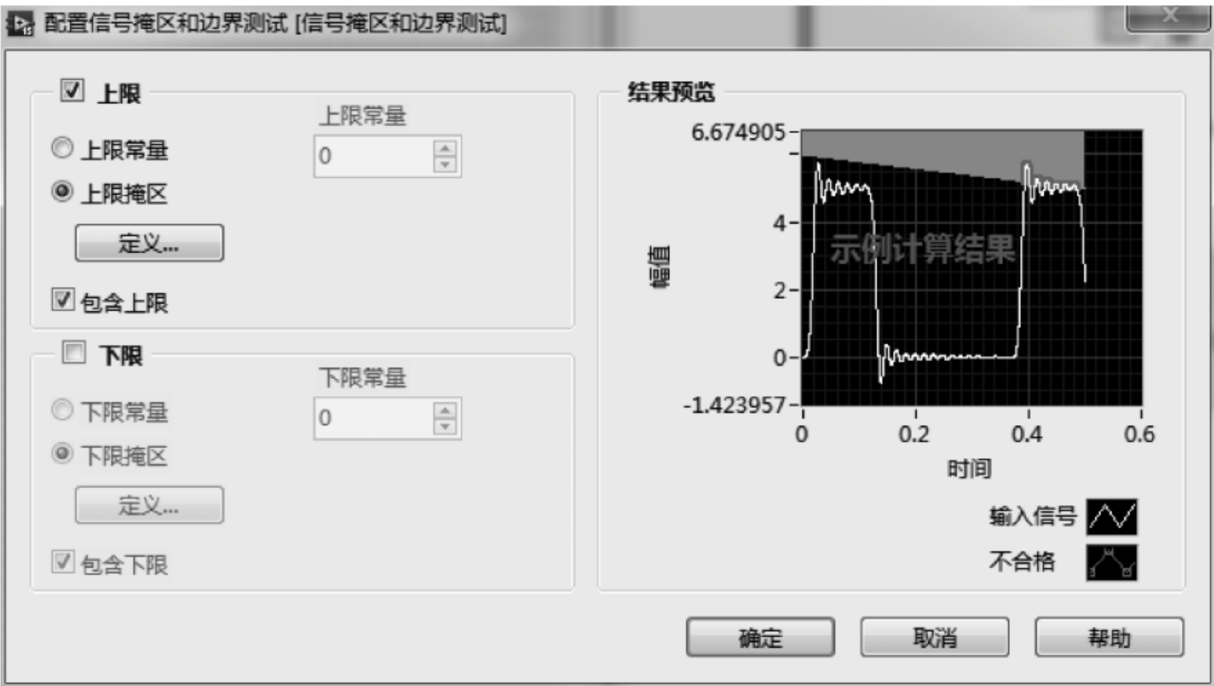
图 7.35 配置信号掩区和边界测试
