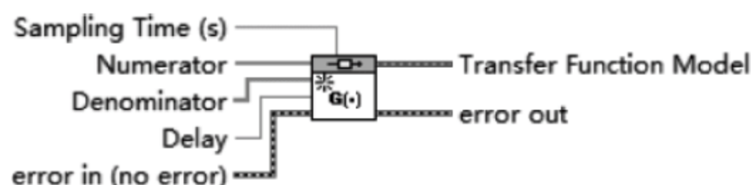
图 9.3 CD Construct Transfer Function Model. vi 函数
