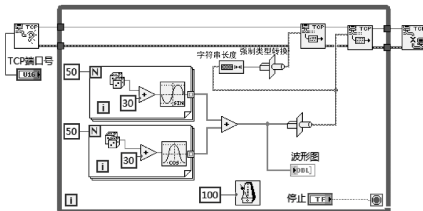
图 6.36 TCP 通信服务器程序框图
