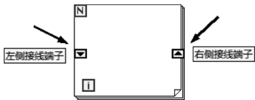
图 4.5 for 循环中添加移位寄存器
