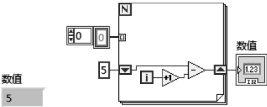
图 4.8 数组为空情况
