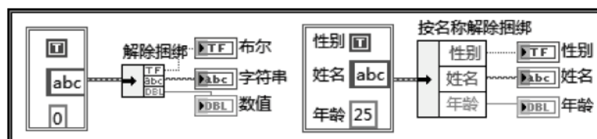
图 3.64 例 3.7 程序框图
