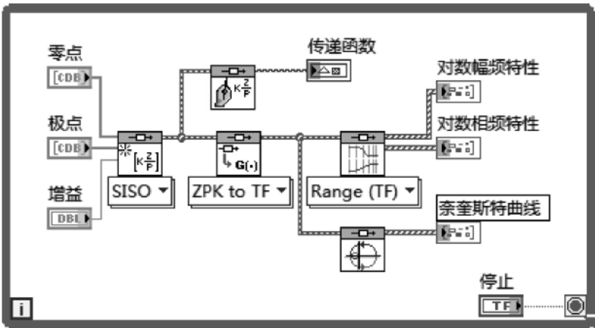
图 9.25 例 9.5 程序框图
