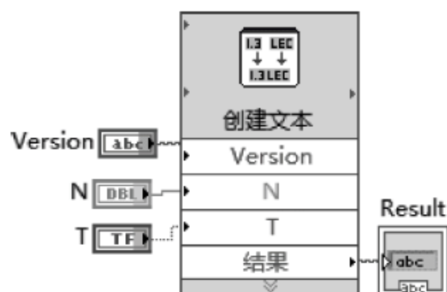
图 7.53 例 7.12 程序框图
