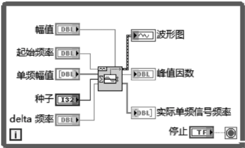
图 7.8 例 7.2 程序框图
