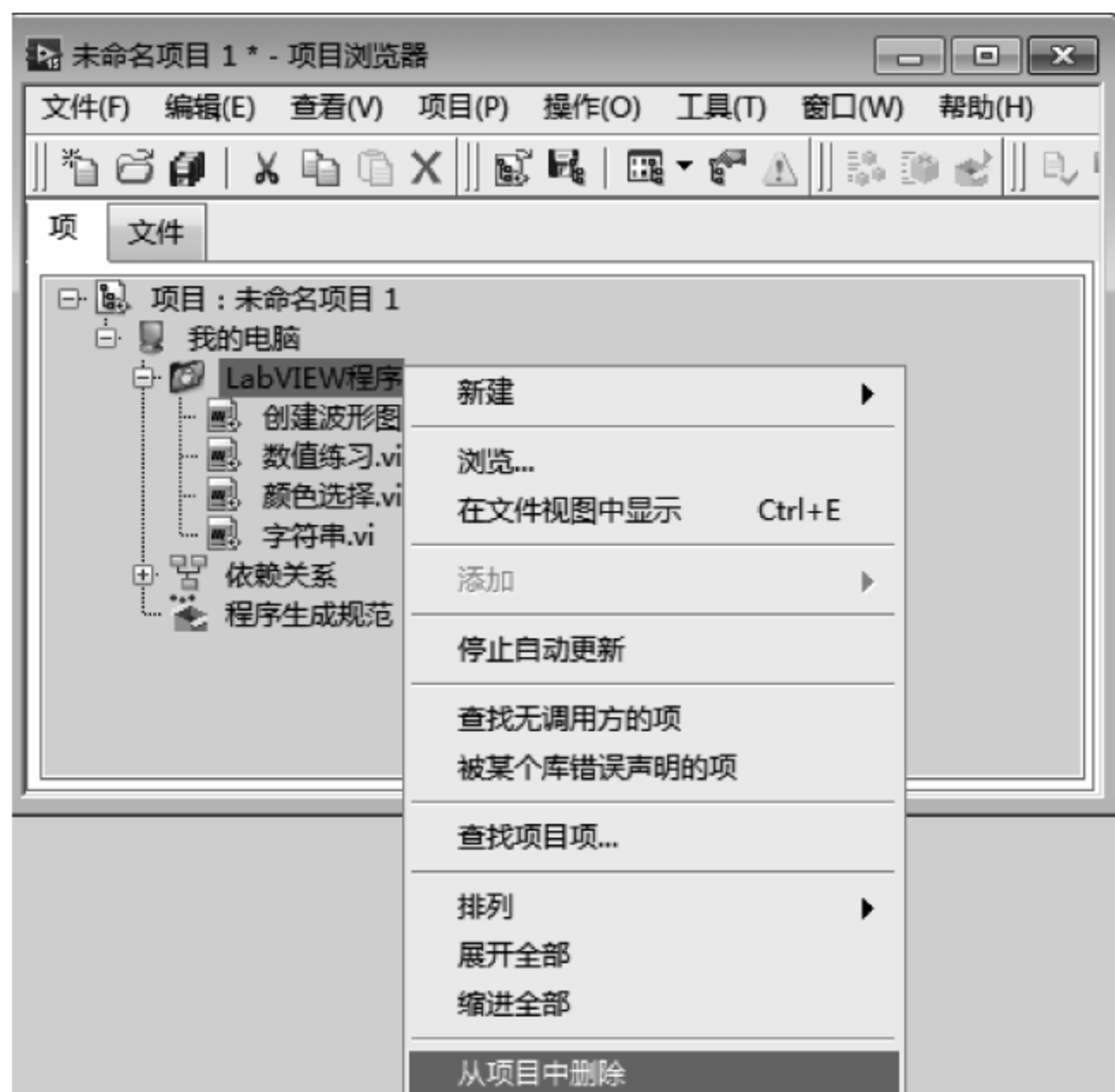
图 1.22 删除操作
