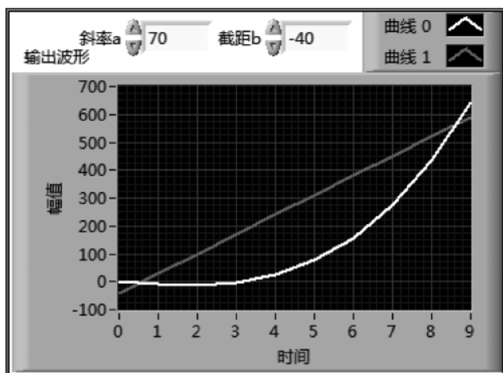
图 4.31 例 4.11 的前面板
