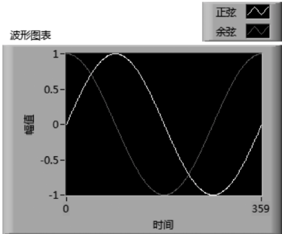
图 5.10 例 5.2 前面板图
