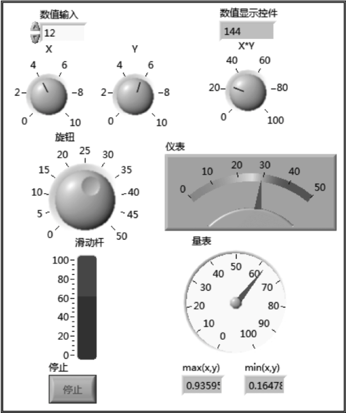
图 3.7 例 3.1 的前面板
