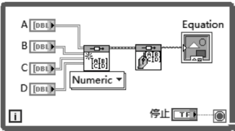
图 9.12 例 9.2 程序框图
