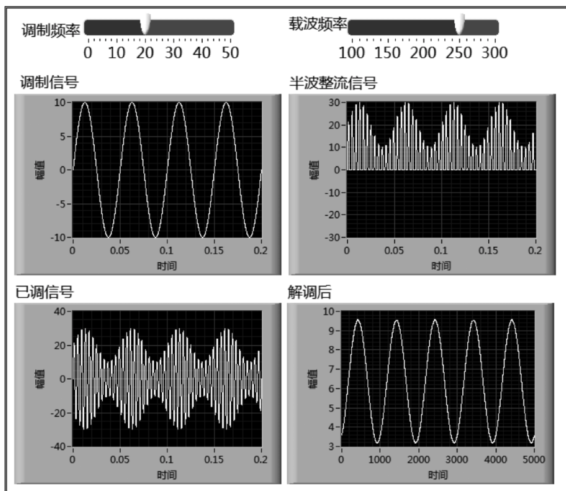
图 8.5 例 8.2 前面板
