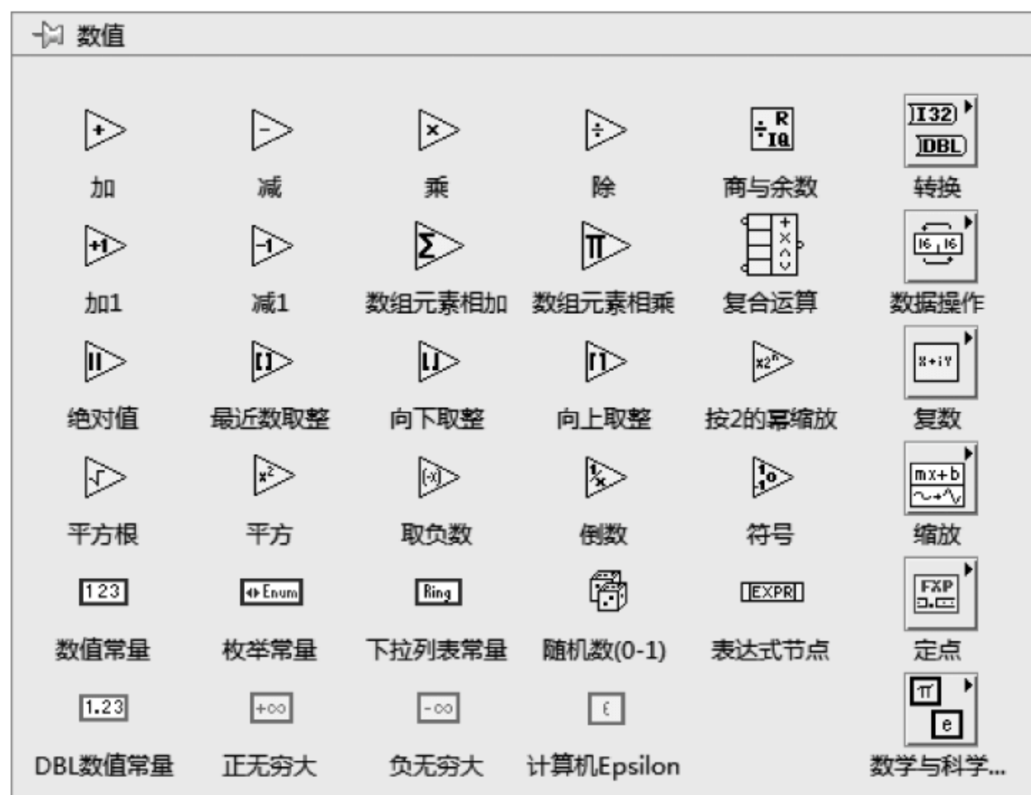
图 3.5 “数值”选板
