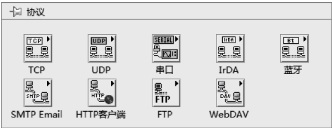
图 6.25 协议子选板
