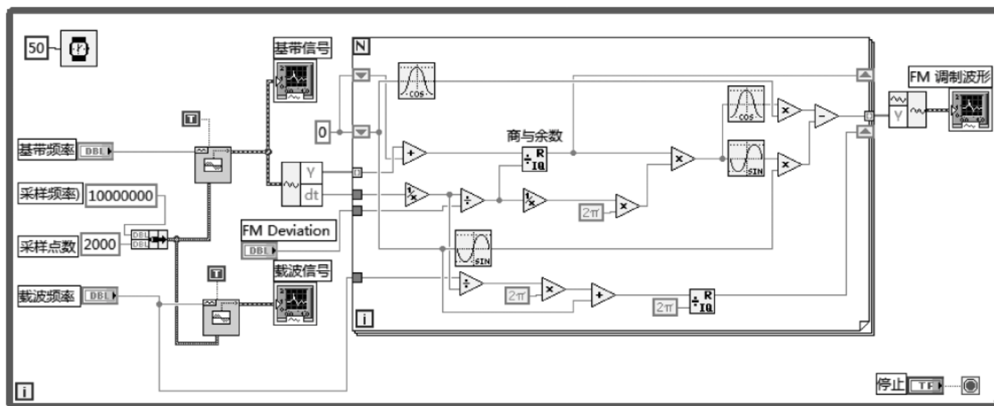
图 8.6 例 8.3 程序框图
