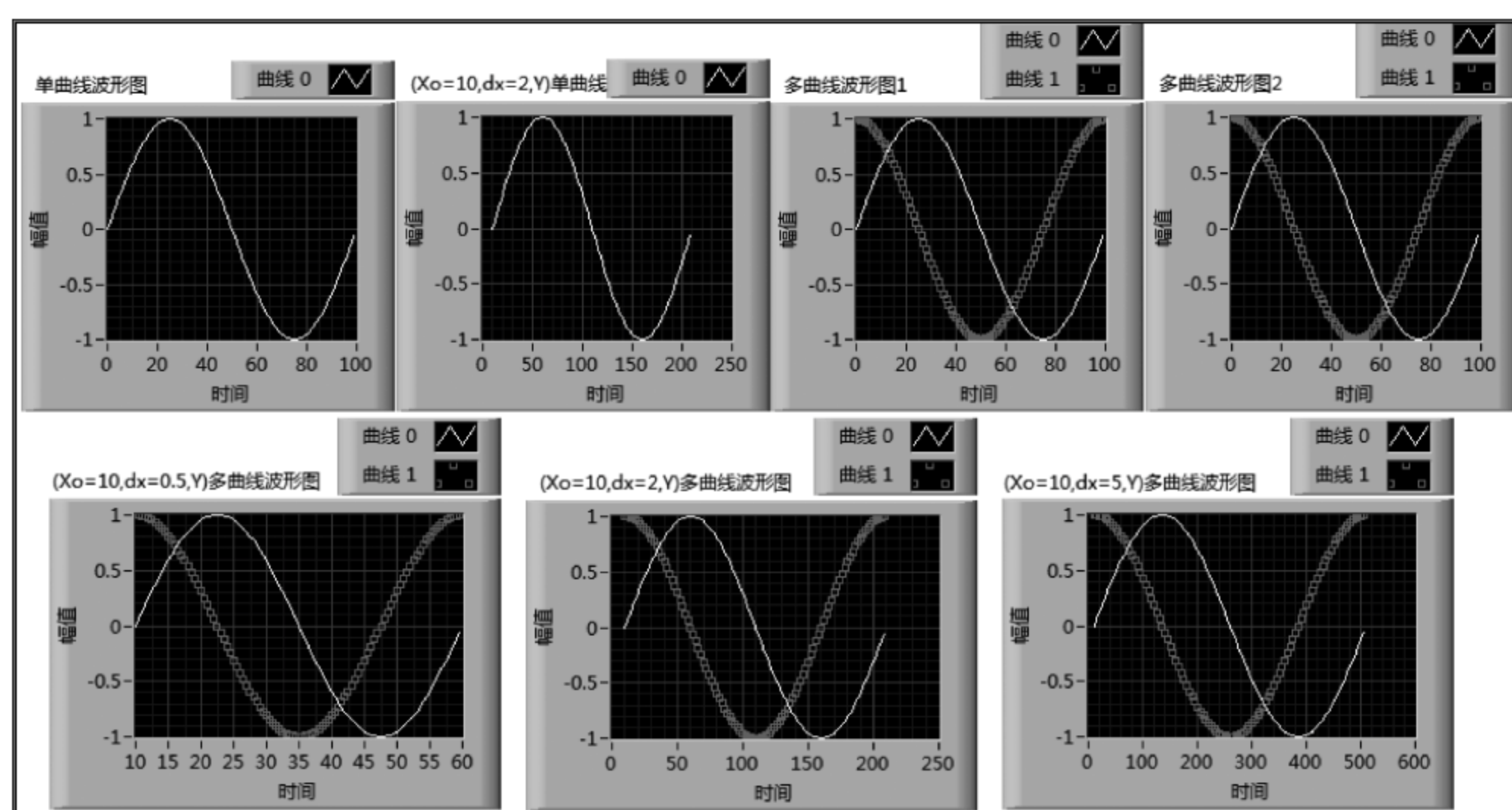
图 5.16 例 5.4 前面板
