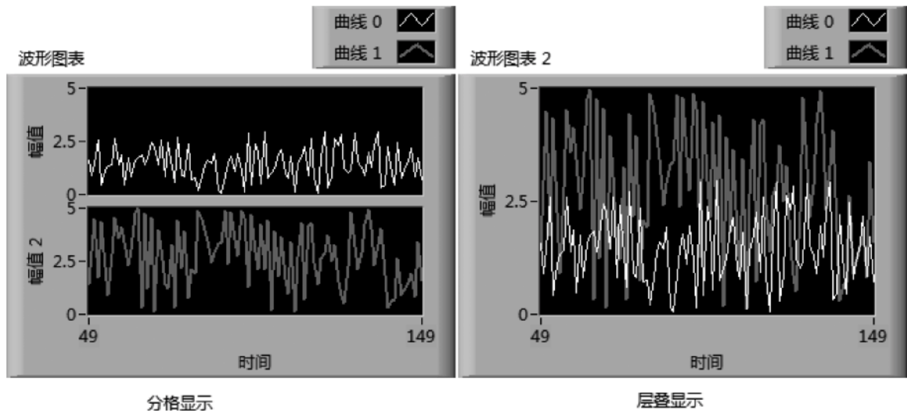
图 5.8 例 5.1 前面板
