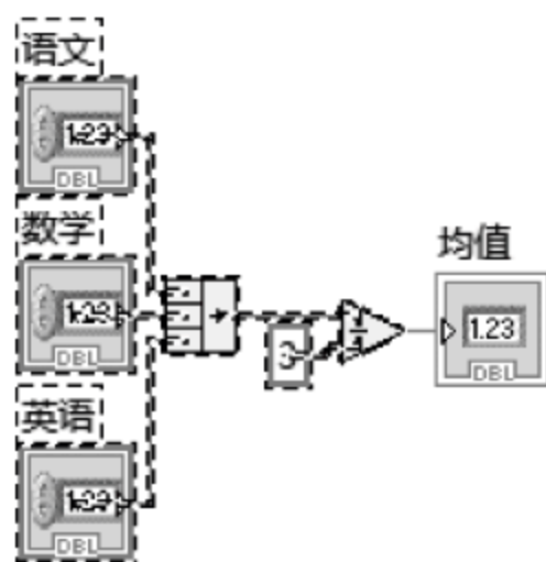
图 2.16 选择子 VI
