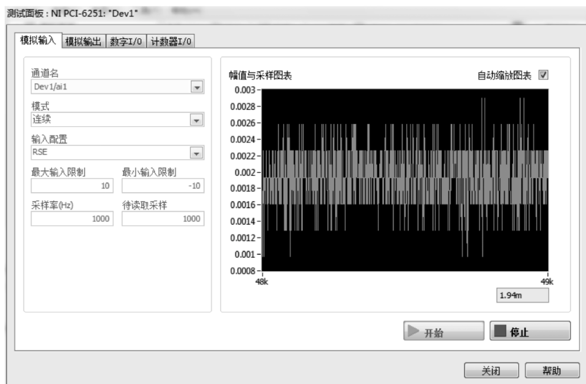
图 10.15 测试面板
