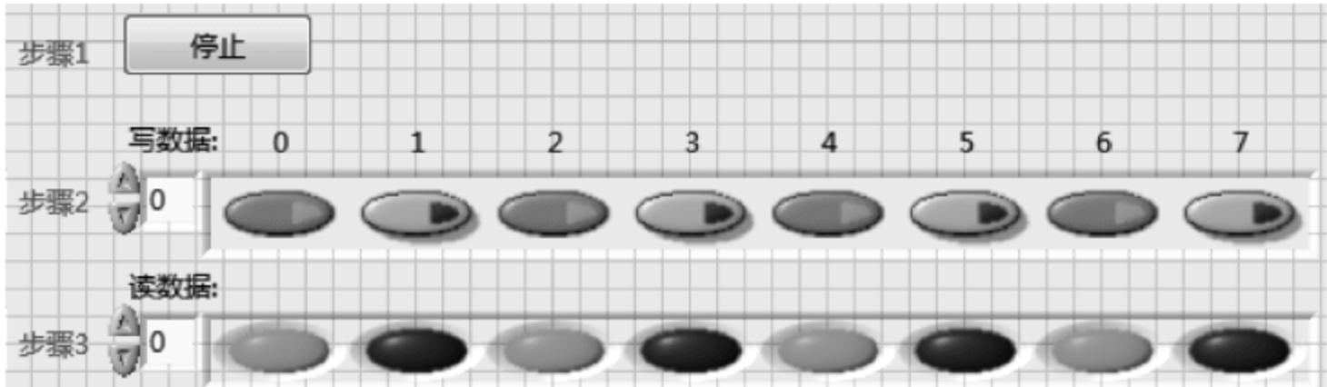
图 11.24 前面板设计
