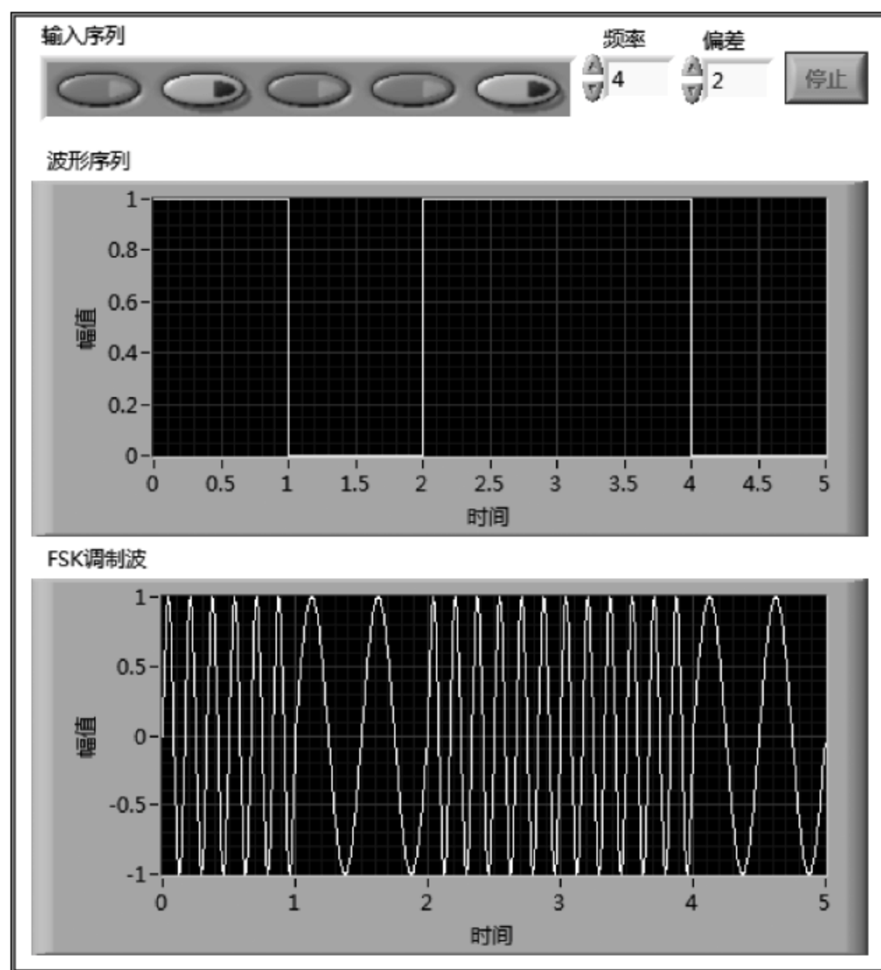
图 8.12 例 8.5 前面板
