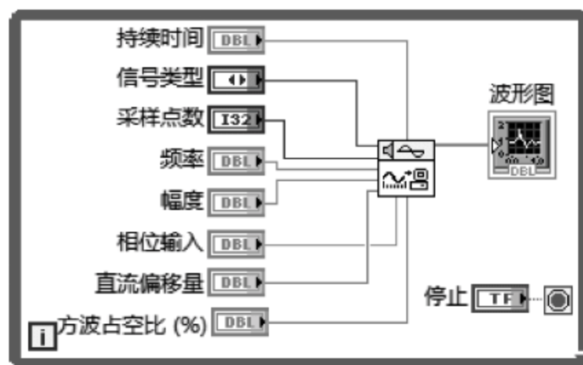
图 7.13 例 7.3 程序框图
