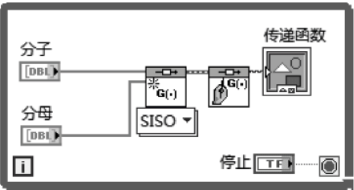
图 9.7 例 9.1 程序框图
