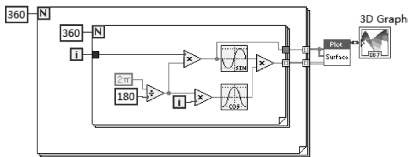
图 5.28 例 5.8 程序框图
