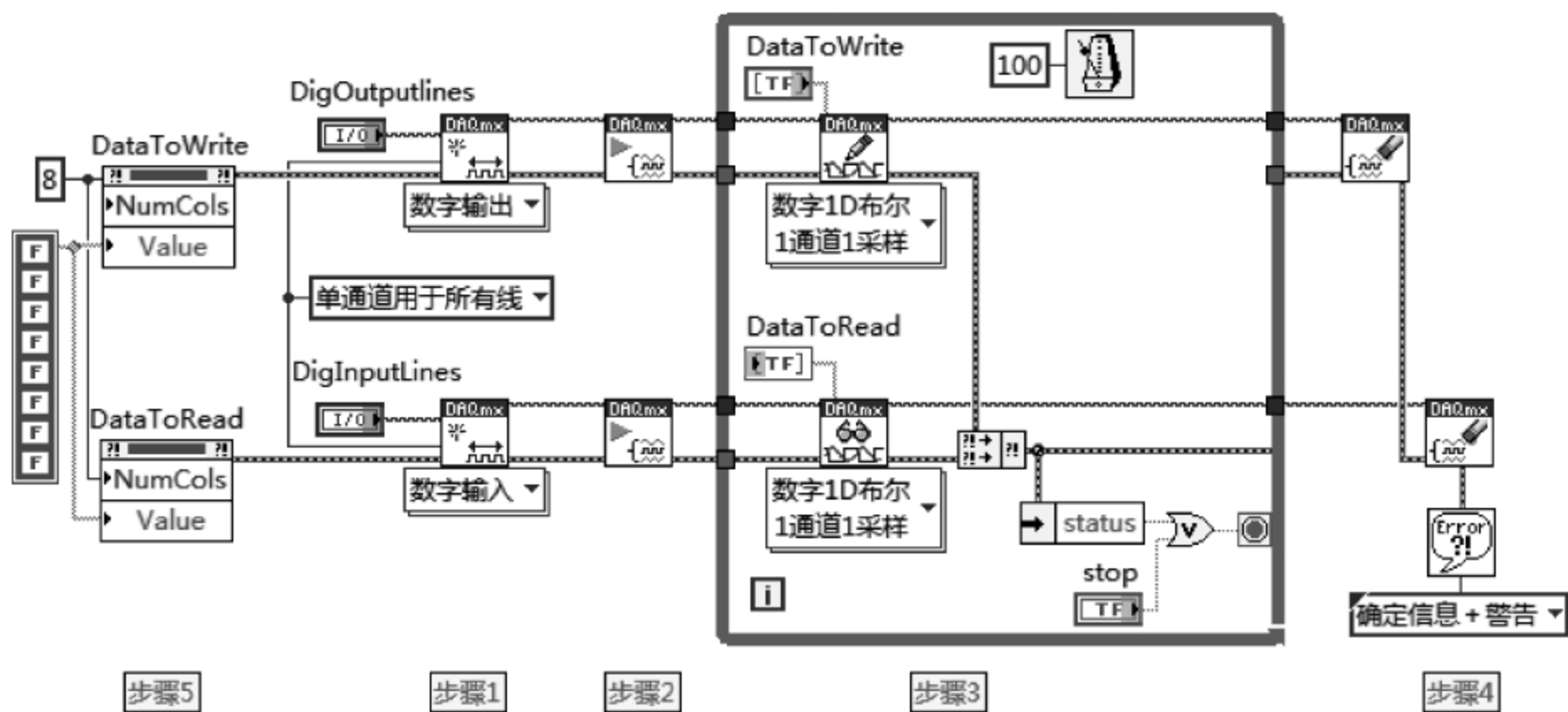
图 11.25 程序框图
