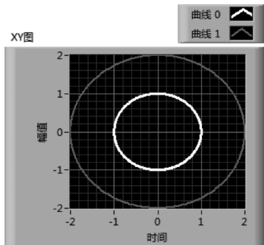
图 5.17 例 5.5 的前面板
