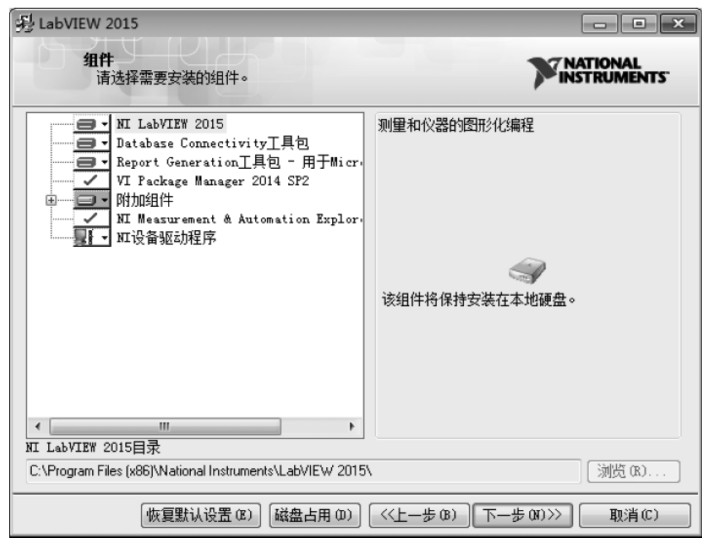
图 1.5 组件目录
