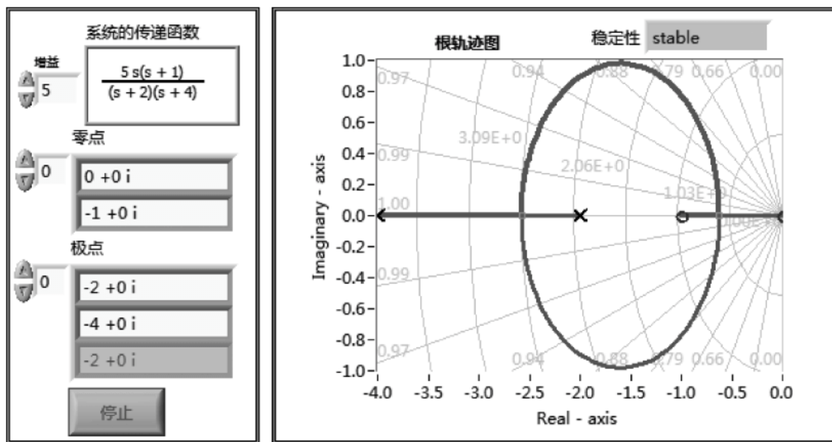
图 9.31 例 9.6 的前面板
