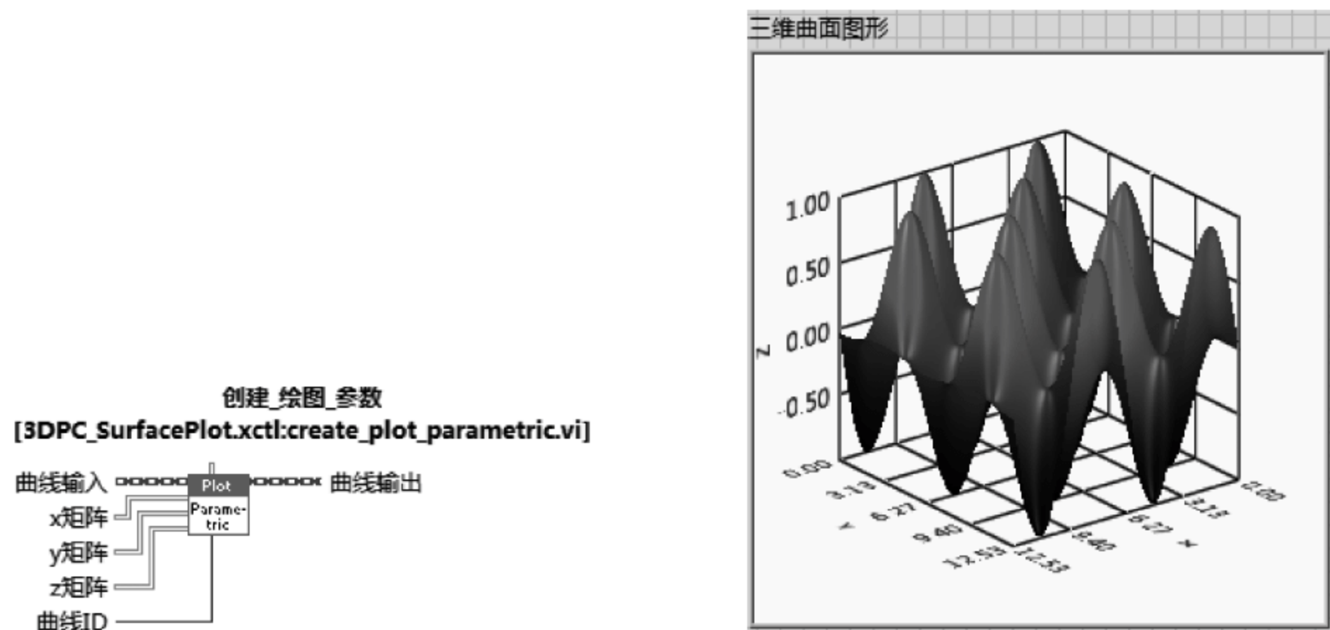
图 5.26 creat_plot_parametric.vi 的端口
