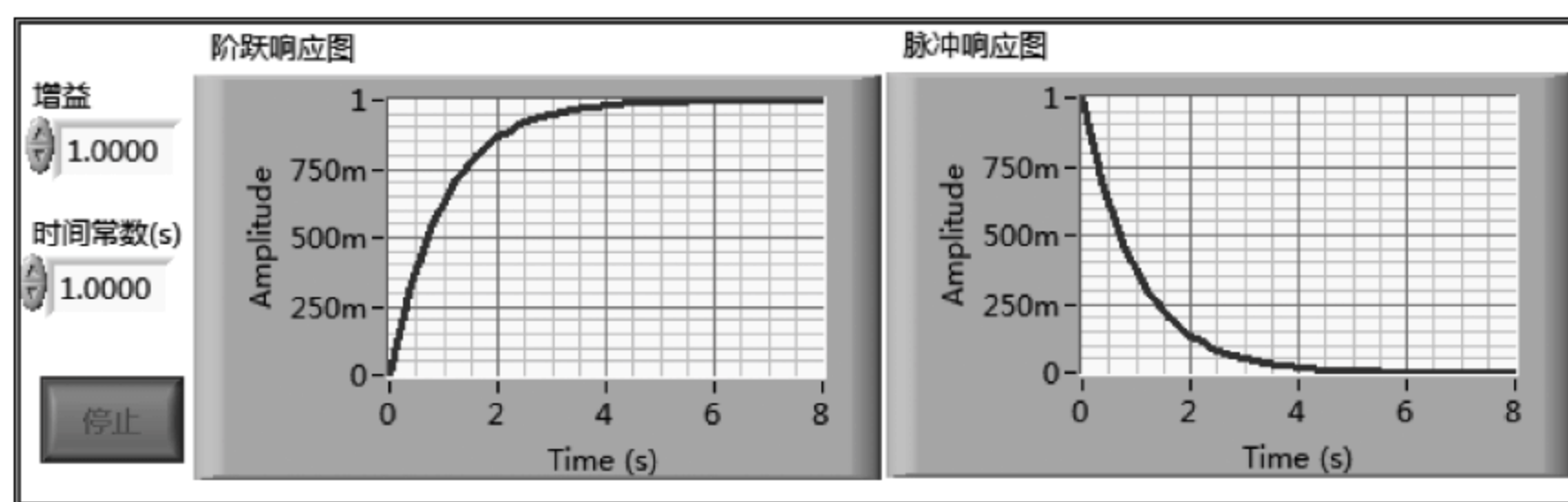
图 9.19 例 9.3 前面板
