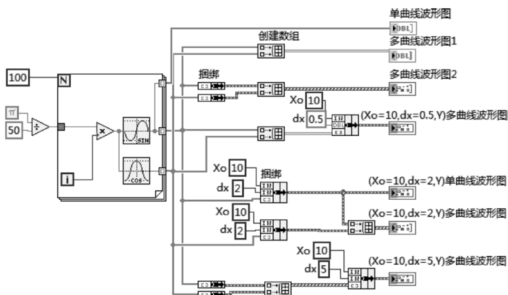
图 5.15 例 5.4 程序框图
