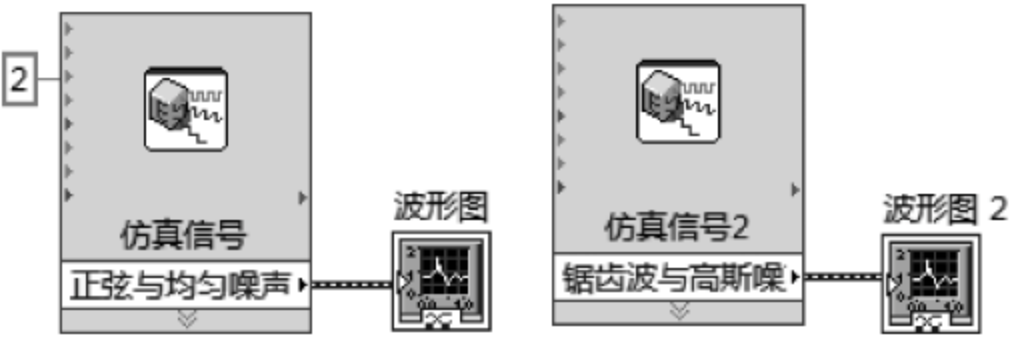
图 7.32 例 7.8 程序框图
