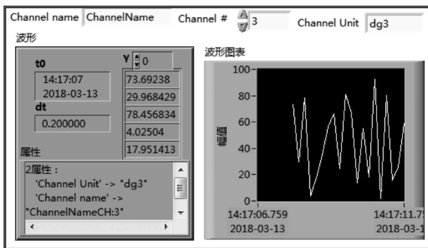
图 3.76 例 3.9 的前面板
