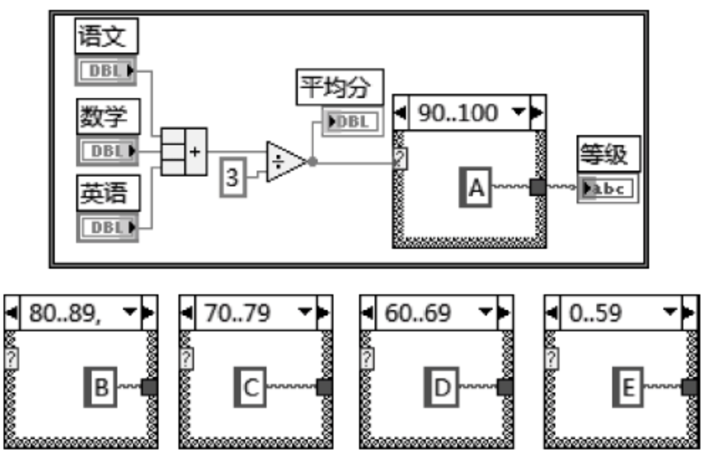
图 4.19 例 4.6 程序框图
