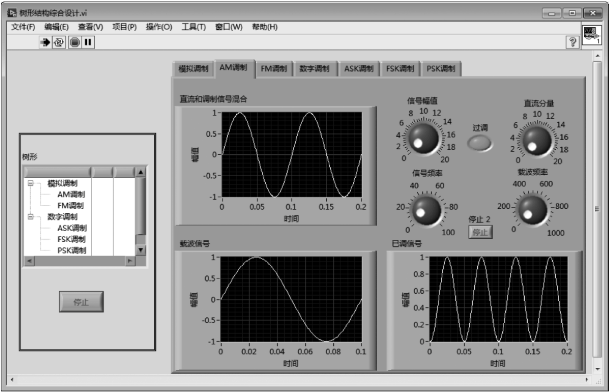
图 8.21 综合设计程序的 AM 调制分支
