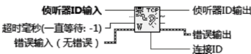
图 6.33 等待 TCP 侦听器节点
