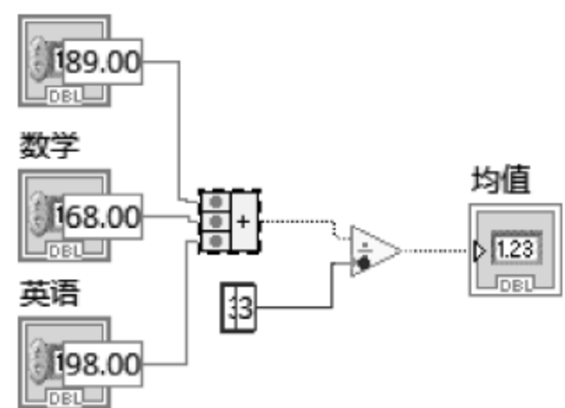
图 2.10 单步步过“复合运算”
