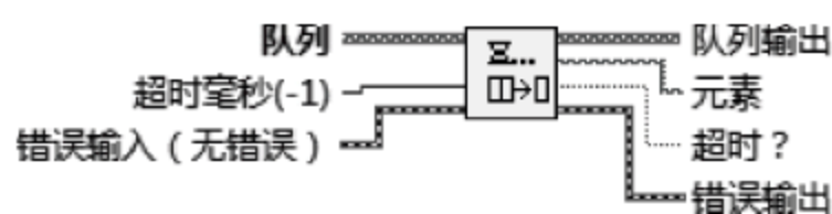
图 6.10 元素队列函数
