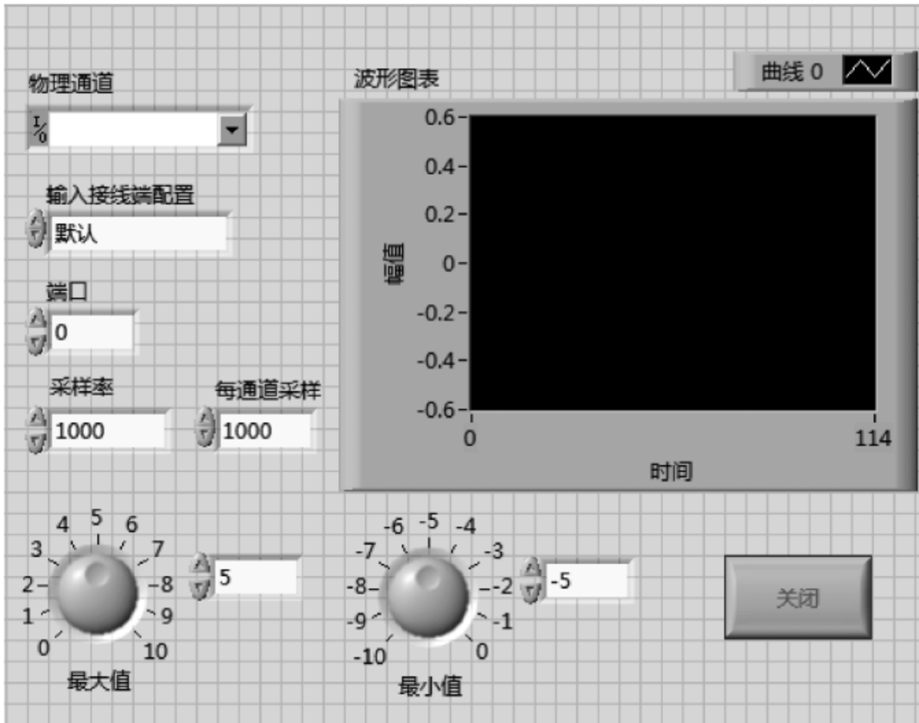
图 12.20 TCP/IP 采集系统发送端前面板设计
