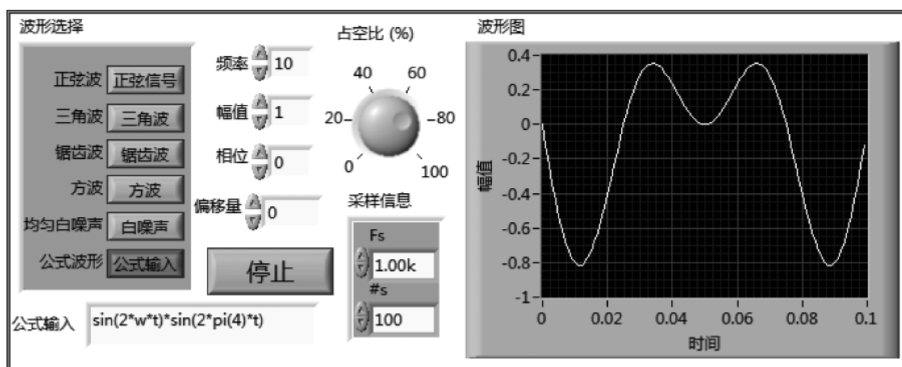
图 7.60 信号发生器前面板
