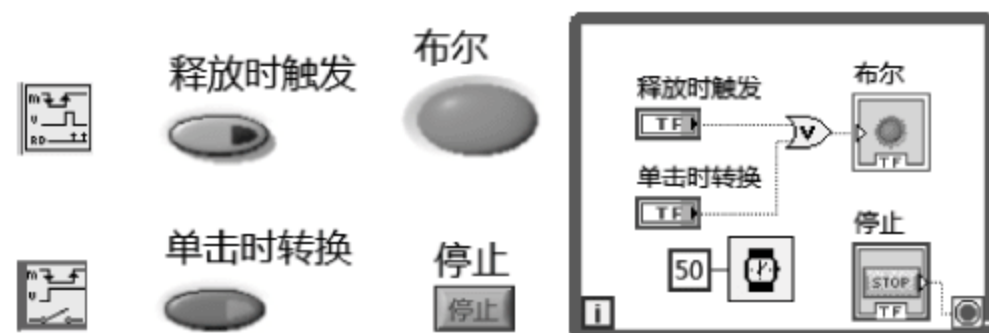
图 3.15 例 3.2 前面板和程序框图
