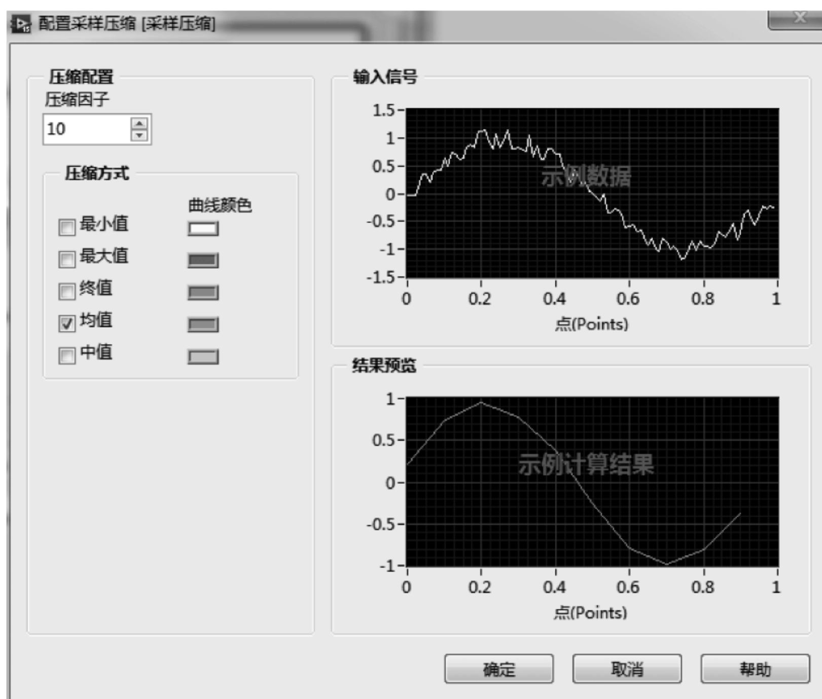
图 7.44 配置采样压缩界面
