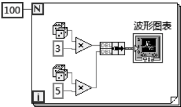
图 5.9 例 5.1 程序框图
