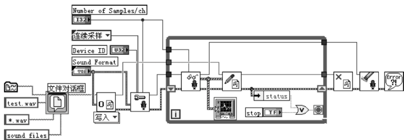
图 13.4 声音采集模块程序框图
