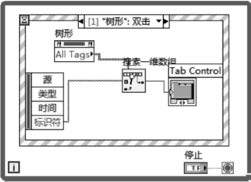
图 8.20 “双击”事件结构分支
