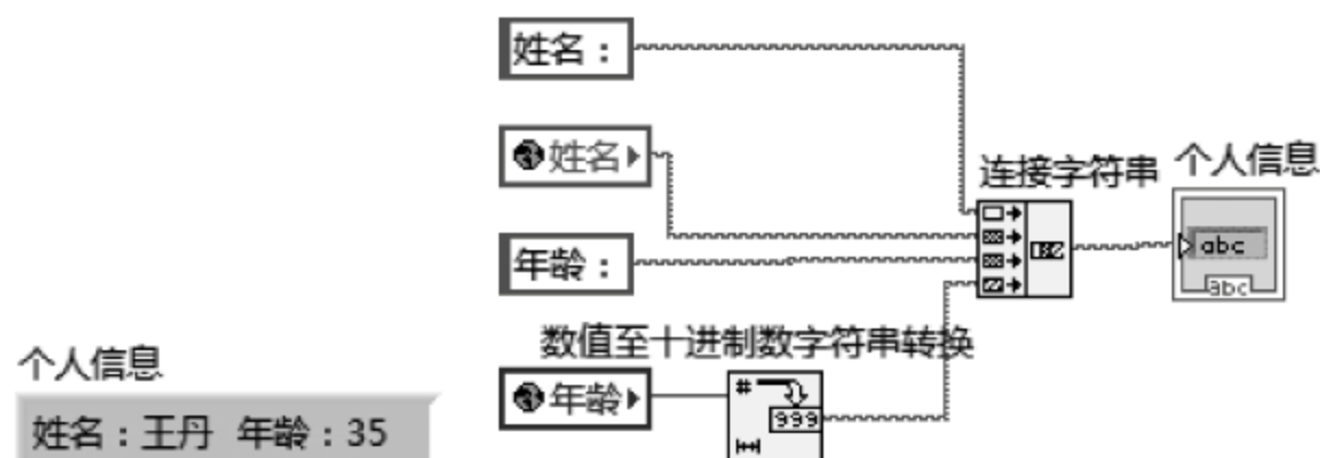
图 4.39 例 4.14 的前面板和程序框图
