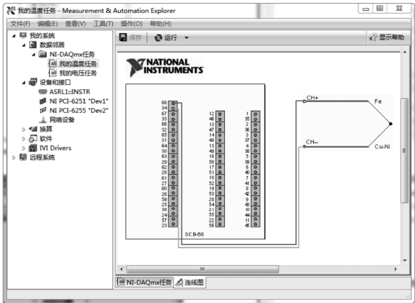
图 10.19 硬件连接示意图
