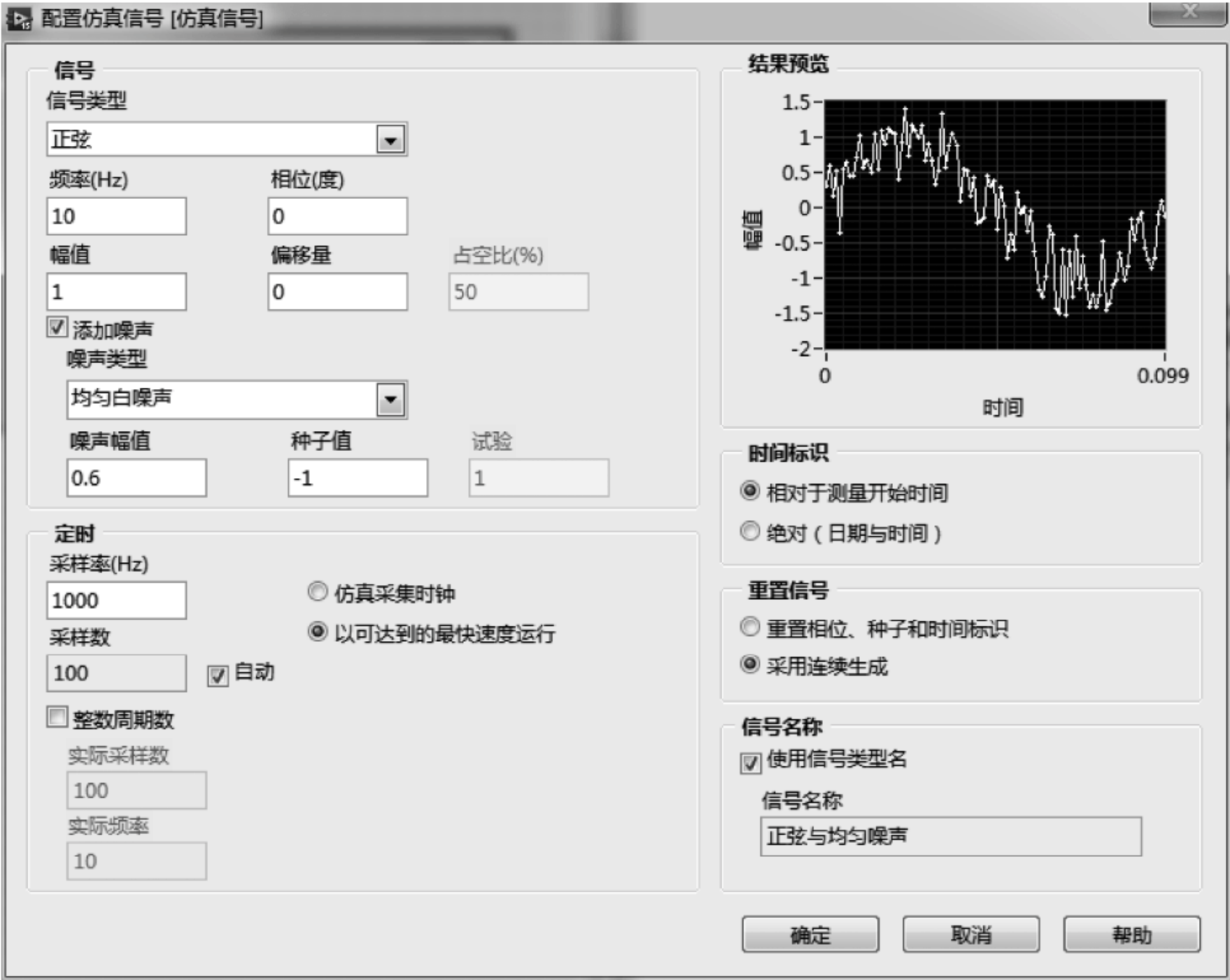
图 7.30 配置仿真信号
