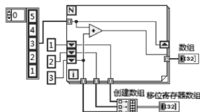
图 4.10 多个移位寄存器输入端子
