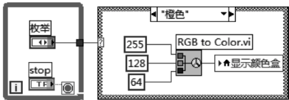
图 4.36 橙色颜色的程序框图
