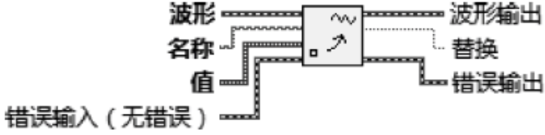
图 3.74 设置波形属性函数
