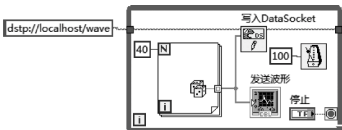
图 6.22 例 6.3 服务器的程序框图
