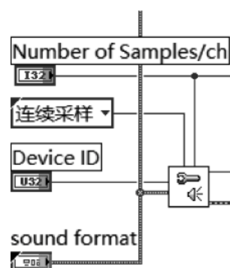
图 13.10 配置声音输出函数
