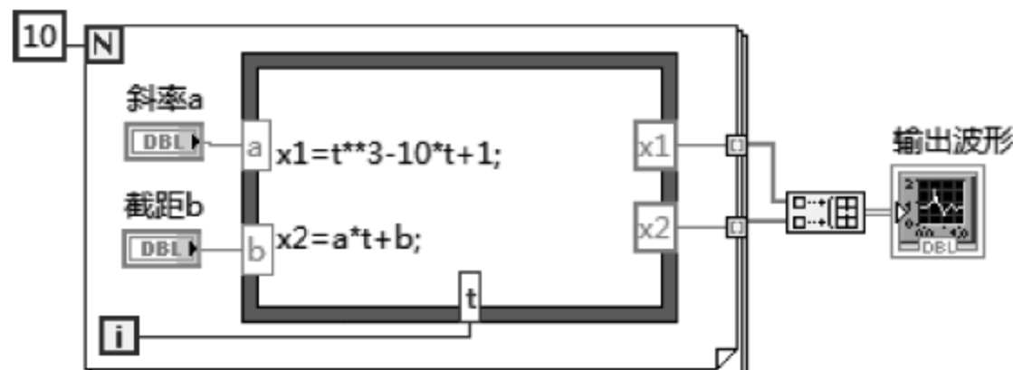
图 4.32 例 4.11 的程序框图
