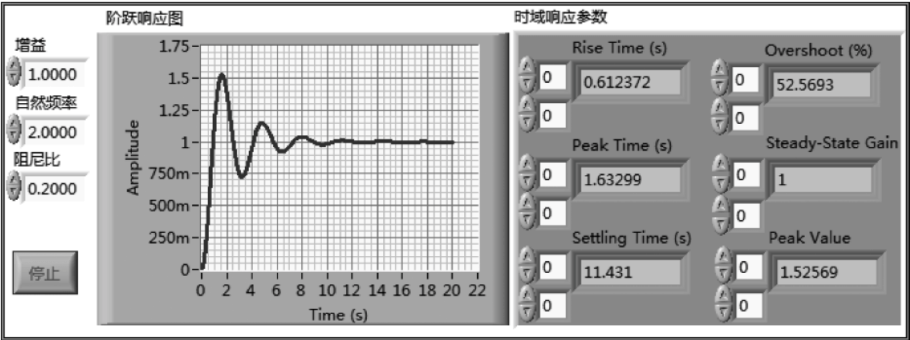
图 9.21 例 9.4 的前面板
