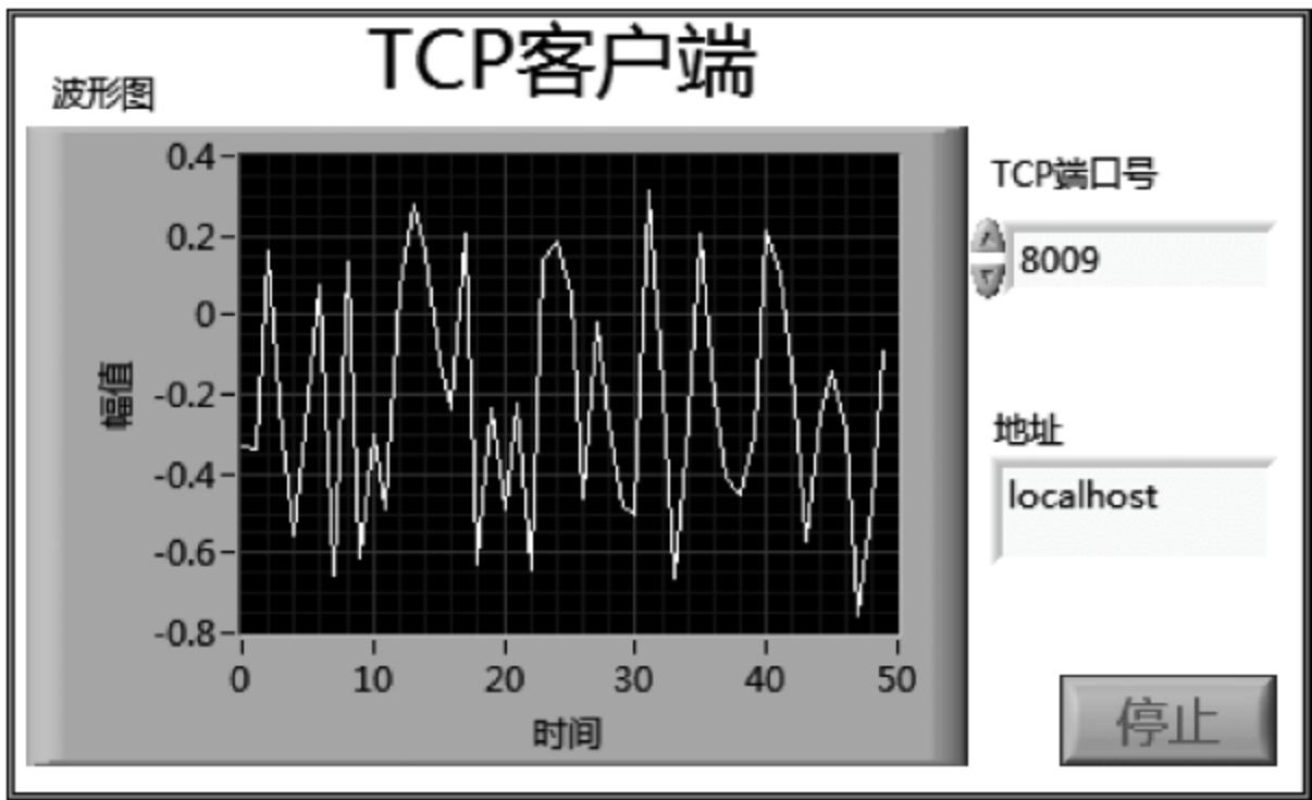
图 6.37 TCP 通信客户机程序前面板
