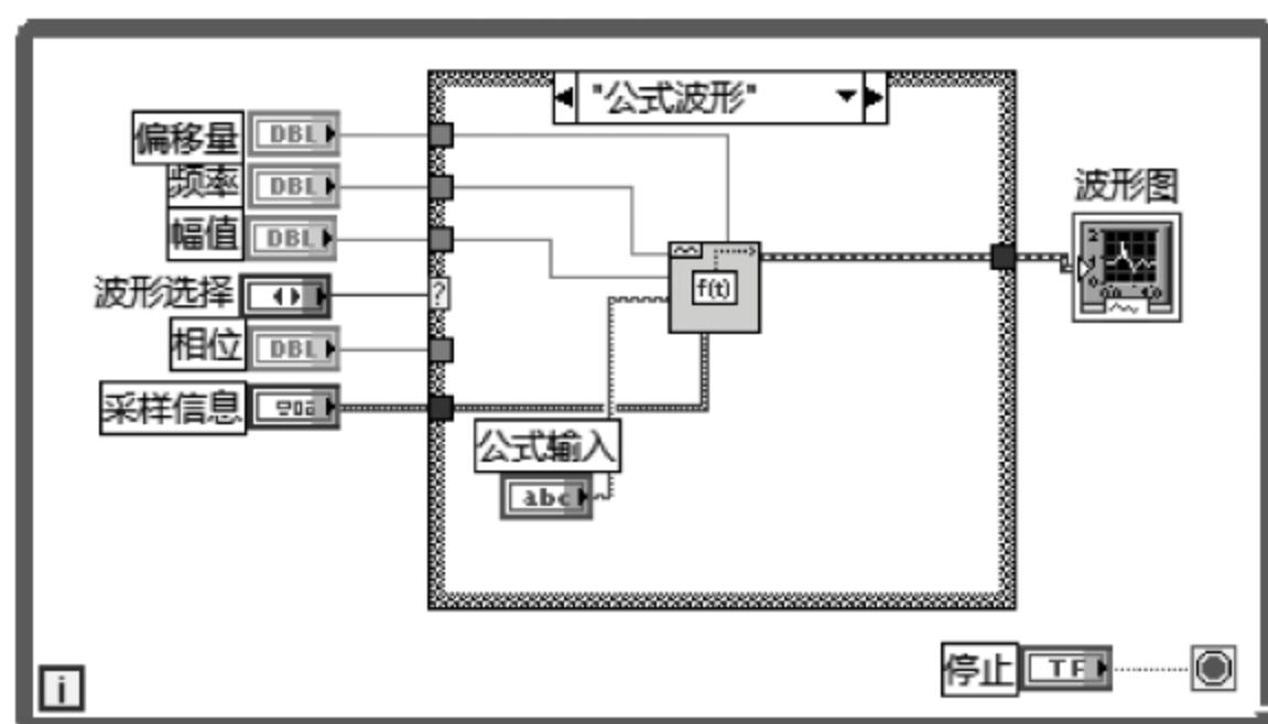
图 7.61 信号发生器程序框图(公式波形分支)
