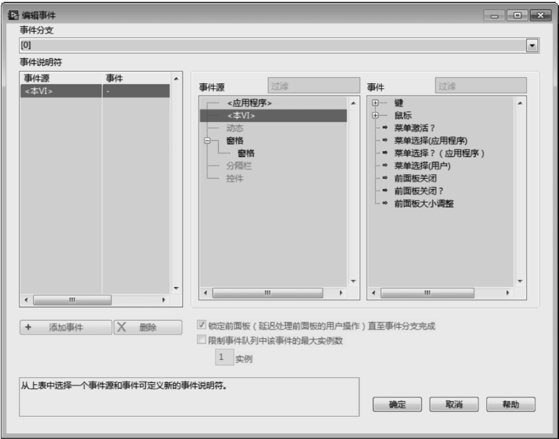
图 4.26 事件结构的编辑事件对话框
