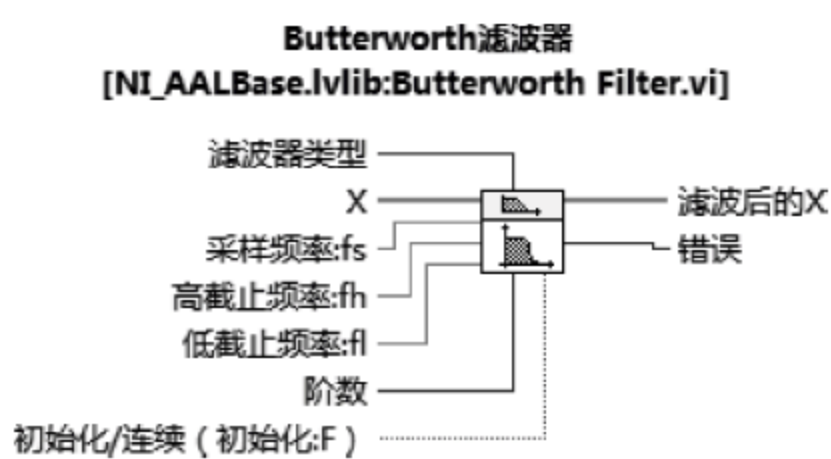
图 8.3 Butterworth 滤波器端口定义
