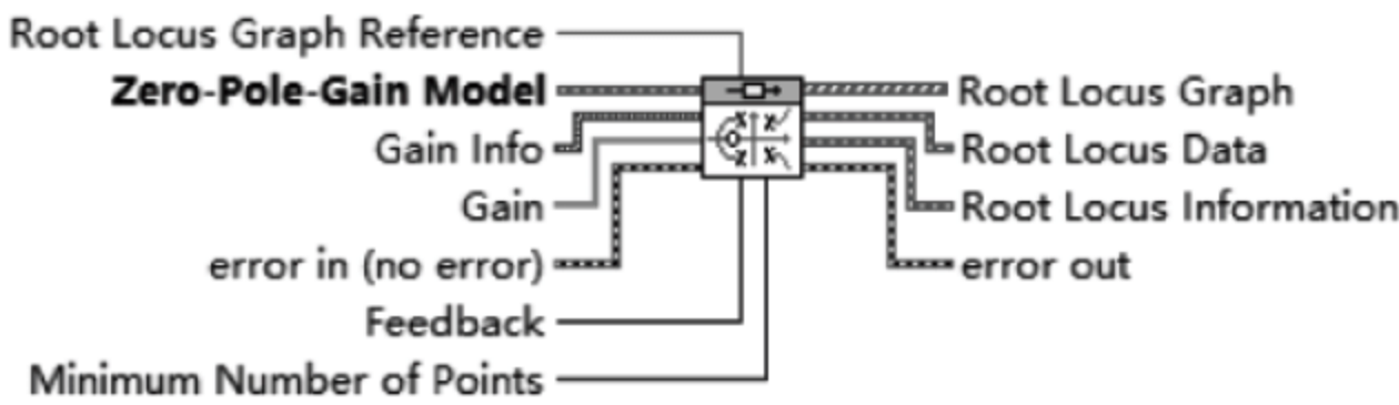
图 9.28 CD Root Locus. vi 函数
