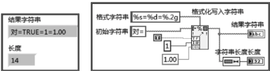
图 3.26 例 3.3 的前面板和程序框图
