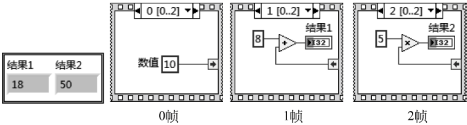
图 4.24 例 4.8 的前面板和程序框图
