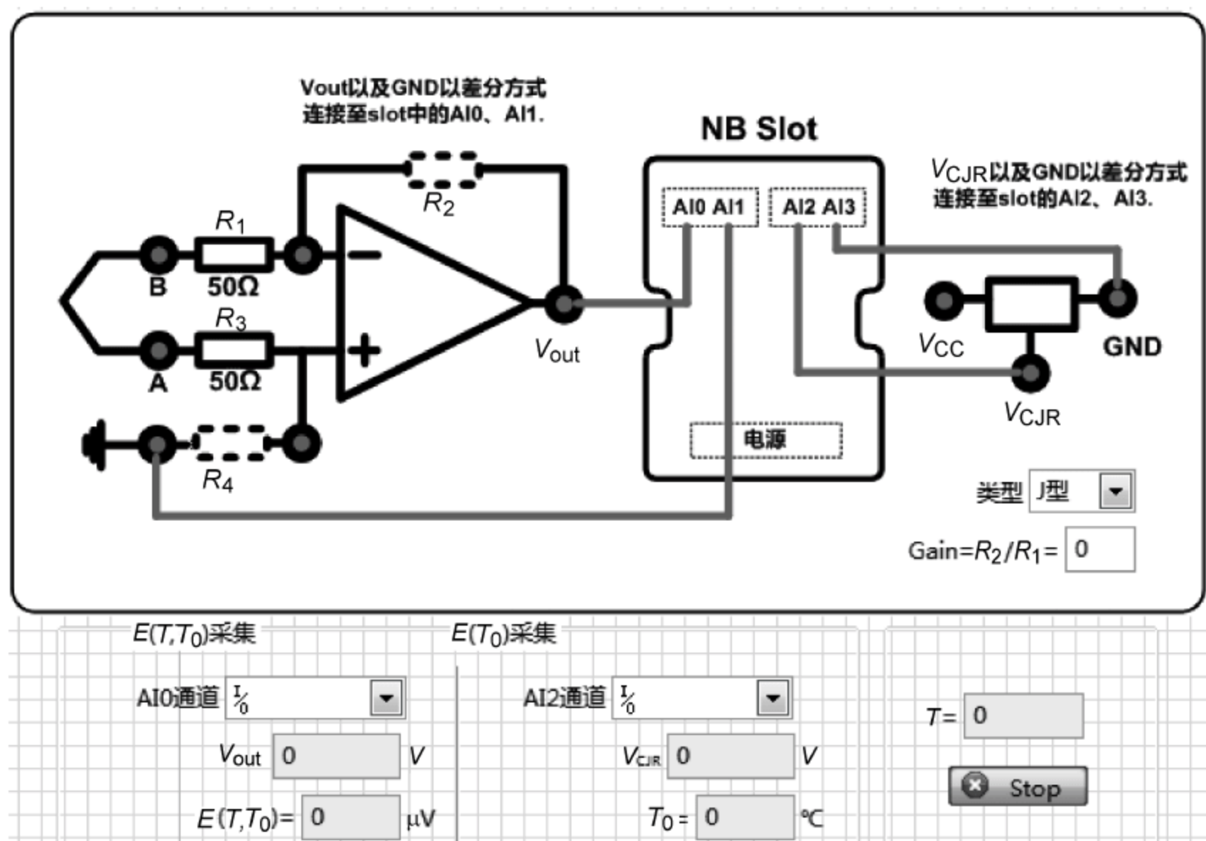
图 11.20 前面板设计框图
