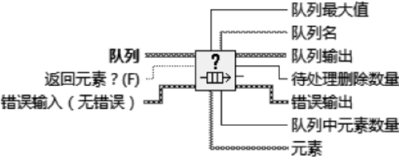
图 6.6 获取队列状态函数
