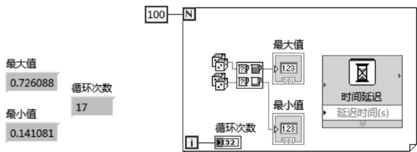
图 4.3 例 4.1 的前面板和程序框图
