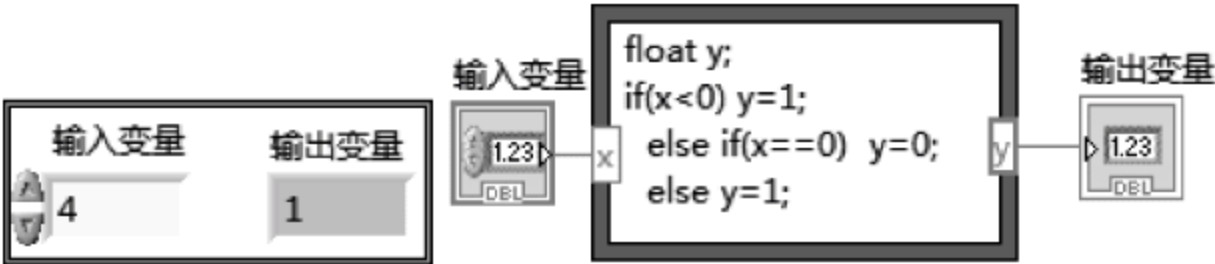
图 4.30 例 4.10 的前面板和程序框图
