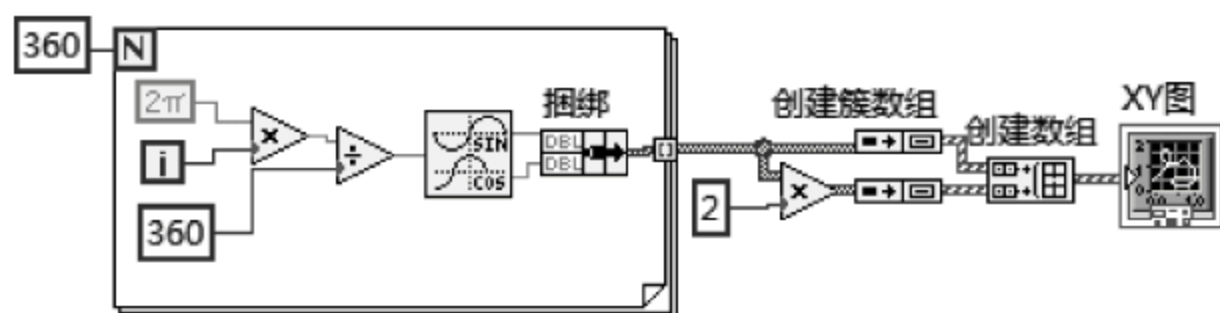
图 5.18 例 5.5 的程序框图
