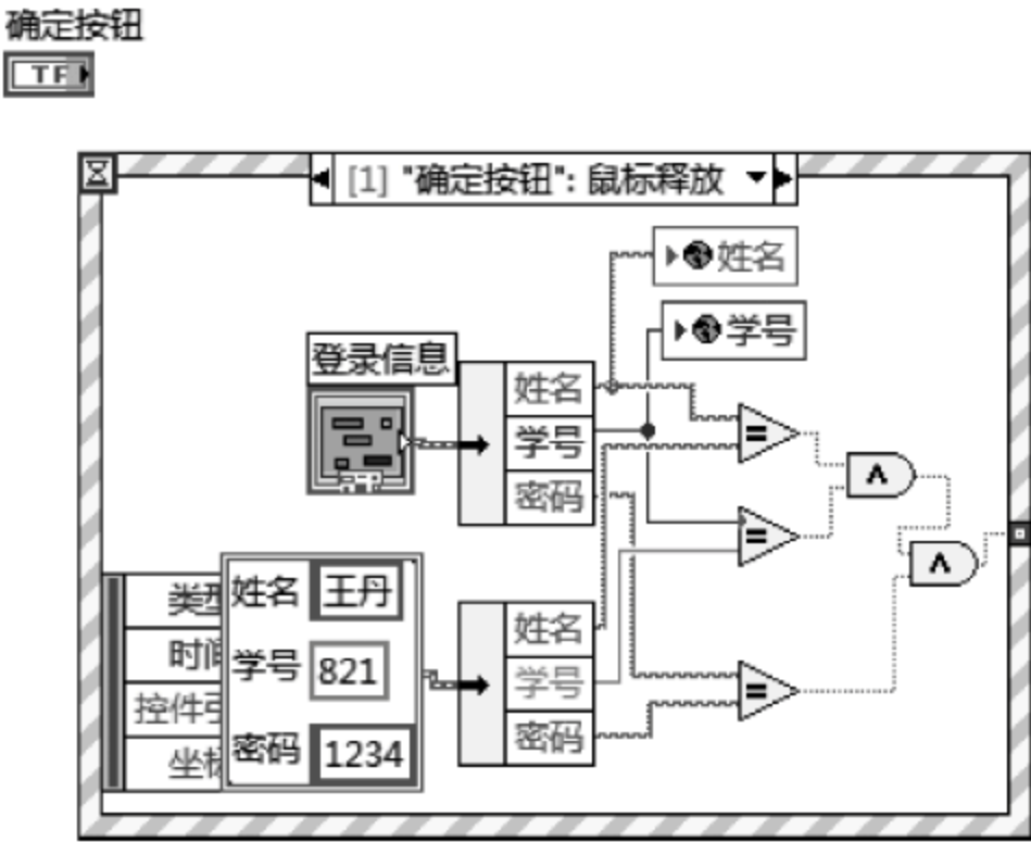
图 7.65 姓名和学号全局变量连线位置
