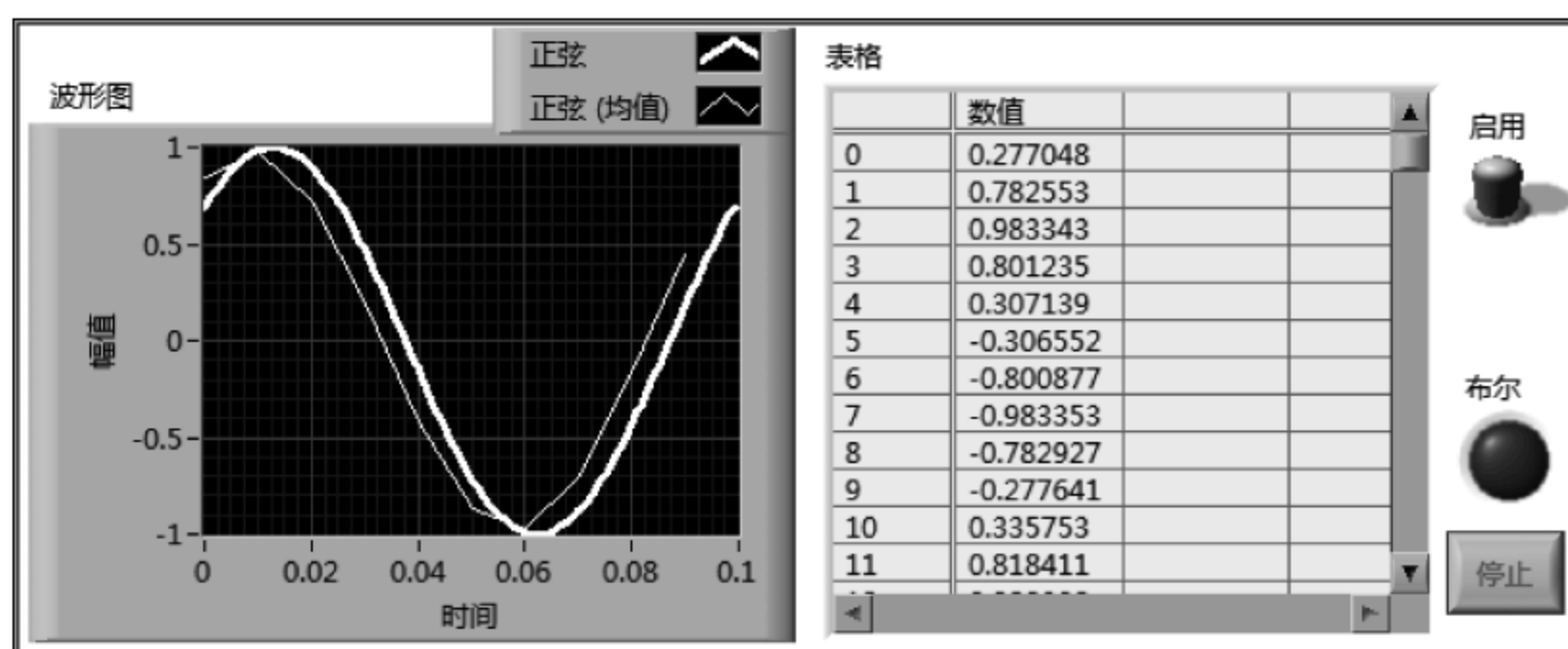
图 7.49 例 7.11 程序前面板
