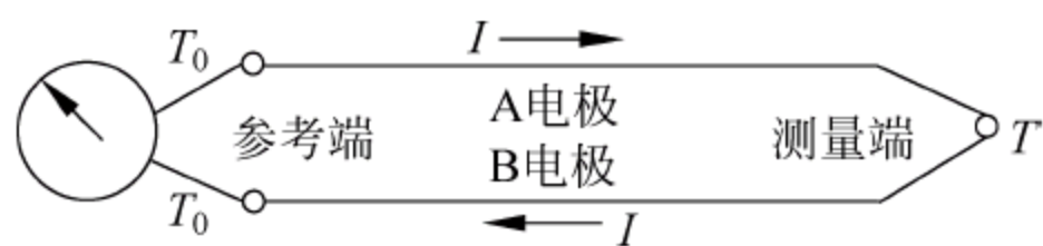
图 11.6 热电偶原理图
