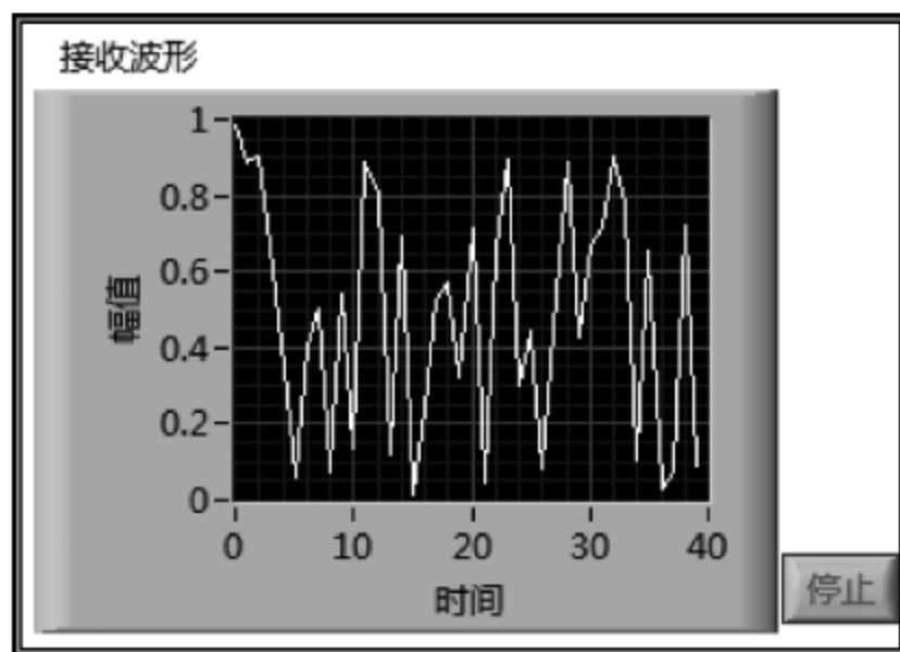
图 6.23 例 6.3 客户机的前面板
