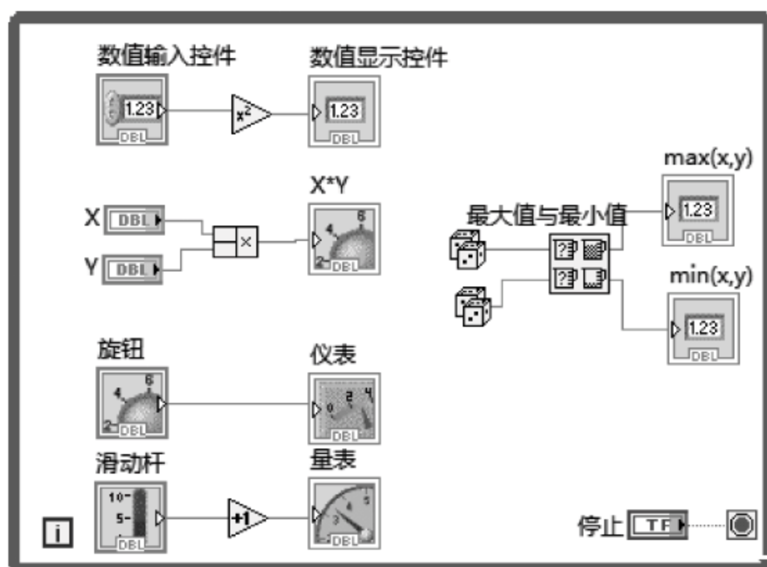
图 3.8 例 3.1 的程序框图
