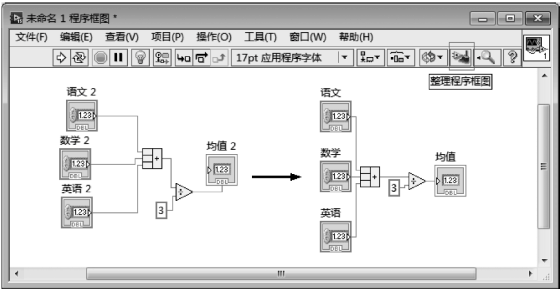
图 2.5 求均值程序框图
