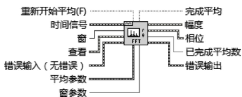
图 7.25 FFT 频谱(幅度-相位)的端口
