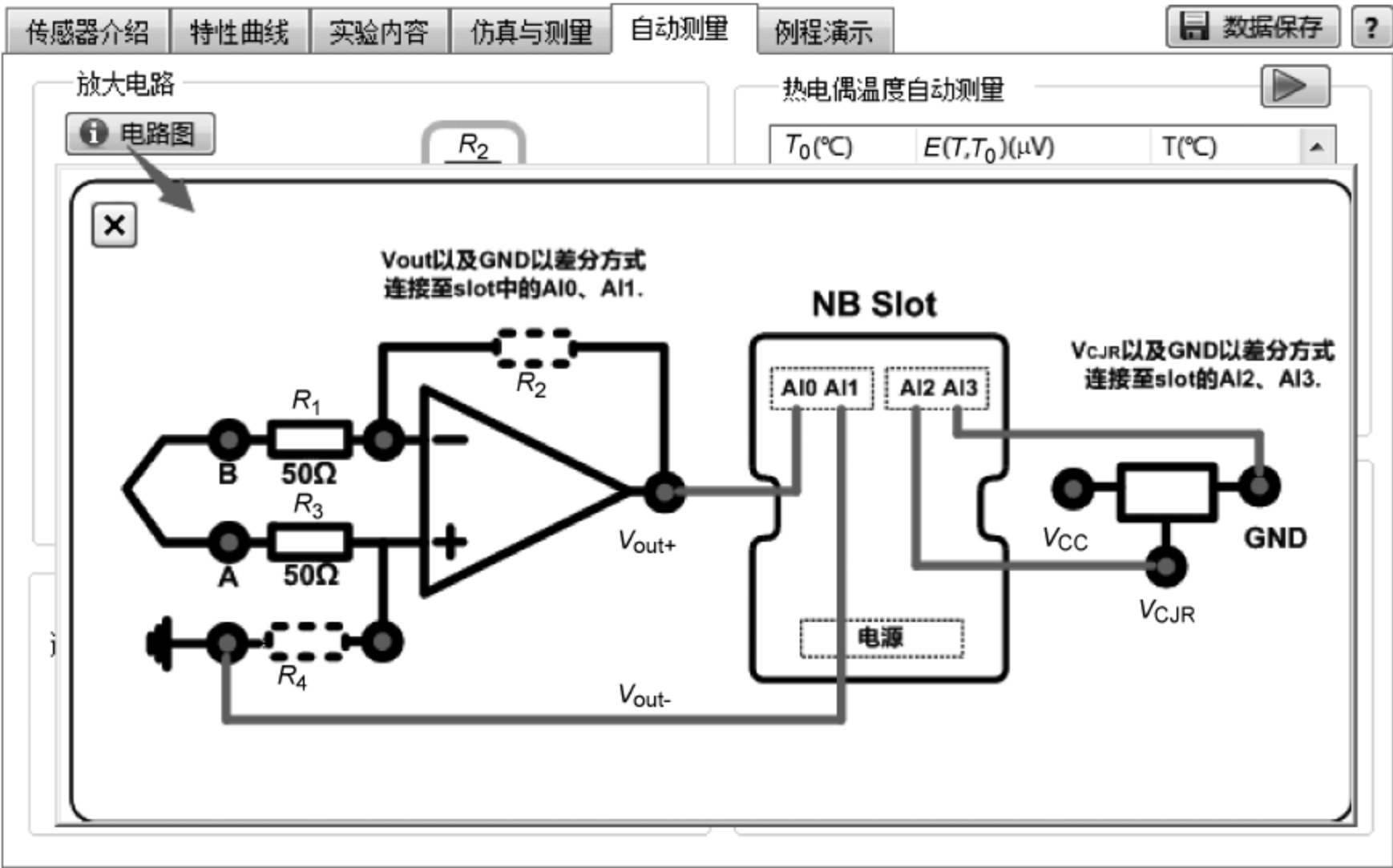
图 11.12 放大原理图
