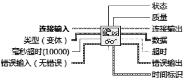
图 6.14 读取 DataSocket 函数
