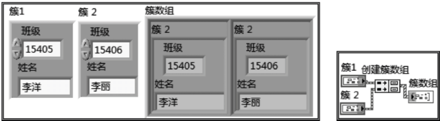
图 3.66 创建簇数组前面板和程序框图
