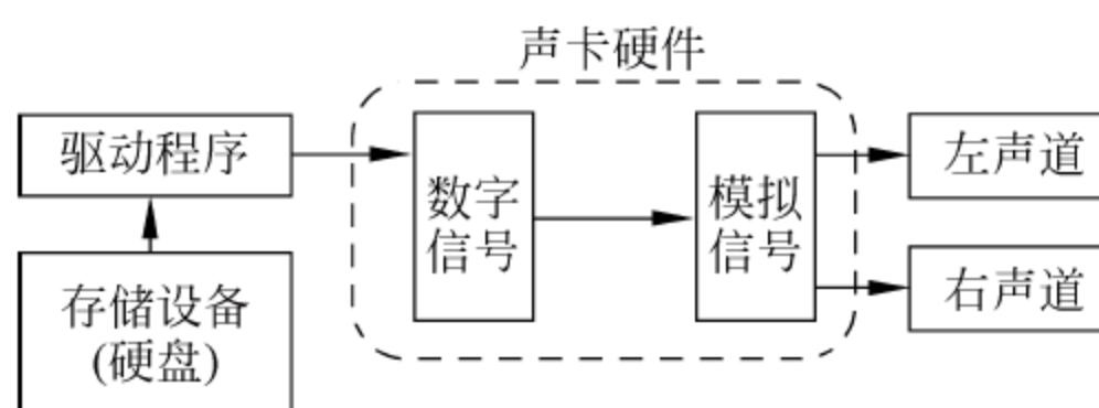
图 13.2 声卡播放原理图
