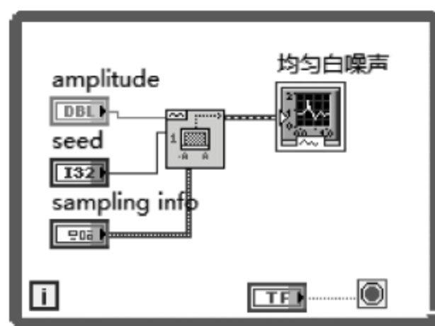
图 7.6 例 7.1 程序框图
