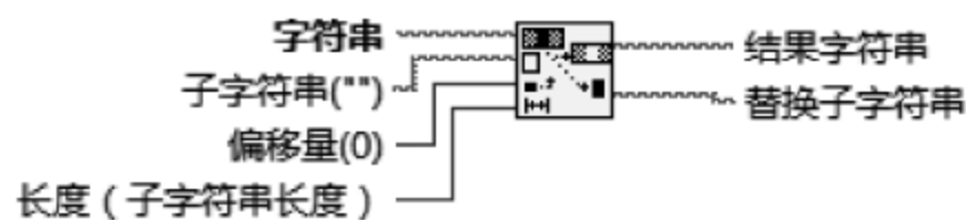
图 3.24 替换子字符串的函数
