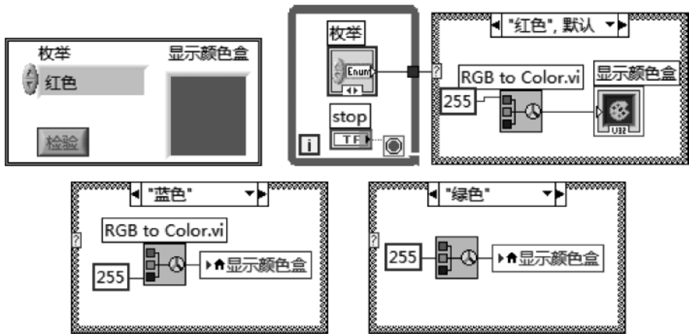
图 4.34 例 4.12 的前面板和程序框图
