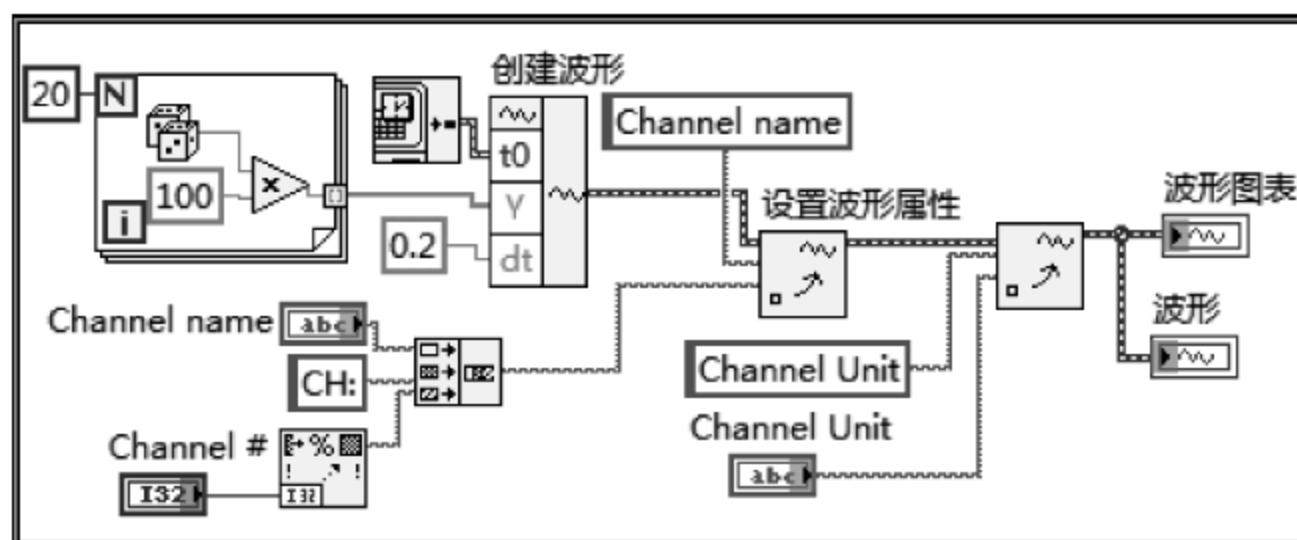
图 3.77 例 3.9 的程序框图
