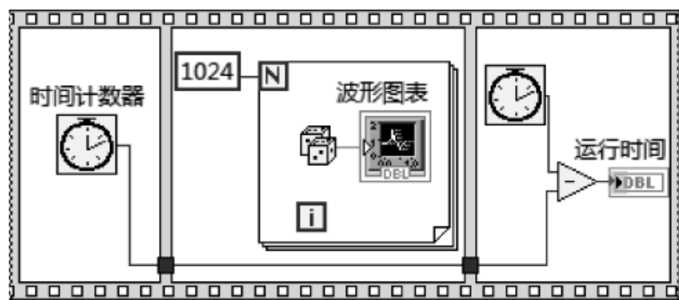
图 4.23 例 4.7 的程序框图
