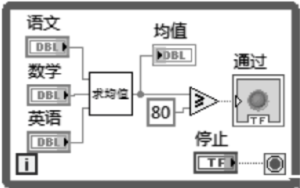
图 2.19 主 VI 的前面板
