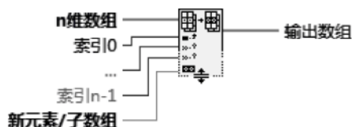
图 3.46 “替换数组子集”的节点图标及端口
