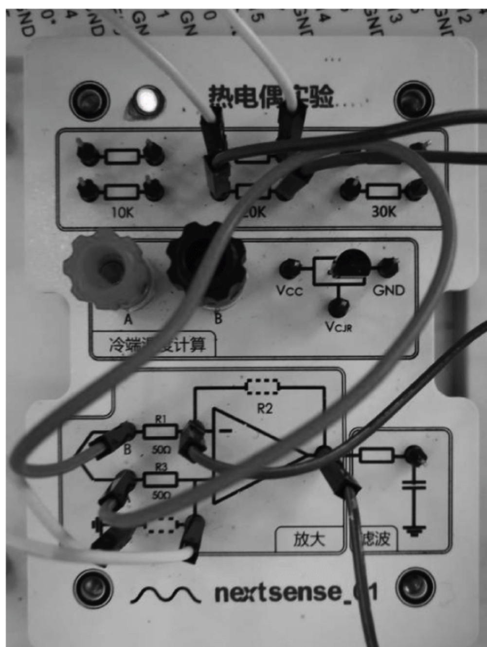
图 11.16 调零电路硬件实物图
