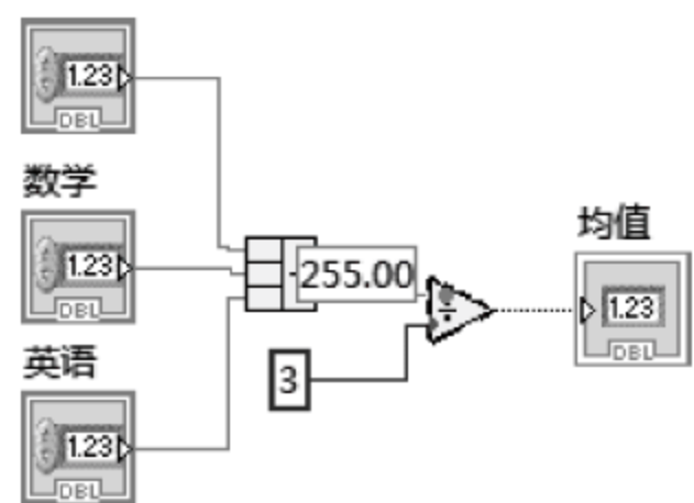
图 2.11 单步步过“除法运算”
