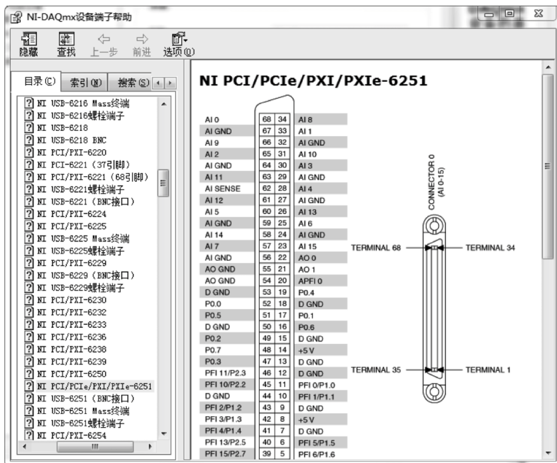
图 10.13 NI-DAQmx 设备端子
