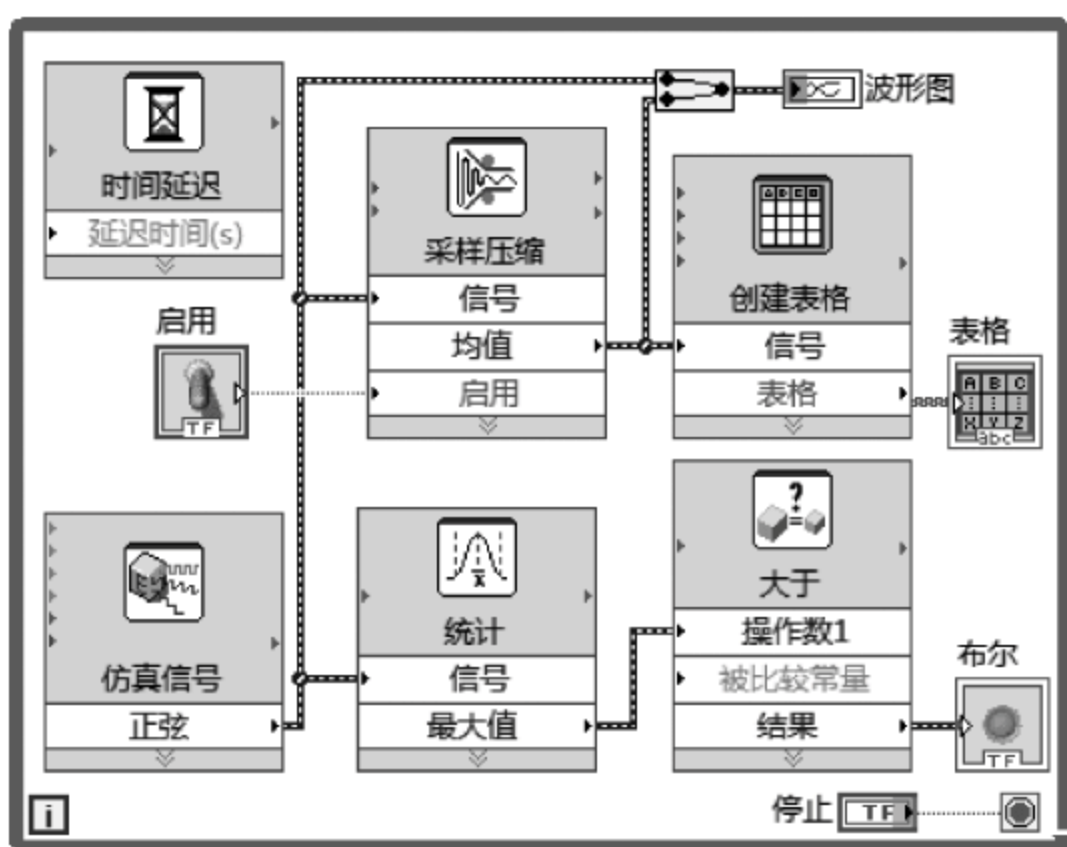
图 7.48 例 7.11 程序的程序框图
