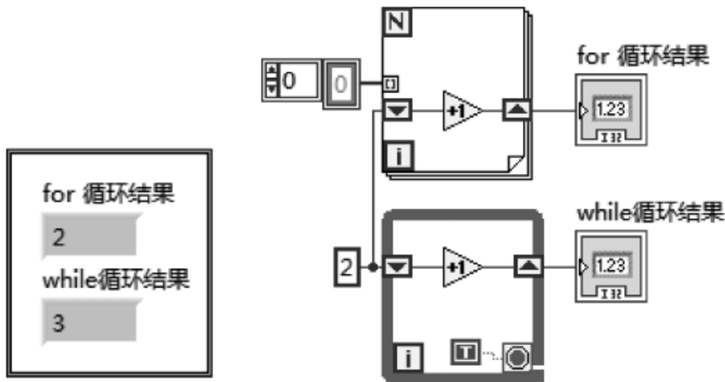
图 4.15 例 4.4 for 和 while 运行次数区别
