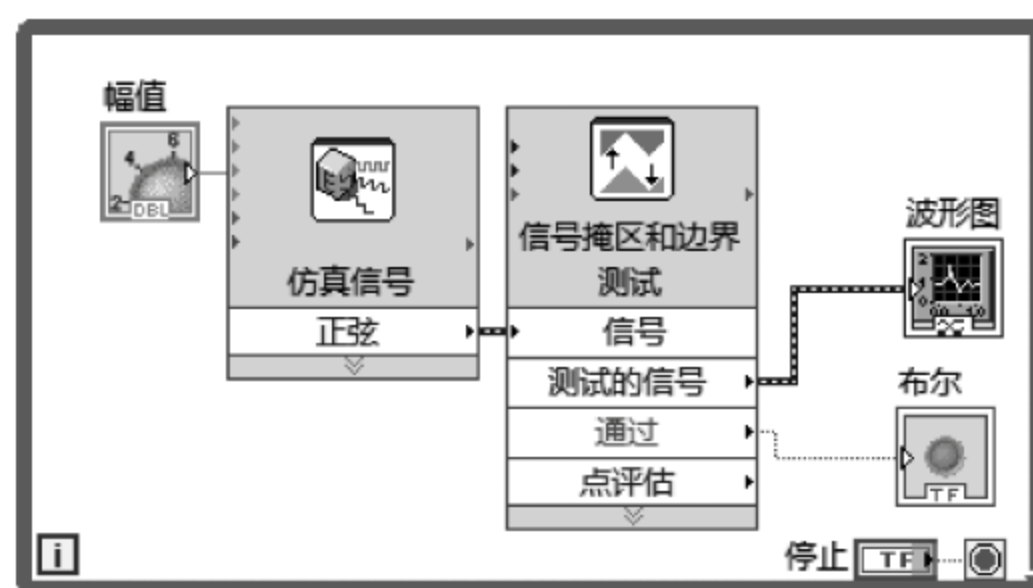
图 7.38 例 7.9 程序框图
