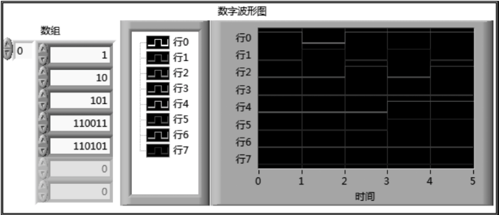
图 5.21 例 5.7 的前面板
