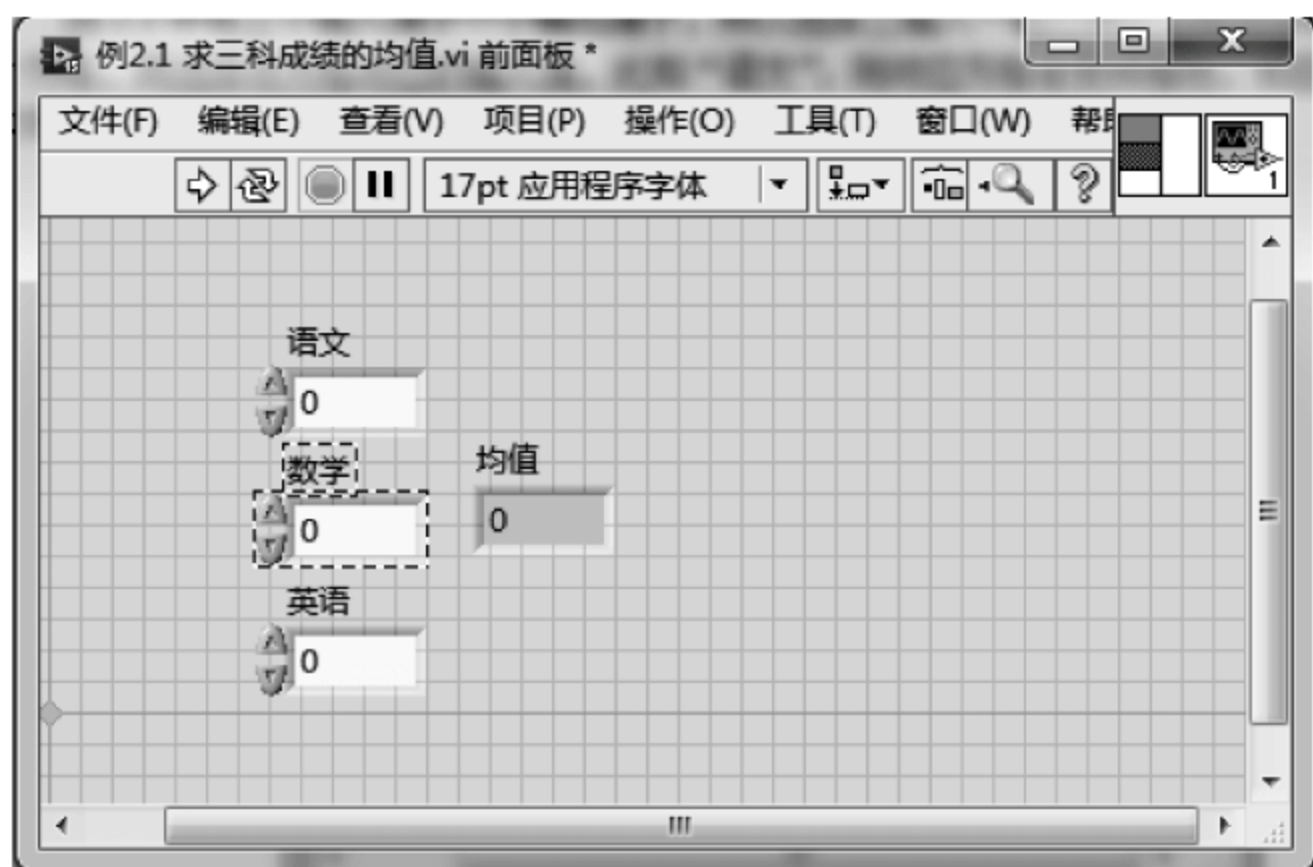
图 2.15 连线板选择
