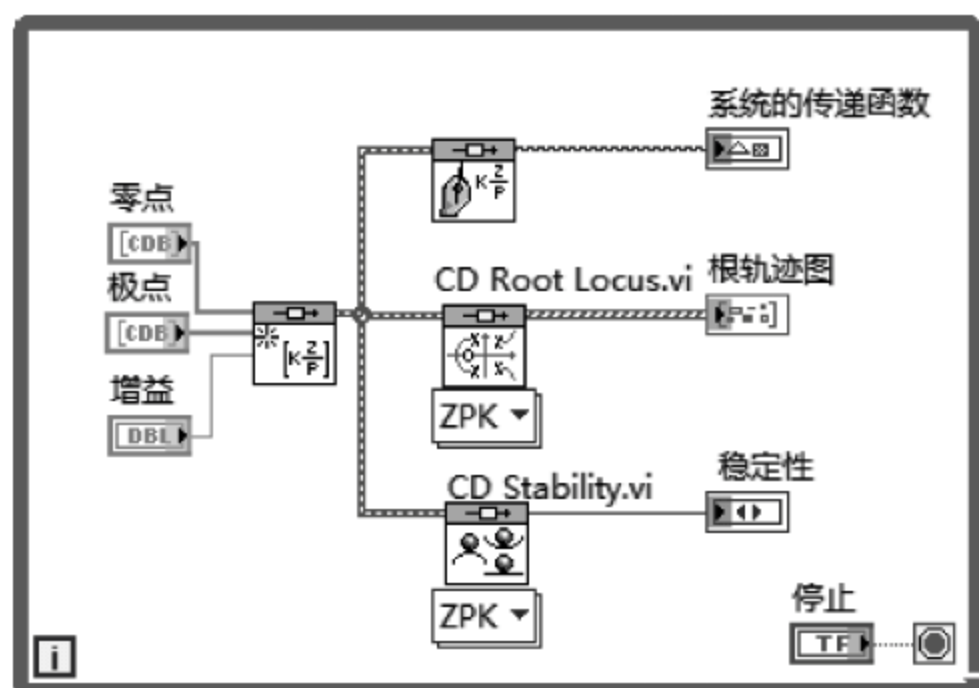
图 9.30 例 9.6 程序框图
