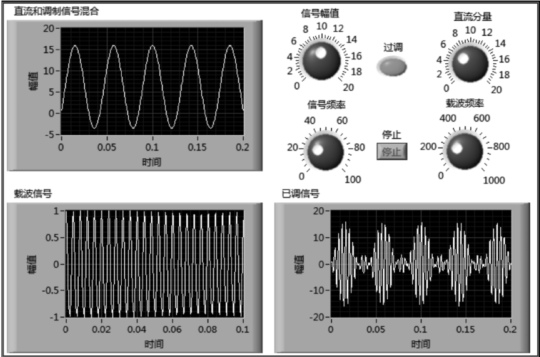
图 8.2 例 8.1 前面板
