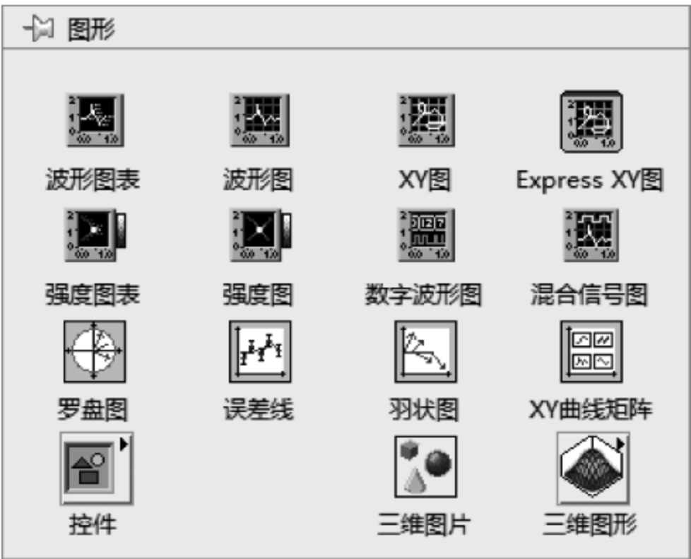
图 5.1 “图形”子选板
