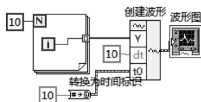
图 5.13 例 5.3 程序框图
