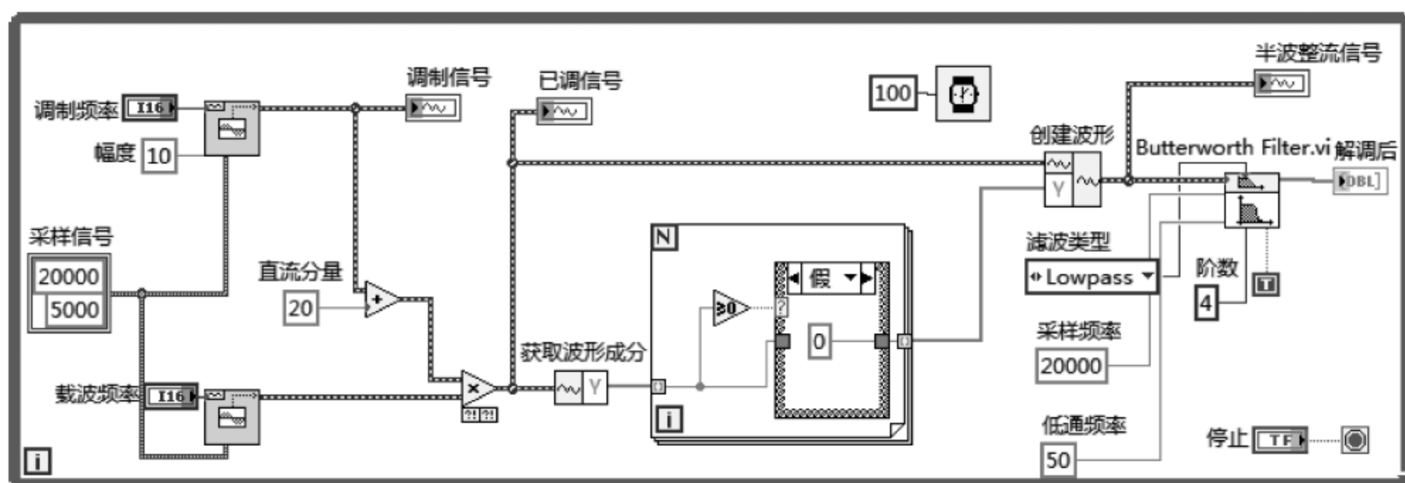
图 8.4 例 8.2 程序框图
