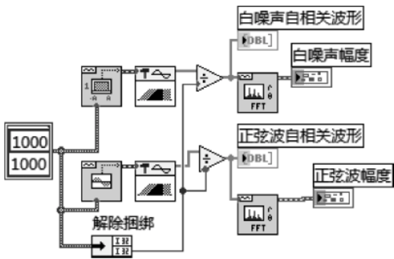
图 7.27 例 7.7 程序框图
