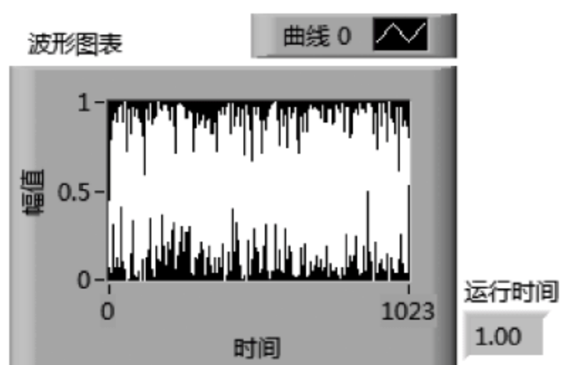
图 4.22 例 4.7 的前面板
