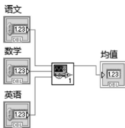
图 2.17 创建子 VI
