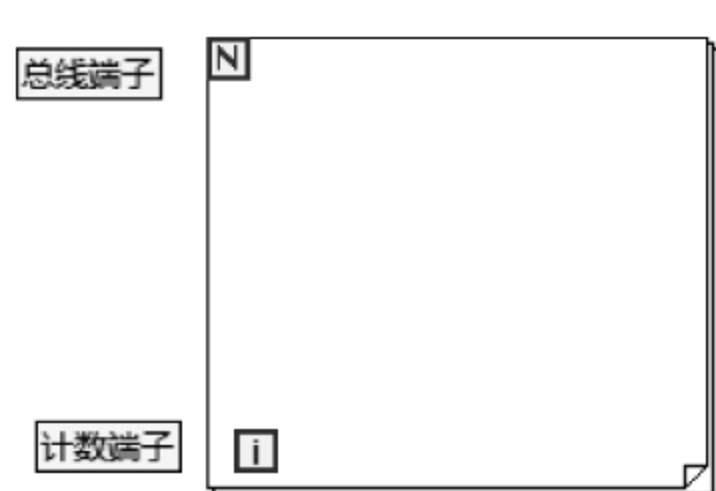
图 4.2 for 循环
