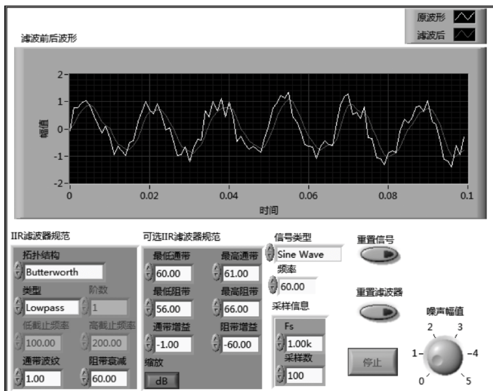
图 7.18 例 7.5 的前面板
