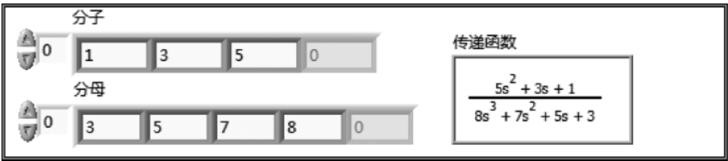
图 9.8 例 9.1 前面板
