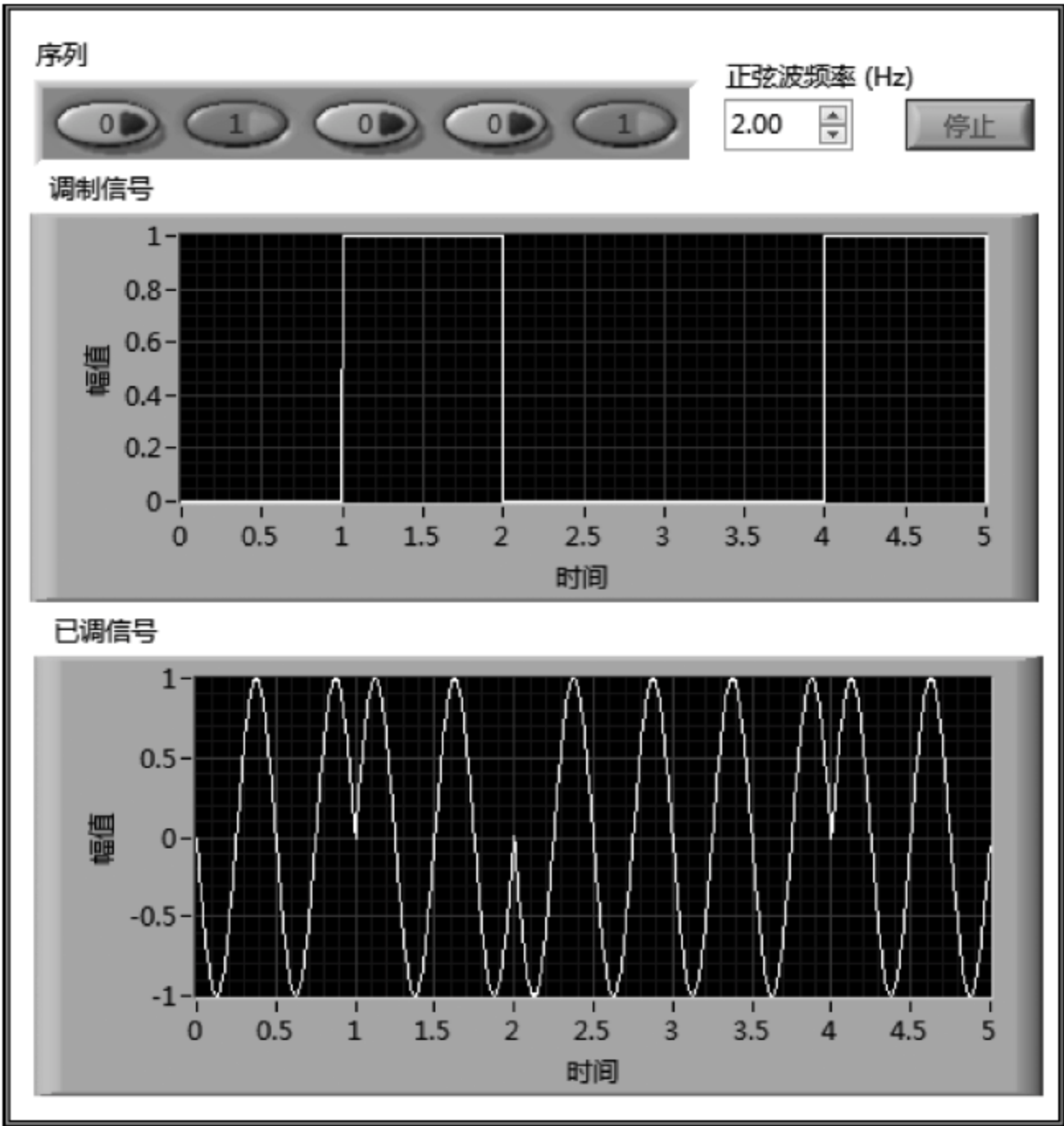
图 8.14 例 8.6 前面板
