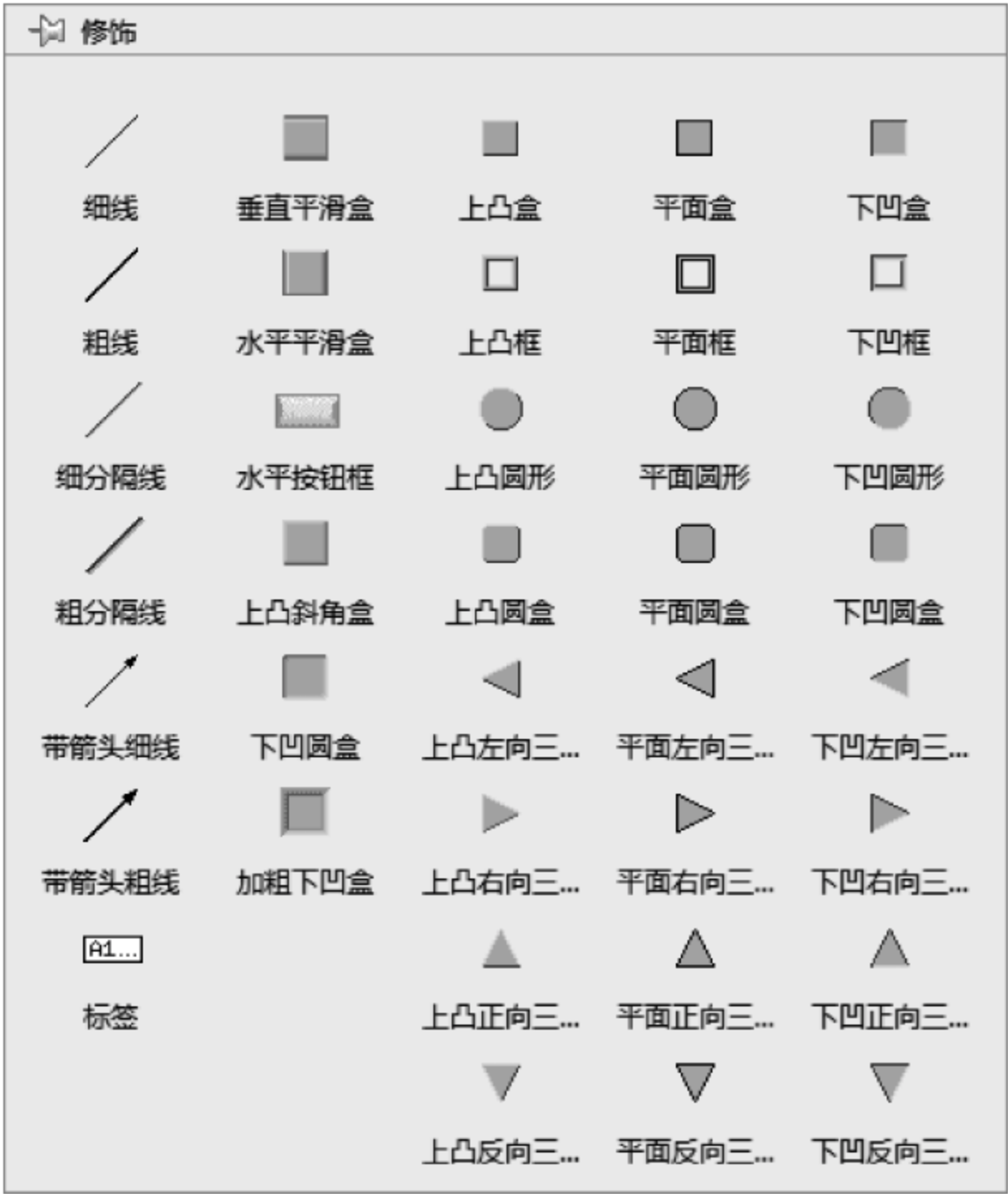
图 2.2 “修饰”子选板
