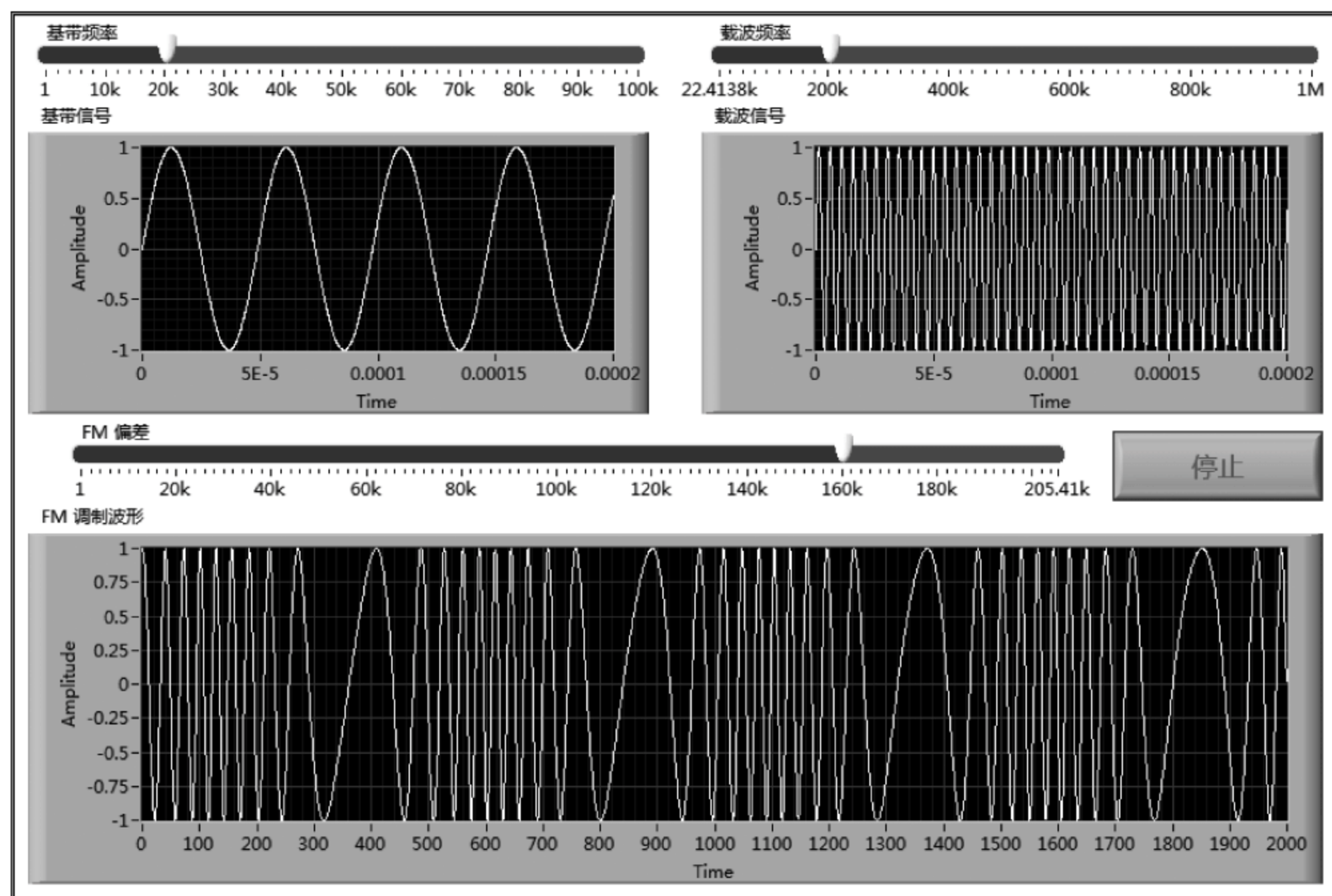
图 8.7 例 8.3 前面板
