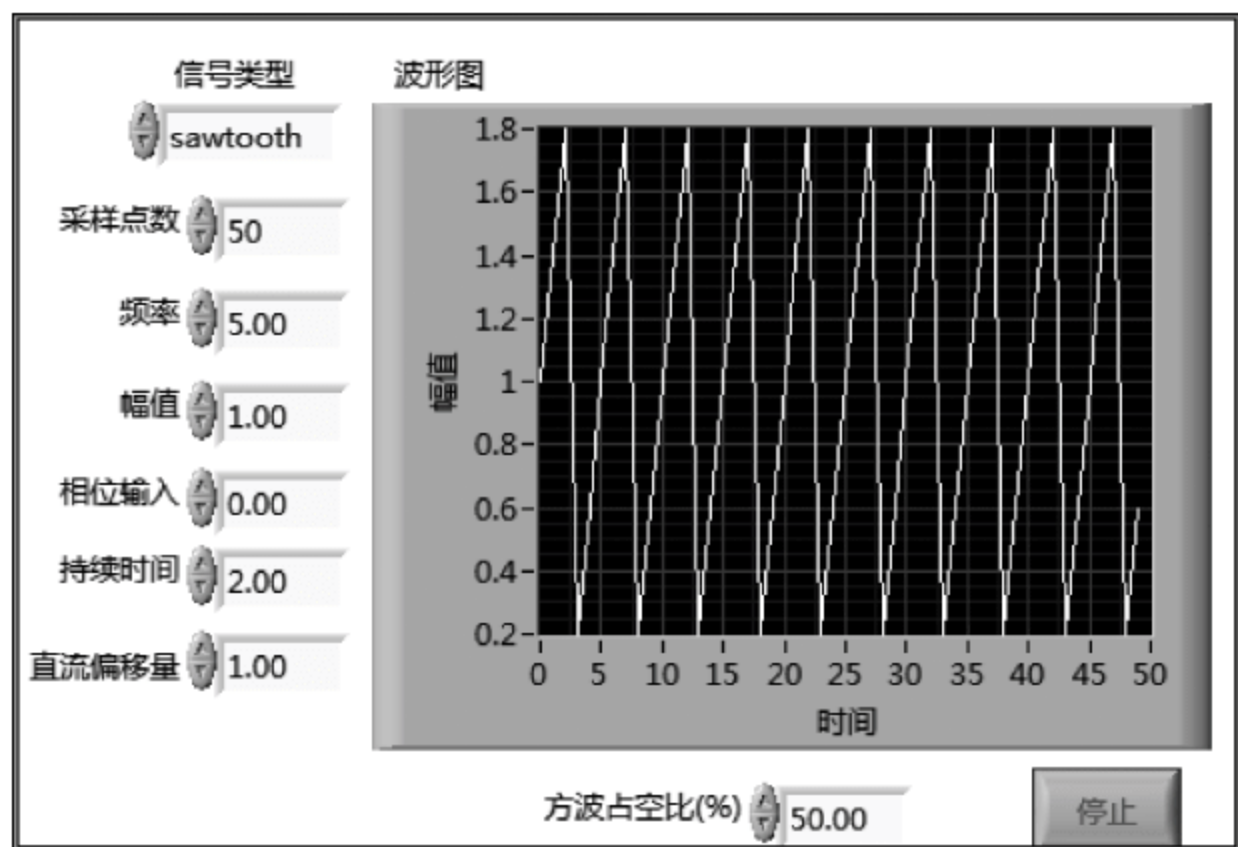
图 7.12 例 7.3 前面板
