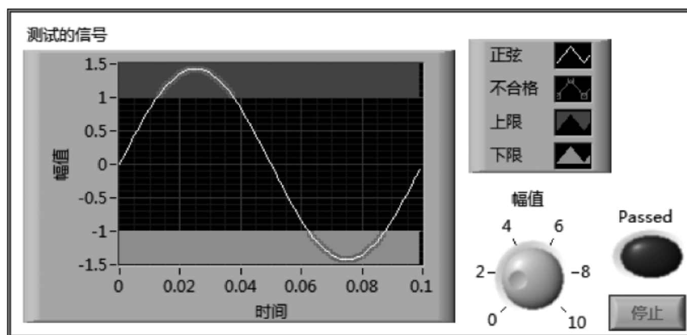
图 7.39 例 7.9 前面板
