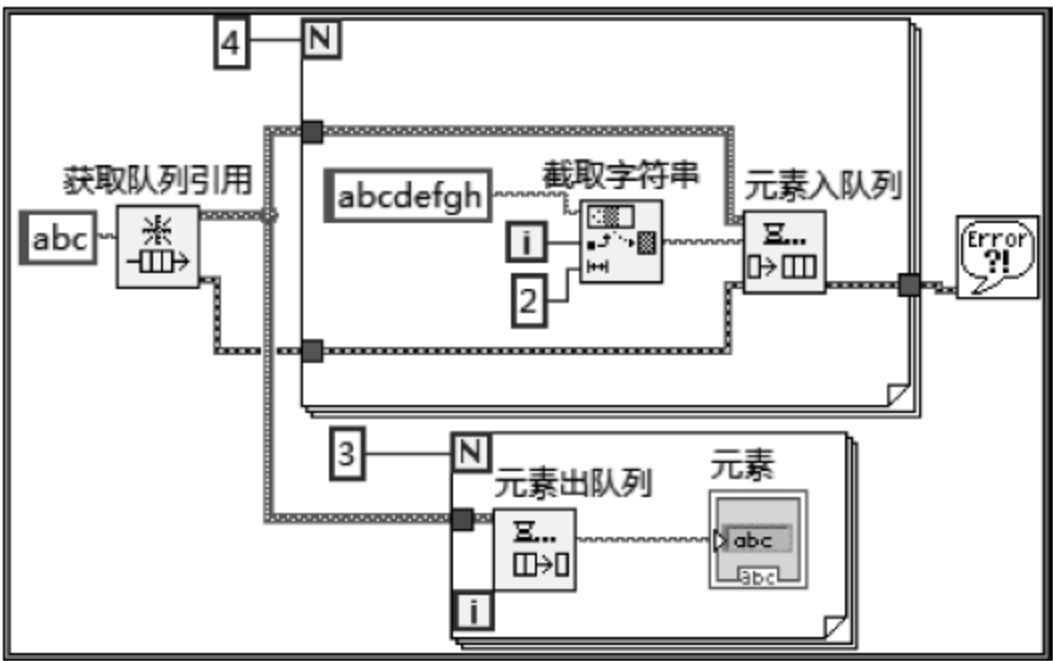
图 6.12 例 6.2 程序框图
