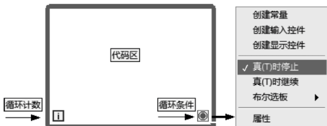
图 4.13 while 循环
