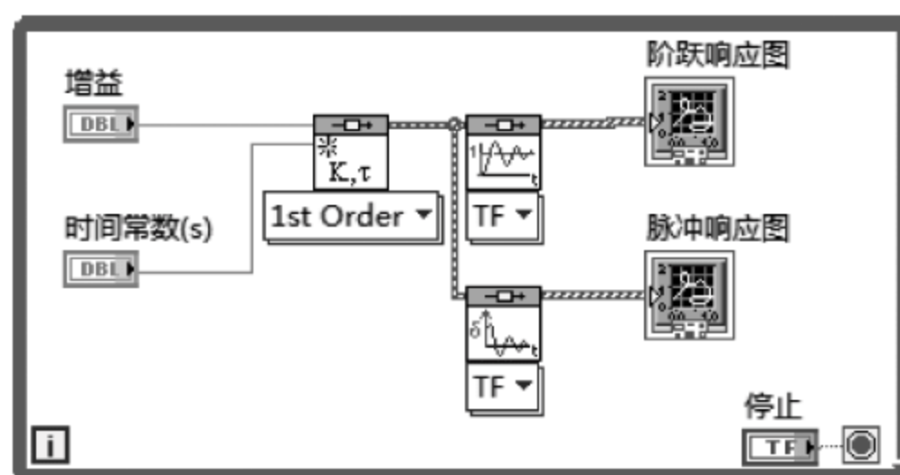
图 9.18 例 9.3 程序框图
