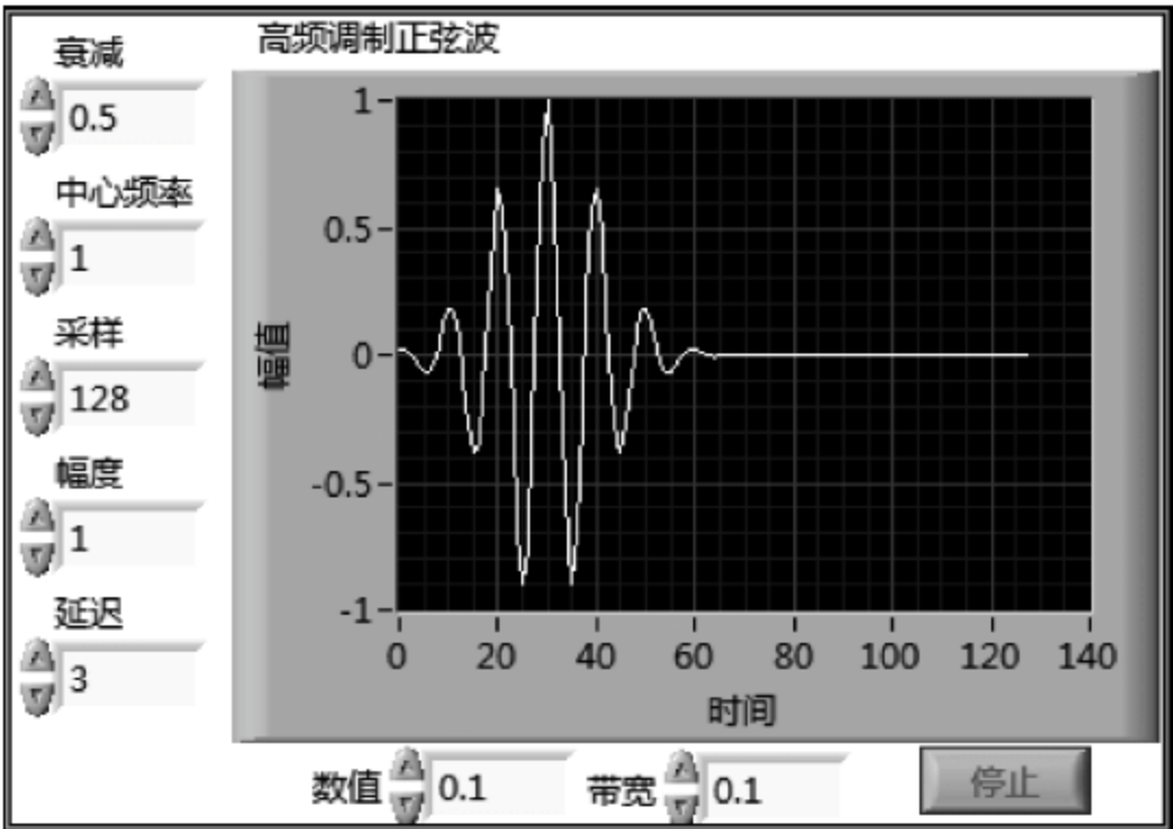
图 7.14 例 7.4 前面板
