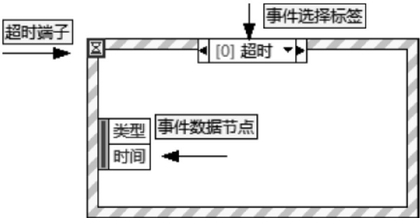
图 4.25 事件结构
