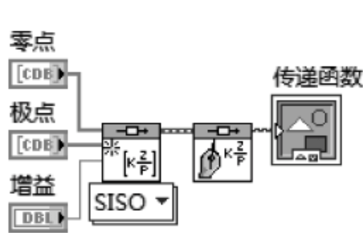
图 9.9 程序框图
