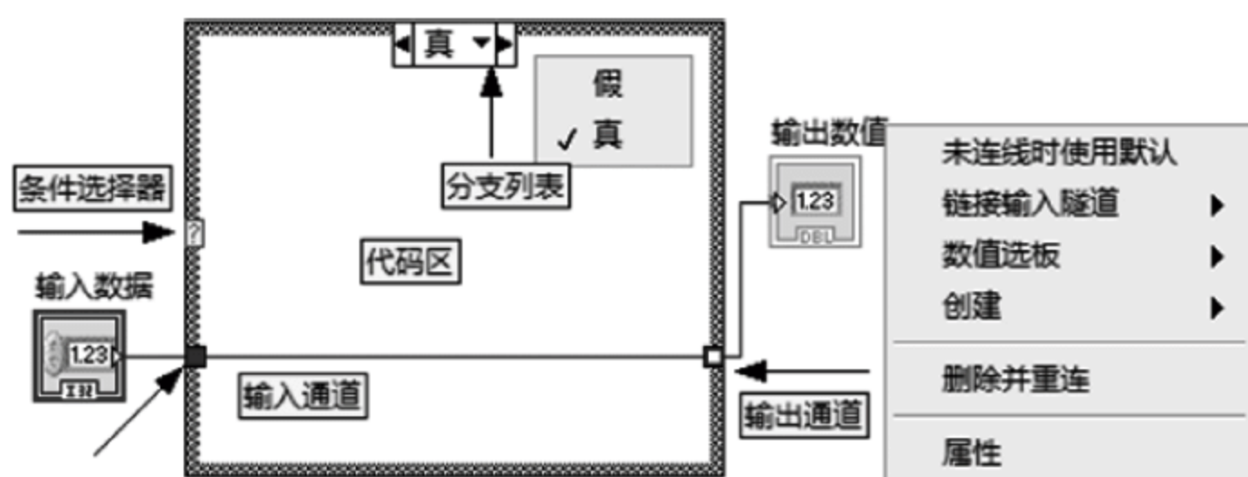
图 4.16 条件结构
