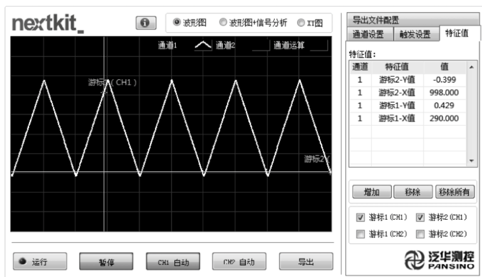
图 12.8 特征值界面
