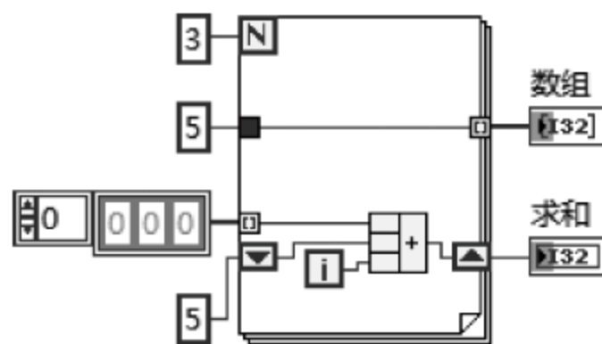
图 4.12 空数组输入
