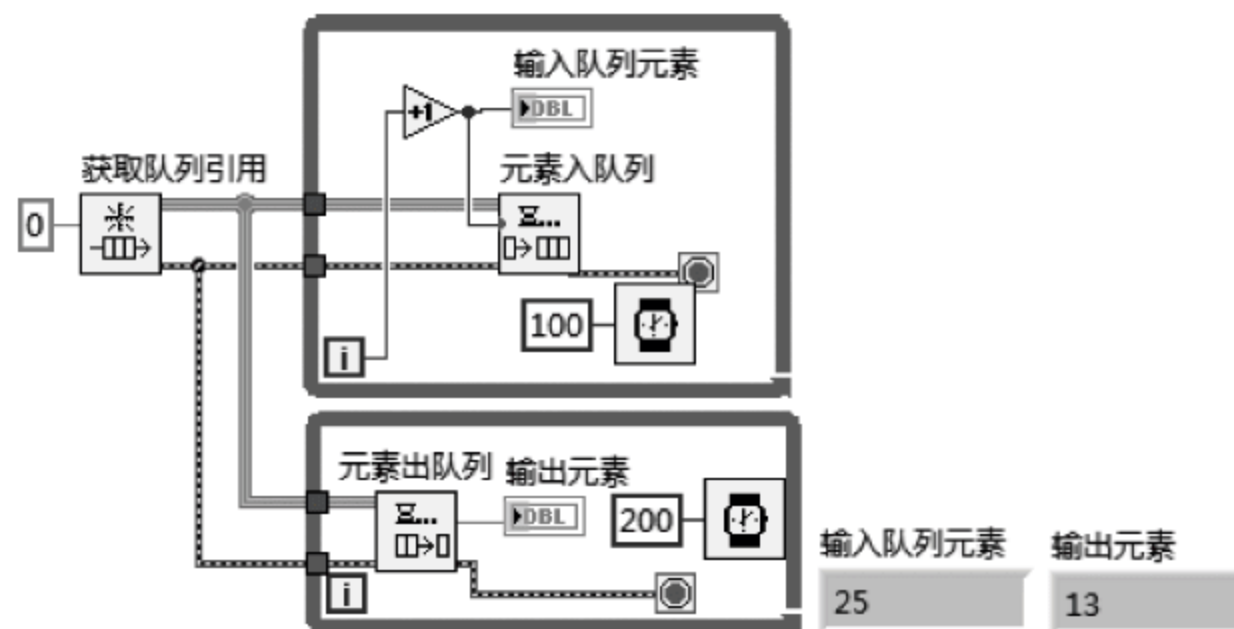
图 6.11 例 6.1 程序框图
