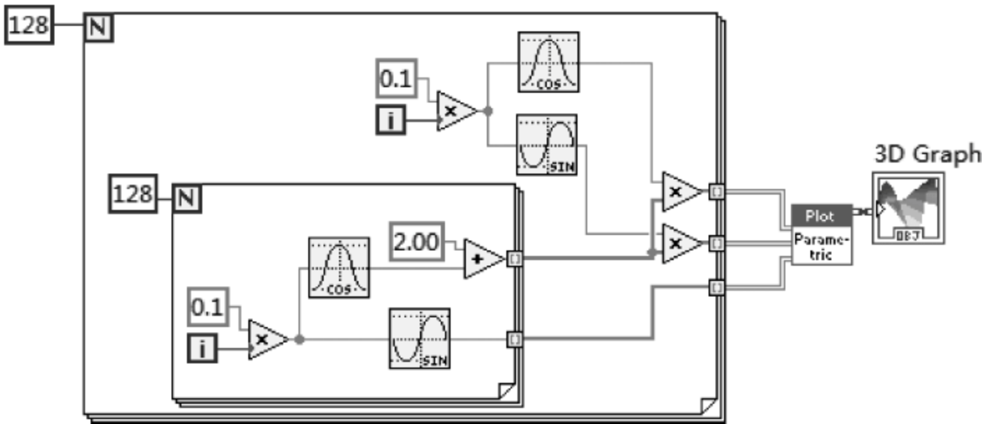
图 5.29 例 5.9 程序框图
