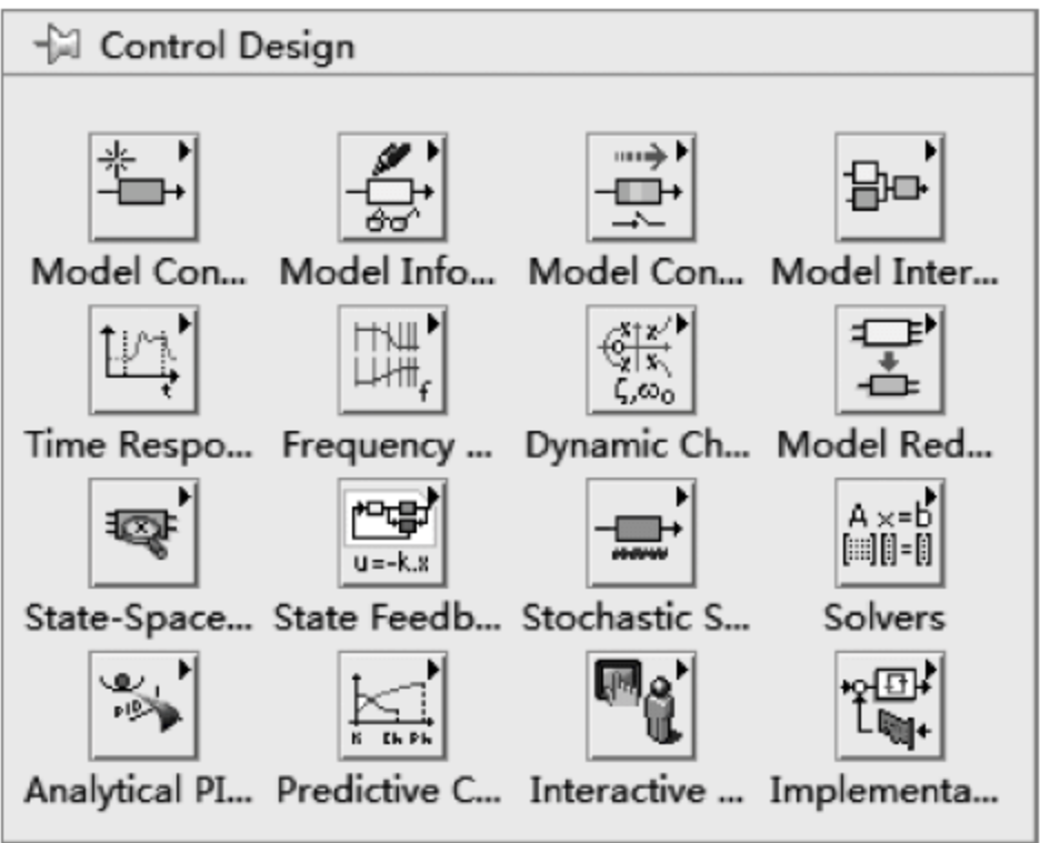
图 9.1 控制模块
