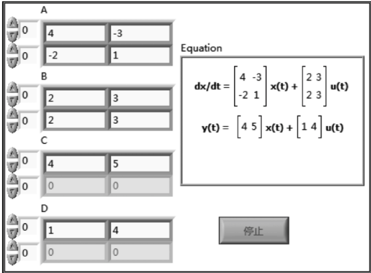
图 9.11 例 9.2 前面板
