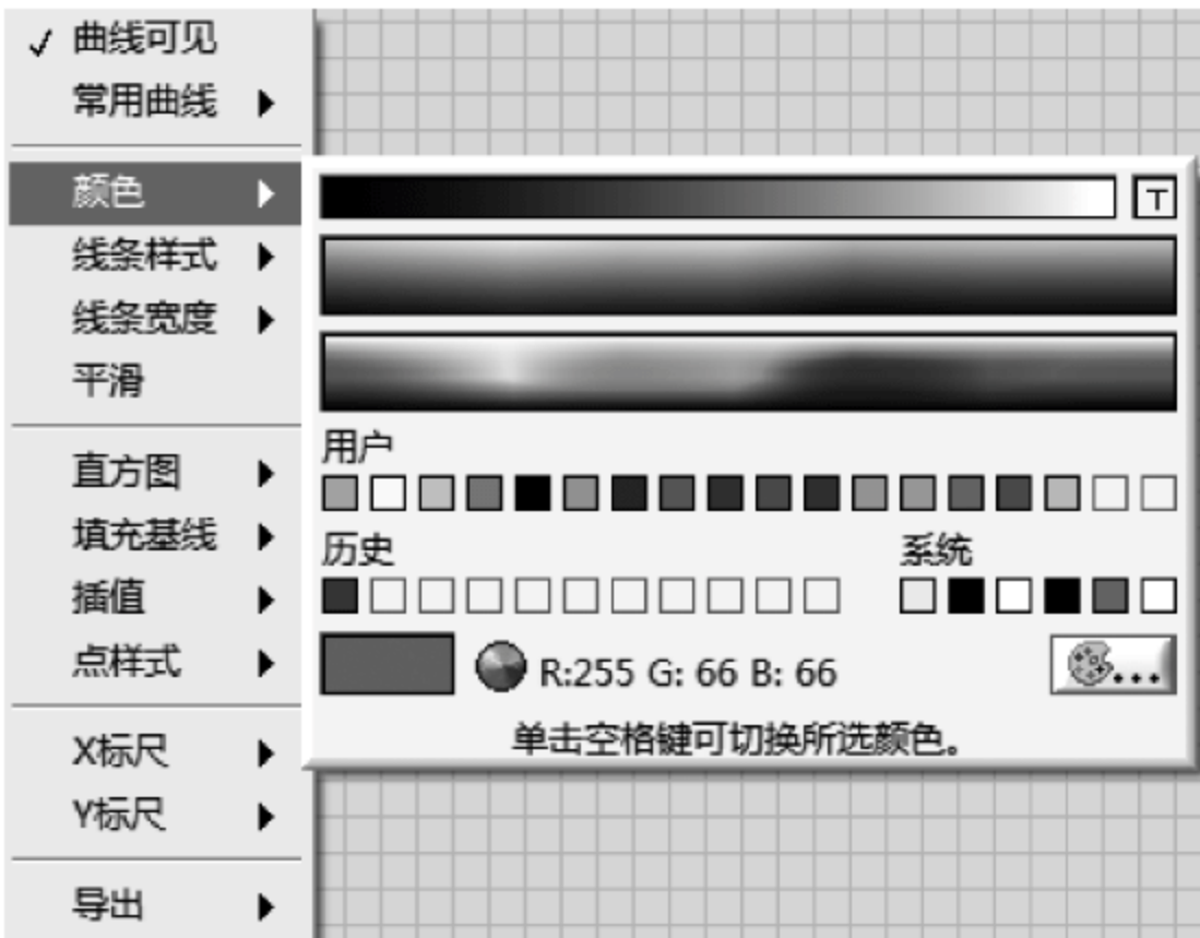
图 5.4 图例对话框
