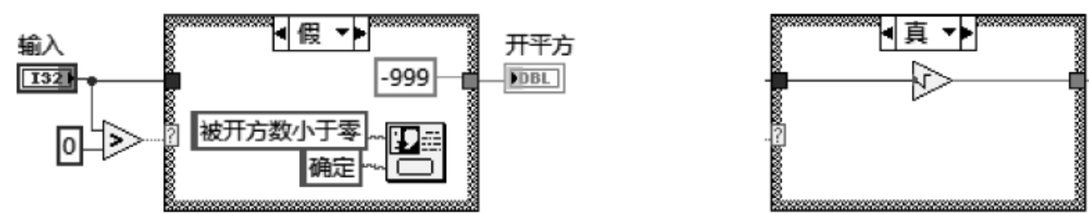
图 4.18 例 4.5 程序框图
