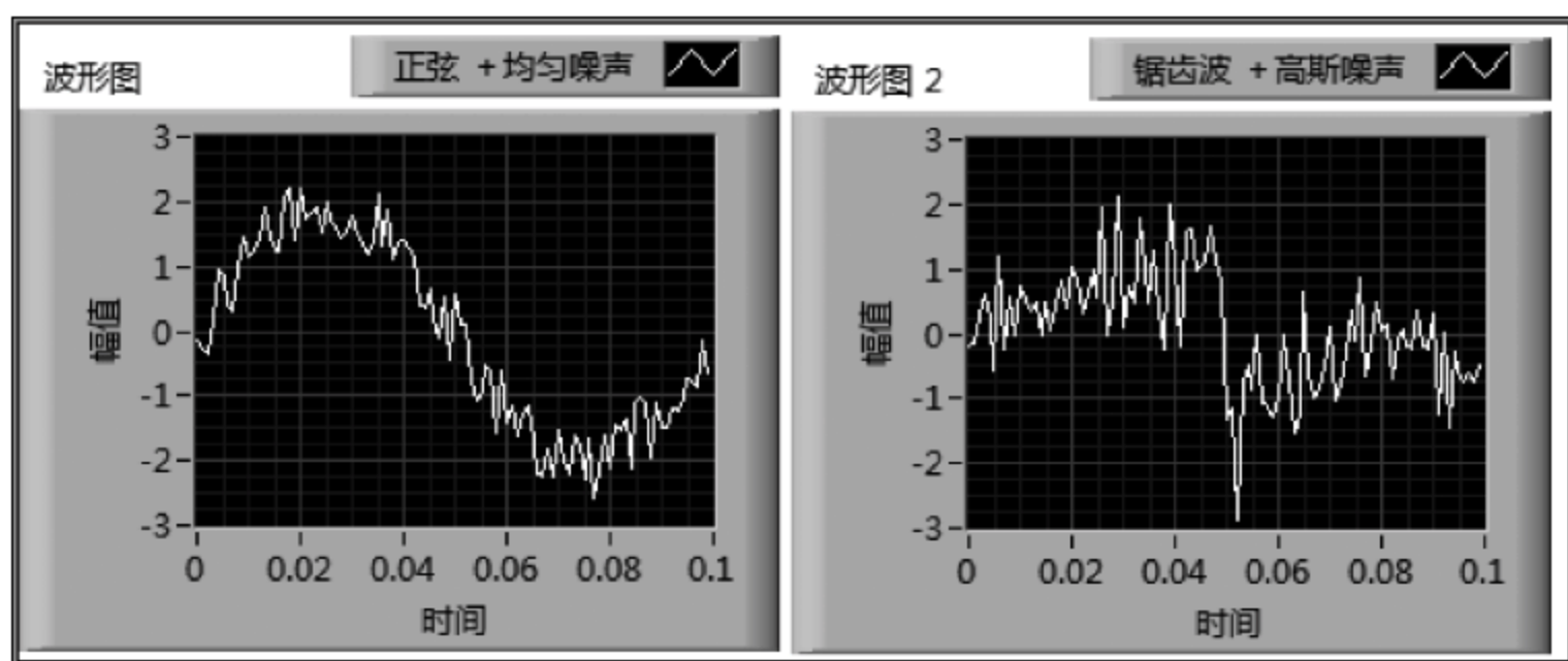
图 7.33 例 7.8 前面板
