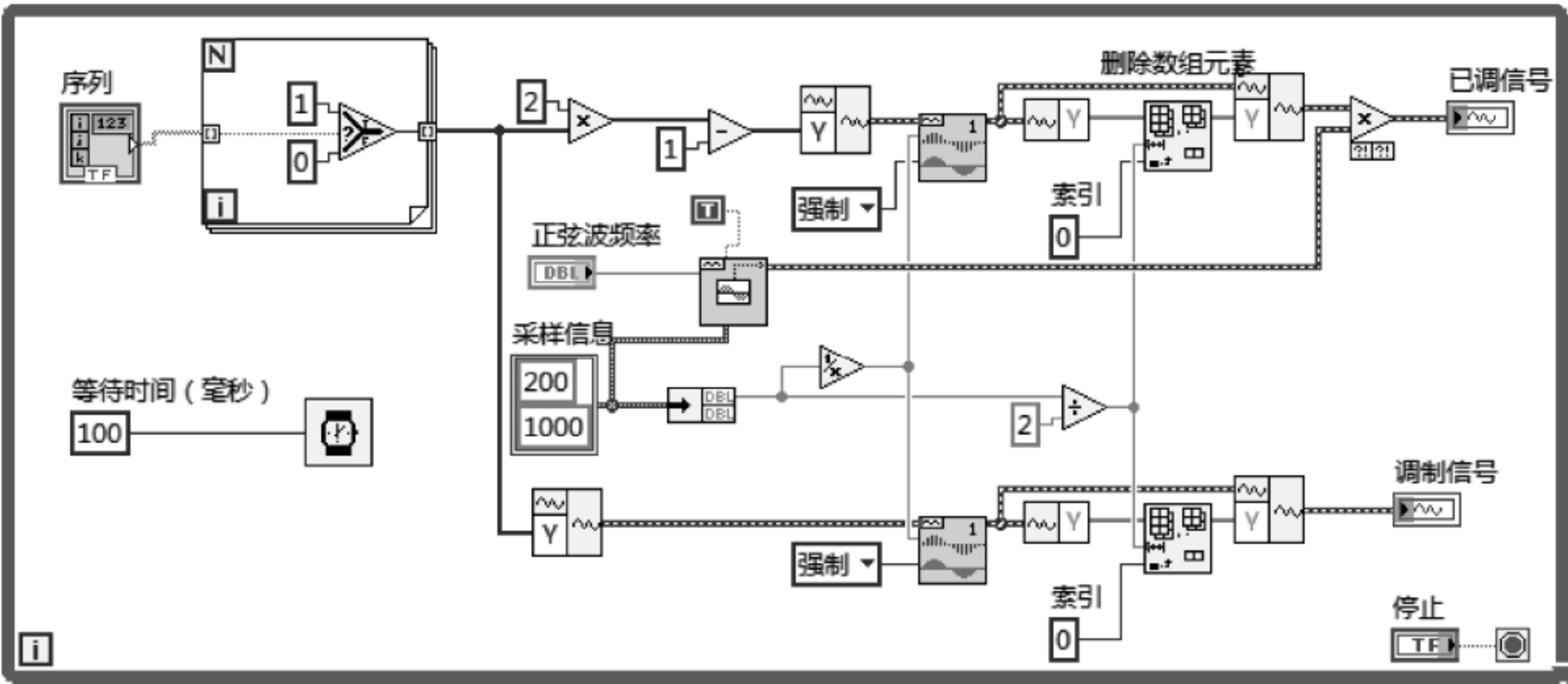
图 8.13 例 8.6 程序框图
