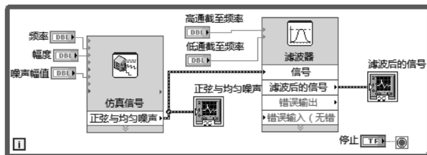
图 7.42 例 7.10 程序框图
