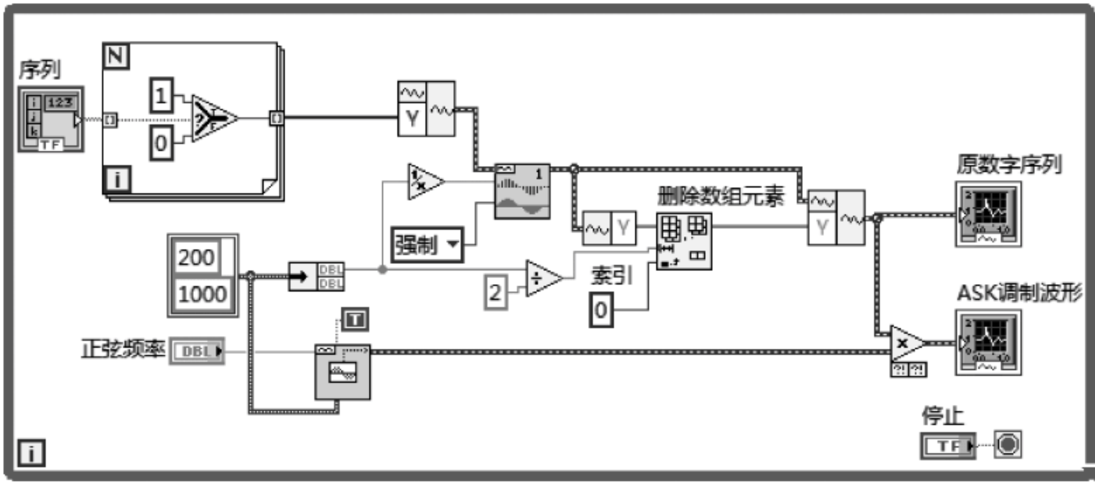
图 8.9 例 8.4 程序框图
