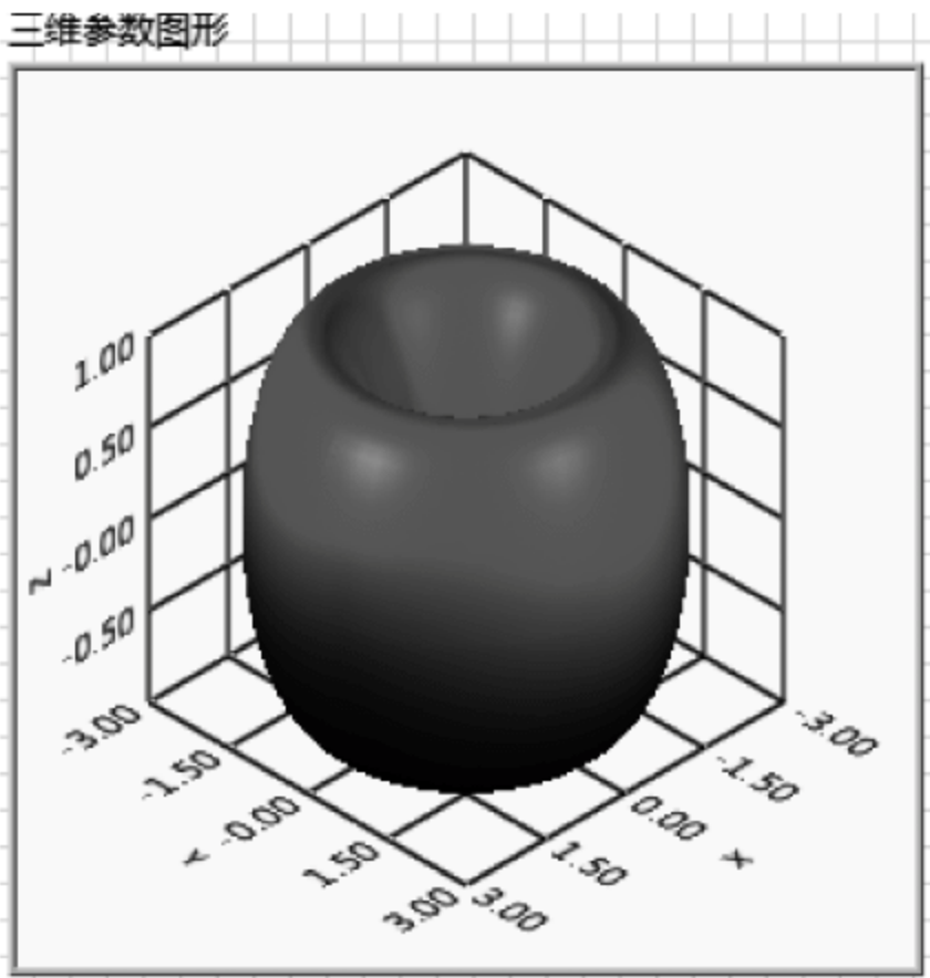
图 5.30 例 5.9 的前面板
