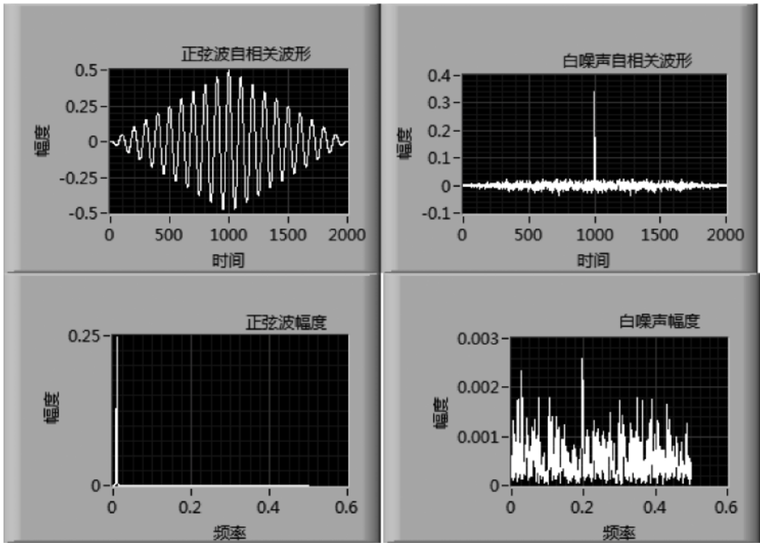
图 7.26 例 7.7 前面板
