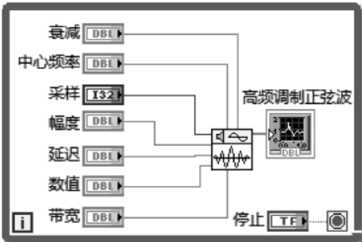
图 7.15 例 7.4 程序框图
