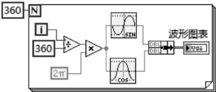
图 5.11 例 5.2 程序框图
