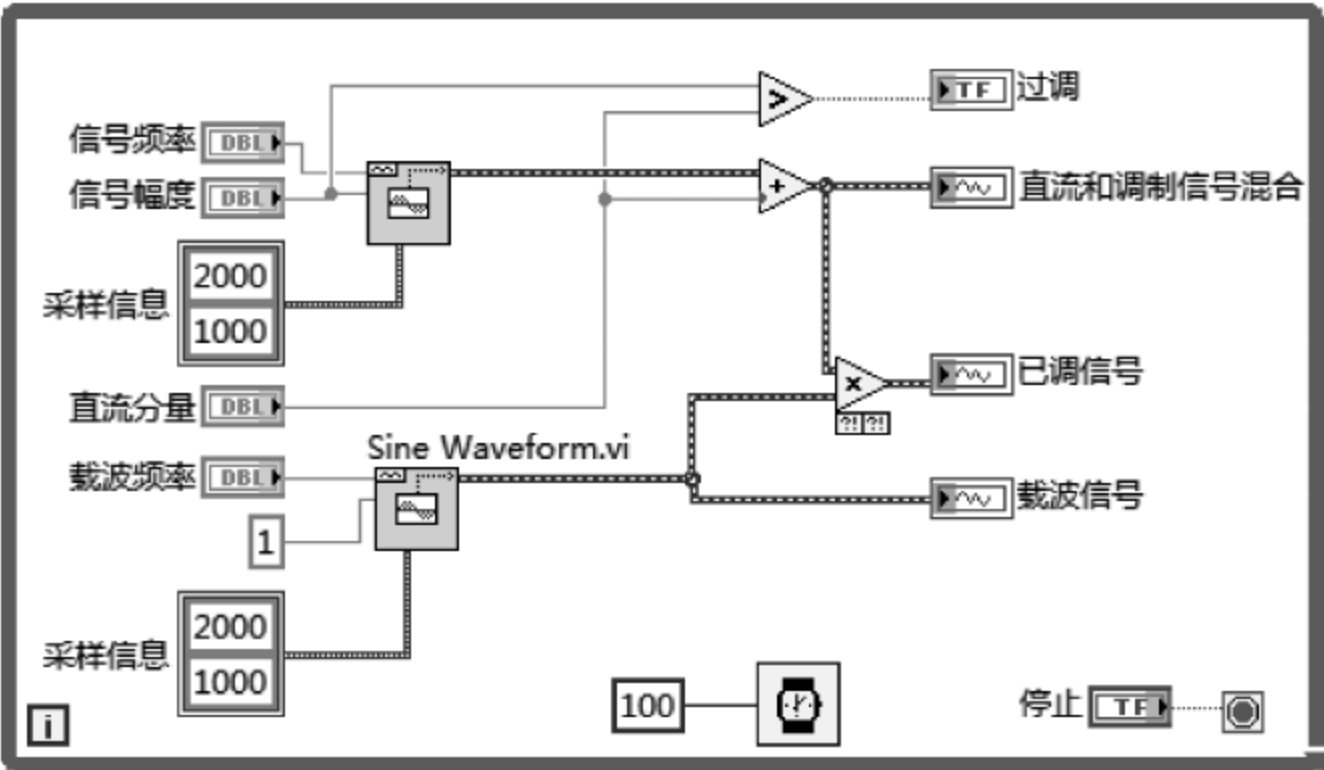
图 8.1 例 8.1 程序框图
