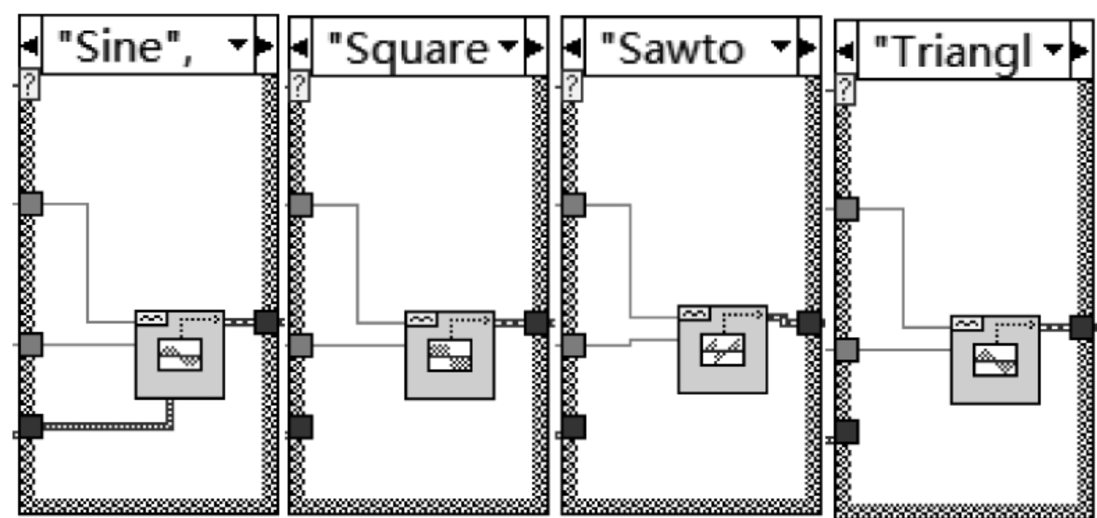
图 13.11 条件结构
