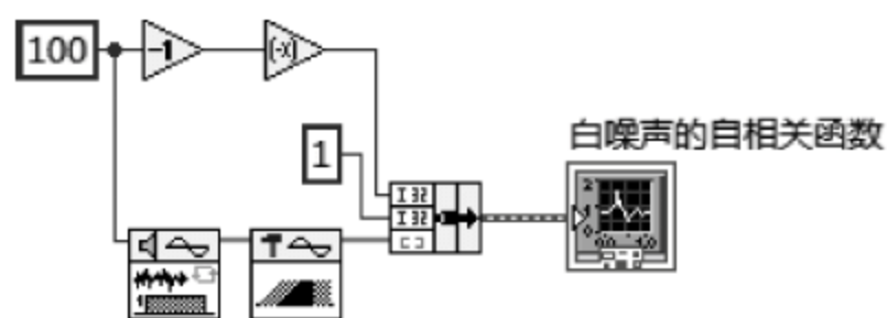
图 7.22 例 7.6 程序框图
