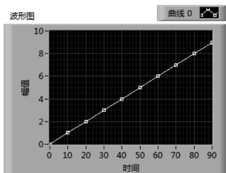
图 5.14 例 5.3 前面板
