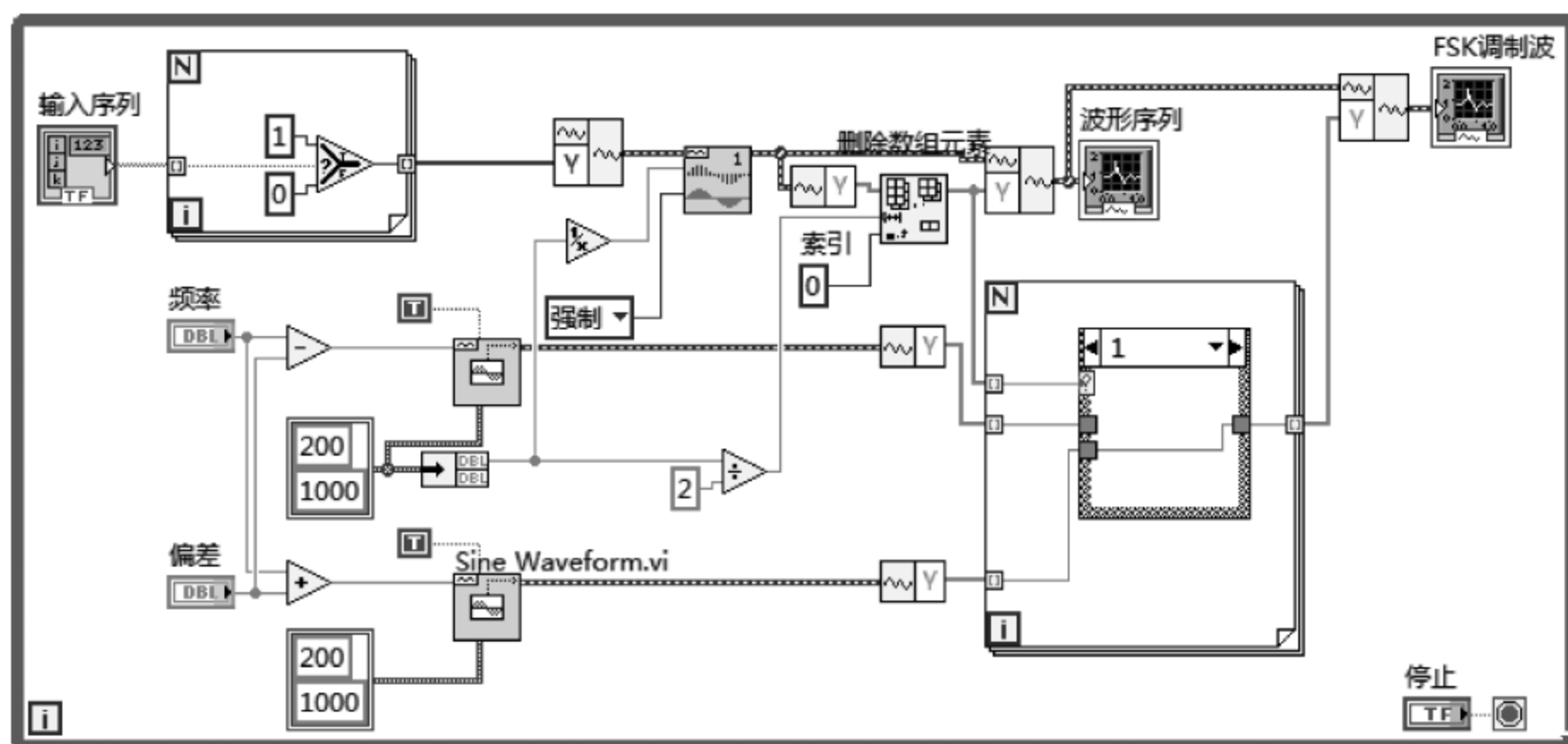
图 8.11 例 8.5 程序框图
