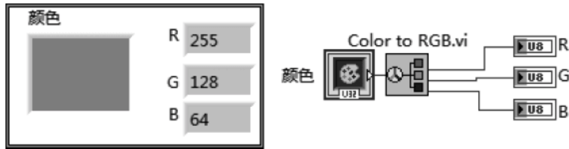
图 4.35 例 4.12 的扩展前面板和程序框图
