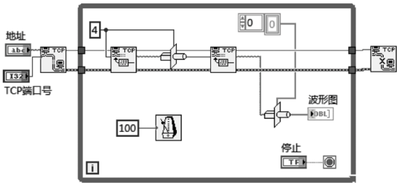
图 6.38 TCP 通信客户机程序框图
