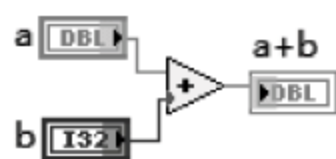
图 3.9 不同数据类型运算结果
