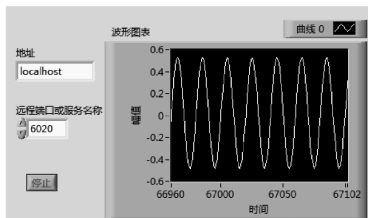
图 12.24 TCP/IP 采集系统接收端前面板调试结果显示
