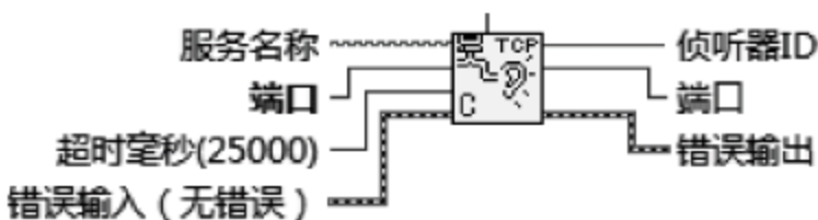
图 6.32 创建 TCP 侦听器节点
