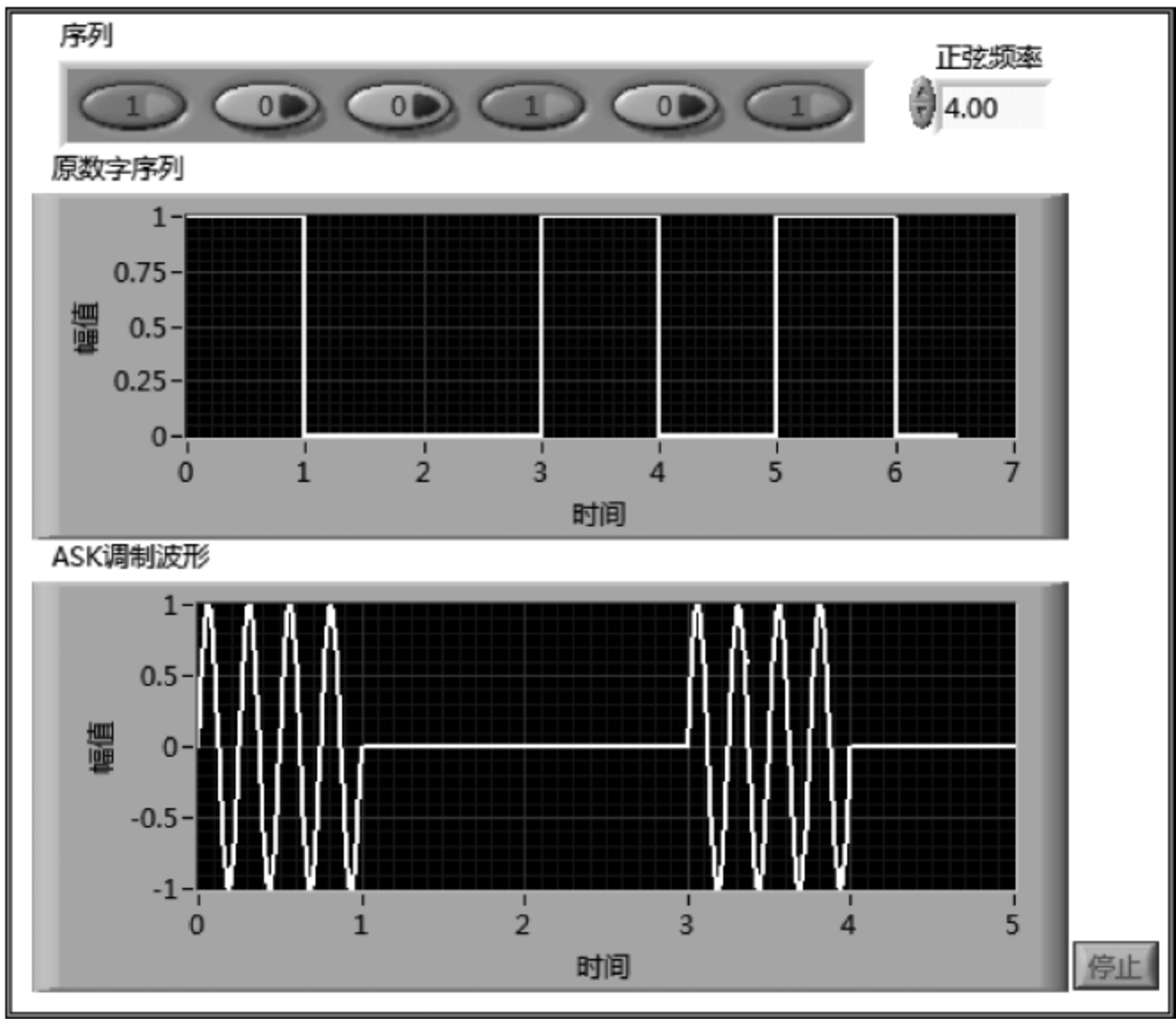
图 8.10 例 8.4 前面板
