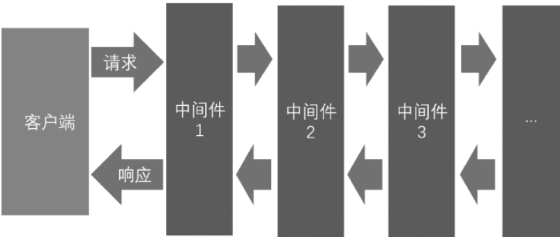
图 15-6 HTTP 通信管道示意图
