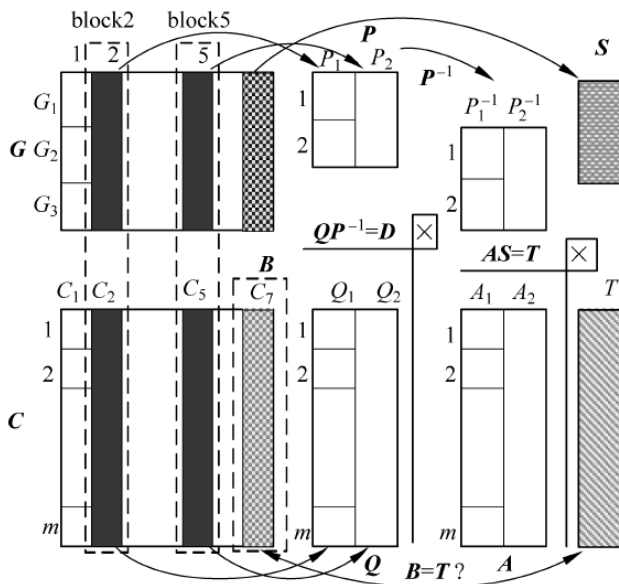
图 8-7 篡改检测原理
