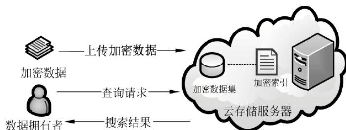
图 6-2 非共享模型
