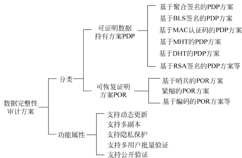
图 7-3 完整性审计方案分类
