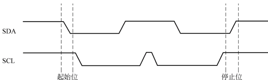
图 10-5 起始/停止时序
