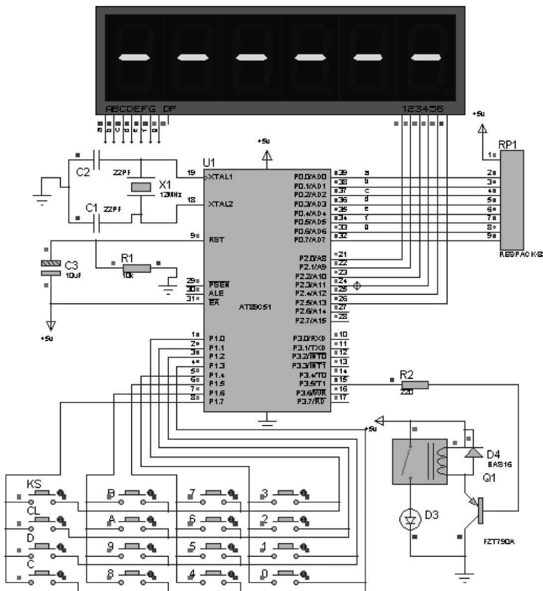
图 6-14 密码锁仿真模型
