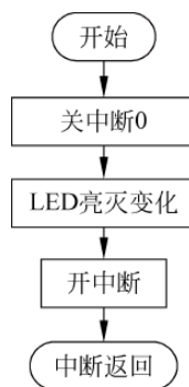
图 2-15 中断服务程序流程
