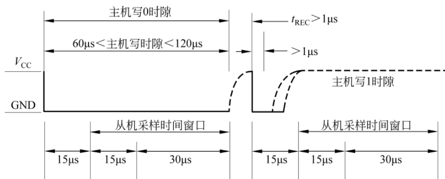
图 12-2 单总线通信协议的写时序
