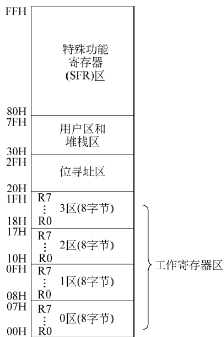
图 1-3 片内 RAM 的配置
