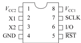
图 11-1 DS1302 引脚分布
