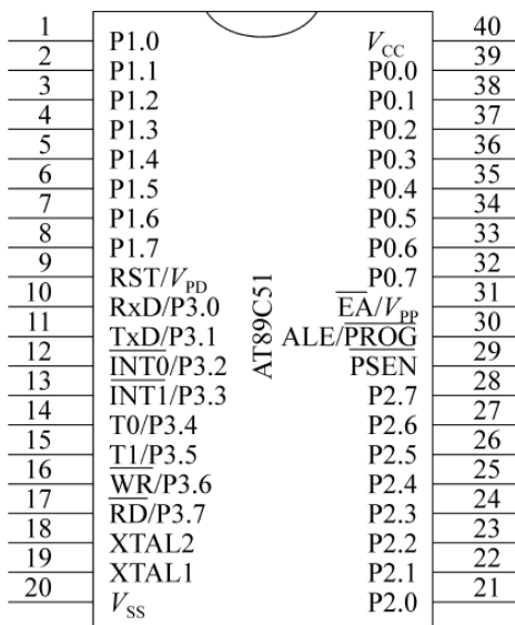
图 1-1 AT89C51 单片机引脚
