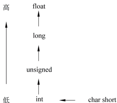
图 1-39 数据类型转换规则
