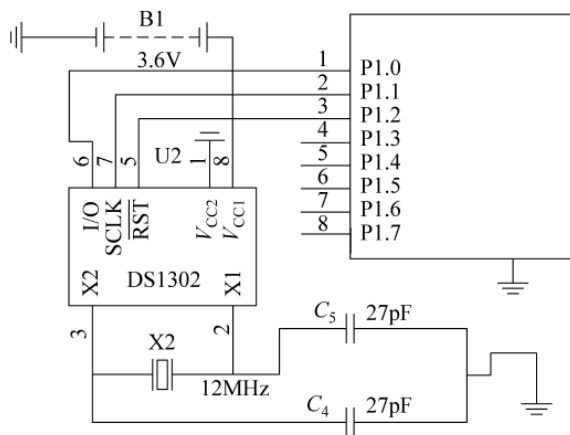
图 11-3 DS1302 与单片机连接
