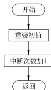
图 4-6 中断服务程序流程
