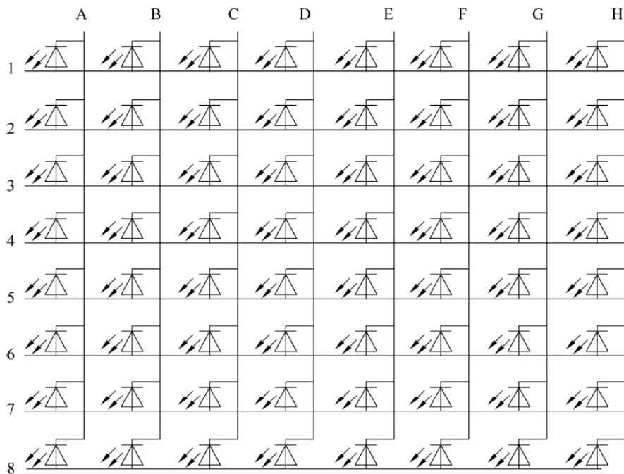
图 2-4 点阵结构图
