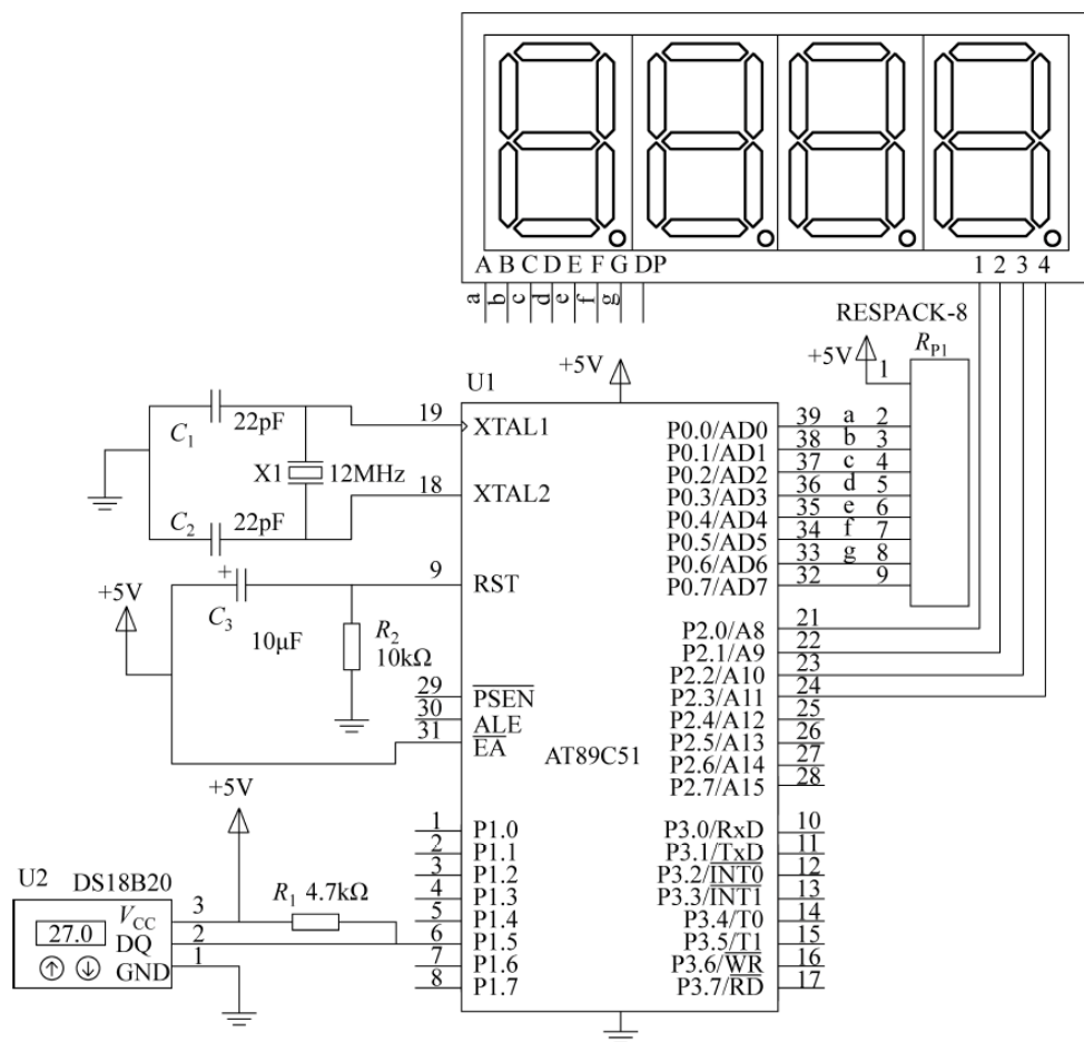
图 12-12 数字温度计硬件电路
