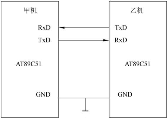
图 9-15 双机异步通信接口电路
