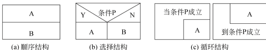
图 1-40 C51 程序基本结构
