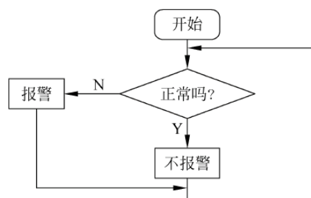
图 1-47 报警主程序流程
