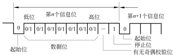
图 9-6 RS-232C 信息格式
