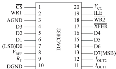
图 8-1 DAC0832 引脚
