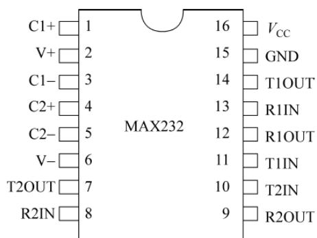
图 9-7 MAX232 引脚
