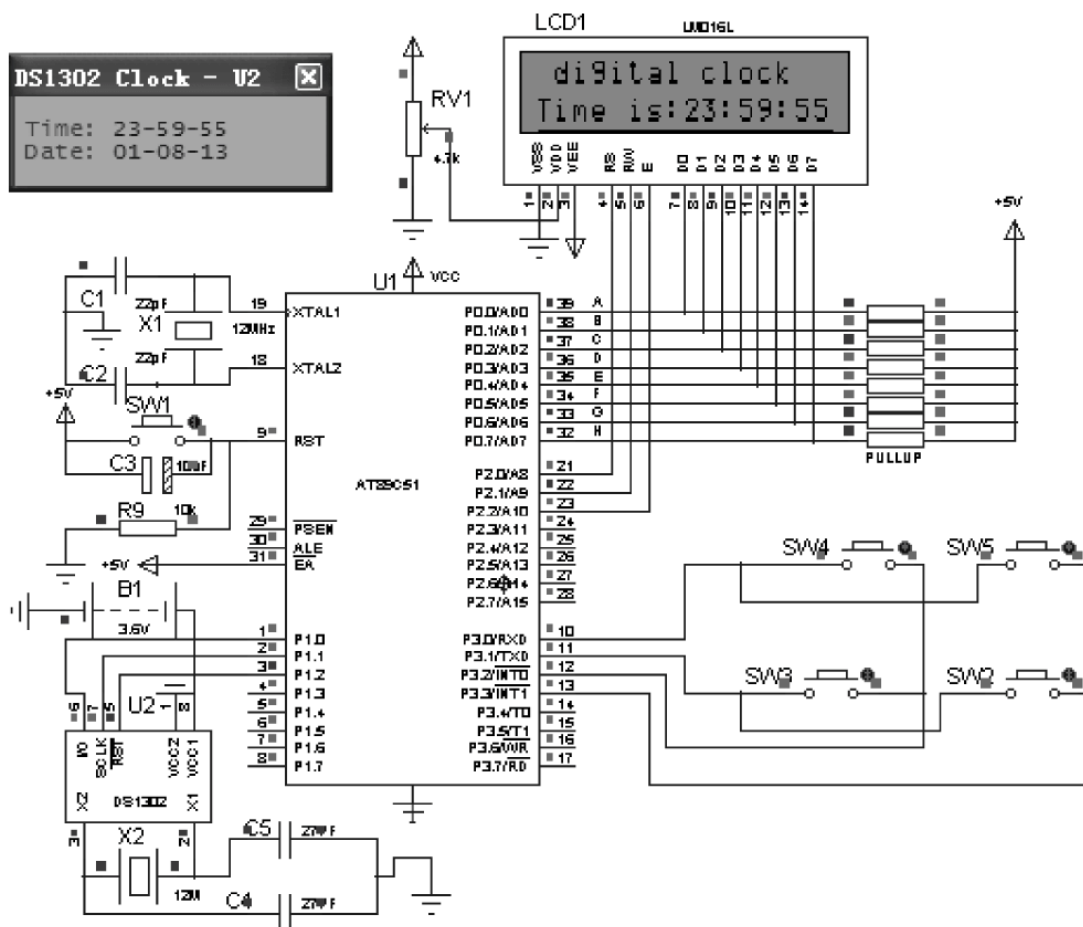
图 11-9 数字钟仿真模型
