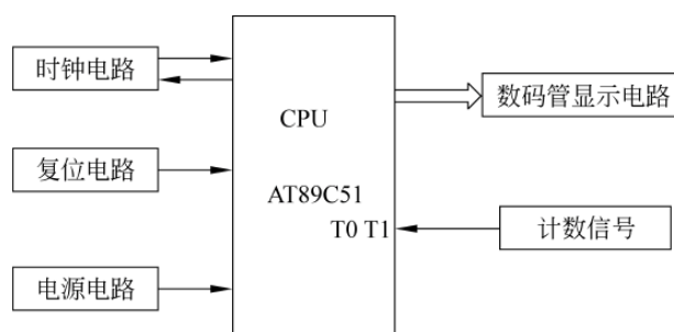
图 3-6 啤酒生产计数器总体框图
