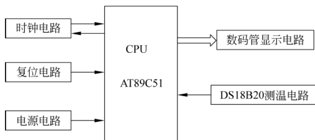
图 12-11 数字温度计总体框图
