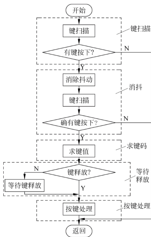
图 6-4 矩阵式键盘的控制流程
