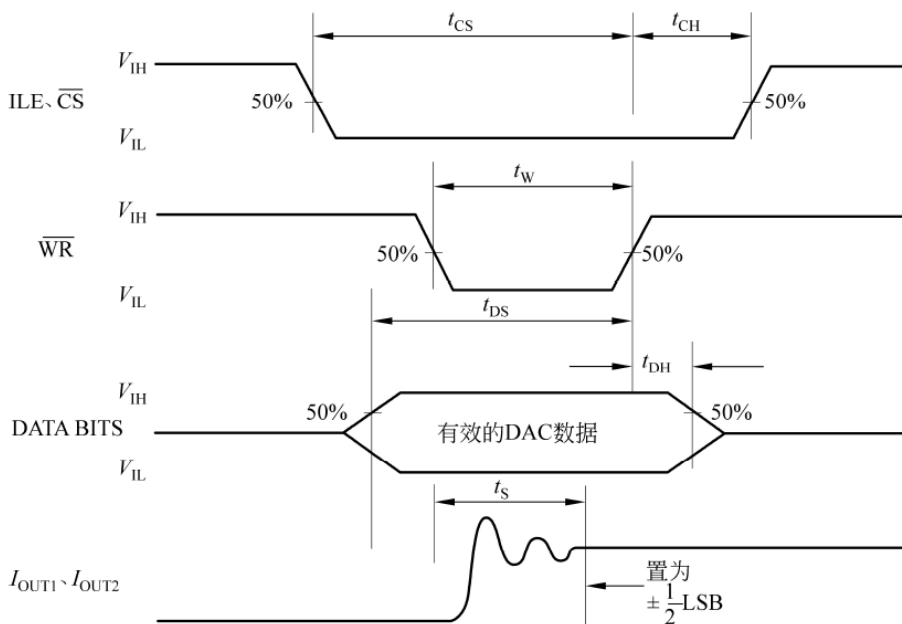
图 8-5 DAC0832 操作时序
