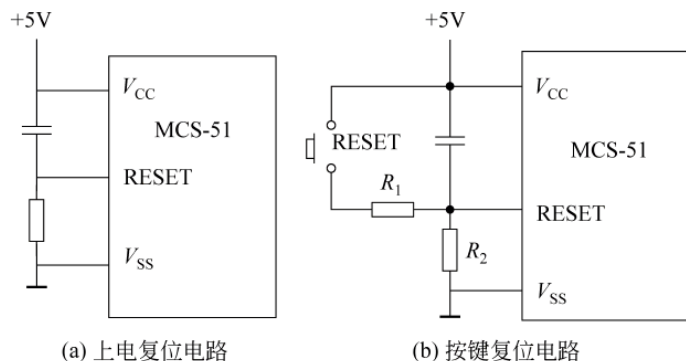
图 1-10 单片机常见的复位电路
