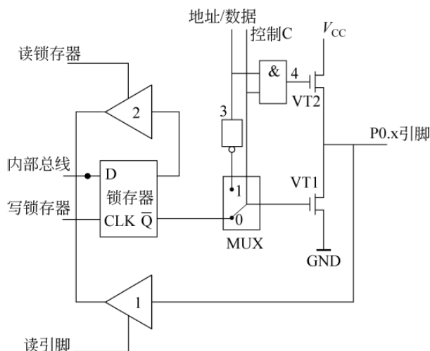
图 1-5 P0 口的一位结构图
