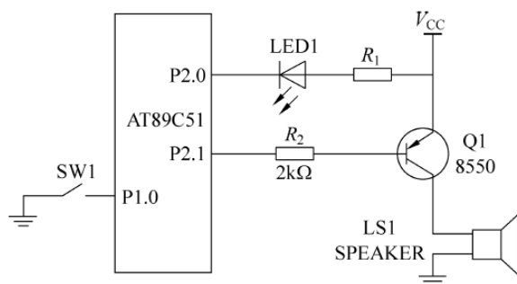
图 1-46 声光报警电路
