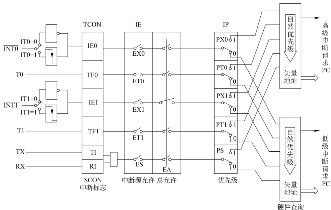
图 2-11 MCS-51 中断系统内部结构示意图
