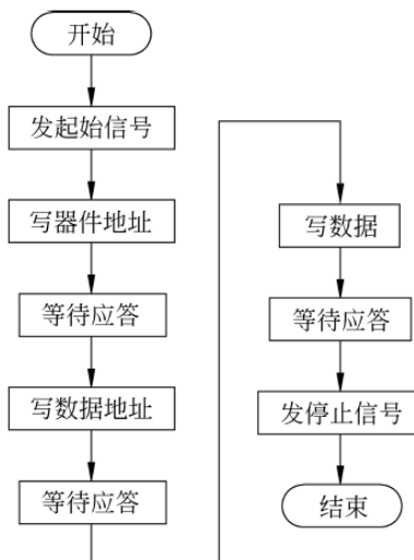
图 10-7 写 1 字节数据的程序流程
