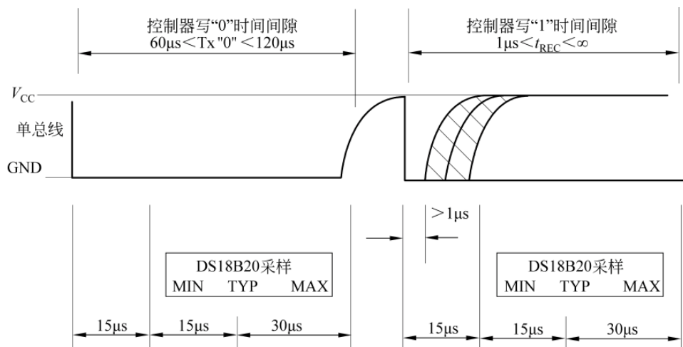
图 12-9 写时序
