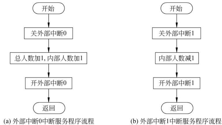
图 2-18 中断服务程序流程
