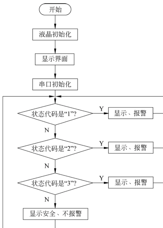
图 9-25 主机主程序流程
