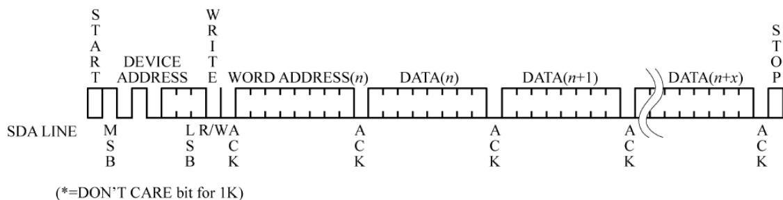
图 10-8 页写流程
