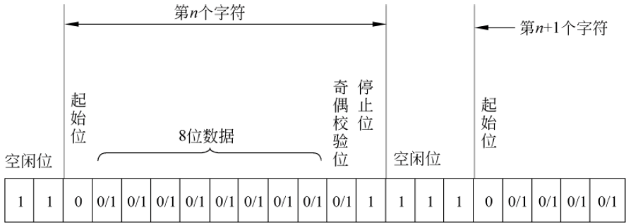
图 9-3 异步通信数据帧格式
