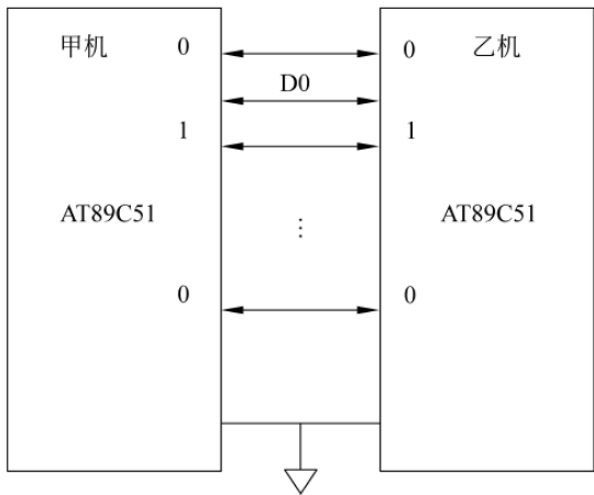
图 9-1 并行通信
