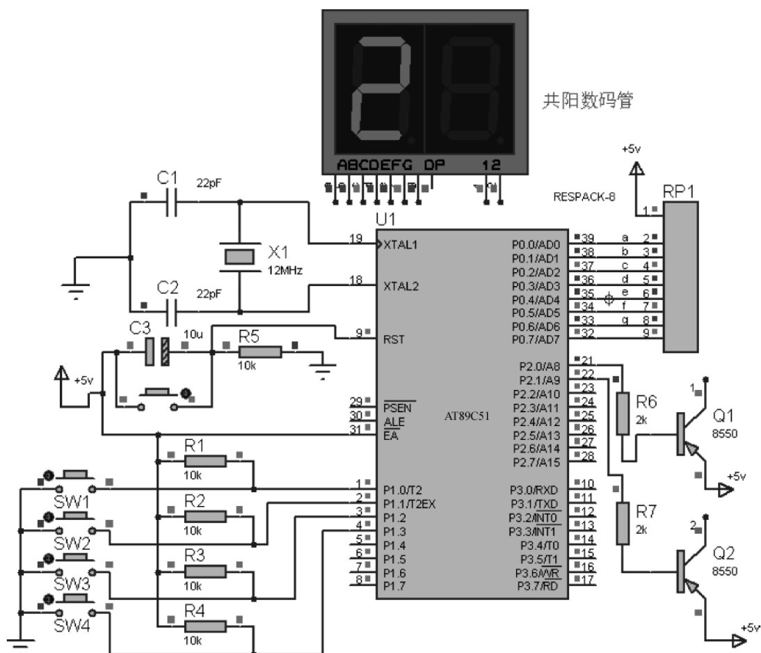
图 5-14 四路抢答器仿真模型
