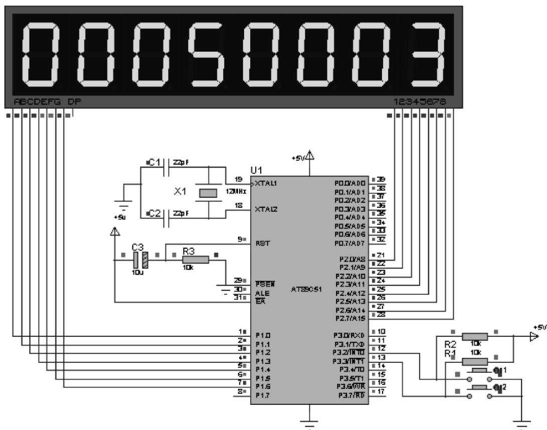
图 2-20 游客流量人数计数器仿真模型
