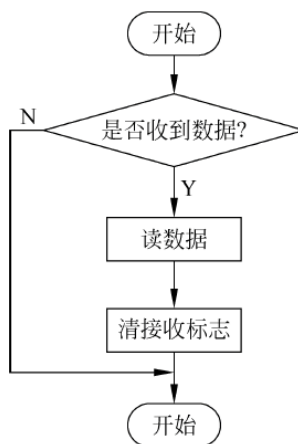
图 9-19 中断服务程序流程
