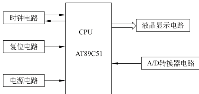
图 7-10 数字电压表总体框图
