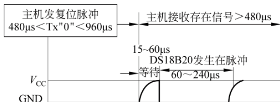
图 12-8 复位操作时序
