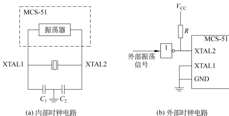
图 1-9 时钟电路
