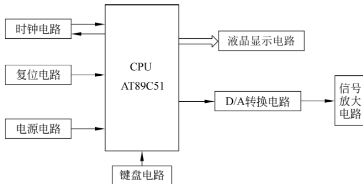
图 8-11 正弦信号发生器总体框图
