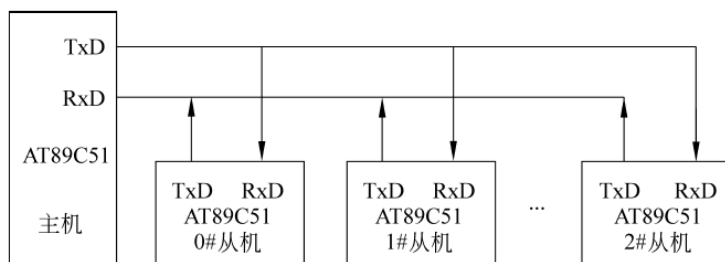
图 9-16 多机通信连接示意图
