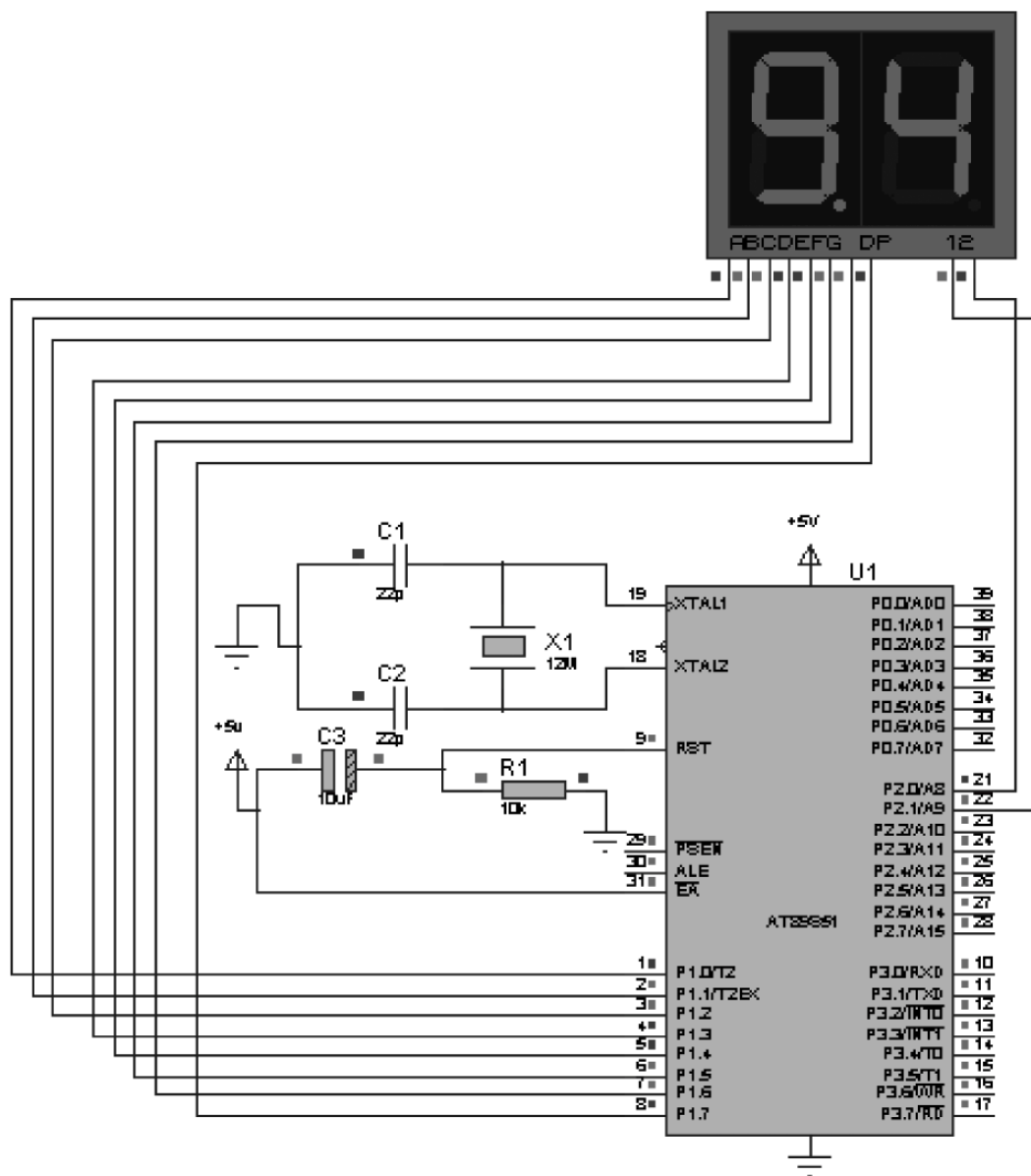
图 4-7 9.9 秒表仿真模型
