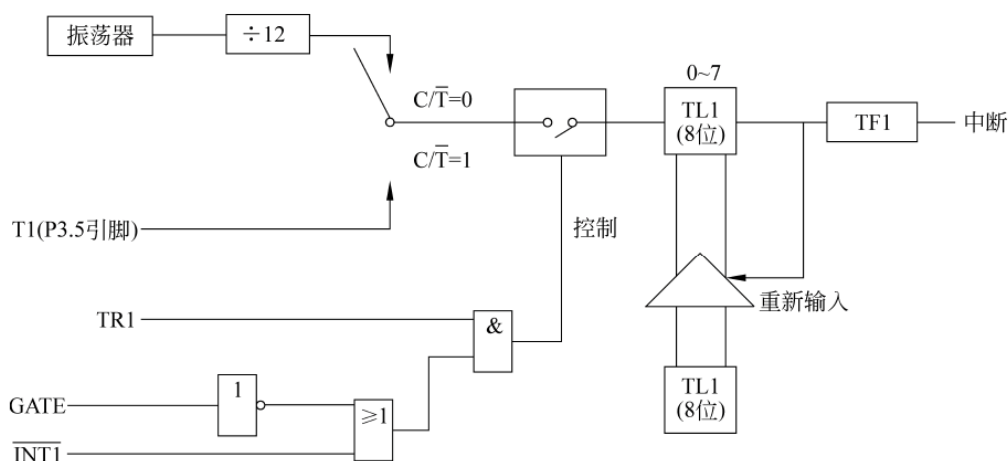
图 3-3 方式 2 时的逻辑结构
