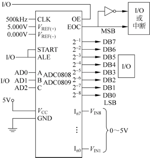
图 7-8 ADC0809 与单片机硬件连接
