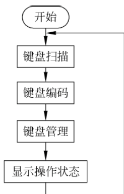
图 6-12 密码锁主程序流程
