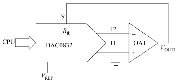
图 8-3 DAC0832 单极性电压输出连接
