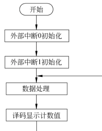
图 2-19 主程序流程
