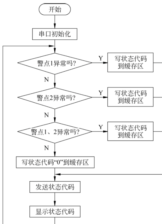
图 9-27 从机主程序流程
