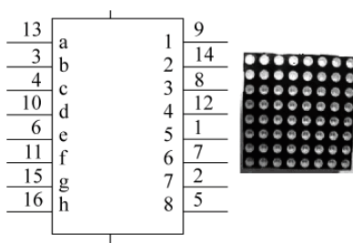
图 2-5 点阵引脚及实物图
