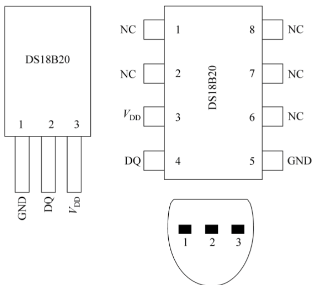
图 12-4 DS18B20 的外观及引脚排列
