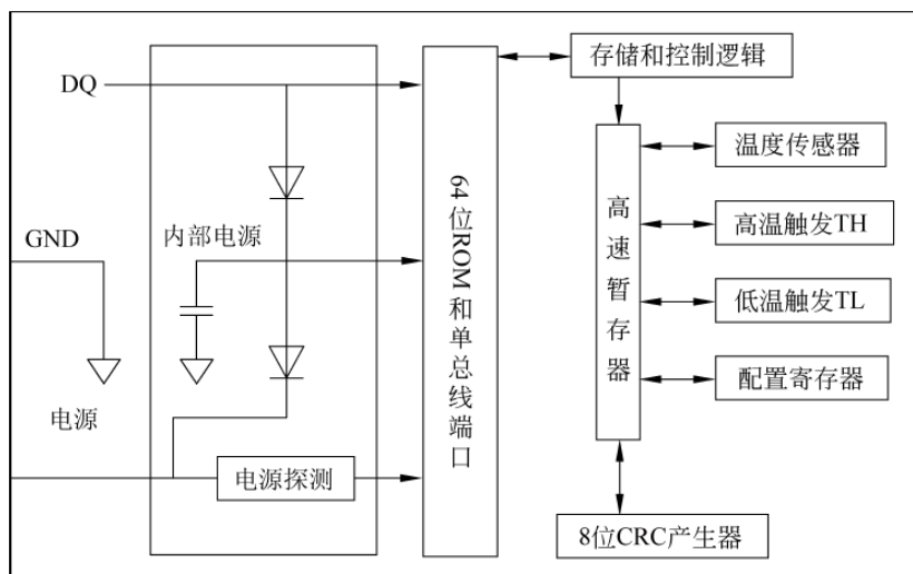
图 12-5 DS18B20 的内部结构
