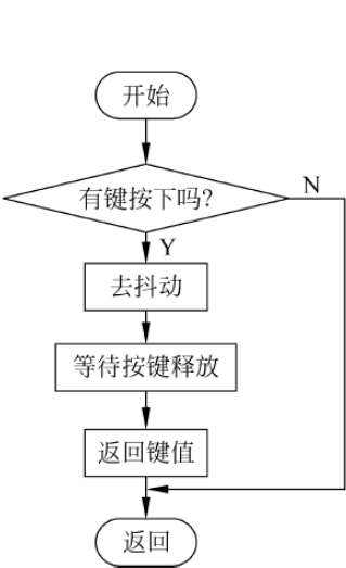
图 5-11 键盘扫描程序流程
