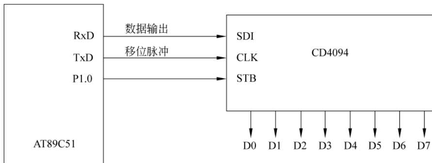
图 9-11 方式 0 扩展 I/O 口输出
