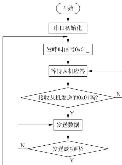
图 9-20 主机通信程序流程
