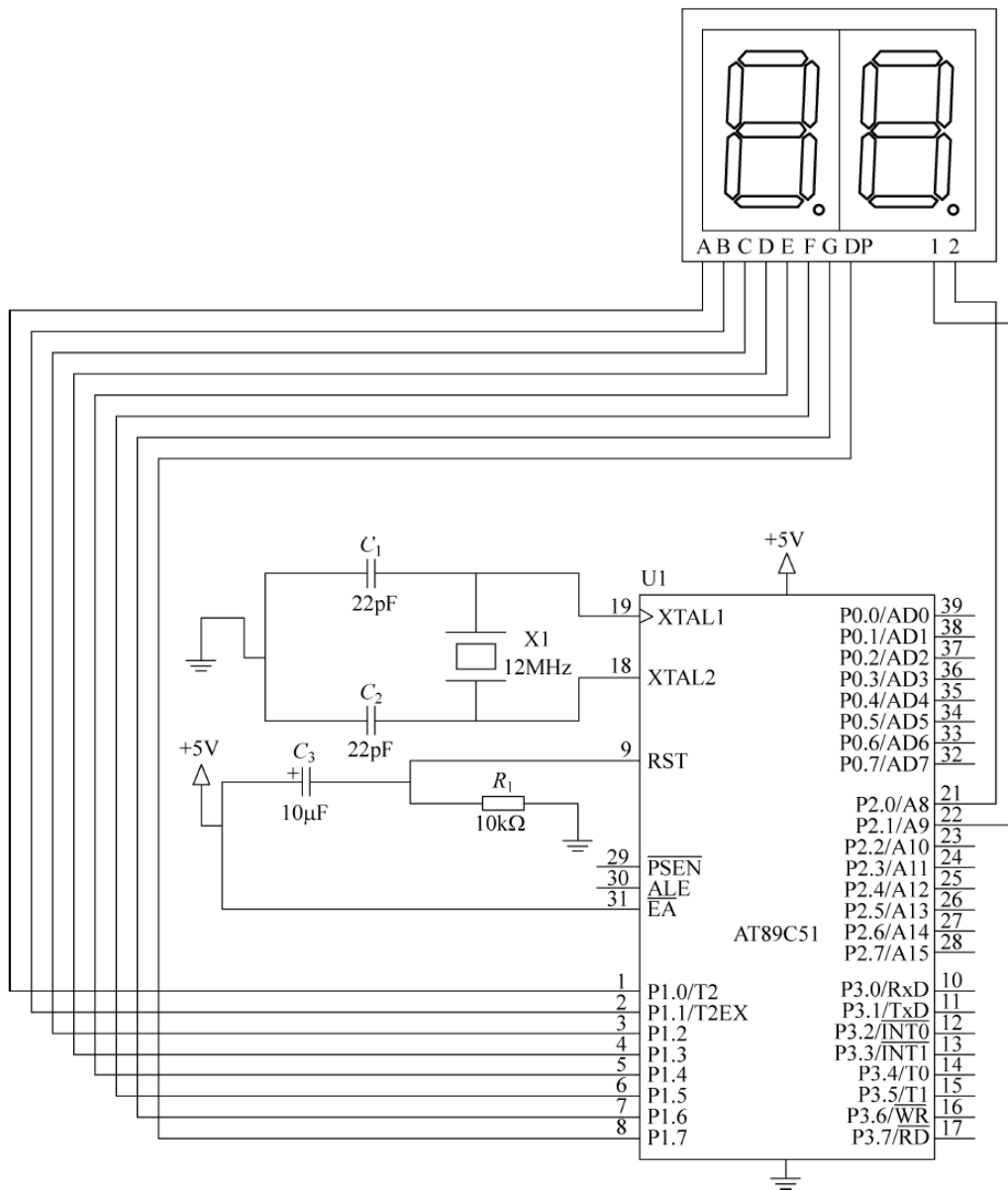
图 4-4 9.9 秒表参考电路
