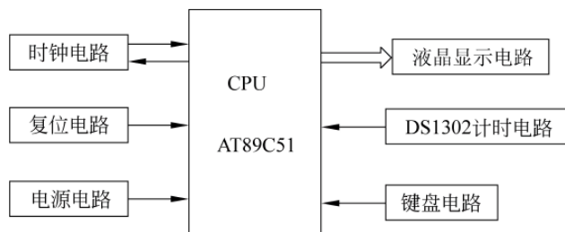
图 11-6 数字钟总体框图
