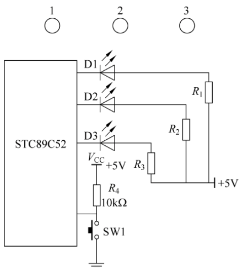
图 5-15 按键控制组合灯电路
