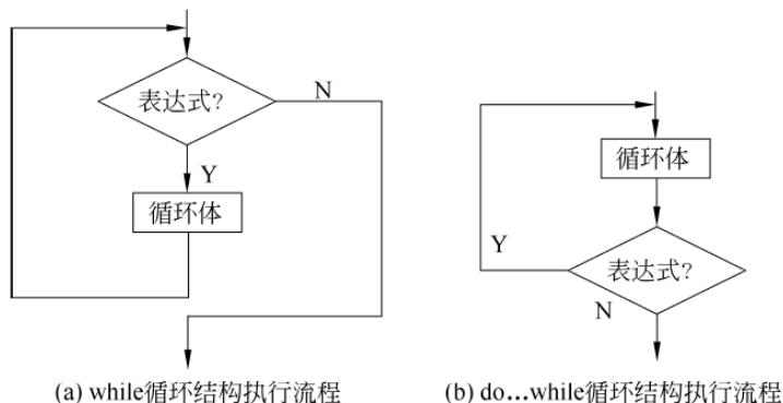
图 1-44 while、do...while 执行流程
