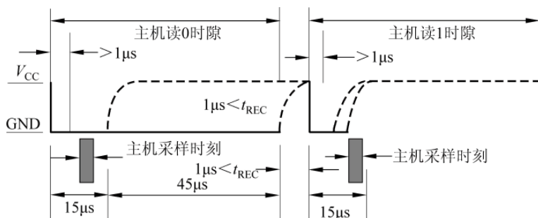
图 12-3 读时序
