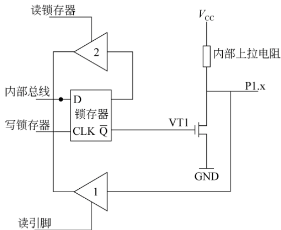
图 1-6 P1 口的一位结构图
