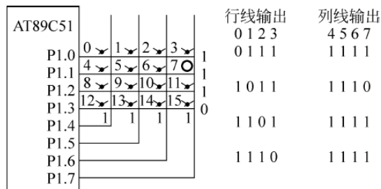
图 6-2 逐行扫描法
