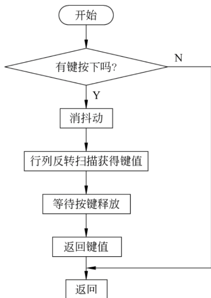
图 6-5 4 \times 4 矩阵式键盘扫描程序流程
