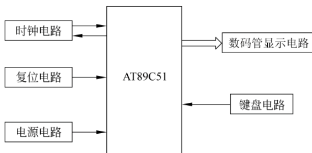
图 5-9 总体框图
