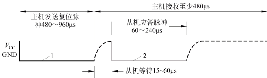
图 12-1 单总线协议的初始化时序
