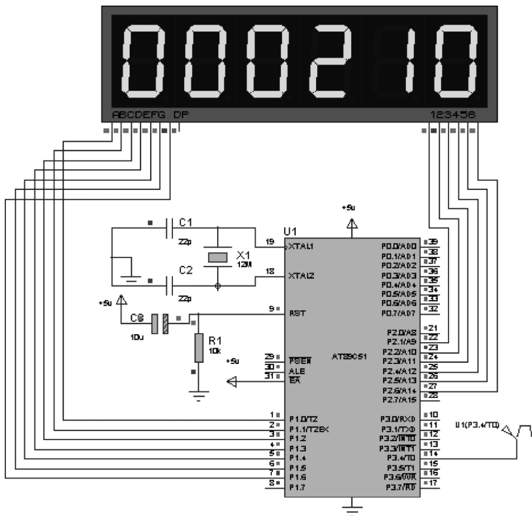
图 3-10 啤酒生产计数器仿真模型
