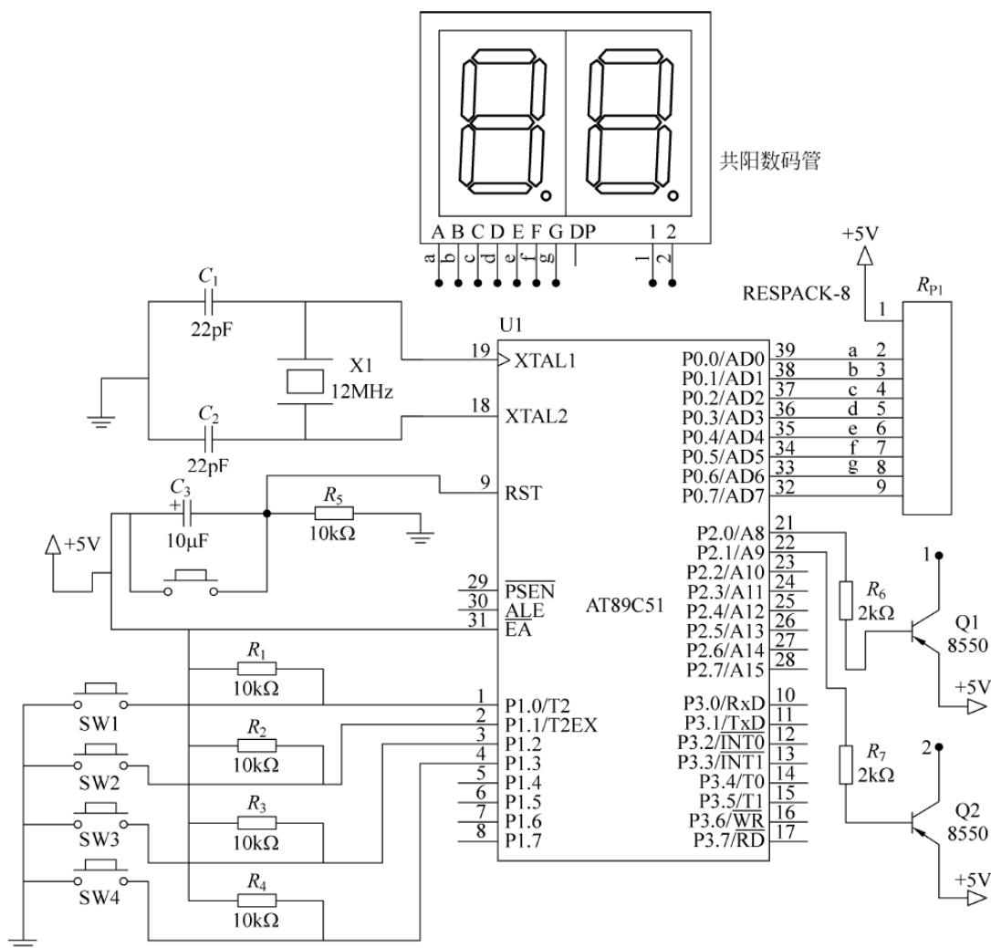
图 5-10 四路抢答器参考电路
