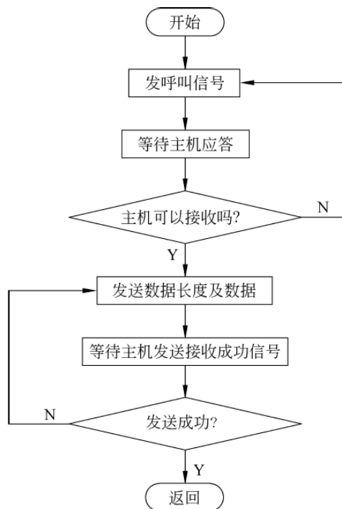
图 9-28 从机发送状态信息流程
