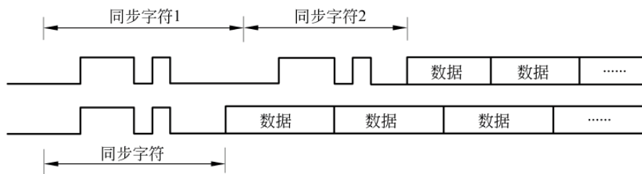
图 9-4 同步传送格式
