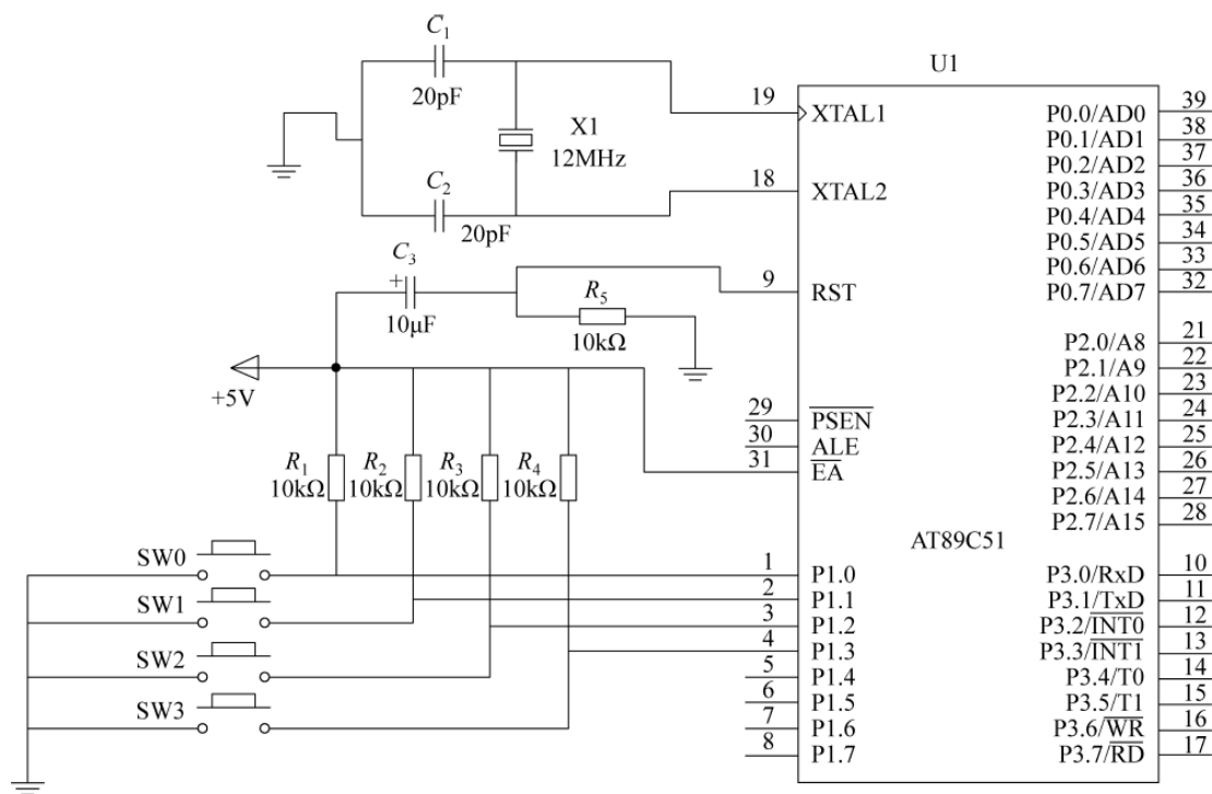
图 5-3 独立式键盘结构
