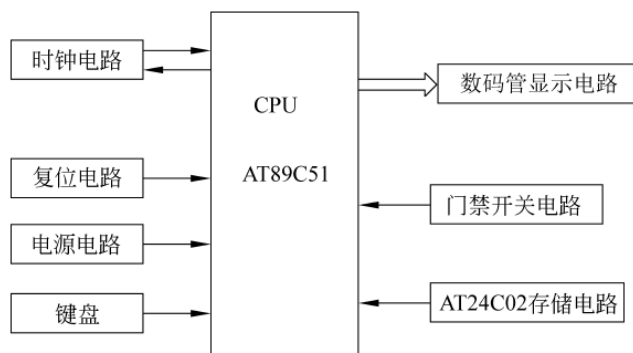
图 6-10 密码锁总体框图
