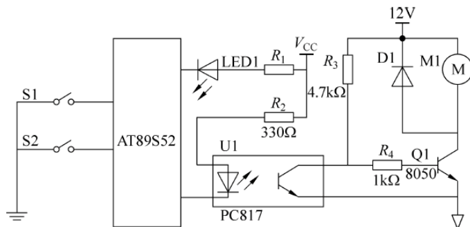
图 5-16 电机运行控制电路
