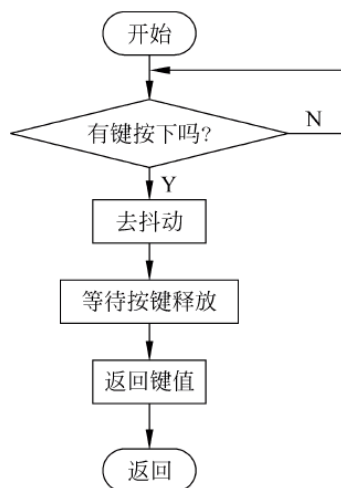
图 5-6 键盘扫描程序流程
