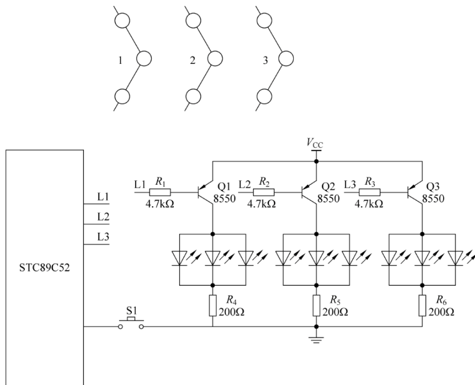
图 1-58 交通方向指示灯电路
