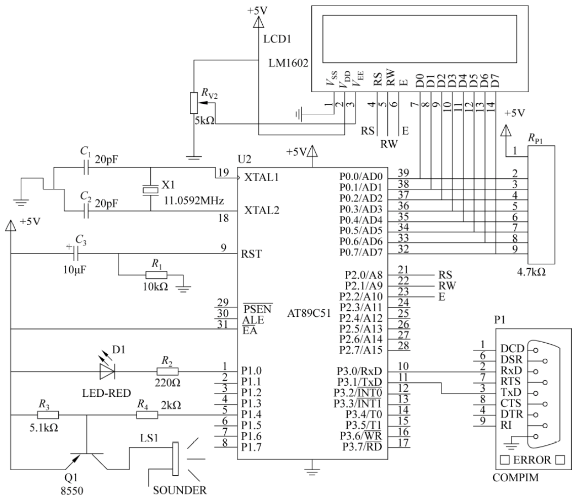
图 9-23 远程报警器主机硬件电路
