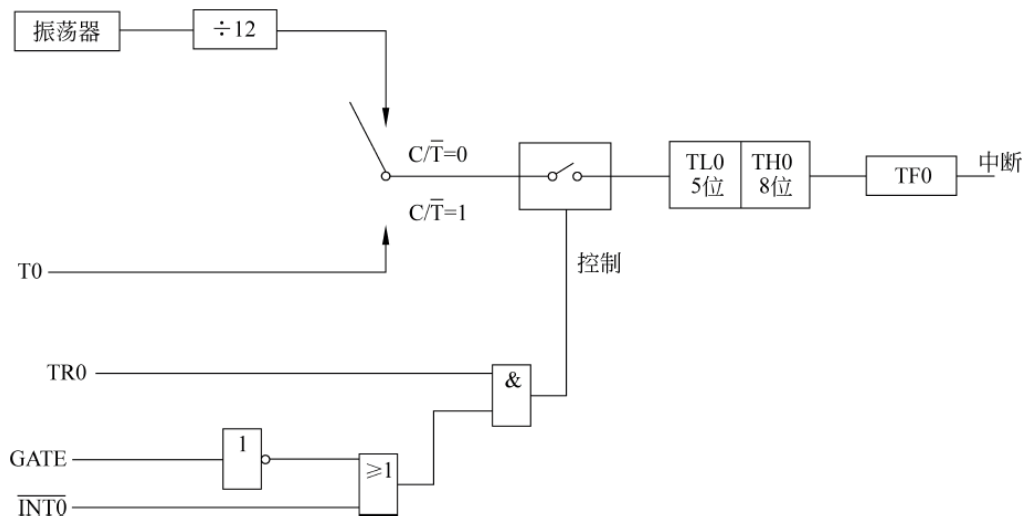
图 3-1 T0(或 T1)逻辑电路结构
