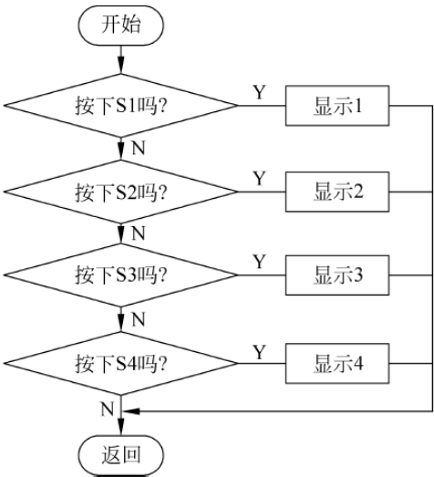
图 5-12 键盘管理程序流程
