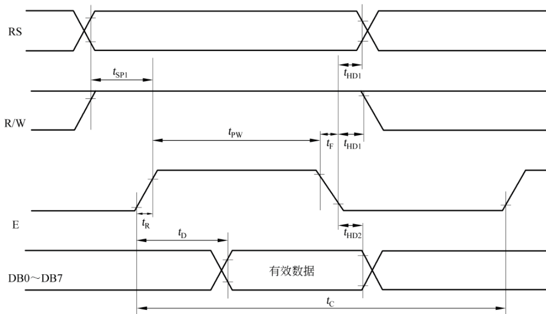
图 7-2 读操作时序
