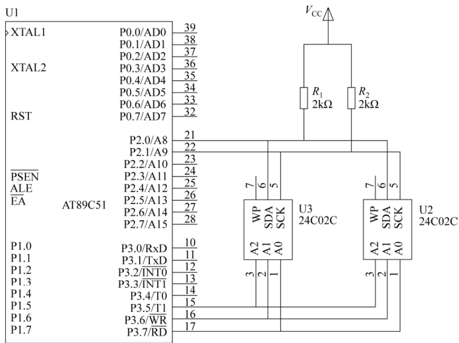
图 10-2 AT24C02 接口结构
