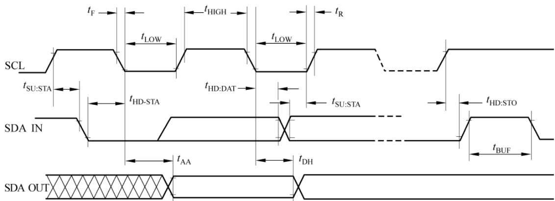
图 10-3 I 2 C 总线时序
