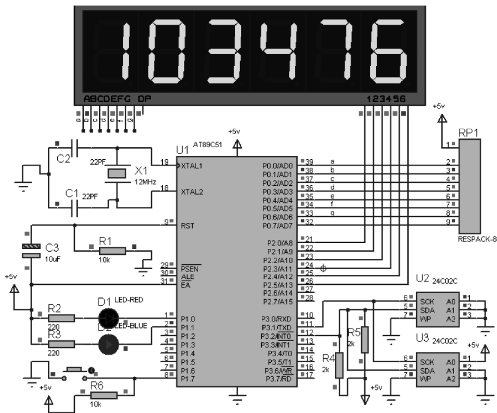
图 10-15 数据复制仪仿真模型
