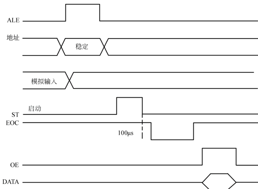
图 7-9 ADC0809 工作时序
