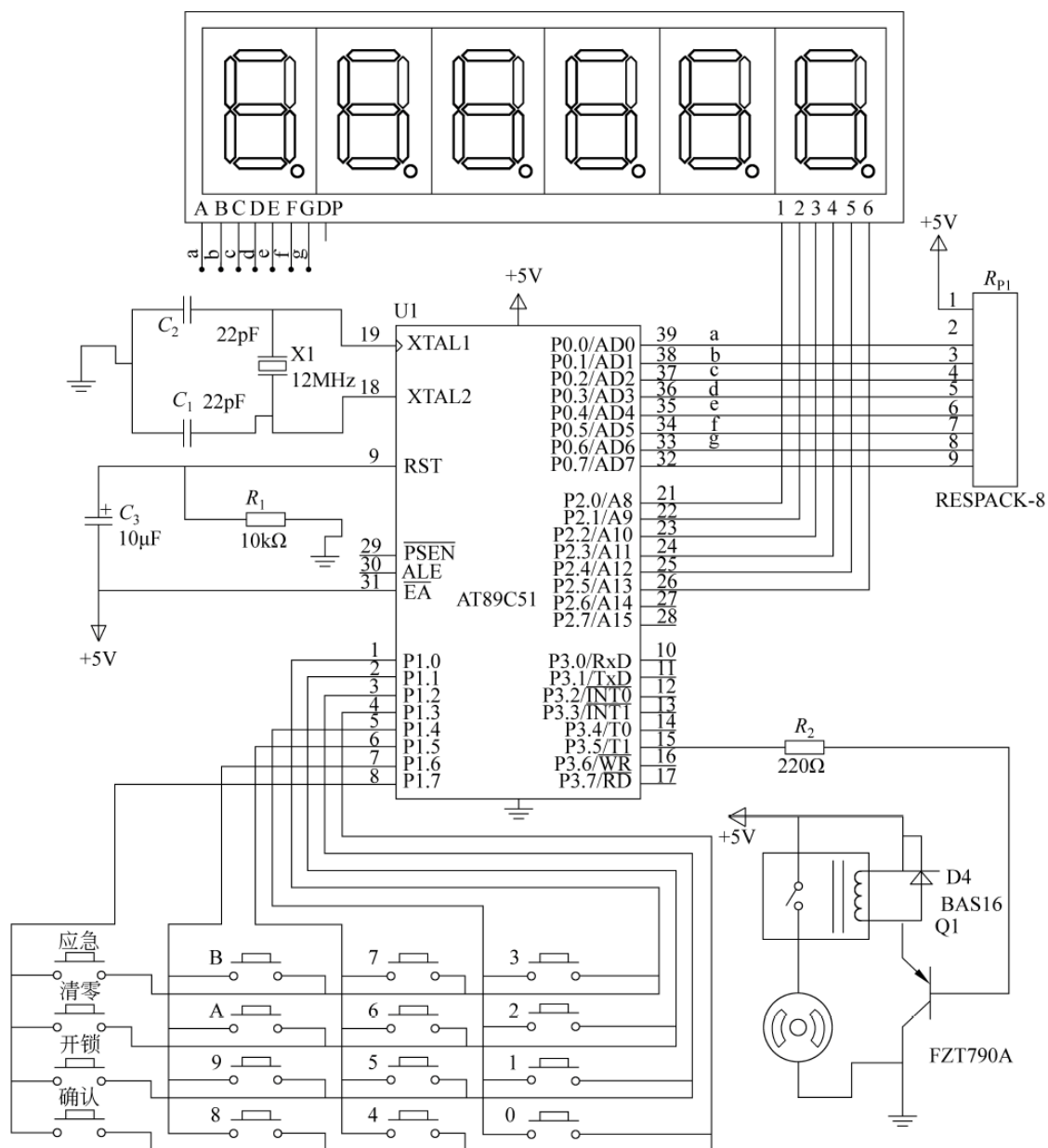
图 6-11 密码锁电路
