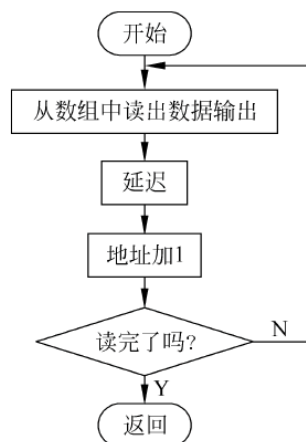
图 8-10 第二种方式产生三角波子程序流程
