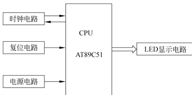
图 1-53 广告灯总体框图
