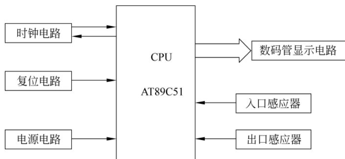
图 2-16 游客流量人数计数器总体框图
