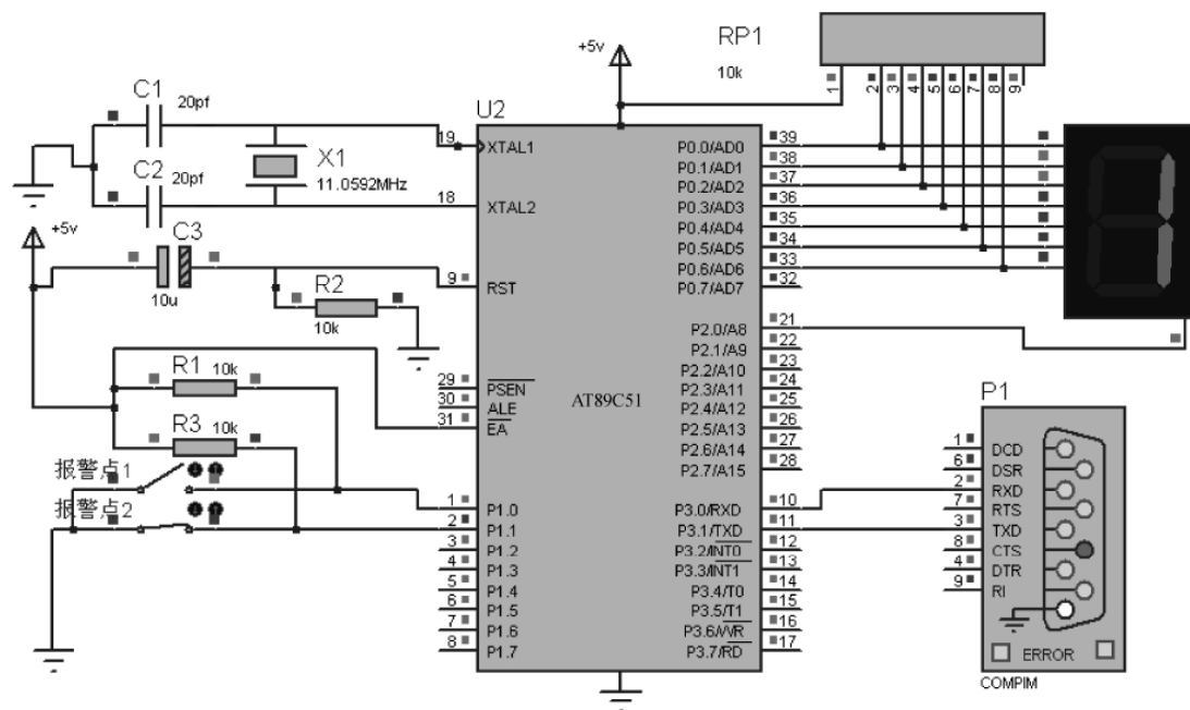
图 9-30 从机仿真模型
