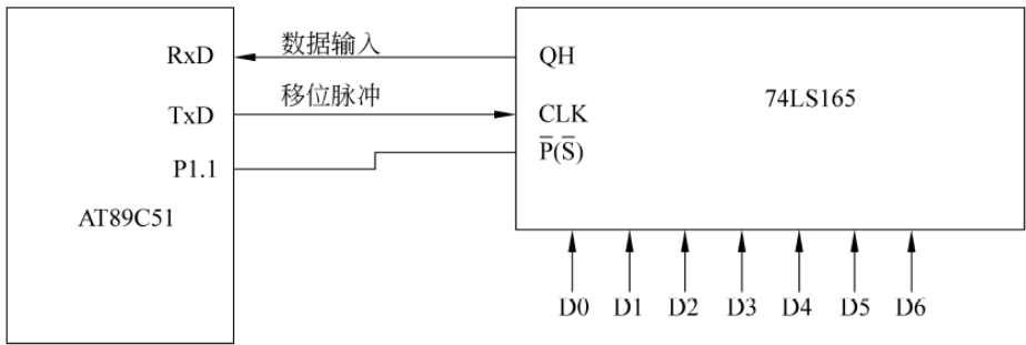
图 9-12 方式 0 用于扩展 I/O 口输入
