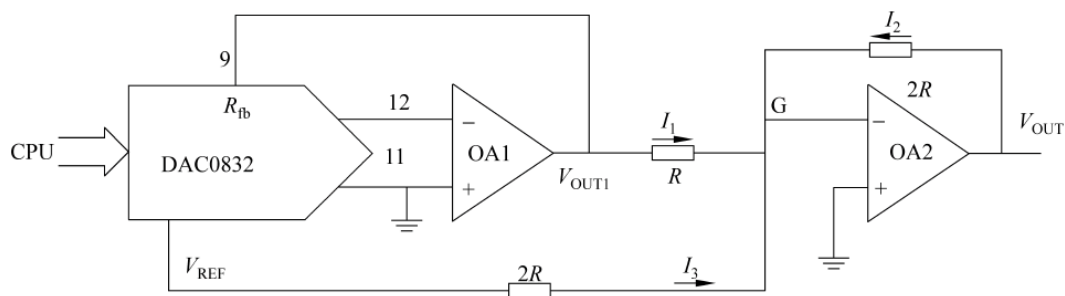
图 8-4 DAC0832 双极性电压输出连接
