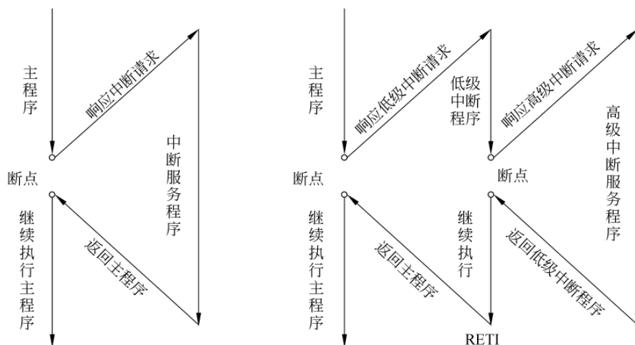
图 2-12 中断嵌套
