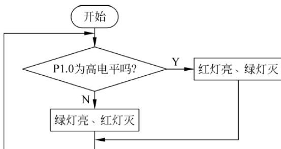
图 1-49 端口状态检测程序流程
