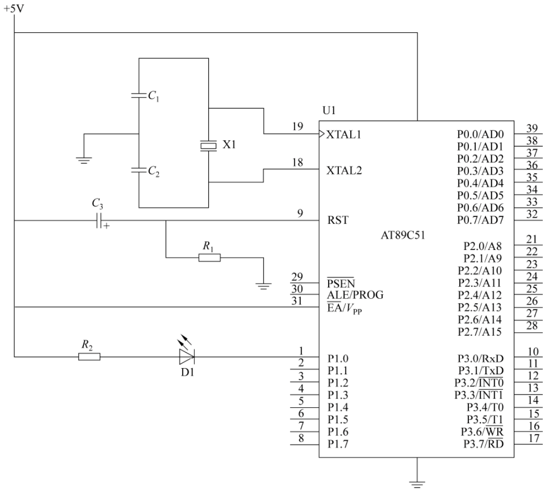
图 1-12 单片机最小系统图
