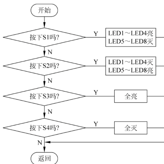
图 5-7 键盘功能处理流程
