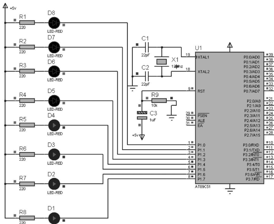
图 1-32 简单仿真电路模型
