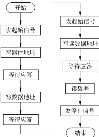
图 10-9 选择性读程序流程
