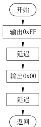
图 8-8 方波子程序流程
