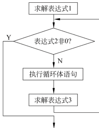
图 1-45 for 语句流程
