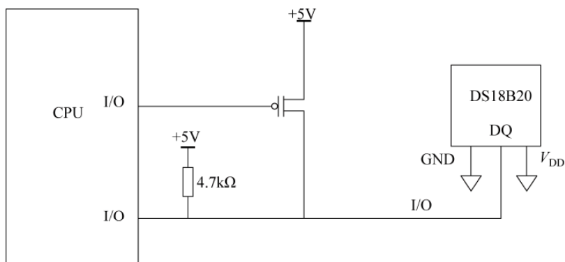
图 12-6 寄生电源工作方式
