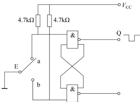
图 5-2 硬件消抖动电路
