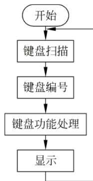
图 6-9 主程序流程
