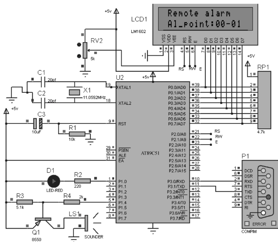
图 9-29 主机仿真模型
