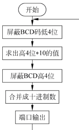
图 1-52 转换程序流程
