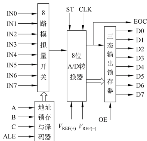
图 7-6 ADC0809 内部结构
