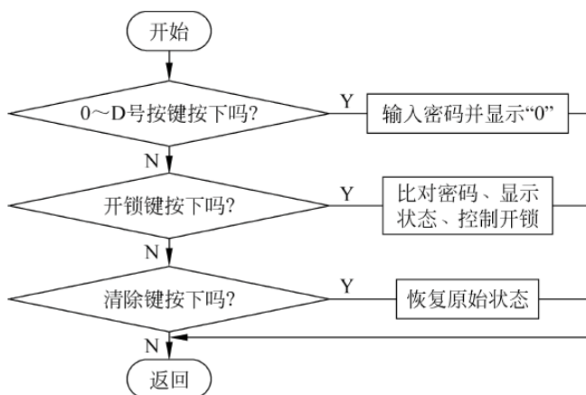
图 6-13 键盘管理程序流程
