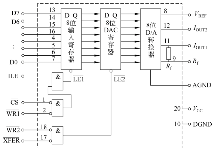
图 8-2 DAC0832 内部结构
