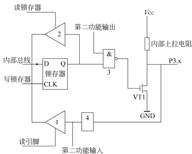
图 1-8 P3 的一位结构图
