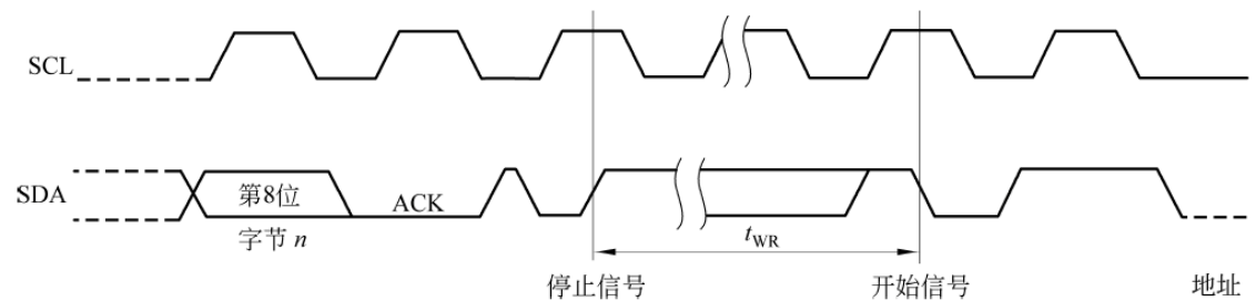
图 10-4 读写周期时序
