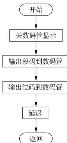
图 2-8 一位数据译码显示程序流程
