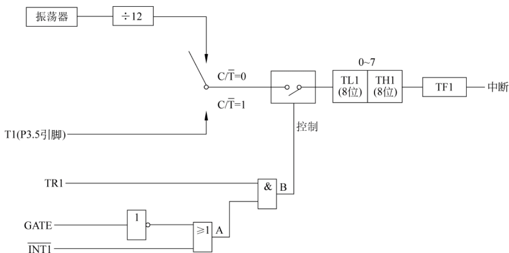
图 3-2 方式 1 时的逻辑结构
