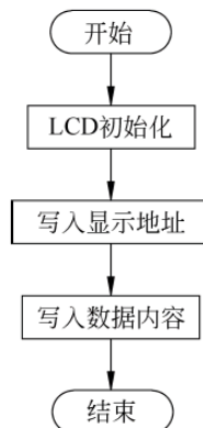
图 7-4 主程序流程
