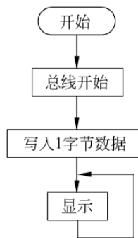
图 10-10 主程序流程
