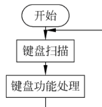
图 6-7 主程序流程
