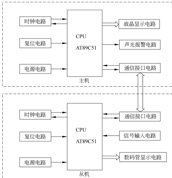
图 9-22 远程报警器总体框图
