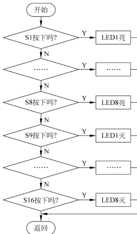
图 6-6 键盘功能处理程序流程
