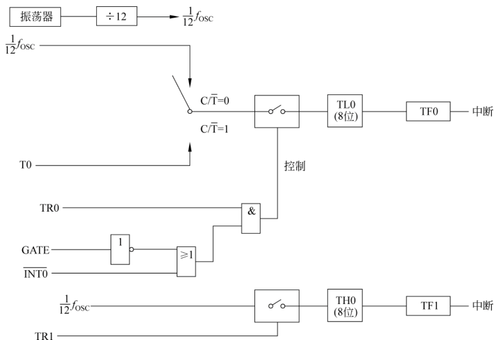
图 3-4 方式 3 时的逻辑结构
