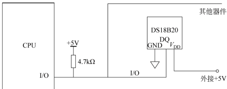
图 12-7 外接电源工作方式
