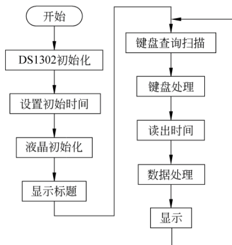
图 11-8 数字钟主程序流程
