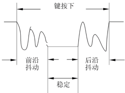
图 5-1 键盘抖动过程
