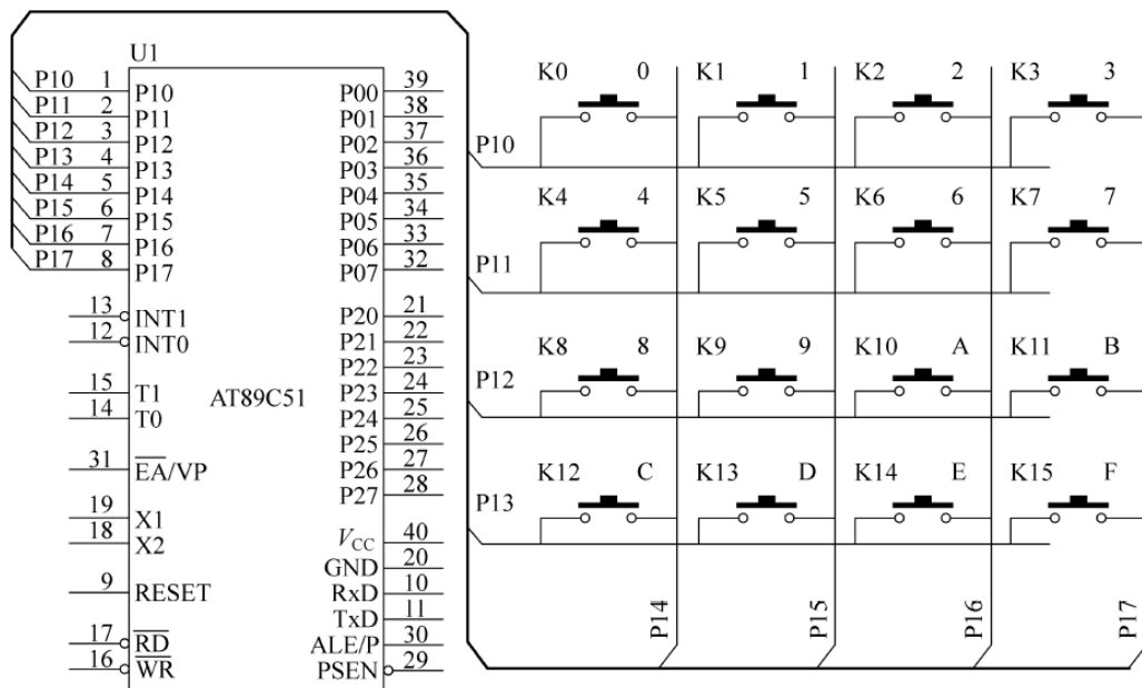
图 6-1 矩阵式键盘结构
