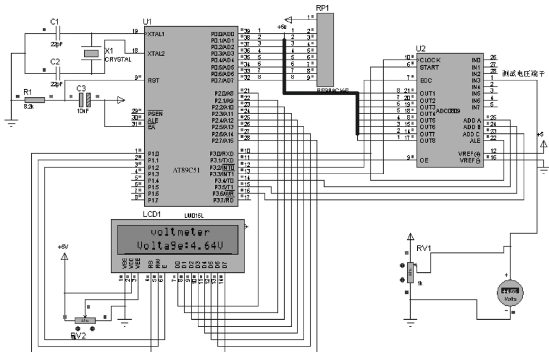
图 7-14 数字电压表仿真模型
