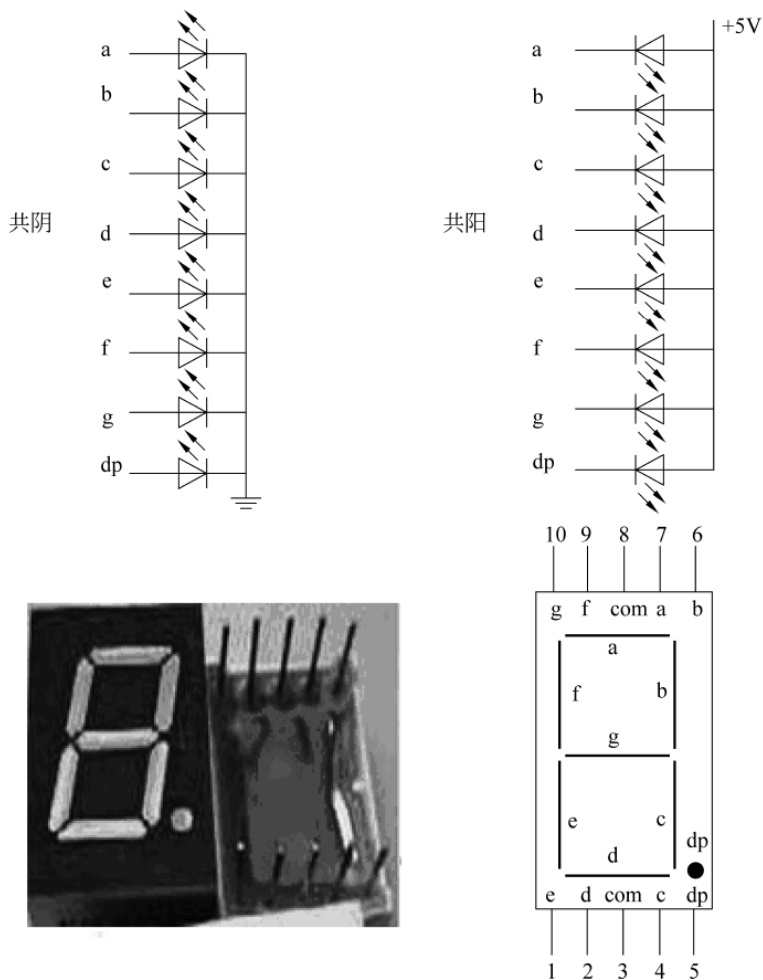
图 2-3 数码管外观和结构
