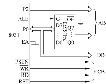
图 8-6 片外扩充时单片机的总线结构
