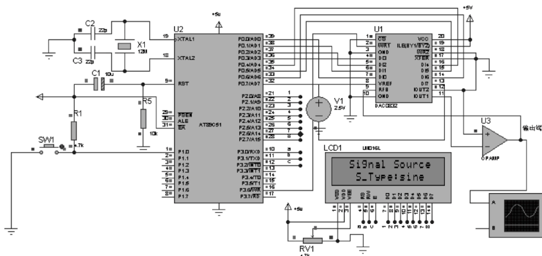
图 8-14 正弦信号发生器仿真模型
