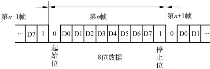
图 9-13 10 位的帧格式
