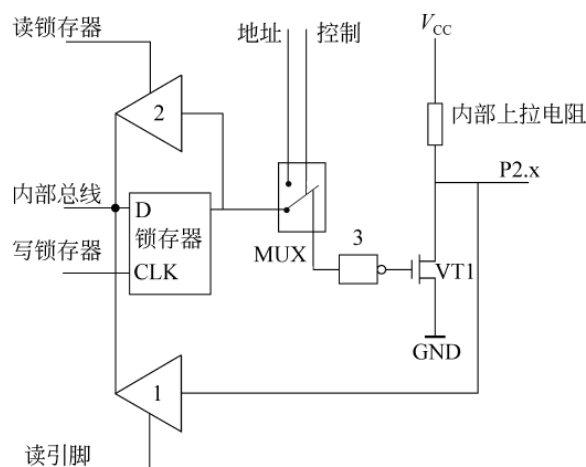
图 1-7 P2 口的一位结构图
