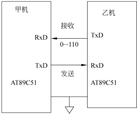
图 9-2 串行通信
