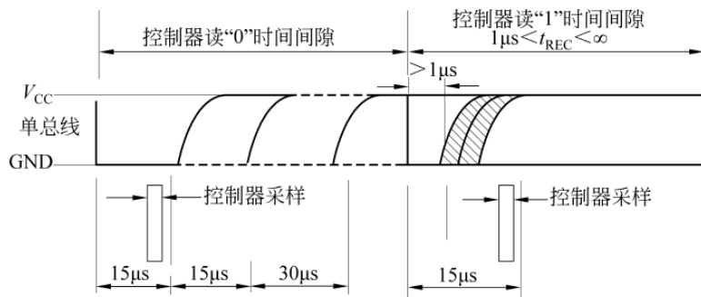
图 12-10 读时序
