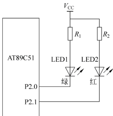
图 1-48 端口状态指示电路
