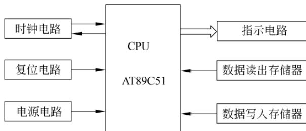
图 10-12 数据复制仪总体框图
