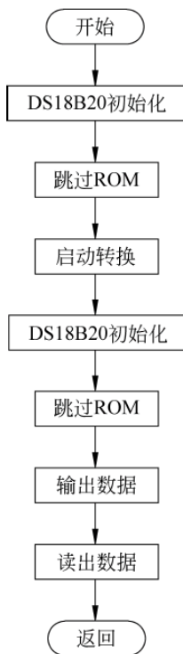
图 12-14 读出温度程序流程
