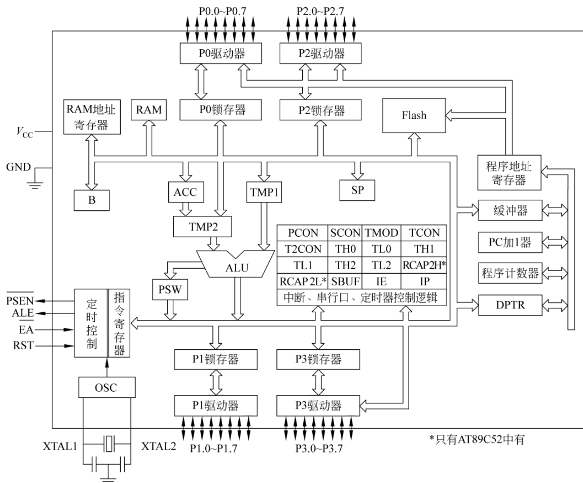
图 1-2 AT89C51 总体框图
