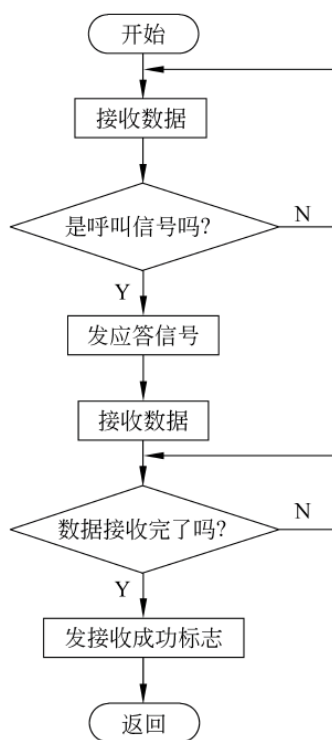
图 9-26 中断服务程序流程
