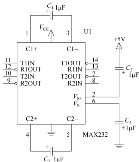
图 9-8 MAX232 接口电路
