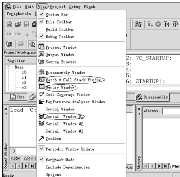
图 1-23 选择调试观察窗口
