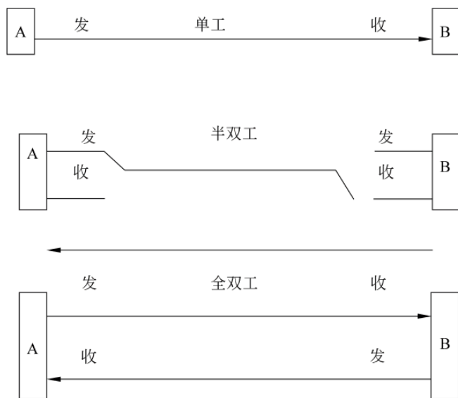
图 9-5 串行通信制式
