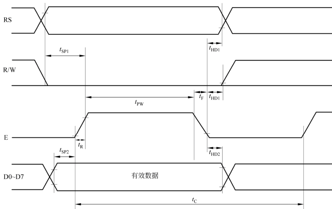
图 7-3 写操作时序
