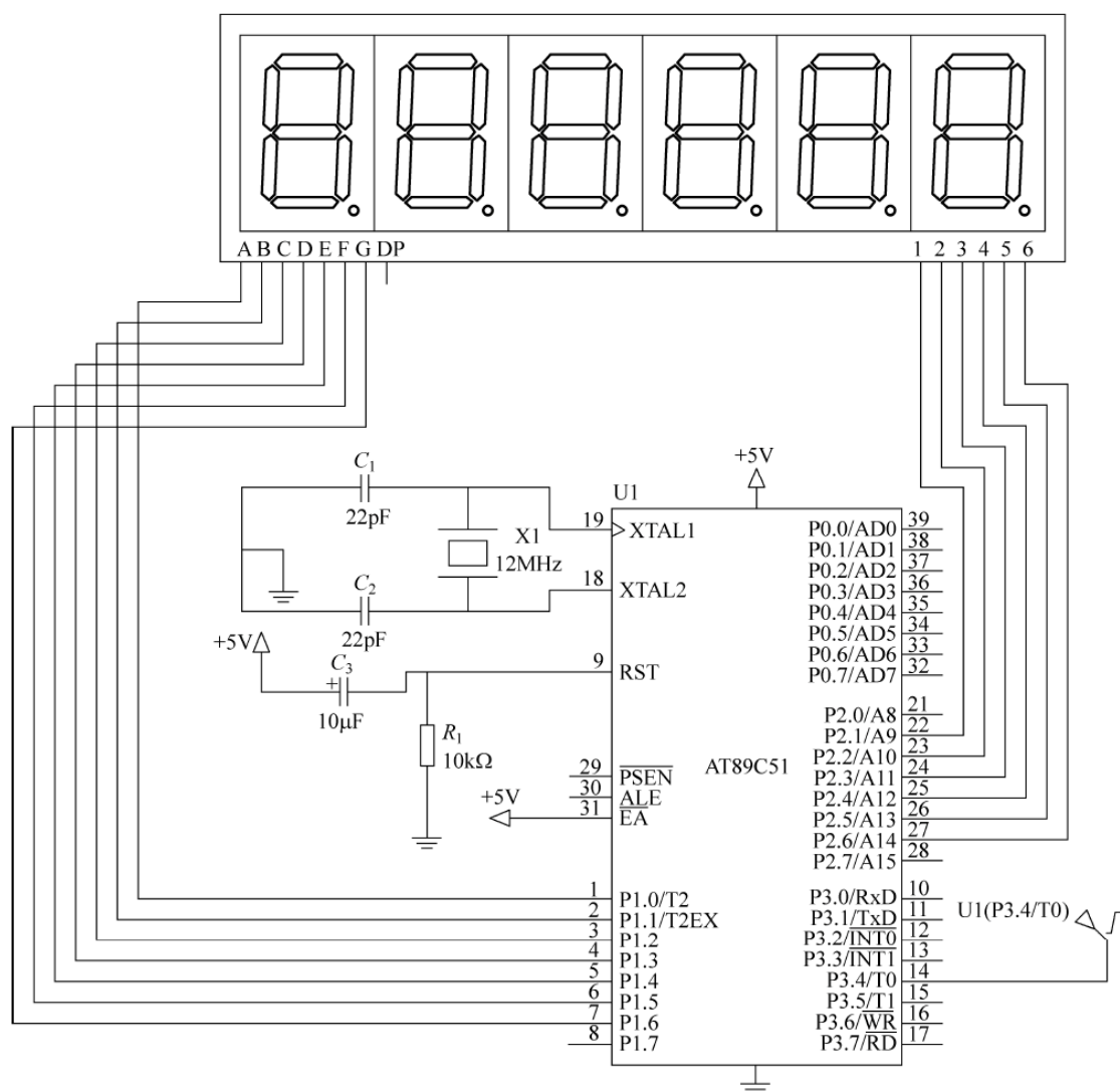
图 3-7 啤酒生产计数器硬件电路
