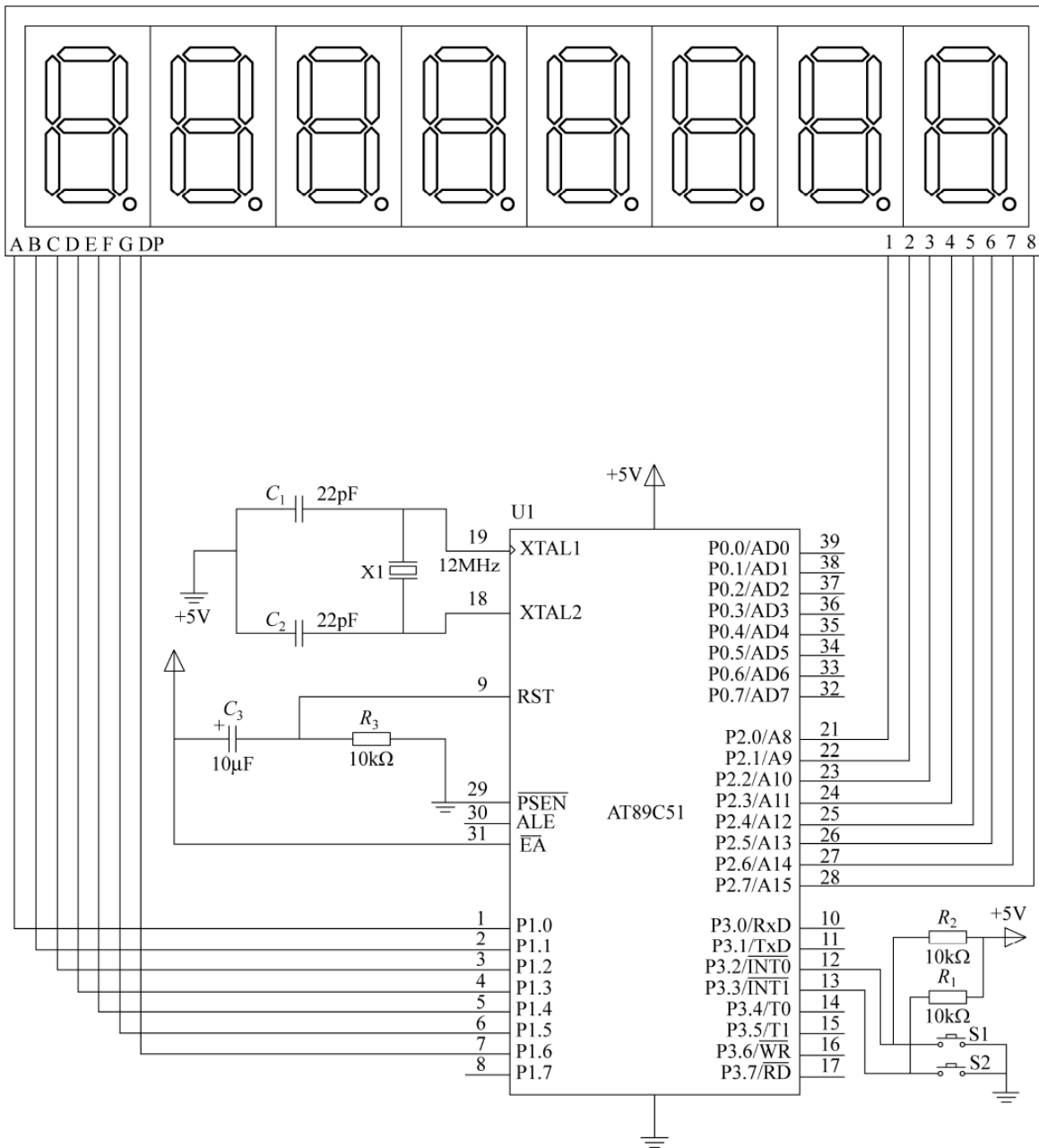
图 2-17 游客流量人数计数器电路
