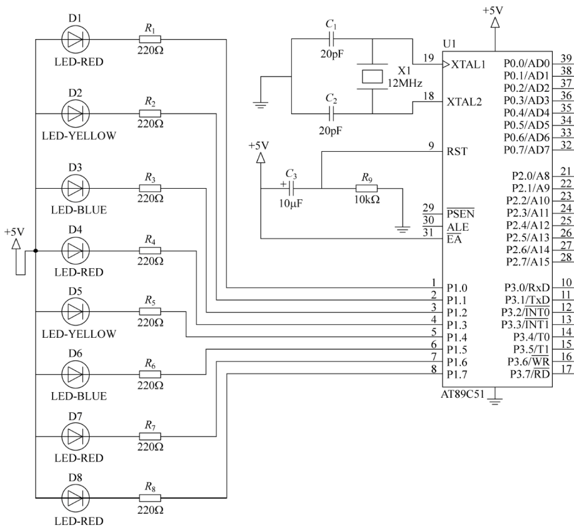
图 1-54 广告灯电路
