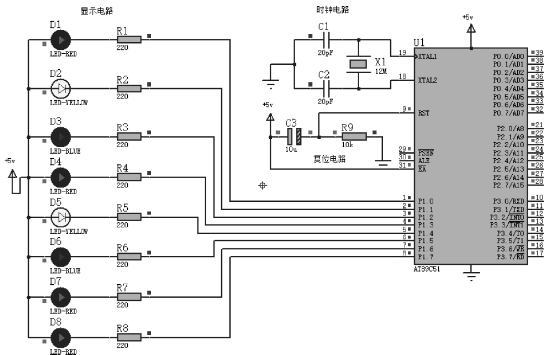
图 1-57 广告灯参考仿真模型
