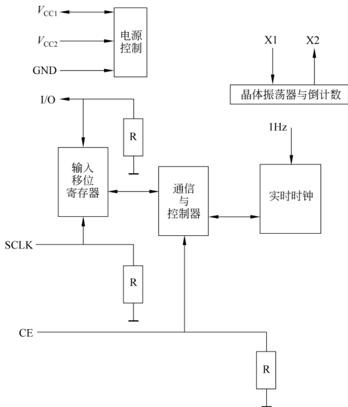
图 11-2 DS1302 内部结构
