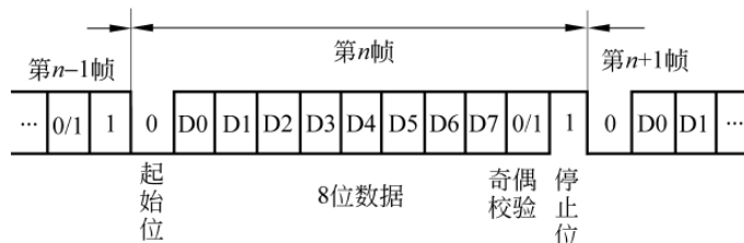
图 9-14 11 位的帧格式
