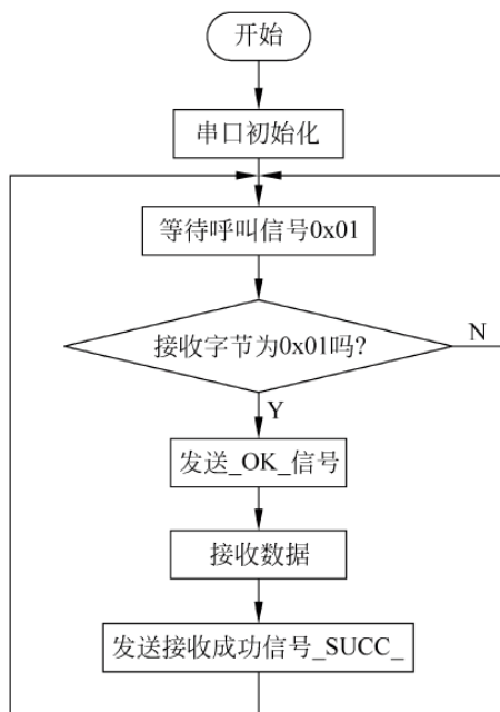
图 9-21 从机通信程序流程
