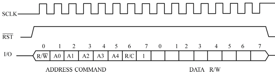
图 11-4 单字节写操作时序
