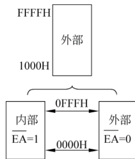
图 1-4 程序存储器选择图
