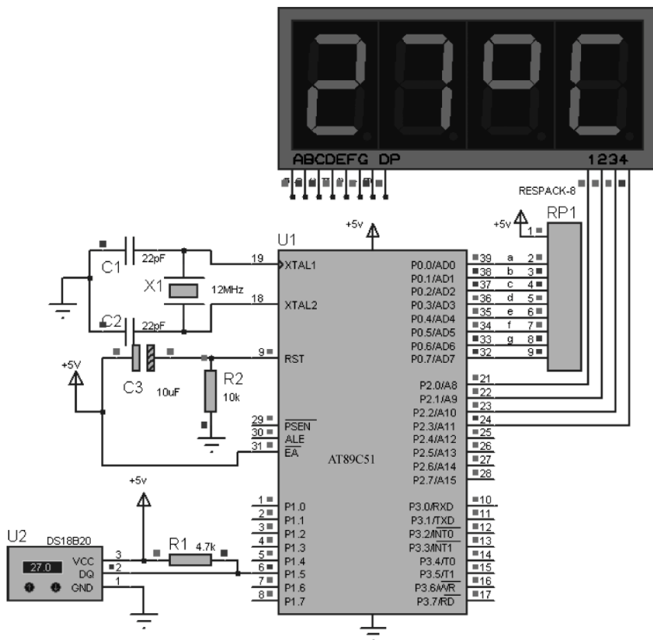
图 12-15 数字温度计仿真模型
