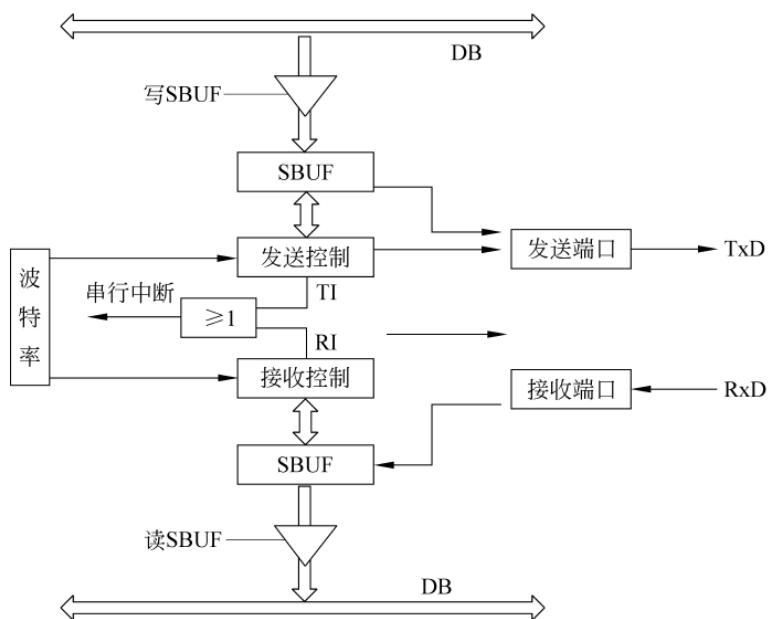
图 9-10 MCS-51 单片机串行口结构
