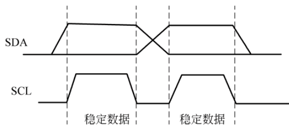
图 10-6 I 2 C 总线有效性示意图
