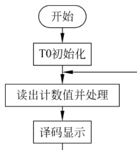
图 3-5 主程序流程
