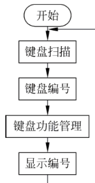
图 6-8 主程序流程
