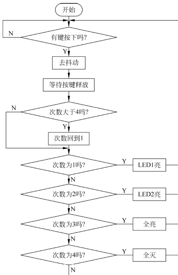
图 5-5 程序流程
