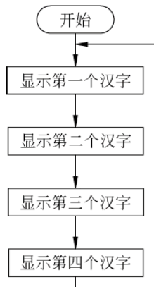
图 2-10 主程序流程
