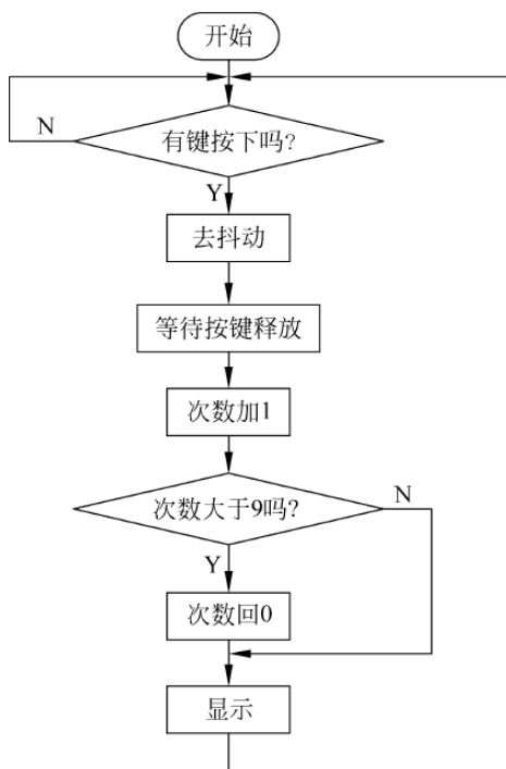
图 5-4 程序流程
