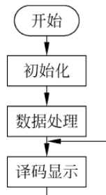
图 2-9 主程序流程
