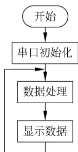
图 9-18 主程序流程
