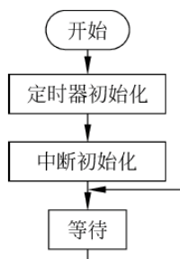
图 4-1 主程序流程
