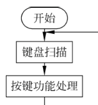
图 5-8 主程序流程
