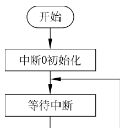
图 2-14 主程序流程
