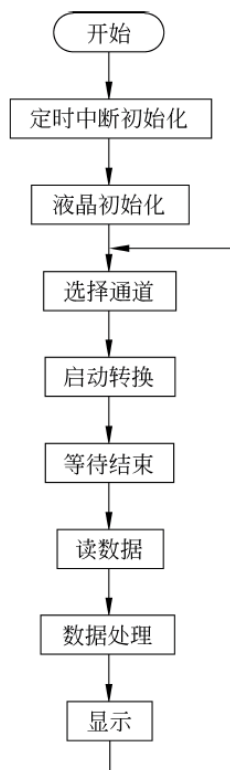
图 7-12 主程序流程
