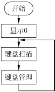
图 5-13 主程序流程
