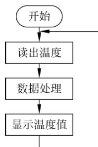
图 12-13 主程序流程
