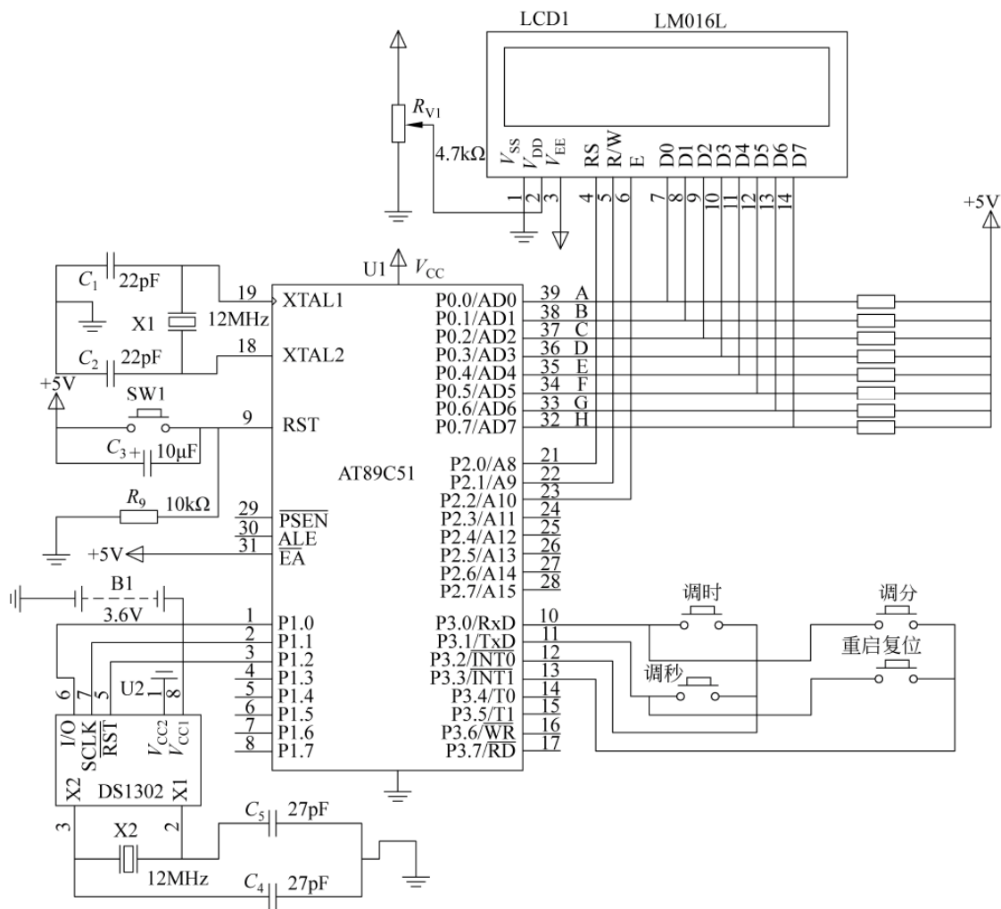
图 11-7 数字钟硬件电路
