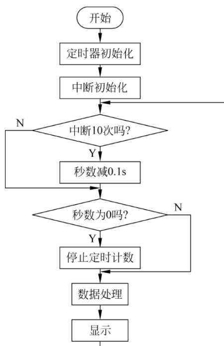
图 4-5 主程序流程
