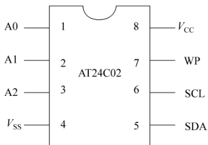
图 10-1 AT24C02 引脚分布
