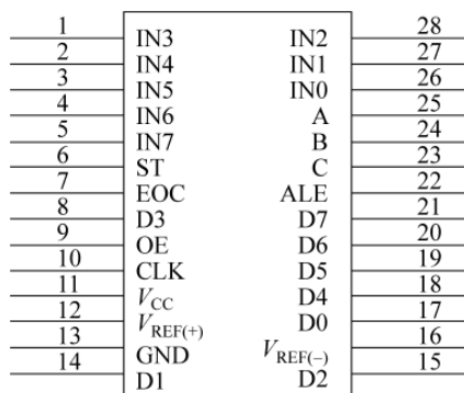
图 7-7 ADC0809 引脚分布
