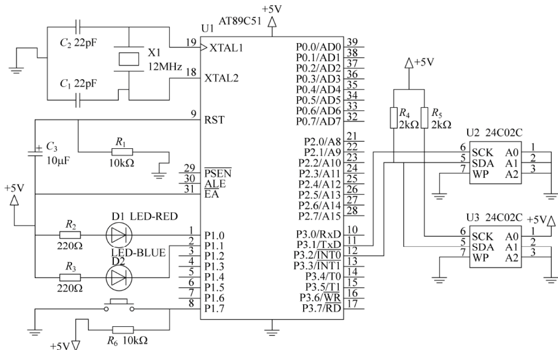
图 10-13 数据复制仪硬件电路
