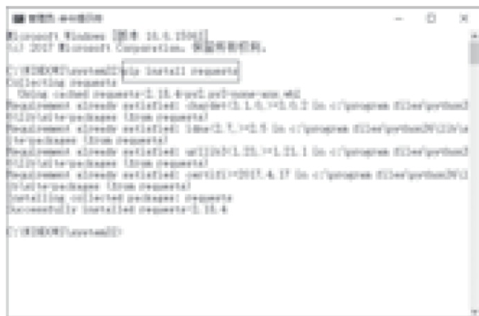
图 14-1 安装 requests 库
