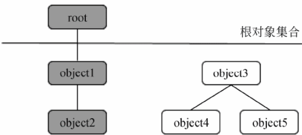
图 10.5 根搜索算法举例
