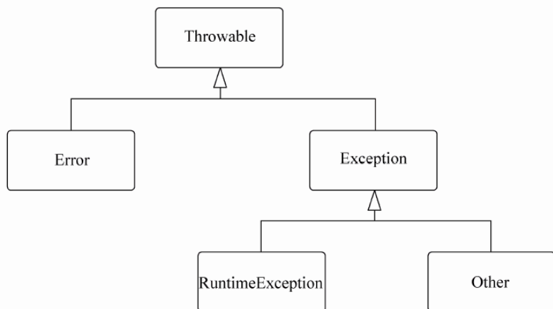
图 21.1 Java 异常 UML 类图
