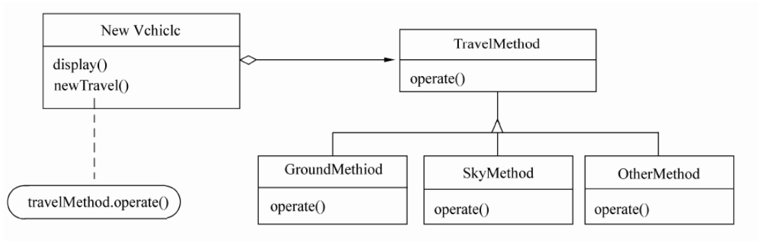
图 17.3 示例代码 17.2 的 UML 类图
