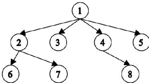
图 14.1 有向图示例
