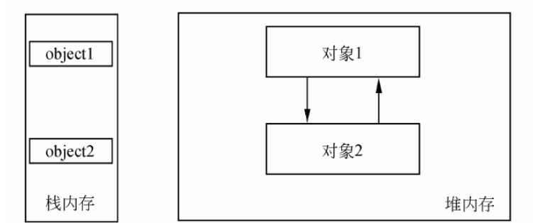
图 10.4 内存结构示意图 4
