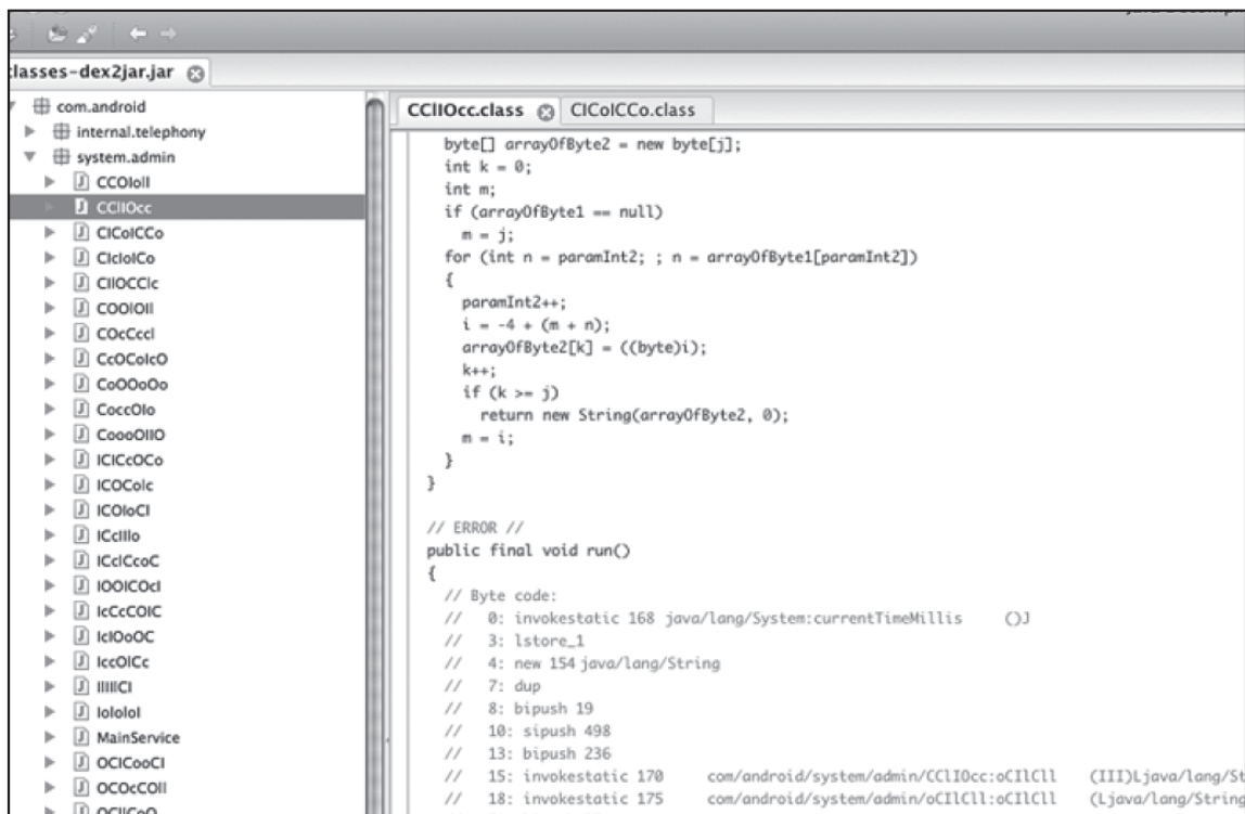
图9-90 Java反编译工具
