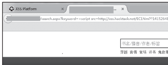
图6-24 XSS实际已被触发
