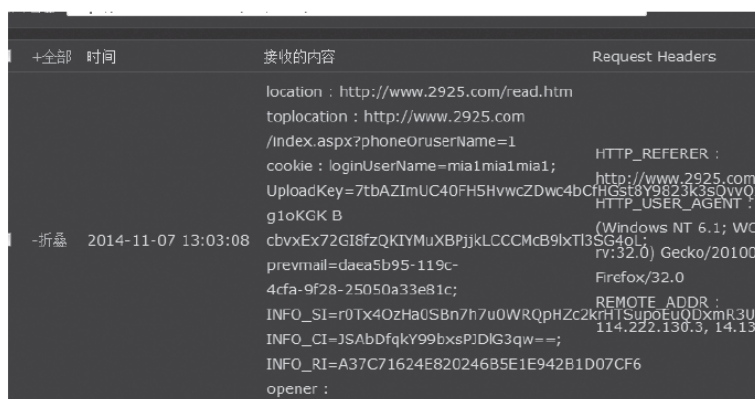
图6-37 查看XSS平台
