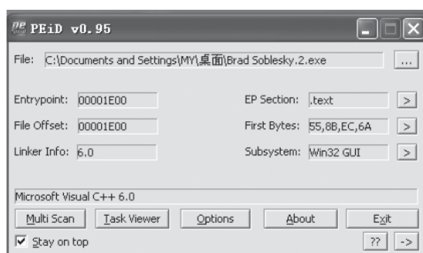
图8-38 PEiD查询结果
