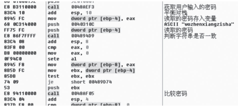
图9-11 “敲竹杠” 密码获得过程
