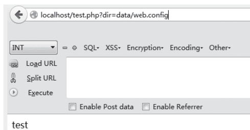
图4-24 读取本地文件
