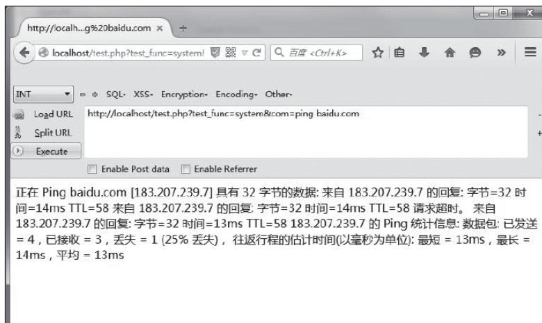
图4-21 直接执行ping命令
