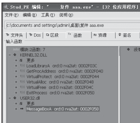
图9-17 函数分析界面
