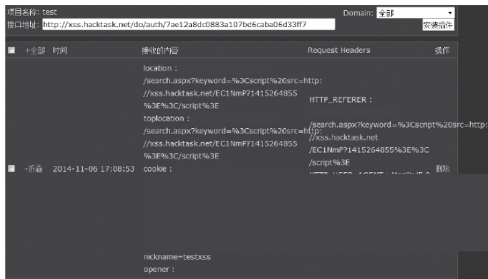
图6-25 接收到窃取的信息
