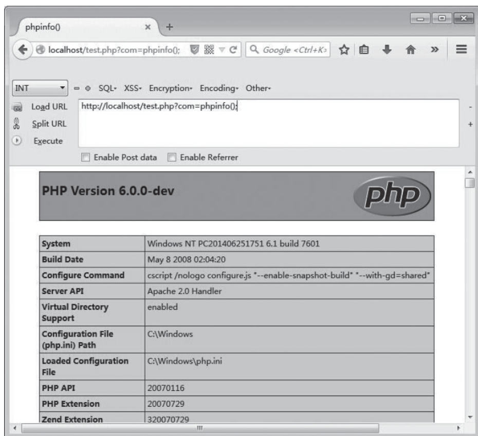
图4-17 执行phpinfo命令
