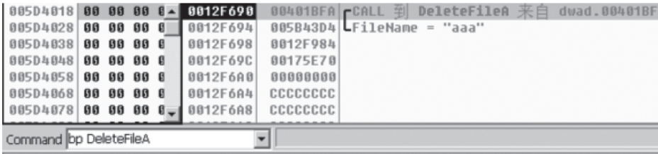
图9-8 bp API函数
