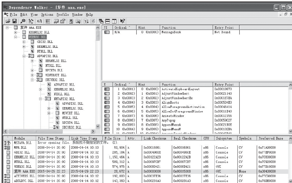
图9-18 Dependency Walker界面
