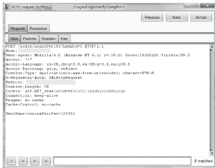
图3-23 登录操作发送的数据包
