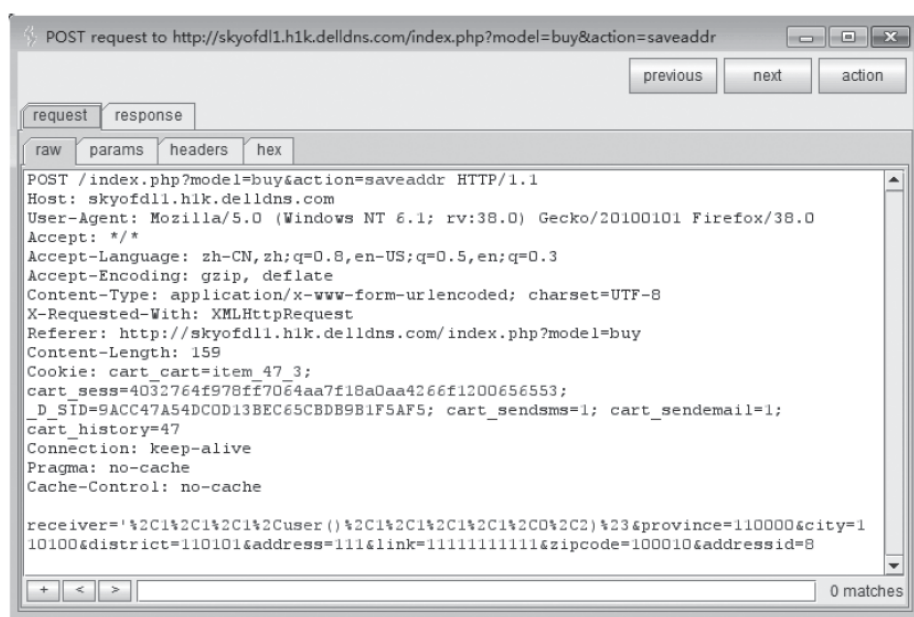
图4-14 提交的数据包
