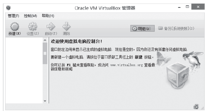
图1-2 VirtualBox主界面
