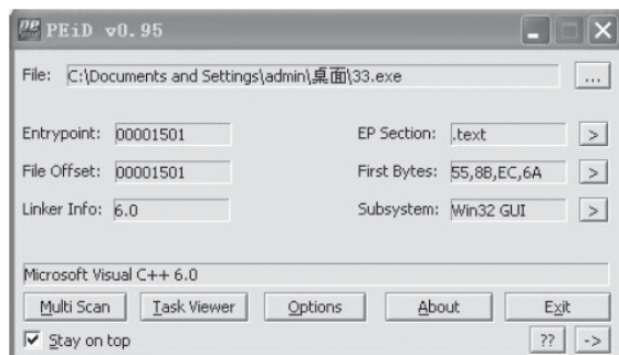
图9-41 查壳
