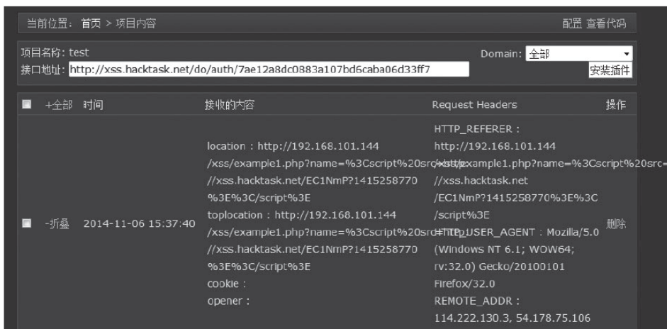
图6-21 劫持信息
