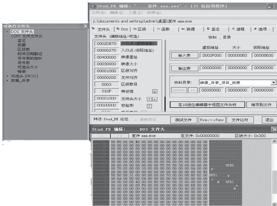
图9-15 Stud_PE功能图
