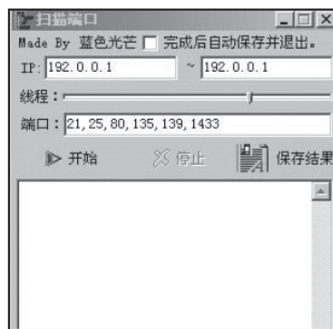
图7-5 扫描端口
