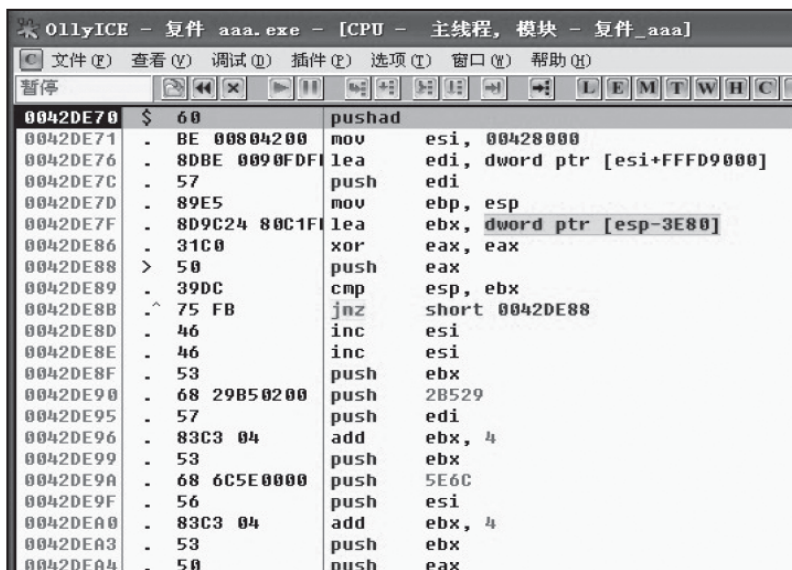
图9-13 加壳文件
