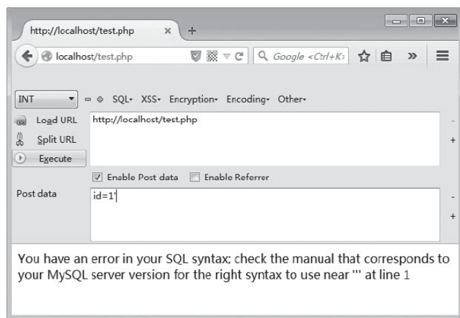
图4-10 POST注入
