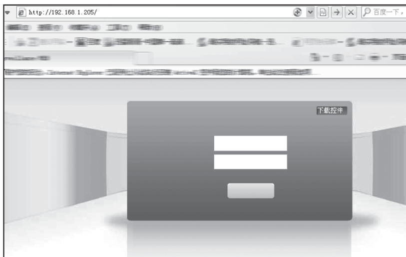
图7-6 登录接口
