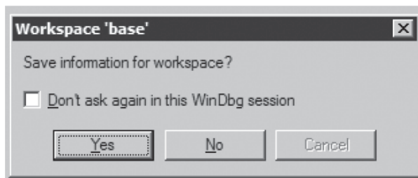
图9-65 工作空间
