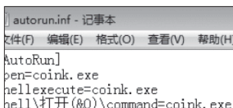
图9-83 autorun.inf(2)
