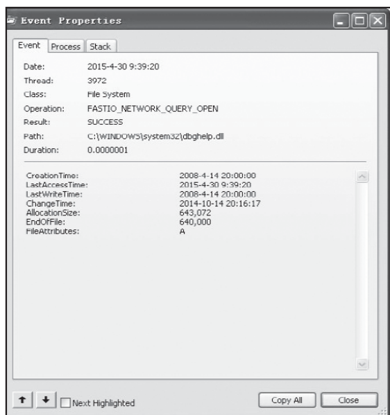
图9-20 Event选项
