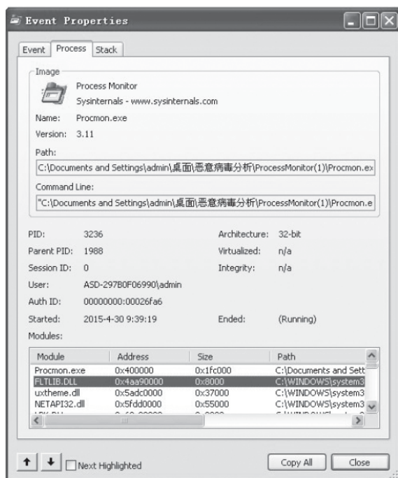
图9-21 Process选项
