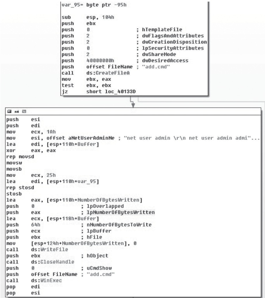
图9-55 CreateFileA（3）
