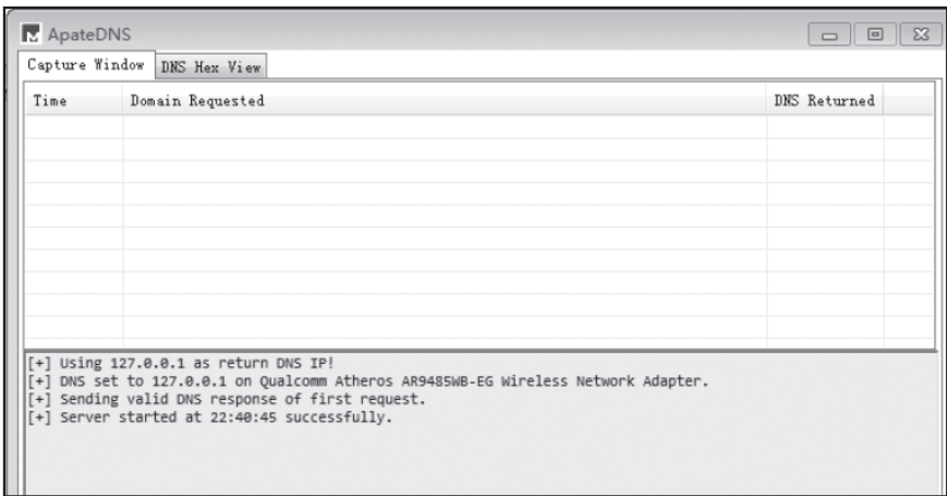
图9-39 ApateDNS截获
