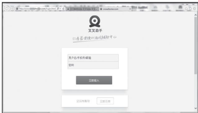
图6-55 钓鱼页面
