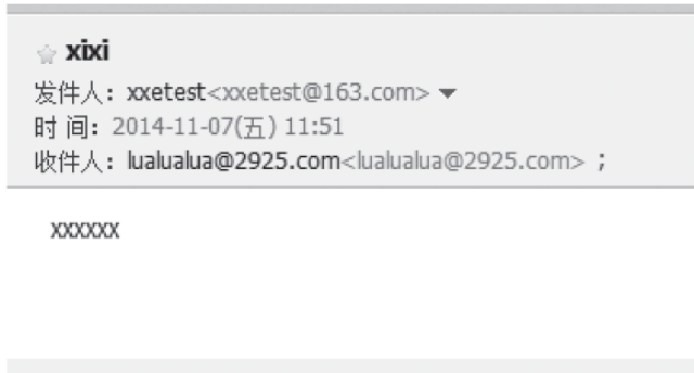
图6-35 发送结果
