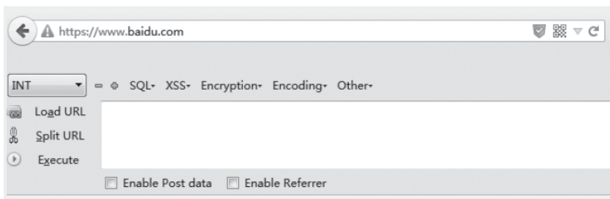
图4-8 Hackbar
