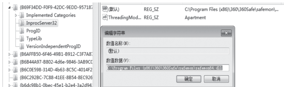
图9-86 加载DLL
