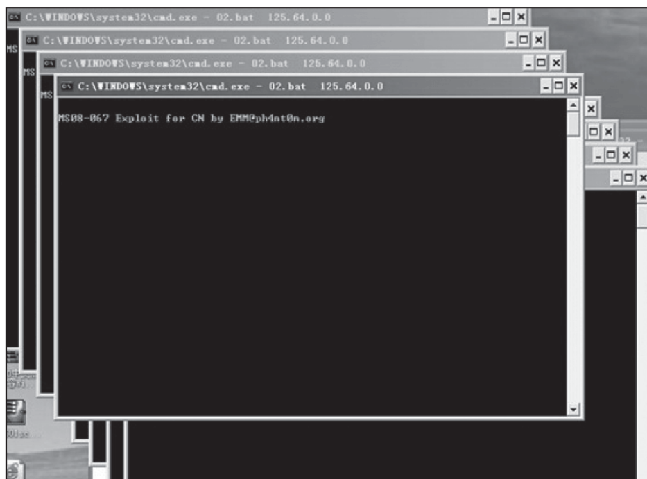
图8-35 工具追踪
