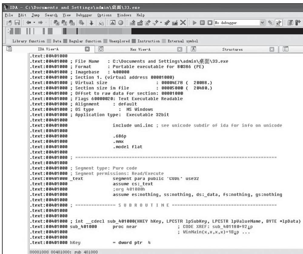
图9-47 文本模式
