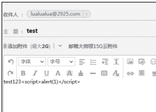
图6-32 正文payload测试
