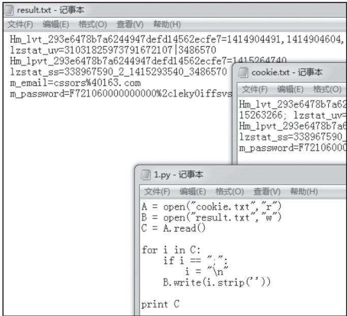
图6-27 用Python脚本整理cookie信息
