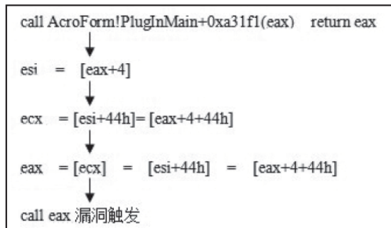
图8-25 PDF漏洞触发流程
