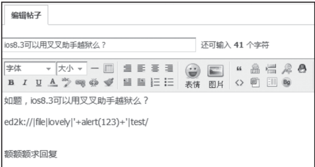
图6-49 跳转到另一个域下的XSS测试
