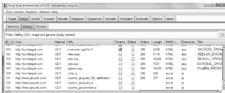
图3-7 对站点操作时的数据包
