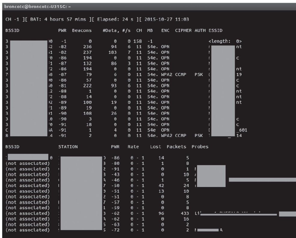
图5-15 airodump-ng对Probe的显示
