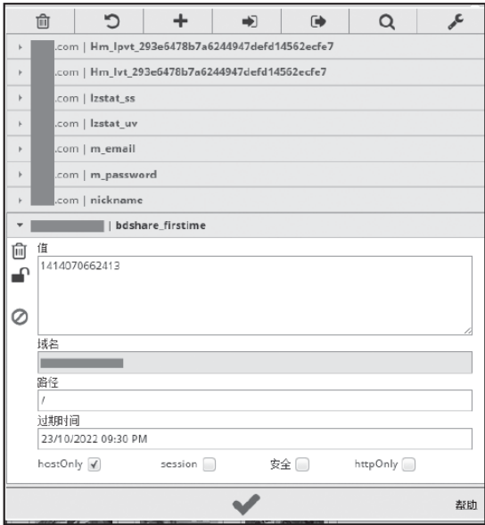
图6-29 查看cookie信息
