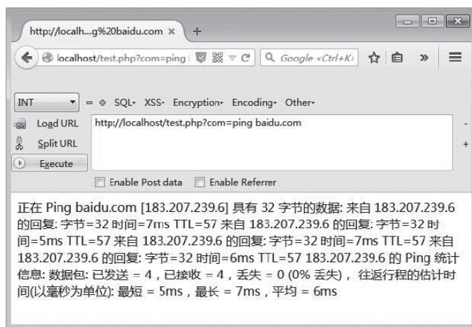
图4-19 执行ping命令
