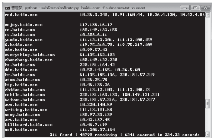
图3-3 利用脚本爆破出211个子域名
