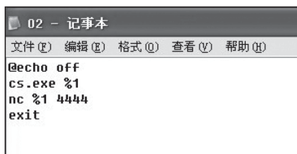
图8-34 跟踪生成的02.bat脚本
