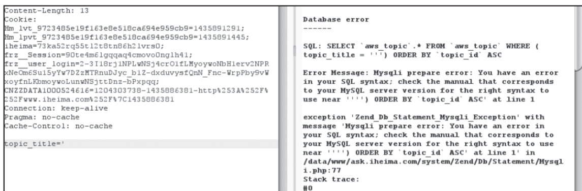
图3-14 MySQL查询语句示例
