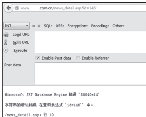
图3-9 单引号报错实例
