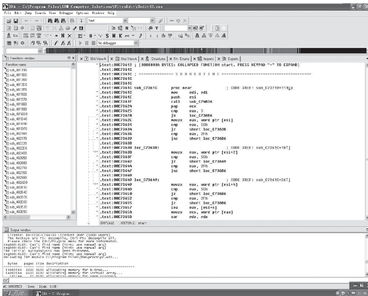
图8-1 IDA Pro主界面
