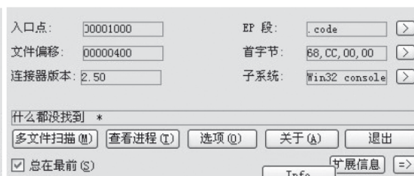
图8-31 UPX脱壳后PEiD显示情况
