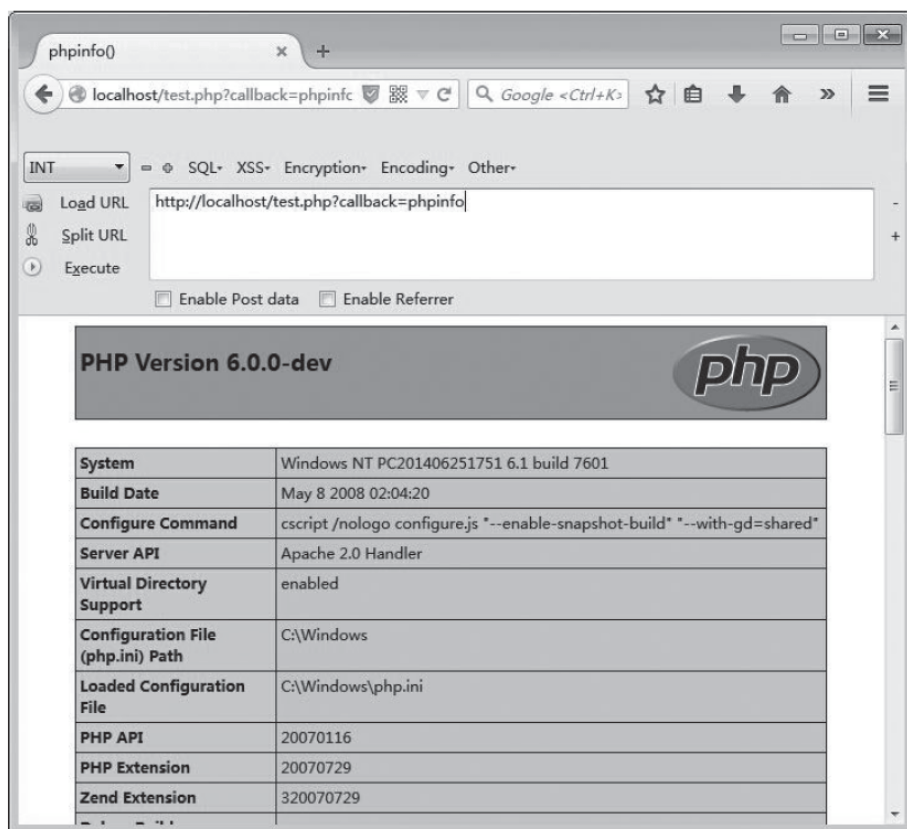
图4-20 执行phpinfo命令
