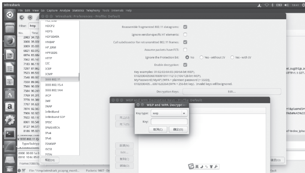
图5-14 Wireshark添加目标WiFi密钥
