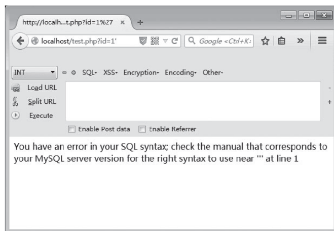
图4-9 提交单引号
