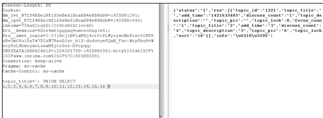
图3-15 联合查询
