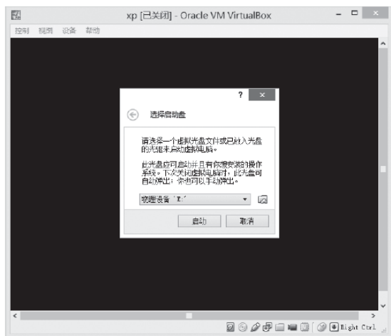
图1-8 开启虚拟机
