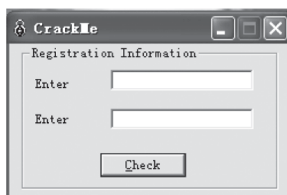
图8-37 程序界面
