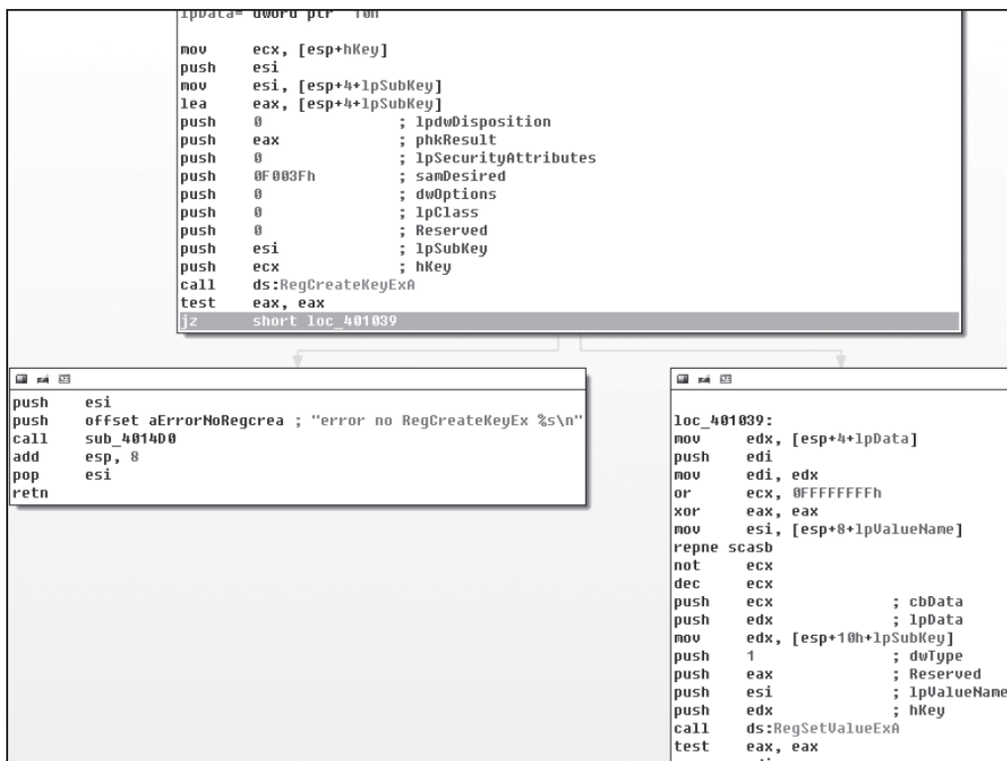
图9-56 注册表过程（1）
