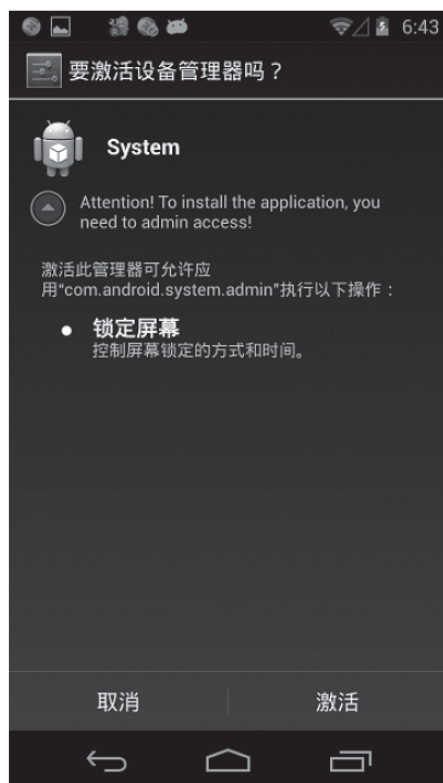
图9-91 激活界面
