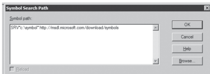
图9-63 符号表设置 (2)
