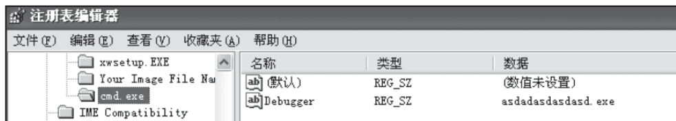
图9-87 IFEO
