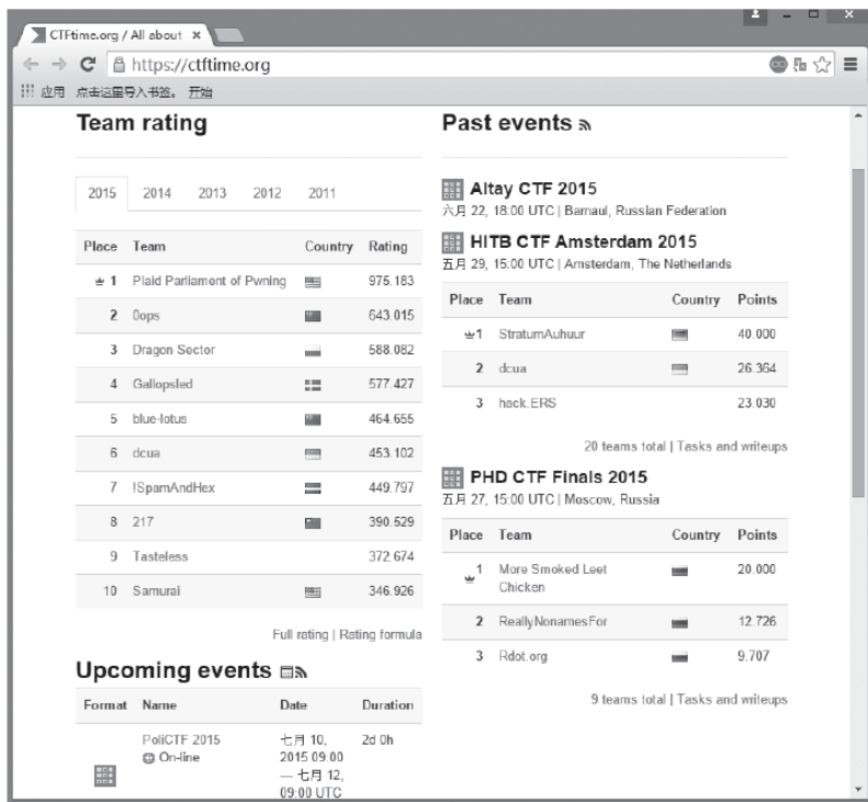
图10-1 CTFTIME网站
