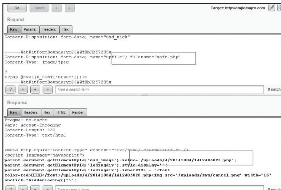
图4-22 改包代替
