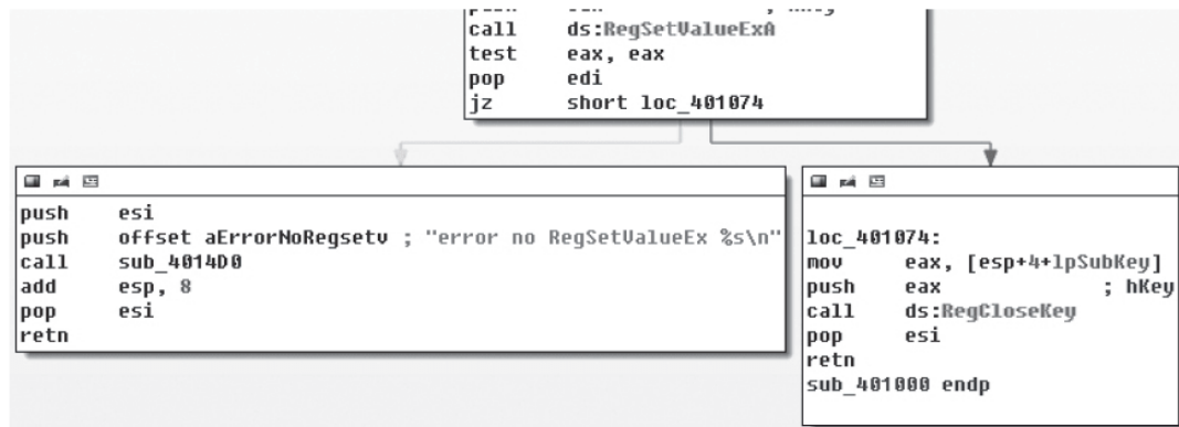
图9-57 注册表过程（2）
