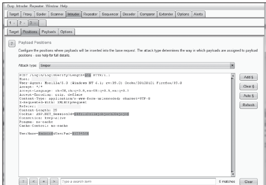
图3-26 登录包
