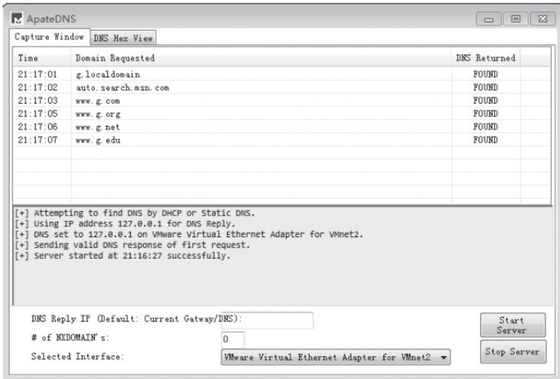
图9-27 运行后结果
