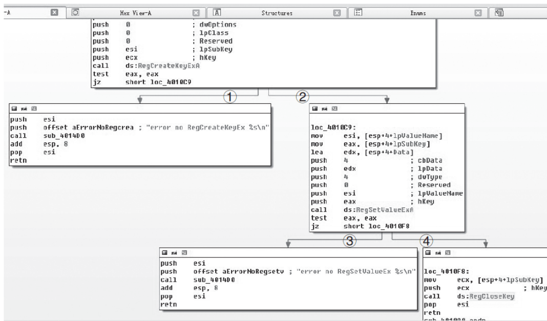
图9-48 图形模式
