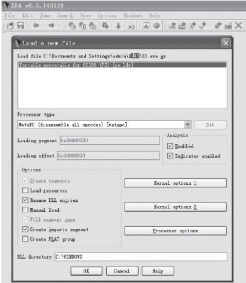
图9-46 IDA Pro
