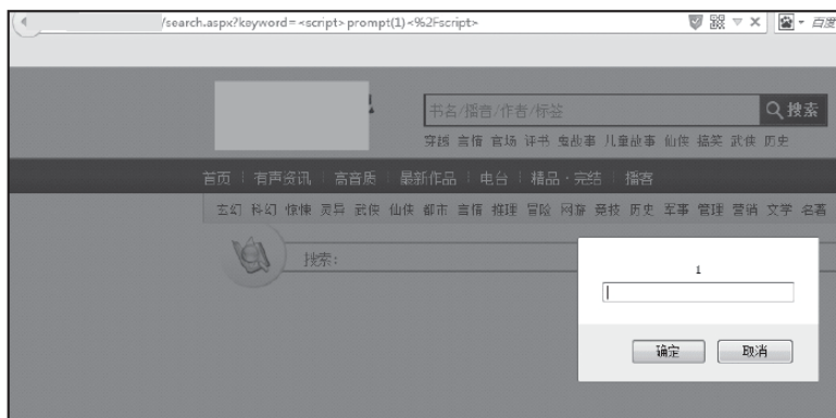
图6-22 存在XSS
