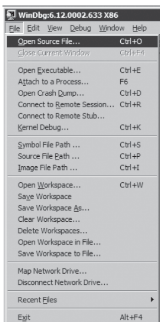
图9-62 符表设置 (1)
