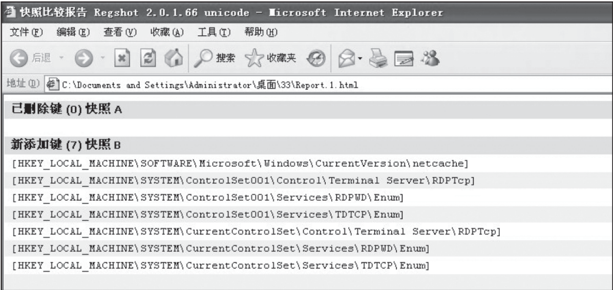
图9-33 注册表变化（1）
