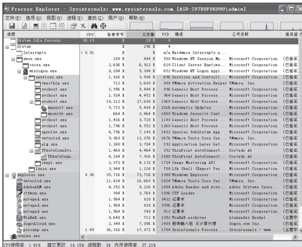
图9-23 procexp进程树
