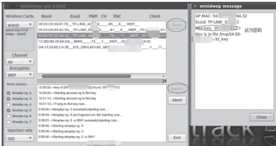
图5-4 minidwep-gtk界面
