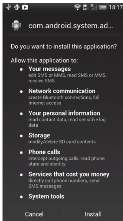
图9-88 安装界面
