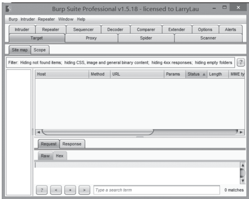
图4-2 Burp Suite
