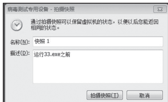
图9-30 拍摄还原点
