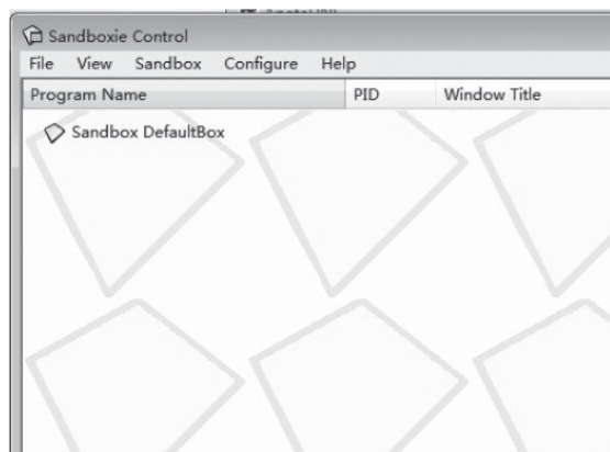
图9-28 沙箱
