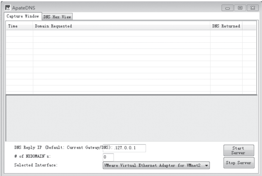
图9-26 ApateDNS主界面
