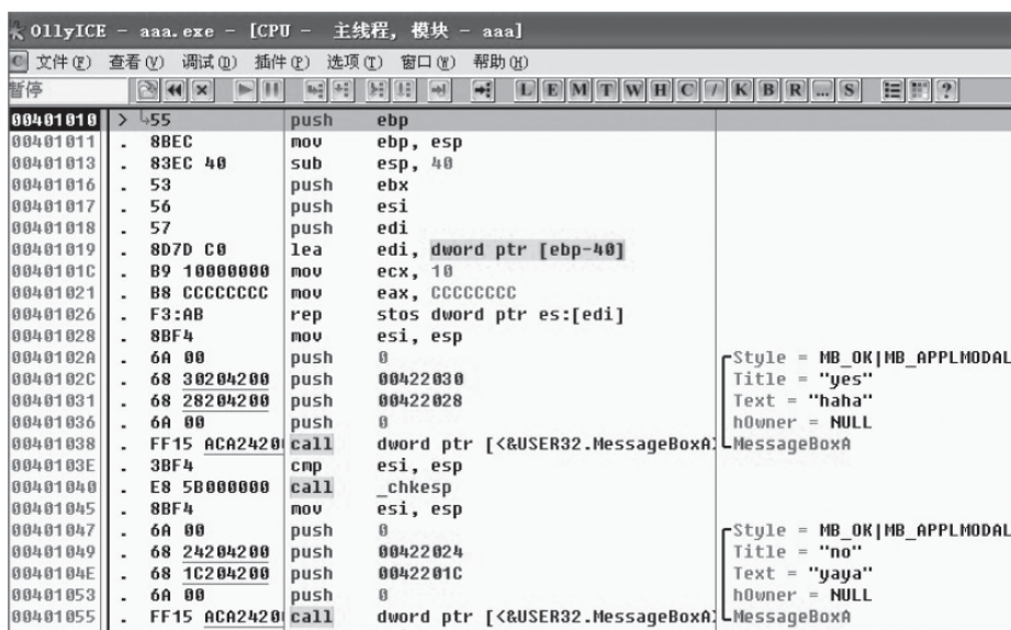
图9-14 文件脱壳后
