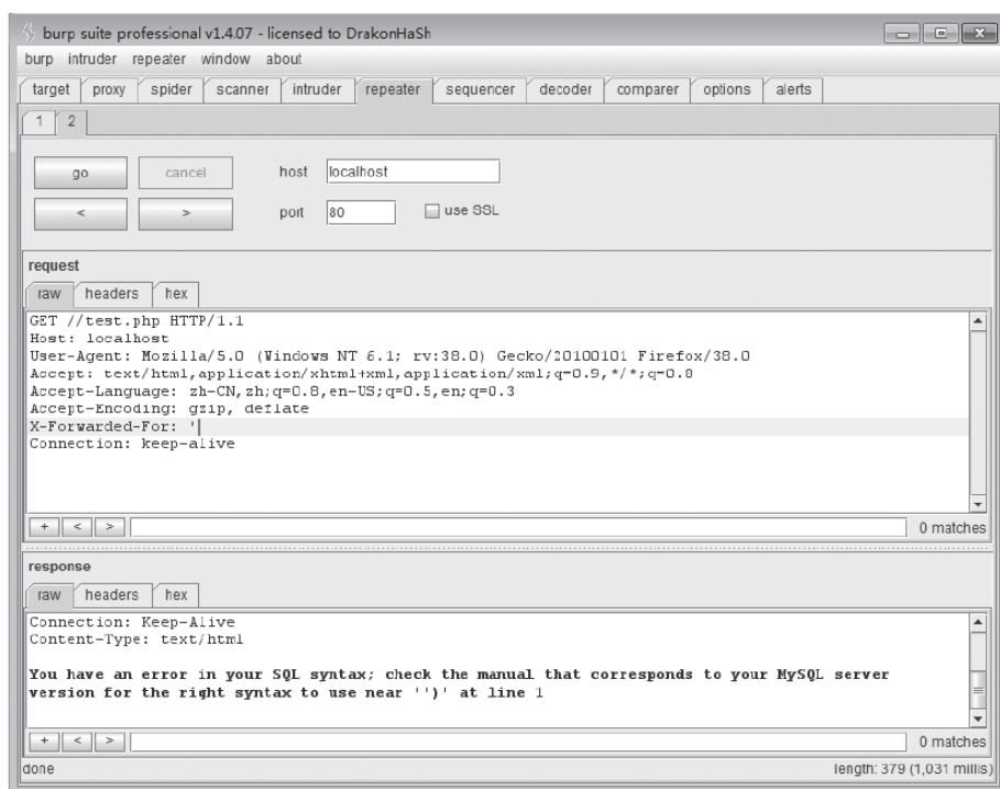
图4-12 http头注入
