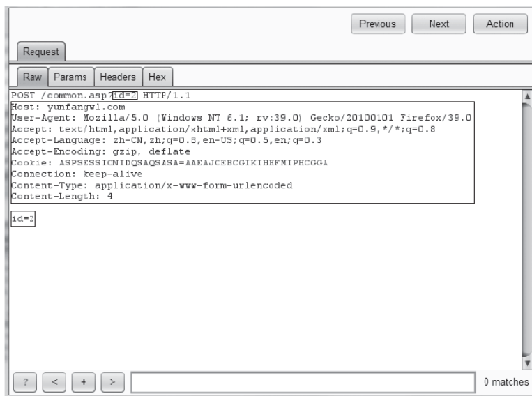
图3-8 分析了http数据包的结构
