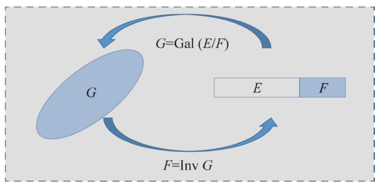
图 8 伽罗瓦群可逆定理示意图
