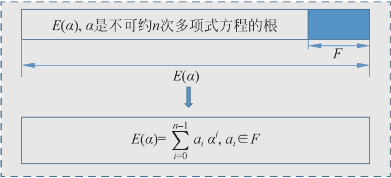
图 1 单代数扩域结构定理示意图
