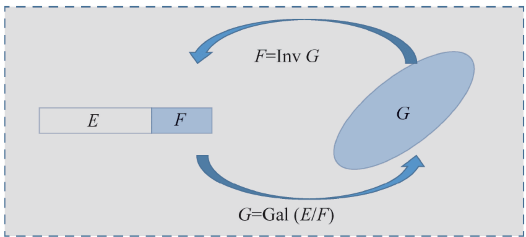
图 7 伽罗瓦子域可逆定理示意图
