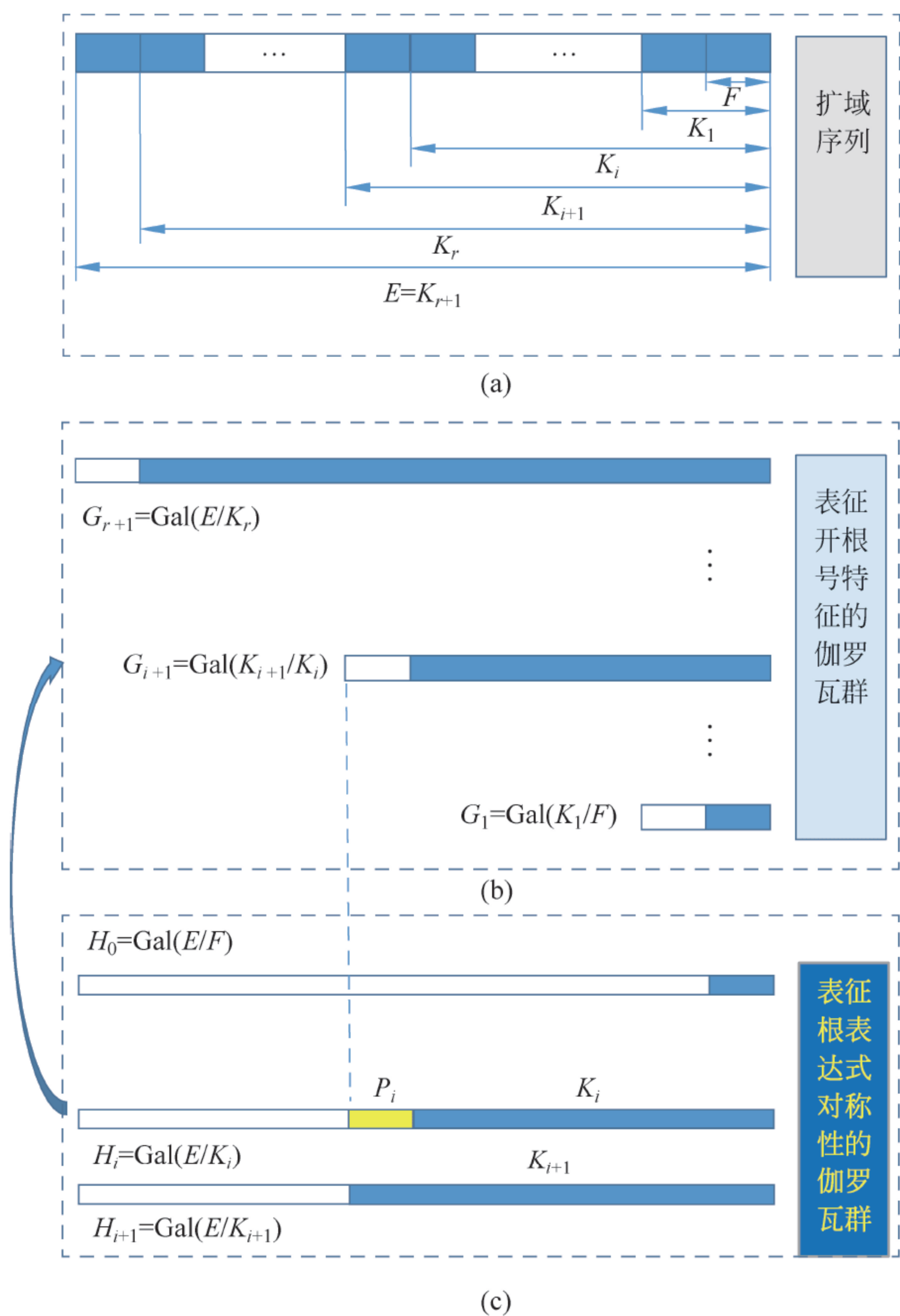
图 5 方程求解所对应扩域序列(a)、表征开根号特征的伽罗瓦群(b),以及表征根表达式的伽罗瓦群之间关系的示意图(c)
