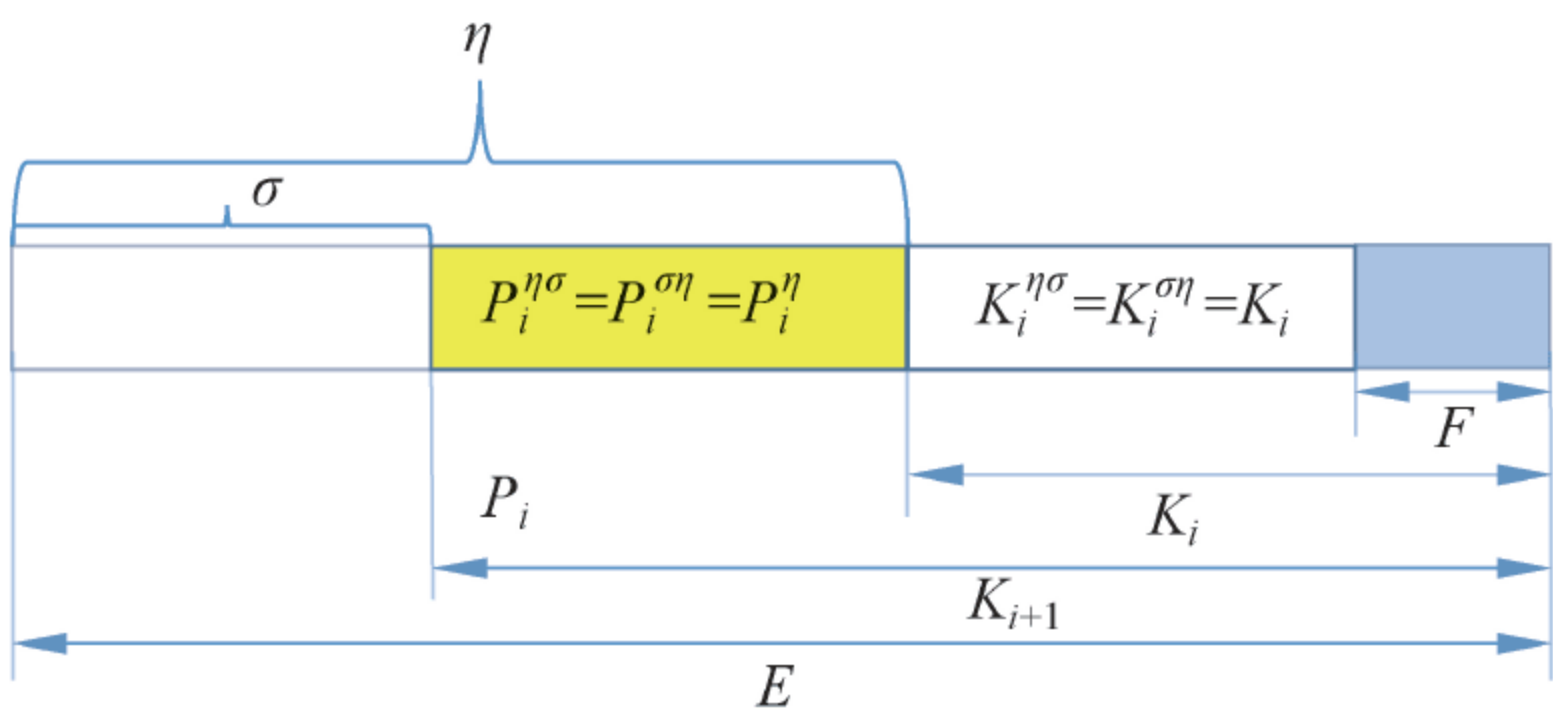
图 6 H_{i+1} 是 H_i 的正规子群理解示意图
