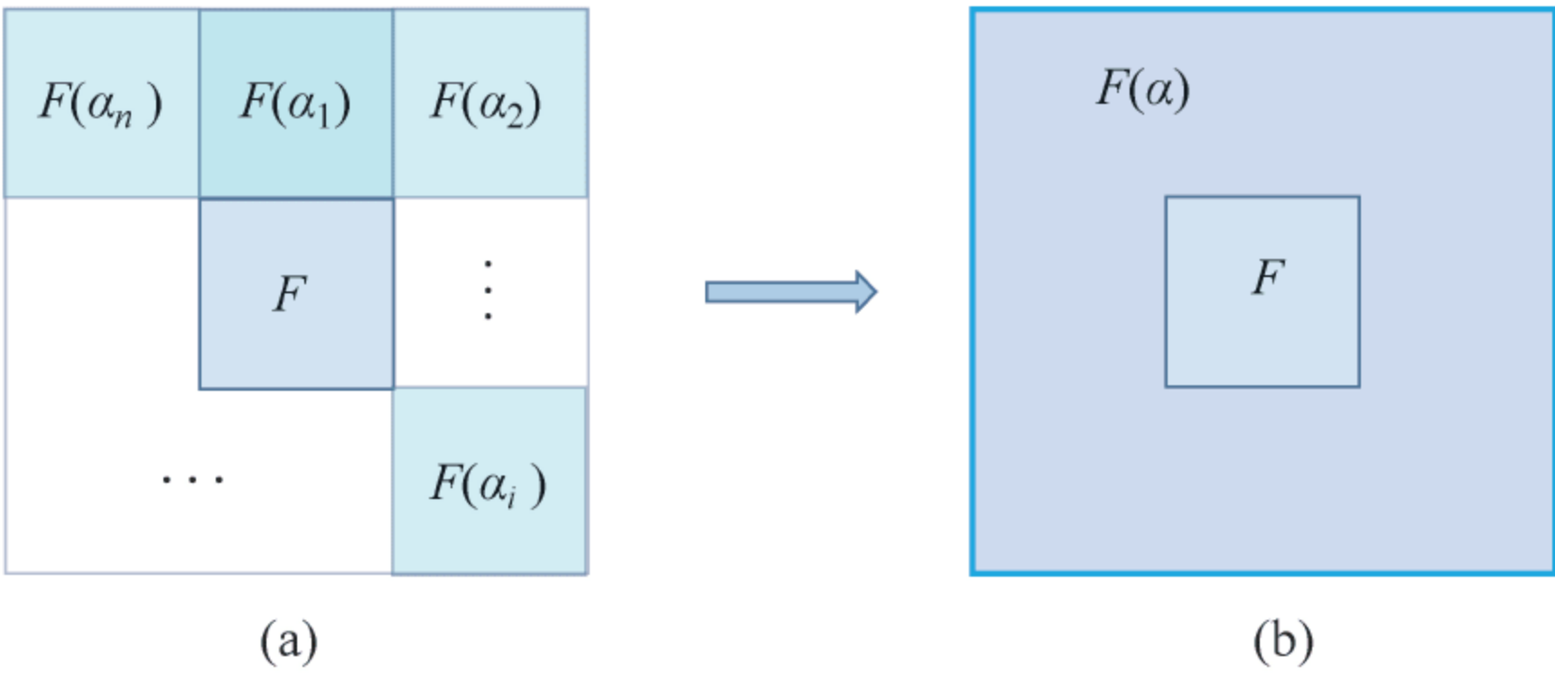
图 3 单代数扩域定理示意图
