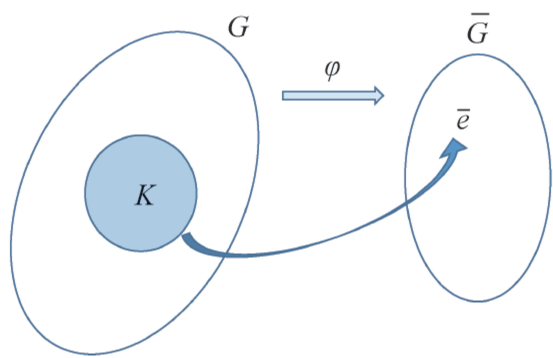
图 4 同态映射示意图
