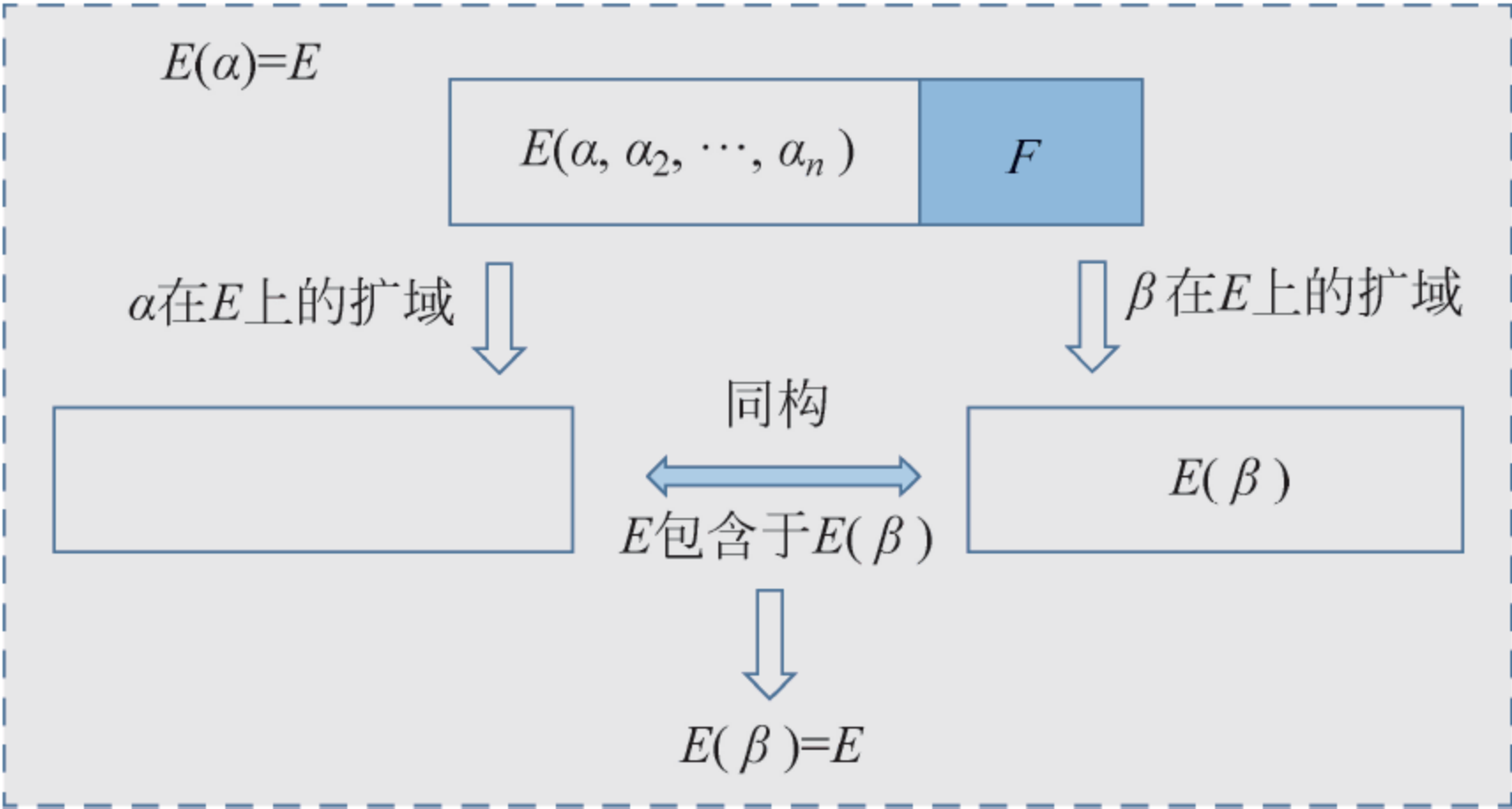
图 2 分裂域属性定理论证示意图
