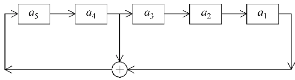
图 4-3 线性反馈移位寄存器(LFSR2)
