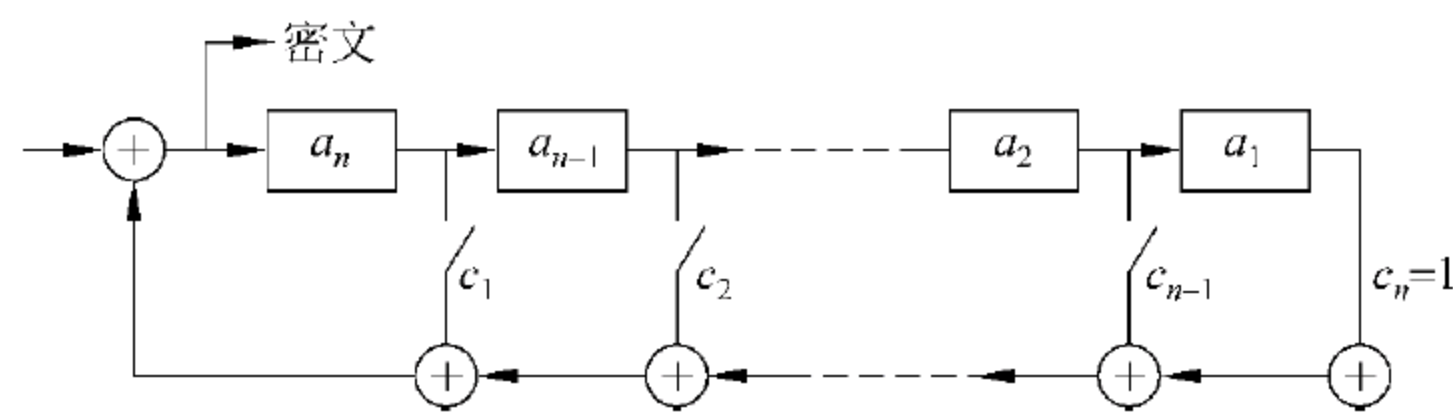
图 4-11 LFSR 1
