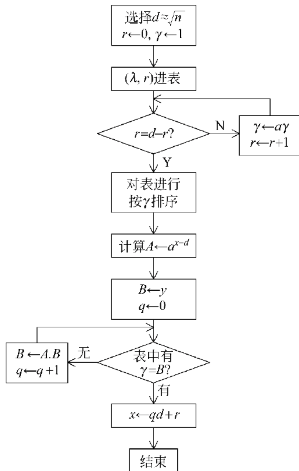
图 7-1 Shank 算法
