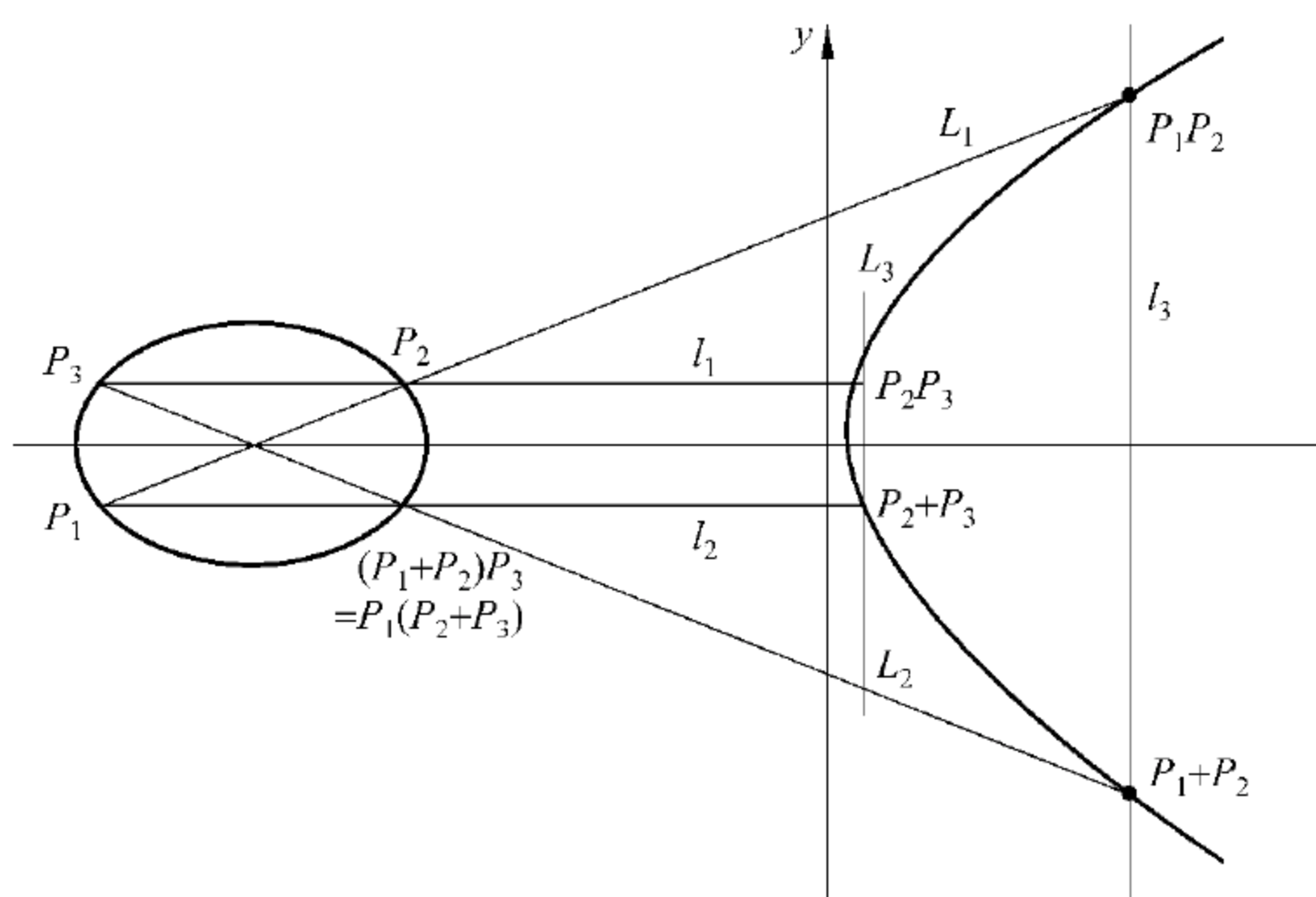
图 8-5 椭圆曲线
