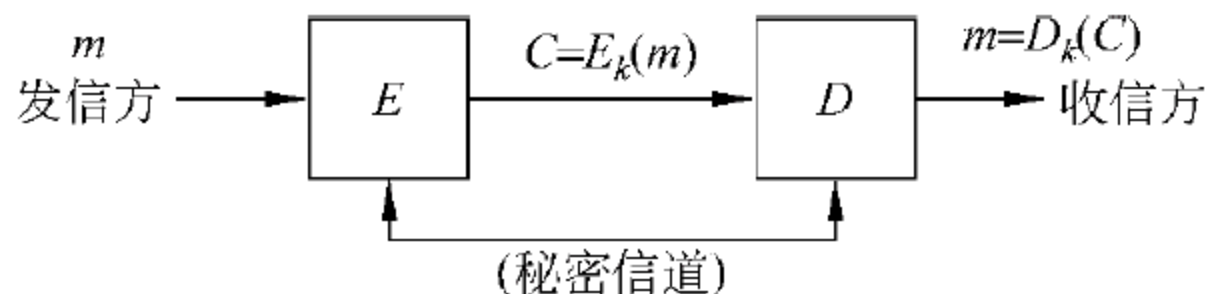
图 1-1 加密图示
