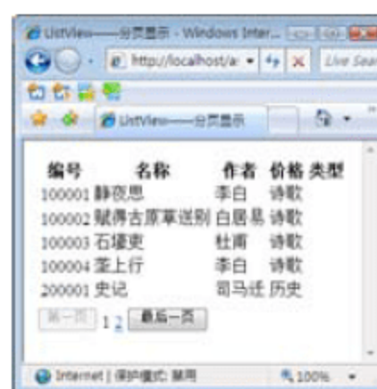
图 7-27 分页显示
