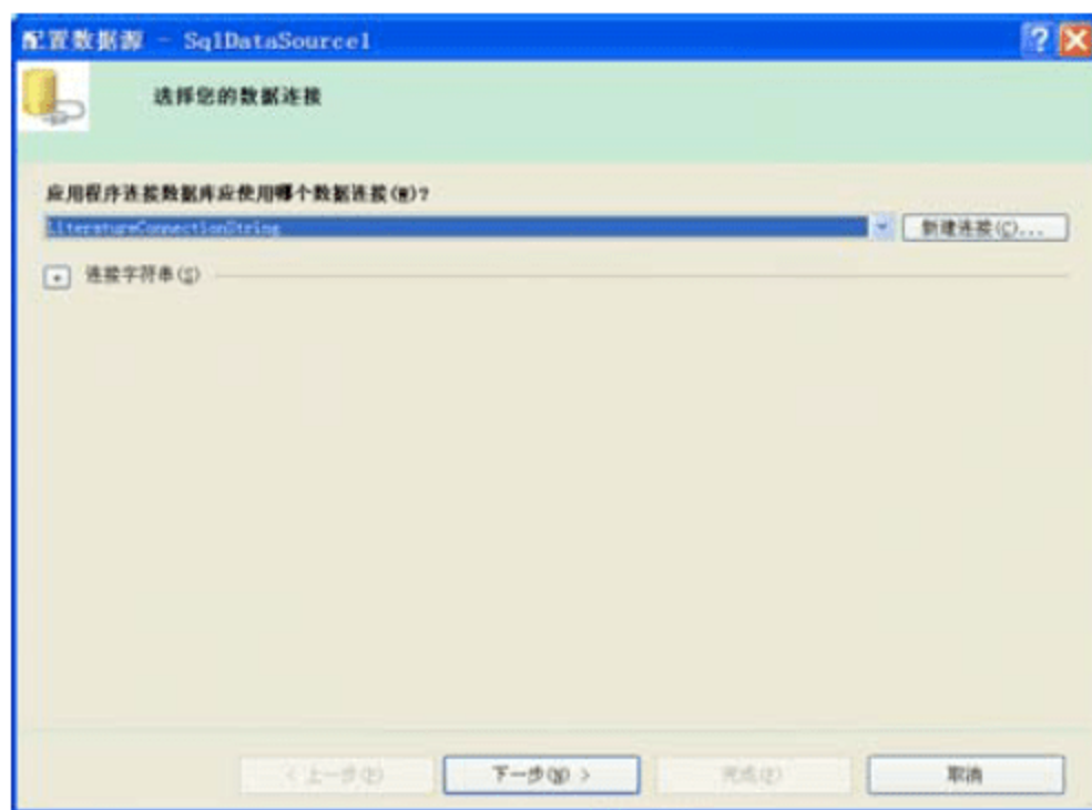
图 7-5 配置数据源(2)
