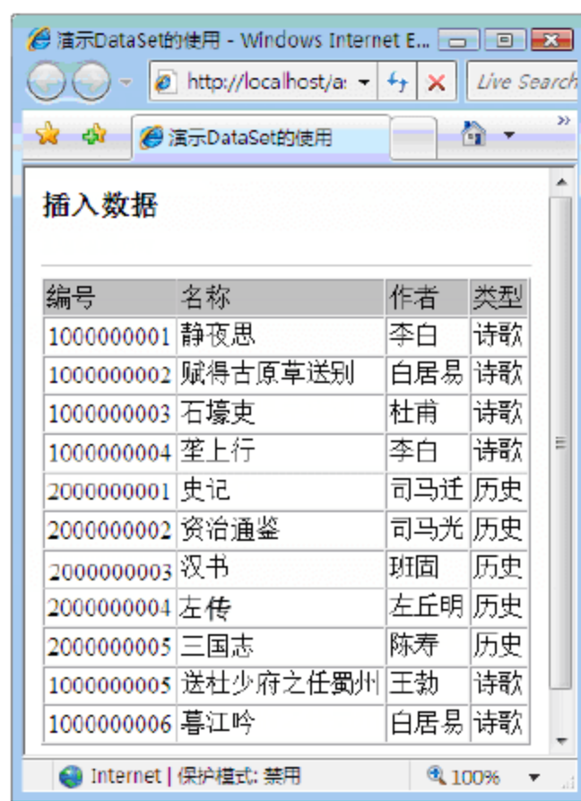
图 6-12 插入数据
