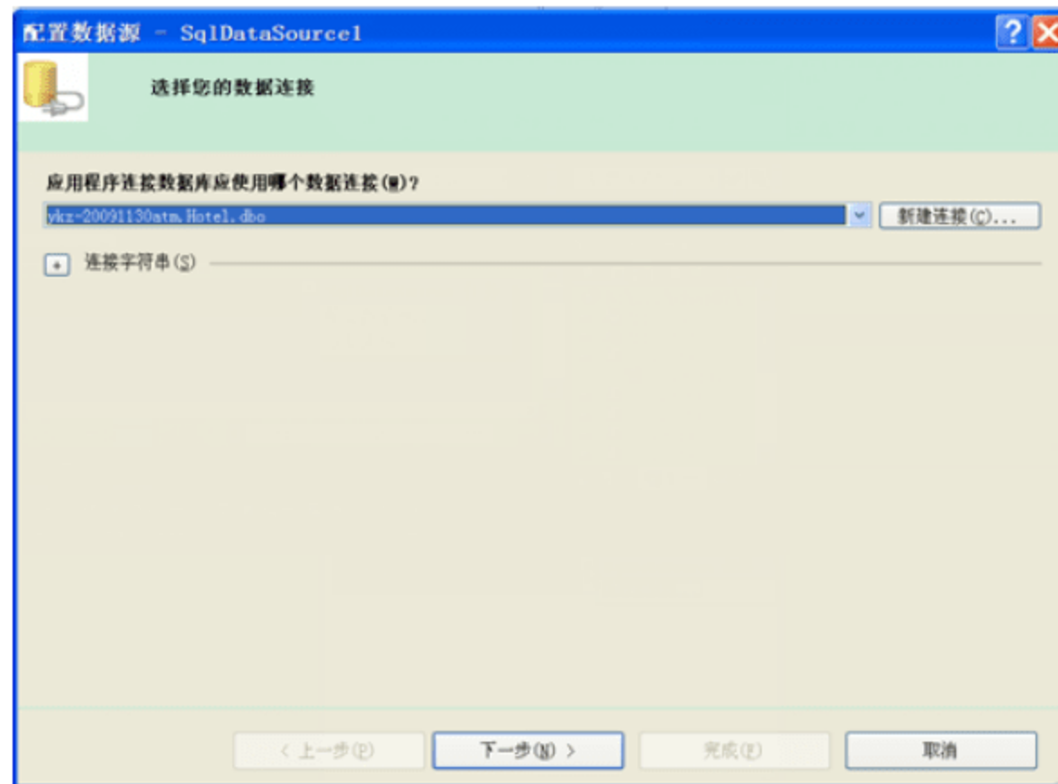
图 7-2 配置数据源(1)
