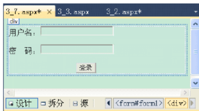
图 3-16 设计视图
