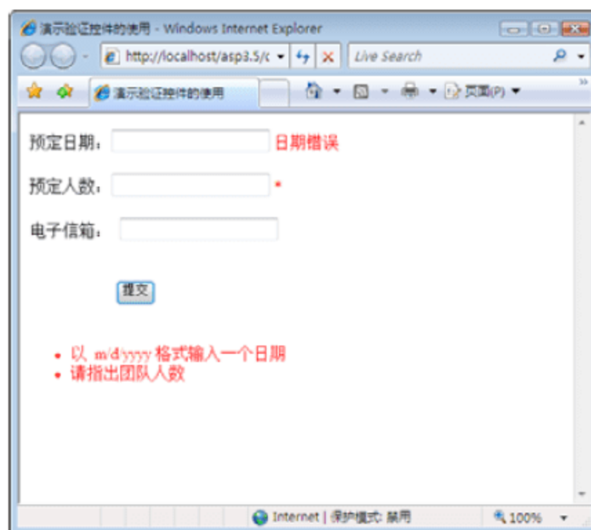
图 5-10 非空验证
