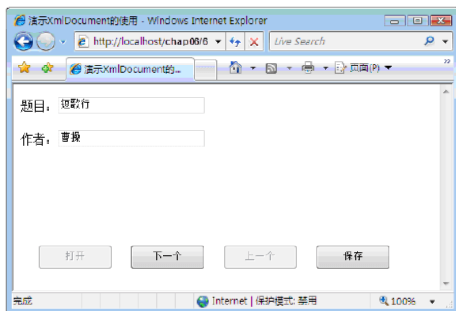
图 6-17 导入文件
