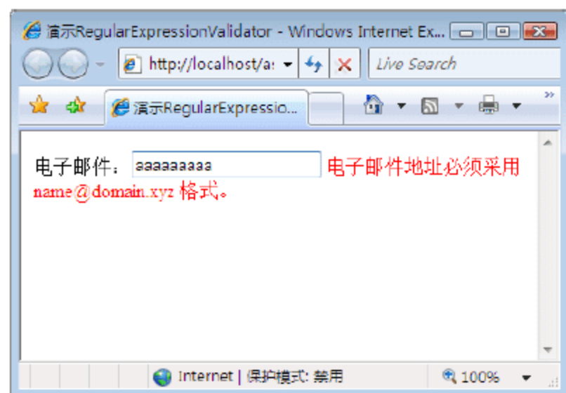
图 5-6 正则表达式
