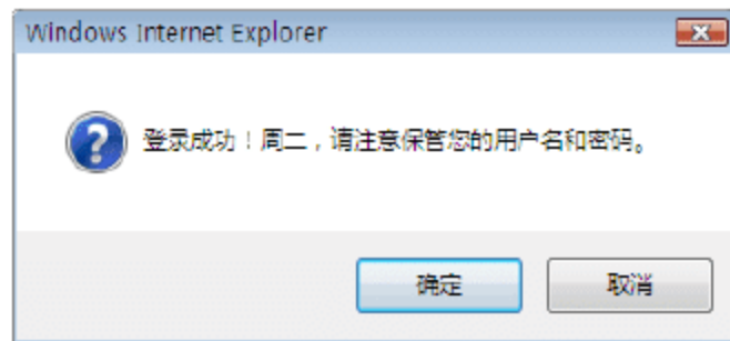
图 3-18 登录成功
