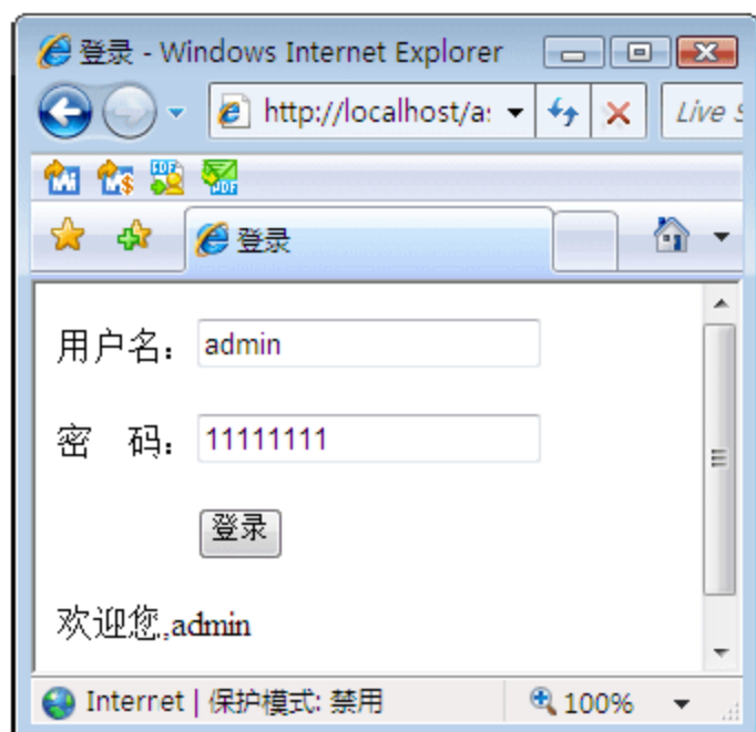
图 10-12 登录成功
