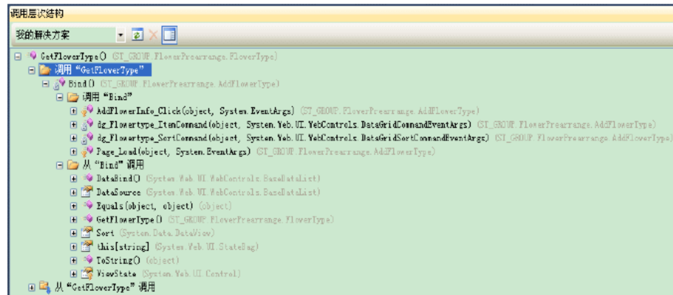
图 1-7 “调用层次结构”窗口
