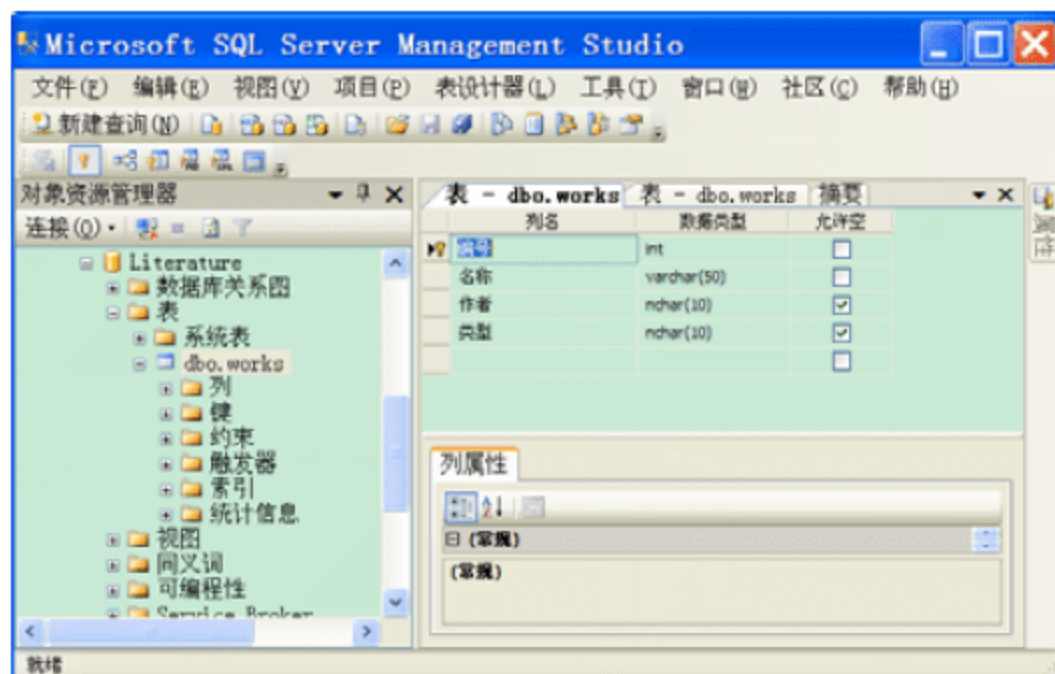
图 6-5 设置主键之后的 Works 表
