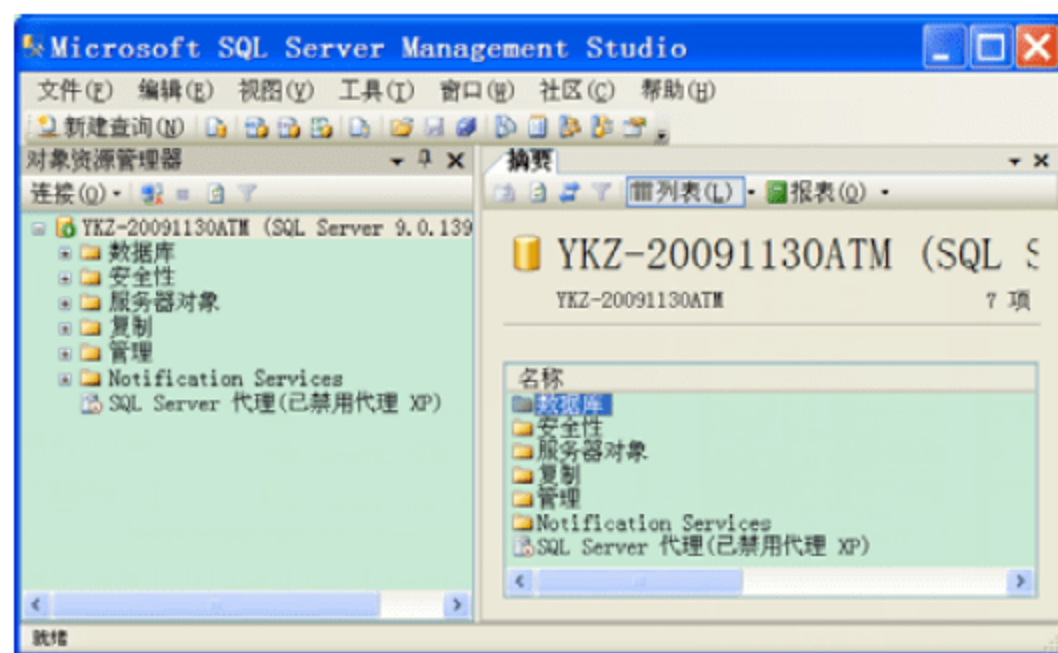
图 6-2 程序主界面
