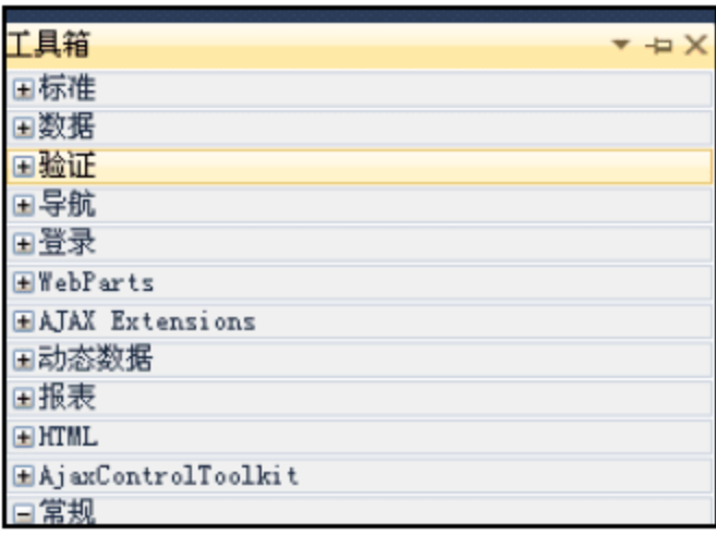
图 1-6 工具箱
