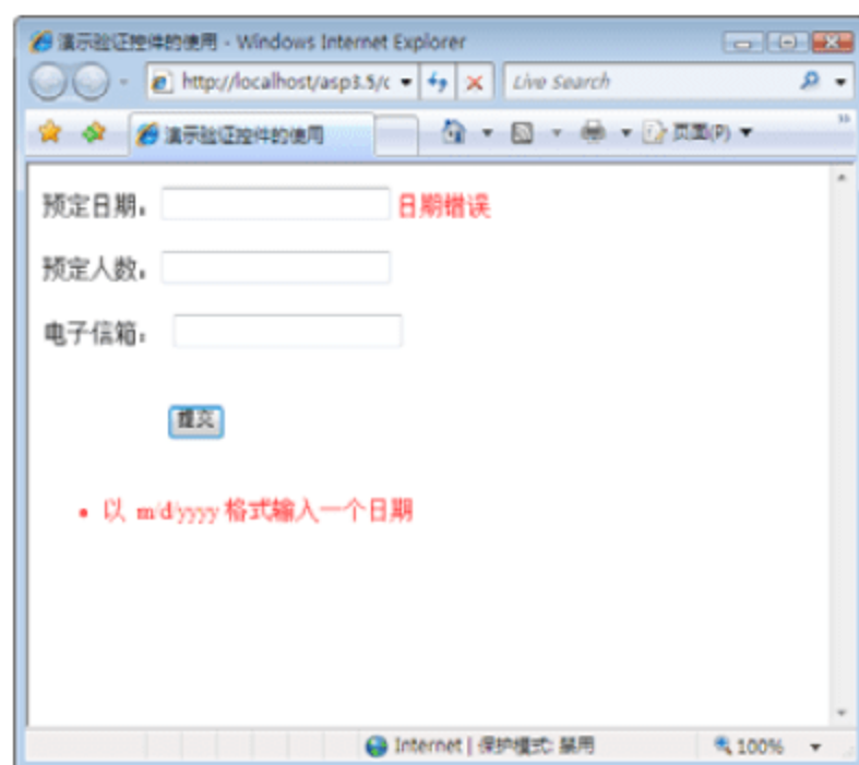
图 5-13 只验证日期
