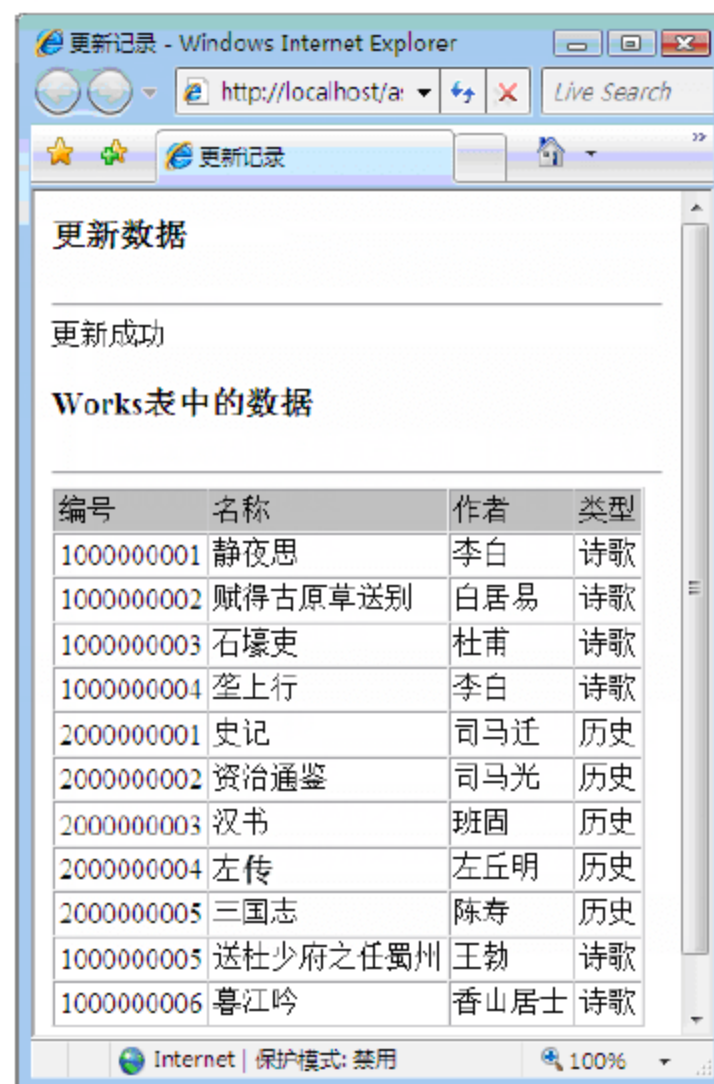
图 6-13 更新数据
