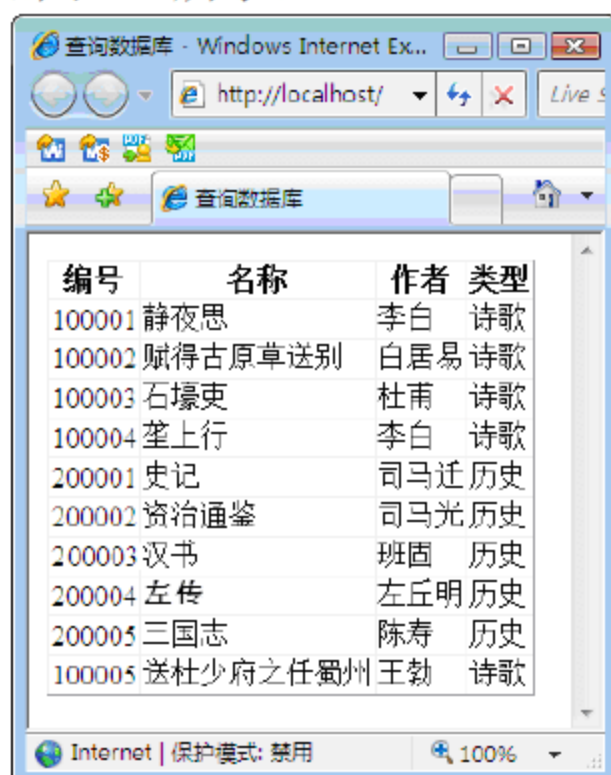
图 8-8 查询数据库
