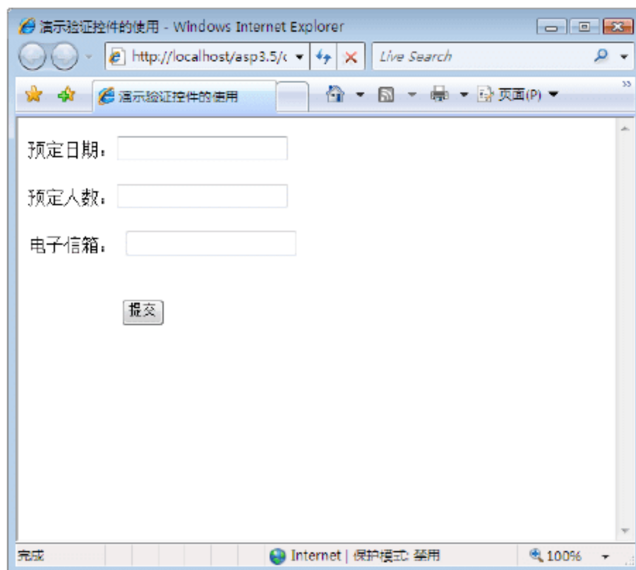
图 5-9 初始界面
