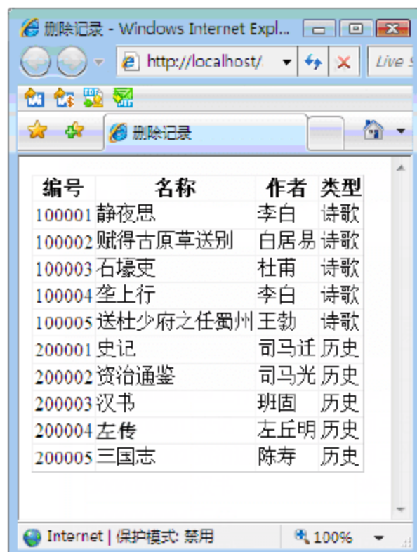
图 8-11 删除记录
