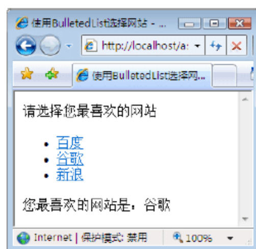
图 4-21 演示 BulletedList
