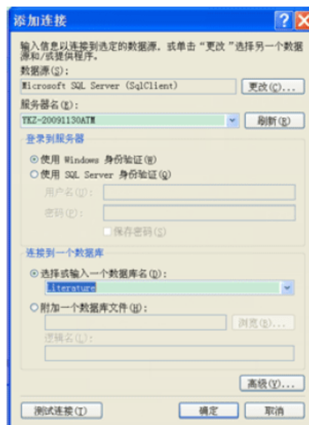
图 7-4 添加连接
