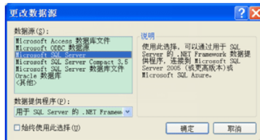
图 7-3 选择数据源
