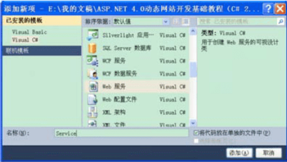
图 10-5 选择位置
