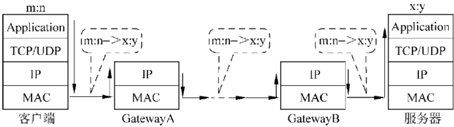
图 3-3 非代理模式下的网络协议处理流程
