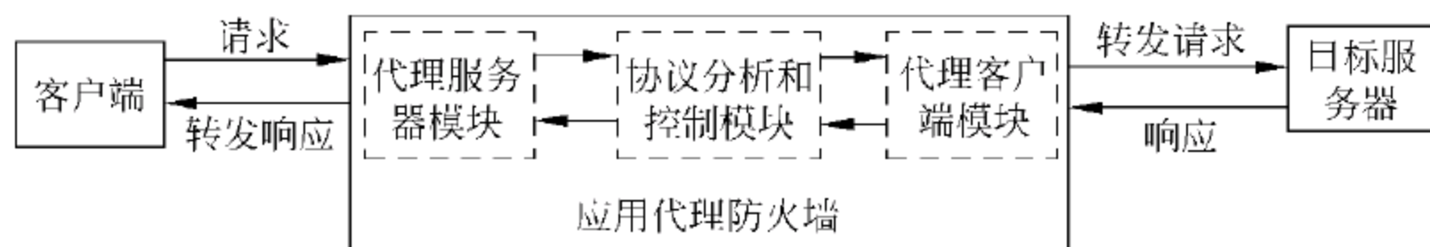
图 4-1 应用代理防火墙的结构和工作原理
