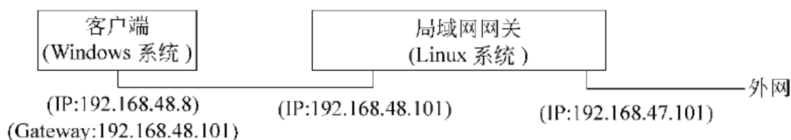
图 13-2 透明代理防火墙的测试网络结构
