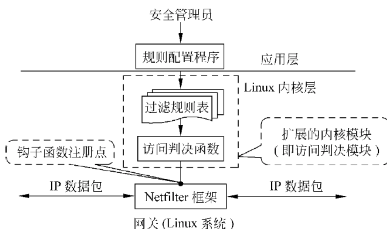
图 5-5 基于内核模块的包过滤防火墙的逻辑结构和运行原理
