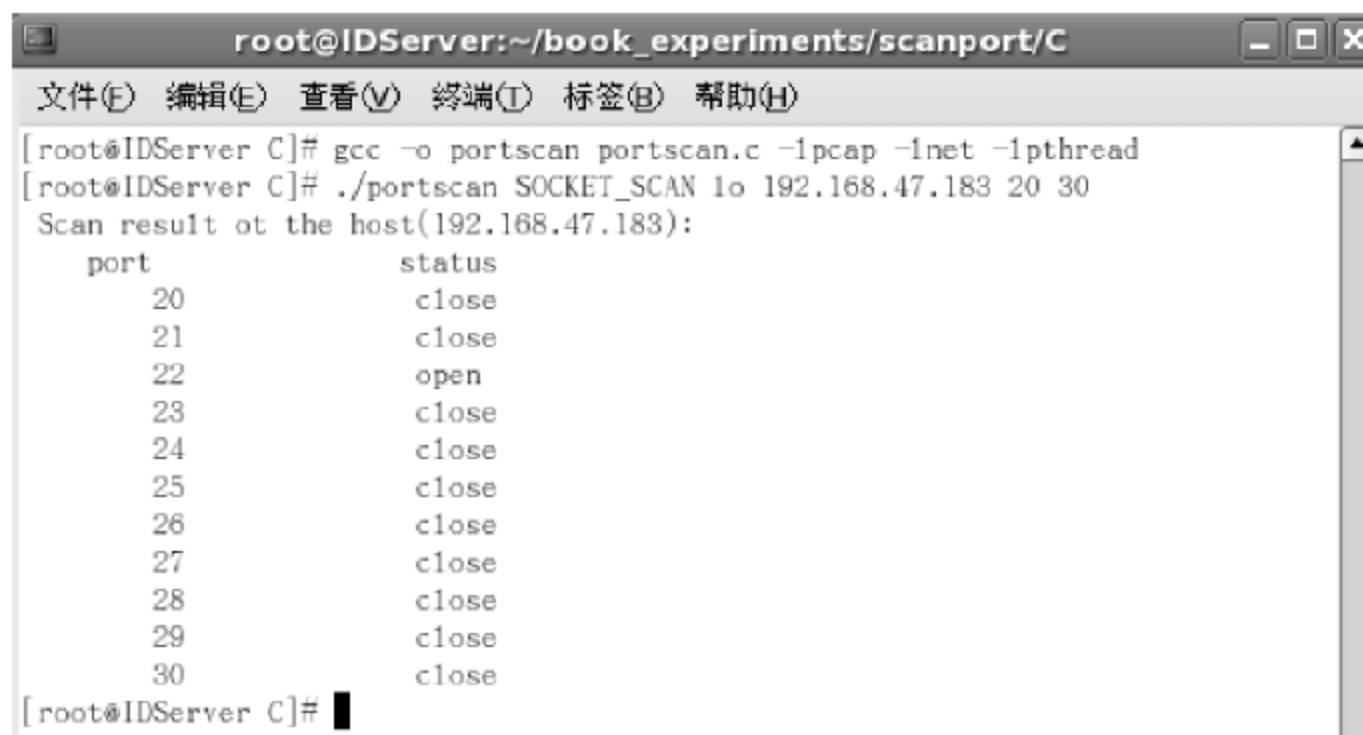
图 14-2 对 Linux 系统的全连接扫描测试结果
