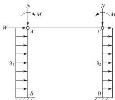
图 4.16 单层弹性方案房屋计算简图
