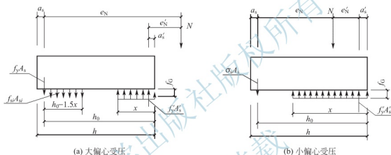
图 3.29 矩形截面偏心受压构件正截面承载力计算简
