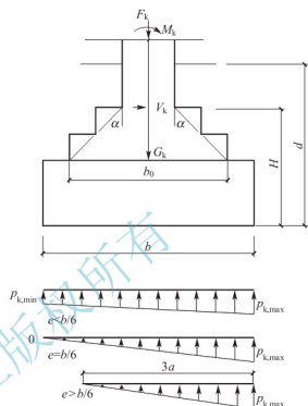
图 4.43 偏心受压基础的计算简图
