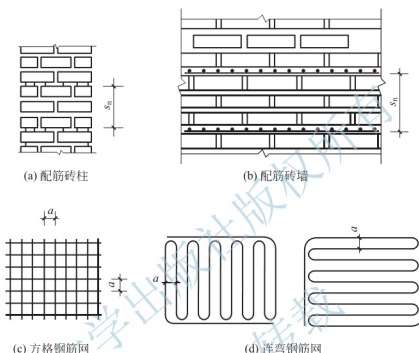
图 3.23 网状配筋砖砌体
