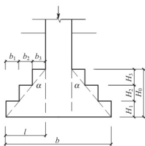
图 4.39 刚性基础
