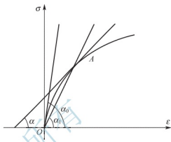
图 2.13 砌体弹性模量的表示方法
