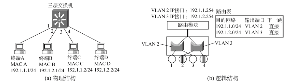
图 9.11 网络结构
