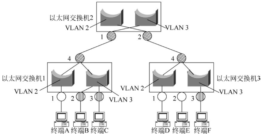
图 2.13 VLAN 配置
