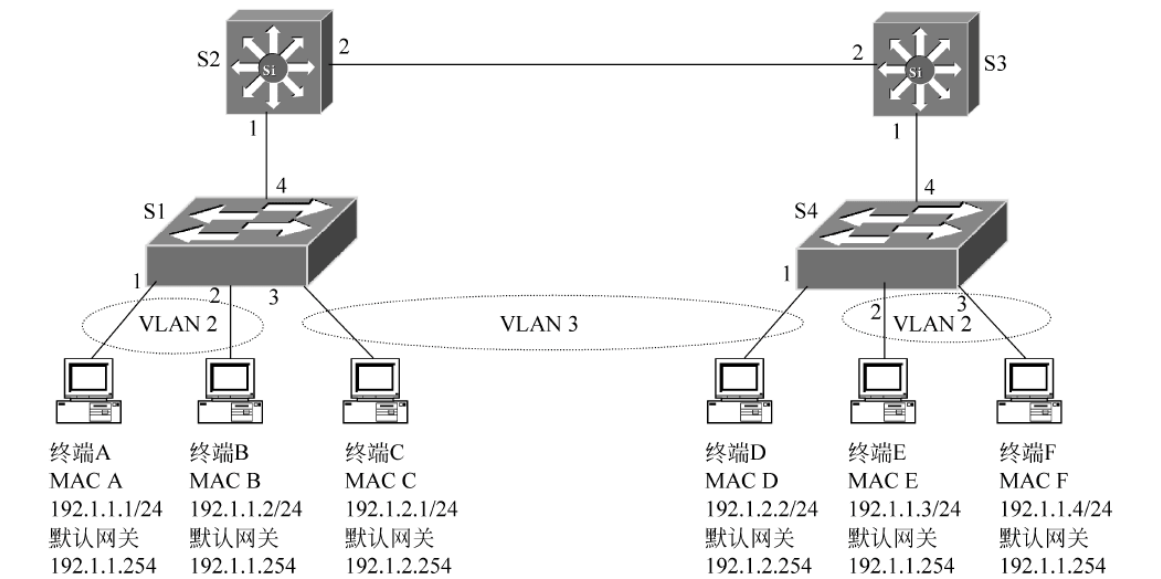
图 9.19 题 9.8 图
