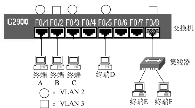
图 2.42 题 2.11 图
