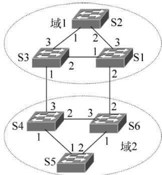
图 3.22 网络结构
