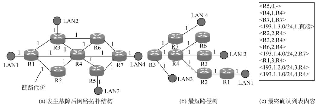
图 6.25 以路由器 R5 为根的最短路径树
