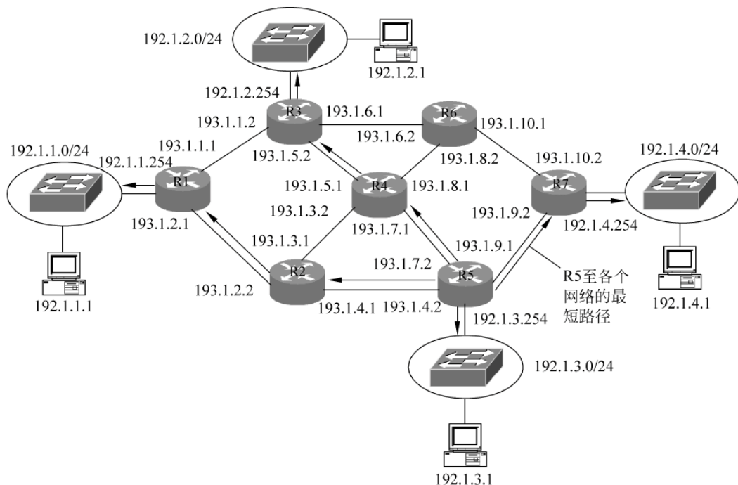
图 5.19 人工配置静态路由表过程
