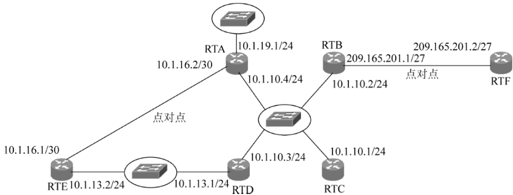
图 6.22 网络结构
