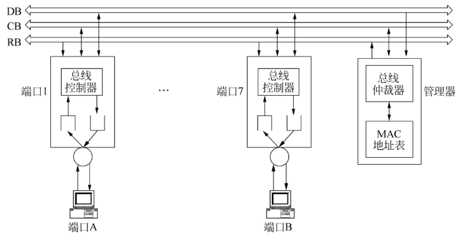
图 1.24 共享总线交换结构
