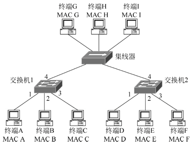
图 1.34 题 1.25 图
