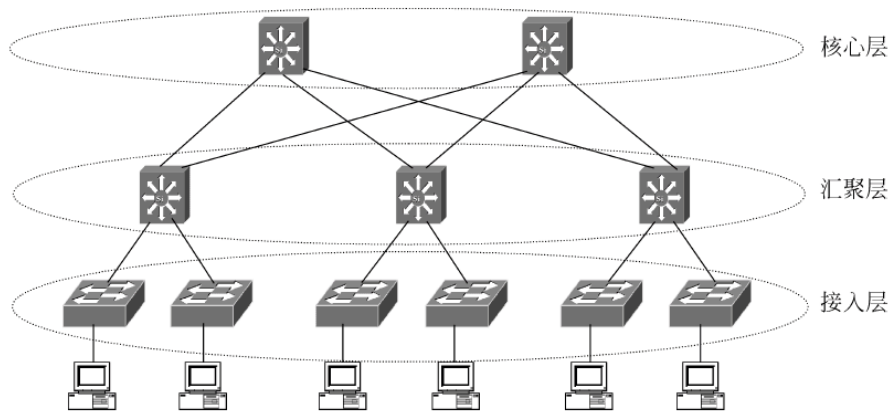
图 9.5 校园网结构
