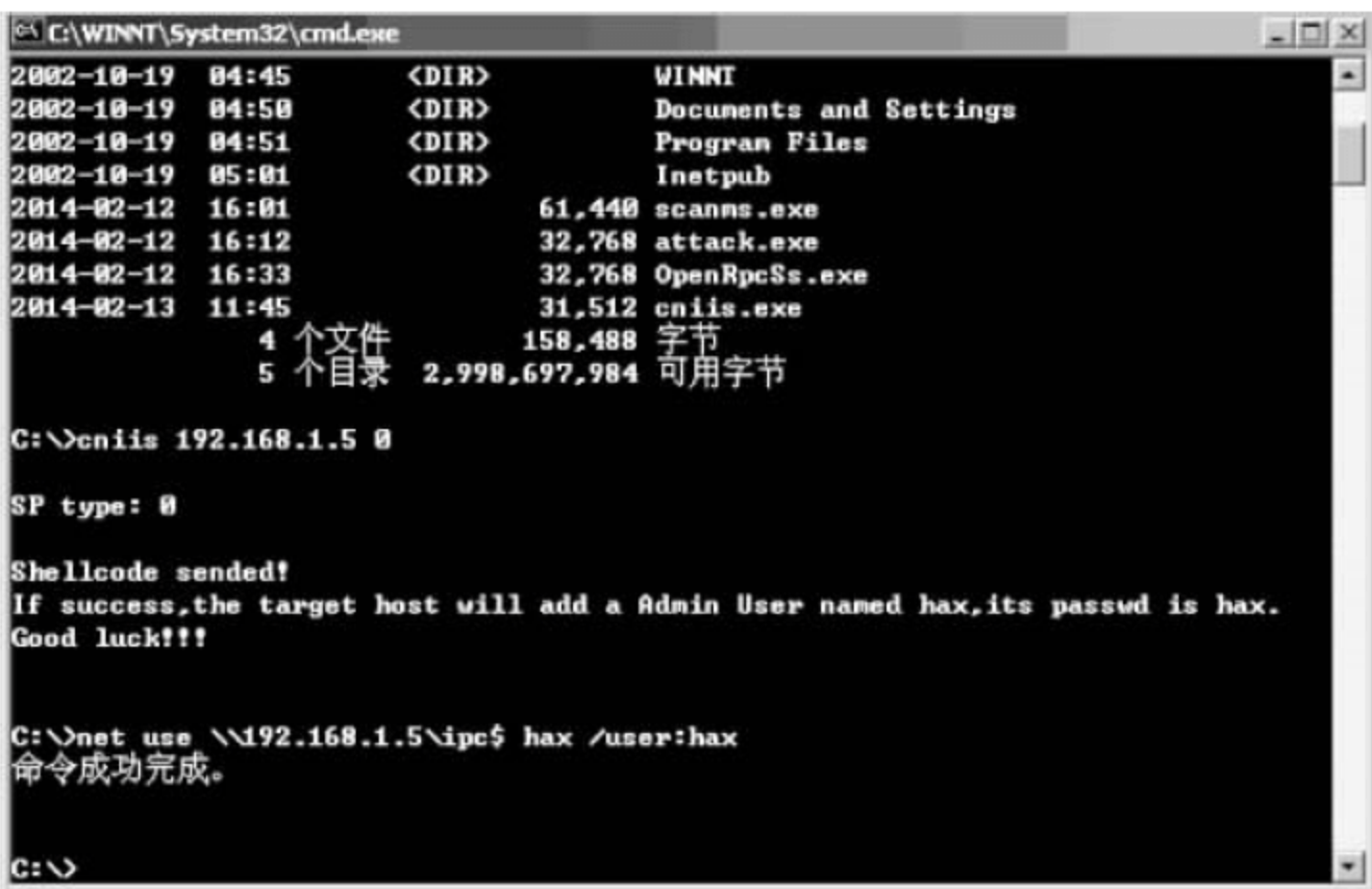
图 6-34 利用打印漏洞
