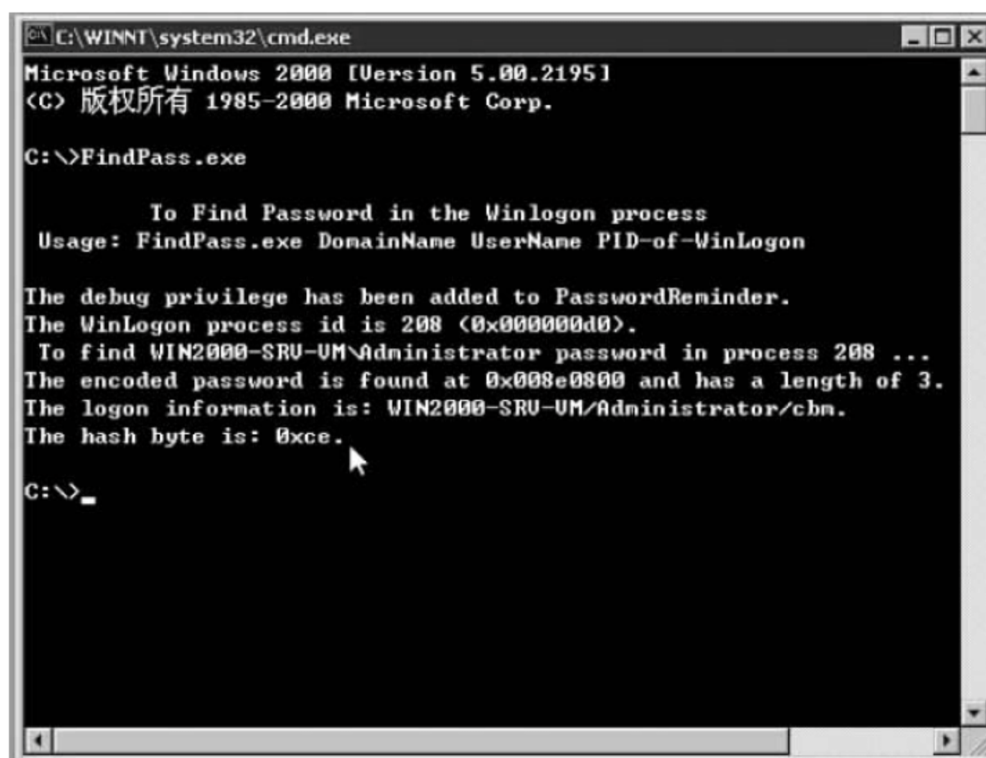
图 9-128 解密出来用户名和密码
