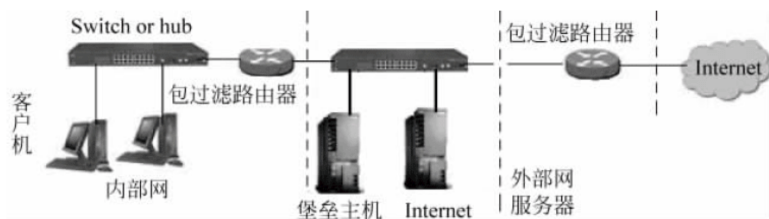
图 5-5 屏蔽子网模型
