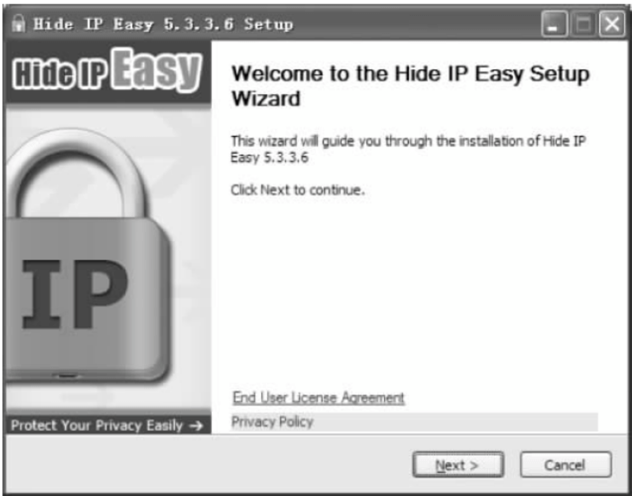
图 9-92 安装界面
