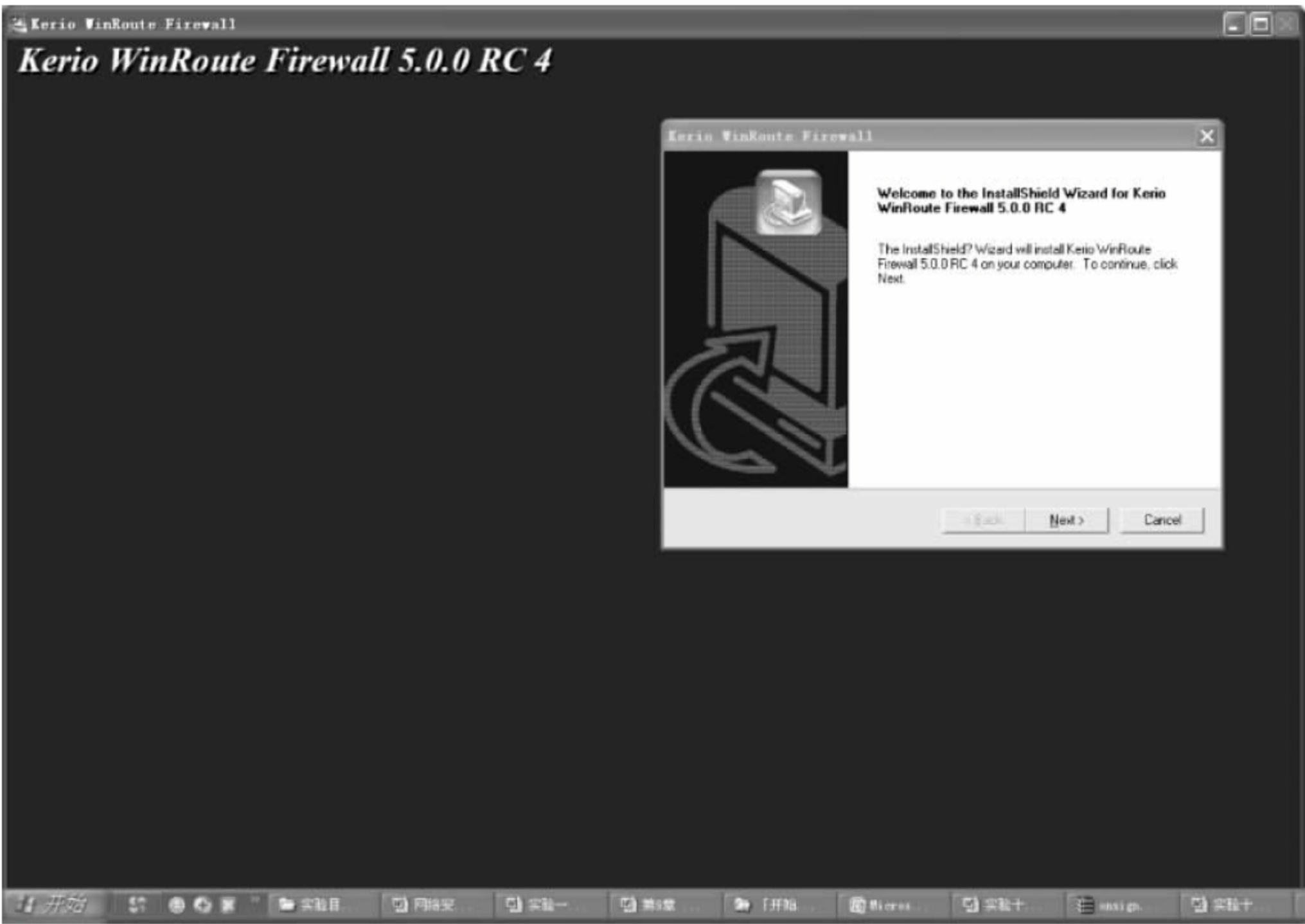
图 9-69 安装界面
