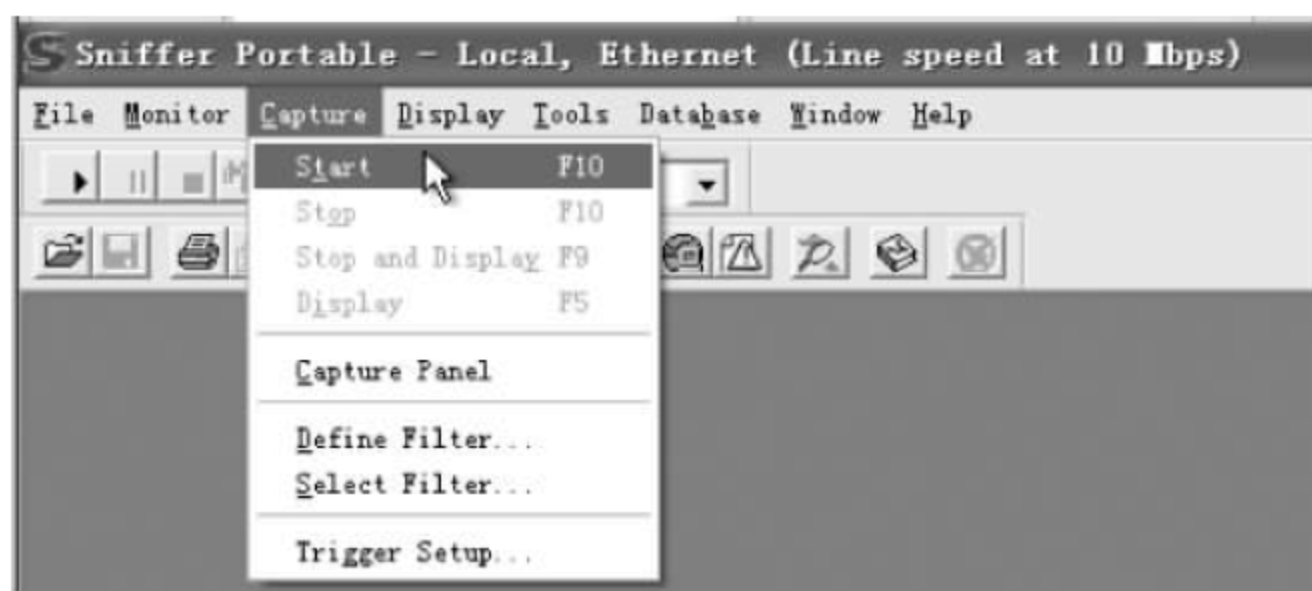
图 9-11 启动抓包
