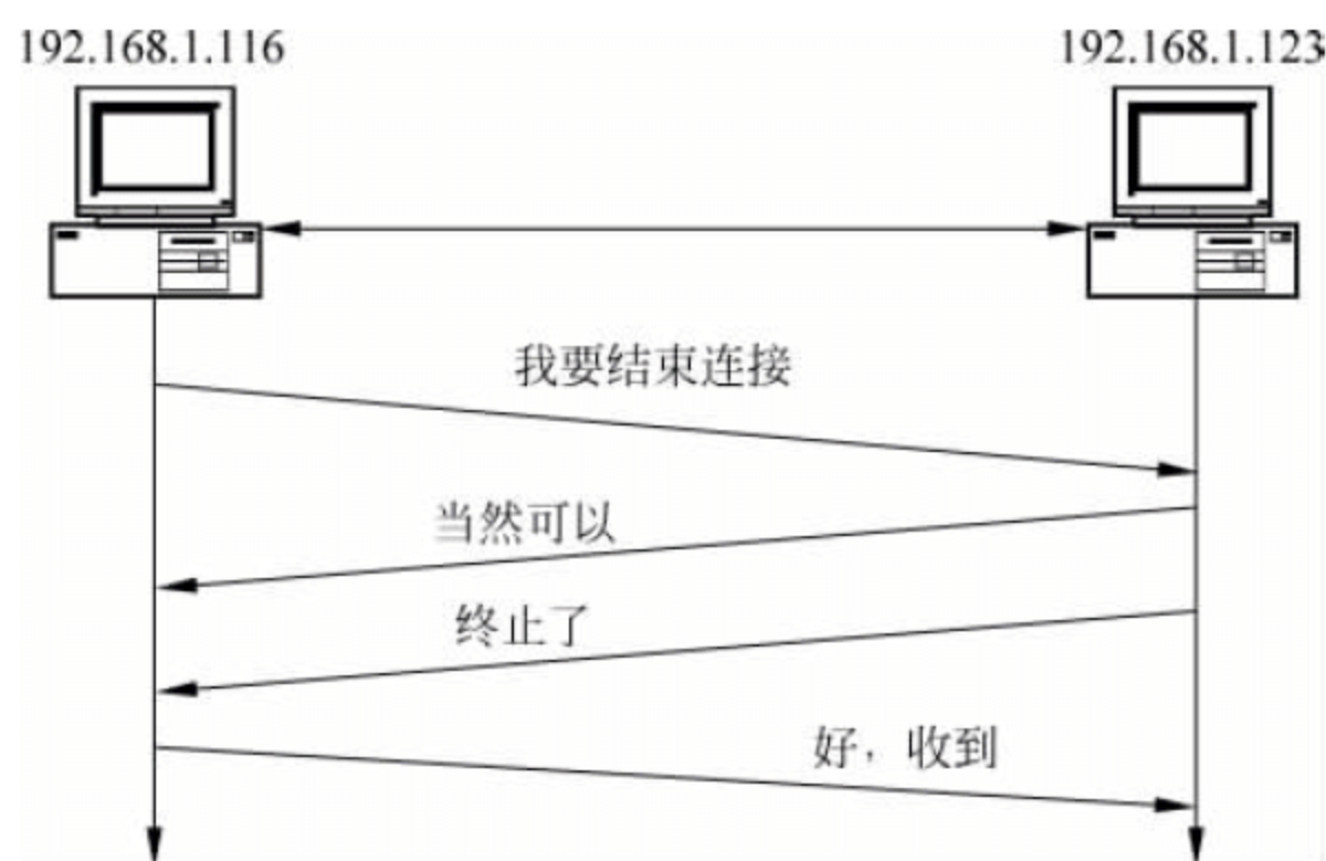
图 2-6 4 次挥手
