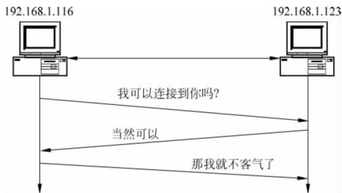
图 2-5 三次握手
