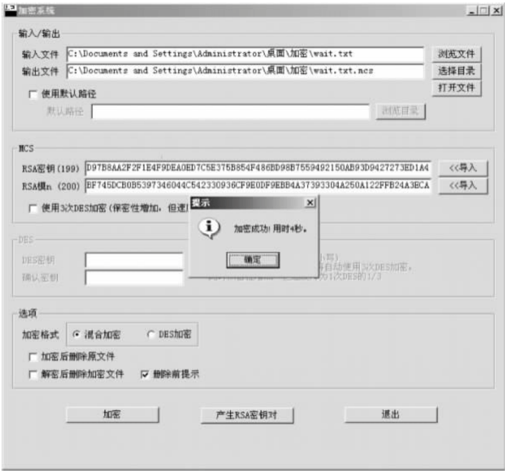
图 9-55 加密过程
