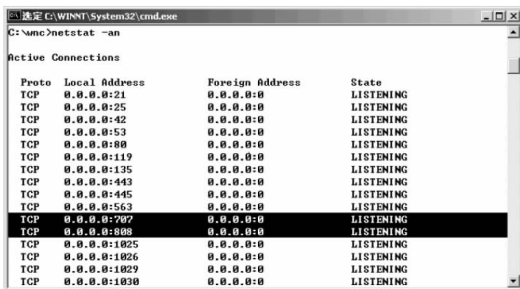
图 8-9 端口开启
