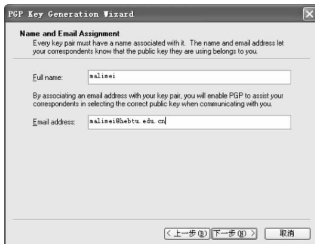
图 4-12 用户信息
