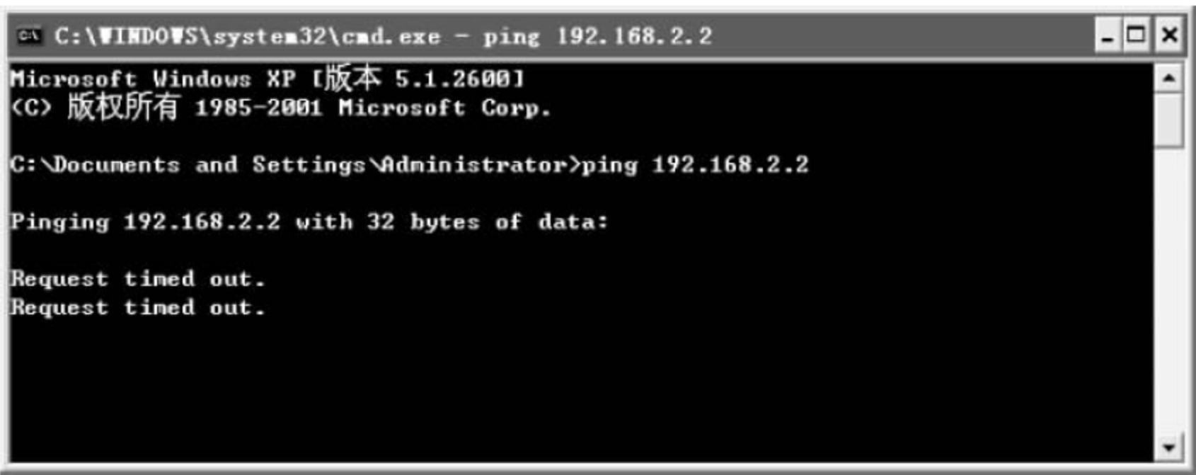
图 9-78 ping 服务器
