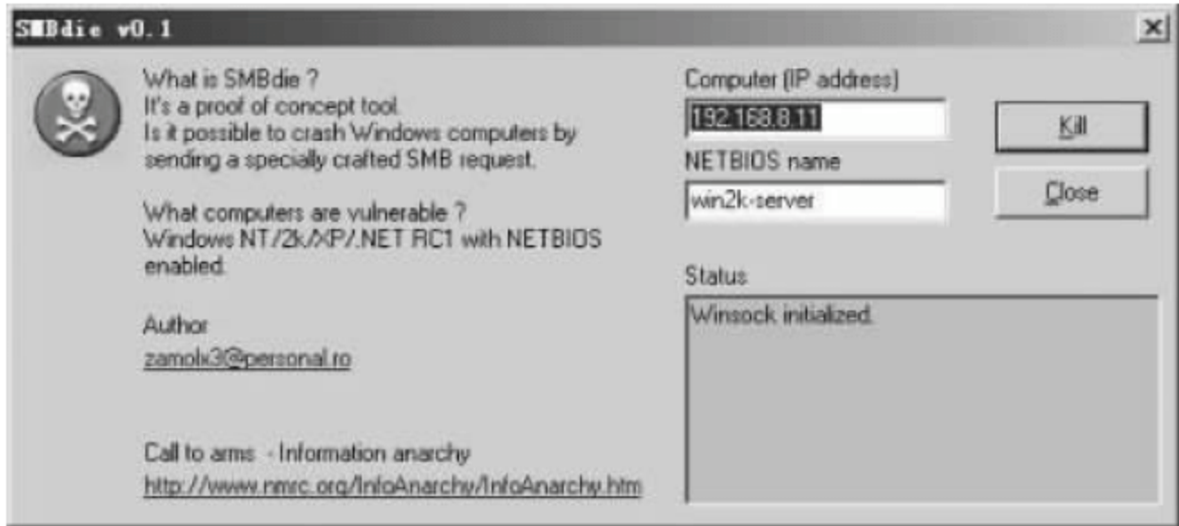
图 9-150 主界面
