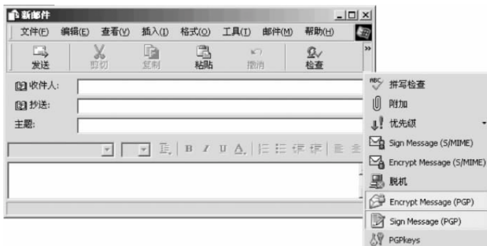
图 9-65 加密邮件
