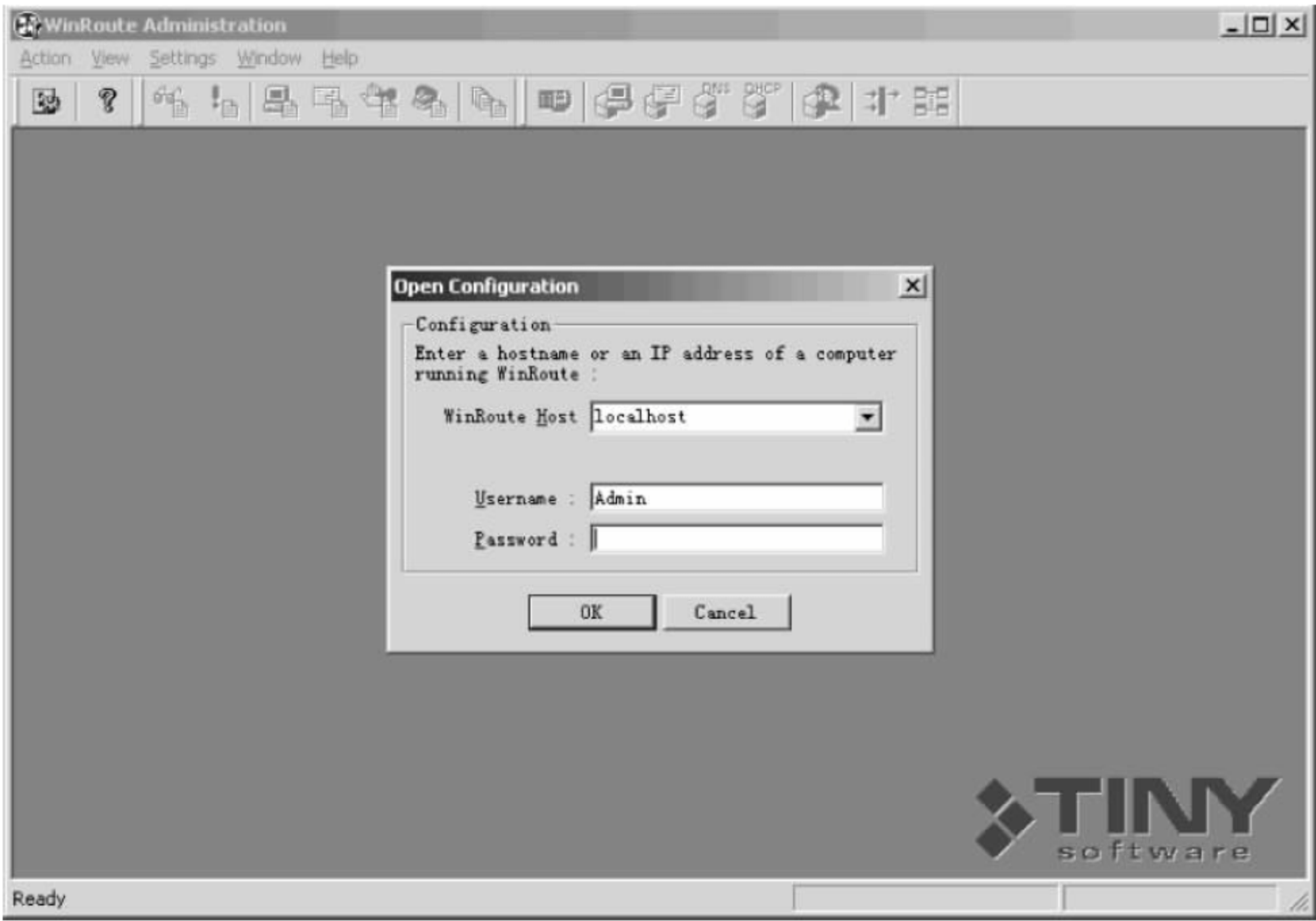
图 9-70 登录界面
