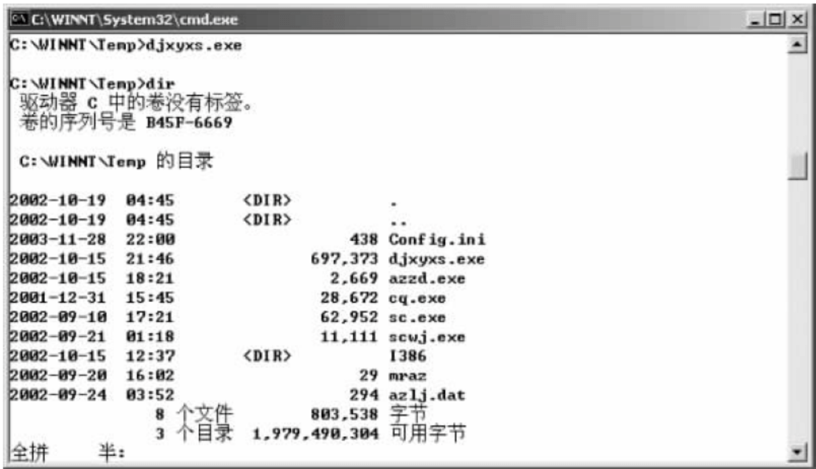
图 9-173 目录列表
