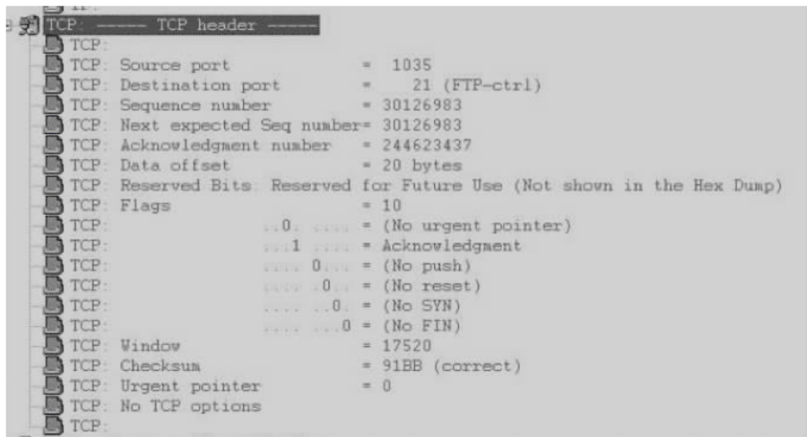
图 9-31 第三次握手
