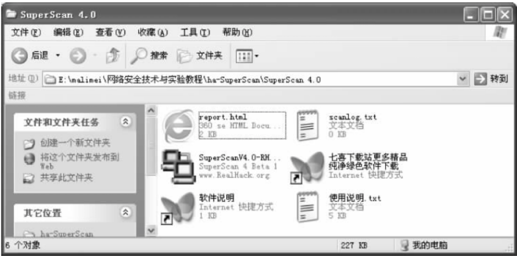
图 9-126 安装的软件
