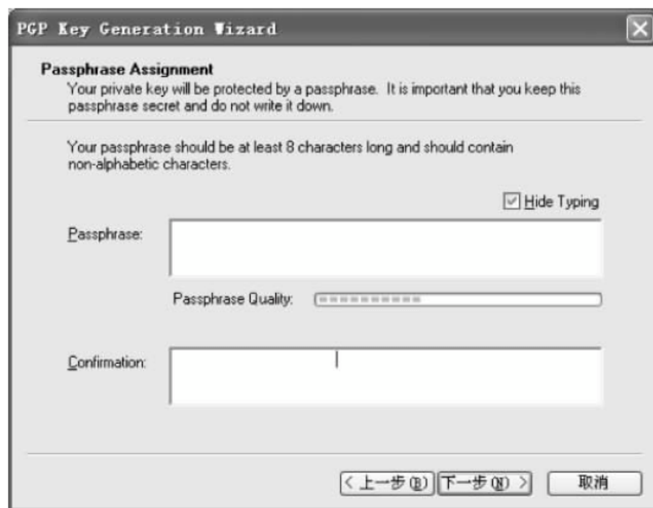
图 4-13 输入密码
