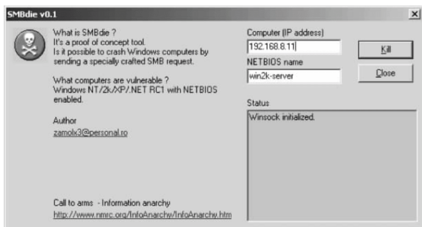
图 6-32 SMB 界面
