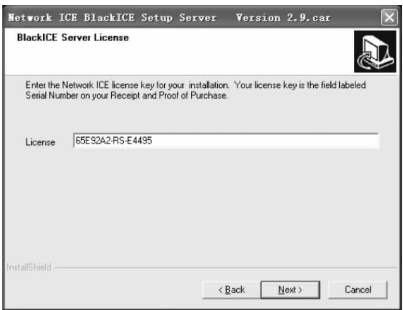
图 9-84 输入序列号
