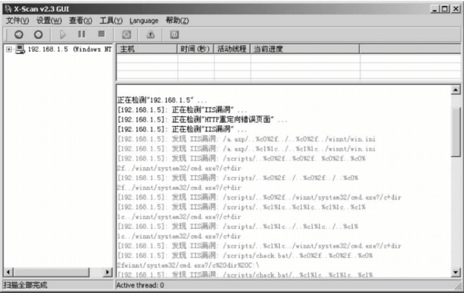
图 6-11 扫描的结果
