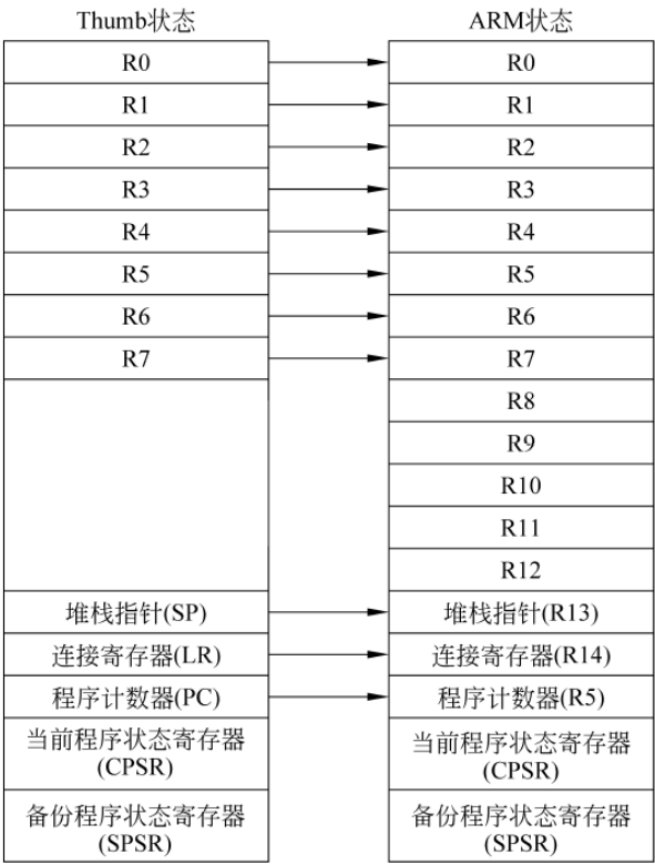
图 3-1 Thumb 寄存器在 ARM 寄存器上的映射
