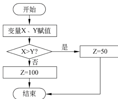
图 3-3 分支程序设计举例—程序流程图
