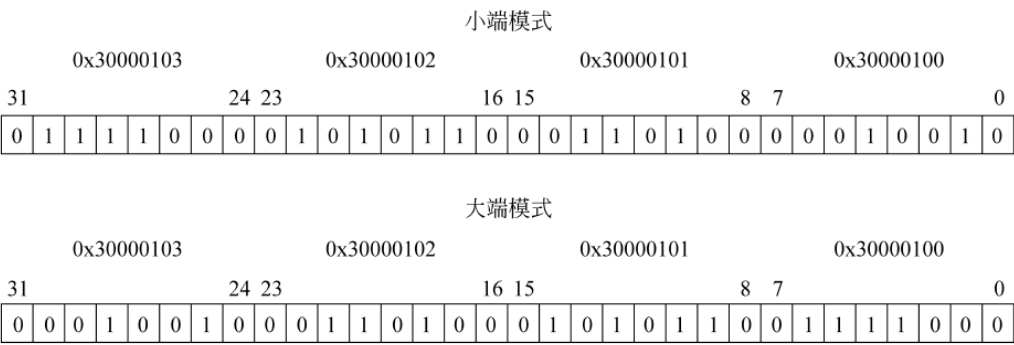
图 2-3 两种存储模式
