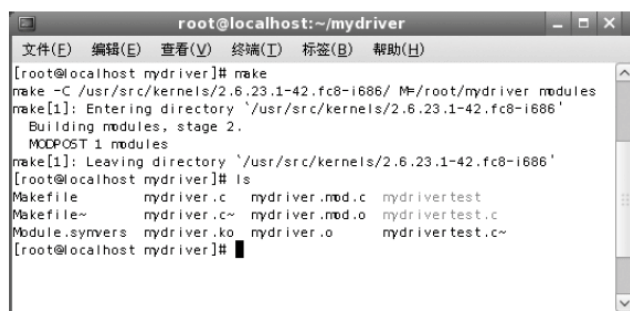
图 8-22 编译结果
