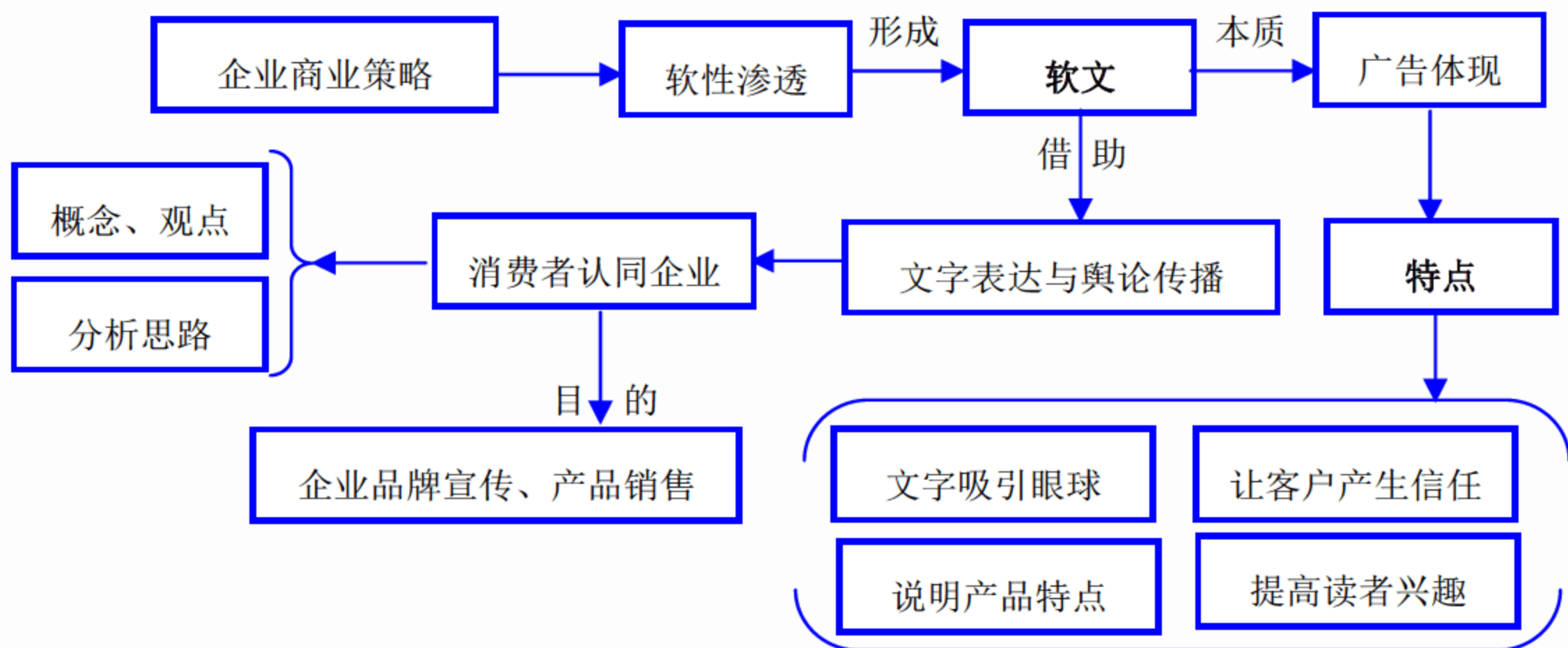
图 4-24 软文的形成
