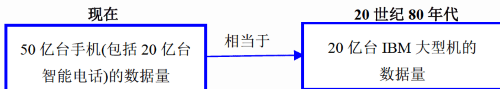
图 1-4 数据量对比
