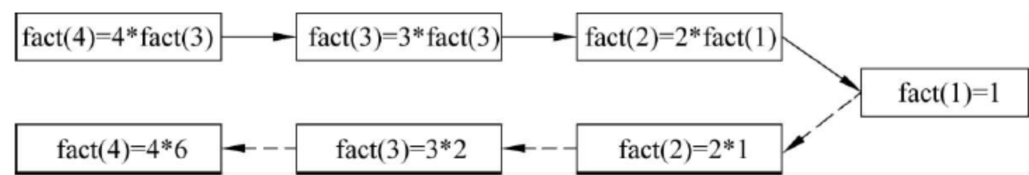
图 7.2 fact(n)的递归求解过程
