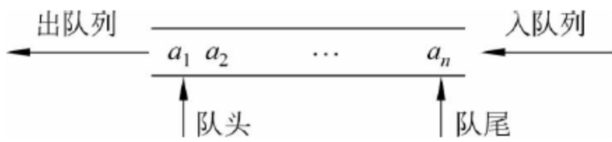
图 6.3 队列的逻辑结构
