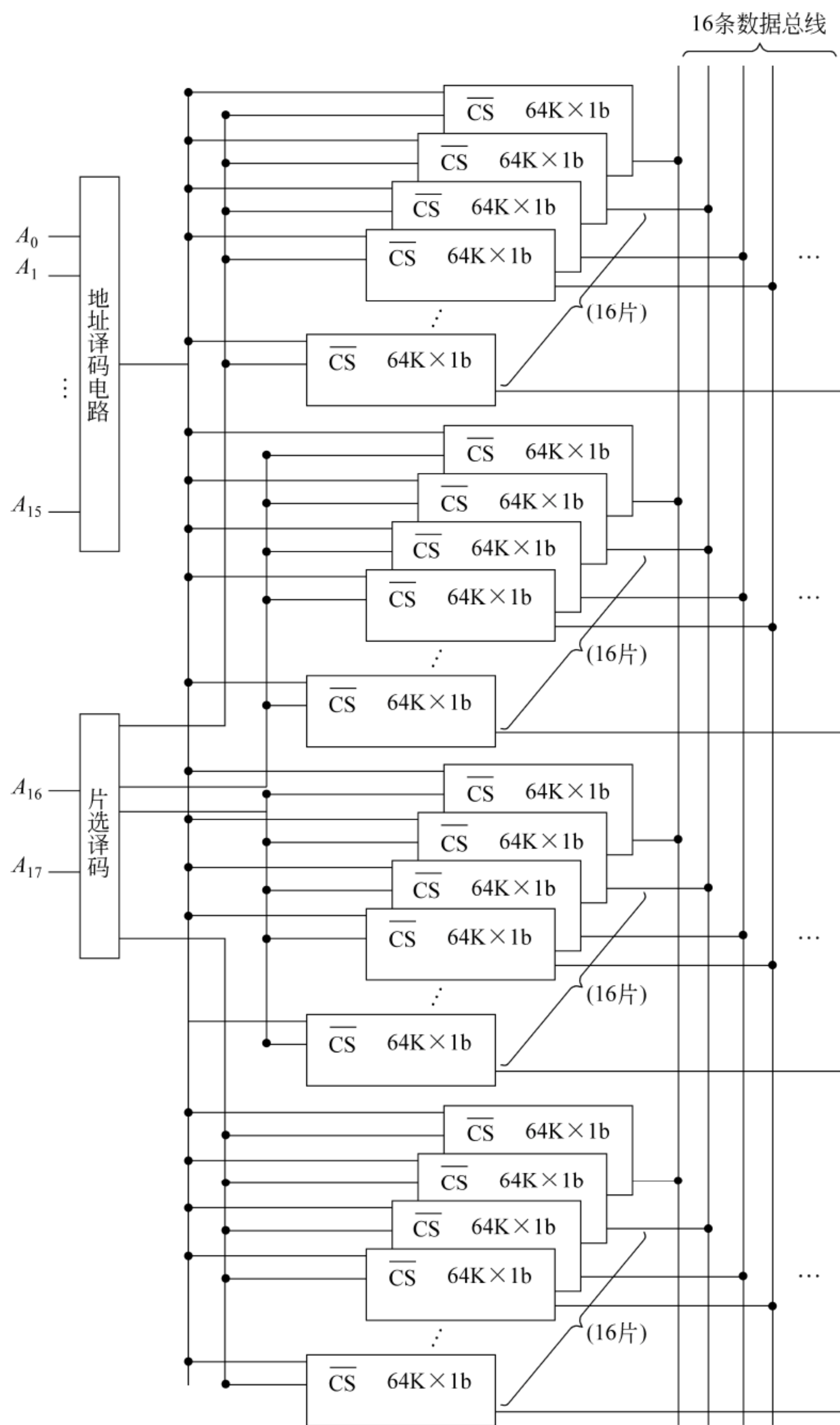
图 2.12 256K×16b 的存储器的组织结构图
