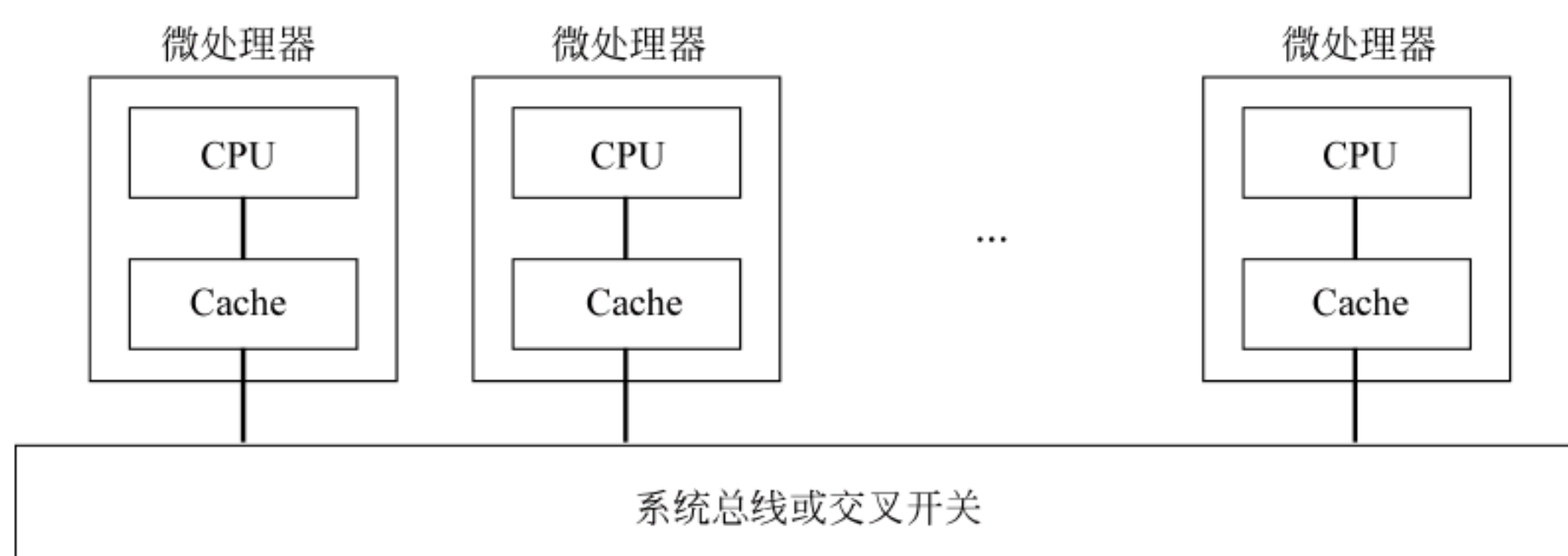
图 1.16 SMP 结构
