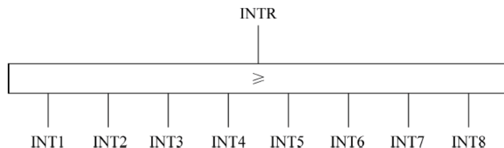
图 4.4 中断源排队判优
