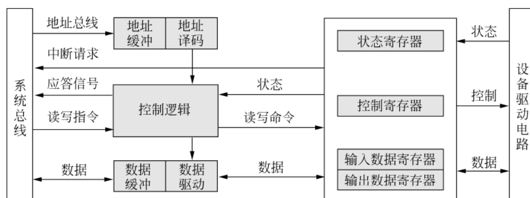
图 4.2 I/O 接口逻辑结构
