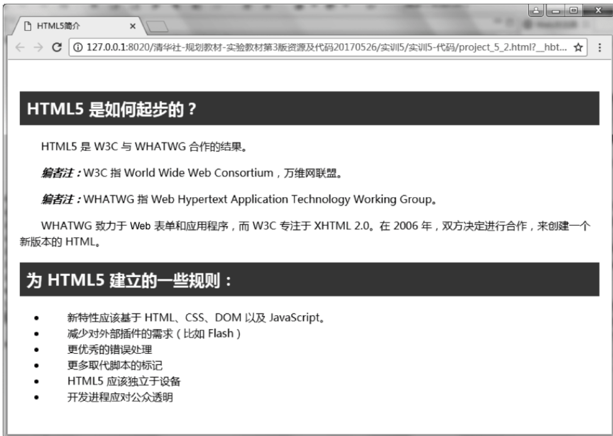
图 1-5-10 HTML5 简介
