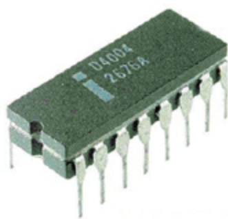
图 7.21 Intel 4004
