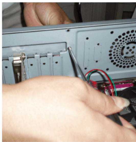
图 2.49 固定扩展卡的保护盖
