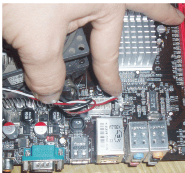
图 2.15 连接散热器风扇的电源
