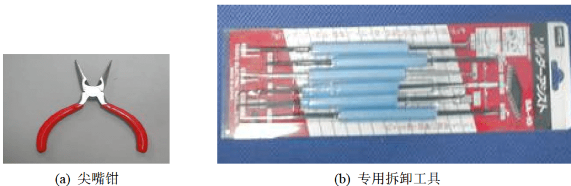
图 12.51 笔记本电脑维修专用工具
