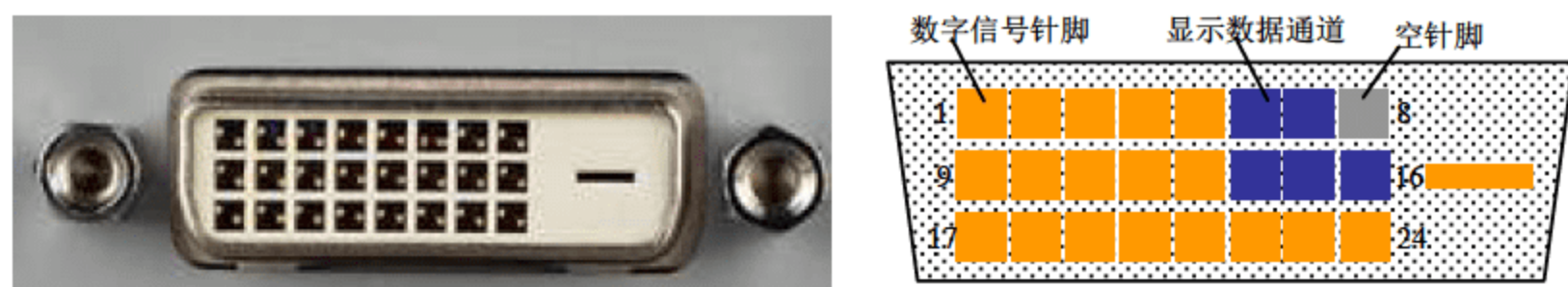
图 9.10 DVI-D 接口
