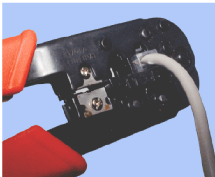
图 10.41 用压线器压制网线接头
