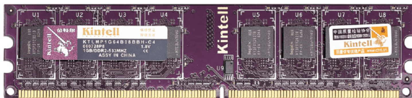
图 8.4 DDR2 内存
