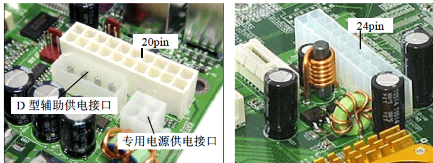
图 7.17 电源插座
