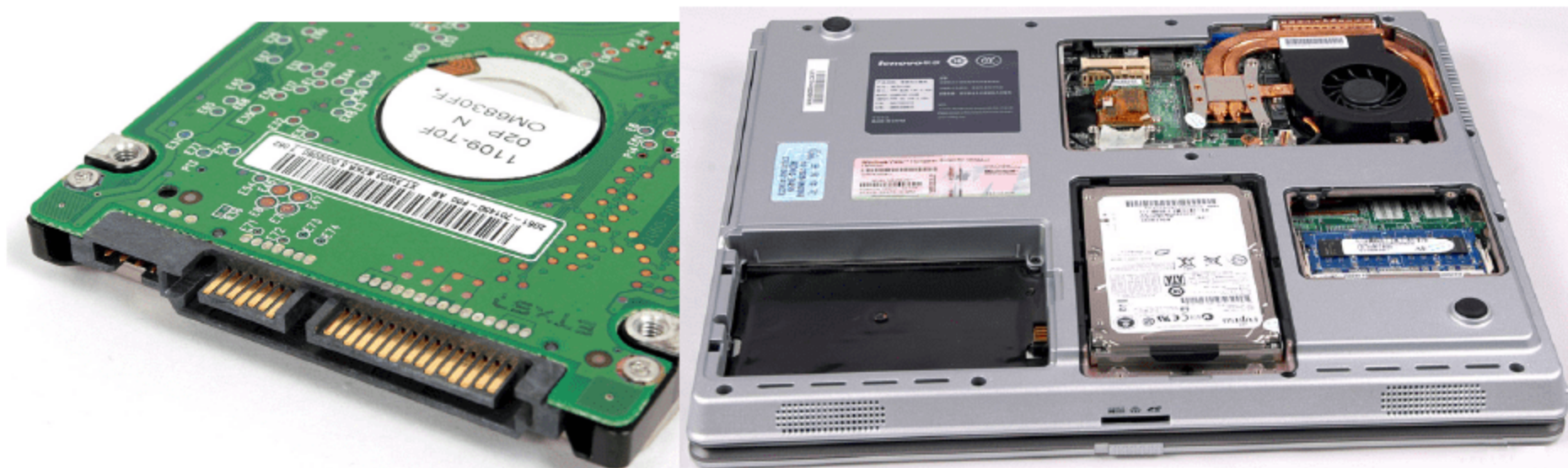
图 12.48 笔记本电脑硬盘
