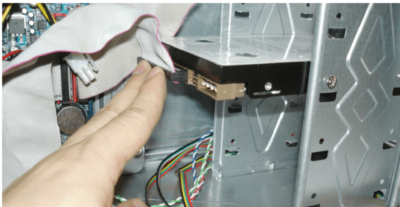
图 2.58 连接硬盘数据线
