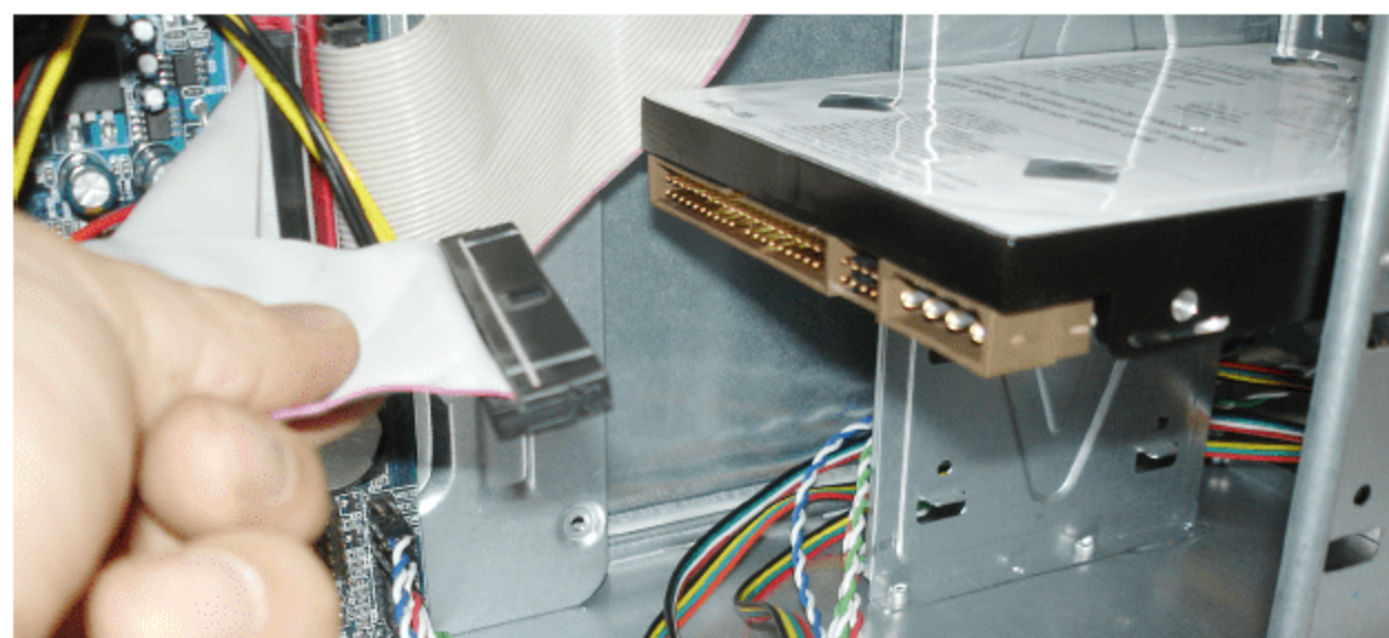
图 2.57 准备把数据线的另一端插入硬盘的 IDE 接口中
