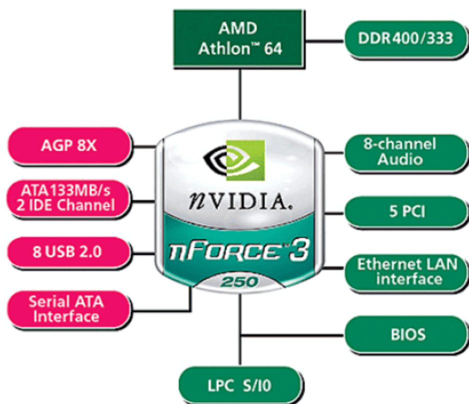
图 7.11 单芯片设计
