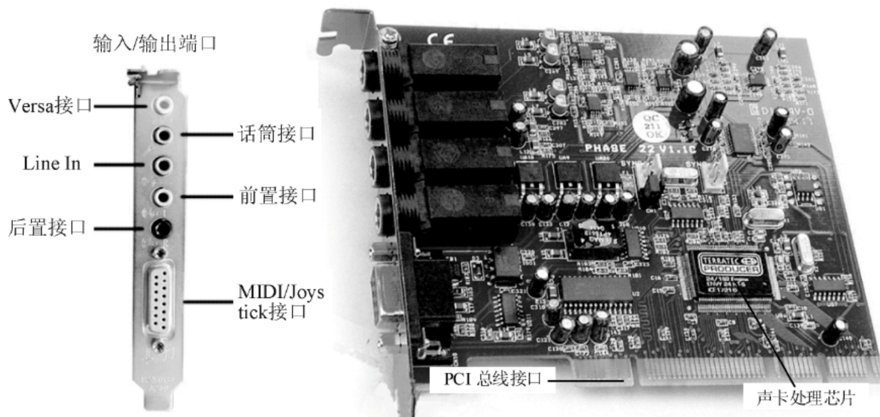
图 10.14 声卡
