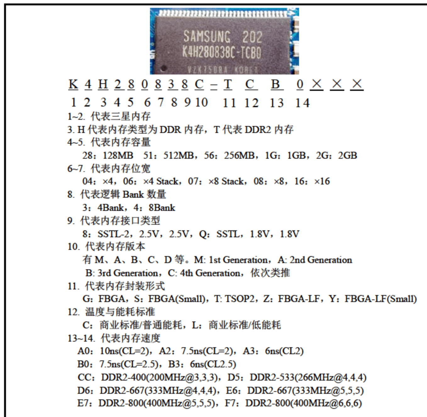
图 8.7 三星内存颗粒的编号表示的意义
