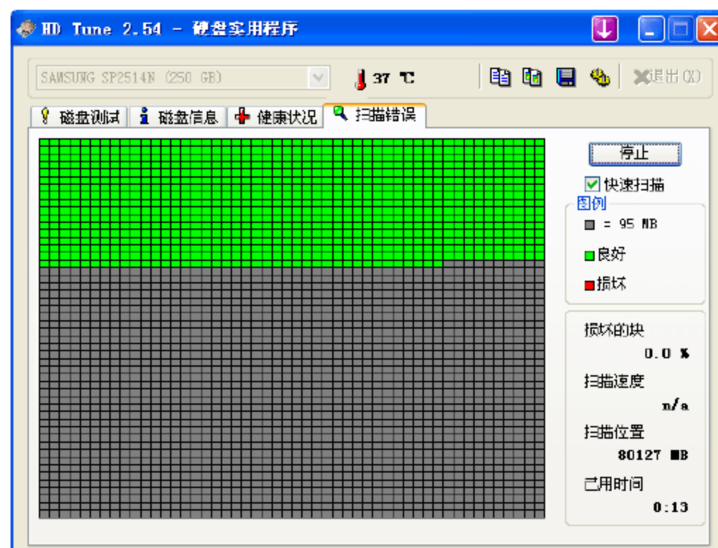
图 8.20 扫描错误
