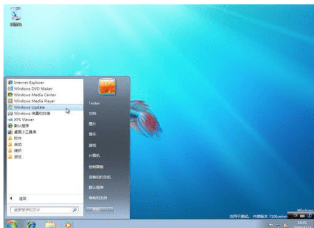
图 5.45 Windows 7 界面
