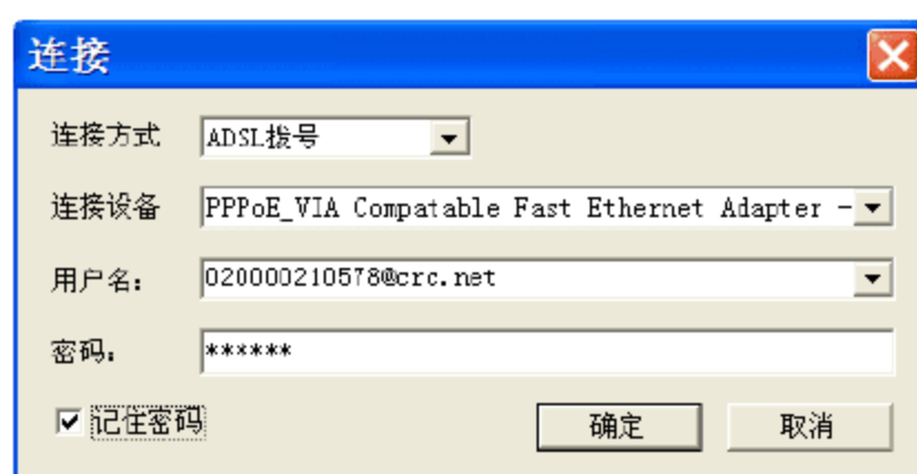
图 11.14 【连接】对话框
