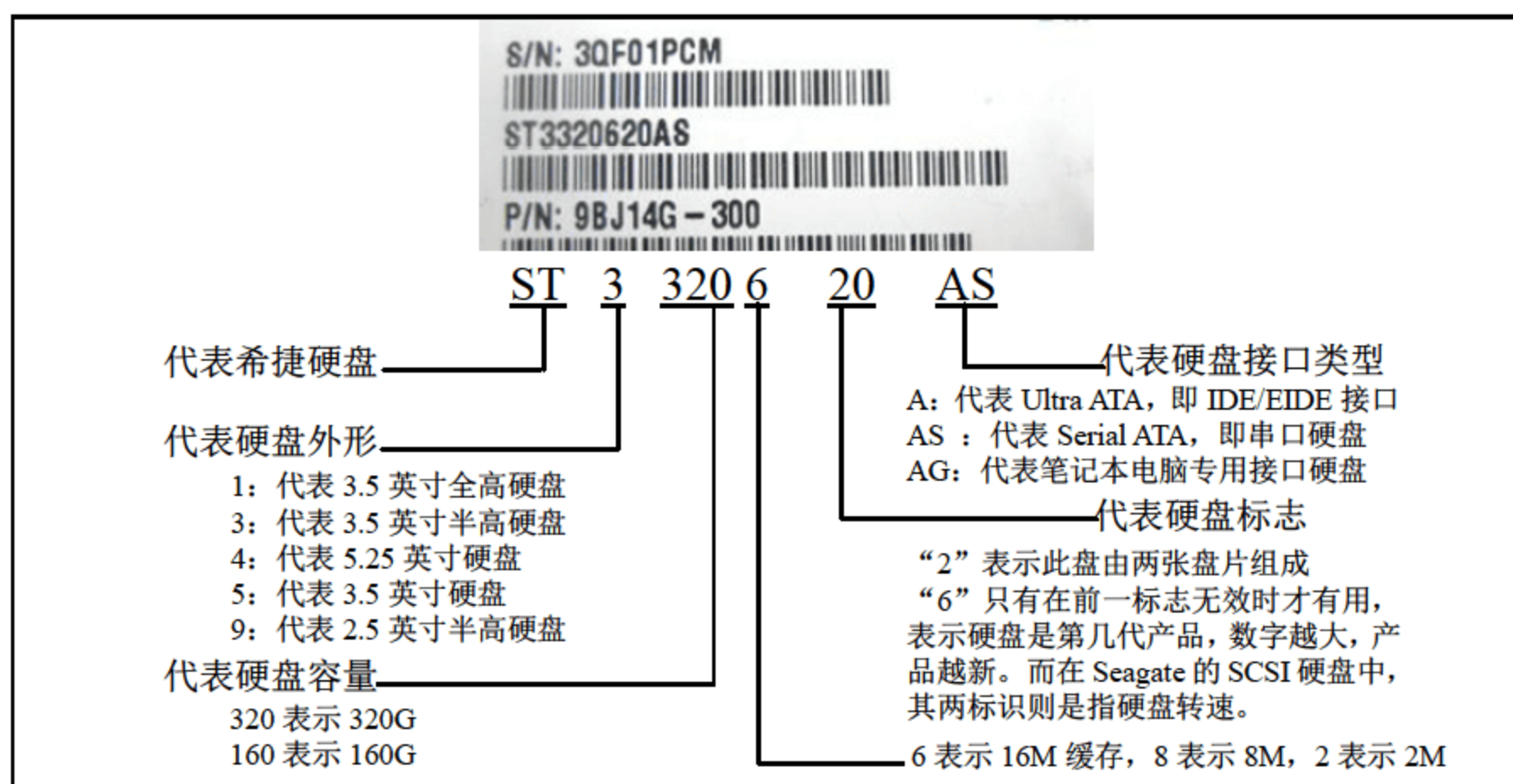
图 8.16 希捷硬盘编号表示意义
