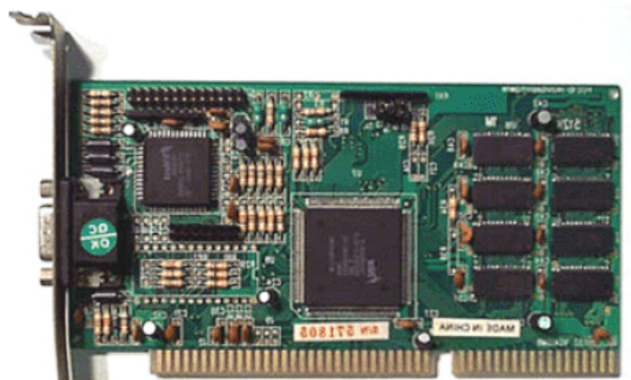
图 9.2 ISA 总线显卡
