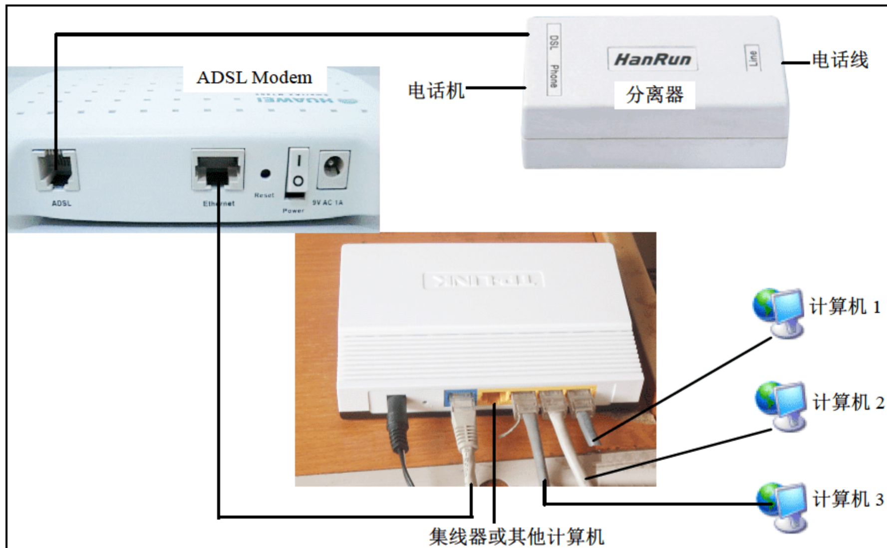
图 11.45 ADSL Modem、宽带路由器和计算机的连接
