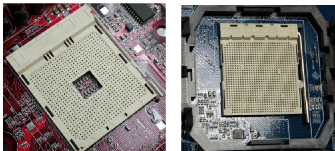
图 7.3 Socket 754 和 Socket AM2 插槽的外观
