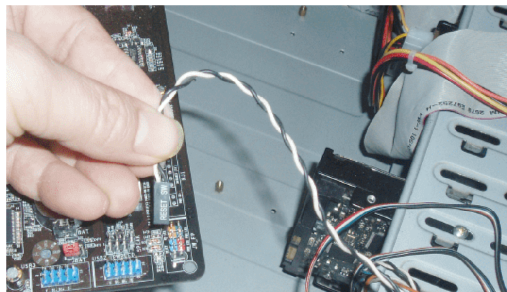
图 2.38 找出 Reset SW 连接线
