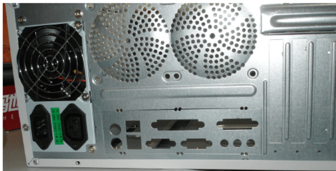
图 2.31 清理好输入/输出孔
