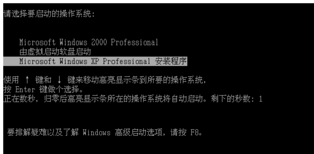
图 5.26 启动菜单
