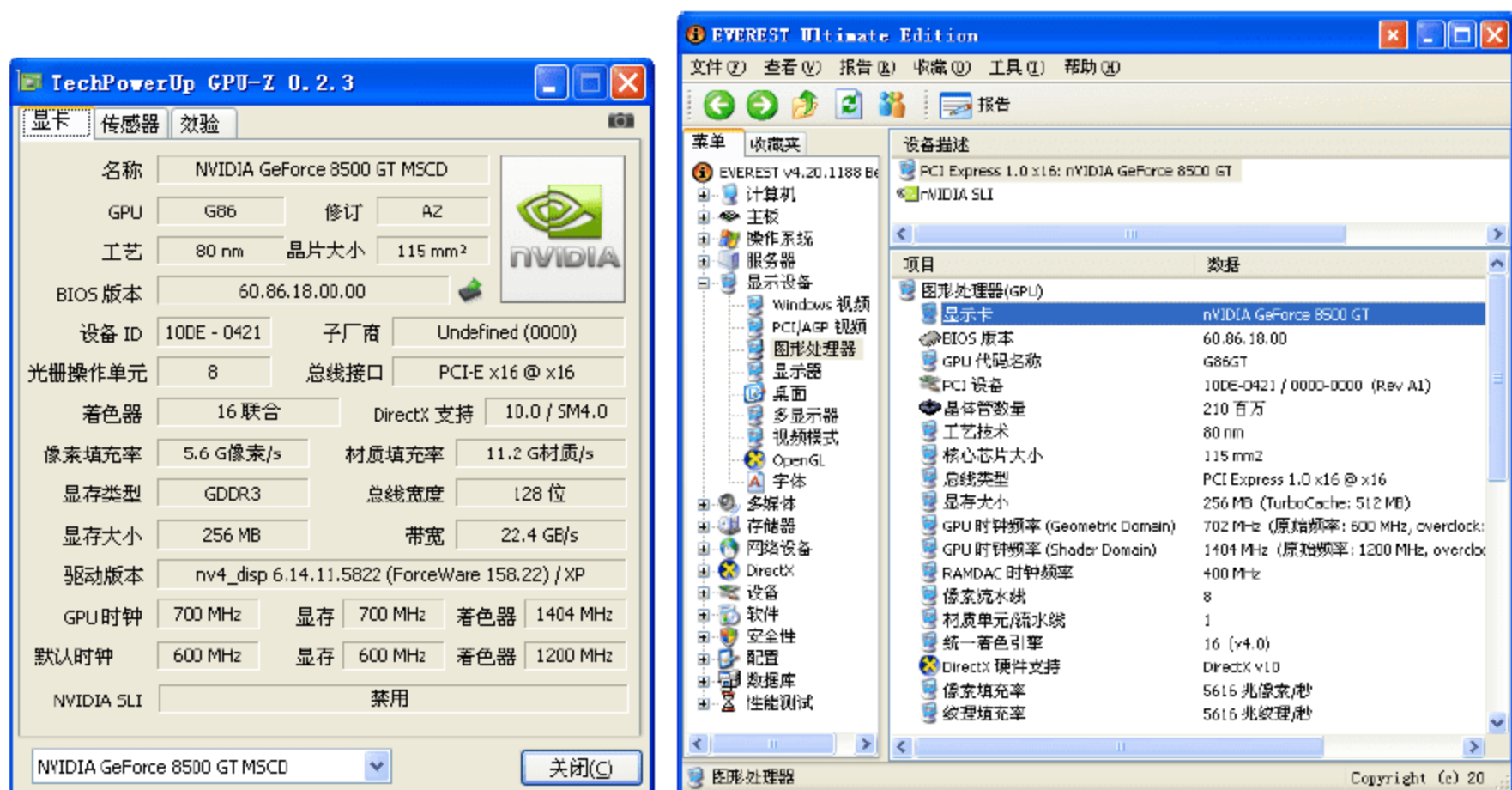
图 9.7 检测显卡
