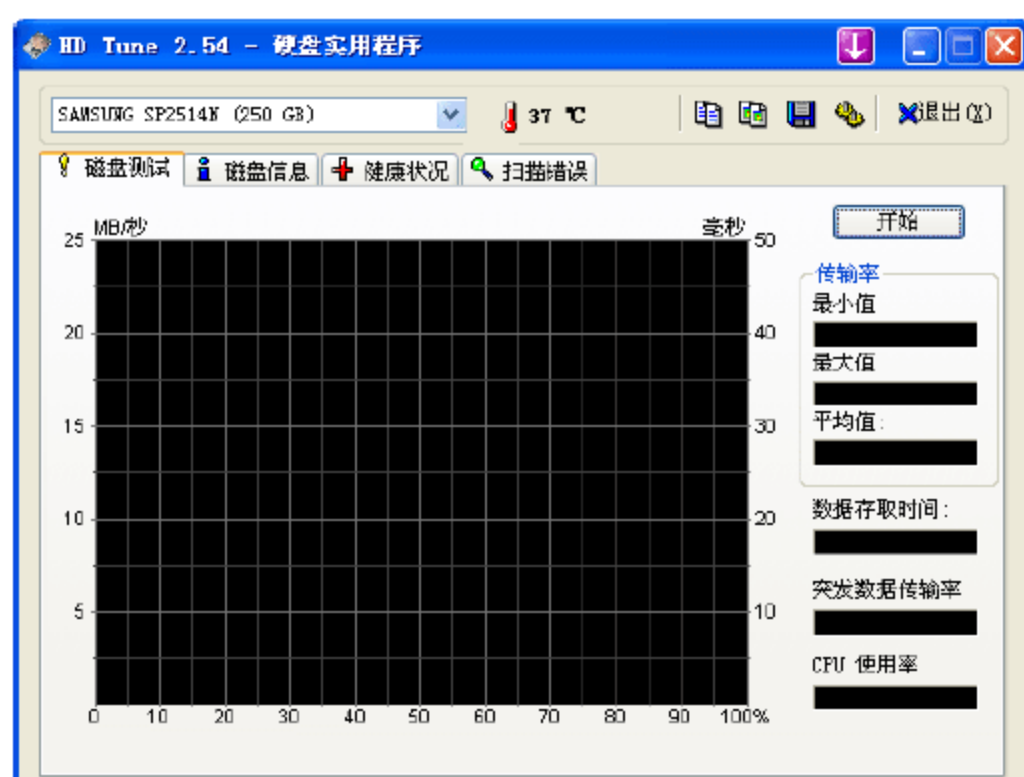
图 8.17 磁盘测试
