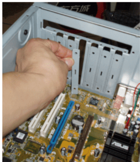
图 2.46 取下机箱后面对应的挡板
