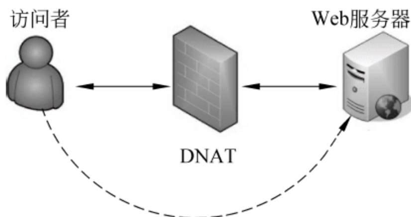
图 13-5 DNAT 原理
