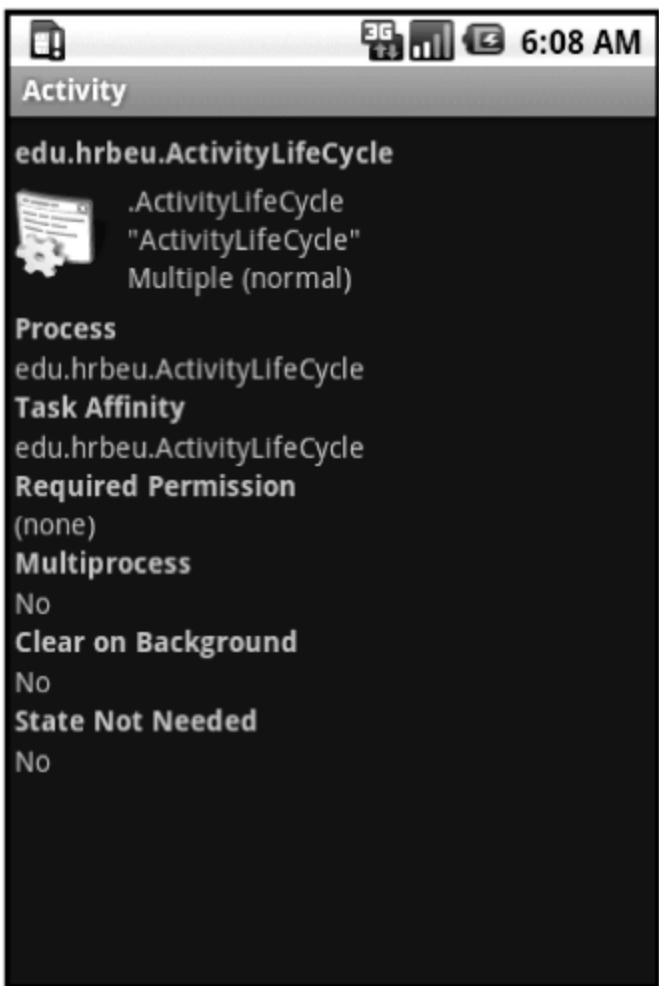
图 4.16 Package Browser
