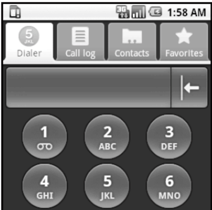
图 5.10 TabHost
