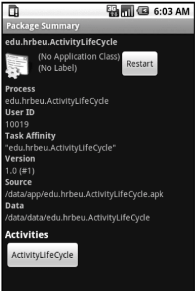
图 4.16 Package Browser
