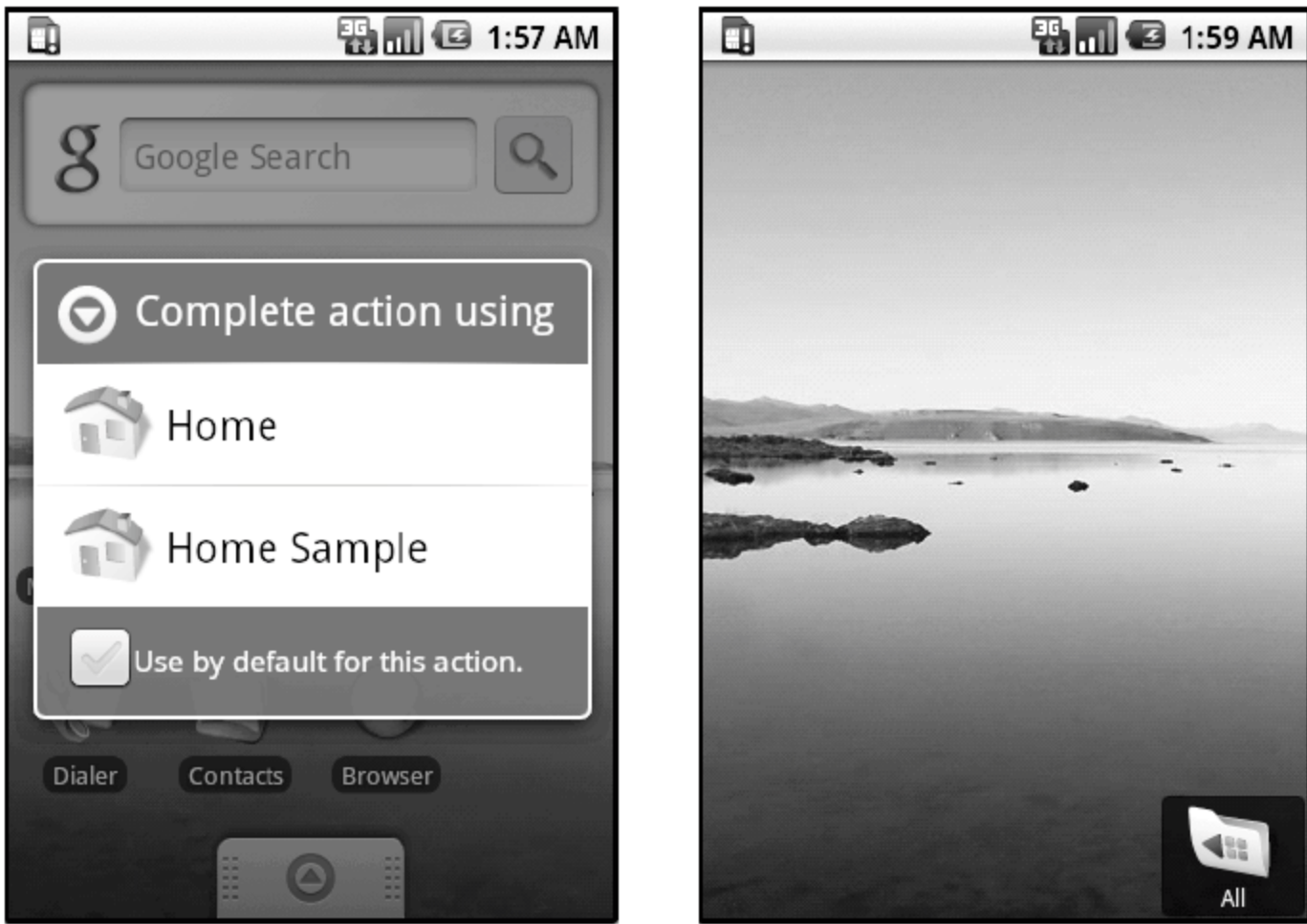
图 2.26 Home 示例
