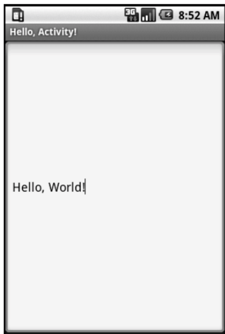
图 2.22 HelloActivity 示例
