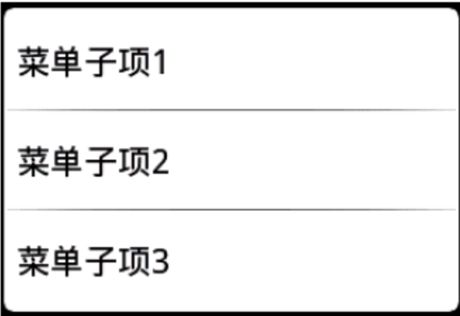
图 5.30 XML 菜单
