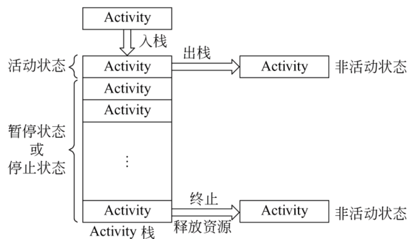
图 4.3 Activity 栈
