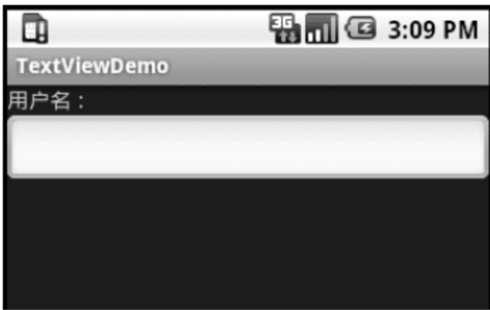
图 5.3 TextView 和 EditText
