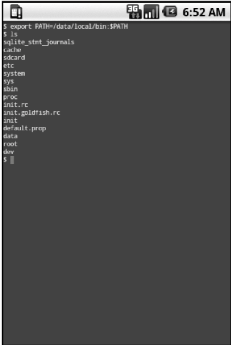
图 4.19 Terminal Emulator
