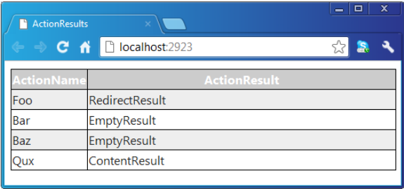
图 8-1 执行具有不同返回值的 Action 方法得到的 ActionResult 类型
