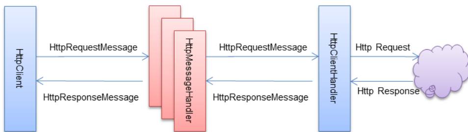
图 9-17 通过 HttpClient 构建的客户端管道
