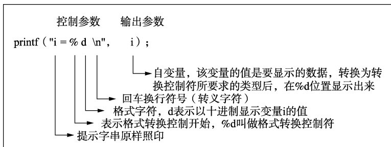
图 4-1 printf() 函数的参数说明
