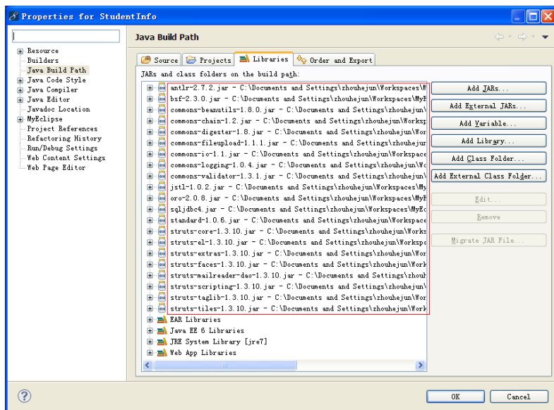
图 8.12 添加 Struts 1 的 jar 包
