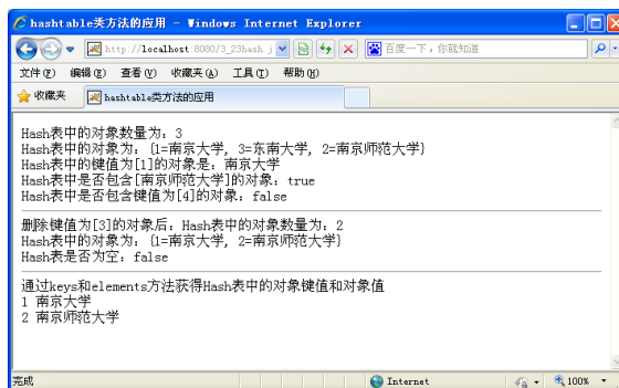
图 3.23 Hashtable 类方法的应用
