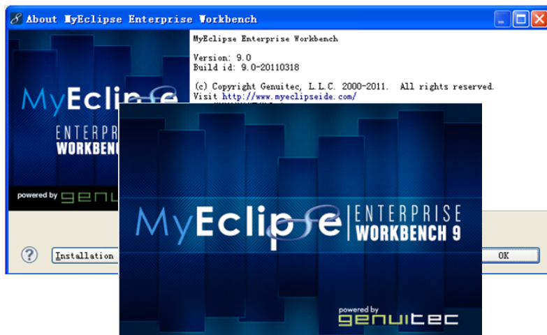
图 2.11 MyEclipse 9.0
