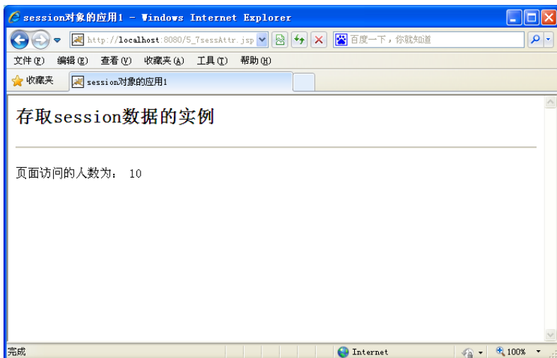
图 5.14 第 10 次被访问
