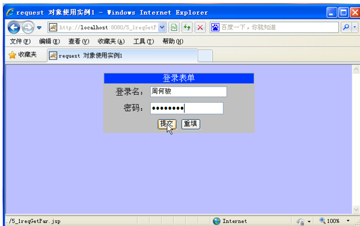
图 5.3 登录表单
