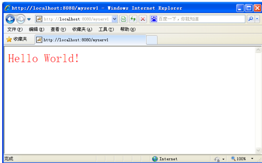
图 2.19 【例 2.1】运行界面
