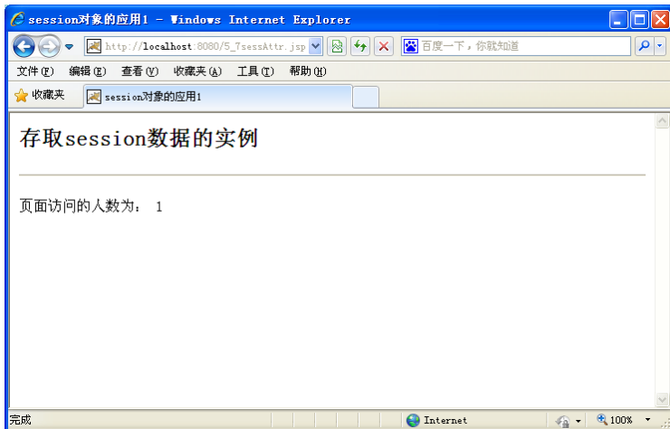
图 5.13 第 1 次运行
