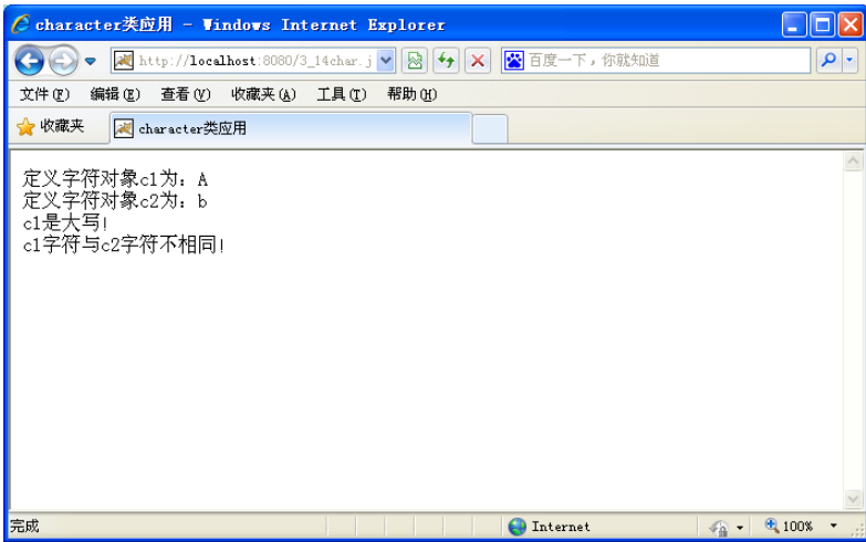
图 3.14 Character 类应用
