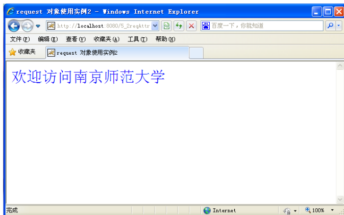
图 5.5 获取属性
